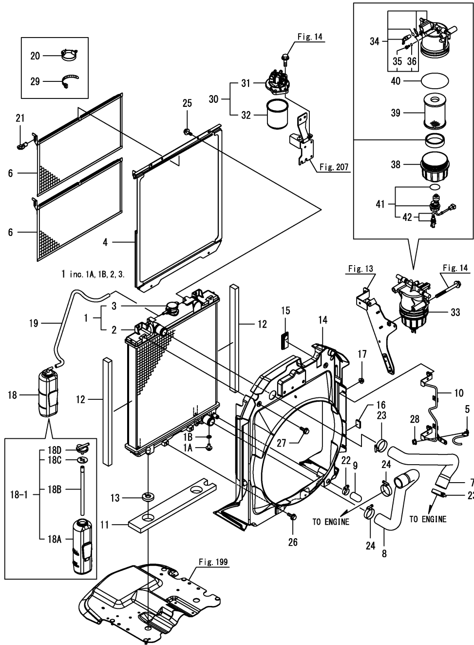
Fig.4. 라디에이터(캐빈)
