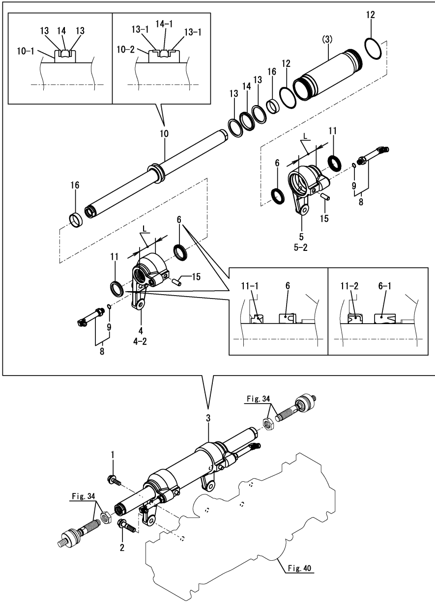
Fig.60. P.S.T.실린더
