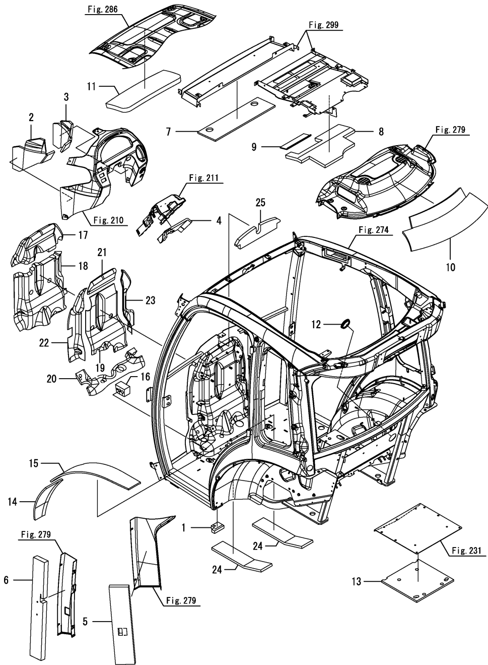
Fig.284. 캐빈시일(4)
