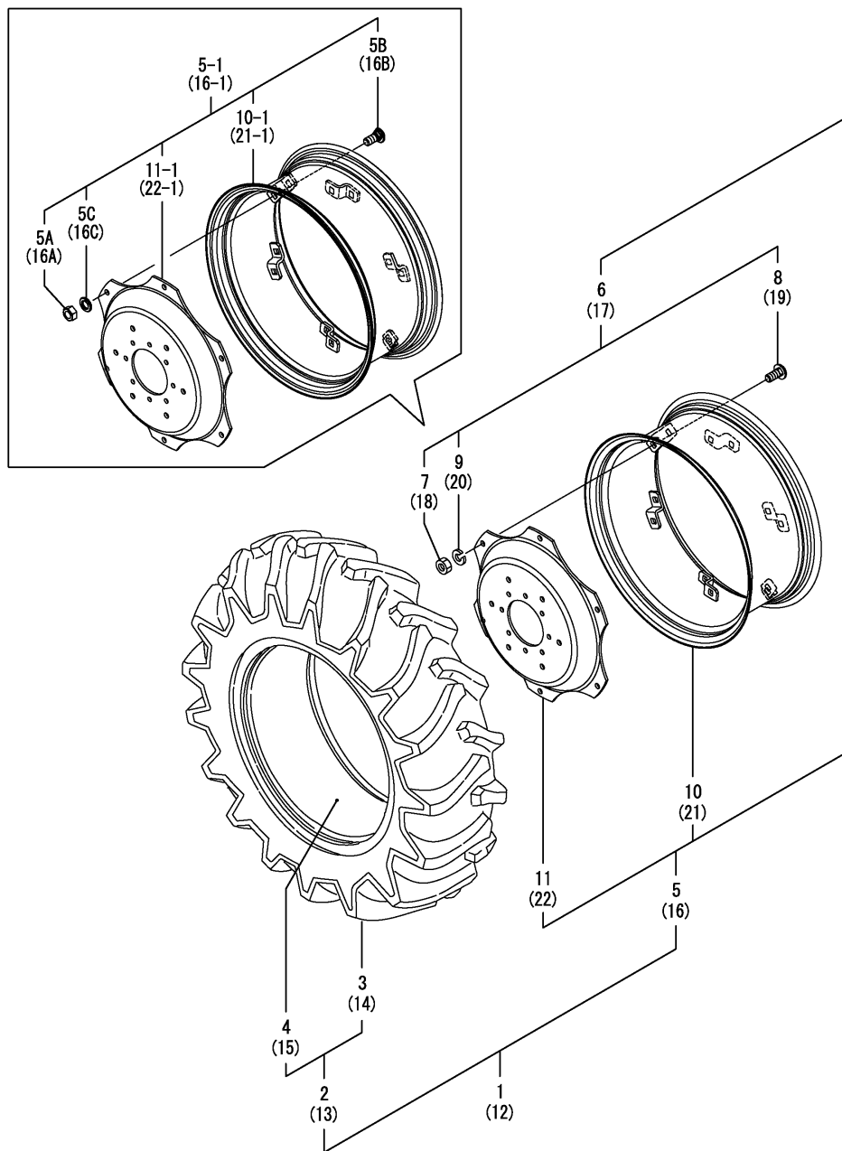
Fig.112. 후륜 타이어(13.6-26H)
