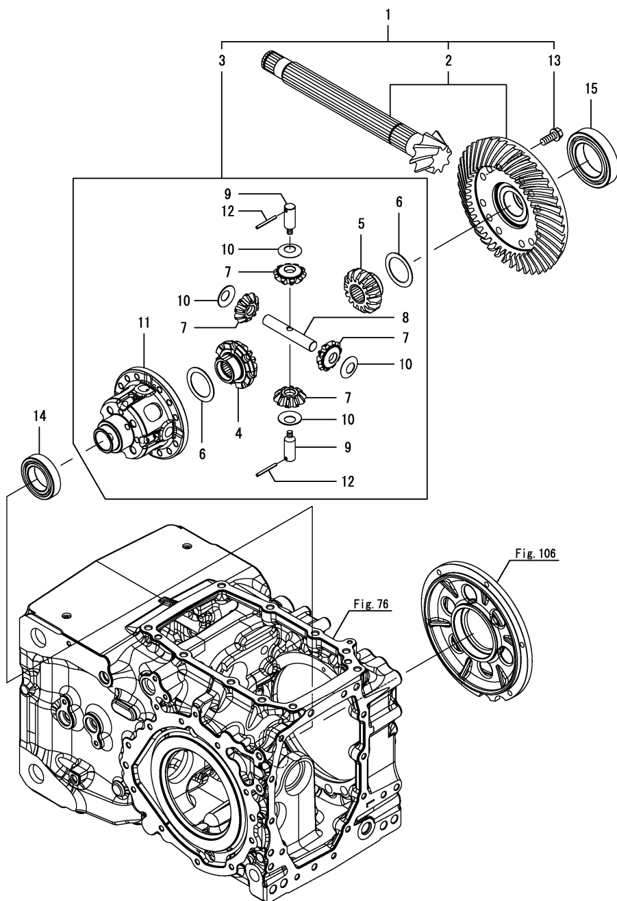
Fig.105. 차동기어
