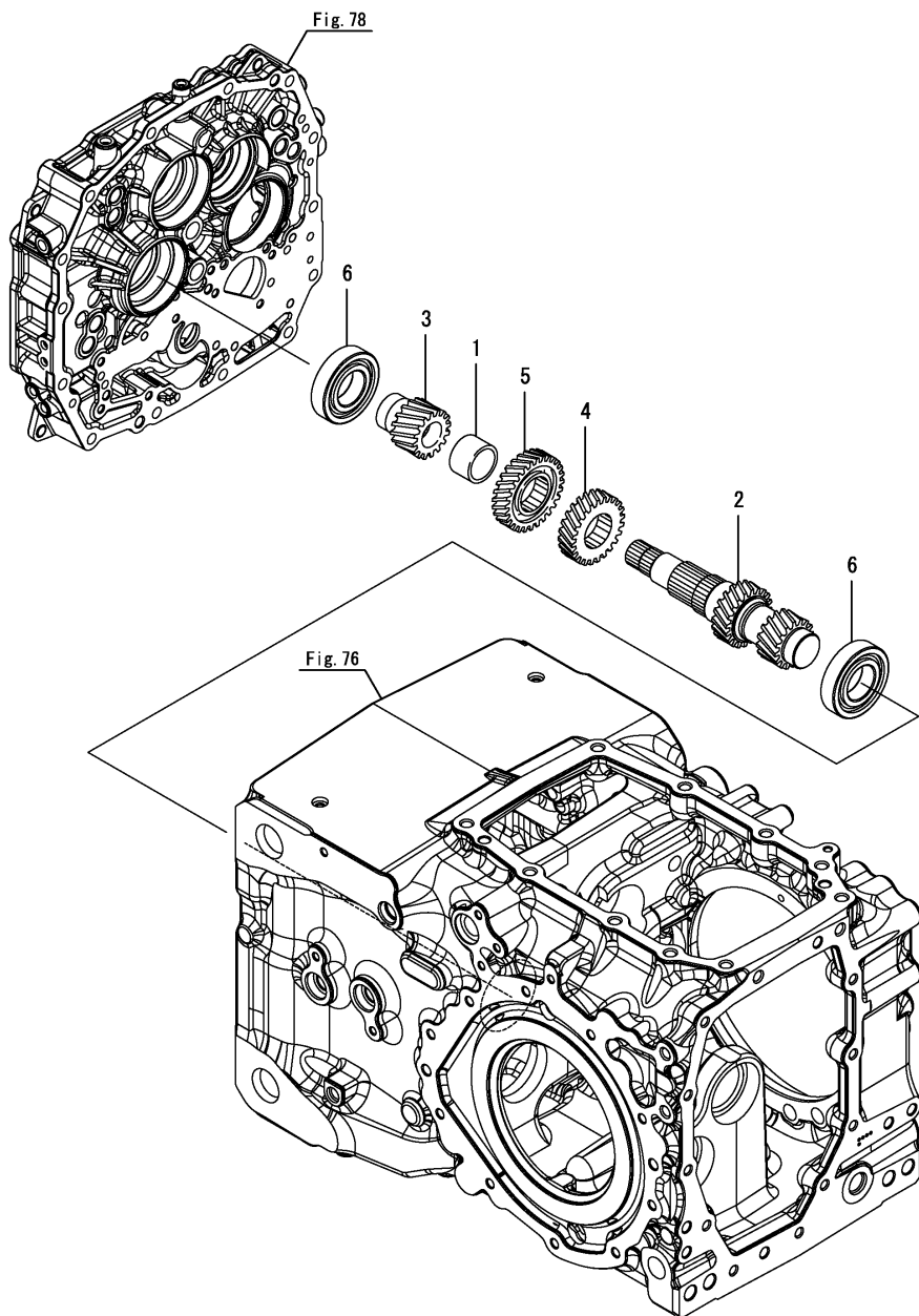
Fig.88. P.T.O. 구동축
