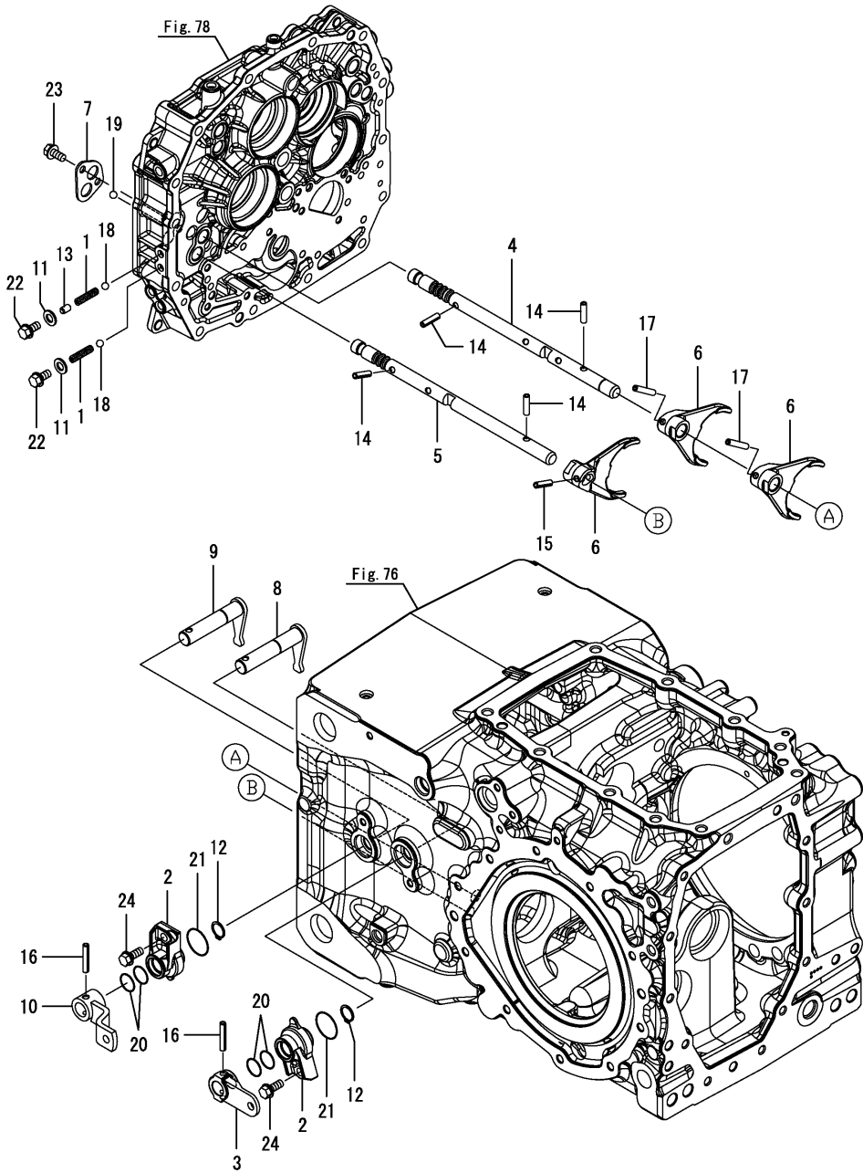
Fig.96. P.T.O. 변속
