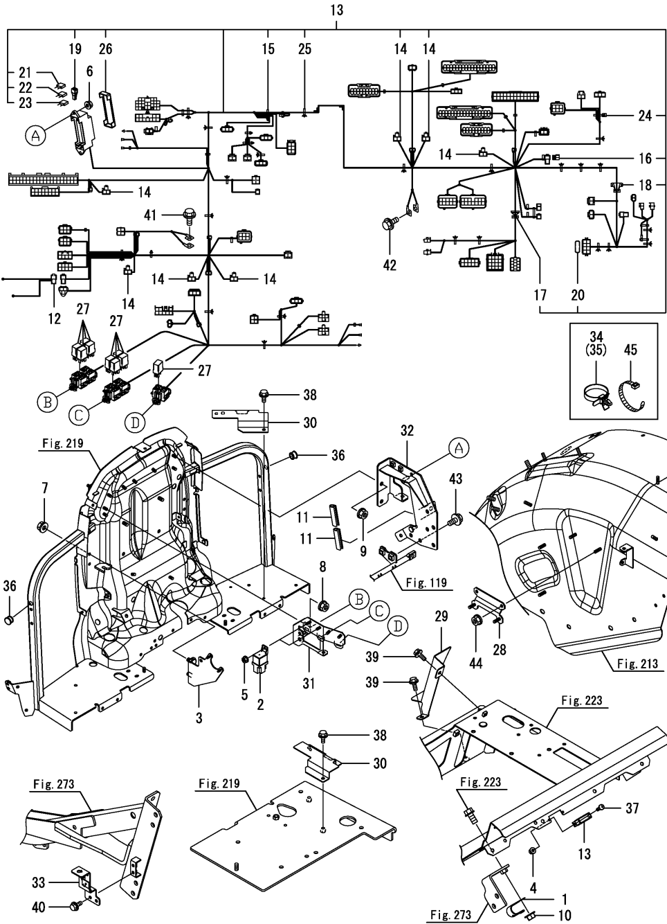
Fig.162. 배선(바닥)
