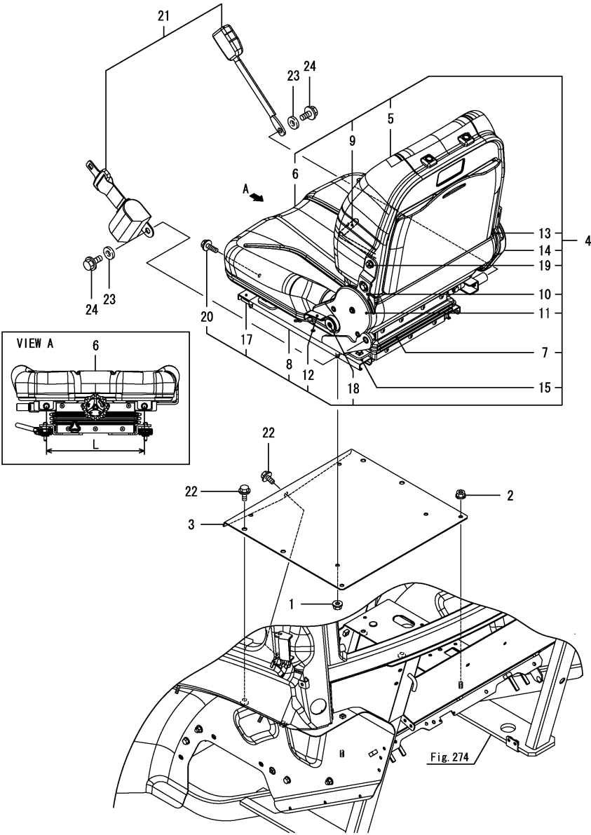
Fig.231. 시트(캐빈)
