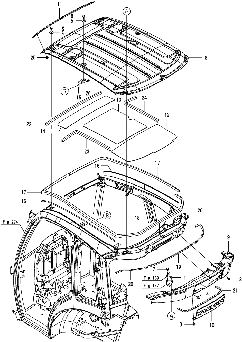
Fig.286. 루프
