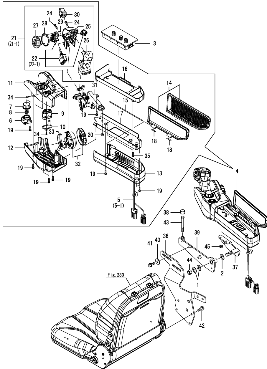
Fig.232. 팔걸이
