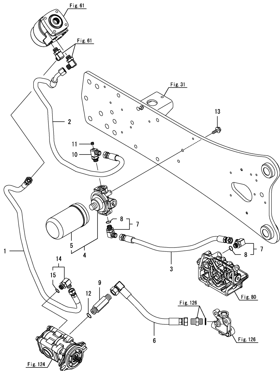
Fig.137. 유압호스
