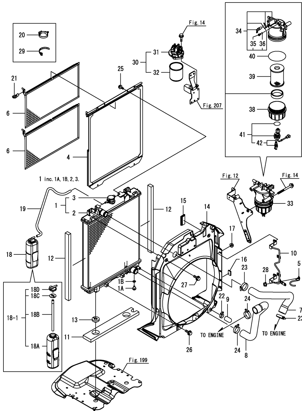
Fig.3. 라디에이터
