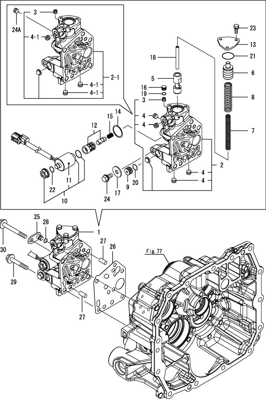
Fig.82. P.T.O. 밸브
