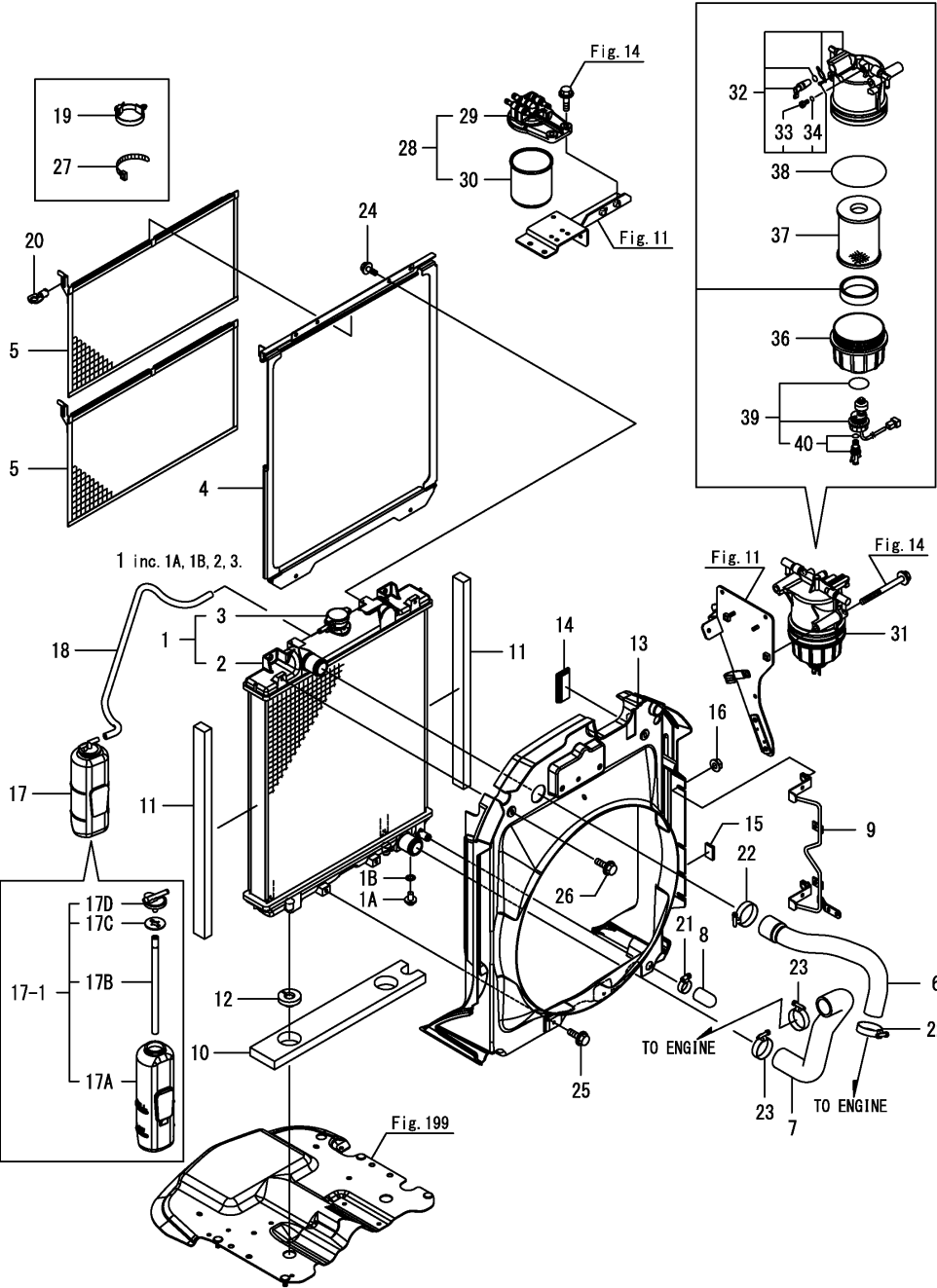
Fig.2. 라디에이터
