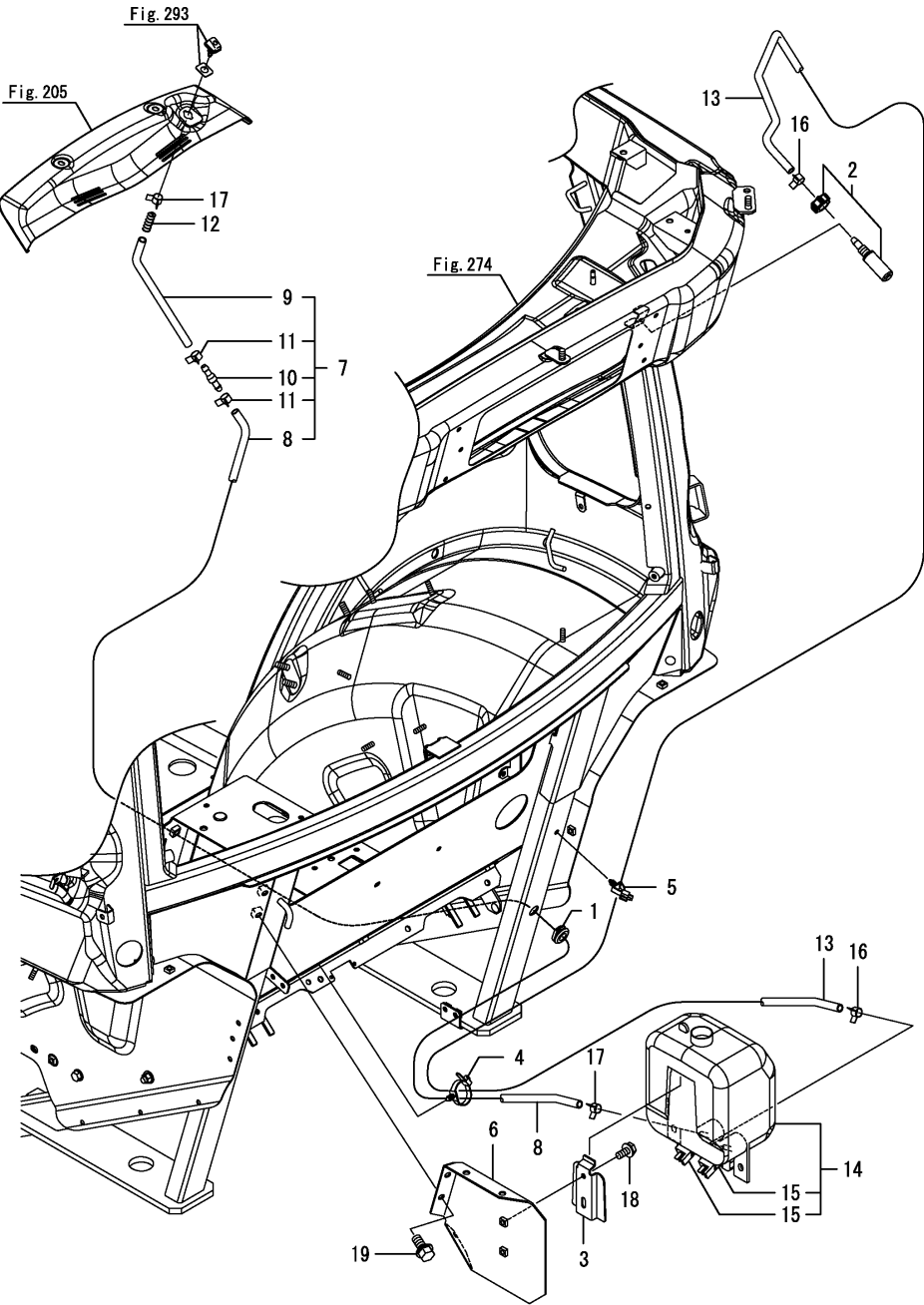
Fig.292. 워셔 탱크(1)
