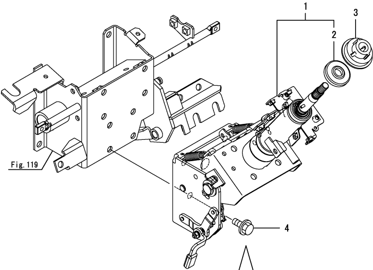
Fig.54. 스티어링칼럼
