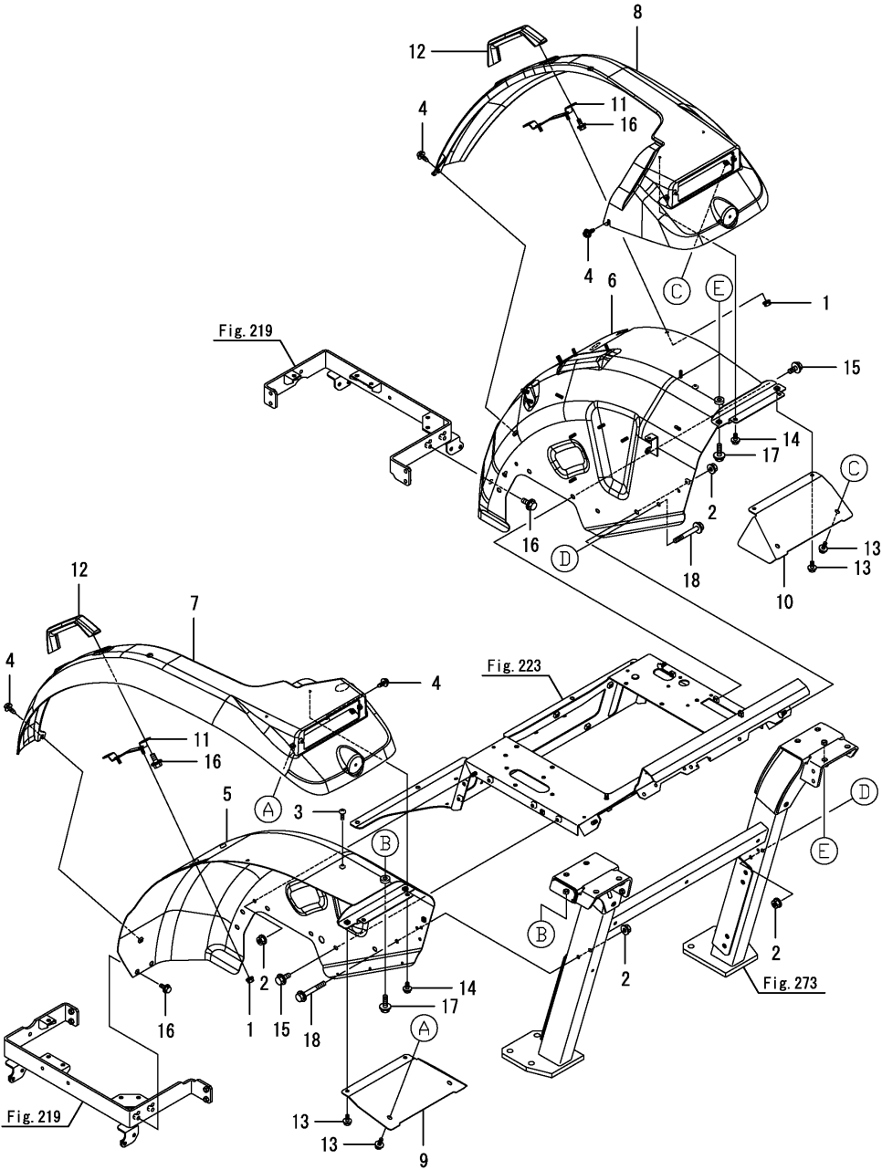
Fig.213. 휠더
