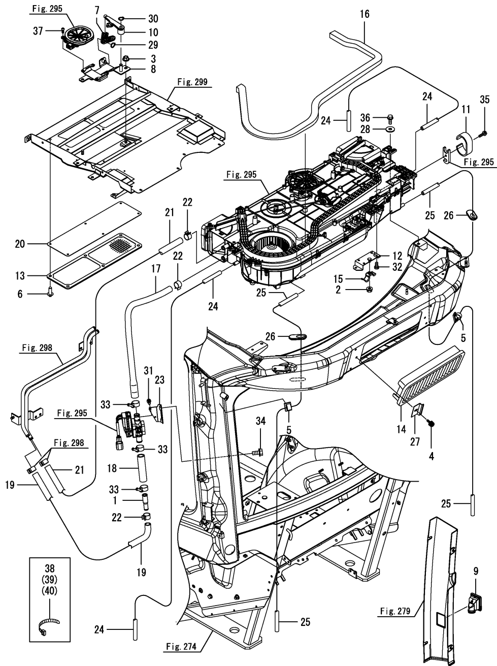
Fig.297. 에어컨(3)
