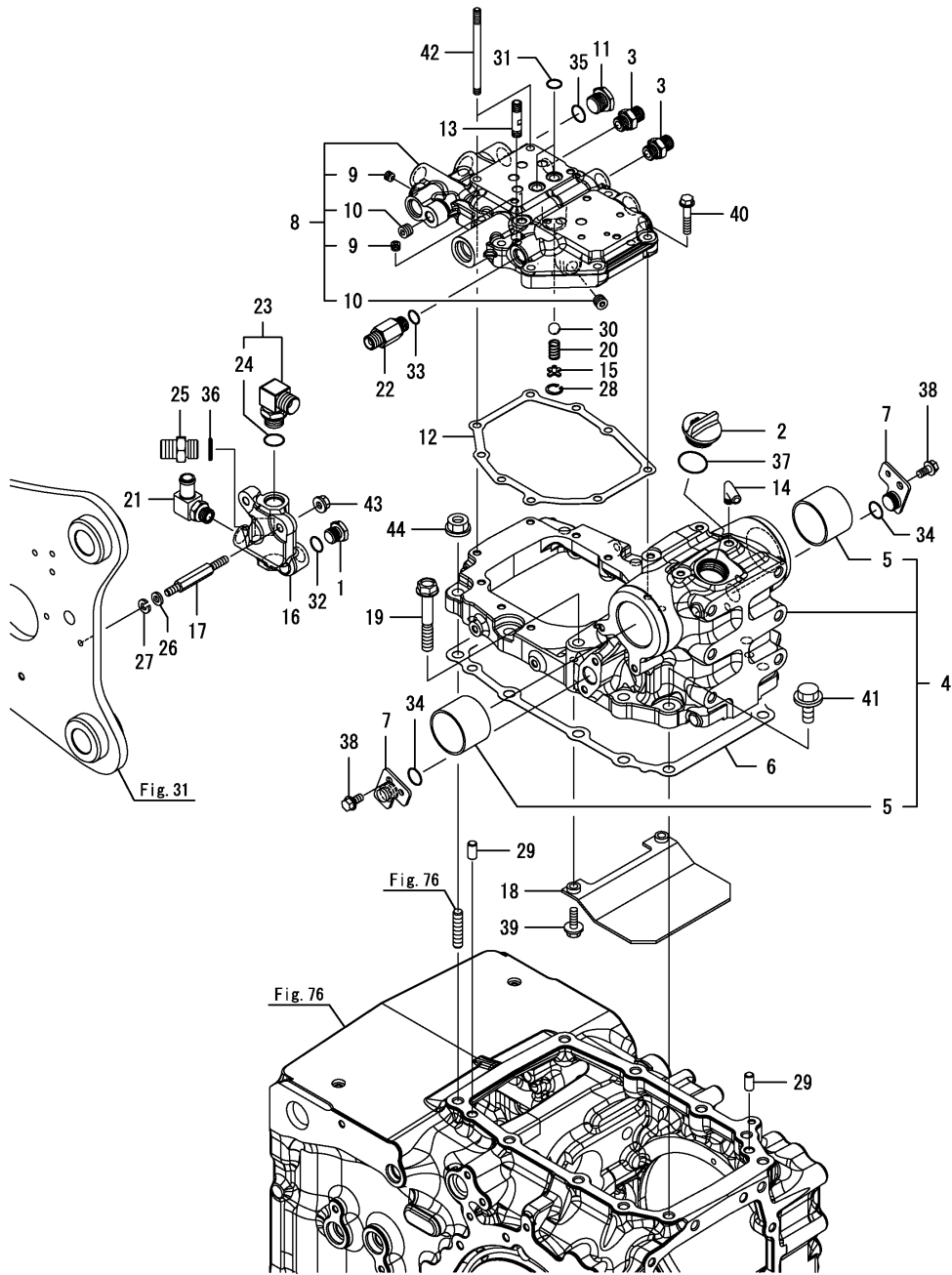
Fig.126. 유압리프트케이스
