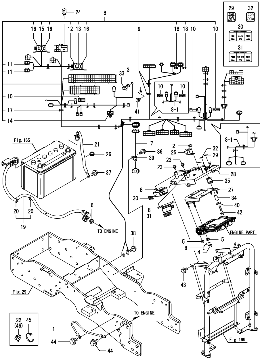
Fig.160. 와이어 하네스(엔진)(캐빈)
