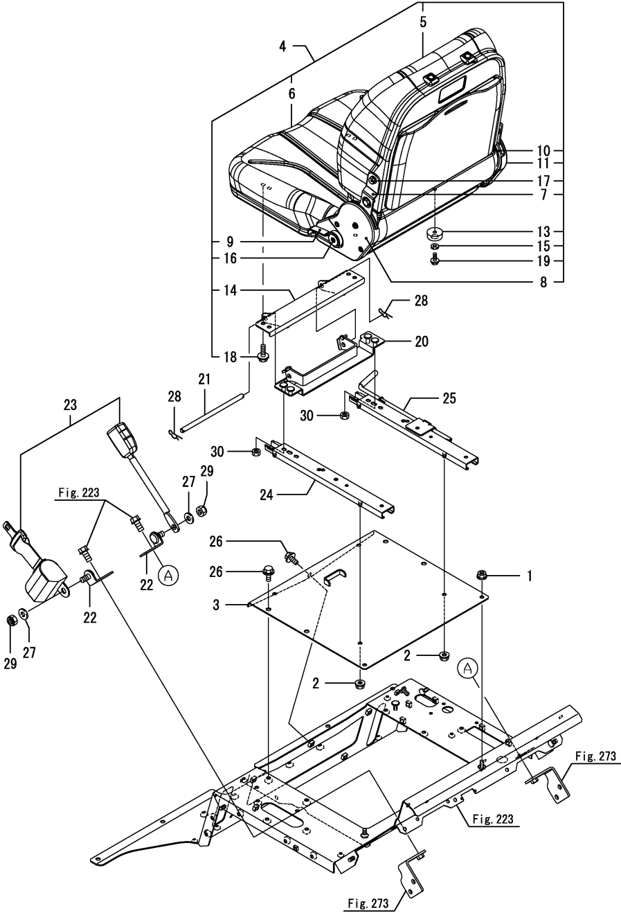
Fig.230. 의자
