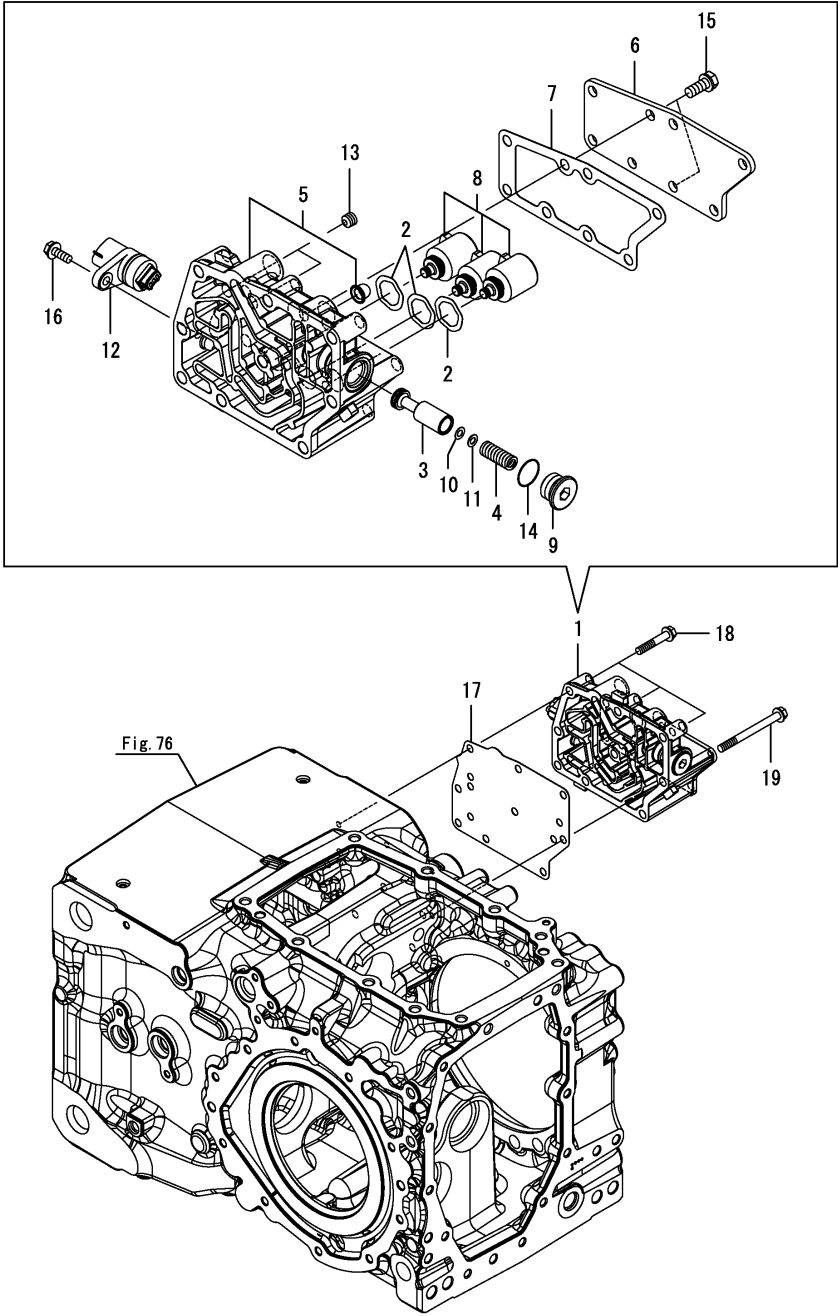
Fig.80. 밸브(I-H.M.T.)
