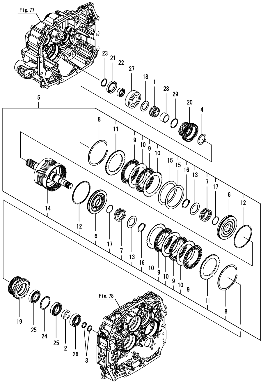
Fig.100. 전륜구동
