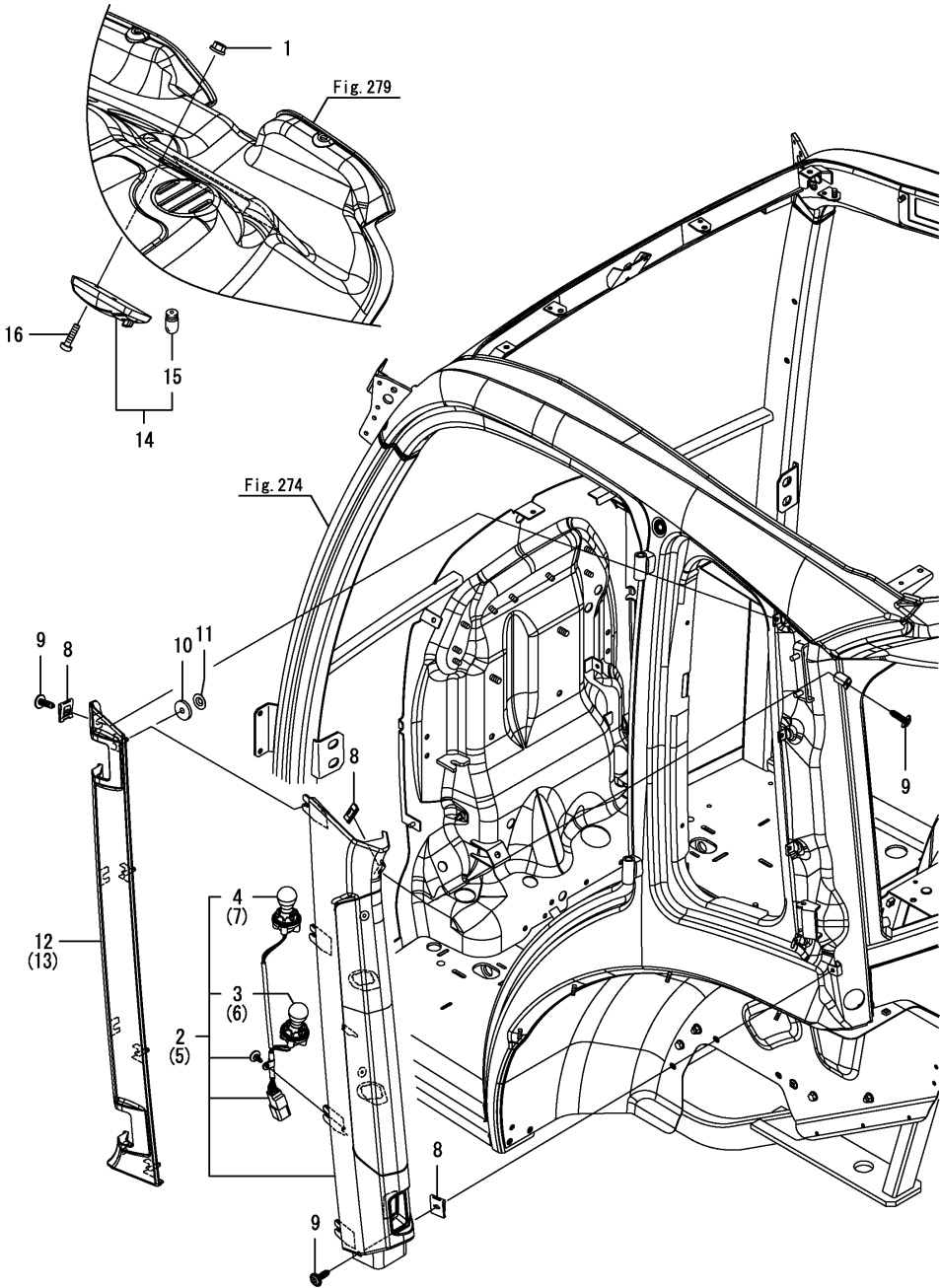
Fig.186. 램프(바닥)(후방)(캐빈)
