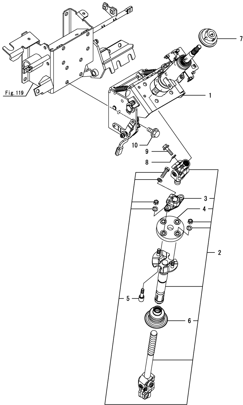
Fig.55. 스티어링칼럼(캐빈)
