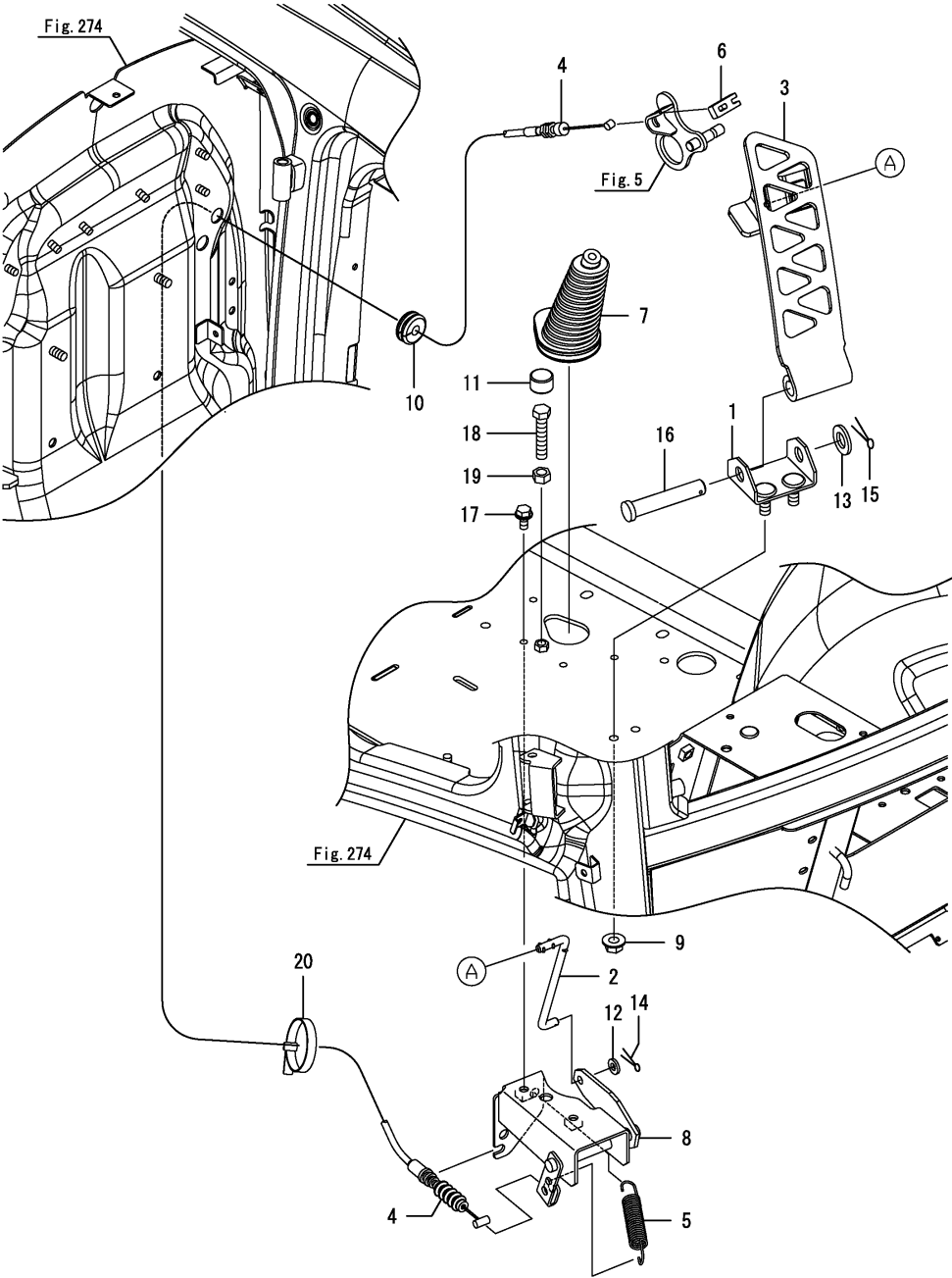
Fig.7. 풋 액셀러레이터(캐빈)
