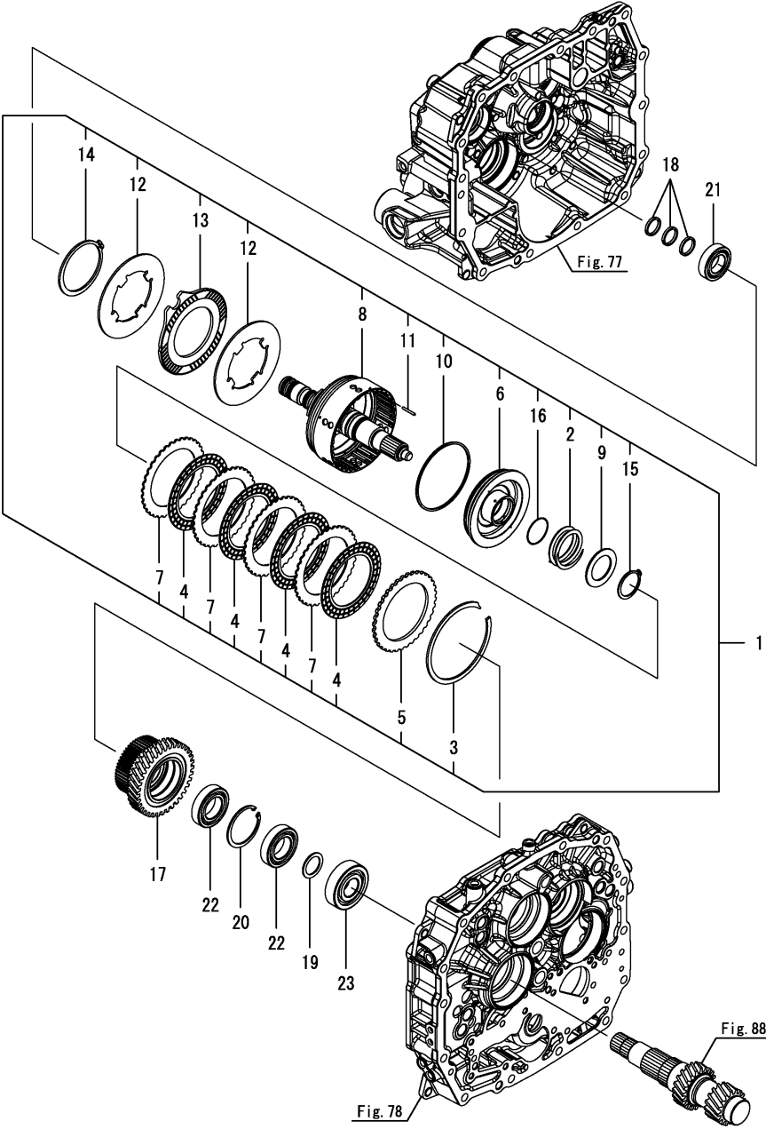
Fig.75. P.T.O. 클러치
