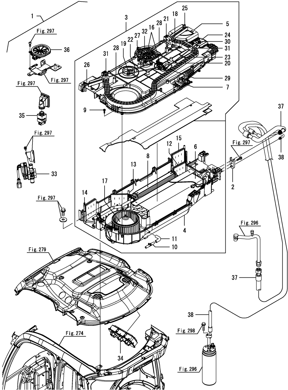
Fig.295. 에어컨(1)
