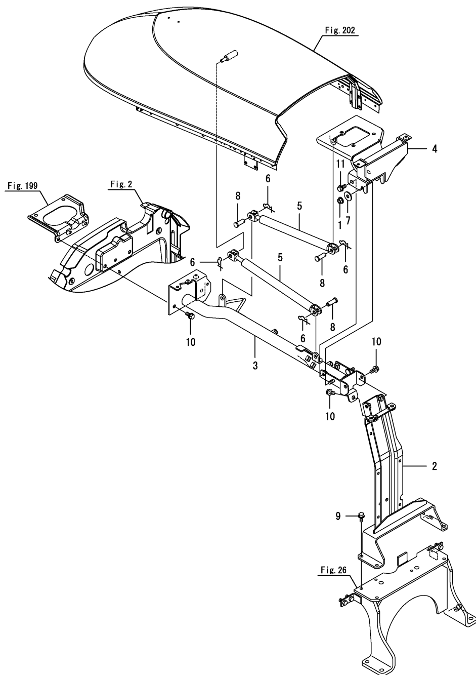
Fig.200. 리어프레임
