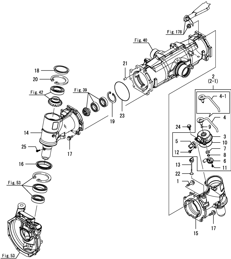
Fig.41. 프론트기어케이스
