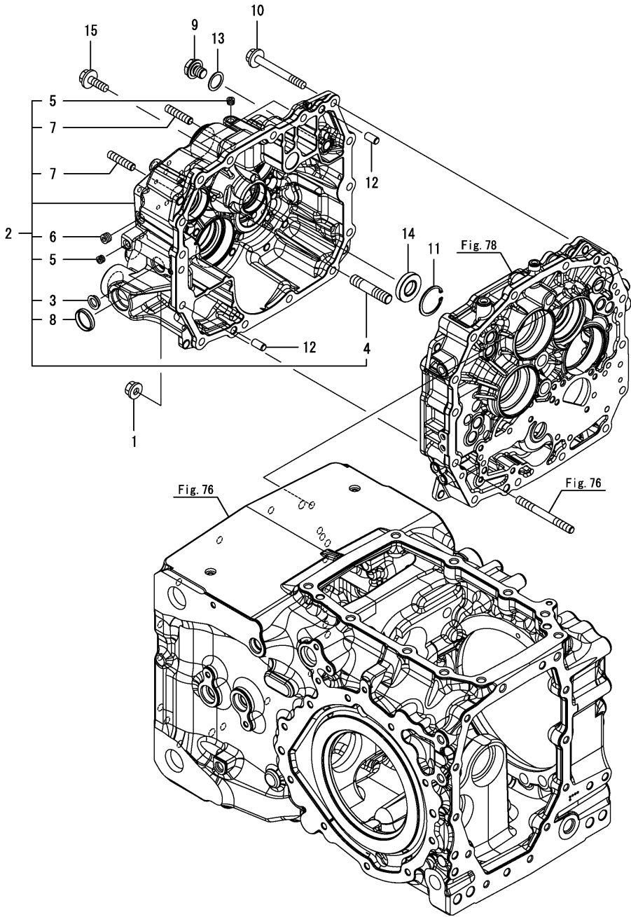
Fig.77. 프론트커버
