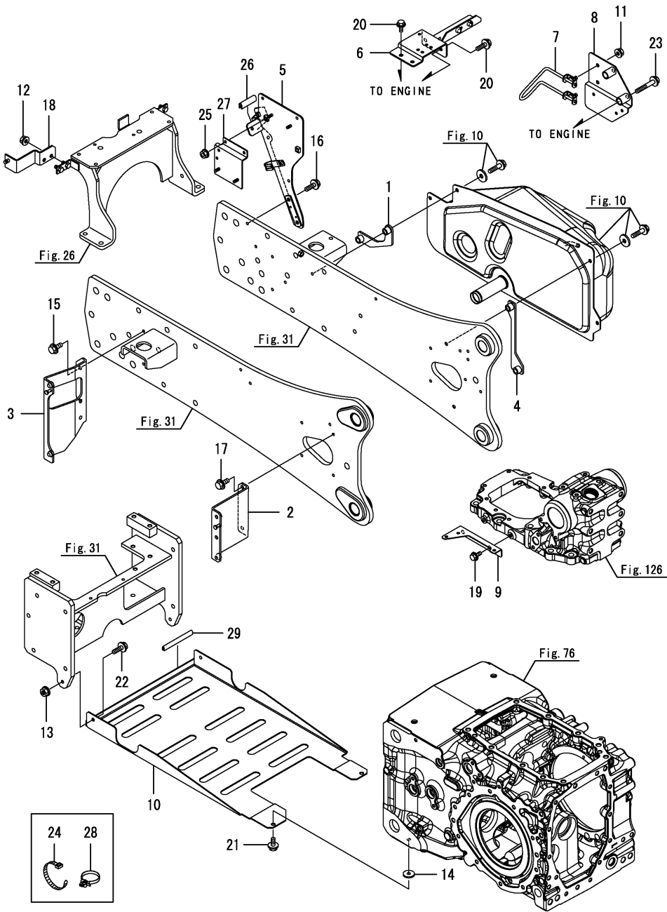
Fig.11. 탱크브라켓
