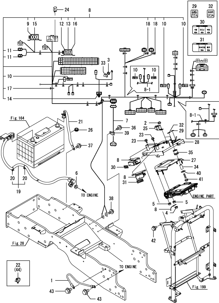
Fig.159. 배선 하네스(엔진)
