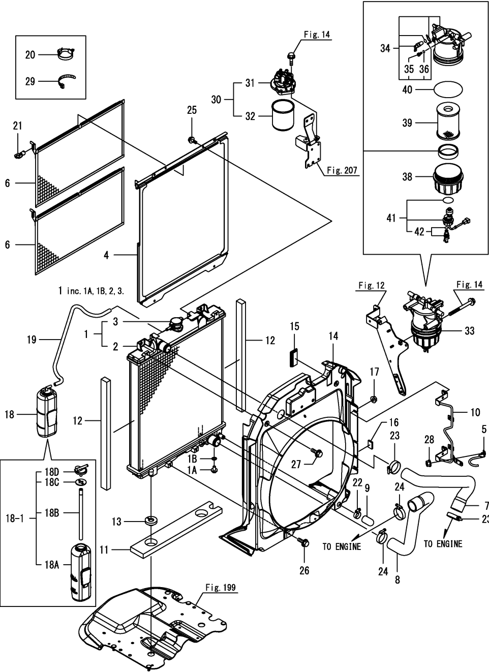
Fig.3. 라디에이터
