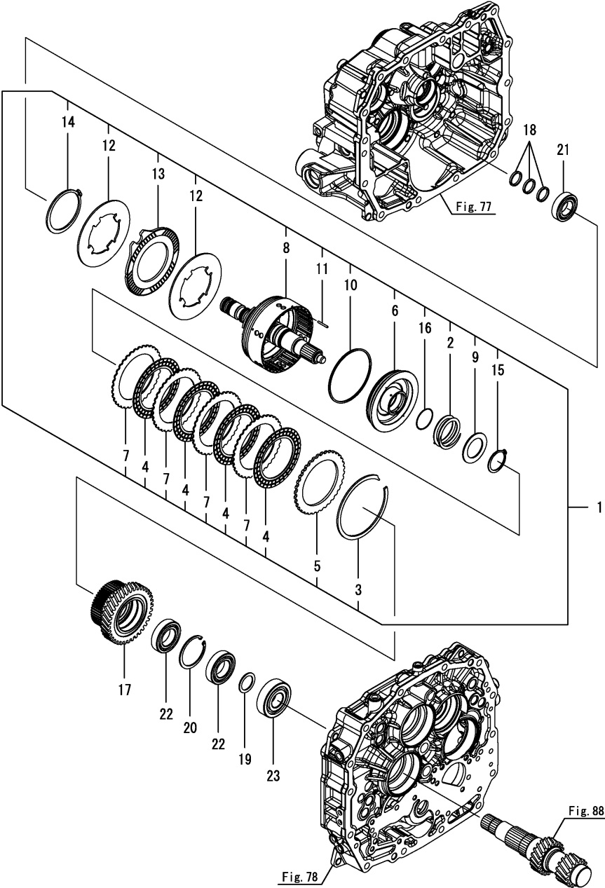
Fig.74. P.T.O. 클러치
