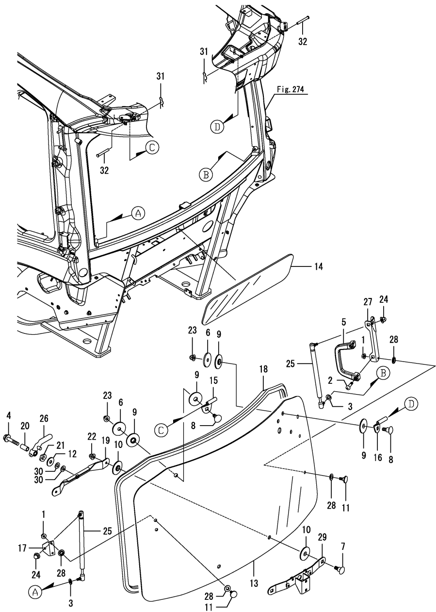
Fig.278. 후방창문
