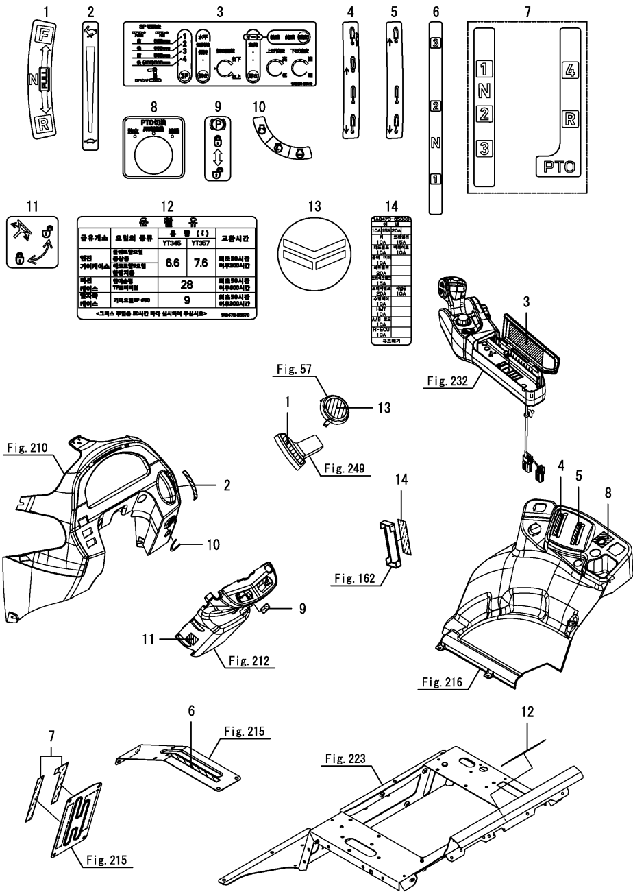
Fig.240. 명판(3)
