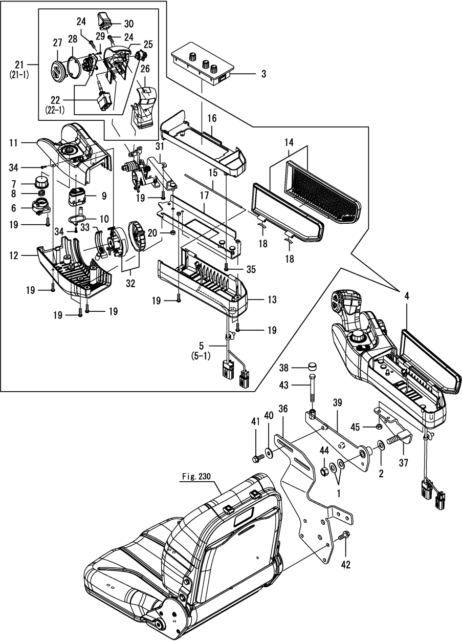
Fig.232. 팔걸이
