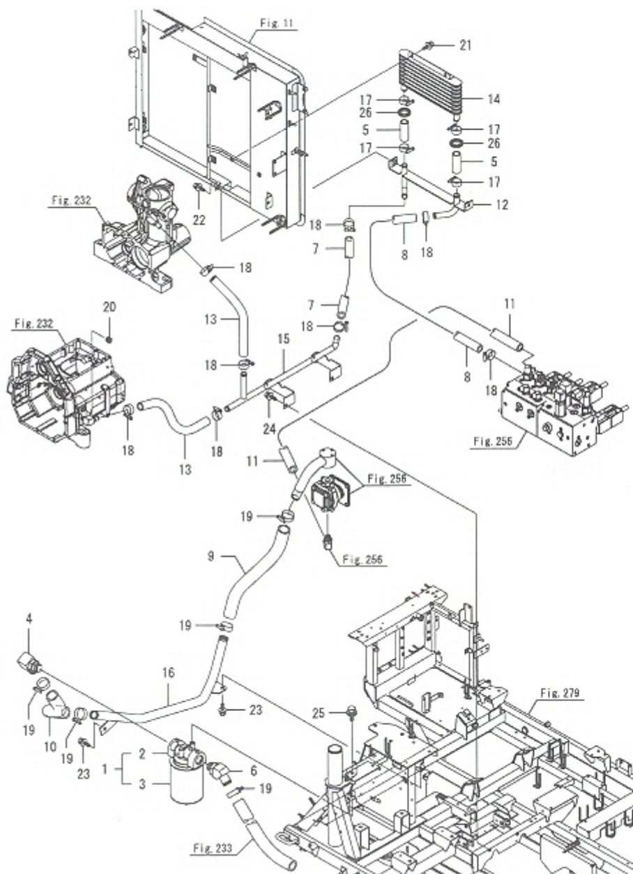
Fig.260. 배관(2)
