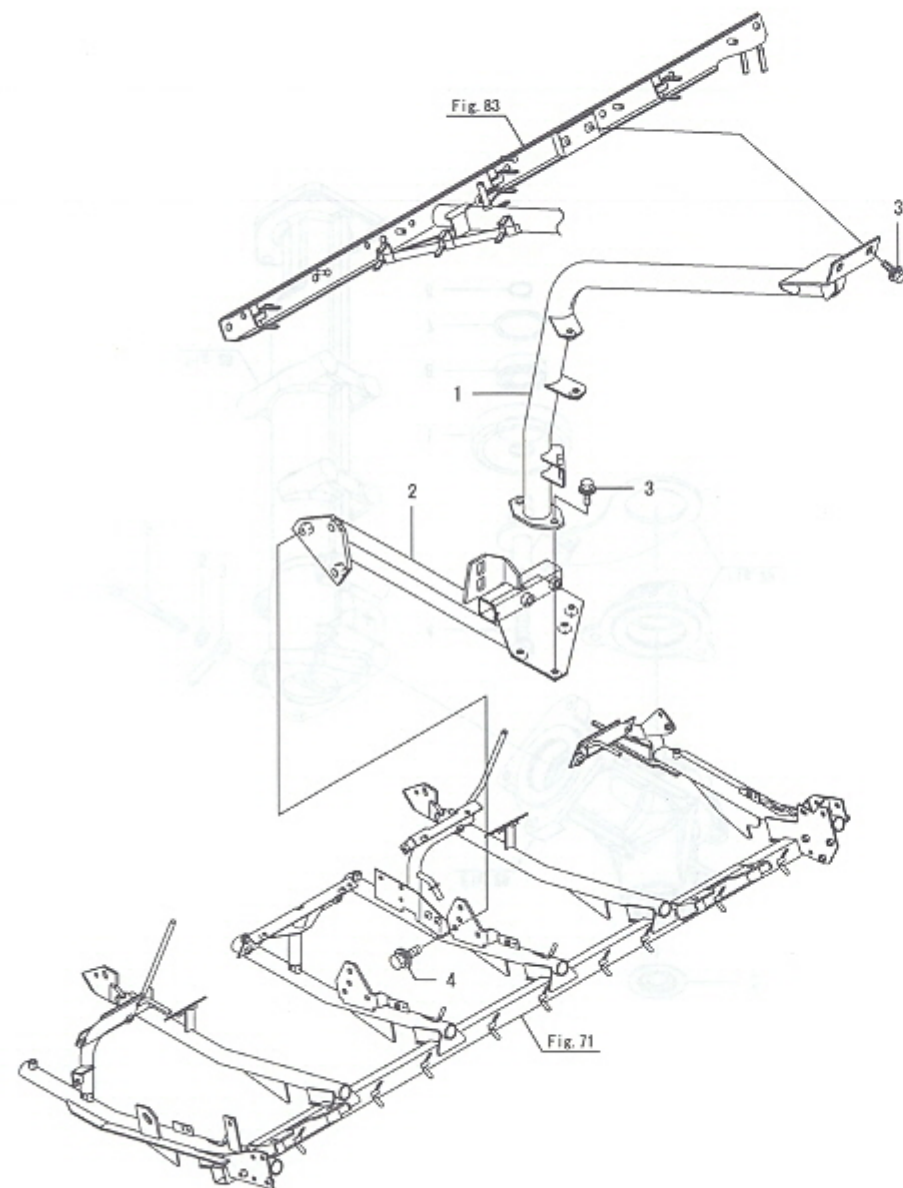
Fig.95. 끌어모음프레임(중-우)
