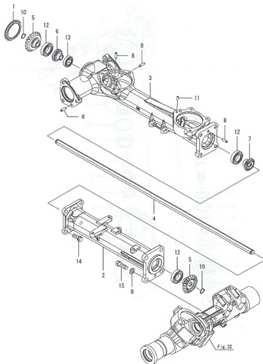
Fig.34. 5드라이브 케이스(3)
