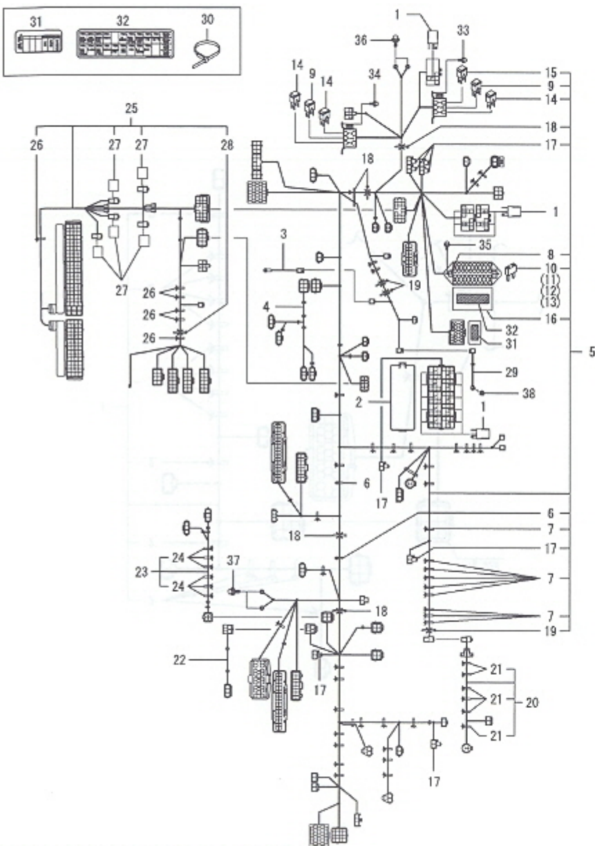
Fig.321. 배선(주행)
