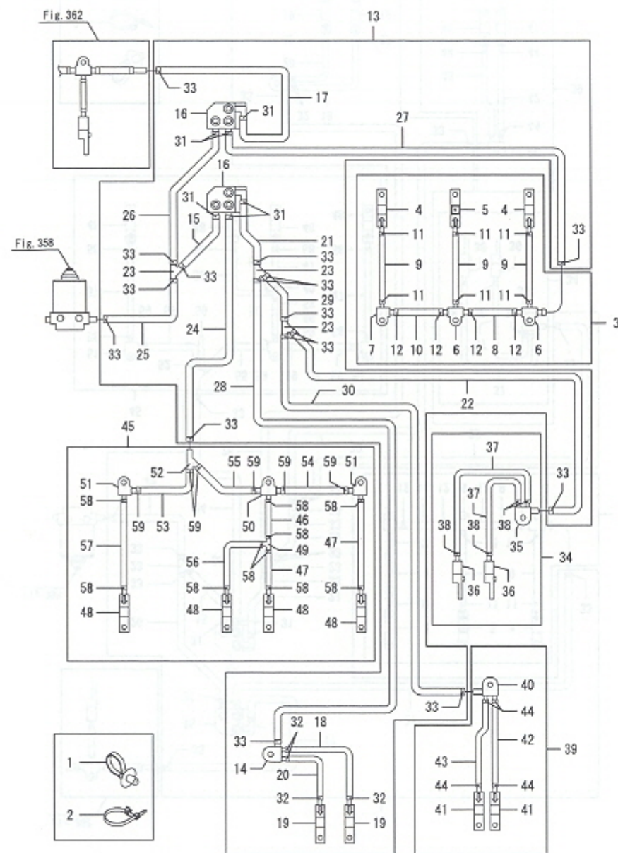
Fig.359. 주유장치(2)
