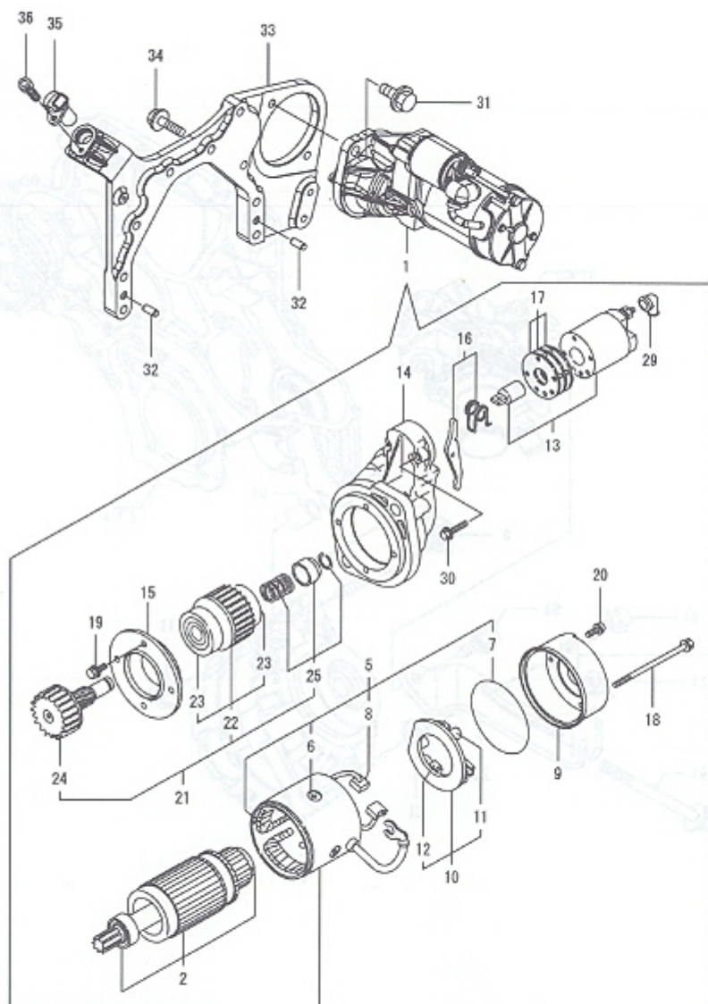
Fig.15. 시동모터
