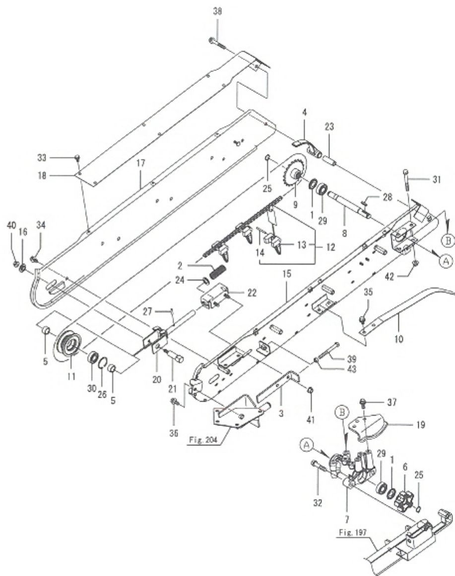
Fig.198. 짚배출반송(이삭끝)
