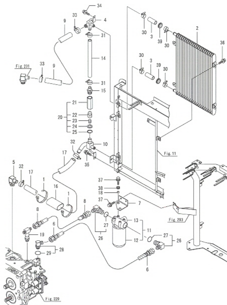
Fig.258. 배관(H.S.T.)
