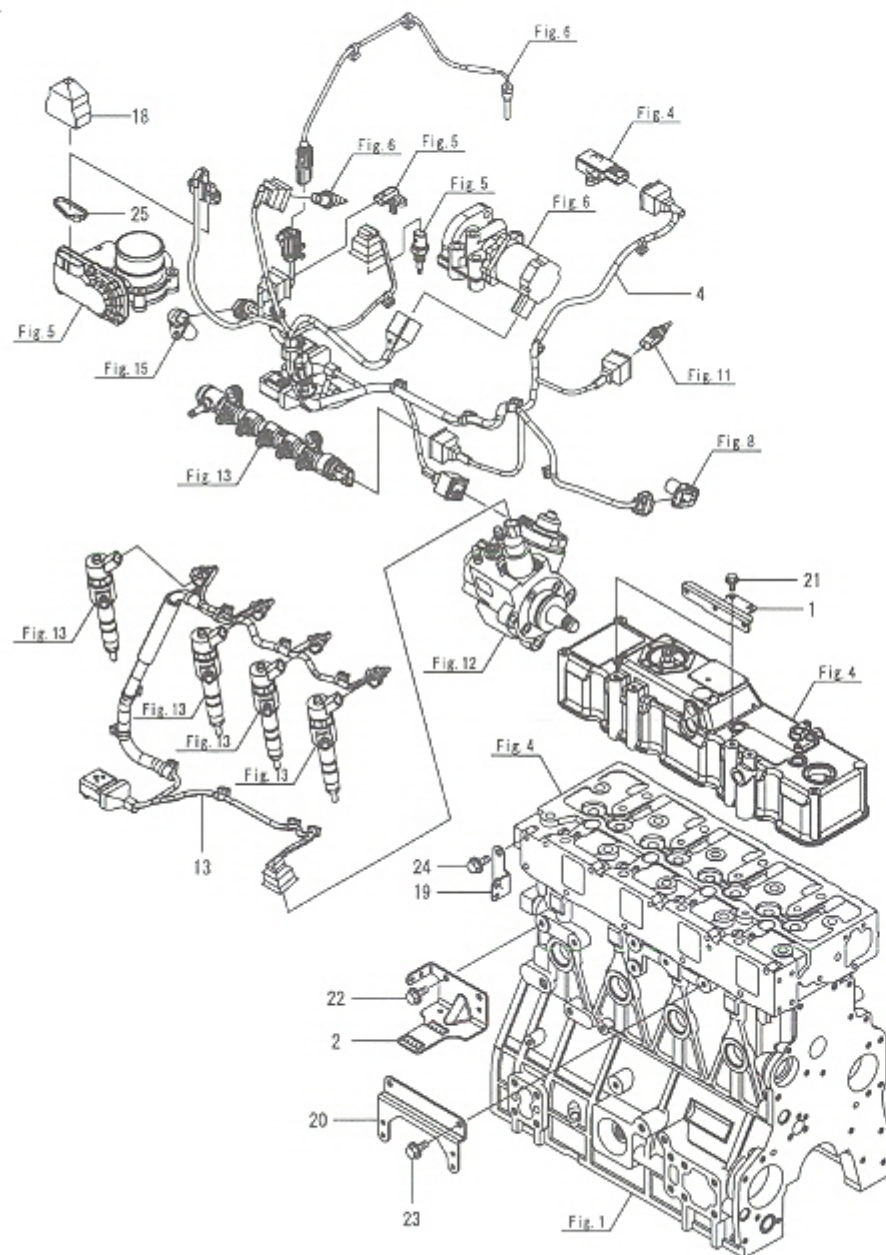
Fig.18. 전장품
