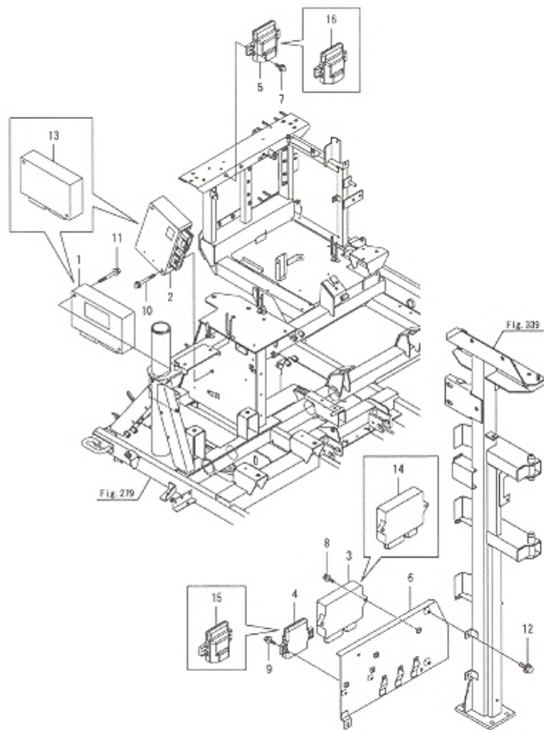
Fig.346. 컨트롤(새시)
