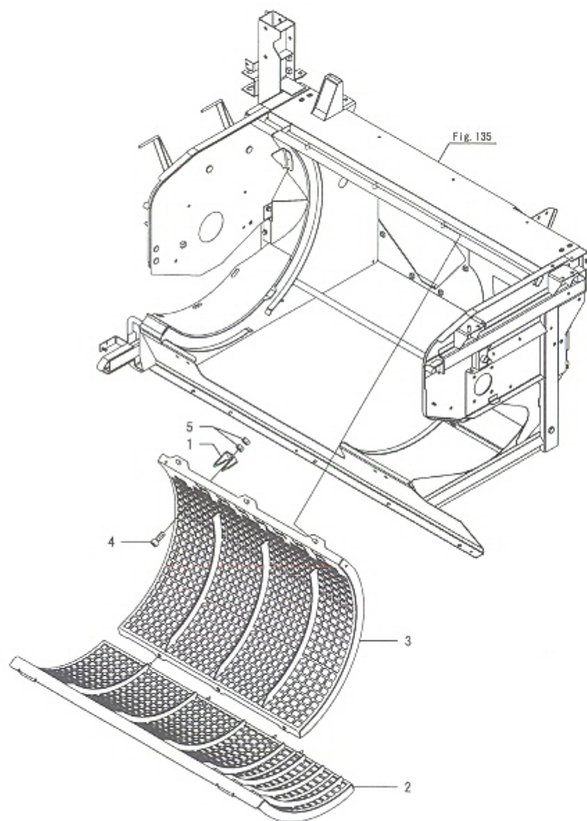
Fig.144. 스크린 프레임
