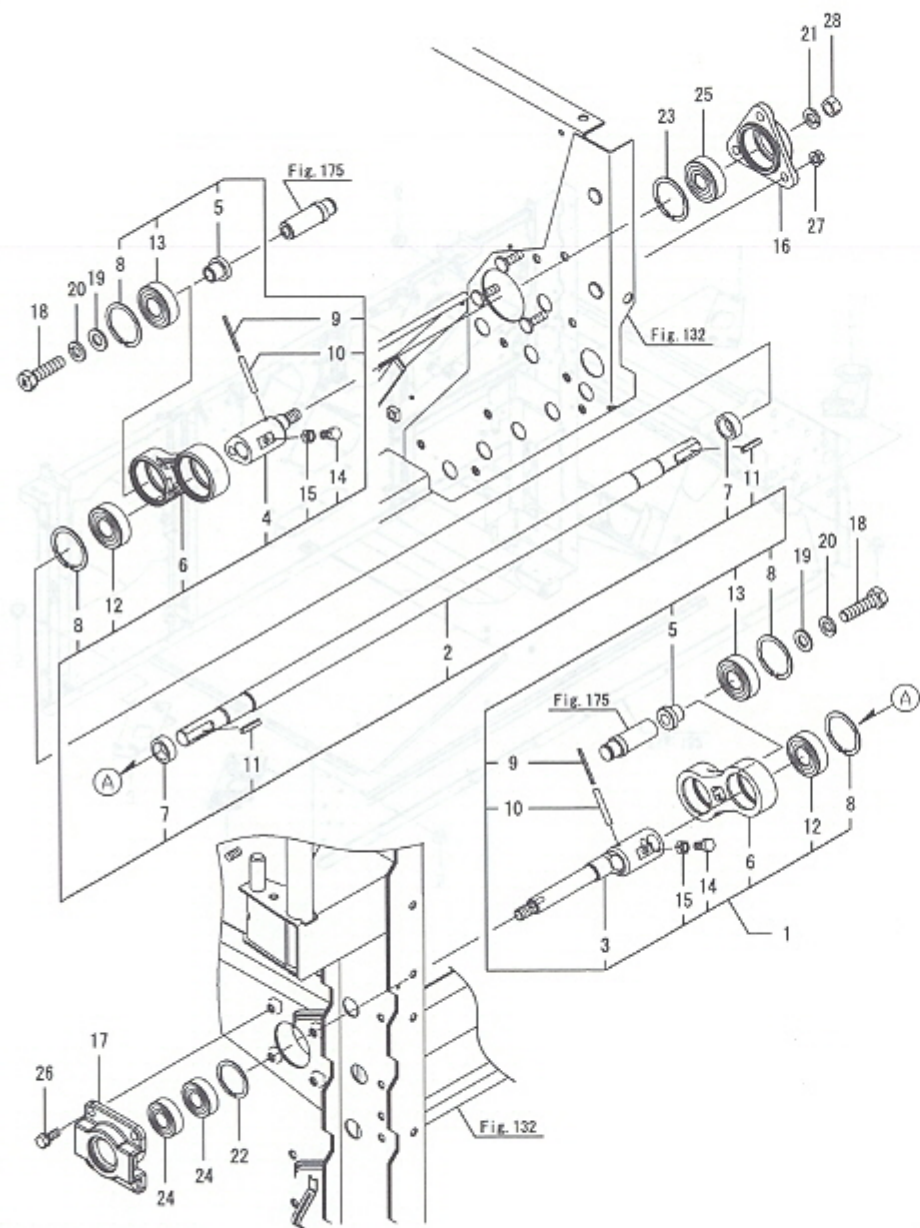
Fig.171. 요동축
