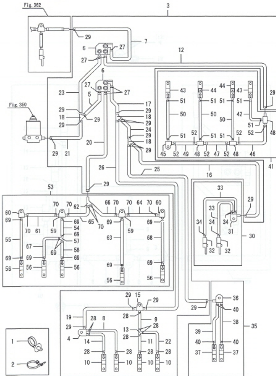
Fig.361. 주유장치(2)
