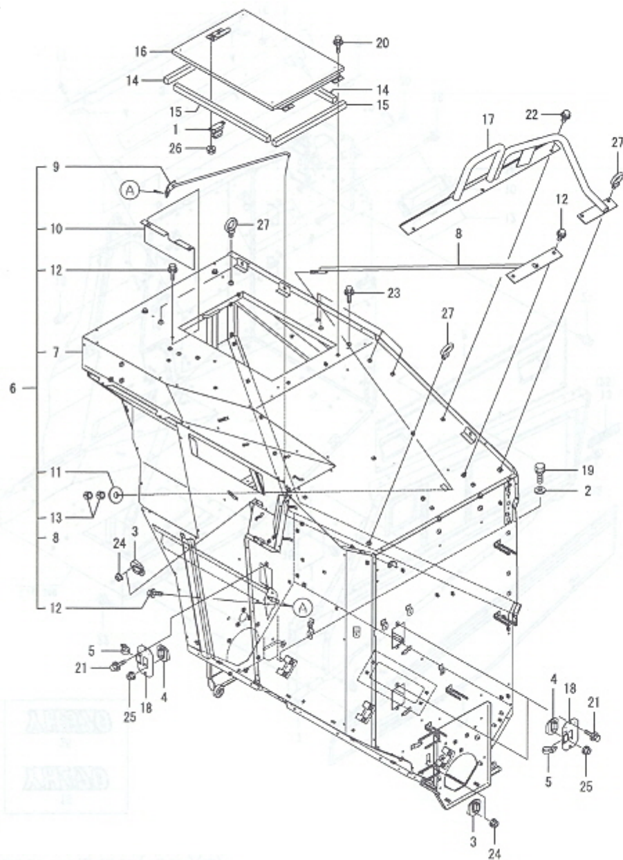
Fig.349. 곡물탱크(캐빈)(1)
