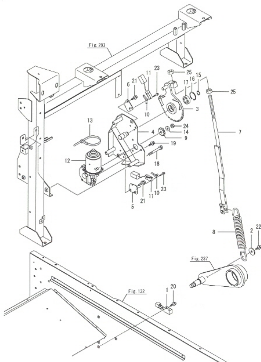
Fig.208. 탈곡구동(2)
