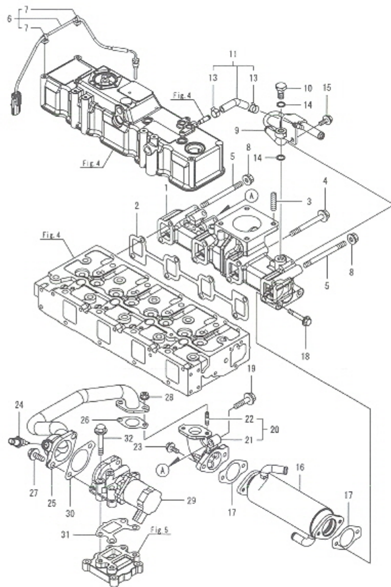
Fig.6. 배기에너지폴드
