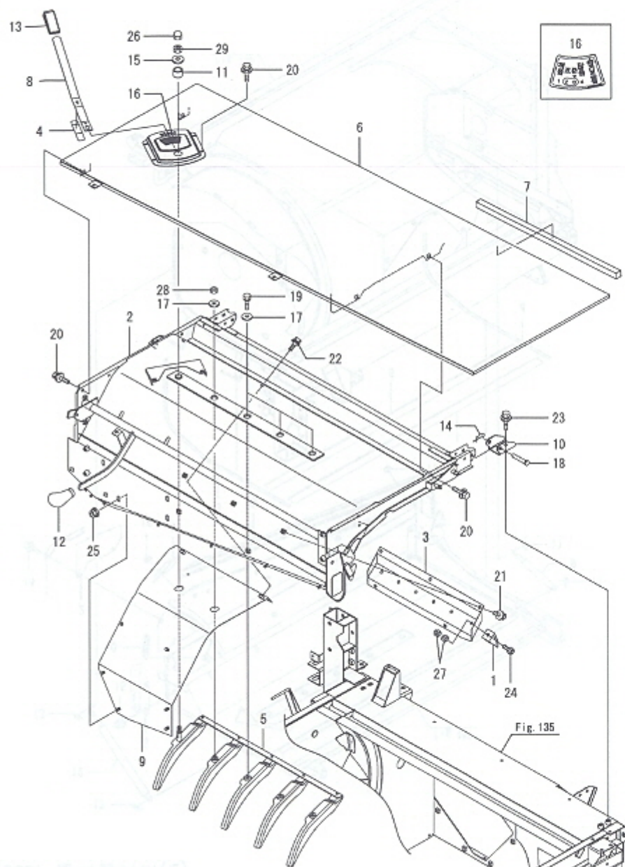
Fig.165. 탈곡실커버(1)
