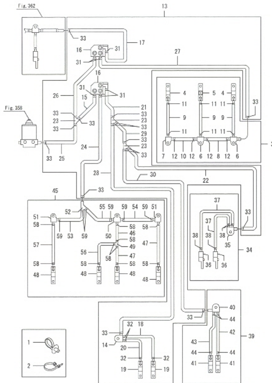
Fig.359. 주유장치(2)
