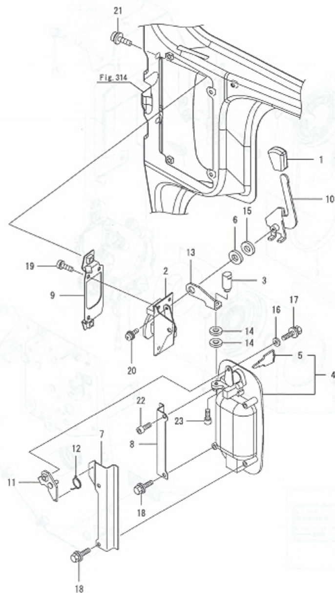
Fig.317. 출입문장금
