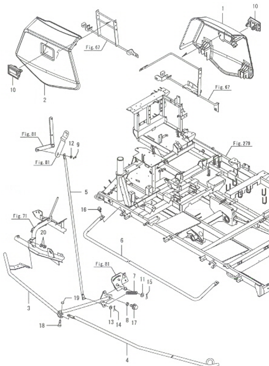
Fig.21. 예취(캐빈)(2)
