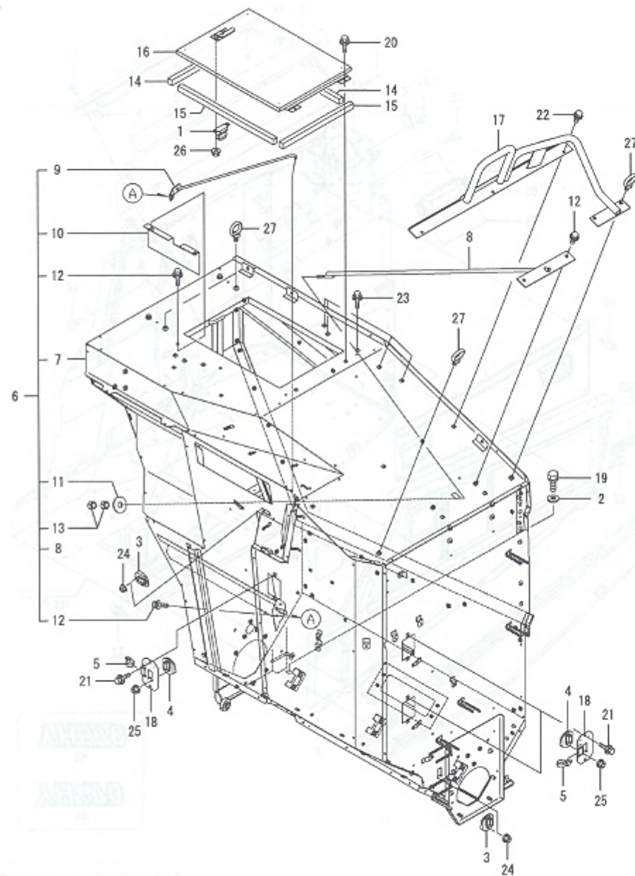
Fig.347. 곡물탱크(1)
