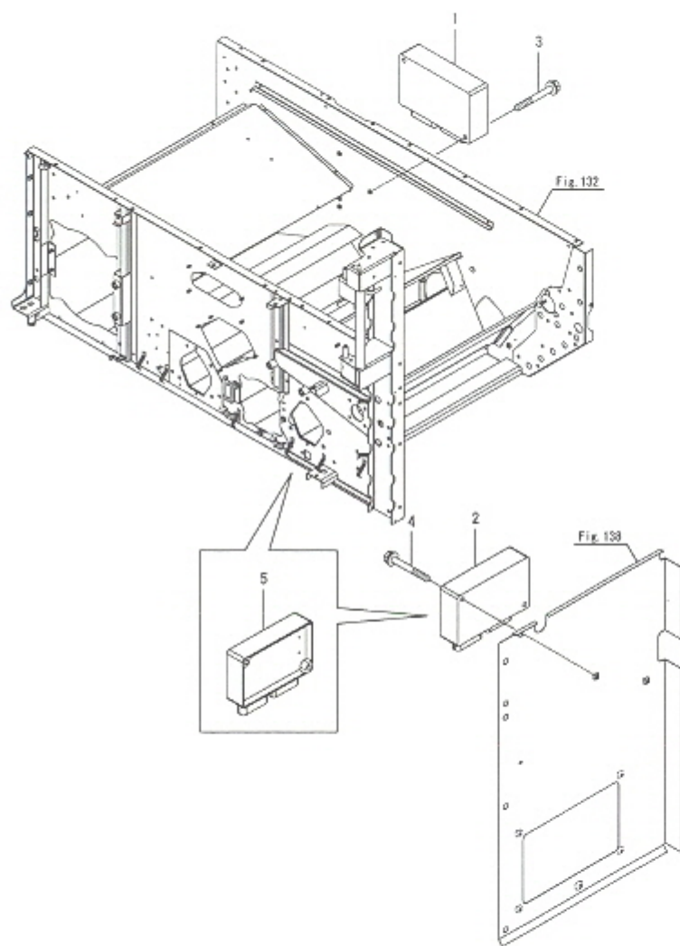
Fig.140. 컨트롤러(탈곡)
