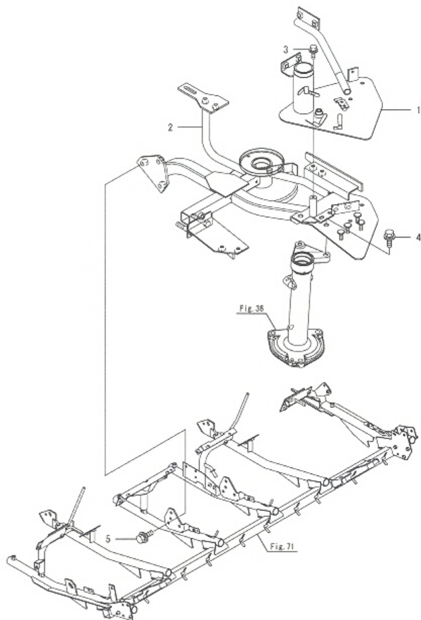
Fig.94. 끌어모음프레임(중-좌)
