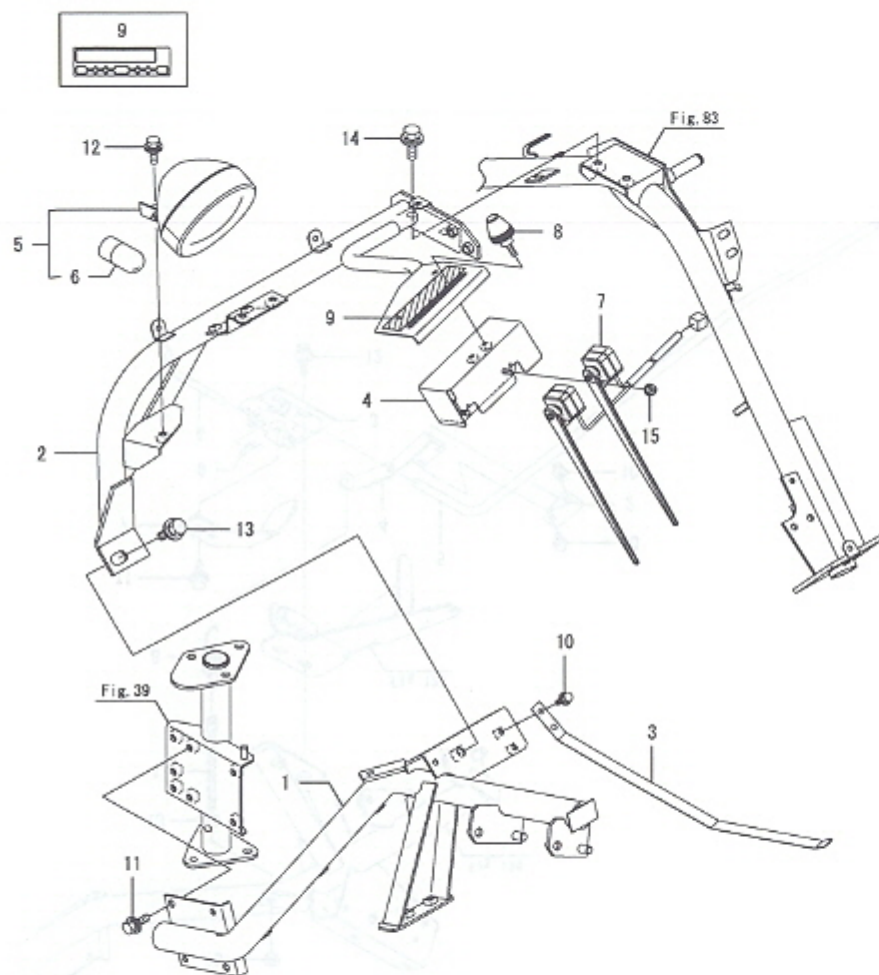
Fig.127. 보조반송프레임
