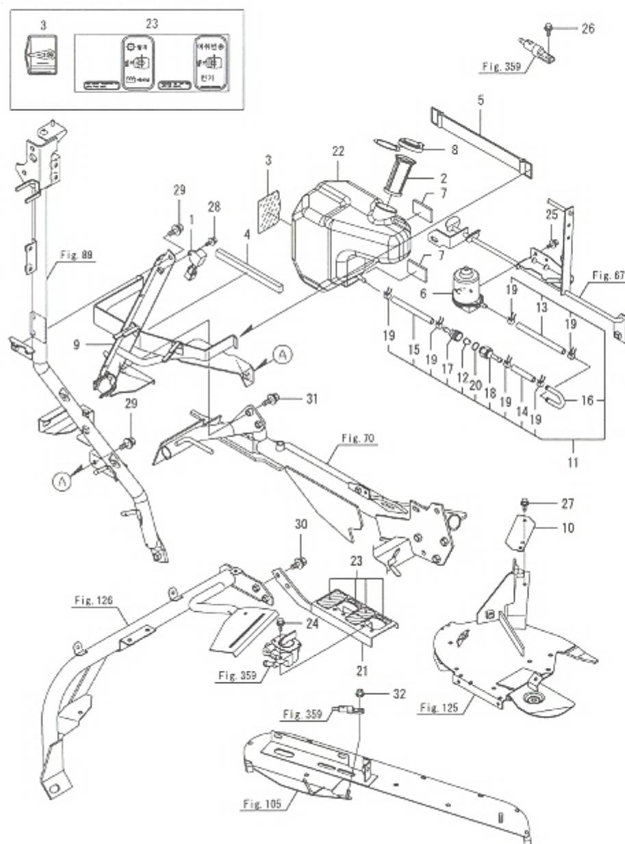
Fig.358. 주유장치(1)
