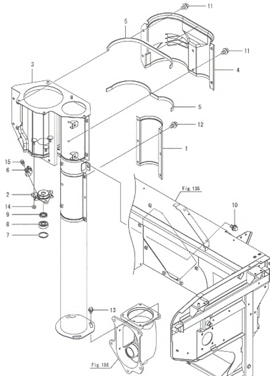
Fig.188. 2번처리통케이스(1)
