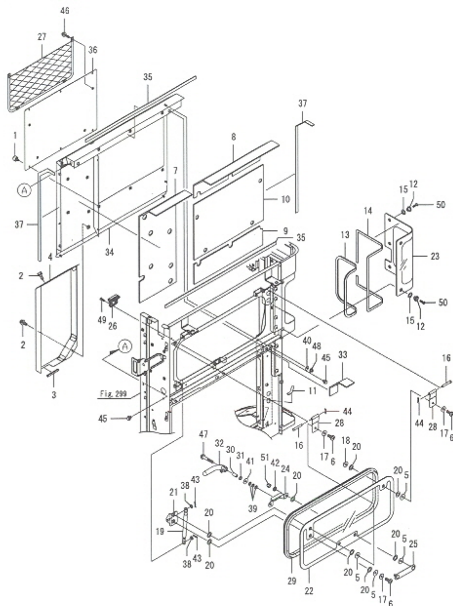
Fig.302. 캐빈 삭구(후면)
