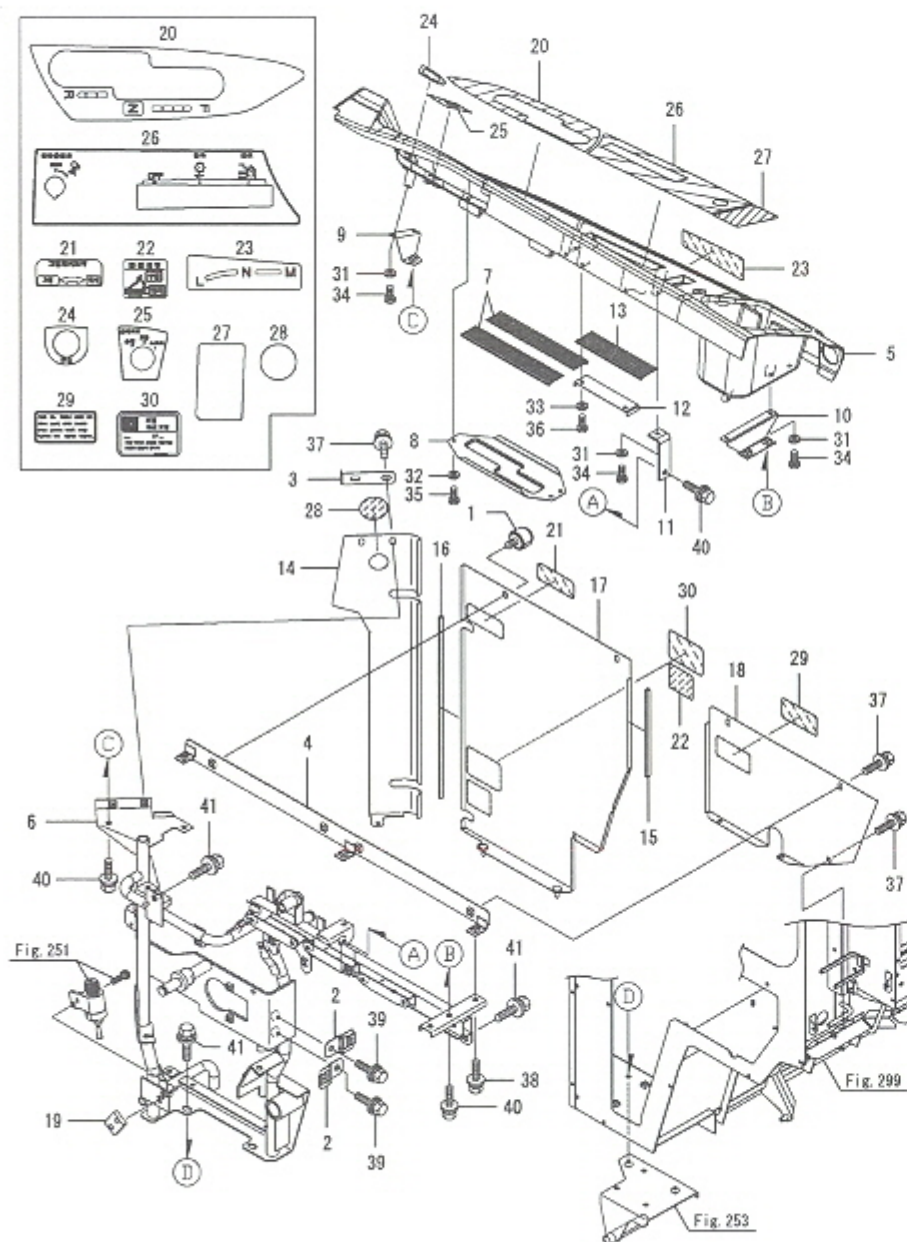
Fig.248. 사이드칼럼(캐빈)(1)
