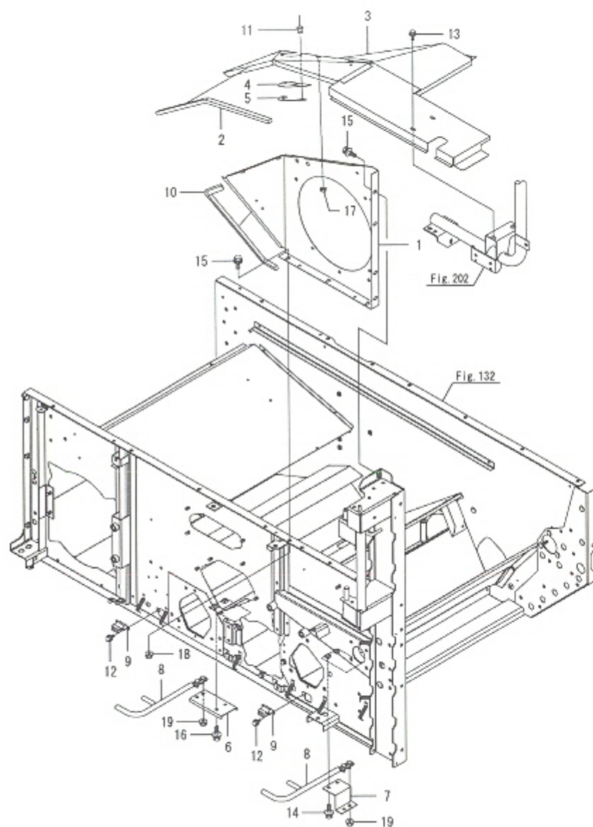
Fig.134. 하부본체취부프레임(3)
