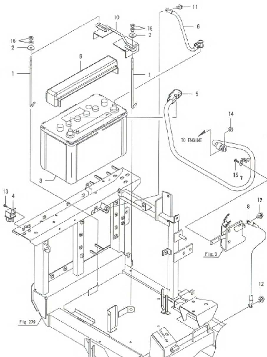
Fig.320. 배터리
