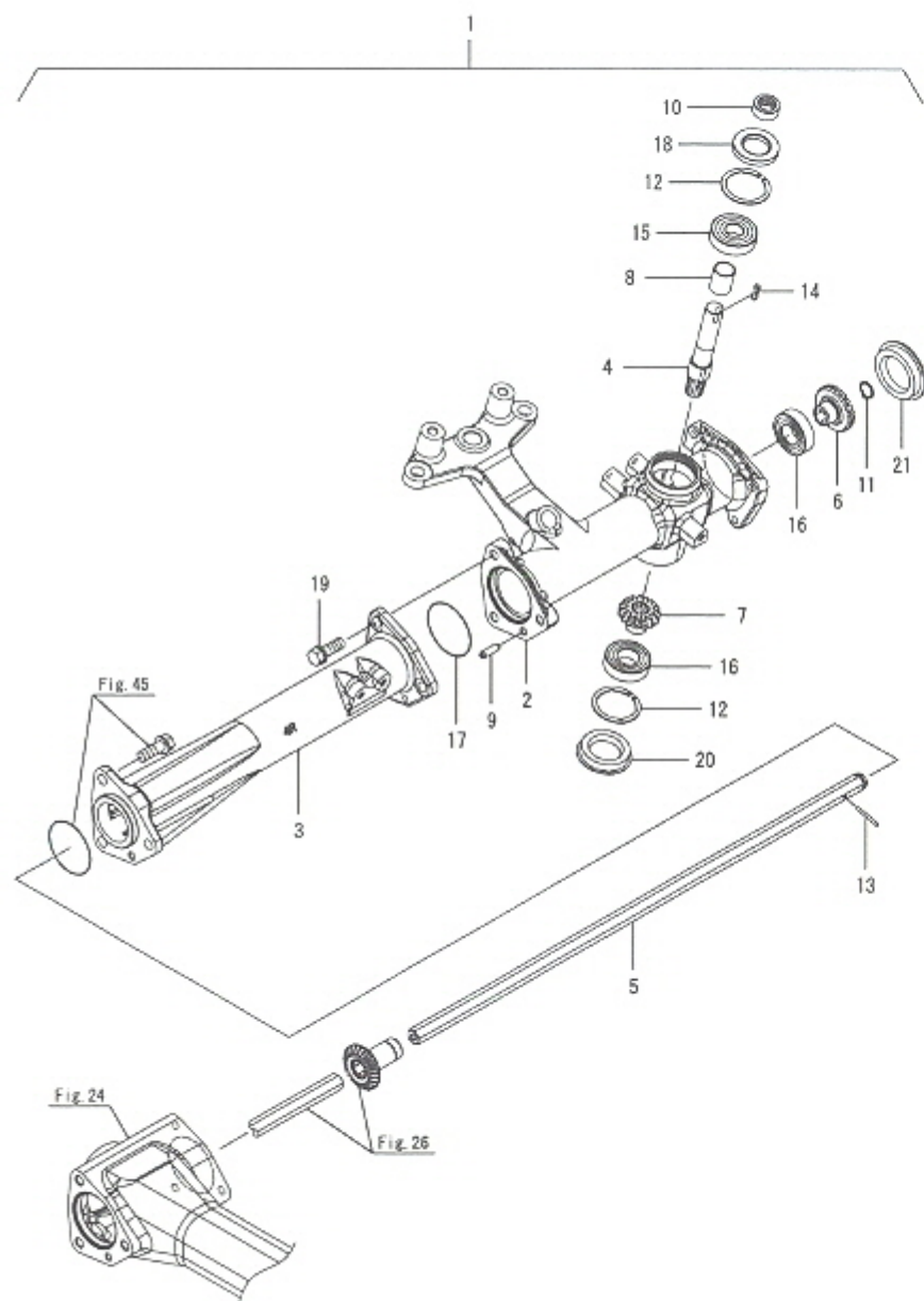
Fig.27. 4드라이브 케이스(6)
