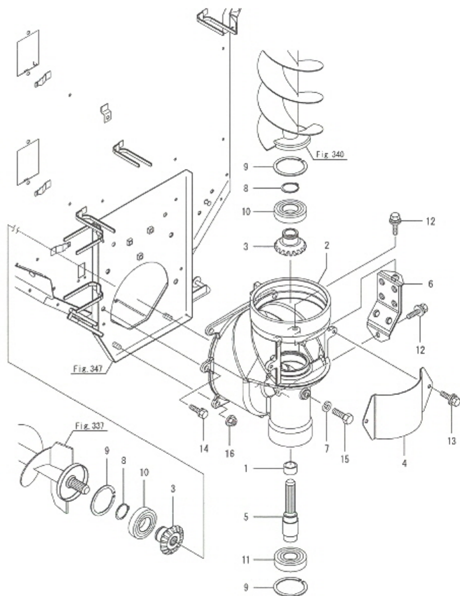
Fig.338. 하부컨베이어연결
