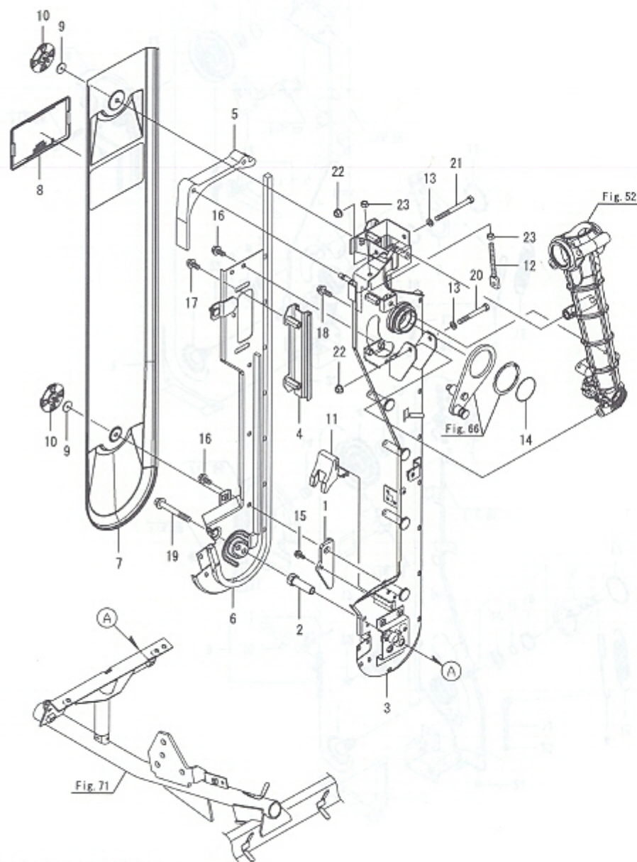
Fig.64. 인기케이스(중)
