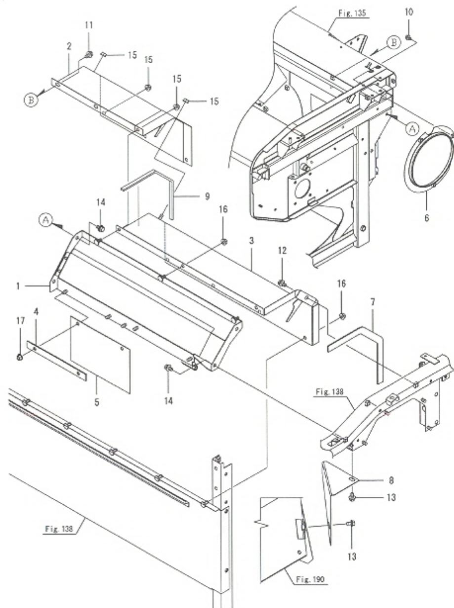
Fig.170. 처리 드럼 커버
