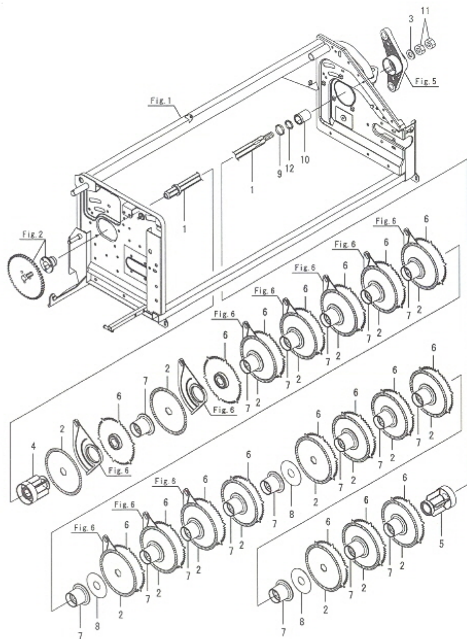
Fig.3. 축(저속)
