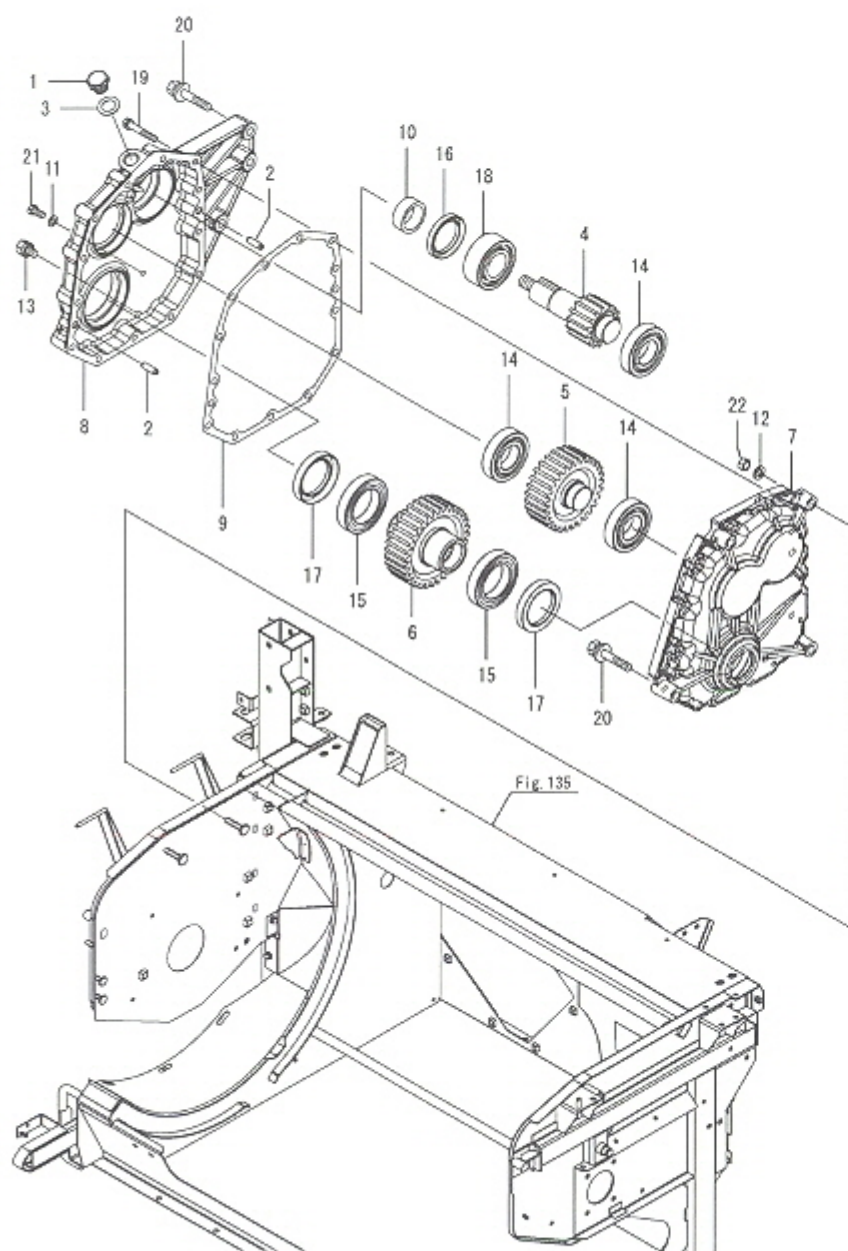
Fig.160. 탈곡동구동
