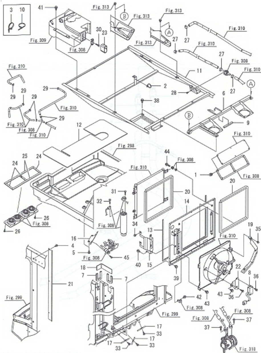
Fig.311. 에어컨취부(1)
