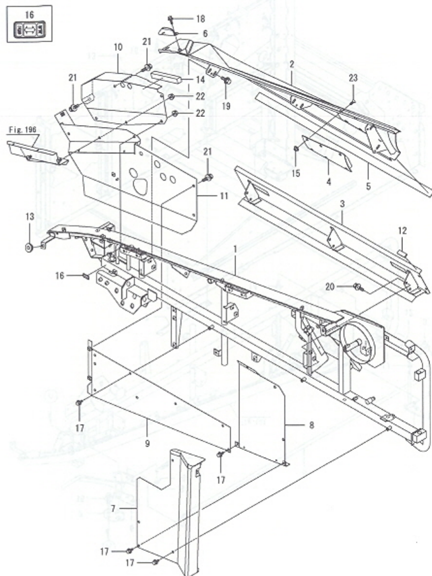
Fig.141. 탈곡실프레임(좌)(1)
