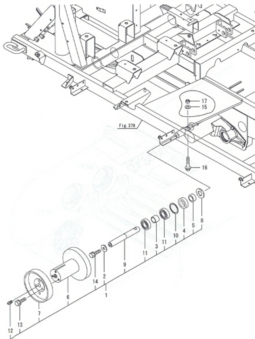
Fig.289. 캐리어 롤러
