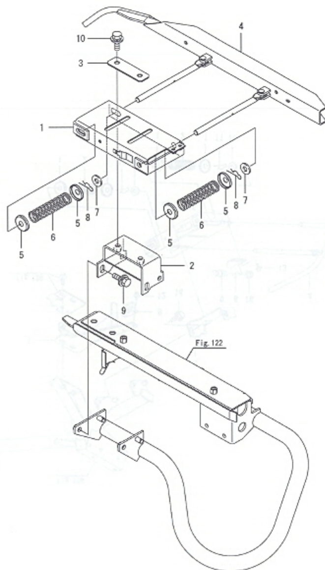
Fig.123. 세로잡이가이드
