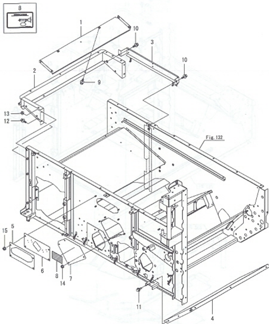
Fig.133. 하부본체취부프레임(2)
