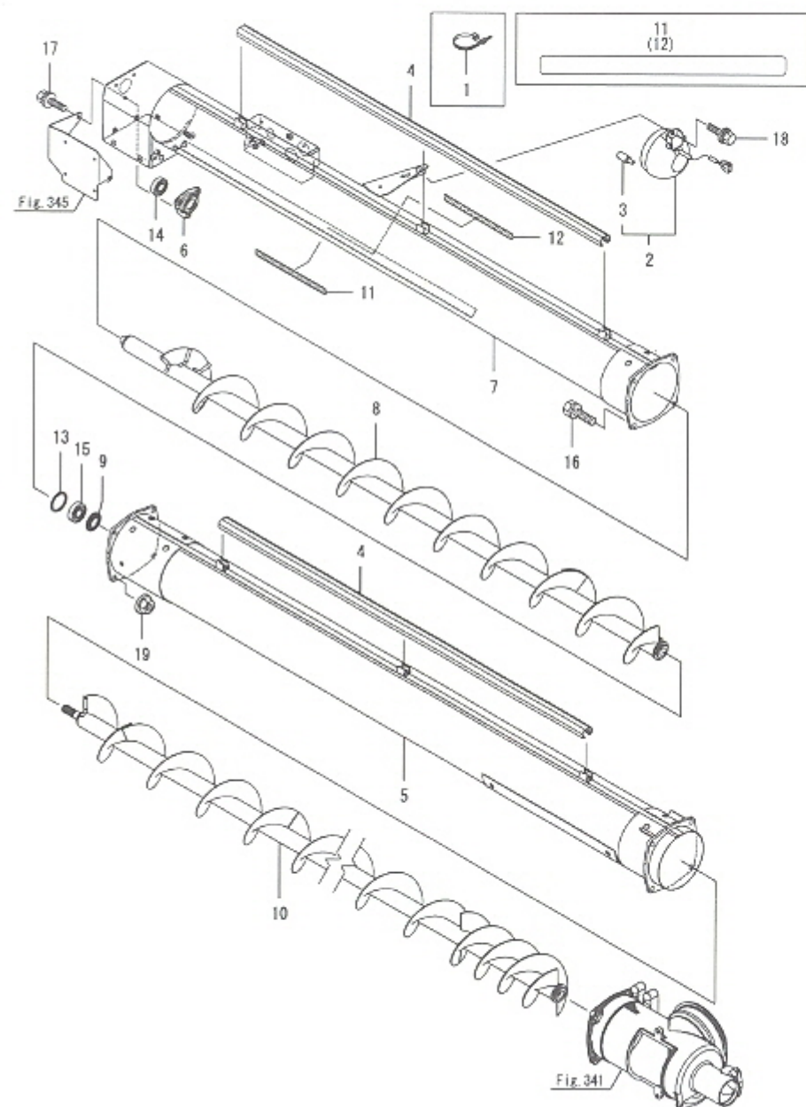
Fig.344. 오거(측면)
