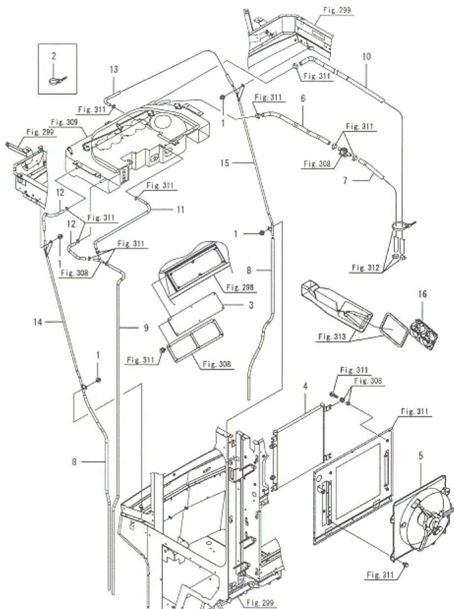
Fig.310. 에어컨(3)
