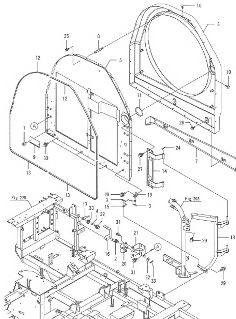
Fig.294. 엔진실 커버
