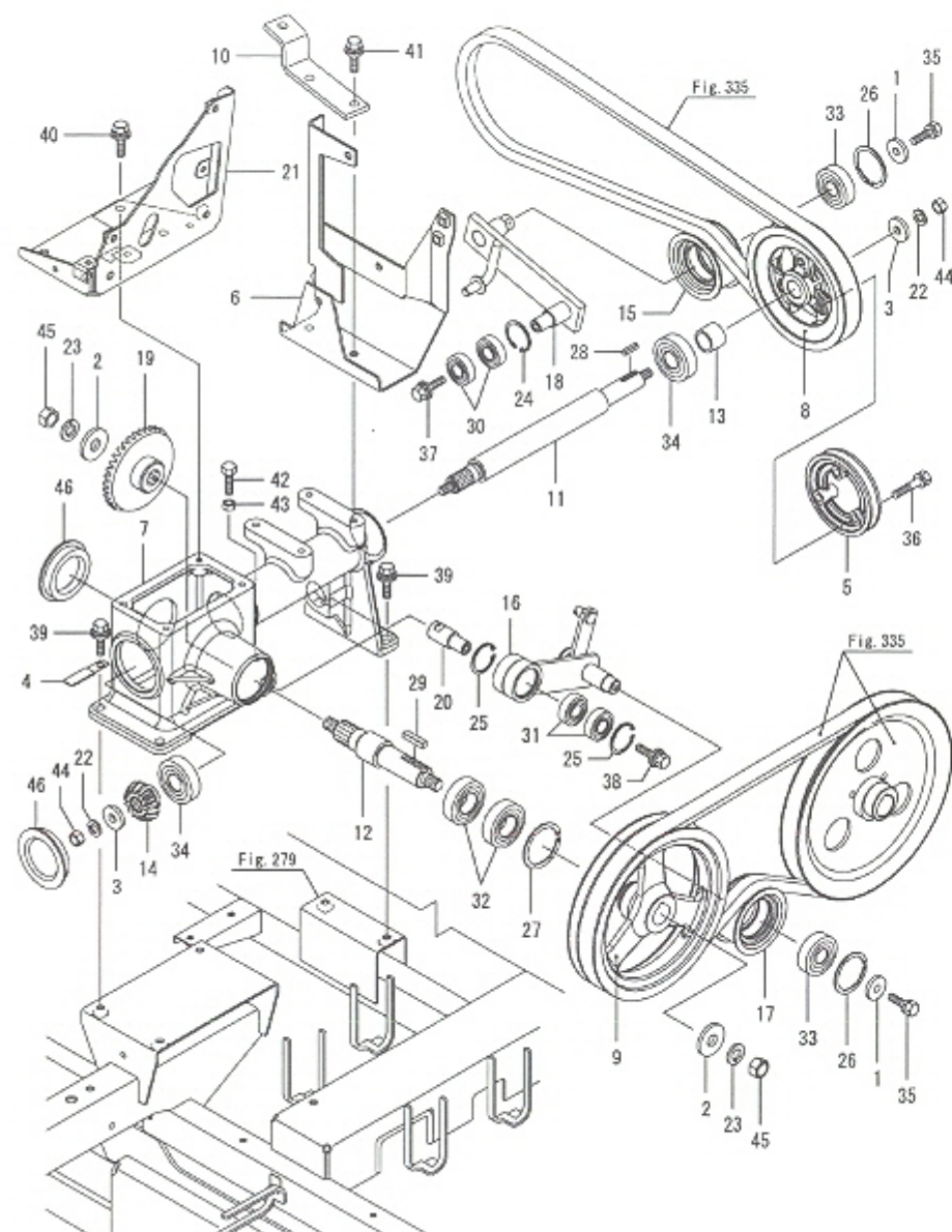
Fig.334. 오기입력(캐빈)
