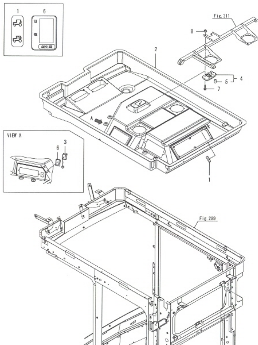
Fig.298. 캐빈(천장)
