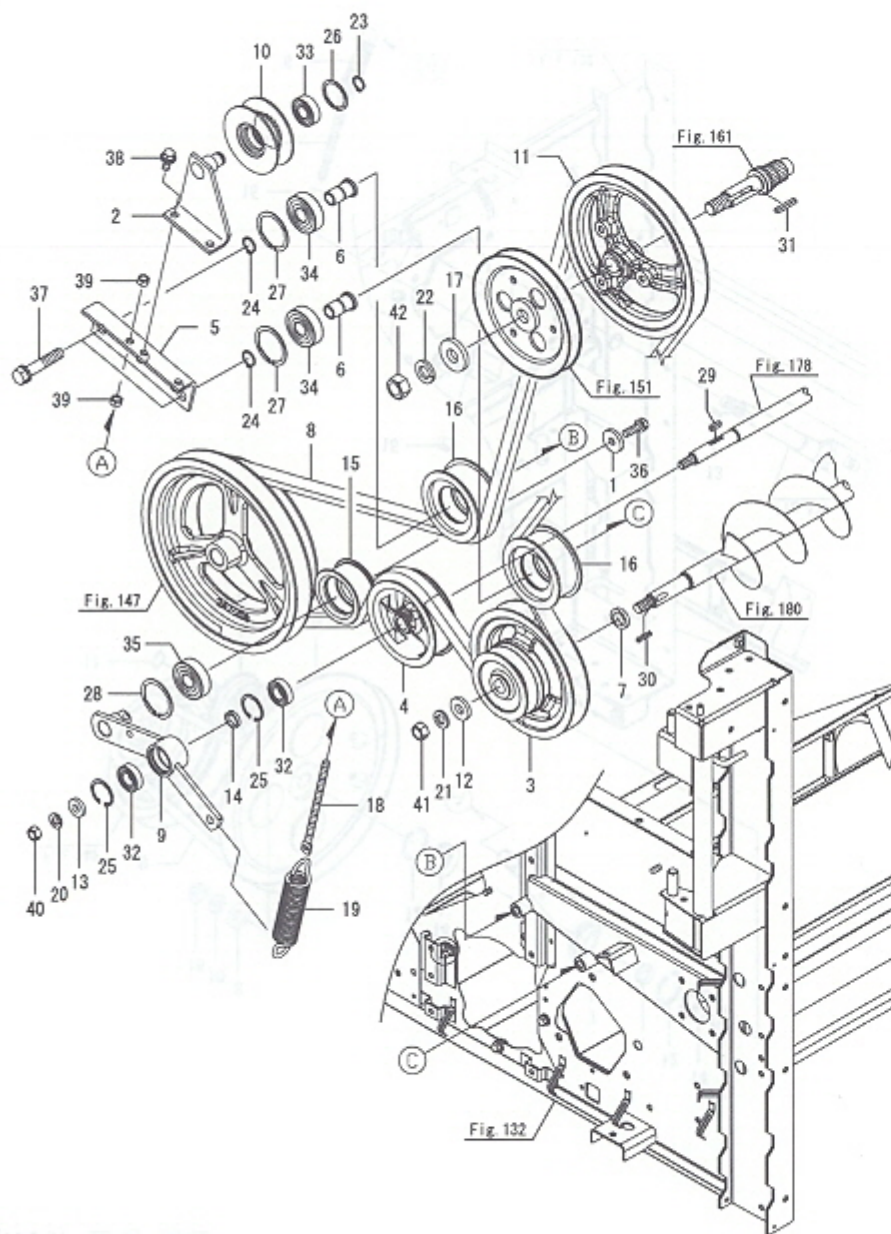
Fig.149. 벨트(2차)
