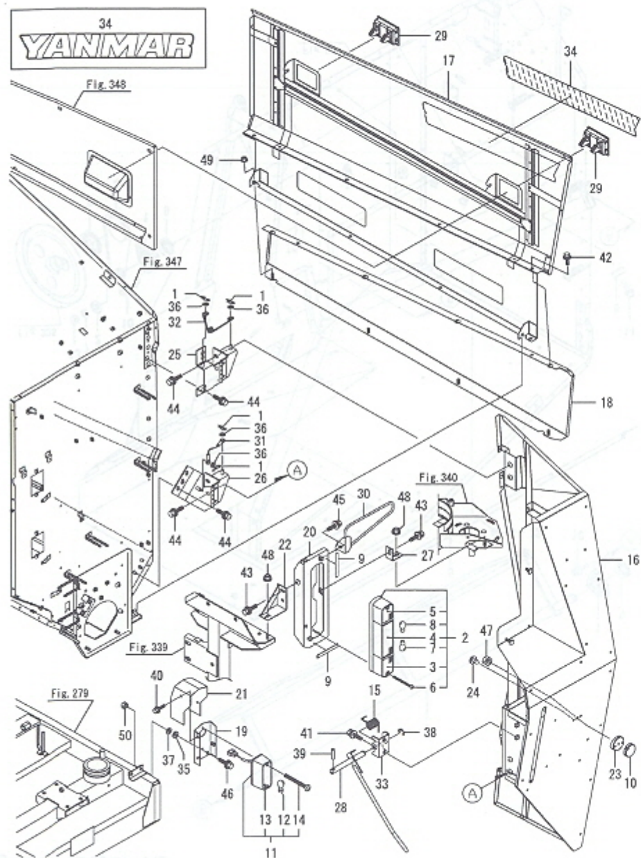
Fig.355. 탱크커버
