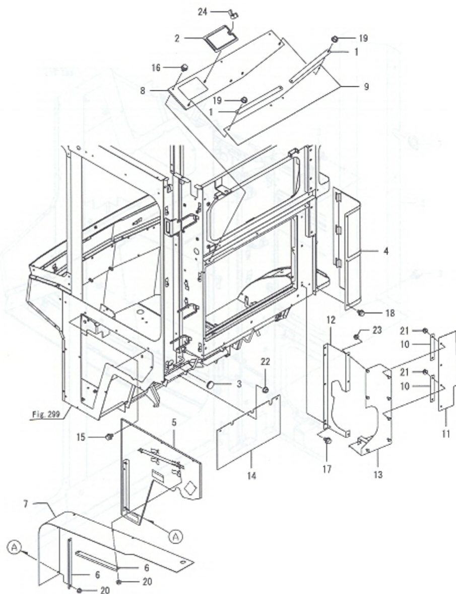
Fig.305. 캐빈시일(1)
