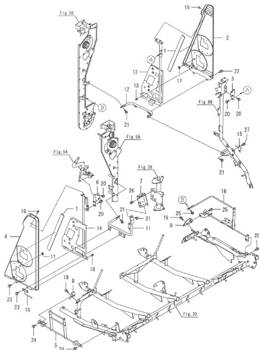
Fig.67. 예취커버(1)
