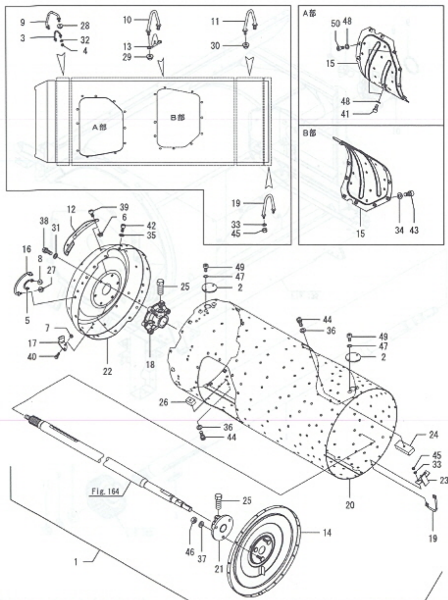
Fig.163. 탈곡통
