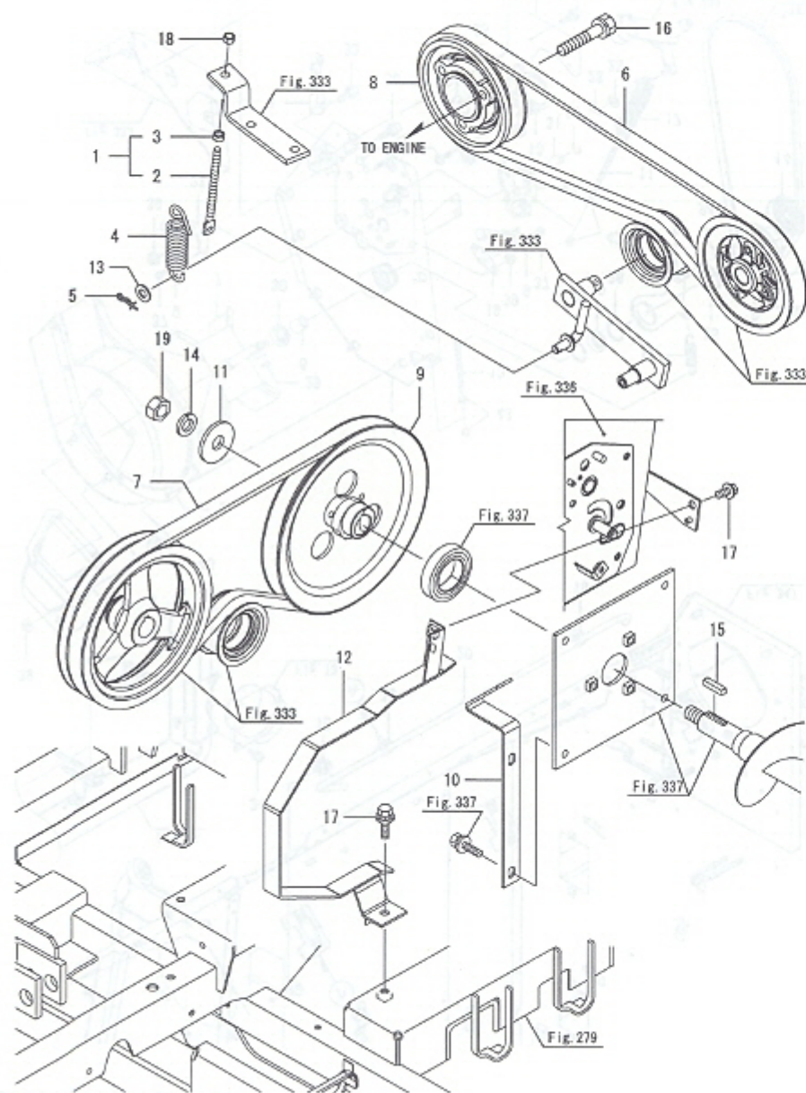
Fig.335. 오거 벨트
