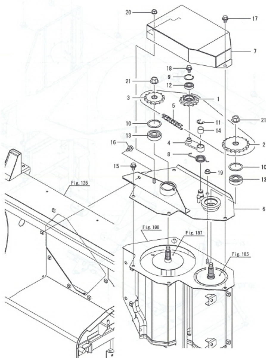
Fig.189. 2번처리통케이스(2)
