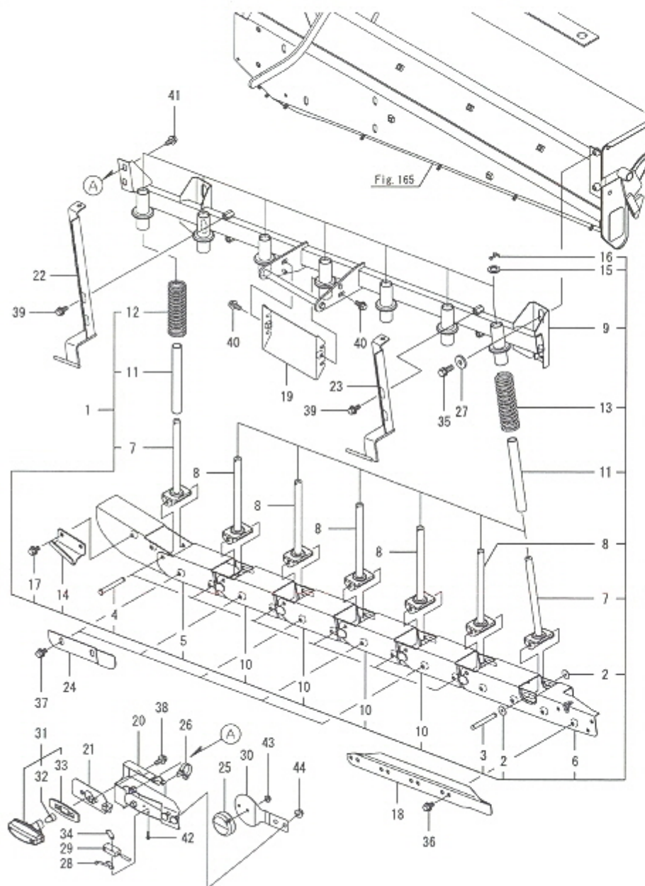
Fig.194. 질 고정 플레이트
