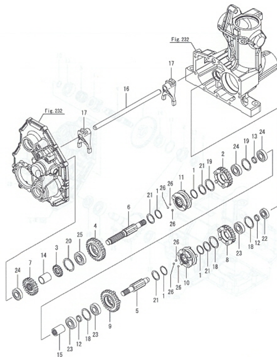
Fig.235. 카운터케이스(4)
