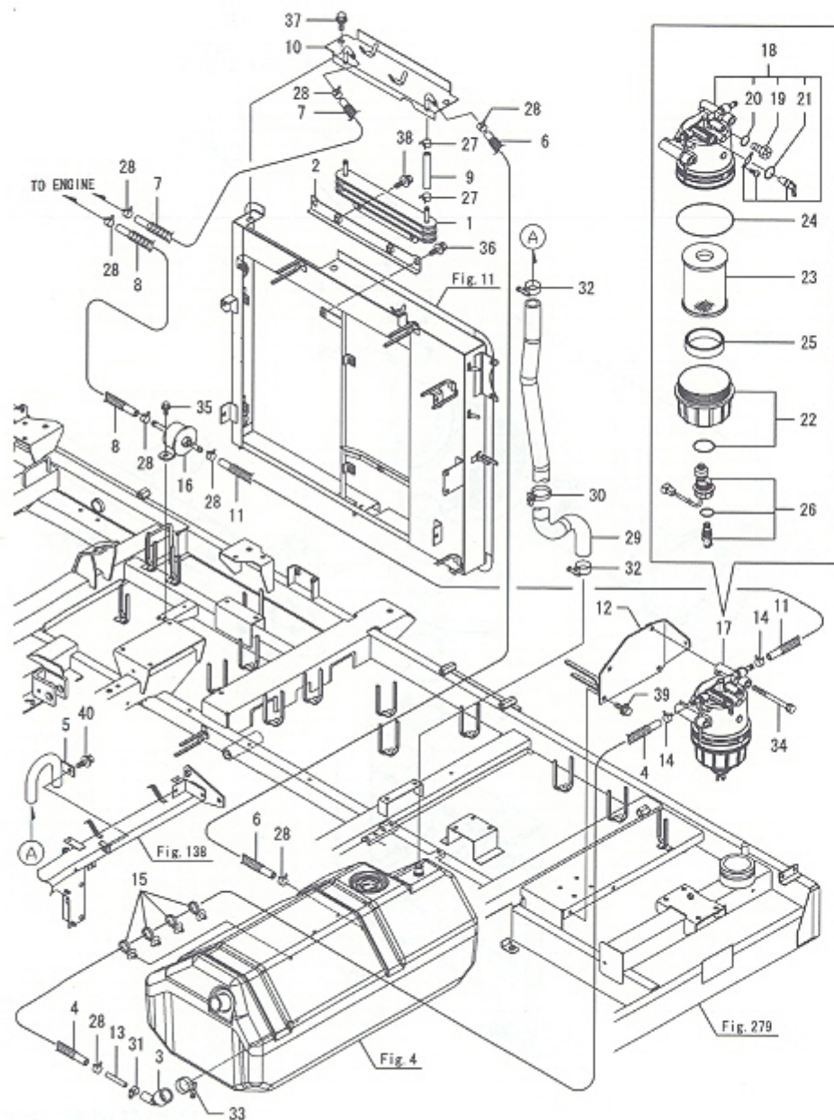
Fig.5. 연료탱크(2)
