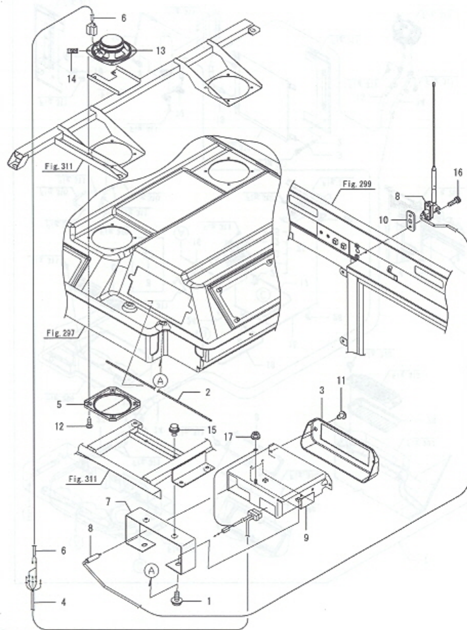
OCNP6-M03670 캐빈부 Fig.307. 스테레오
