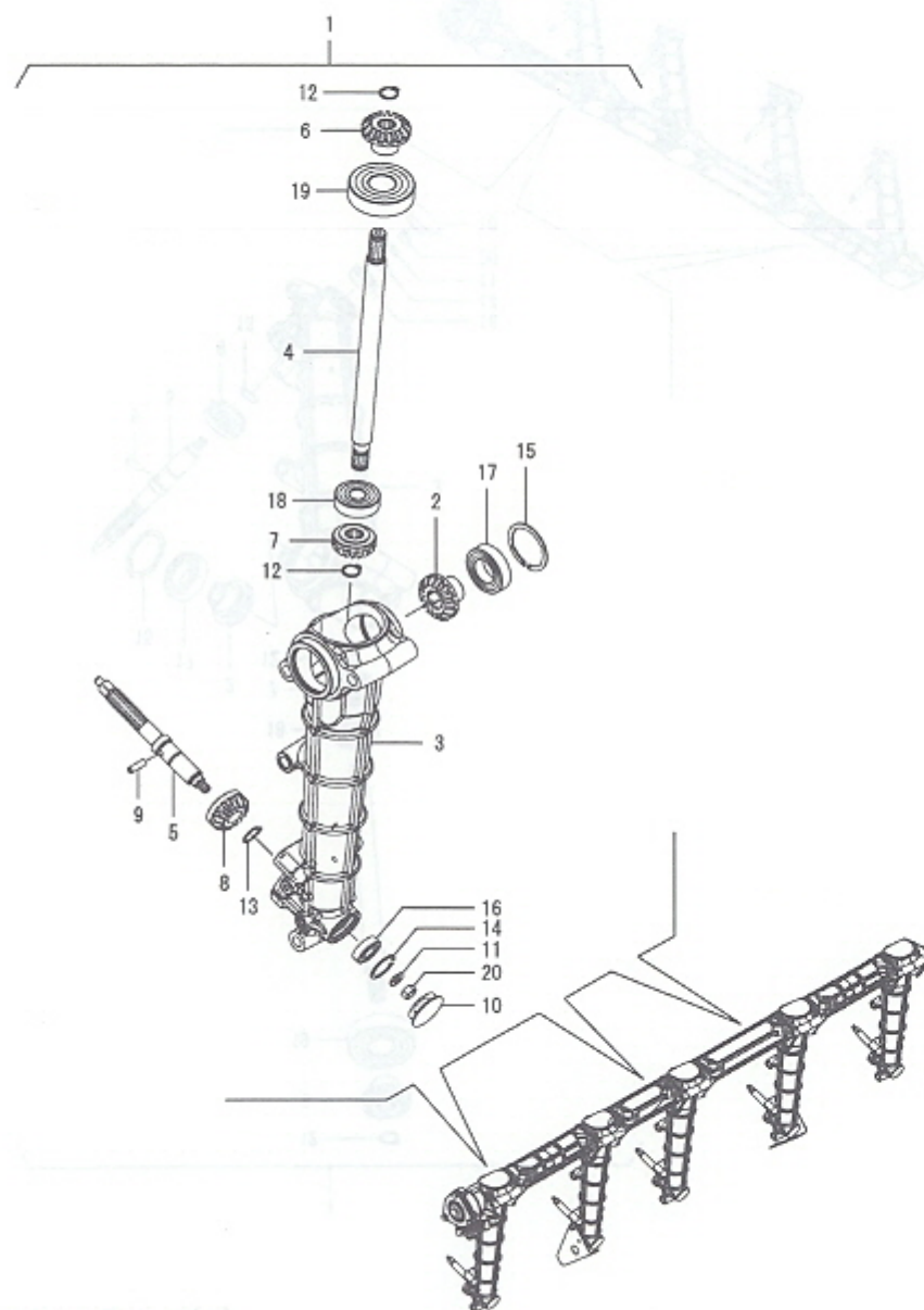
Fig.52. 인기형구동(2)
