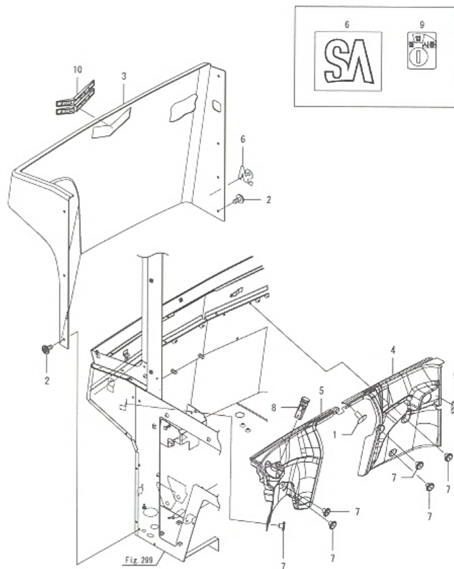
Fig.304. 캐빈의장(앞-하)
