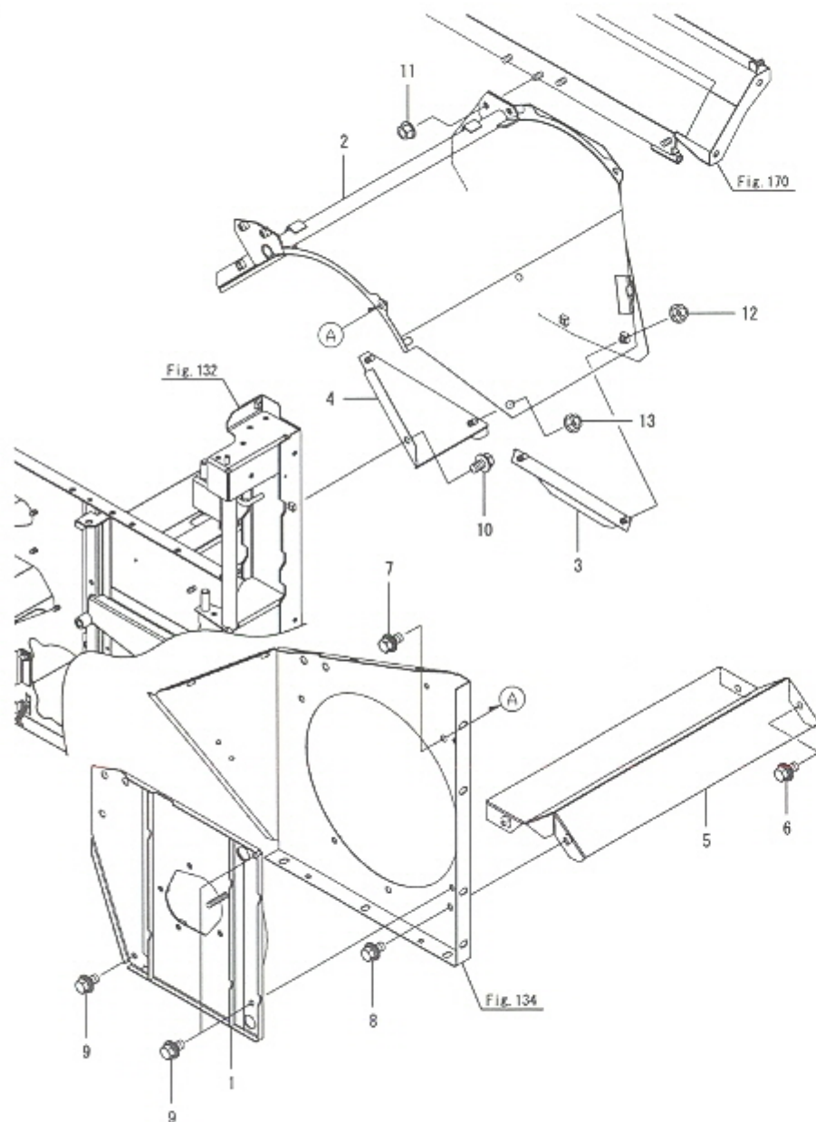
OCNP6-M03670 달곡(2) Fig.190. 흡입 드럼
