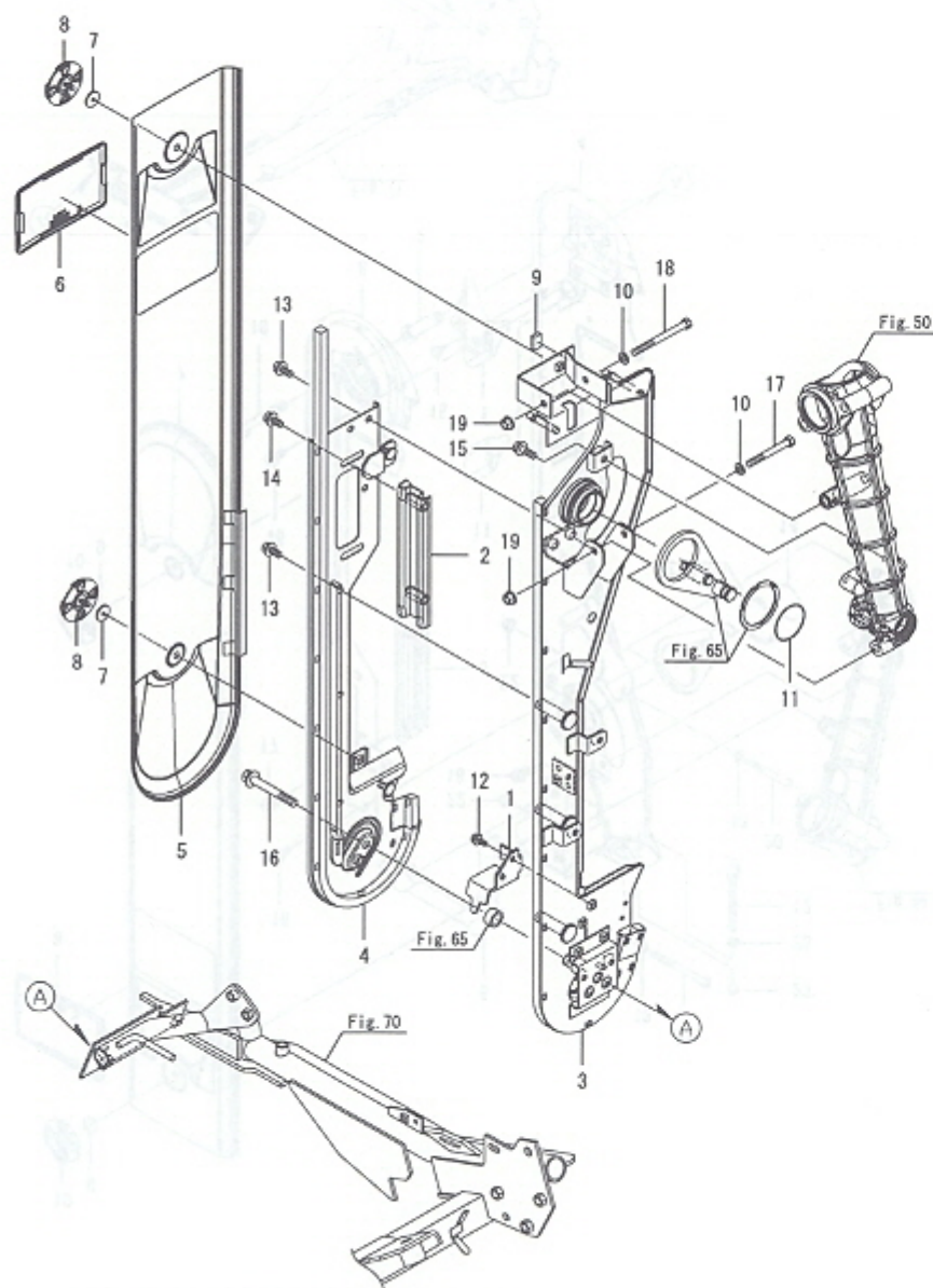
Fig.56. 픽업 케이스(오른쪽)
