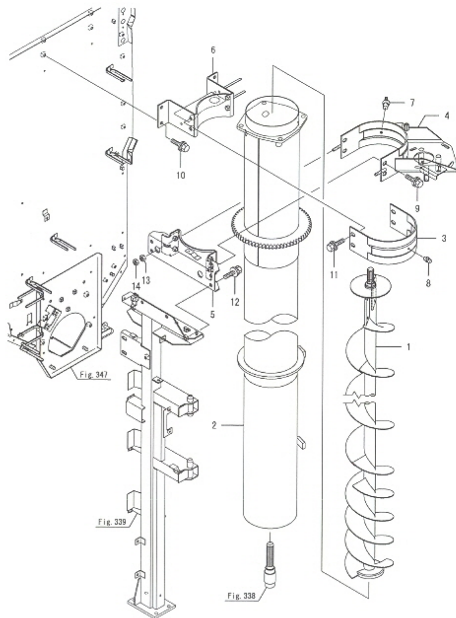
Fig.340. 수직 컨베이어
