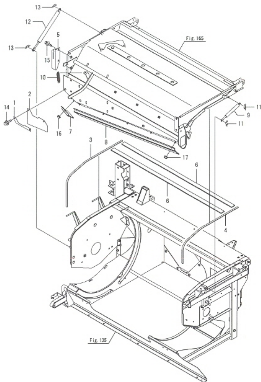
Fig.166. 탈곡실커버(2)
