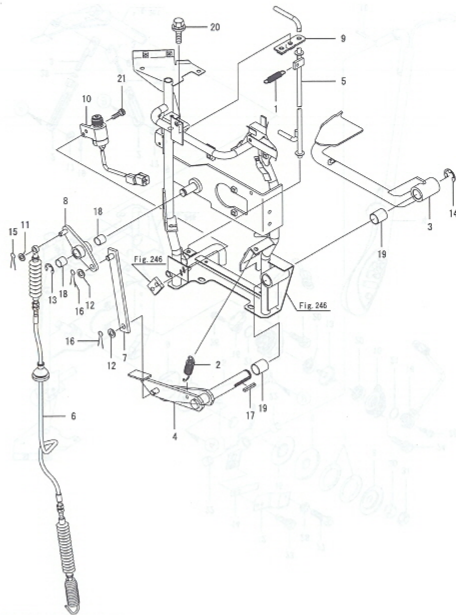
Fig.251. 브레이크조작
