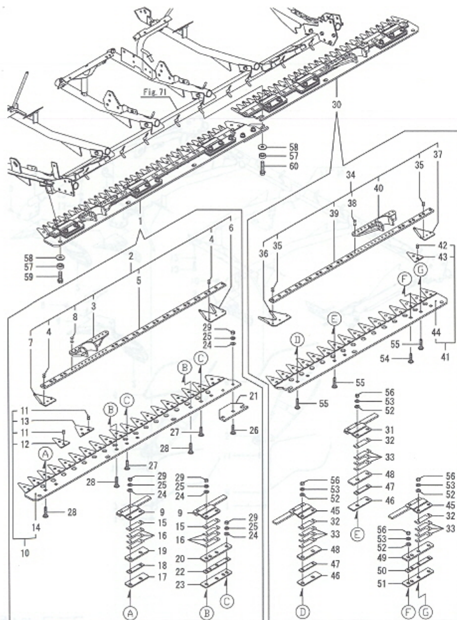
Fig.75. 예취날
