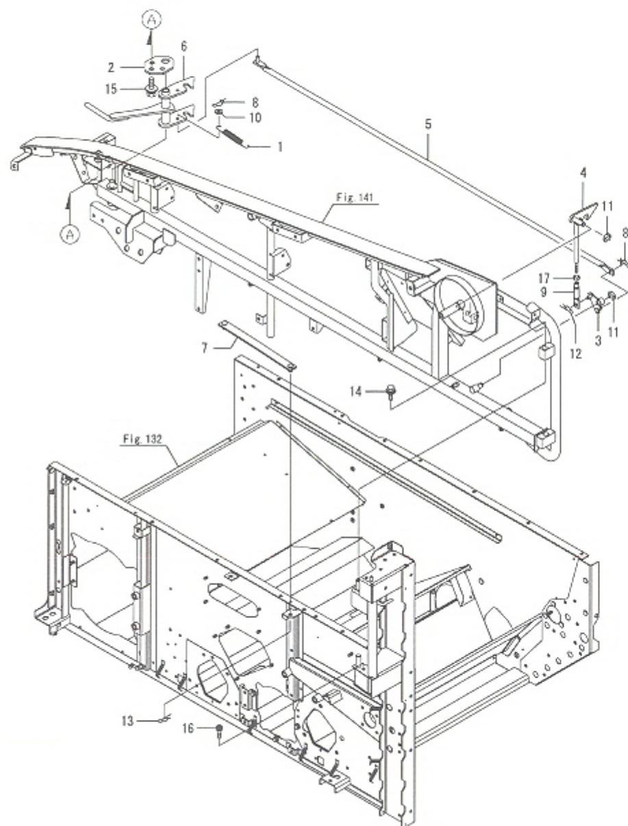
Fig.142. 탈곡실프레임(좌)(2)
