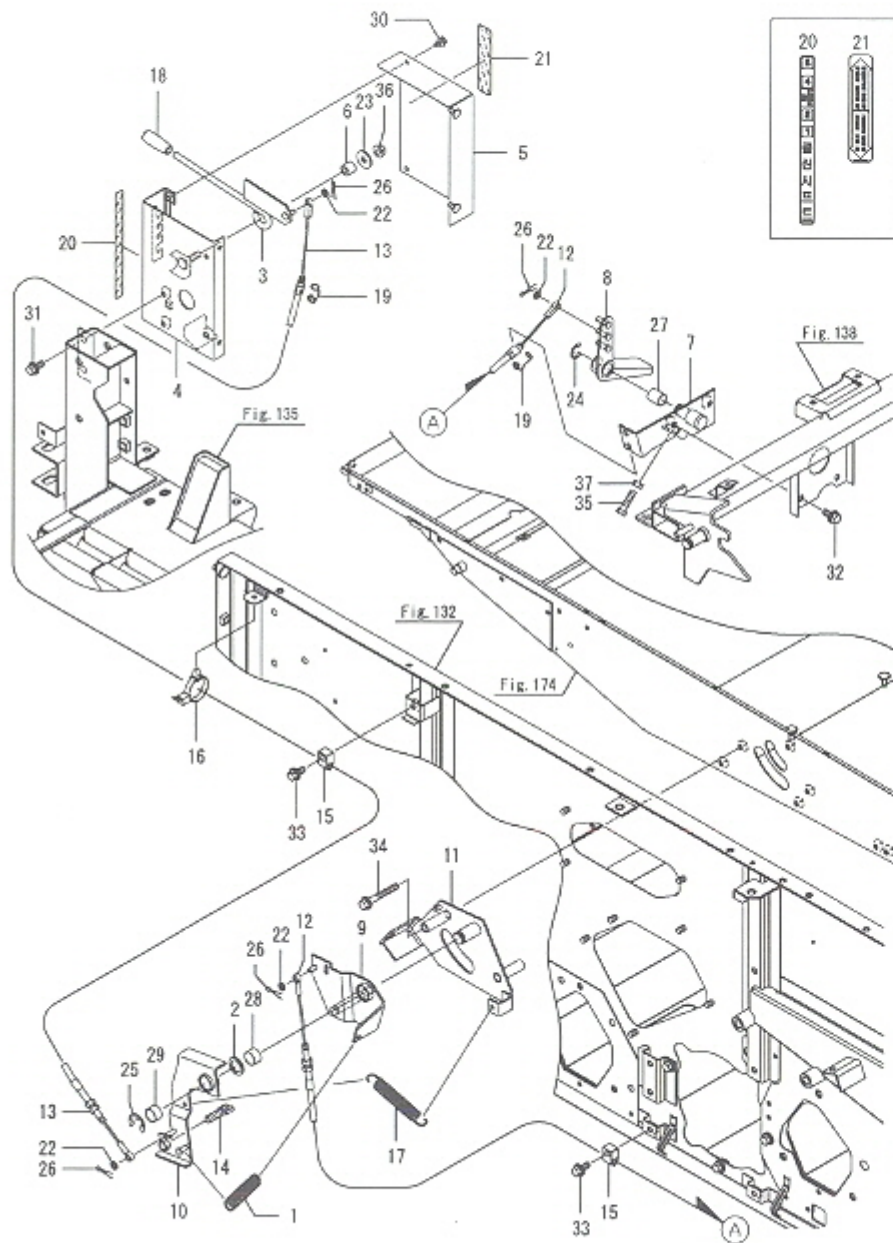
Fig.176. 요동선별조작
