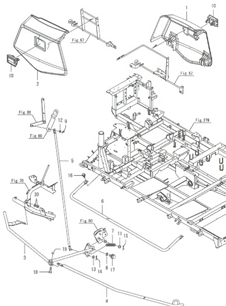
Fig.17. 예취(캐빈)(2)
