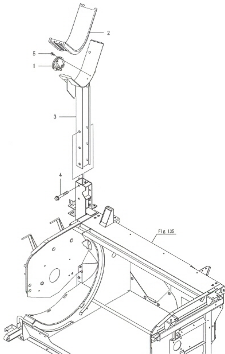
Fig.354. 오거 받침
