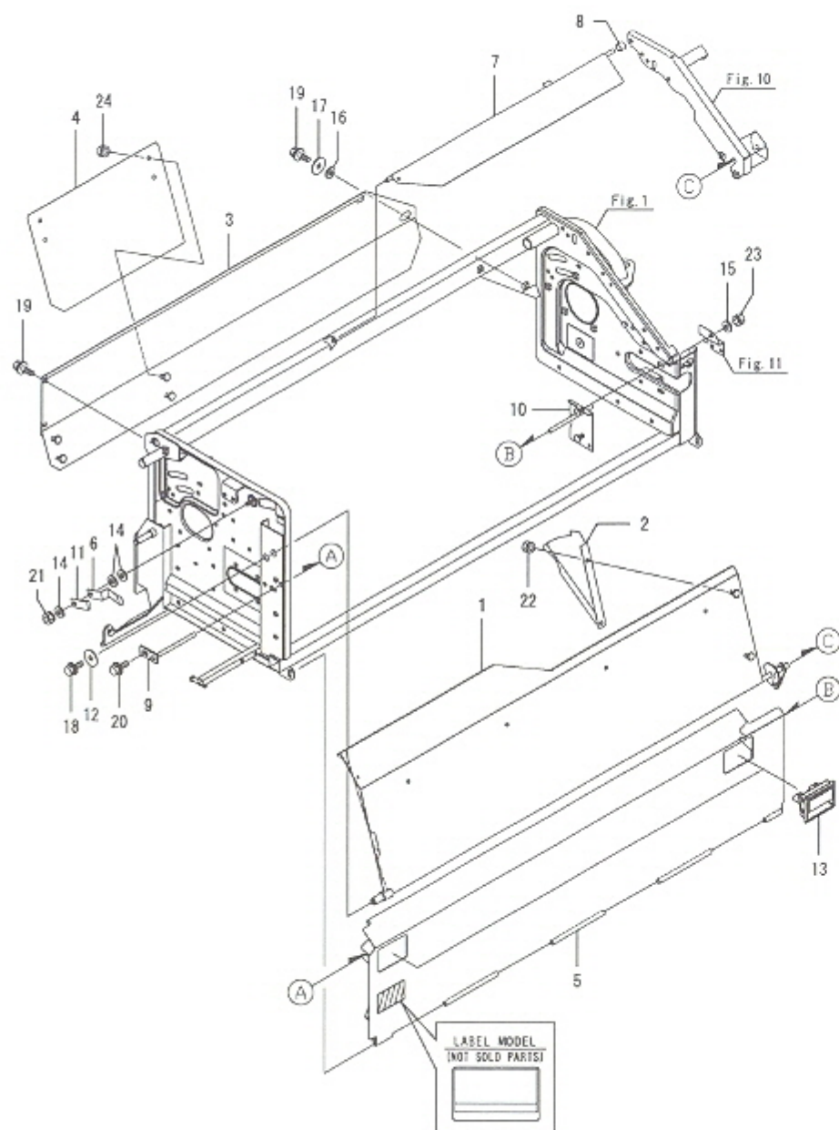
Fig.7. 본체커버
