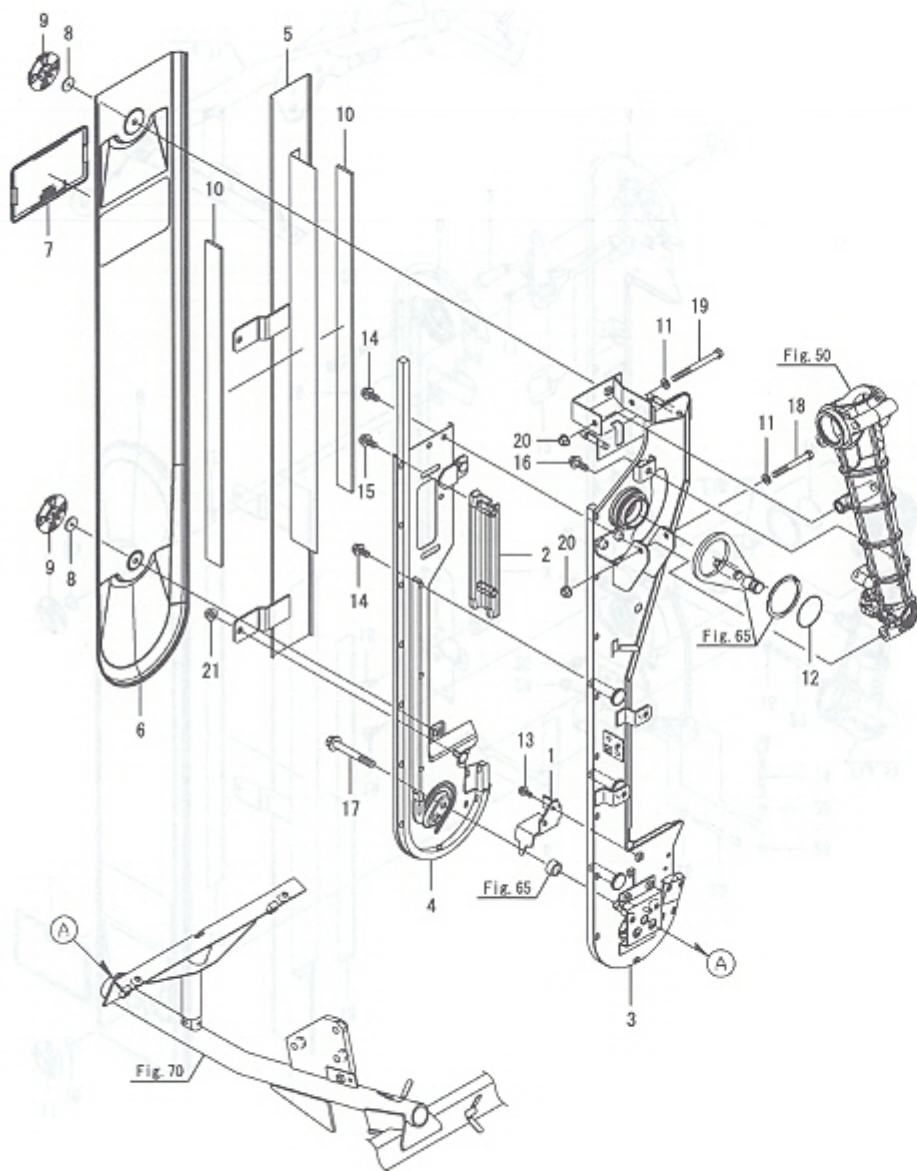
Fig.60. 인기케이스(중-좌)
