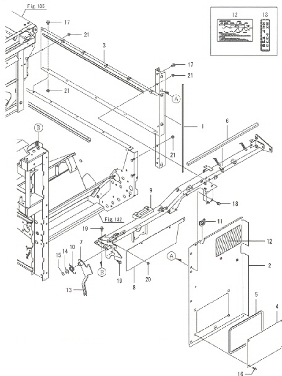
Fig.138. 상부본체(뒤)
