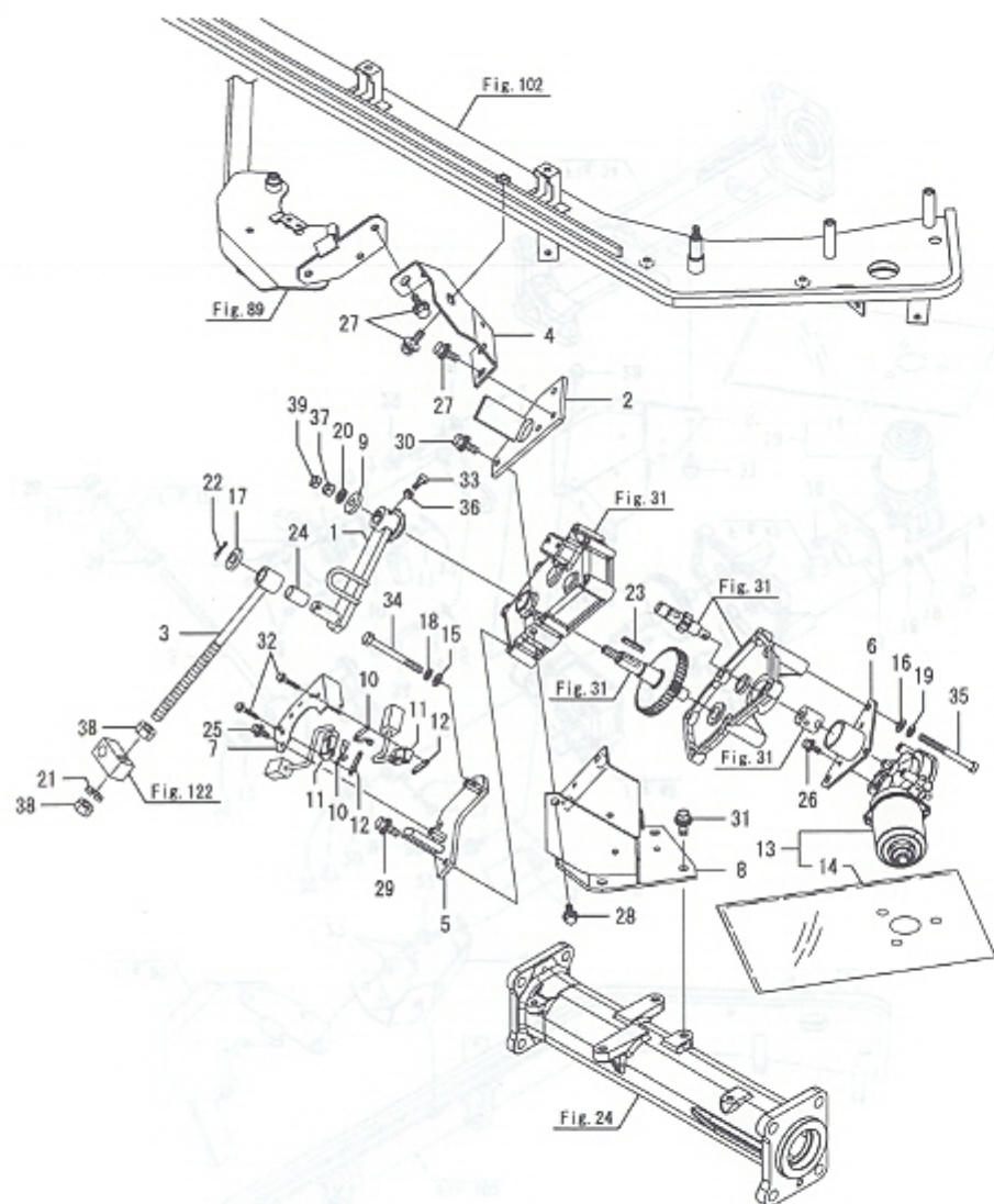
Fig.129. 탈곡깊이조절
