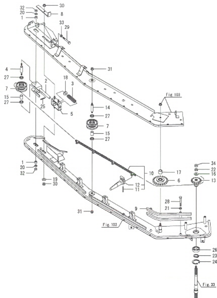
Fig.108. 상반승롤러(우)
