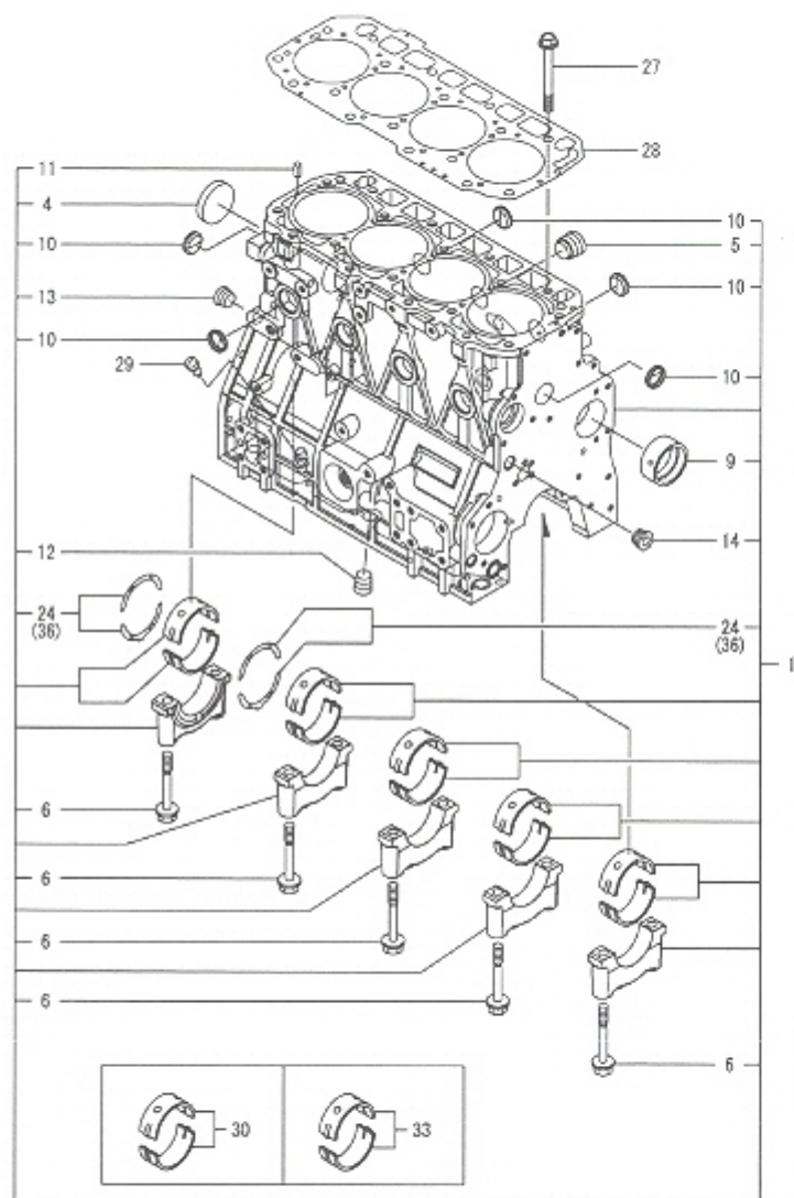
Fig.1. 실린더블럭
