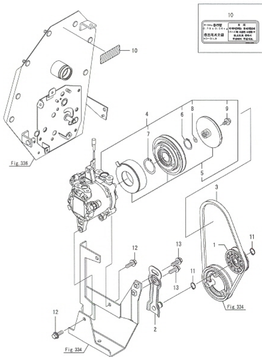
Fig.318. 콤프레셔취부
