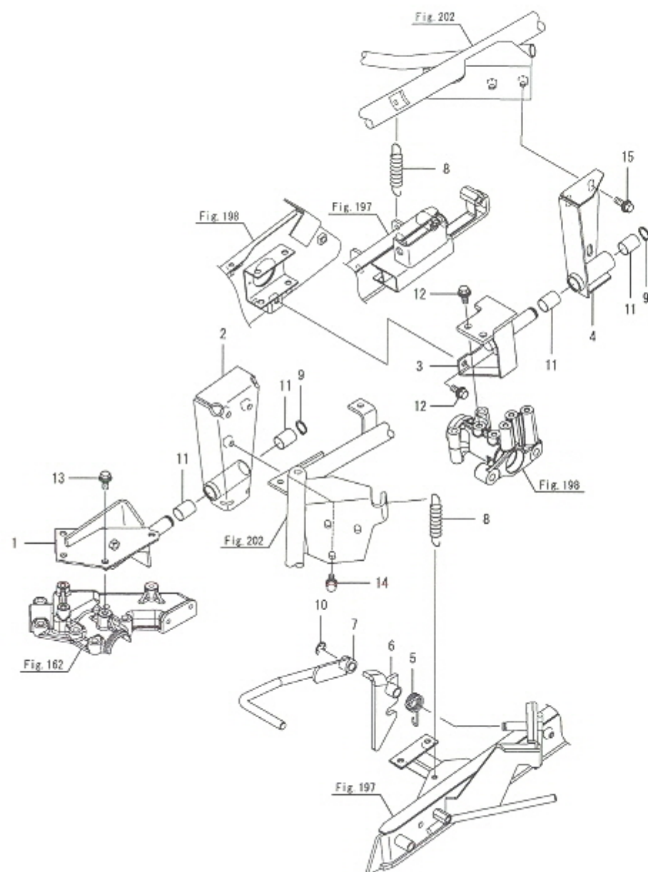
Fig.204. 짚배출오픈
