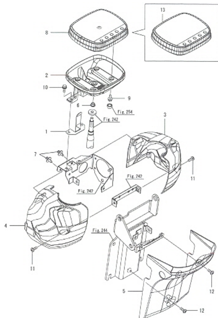
Fig.250. 전면 칼럼
