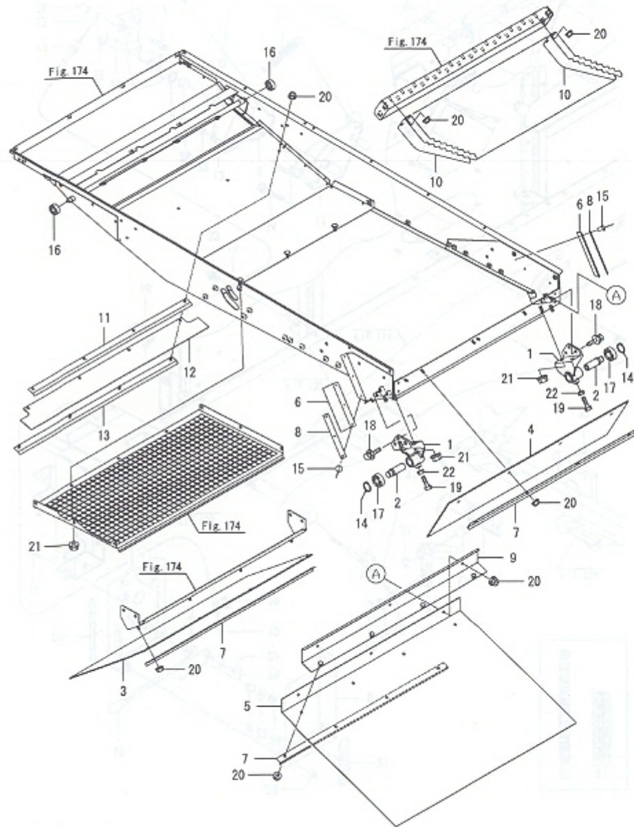
Fig.175. 스윙(3)
