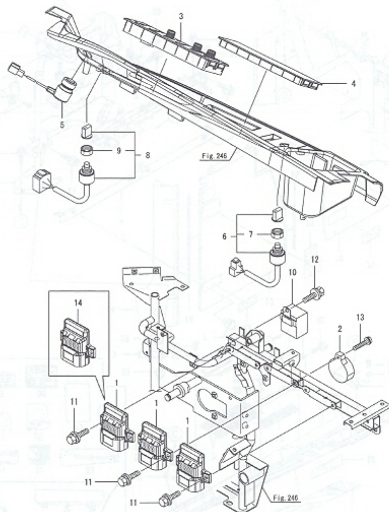
Fig.247. 사이드칼럼(2)
