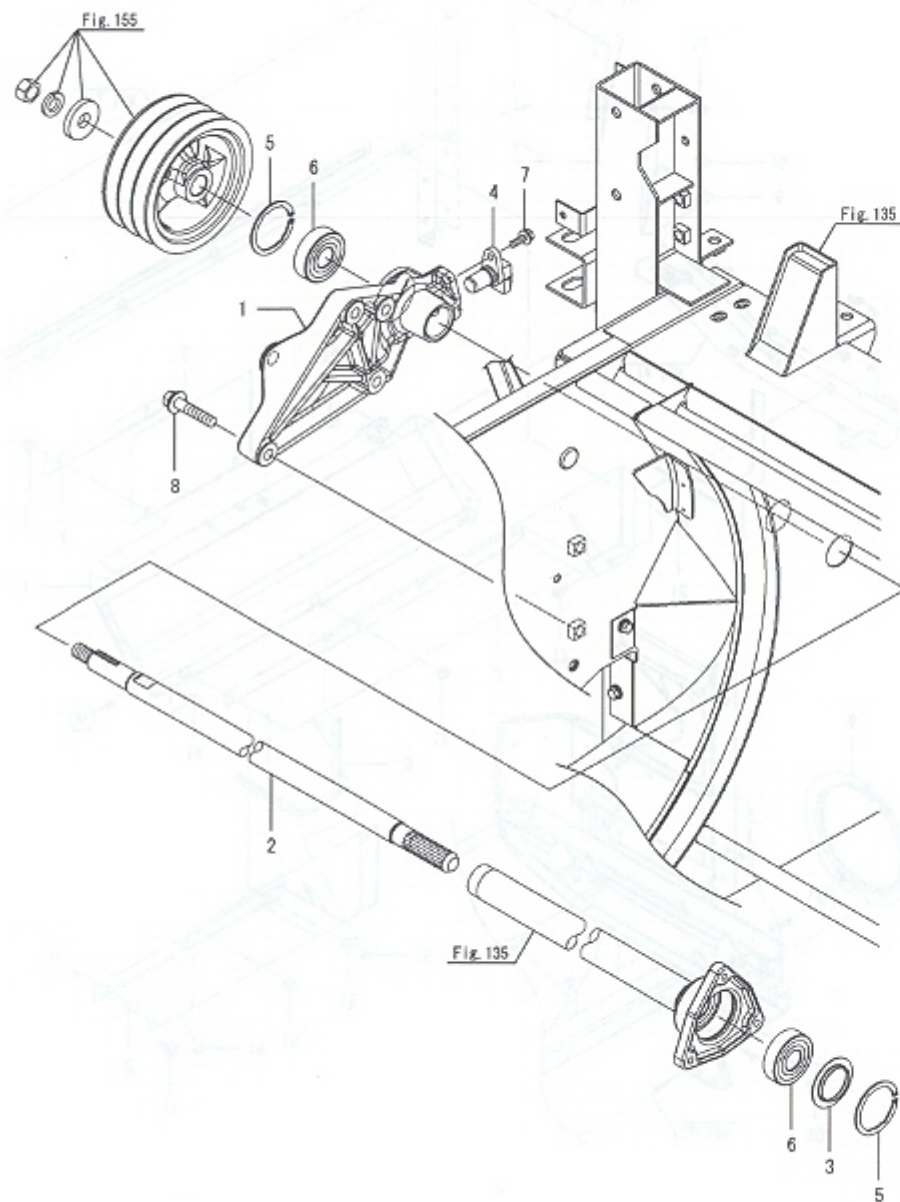
Fig.169. 처리 드럼 드라이브 축
