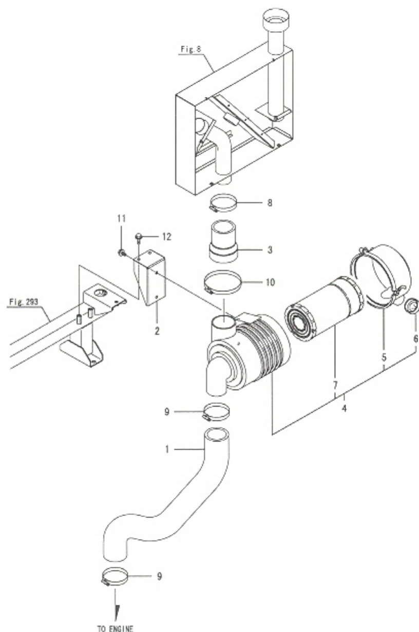
Fig.6. 에어클리너
