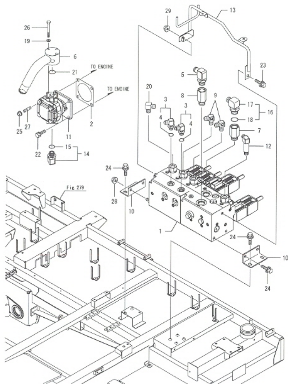
OCNP6-M03670 이동(2) Fig.256. 유압밸브
