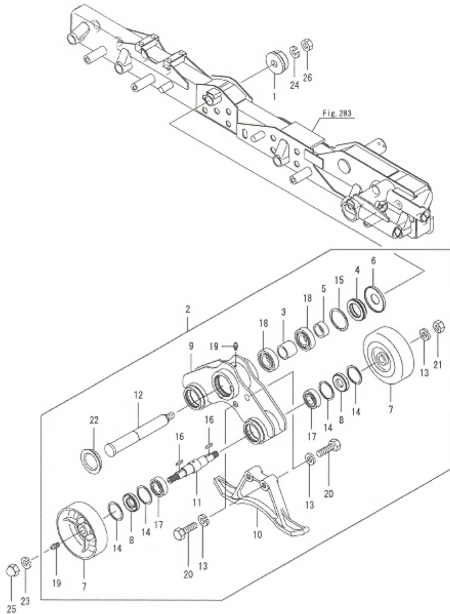
Fig.286. 이퀄라이저
