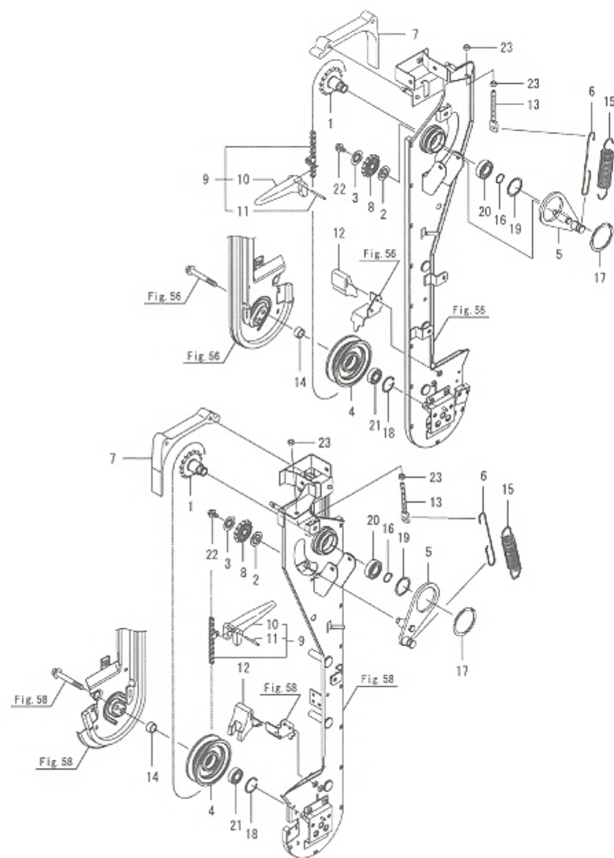
Fig.65. 인기체인롤러
