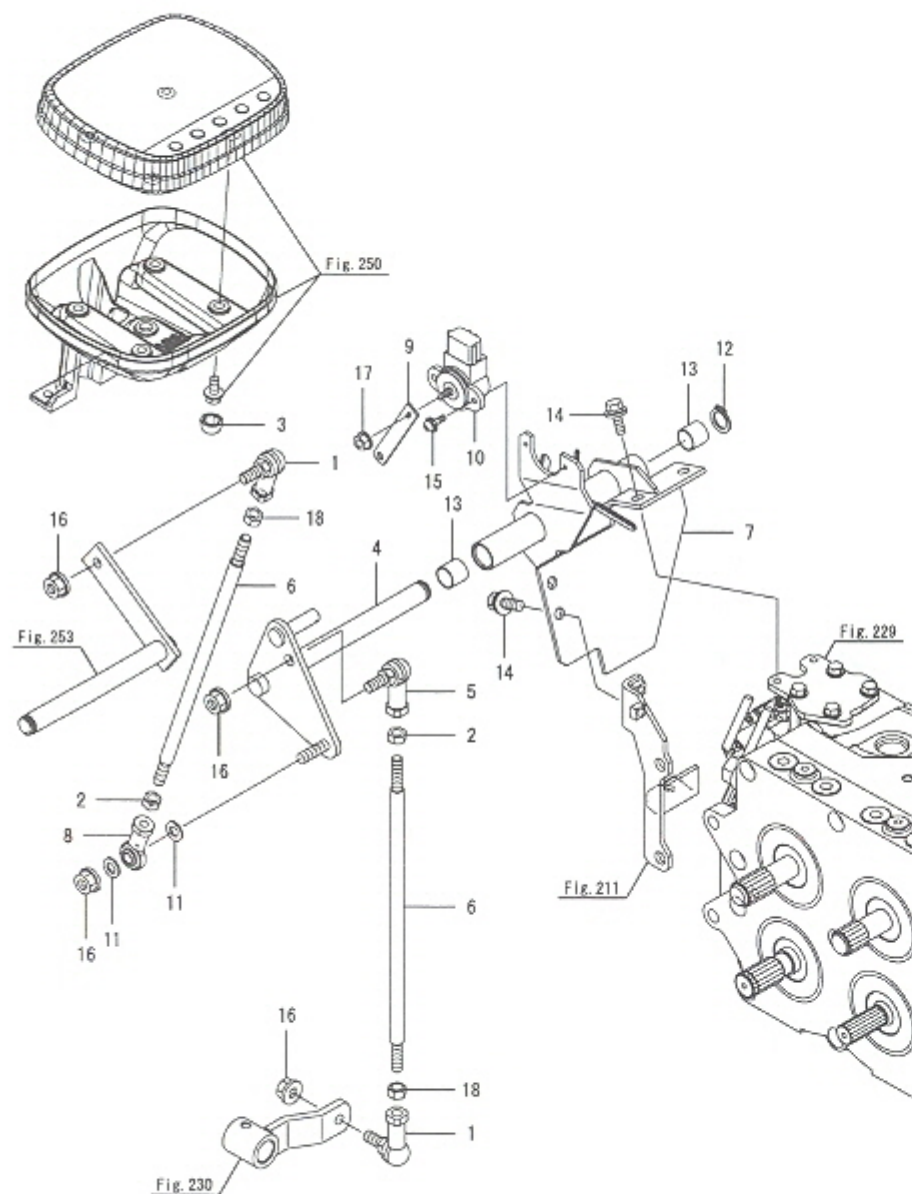
Fig.254. 부변속(2)
