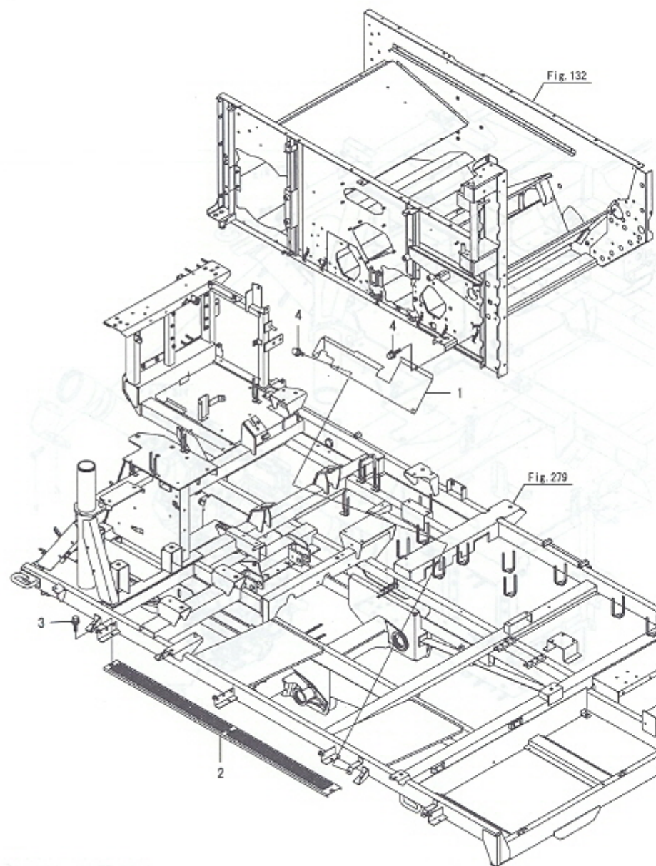
Fig.281. 머드가이드
