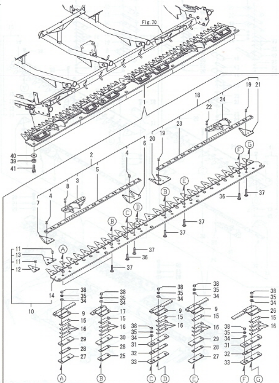
Fig.74. 예취날
