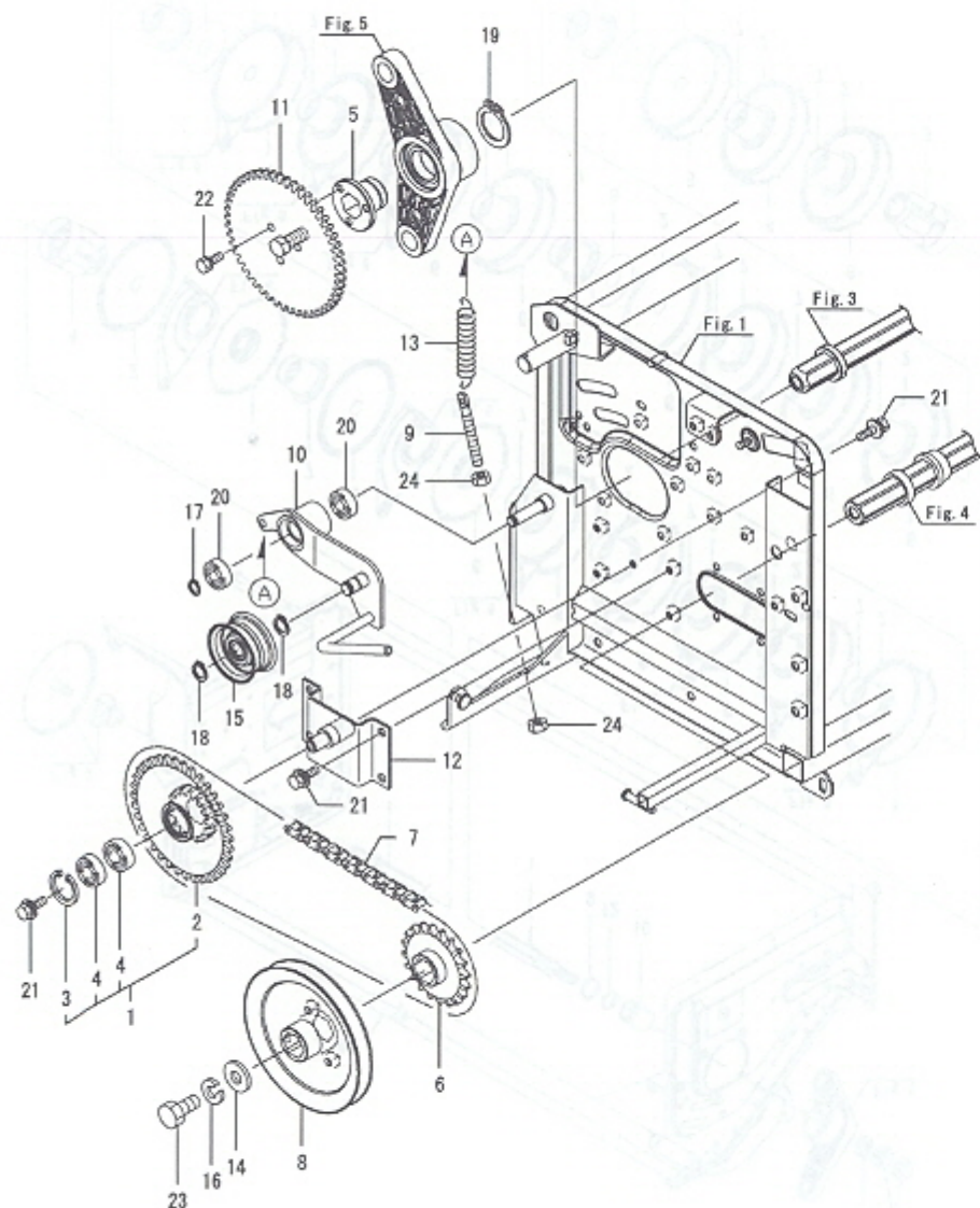
Fig.2. 구동
