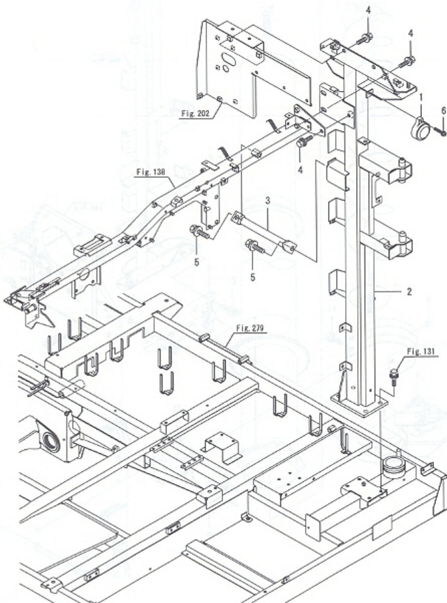
Fig.339. 종오거프레임
