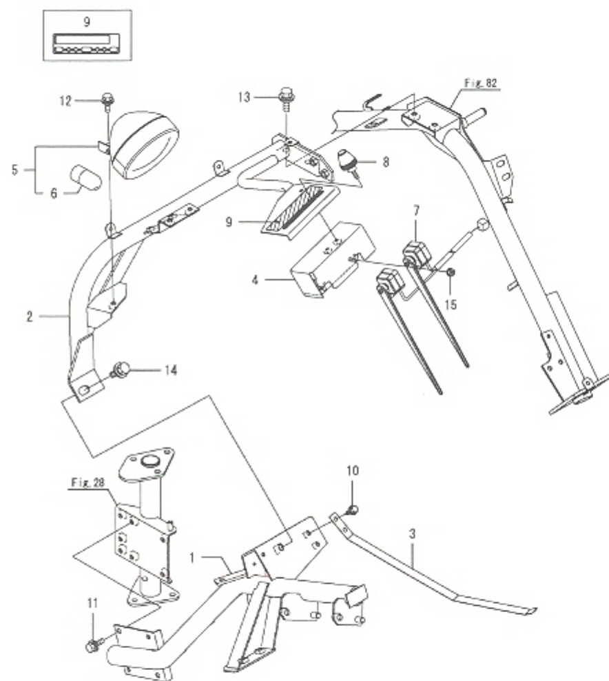
Fig.126. 보조반송프레임
