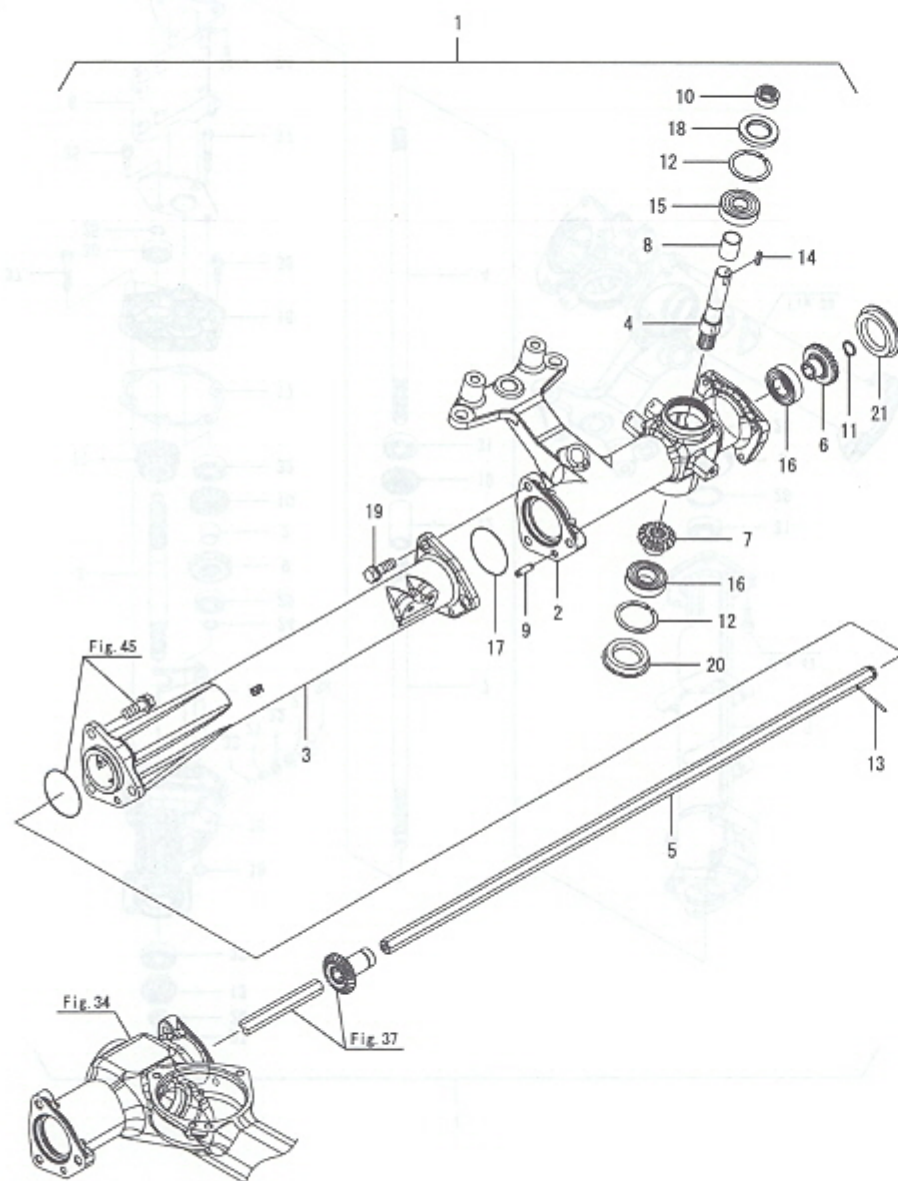
Fig.38. 5드라이브 케이스(7)
