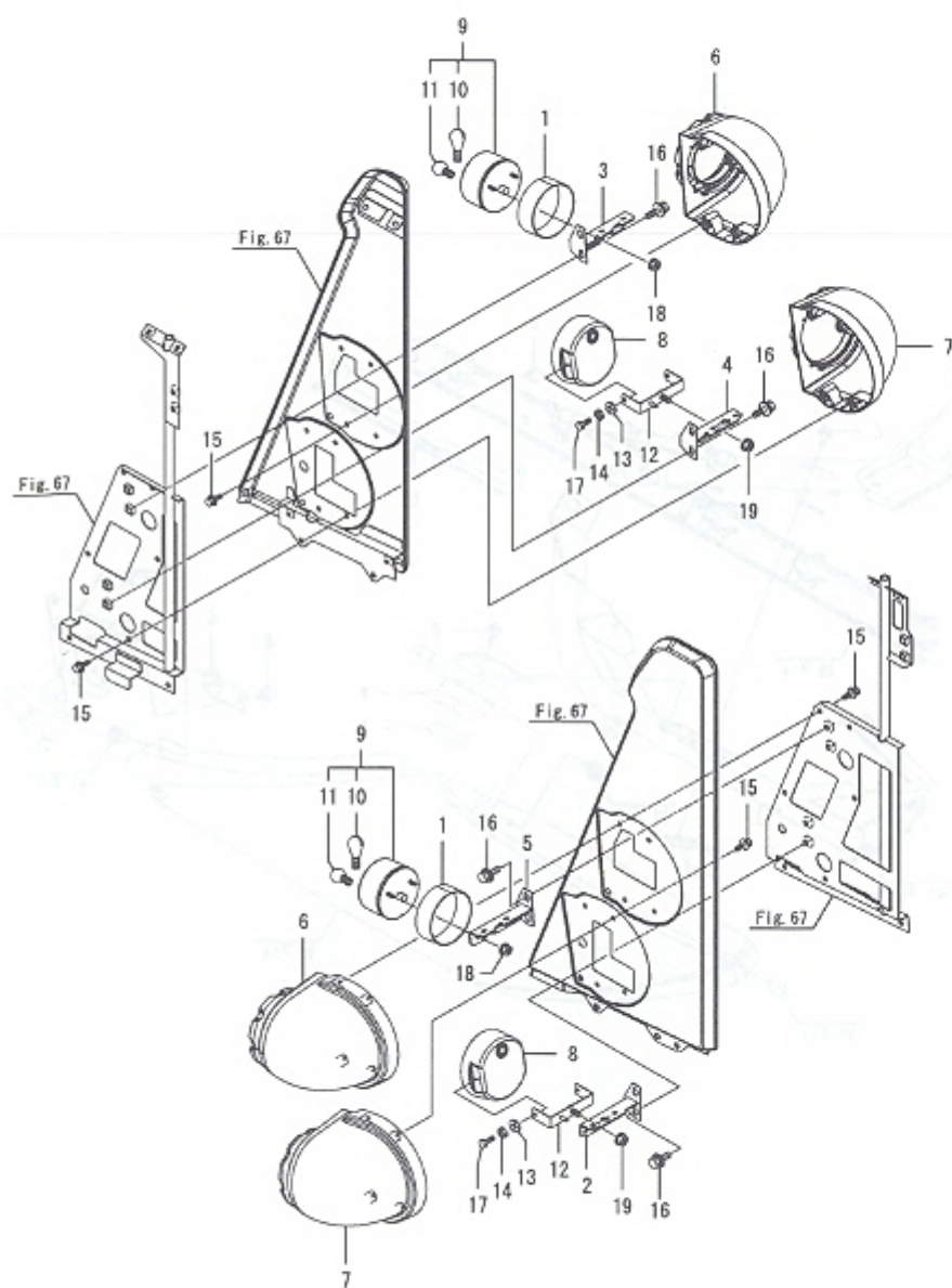
Fig.68. 예취커버(2)
