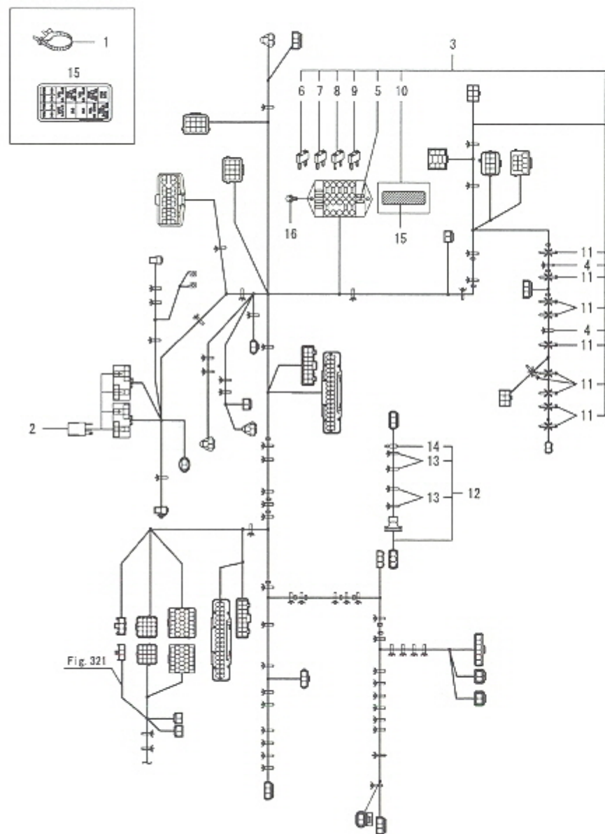
Fig.328. 배선(탈곡)
