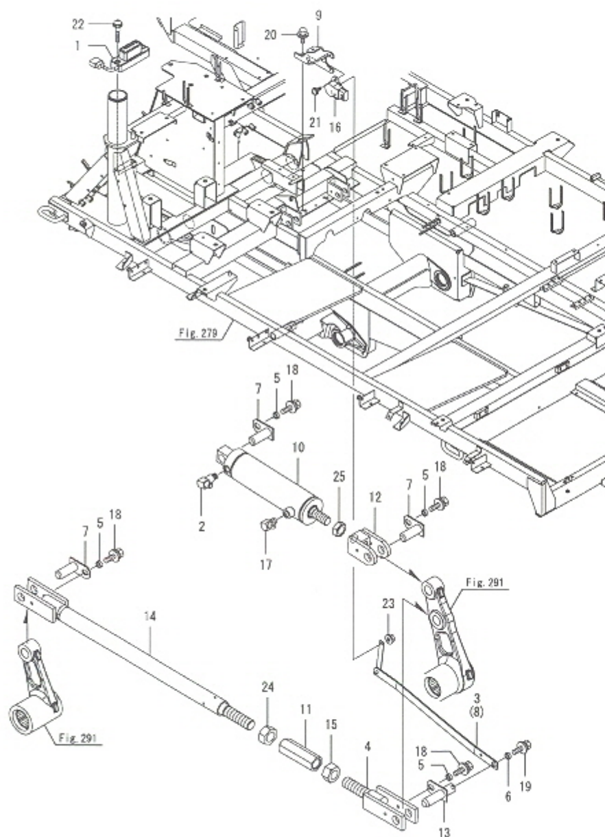
Fig.292. 스윙(2)
