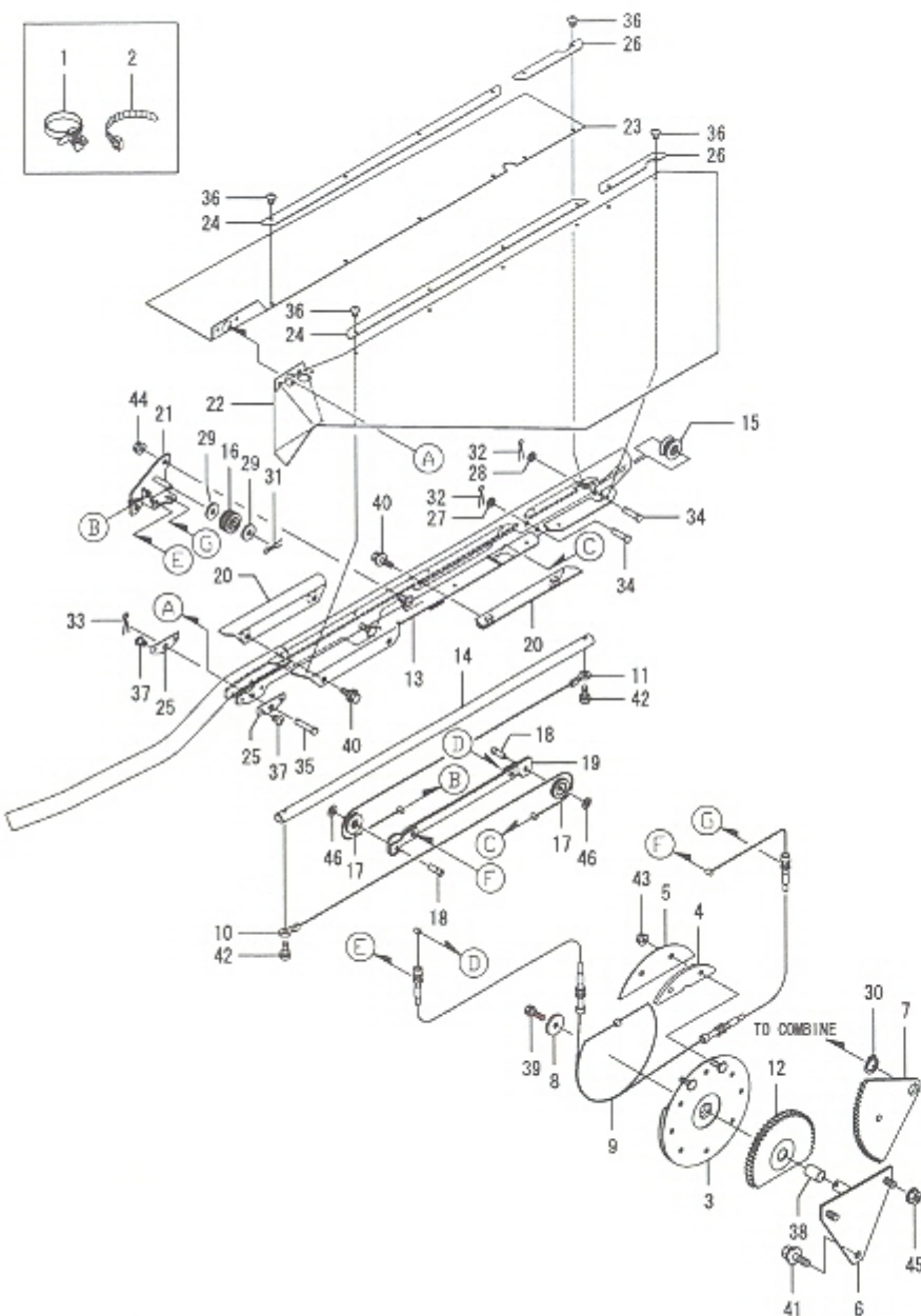
Fig.1. 짐배출가이드
