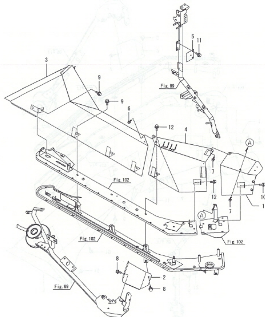
Fig.113. 상단 이송 가이드(오른쪽)
