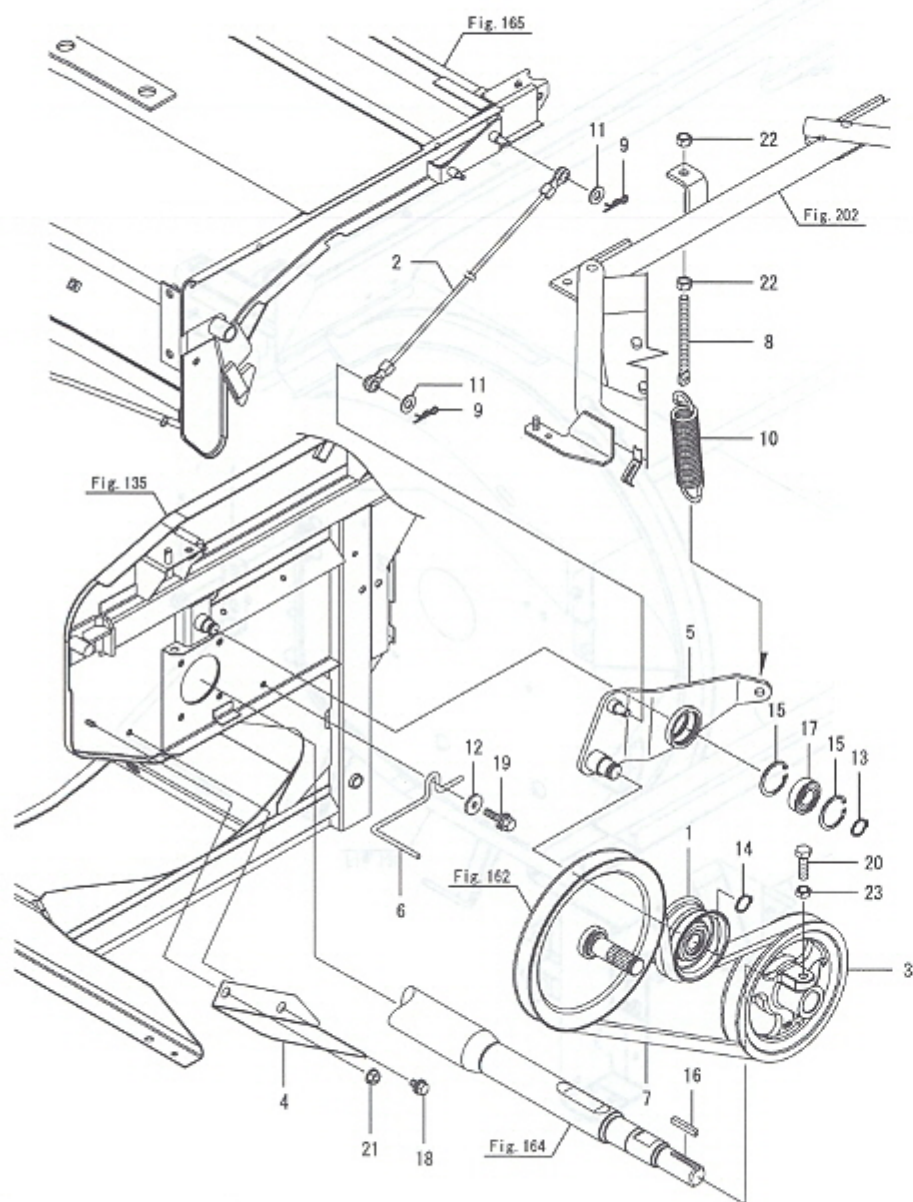
Fig.157. 짚 방출 벨트
