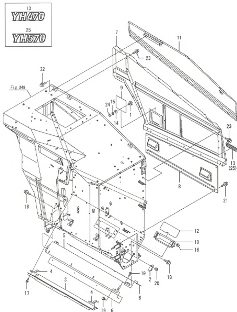
Fig.350. 곡물탱크(캐빈)(2)
