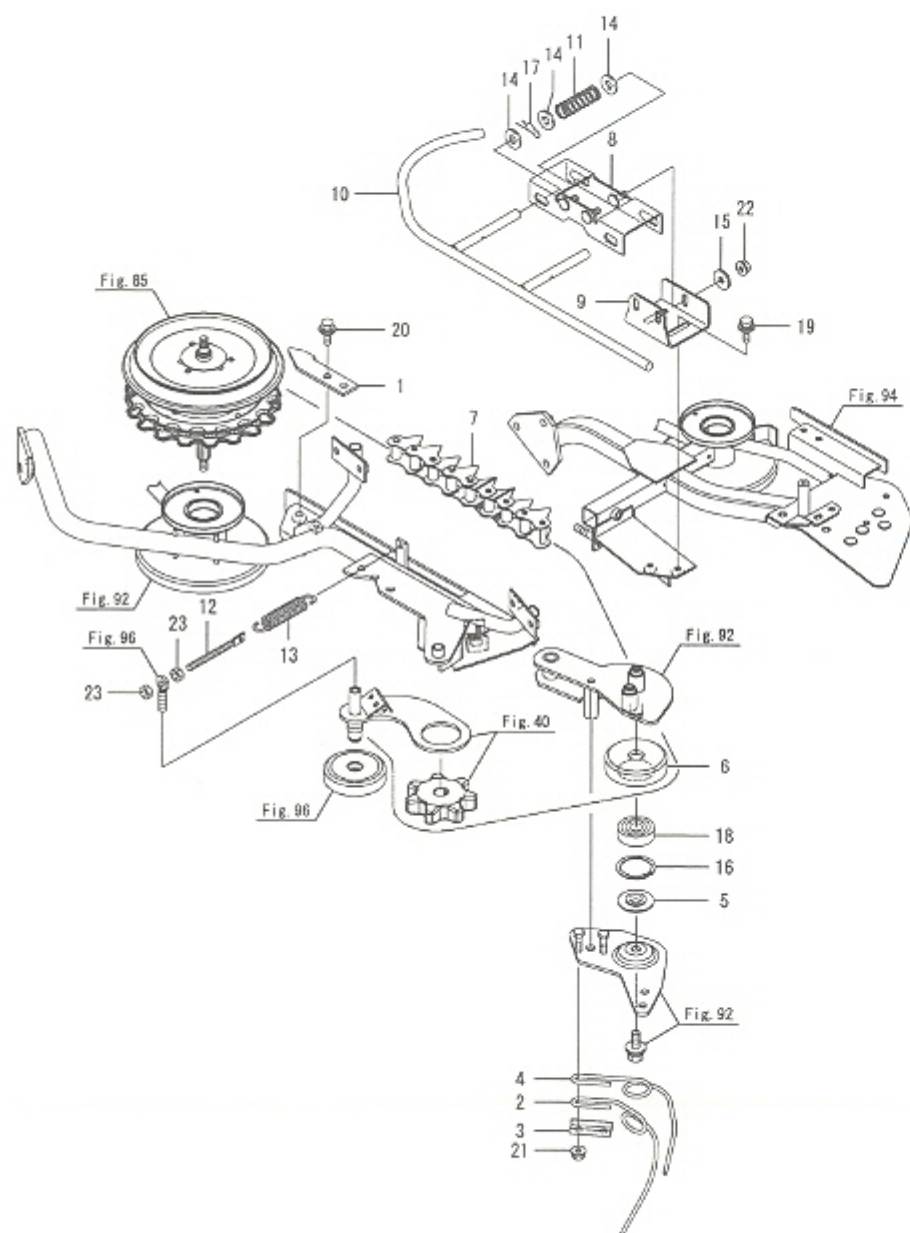
Fig.100. 하단 이송 가이드(왼쪽)
