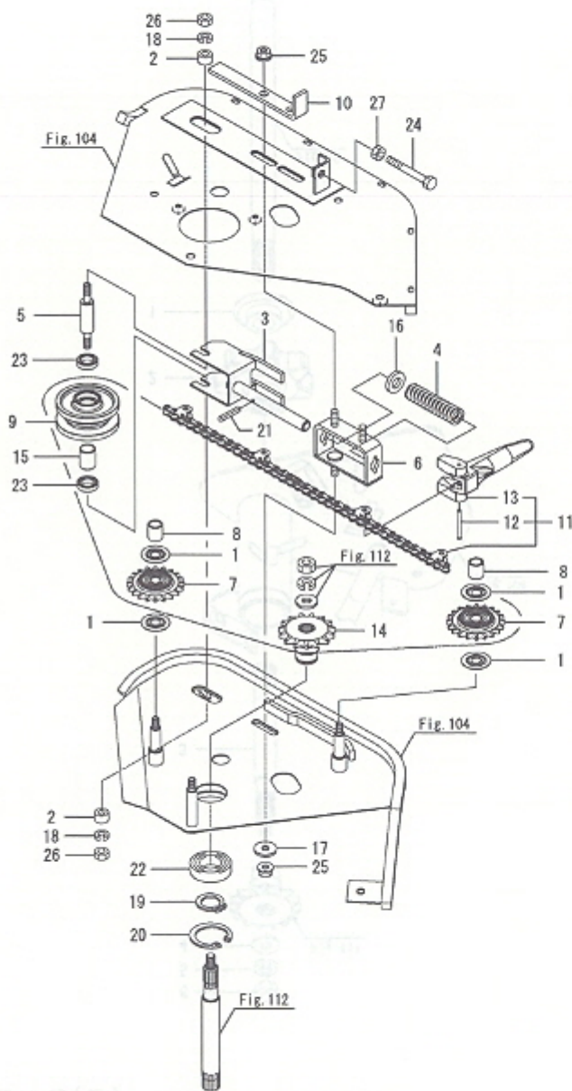
Fig.111. 상반송롤러(중)
