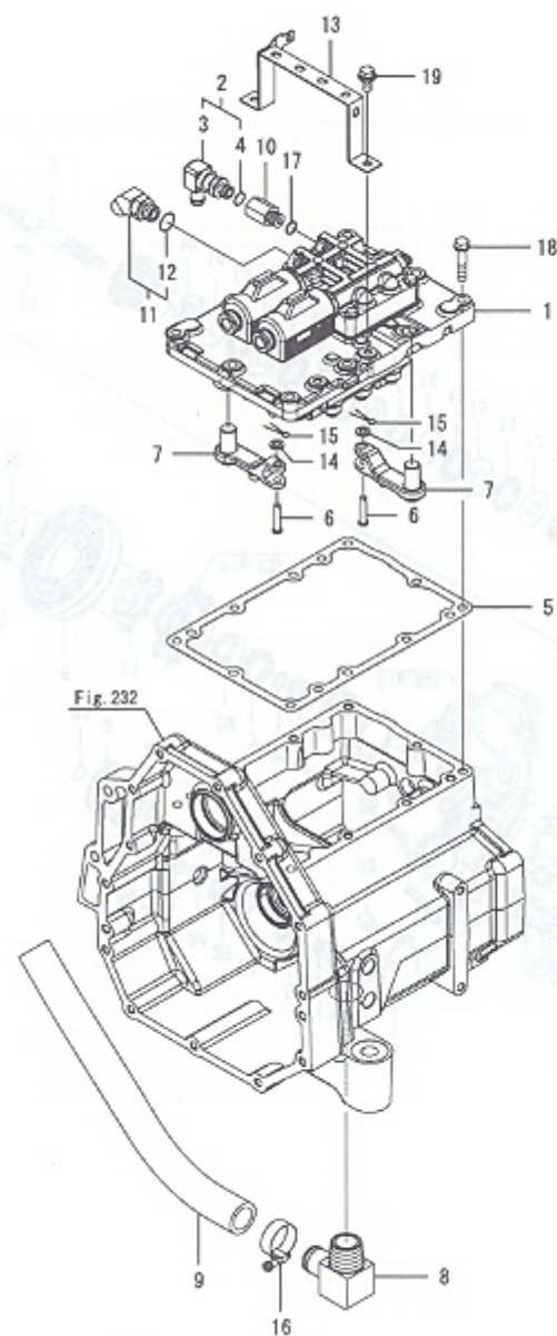
Fig.233. 카운터케이스(2)
