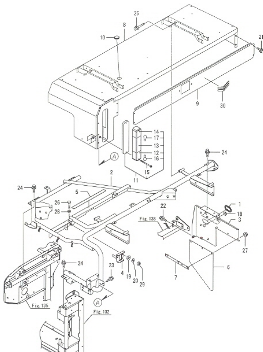
Fig.202. 짚배출(상)
