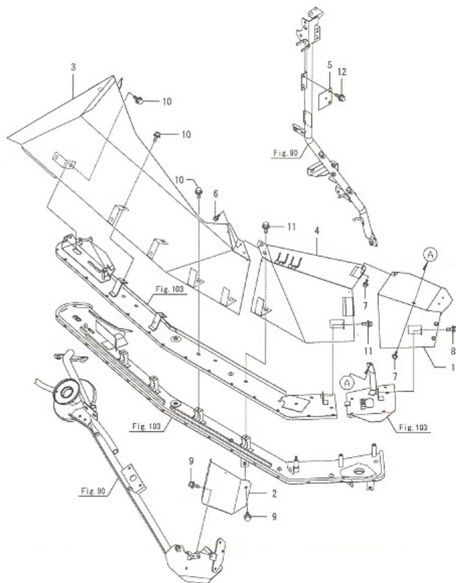
Fig.114. 상단 이송 가이드(오른쪽)
