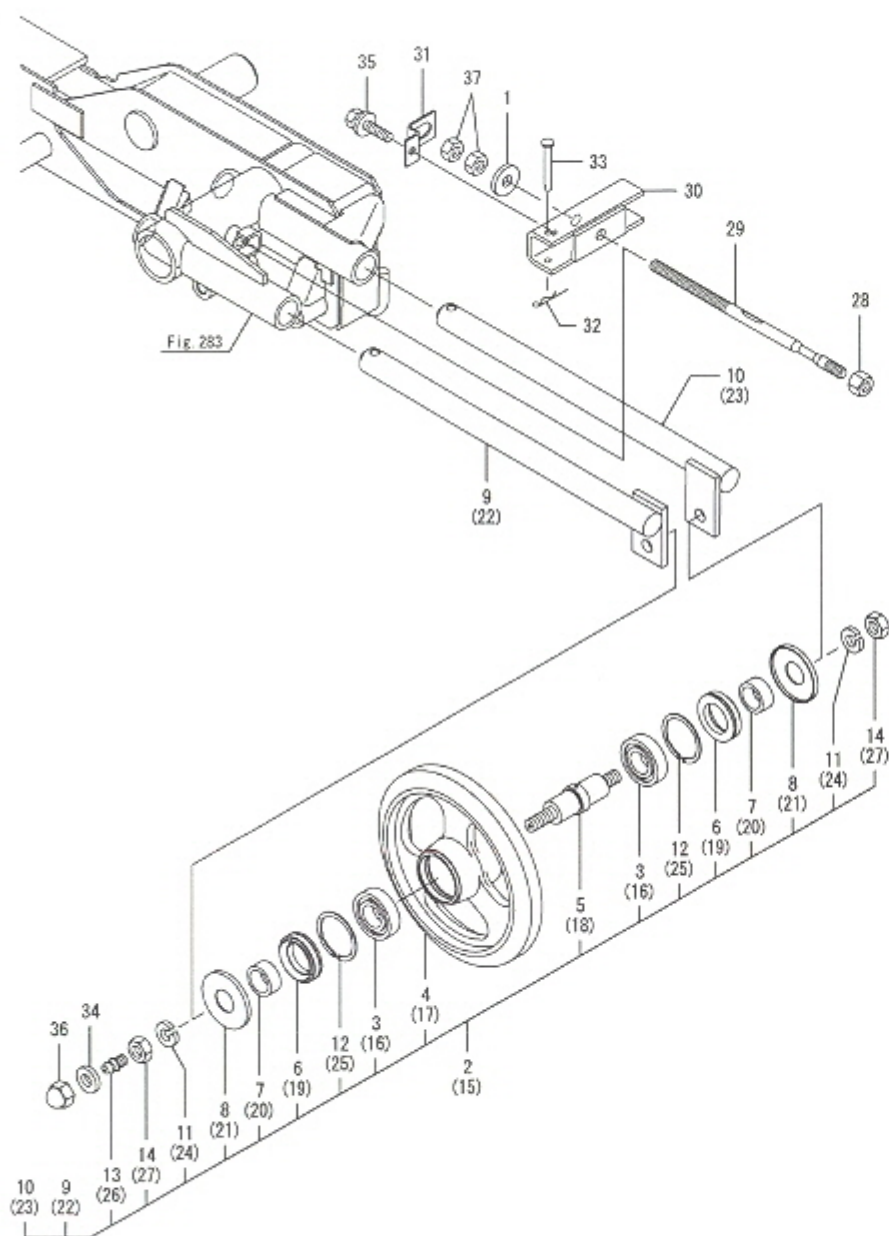
Fig.284. 아이들러
