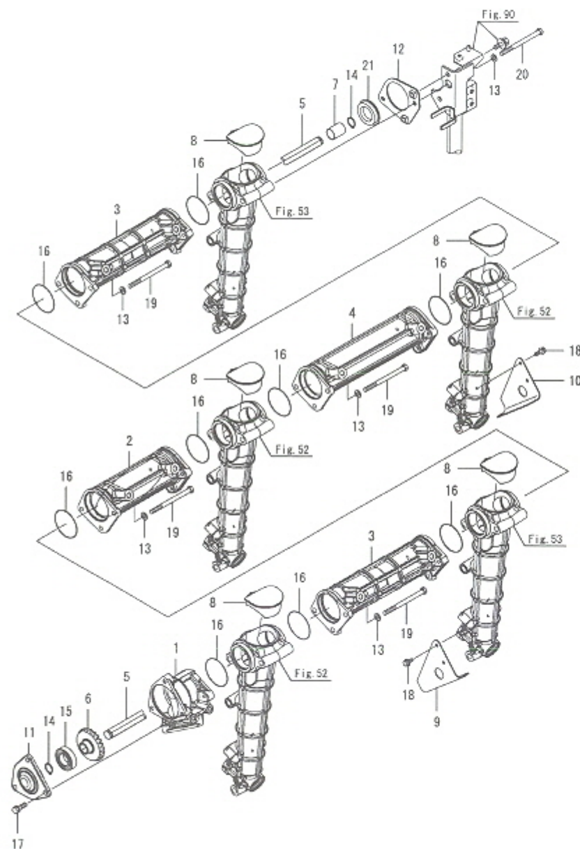
Fig.51. 인기힐구동(1)
