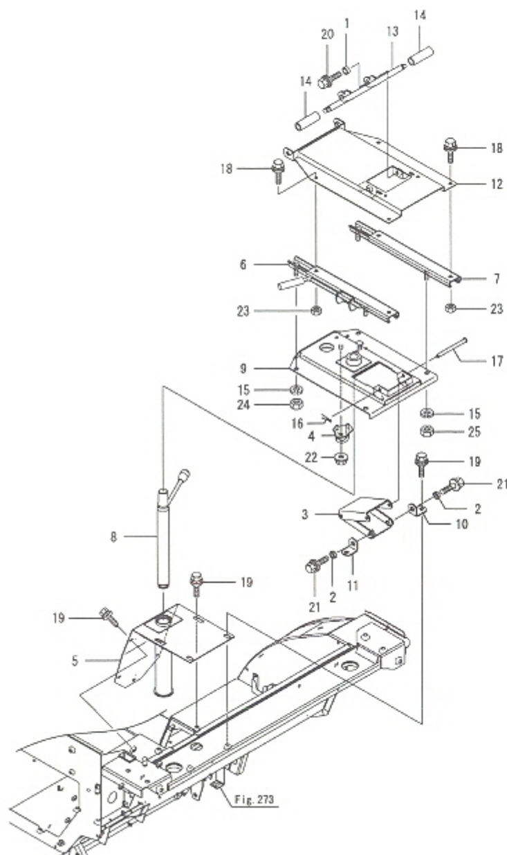
OCNP6-M03670 이동(2) Fig.272. 시트틸트
