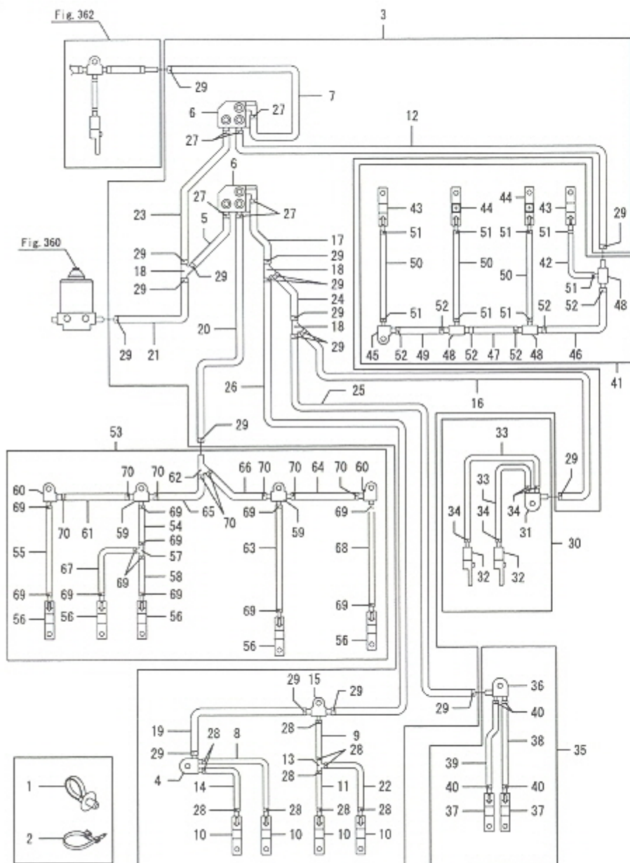
Fig.361. 주유장치(2)
