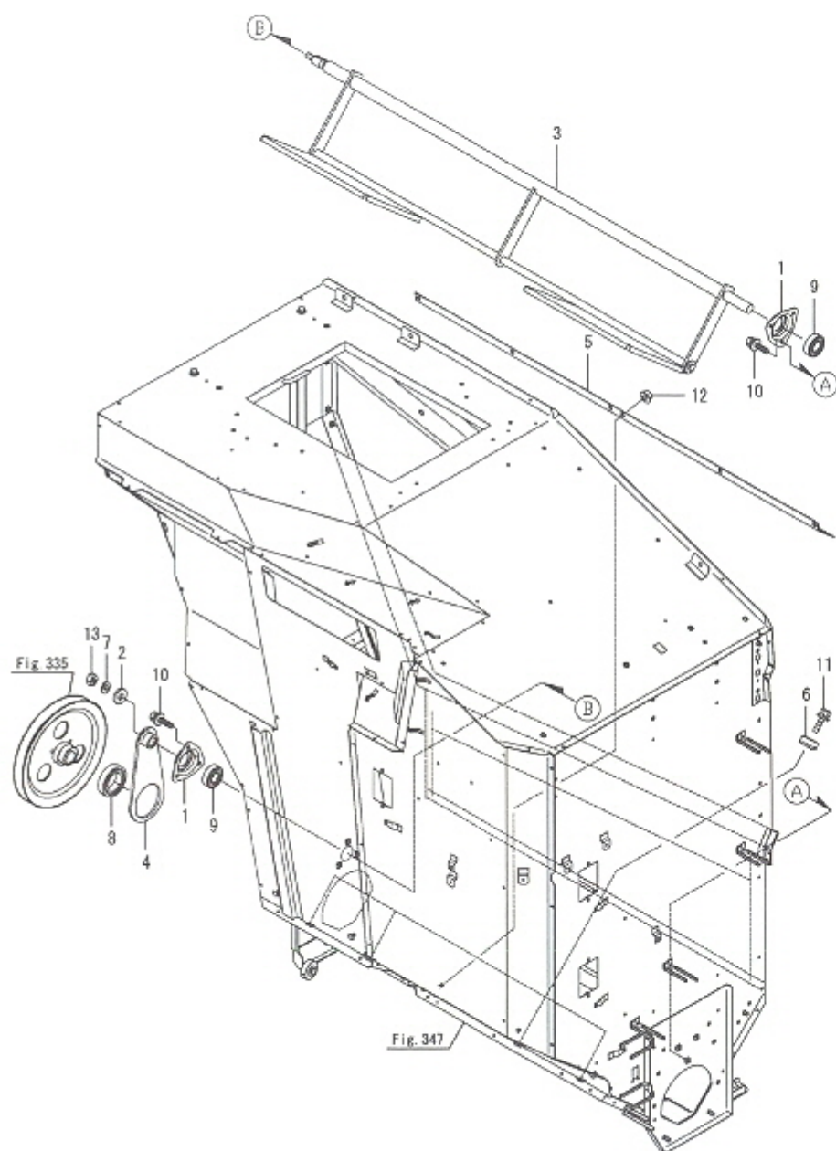
Fig.356. 요동바닥판
