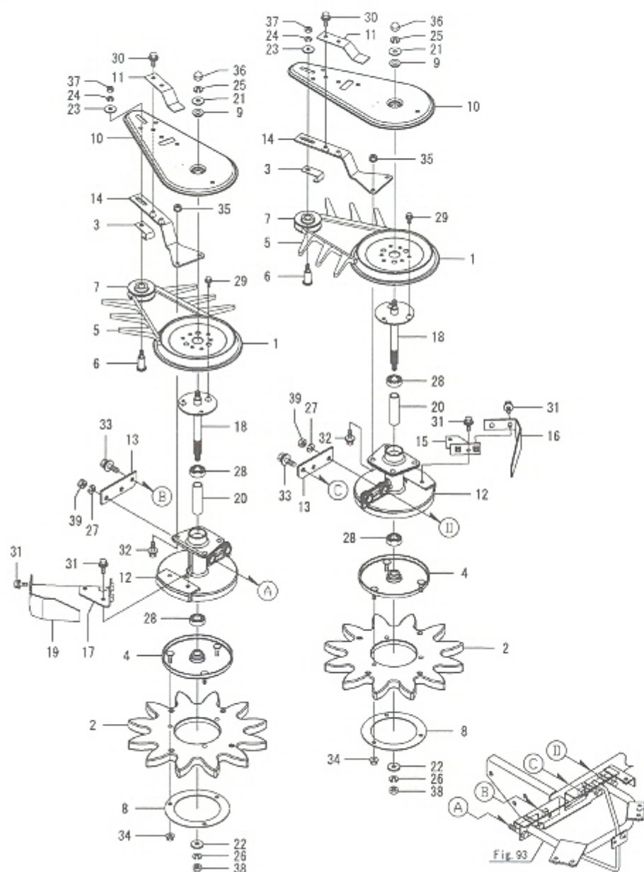
Fig.86. 스타휠(중)
