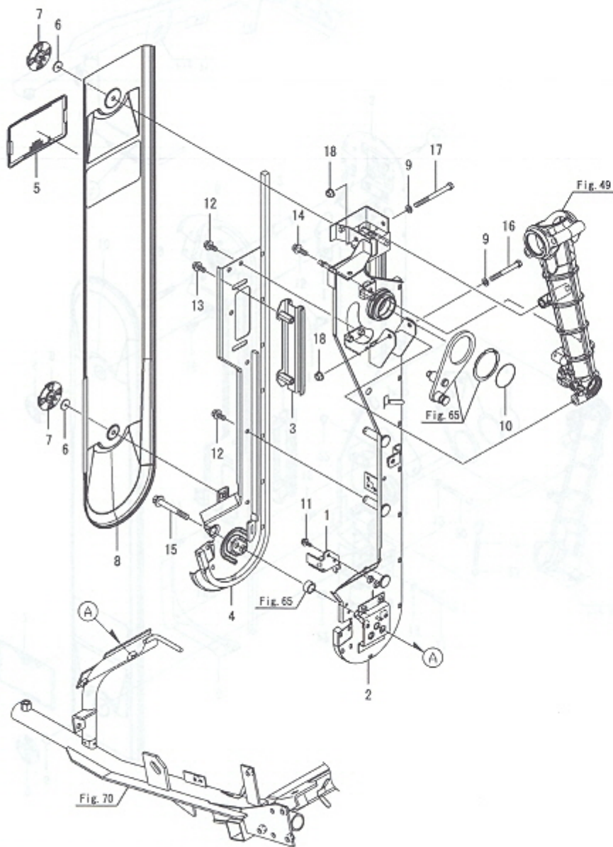
Fig.58. 픽업 케이스(왼쪽)
