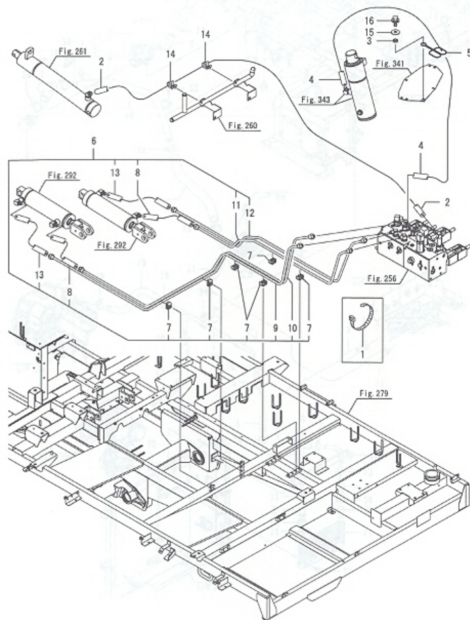
Fig.259. 배관(1)
