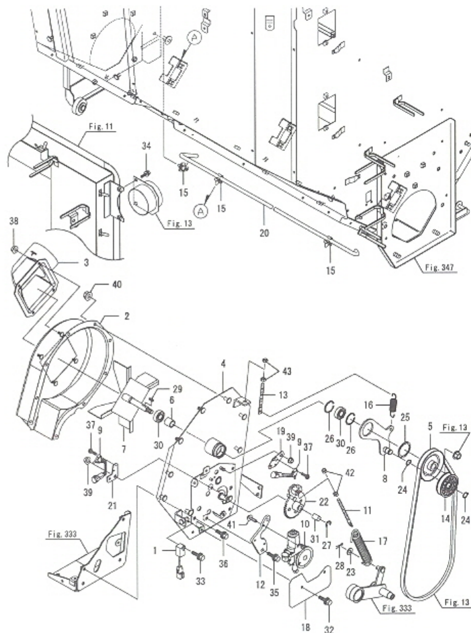
Fig.336. 오거 클러치
