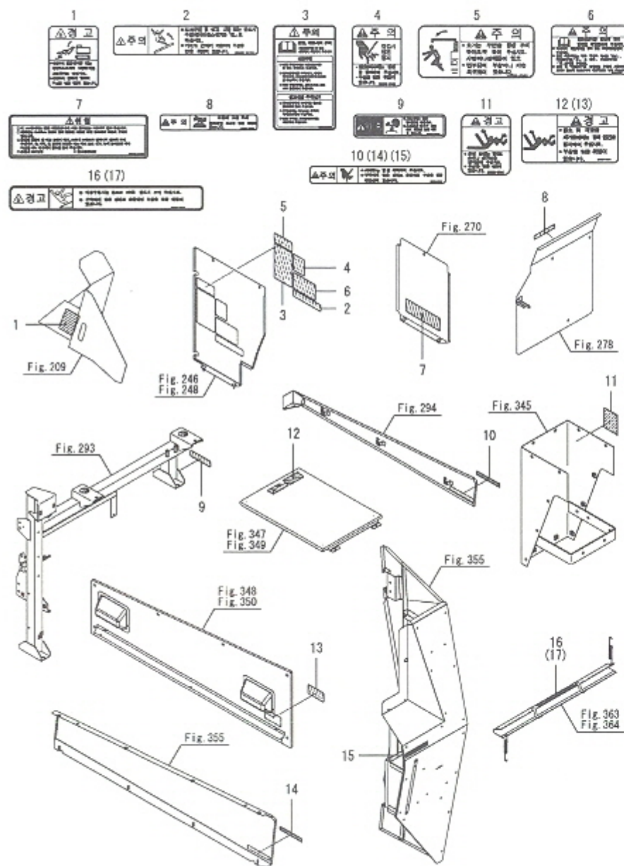
Fig.366. 명판(안전)(2)
