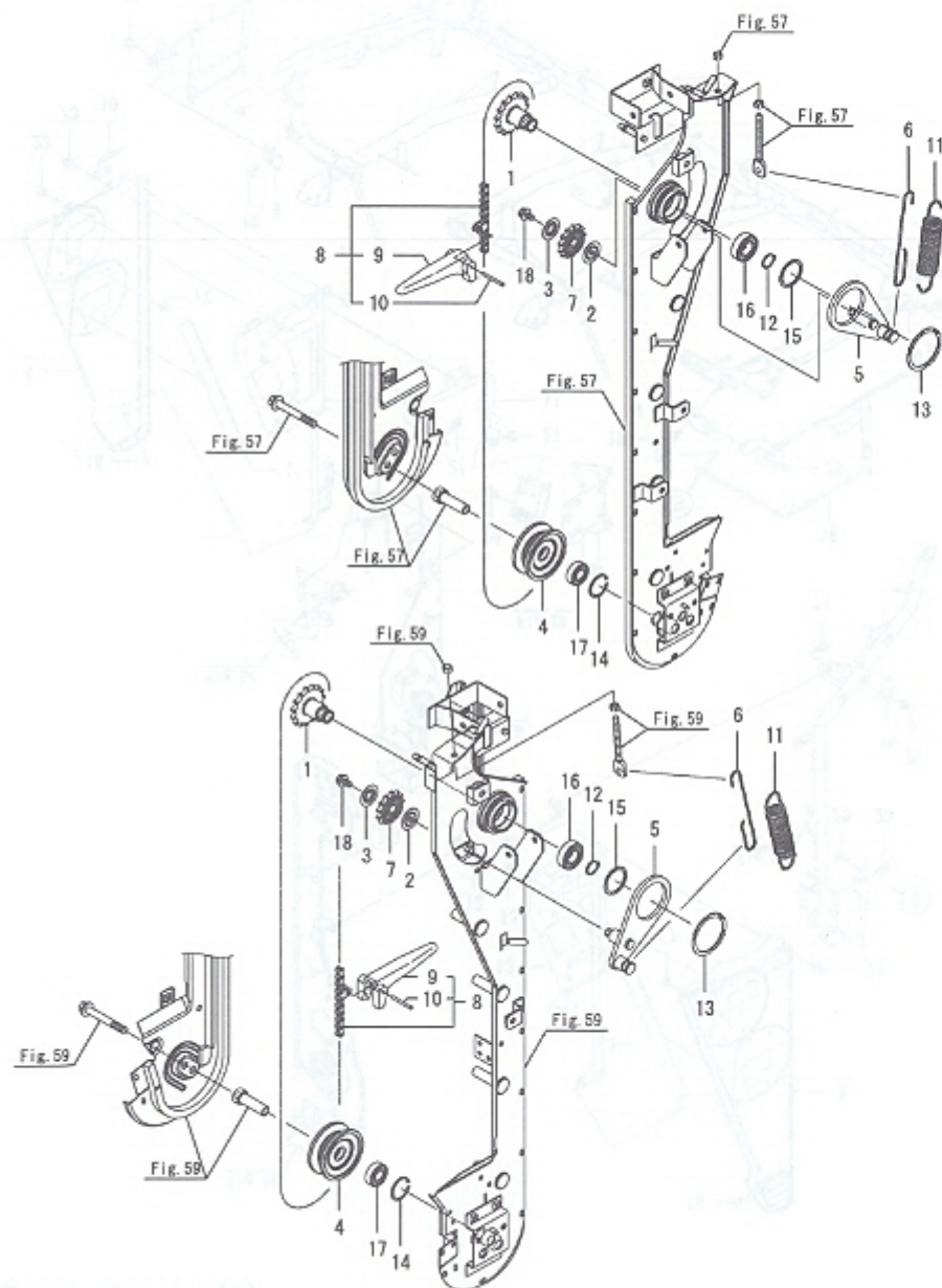
Fig.66. 인기체인롤러
