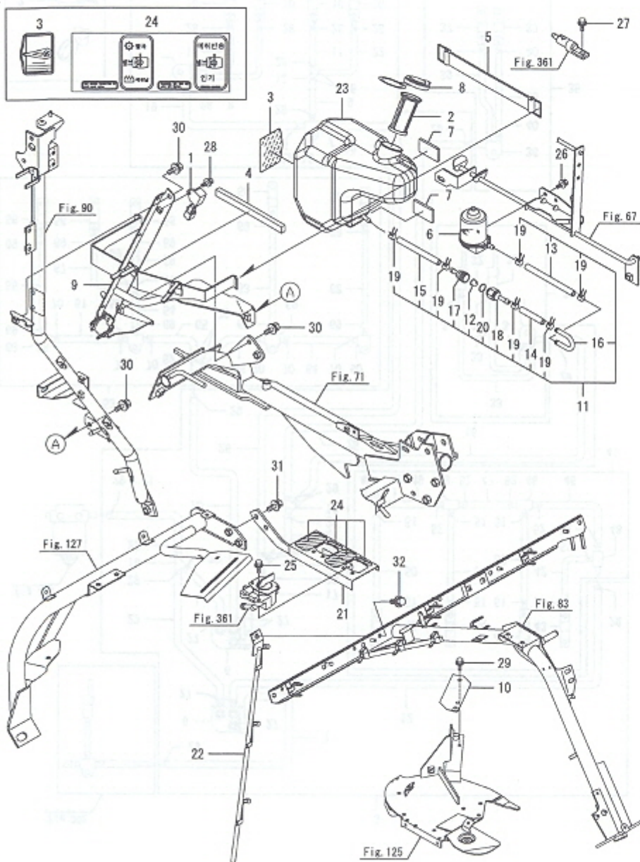
Fig.360. 주유장치(1)
