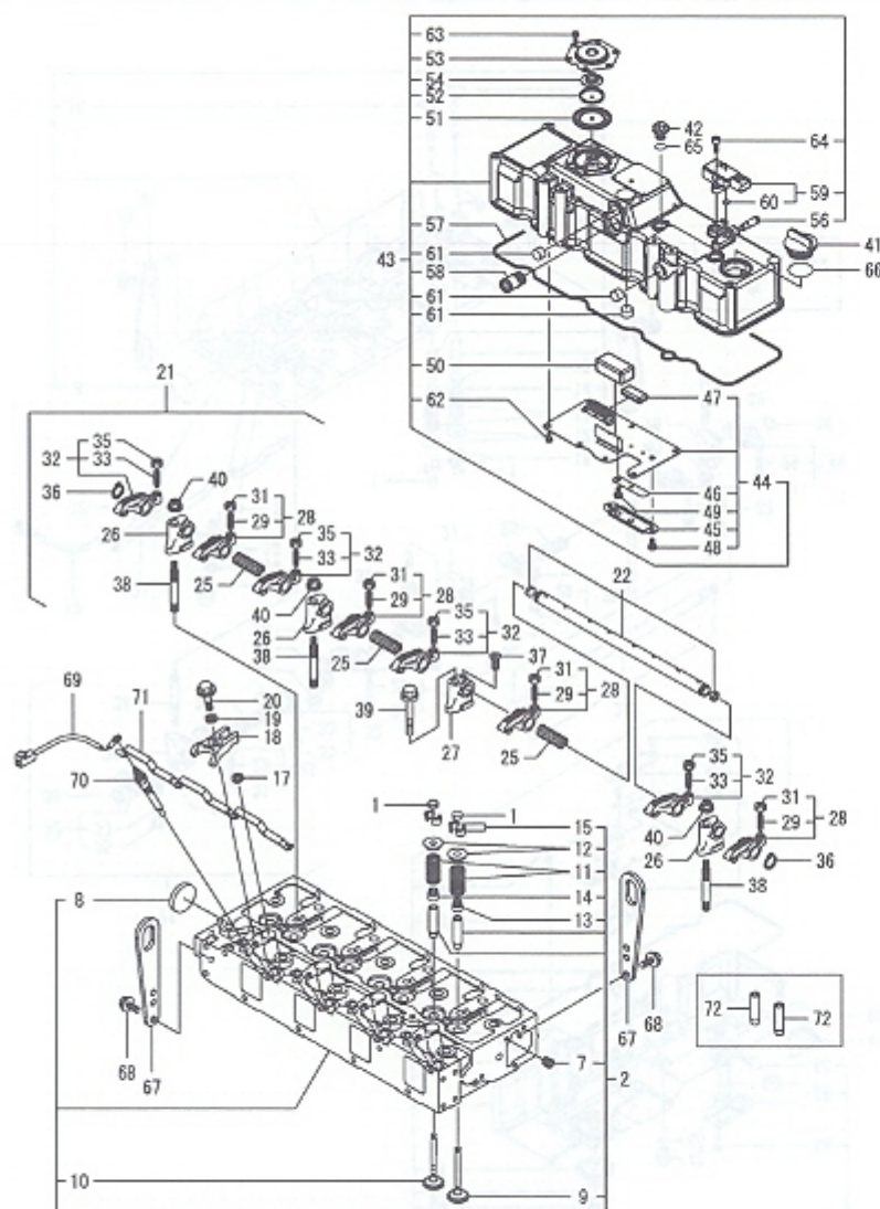
Fig.4. 실린더헤드&amp;본넷
