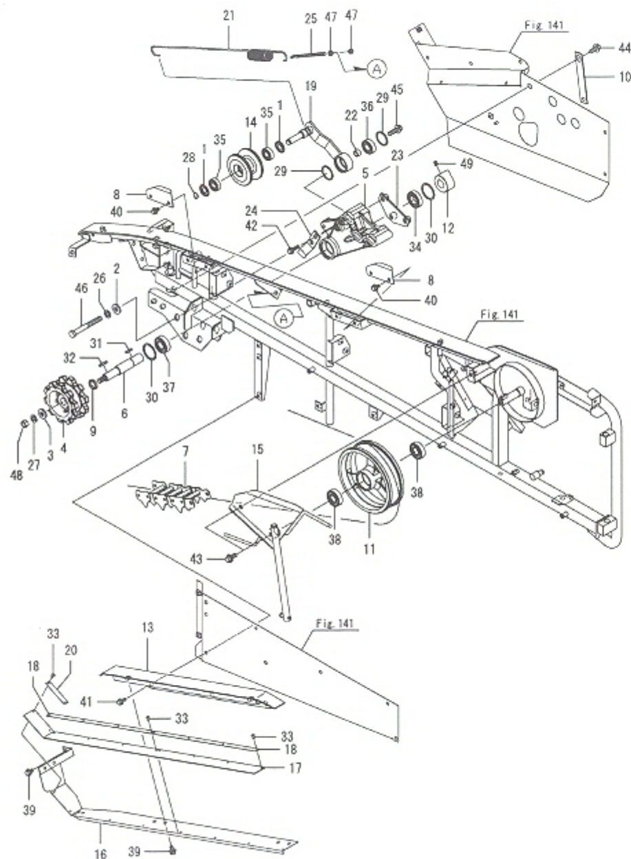
Fig.192. 피드체인
