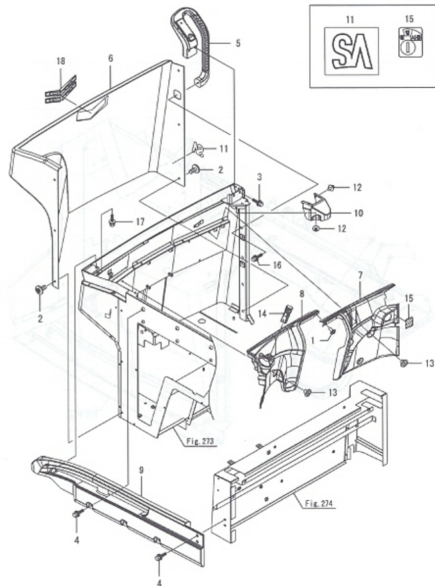
Fig.275. 바닥판의장(상)
