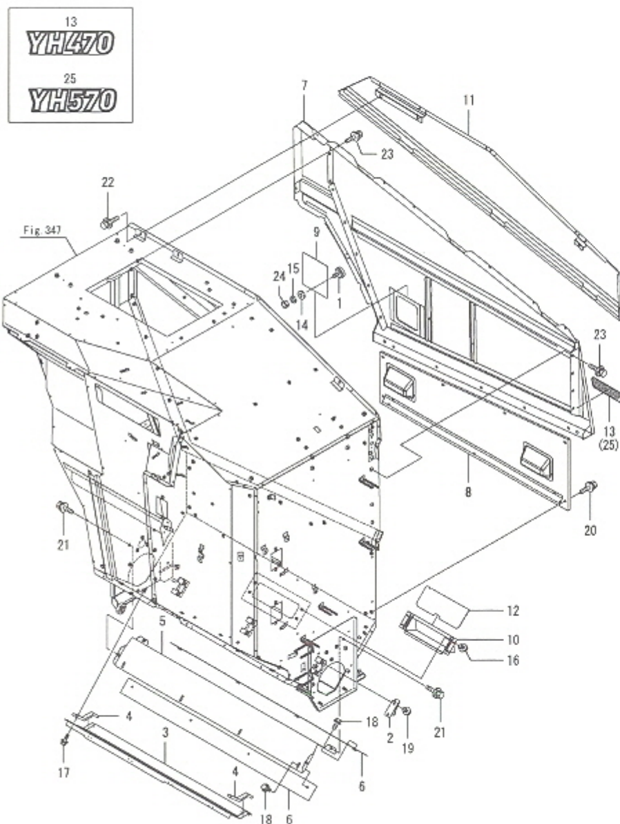
Fig.348. 곡물탱크(2)
