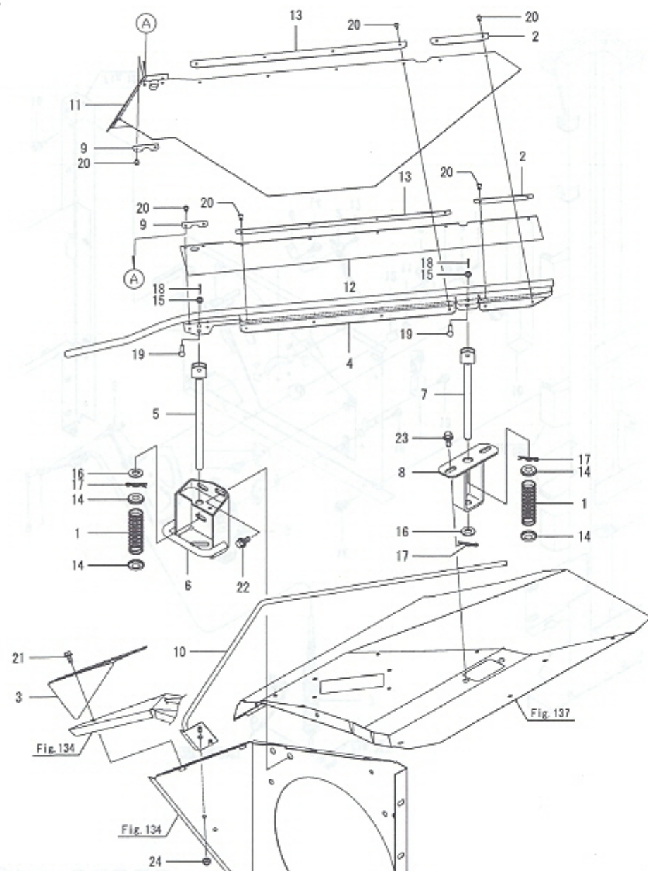
Fig.199. 짚배출잡이
