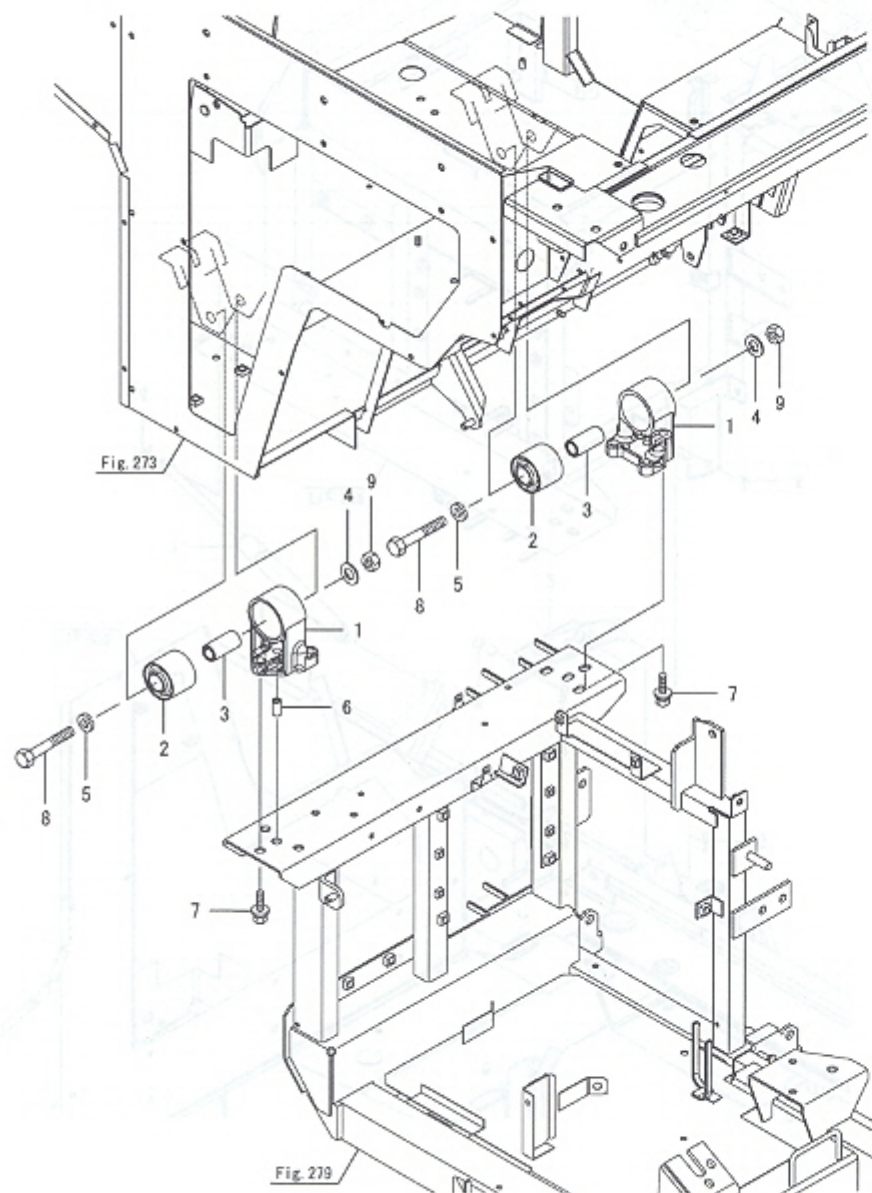
Fig.267. 발판방진(앞)
