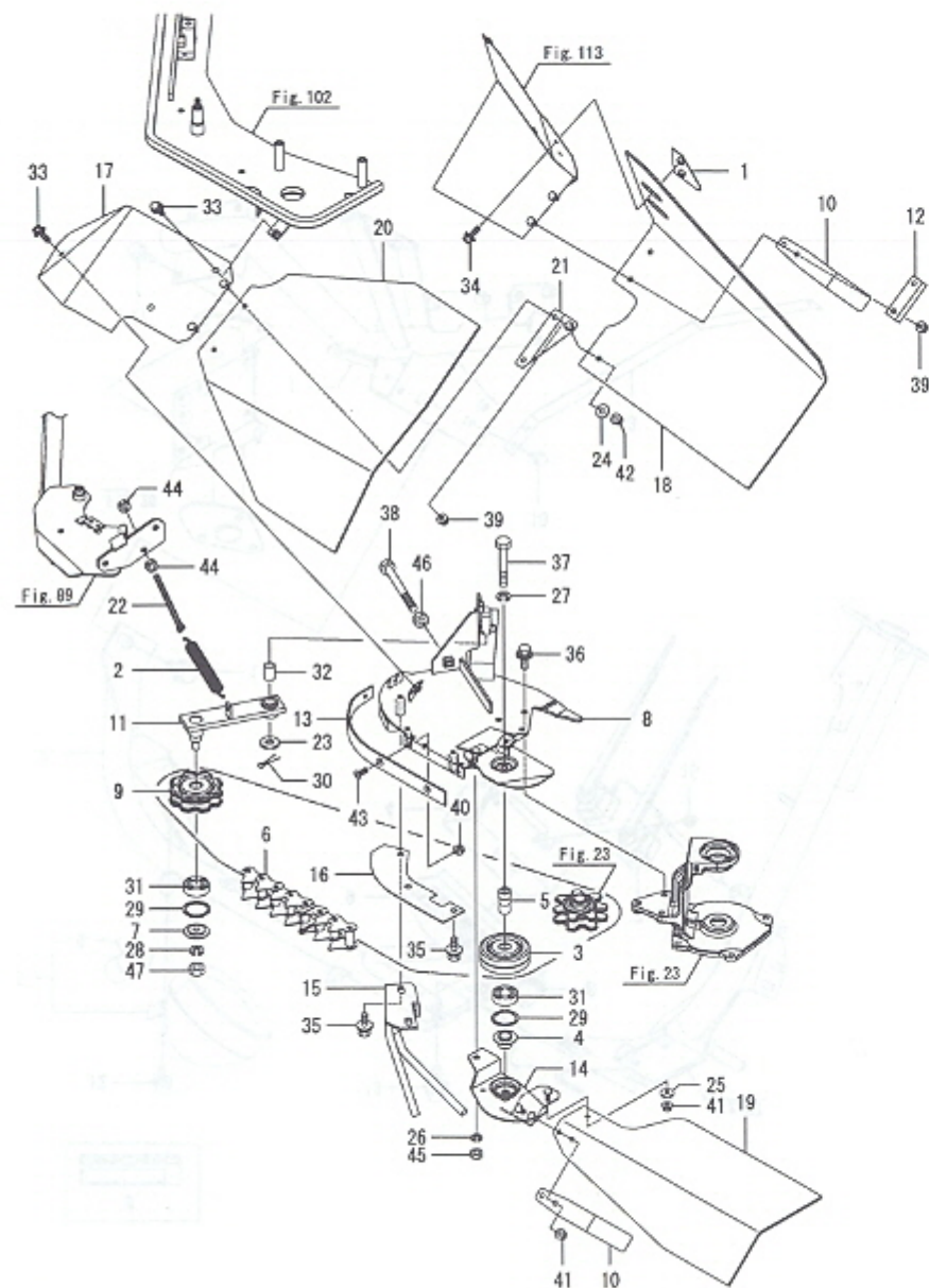
Fig.125. 보조반송케이스
