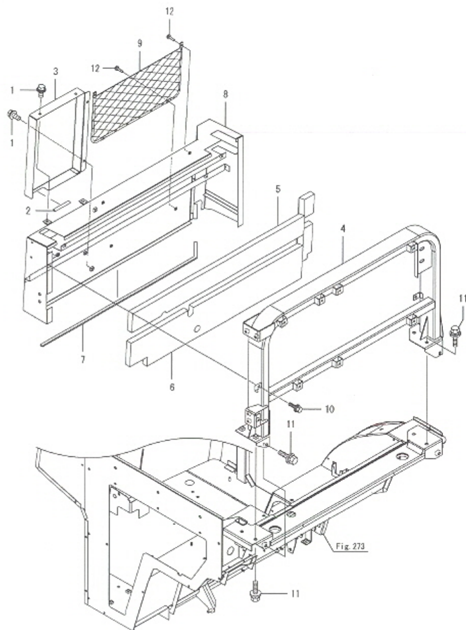
Fig.274. 후면 칼럼
