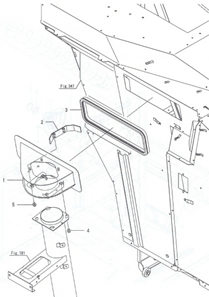
Fig.183. 양곡투입구
