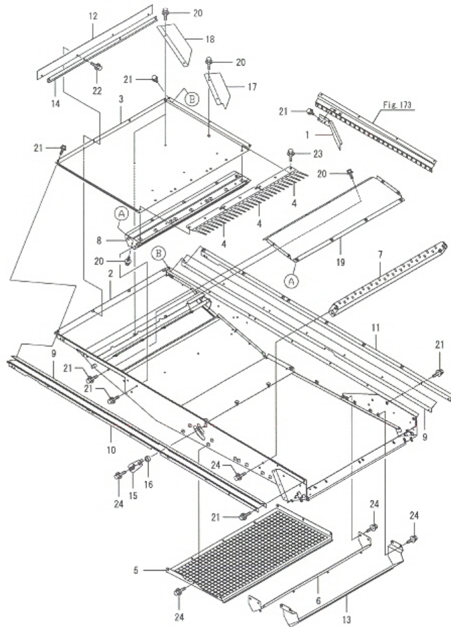
Fig.174. 스윙(2)
