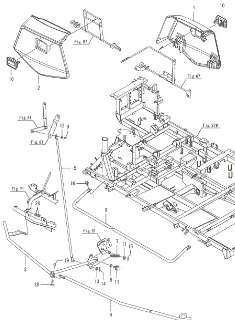
Fig.19. 예취(2)
