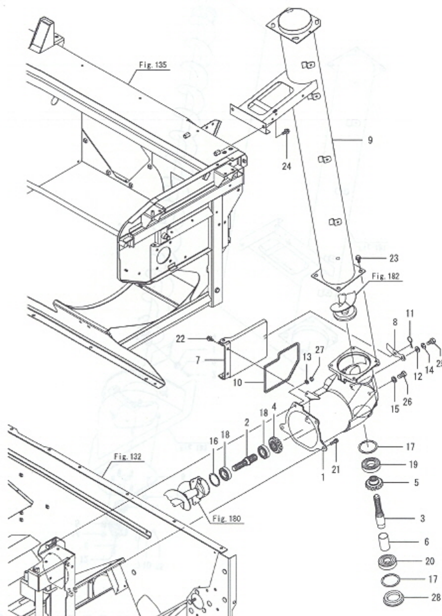
Fig.181. 컨베이어케이스
