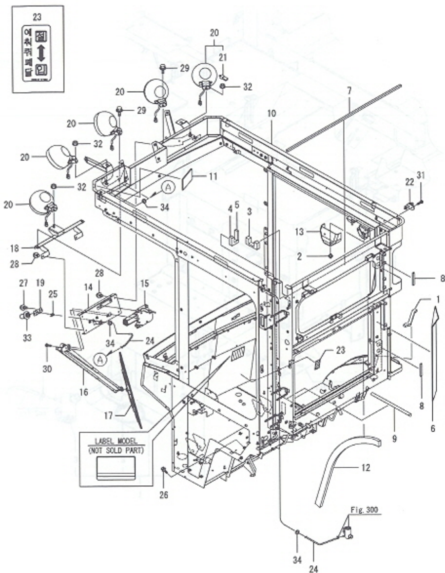
Fig.299. 캐빈(몸체)
