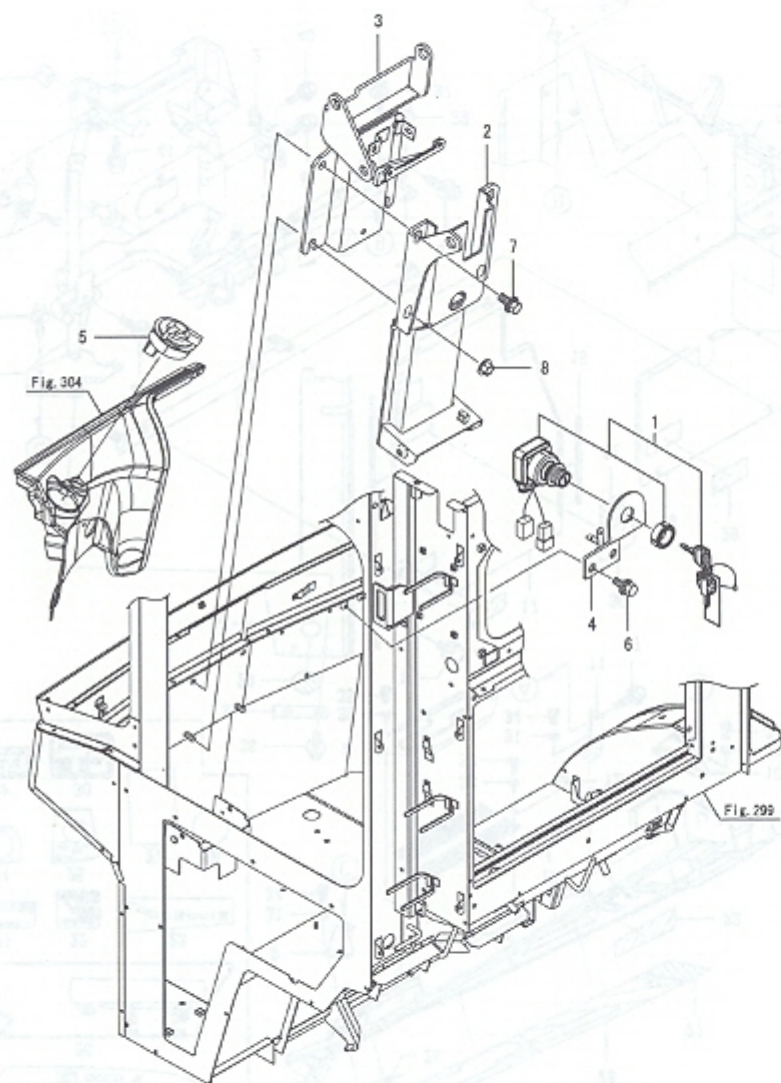
Fig.245. 스티어링칼럼(캐빈)
