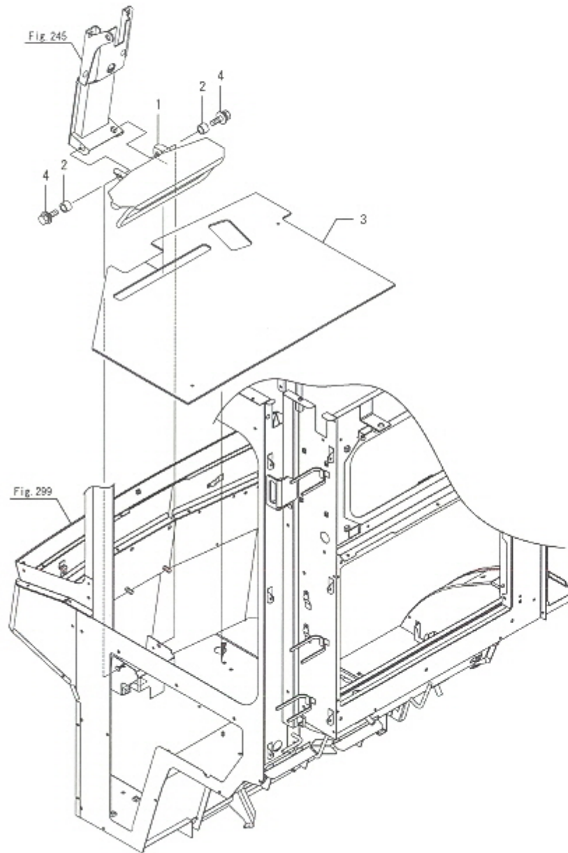
0CNP6-M03670 이동(2) Fig.264. 단(1)(캐빈)
