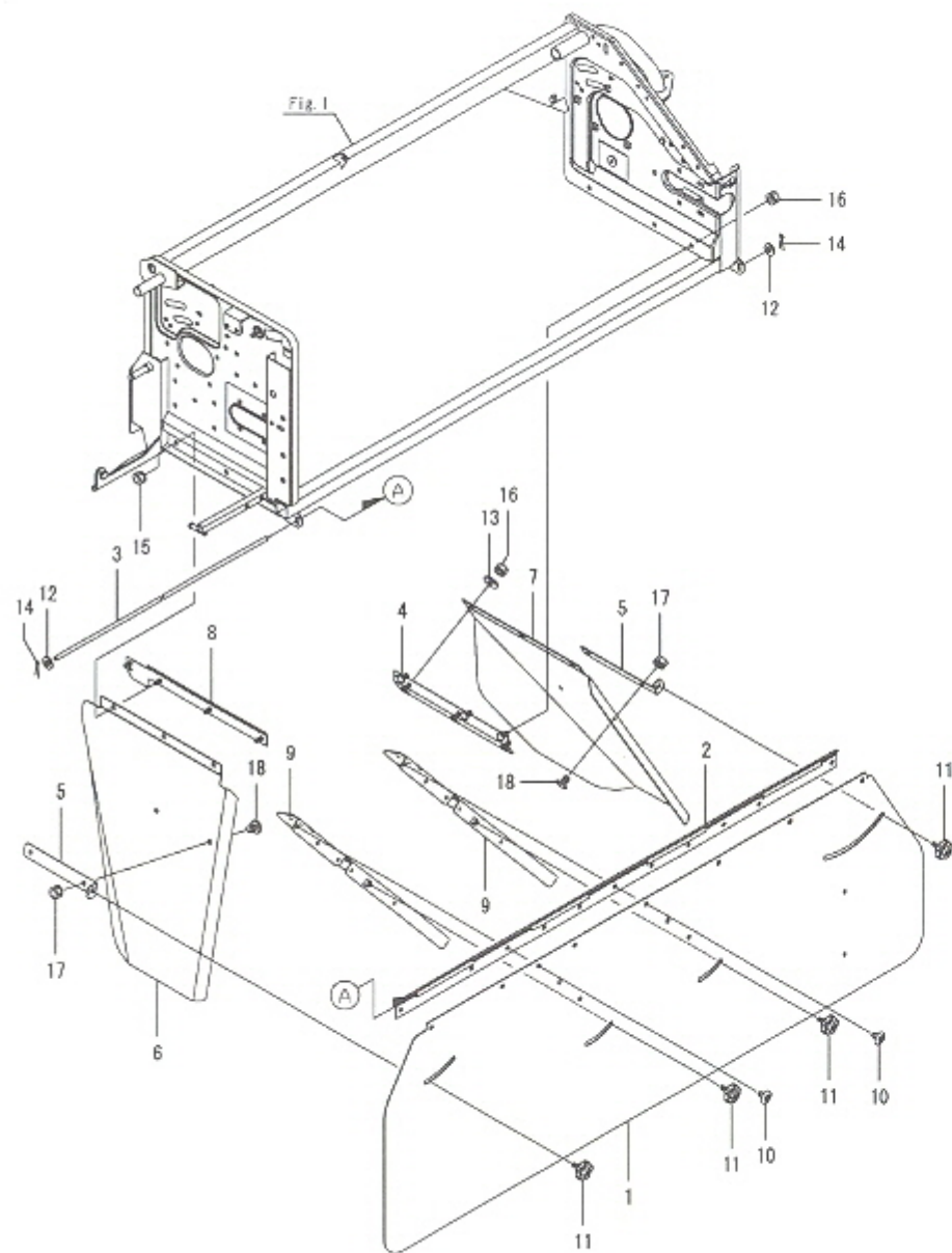
Fig.9. 하부커버
