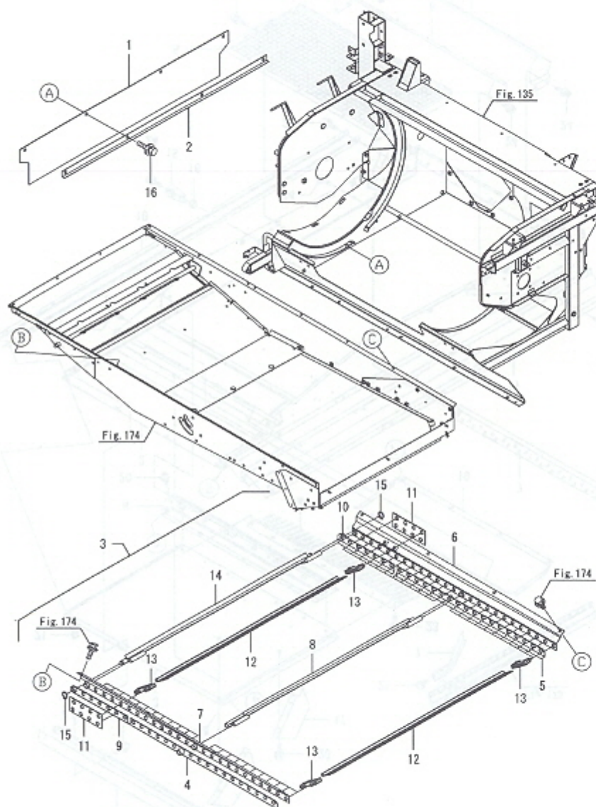
Fig.173. 스윙(1)
