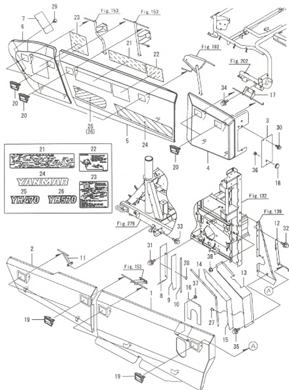
Fig.154. 사이드커버
