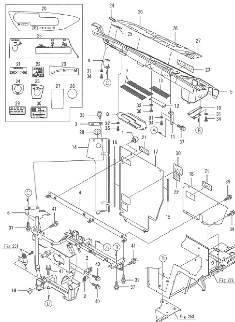
Fig.246. 사이드칼럼(1)
