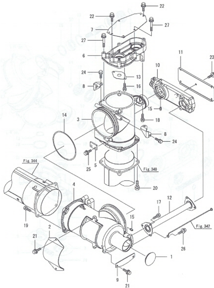
Fig.341. 오거연결케이스(1)
