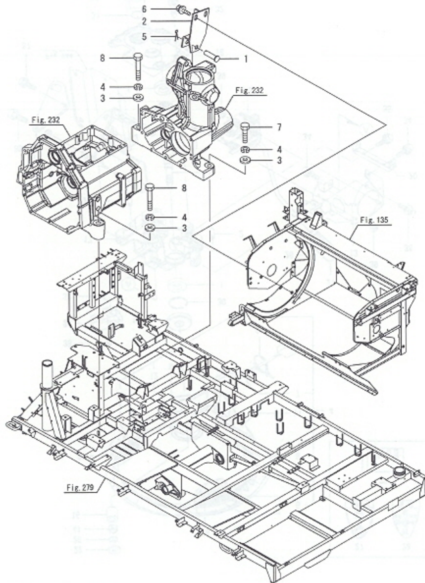
Fig.241. 카운터케이스취부
