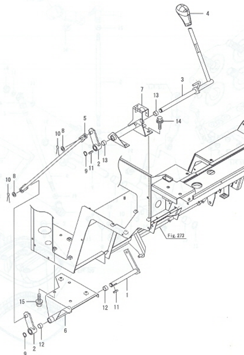
0CNP6-M03670 이동(2) Fig.253. 부변속(1)
