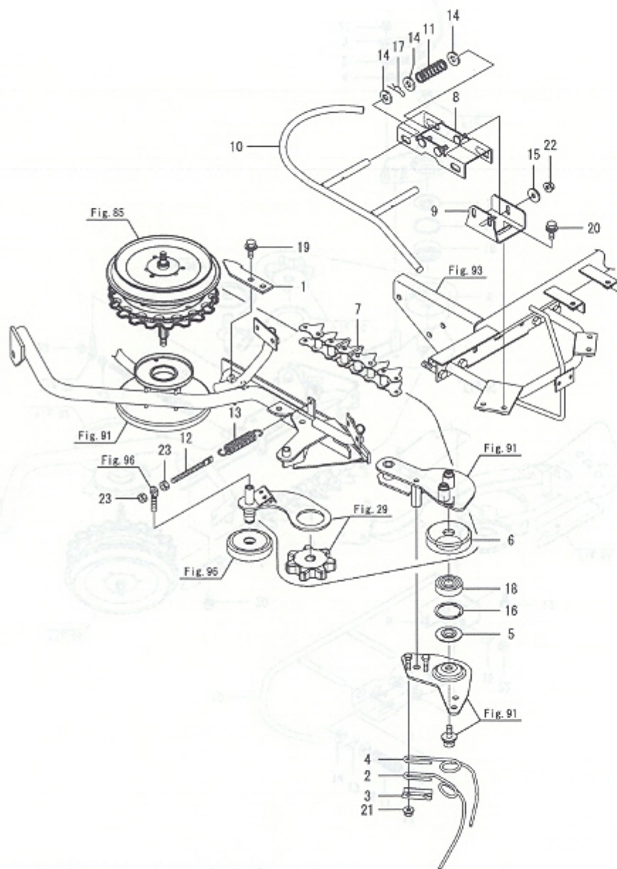
Fig.99. 하단 이송 가이드(왼쪽)
