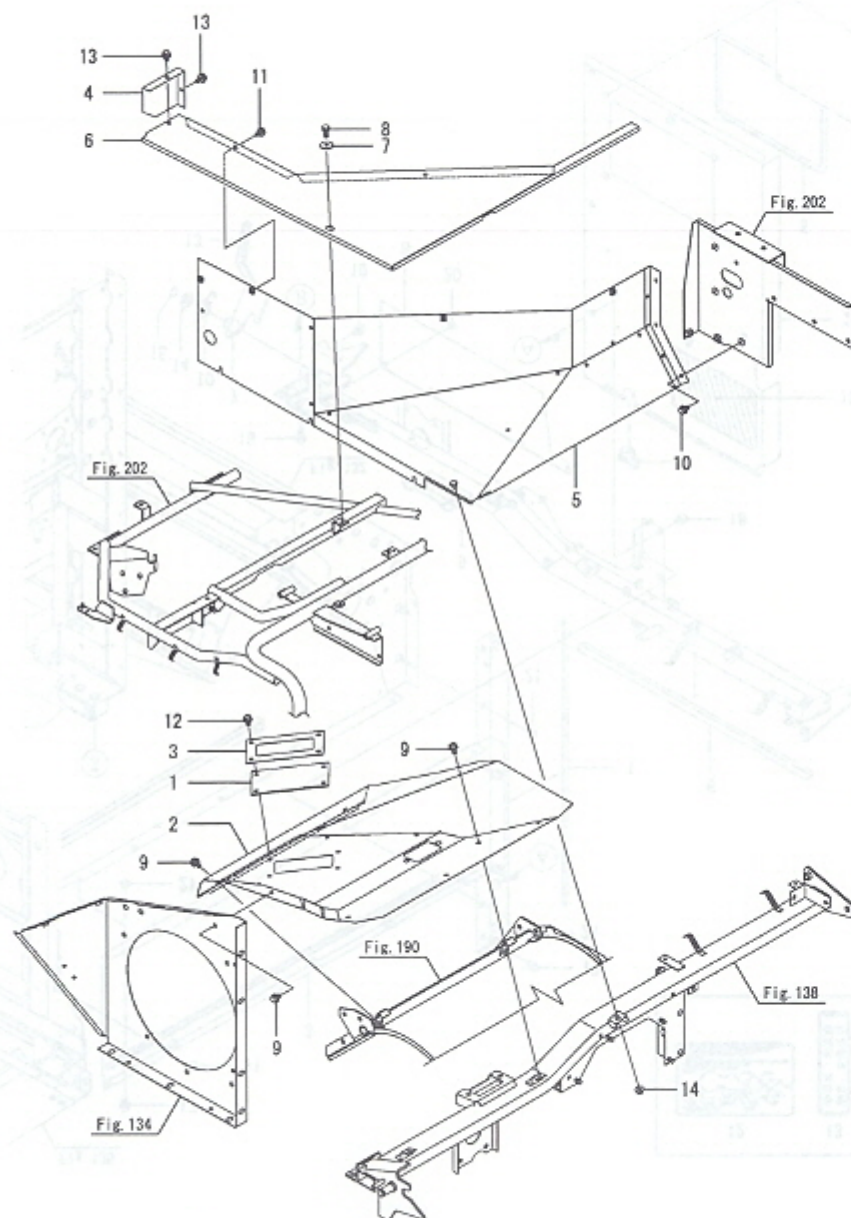
Fig.137. 상부분체(출구)
