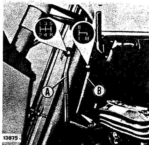
주변속 및 부변속레버 위치
