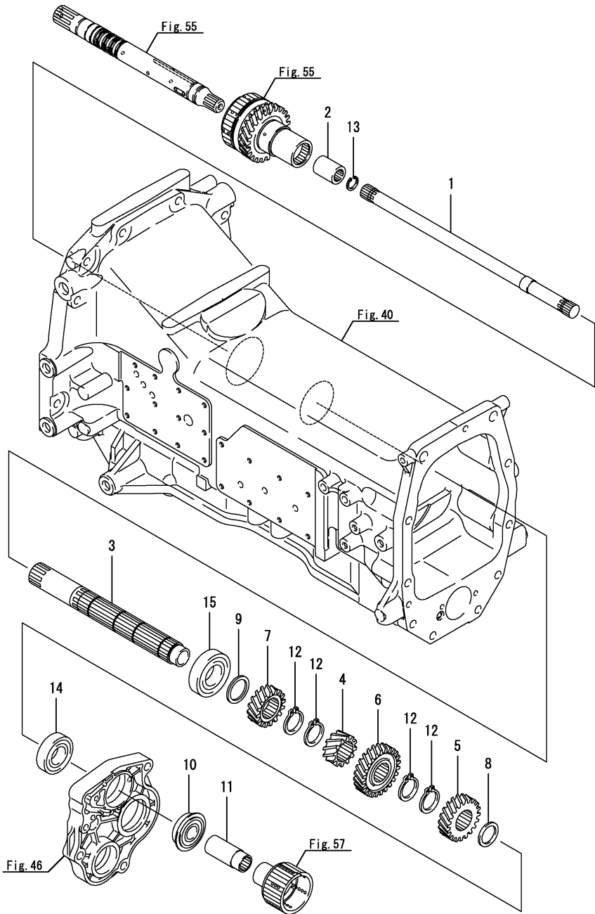
Fig.51. 주축
