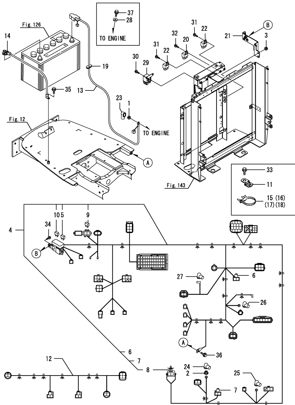
Fig.121. 배선(A)(캐빈)
