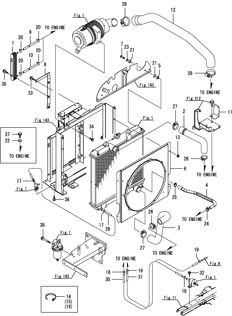
Fig.3. 엔진악세사리(캐빈)
