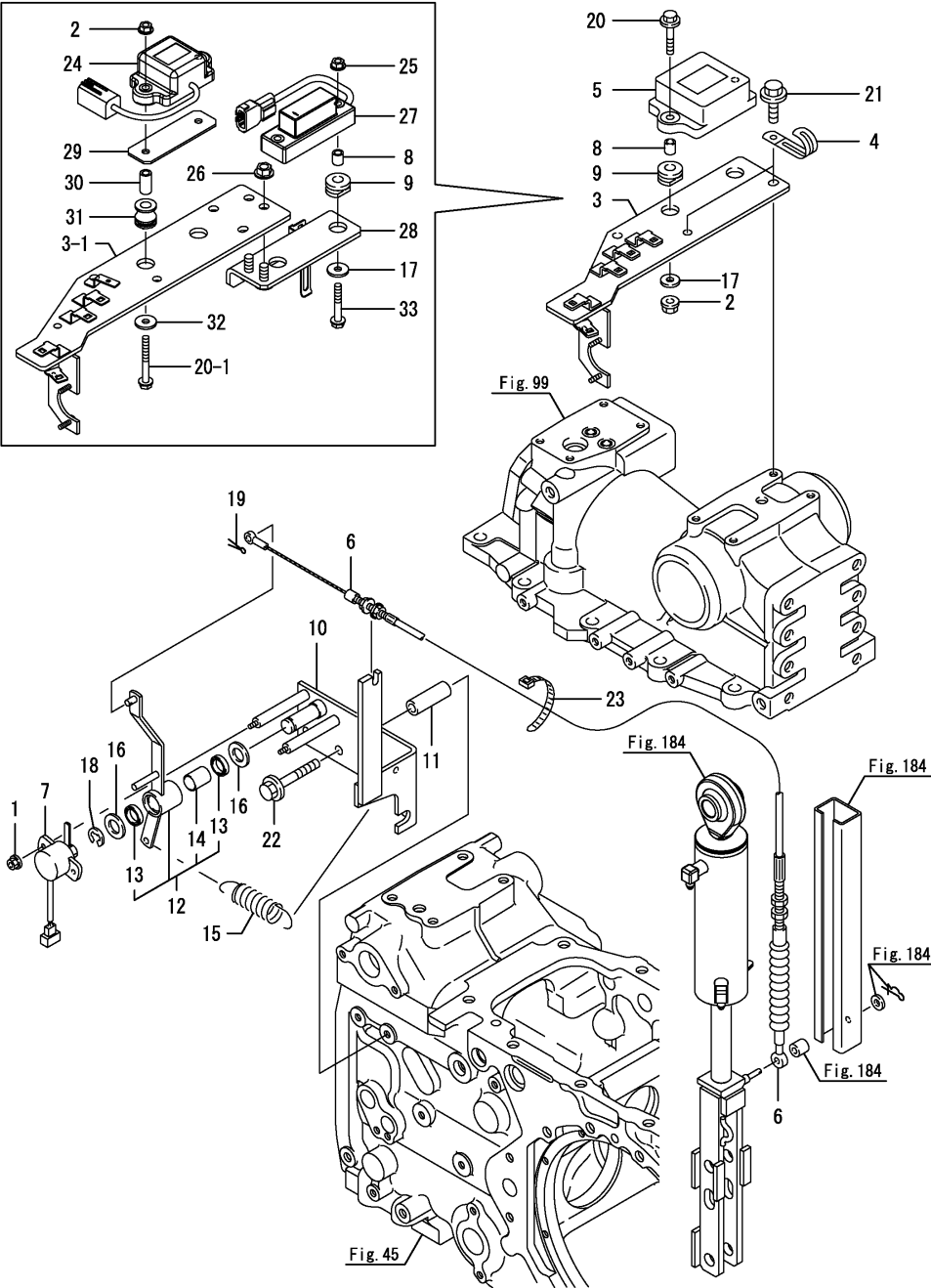
Fig.190. 수평제어센서
