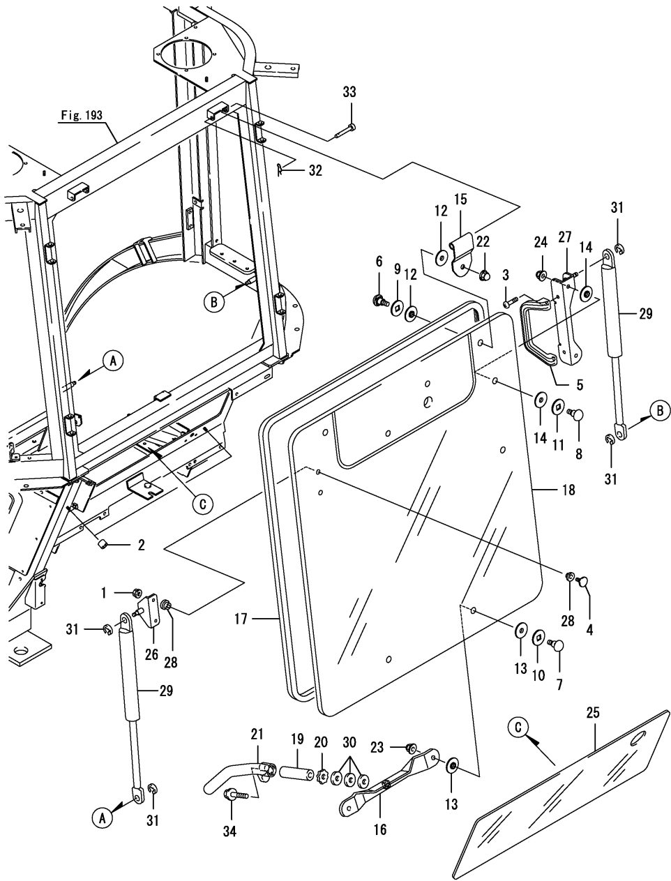
Fig.199. 후방창문
