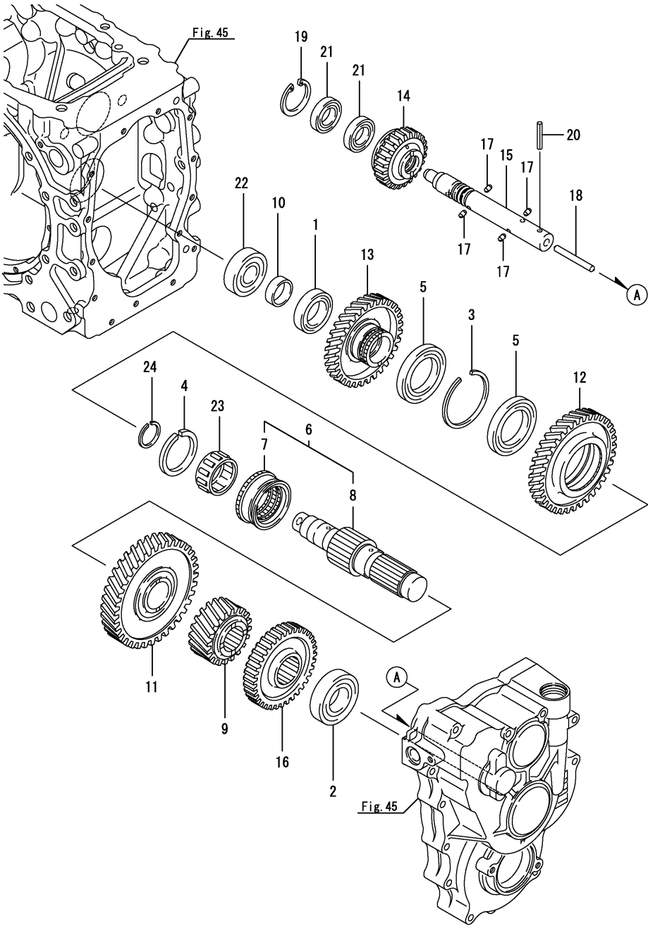
Fig.59. P.T.O. 피구동축
