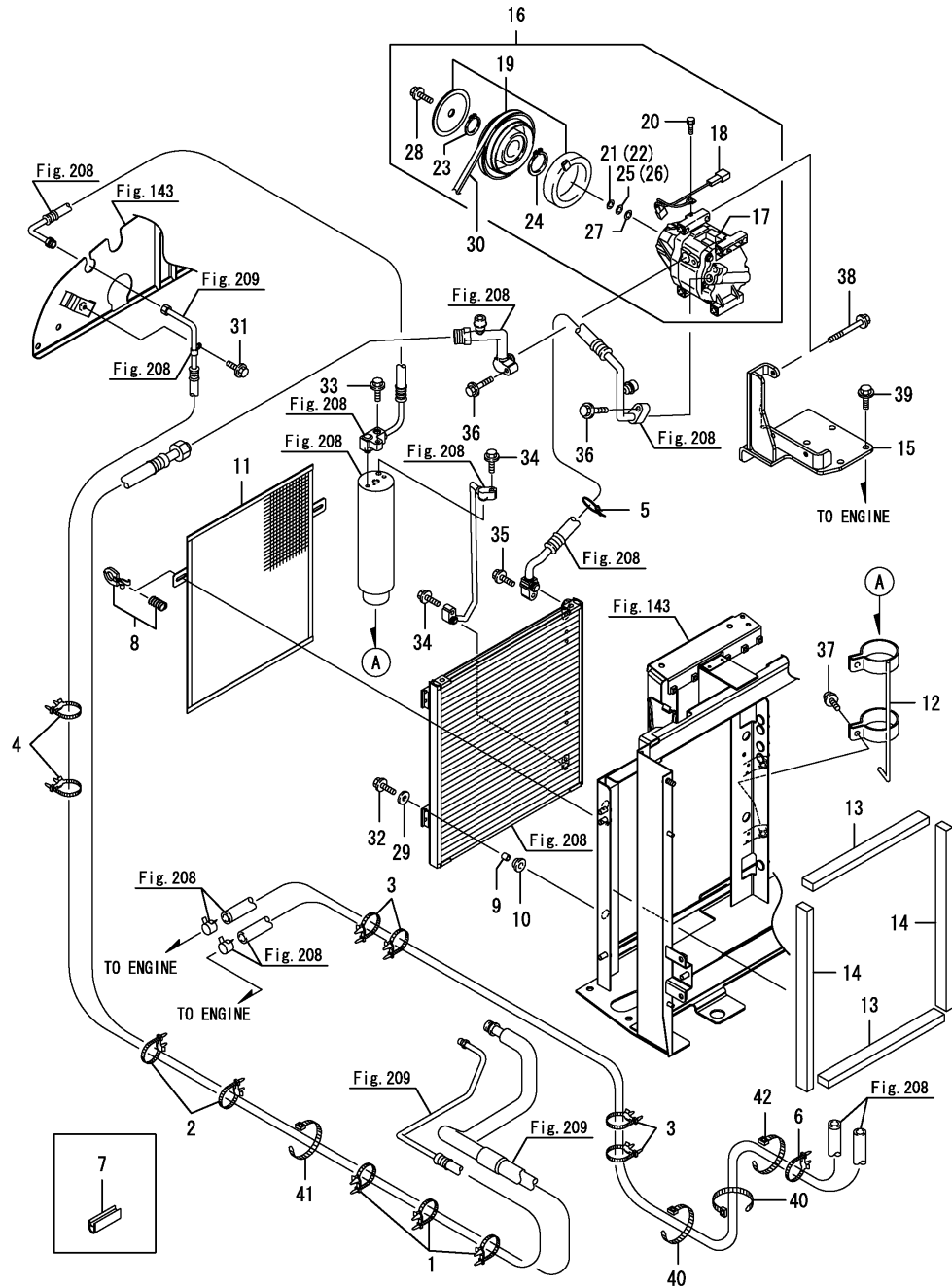
Fig.212. 에어컨(4)
