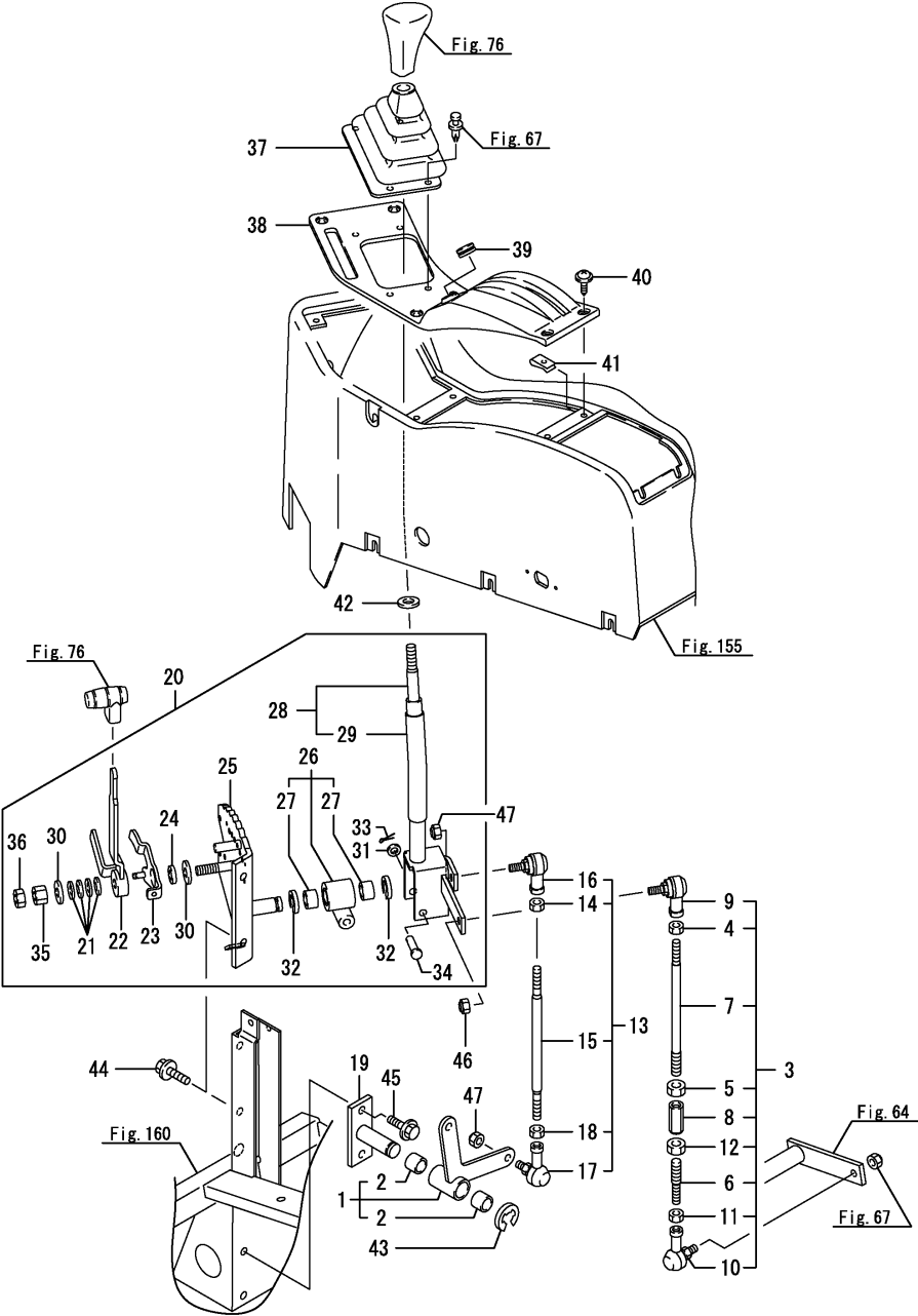
Fig.65. 시프트레버
