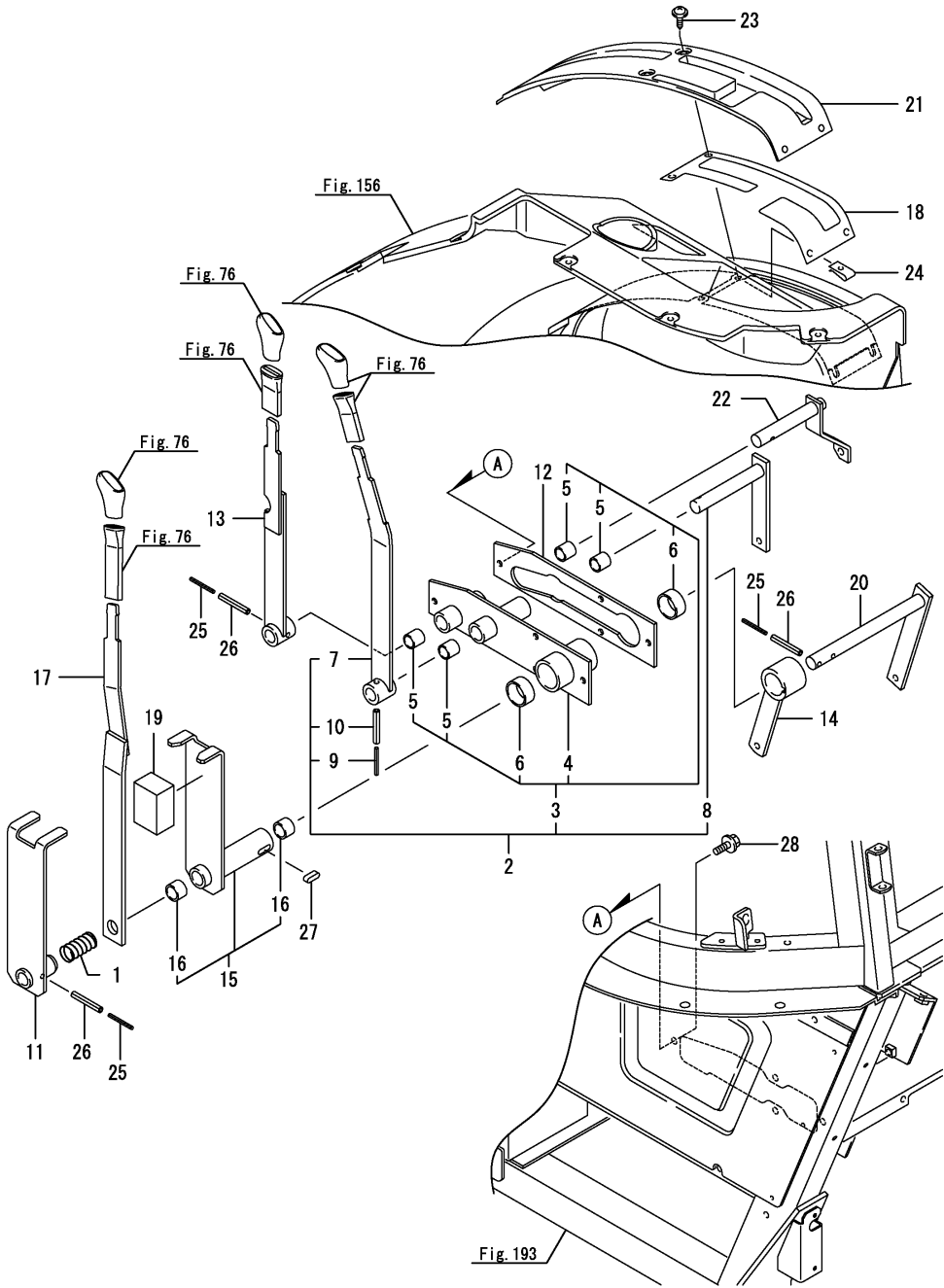
Fig.72. 보조레버(캐빈)
