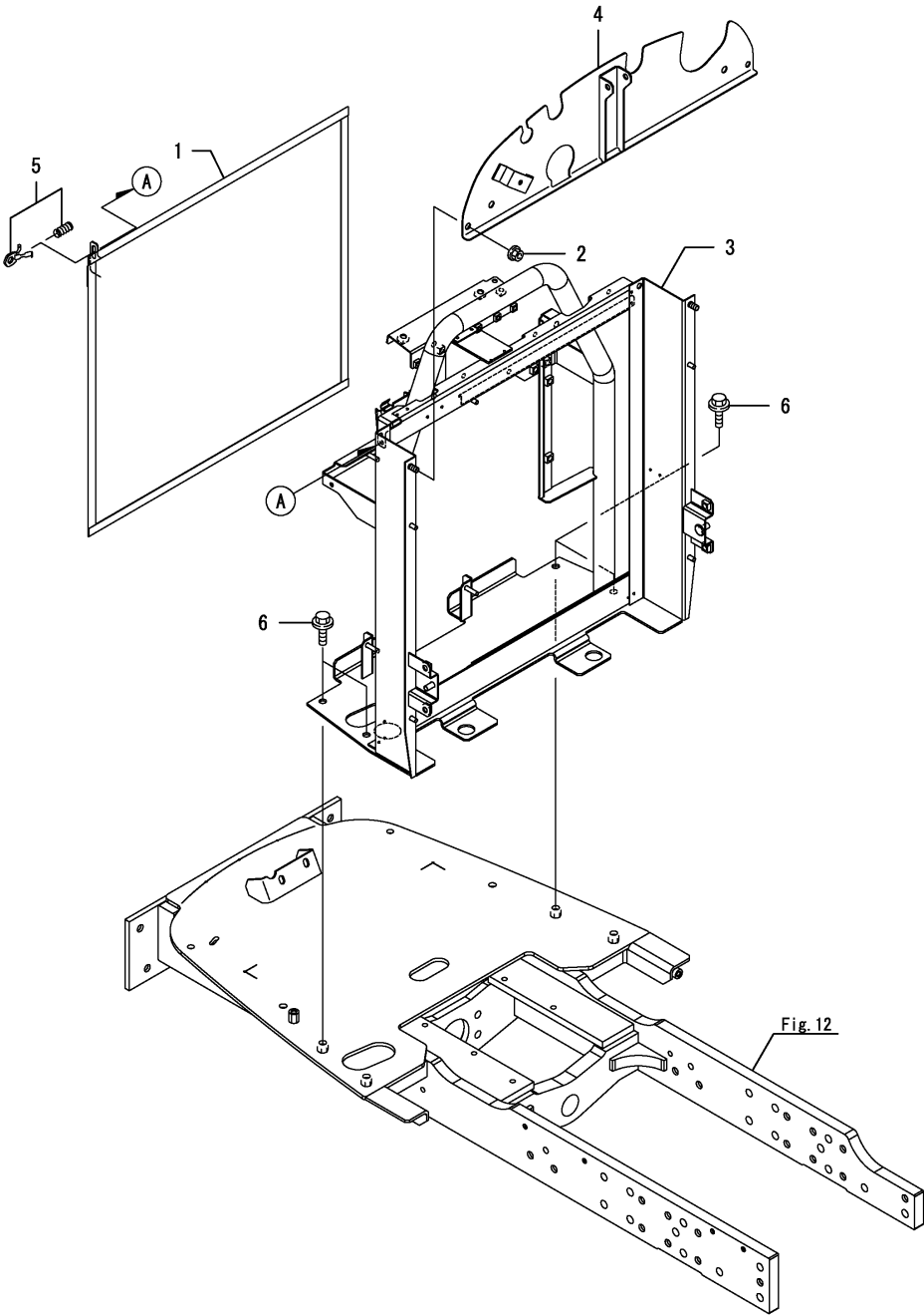
Fig.142. 프론트프레임
