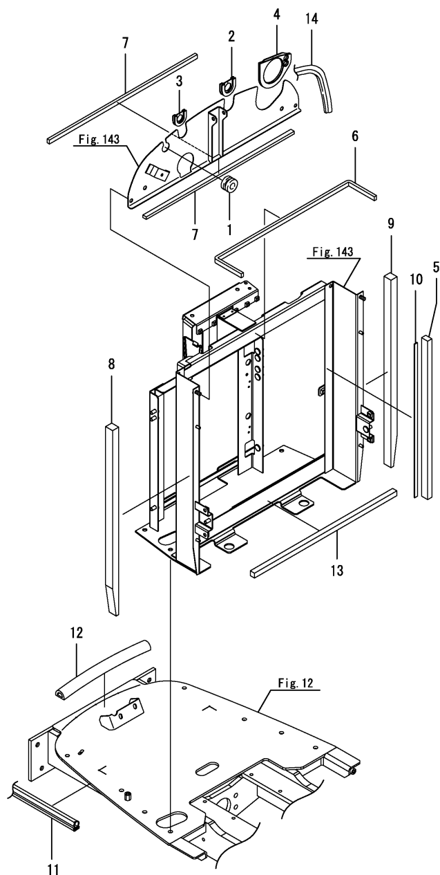
Fig.150. 본네트시일(캐빈)
