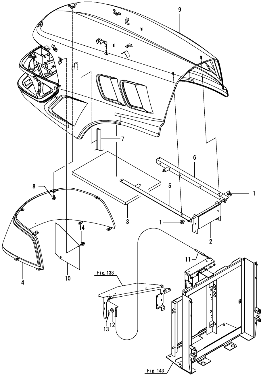
Fig.147. 본넷(캐빈)
