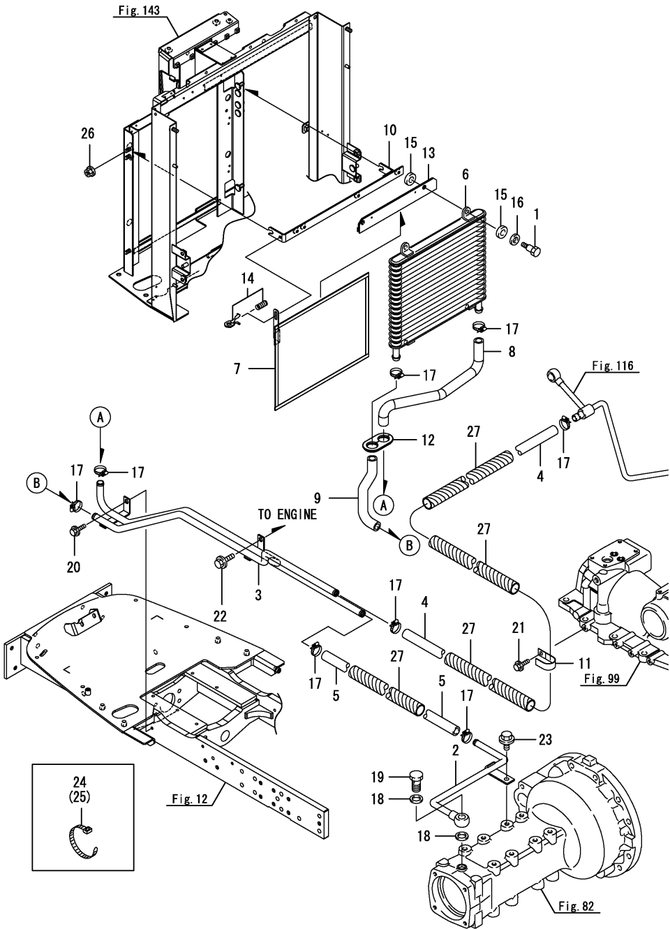
Fig.119. 오일쿨러(캐빈)
