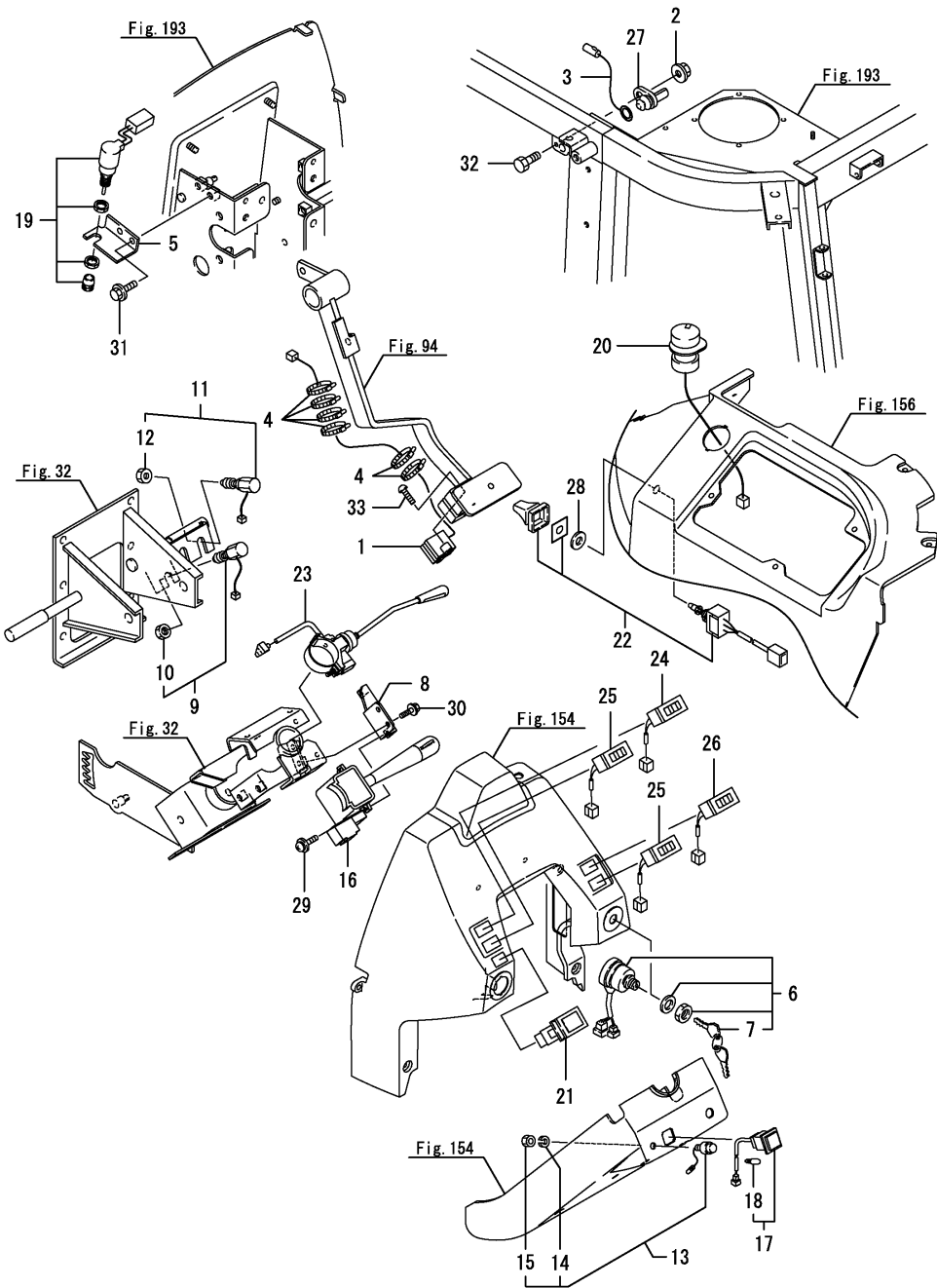
Fig.129. 스위치(캐빈)
