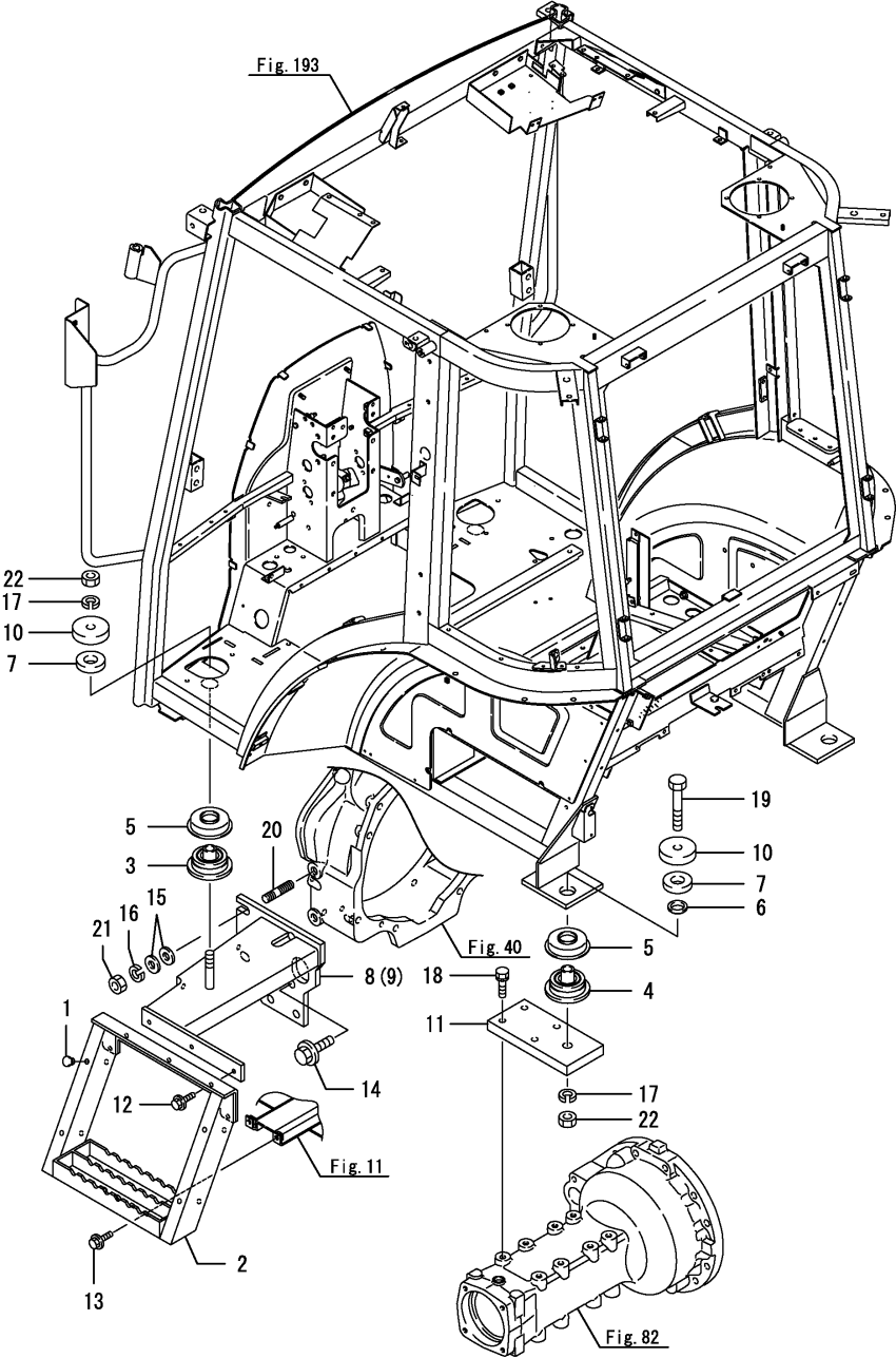
Fig.163. 바닥서포트(캐빈)
