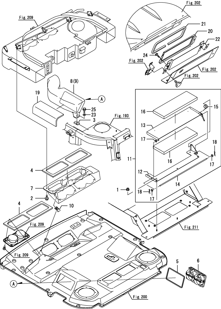
Fig.213. 에어컨덕트
