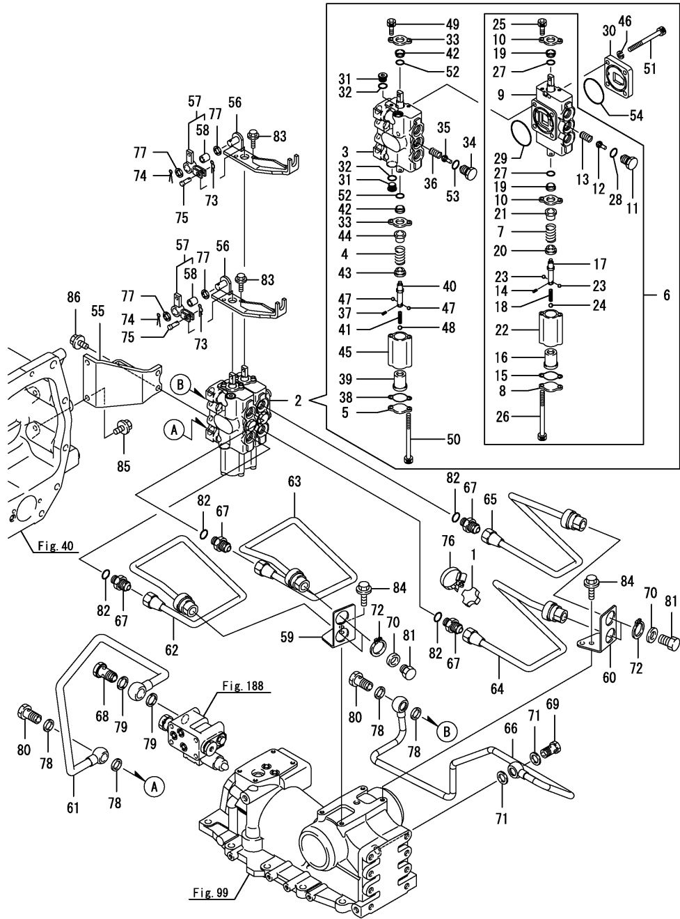
Fig.106. S.C.V.
