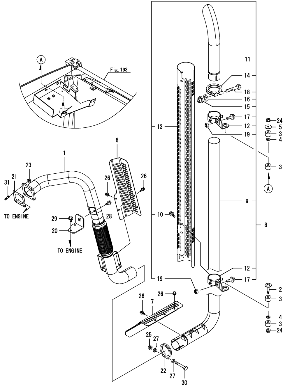
Fig.7. 배기구(캐빈)
