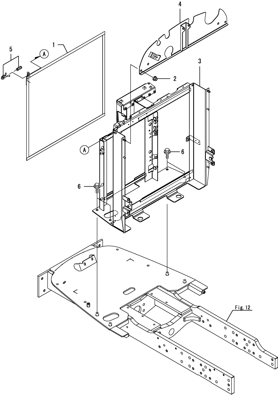
Fig.143. 프론트프레임(캐빈)
