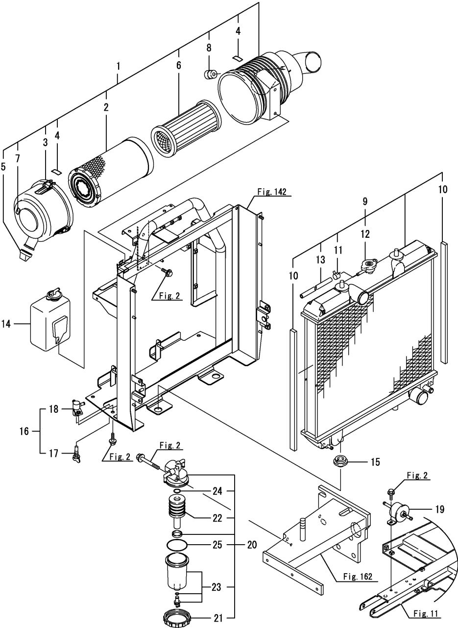
Fig.1. 엔진관련
