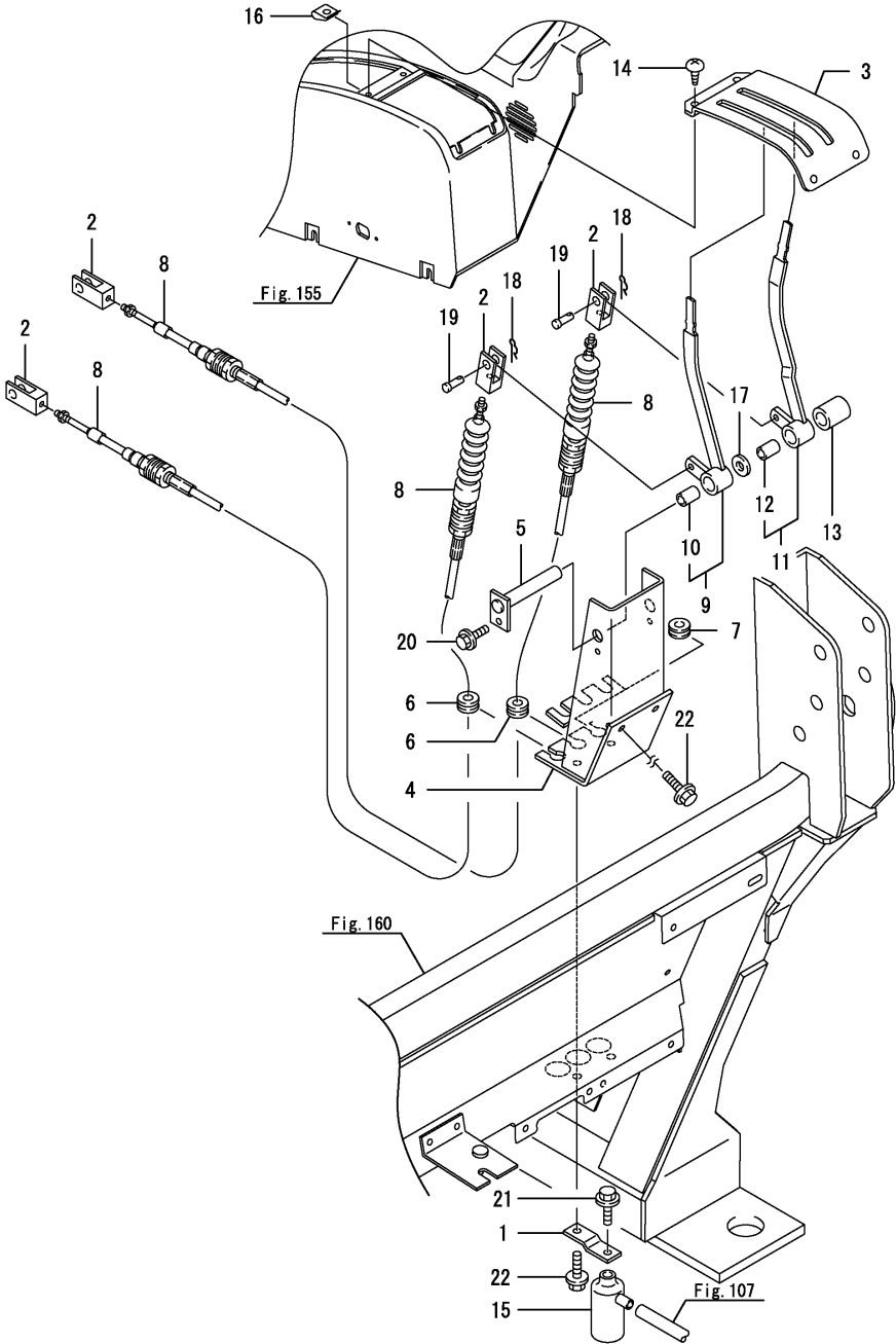
Fig.108. S.C.V.컨트롤(2)
