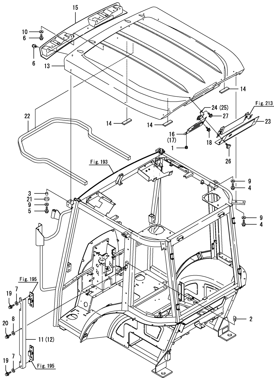
Fig.202. 루프
