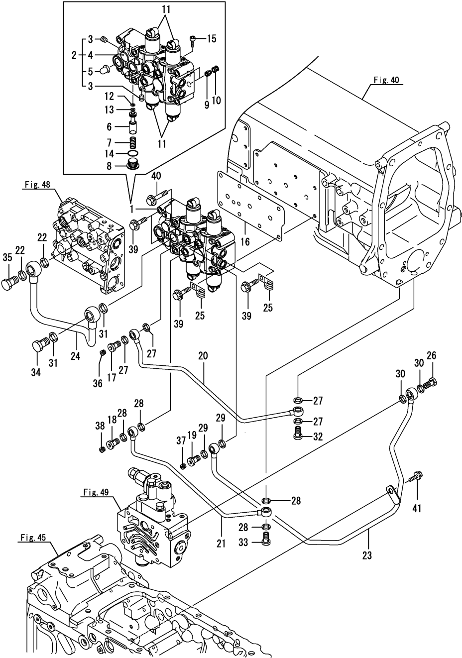
Fig.47. 메인밸브
