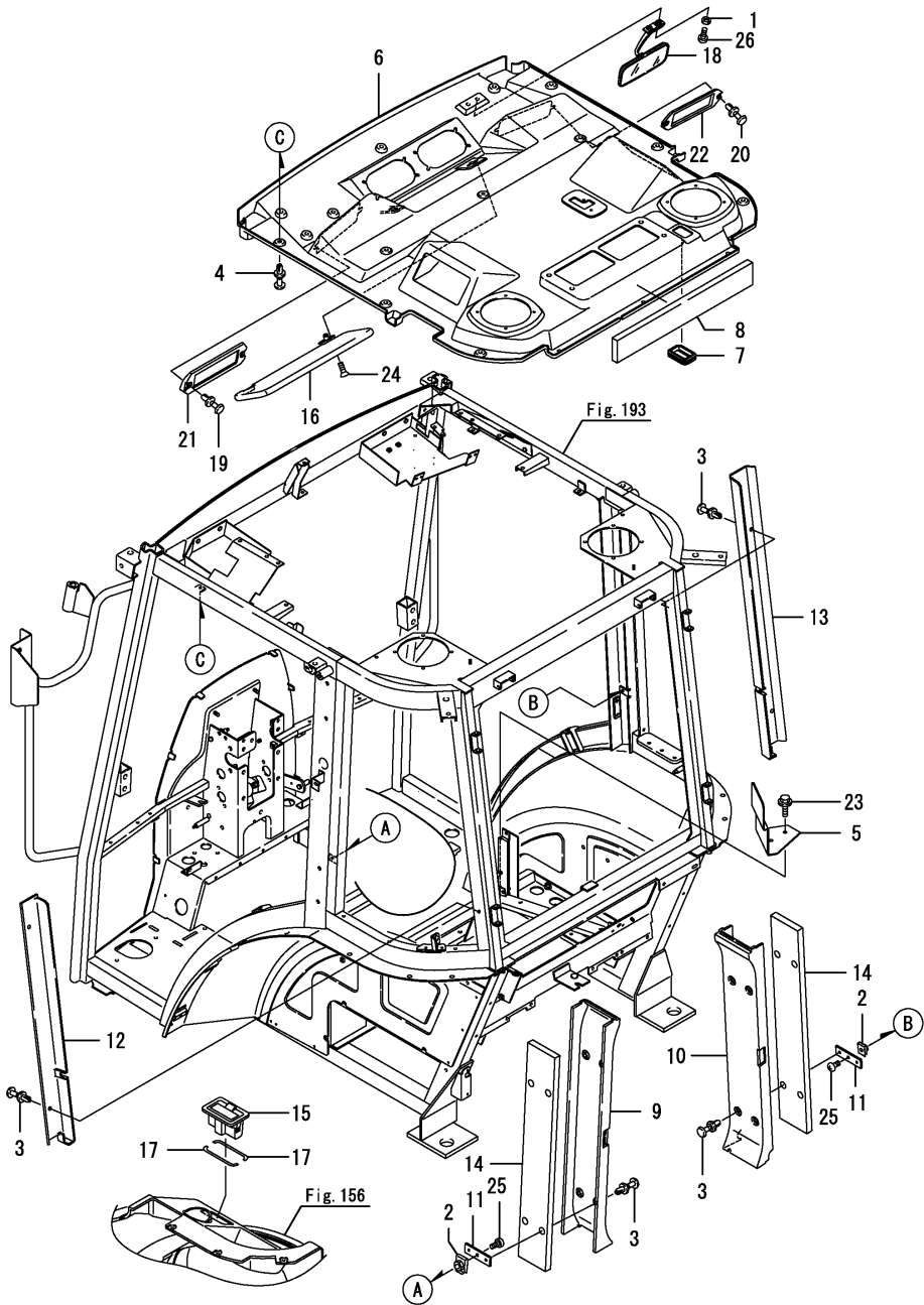
Fig.200. 인테리어
