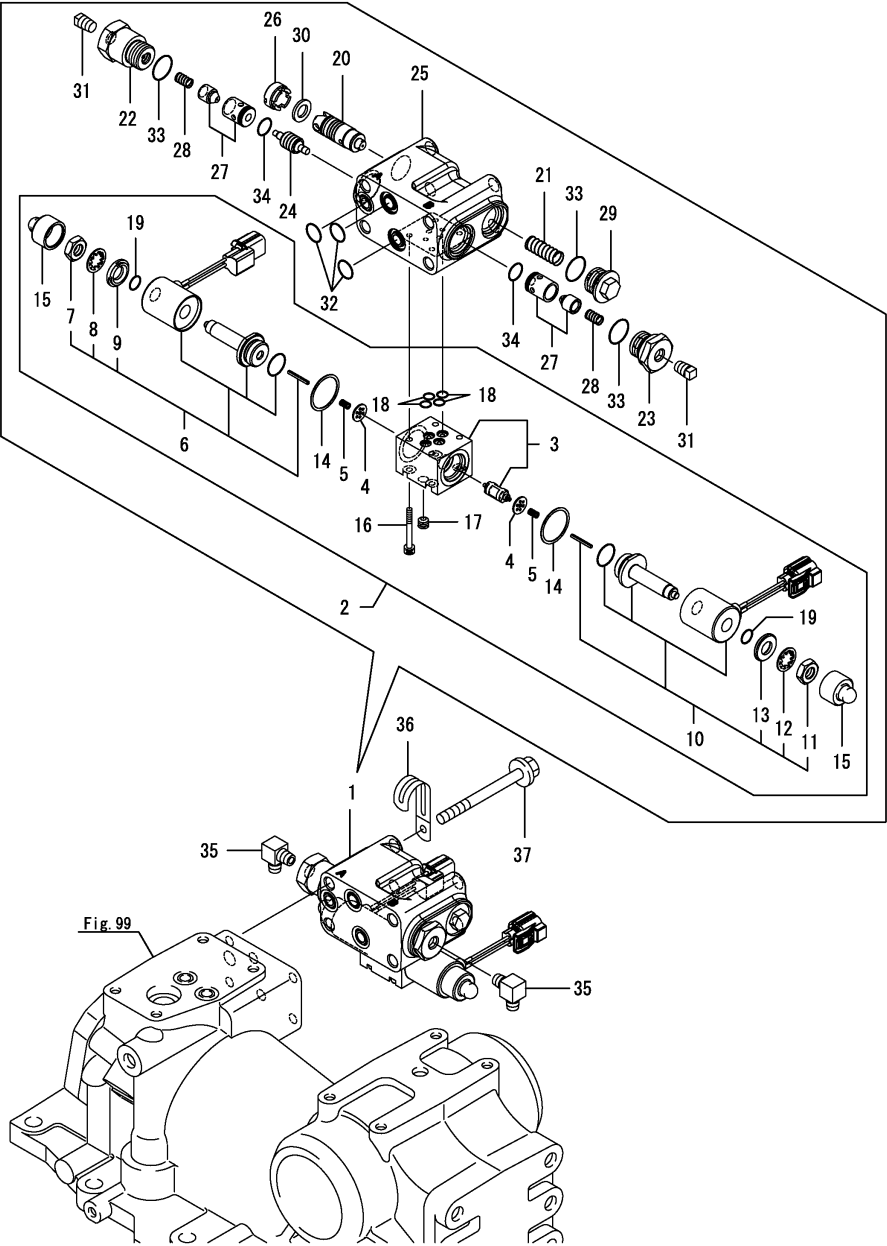
Fig.188. 수평제어밸브
