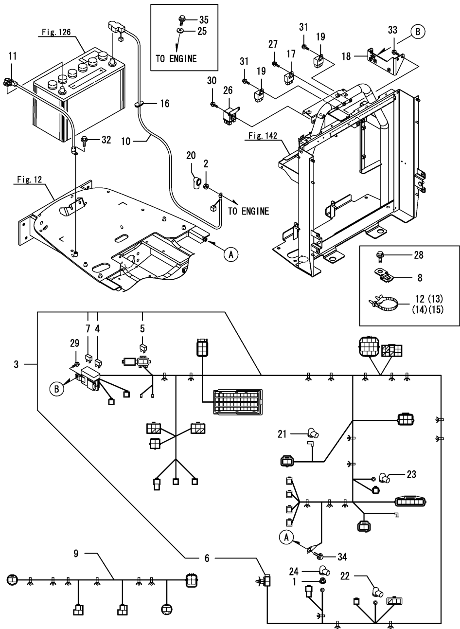
Fig.120. 배선(A)
