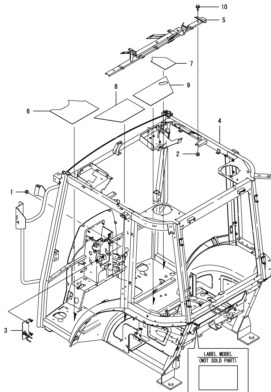
Fig.193. 캐빈프레임
