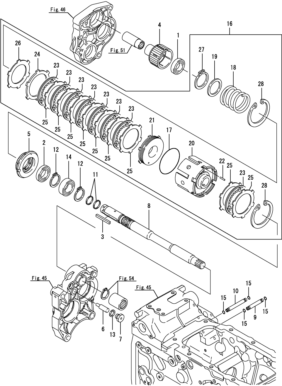
Fig.57. P.T.O. 클러치
