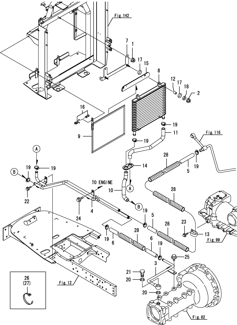
Fig.118. 오일쿨러
