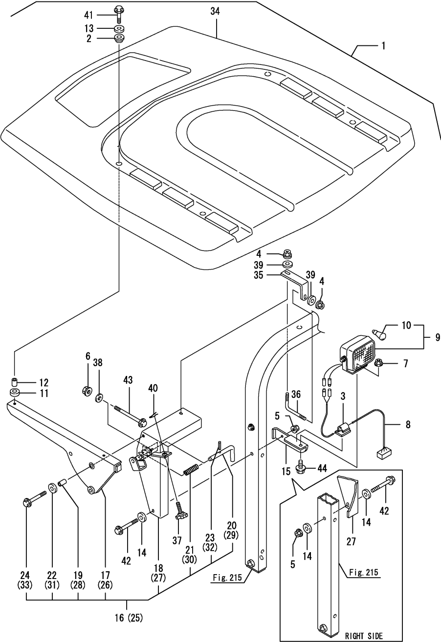
Fig.218. 캐노피
