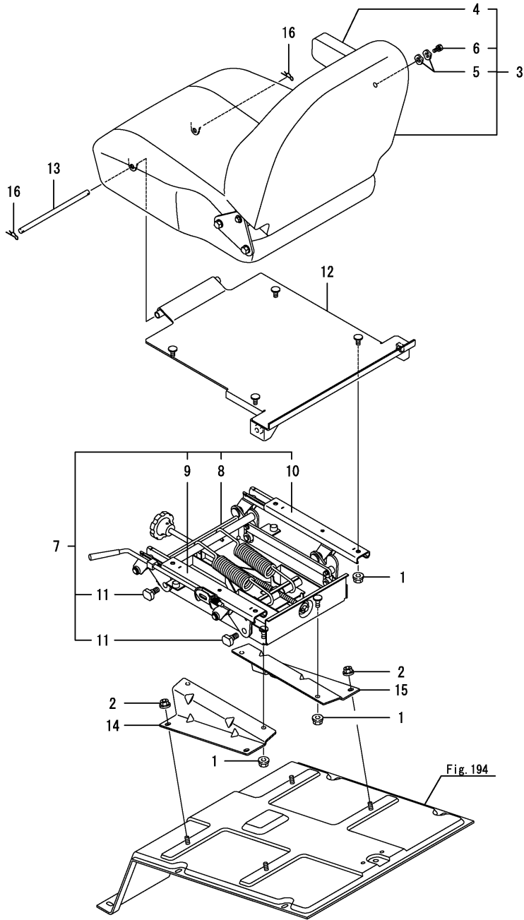
Fig.166. 시트조작(캐빈)
