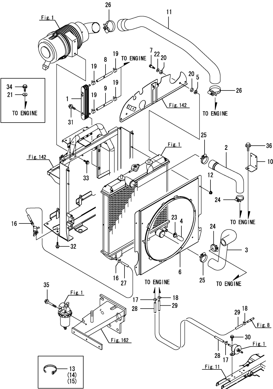
Fig.2. 엔진악세사리
