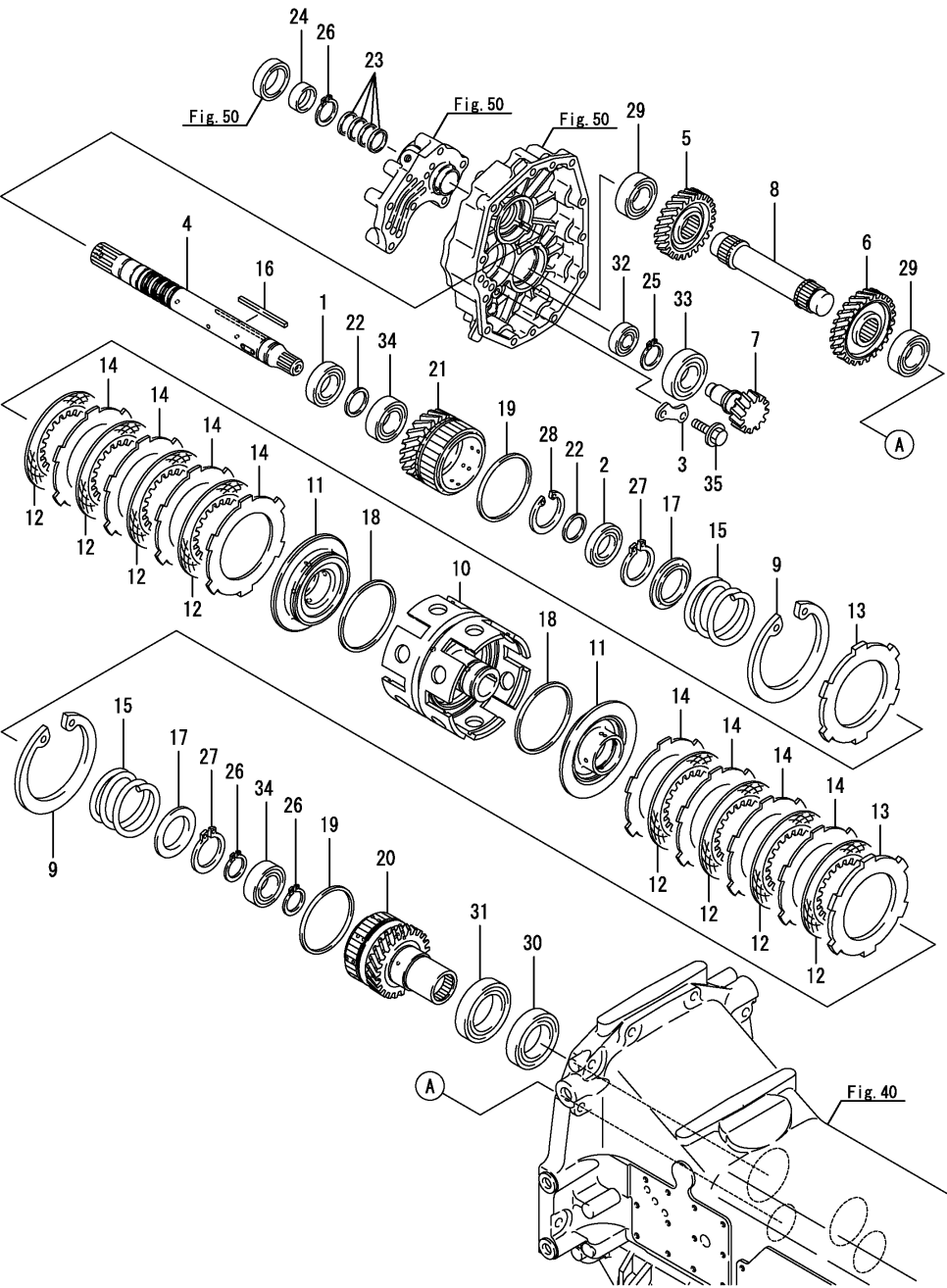
Fig.55. 파워리버서
