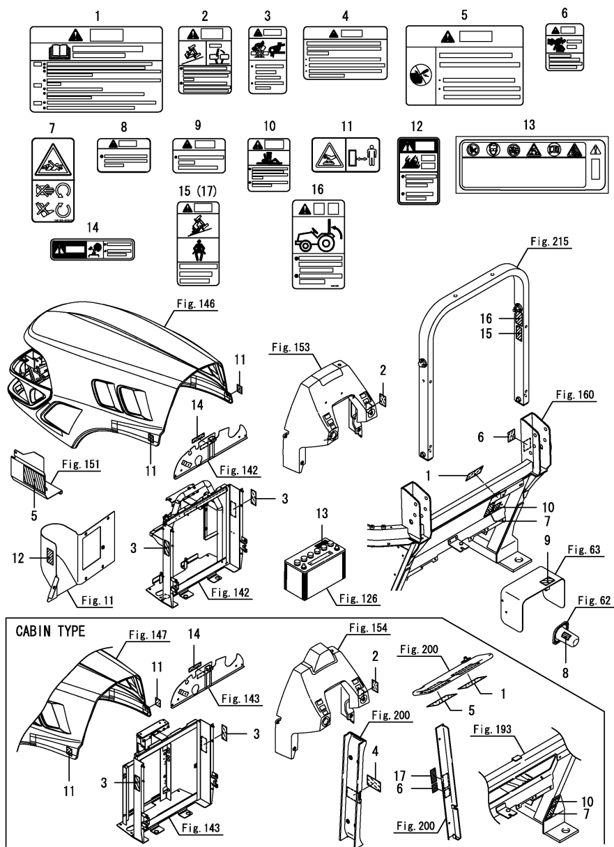
Fig.181. 명판(안전)
