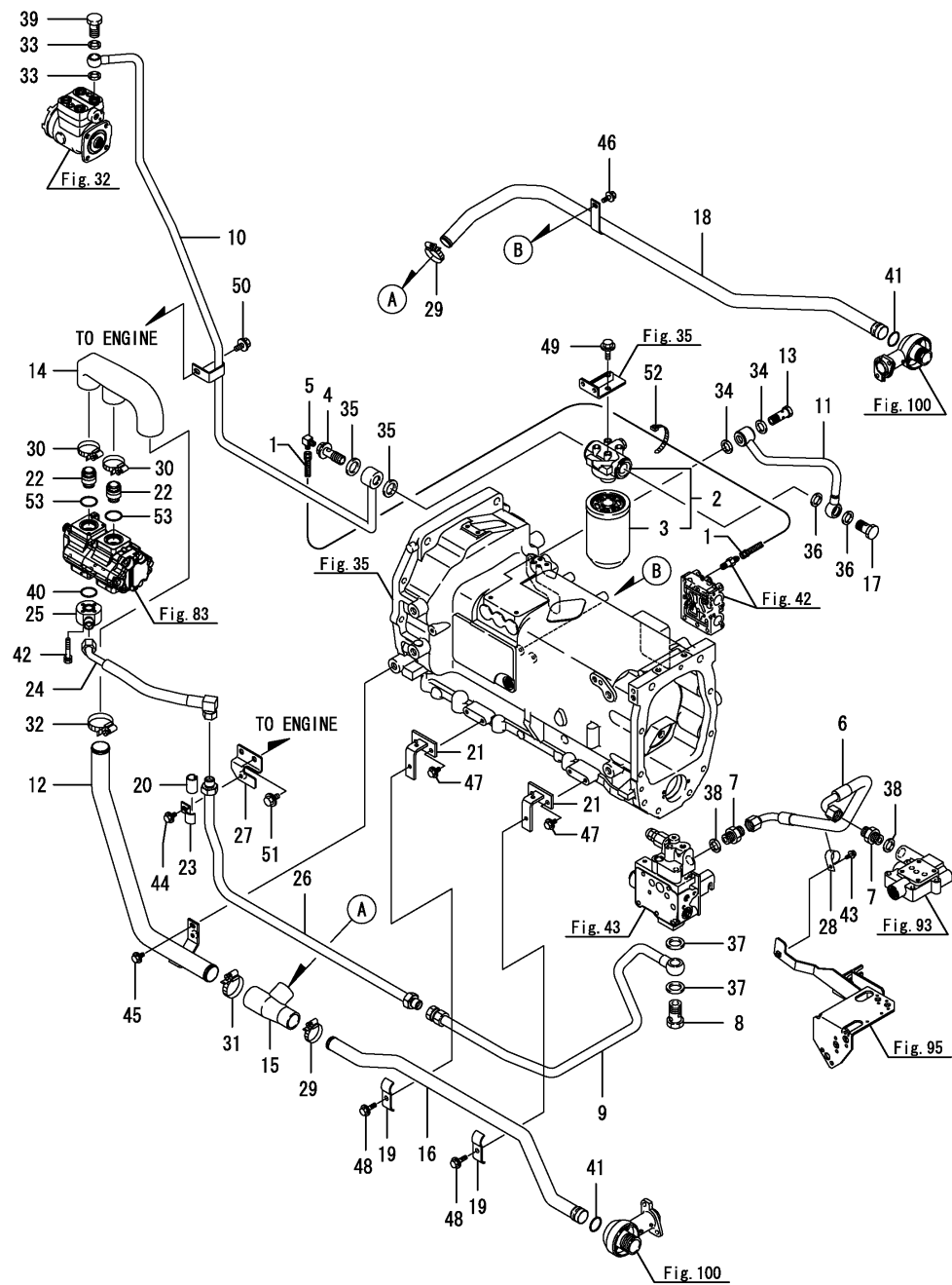
Fig.98. 유압배관(1)
