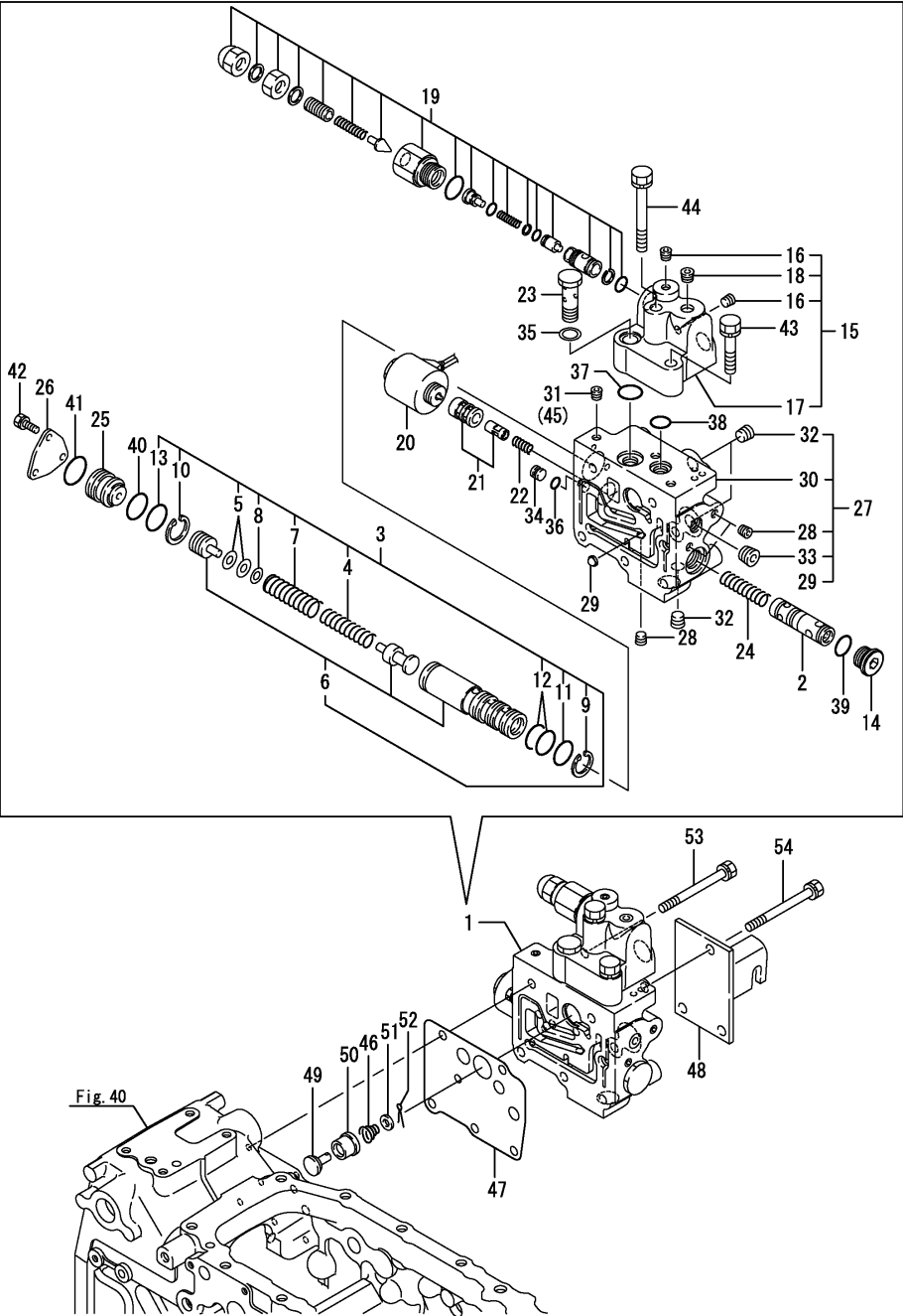
Fig.43. P.T.O. 밸브
