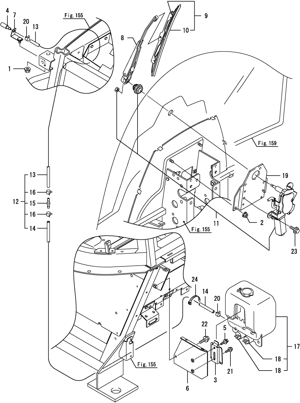
Fig.168. 전방와이퍼
