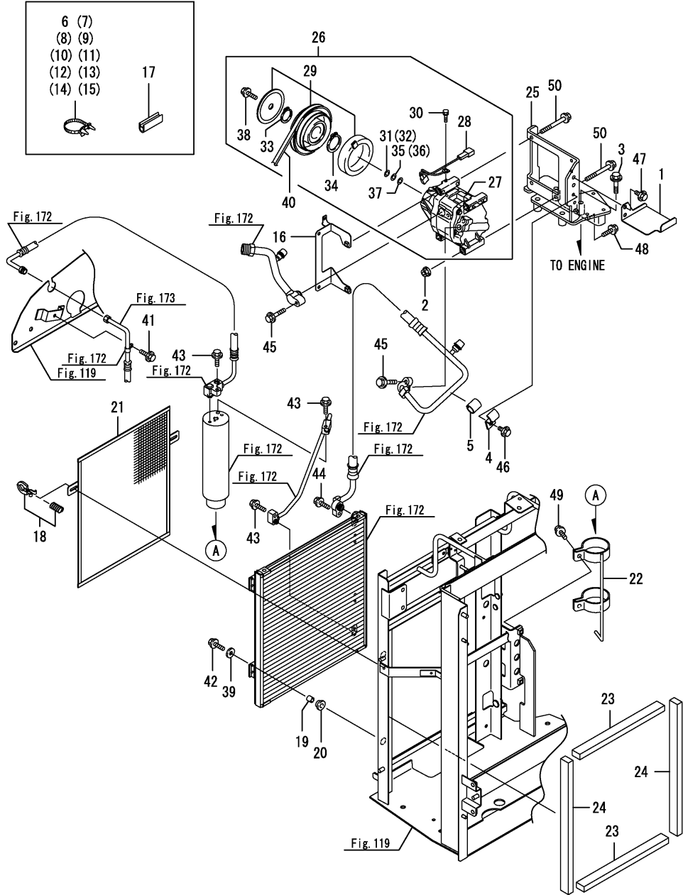
Fig.176. 에어컨(4)
