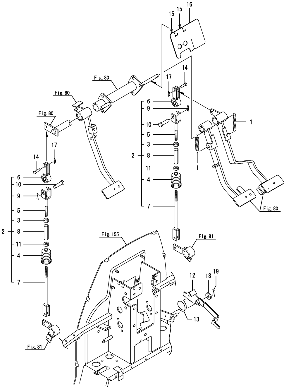
Fig.82. 브레이크링크(2)
