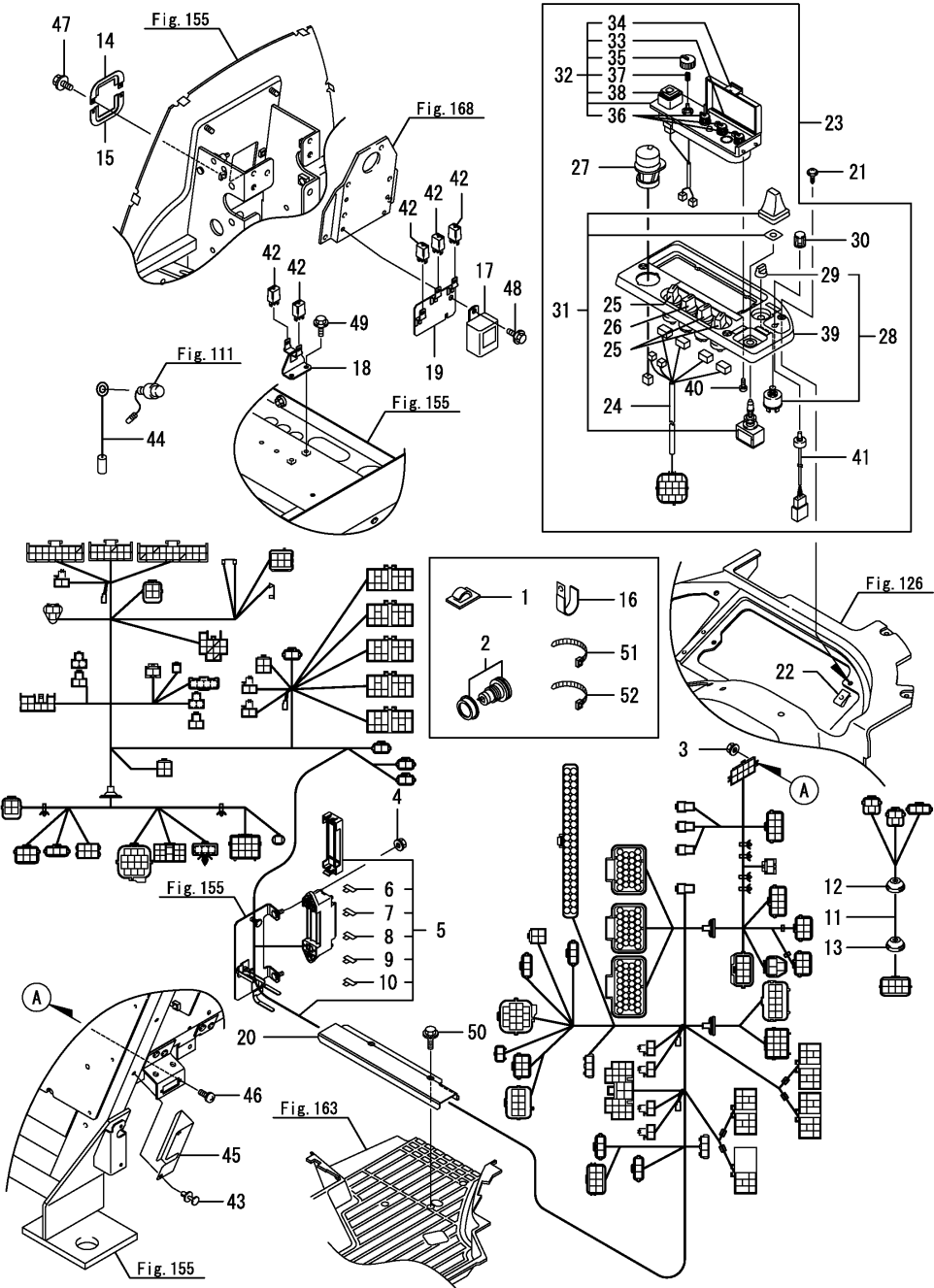
Fig.104. 배선(F)
