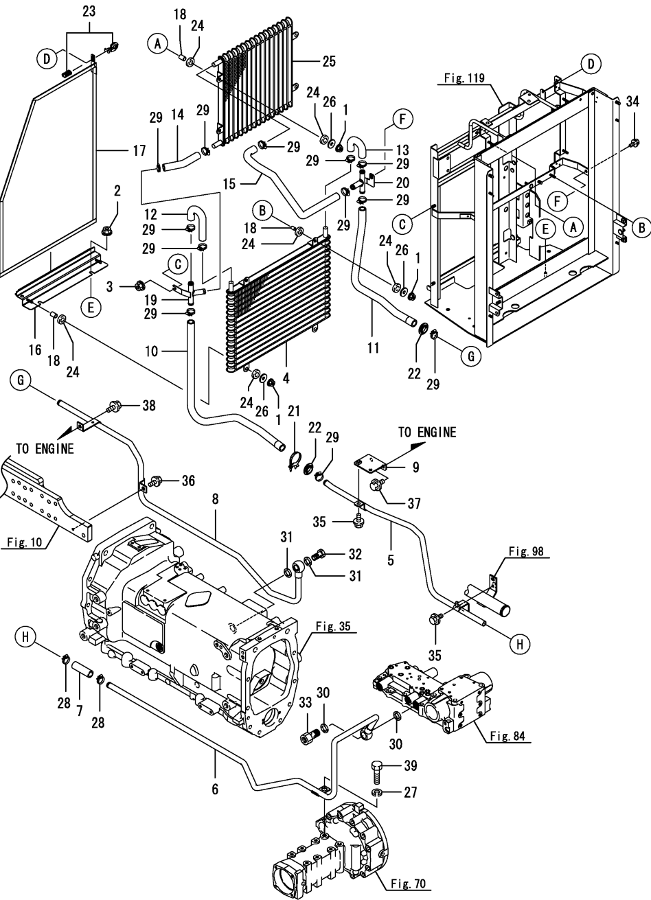
Fig.101. 오일쿨러
