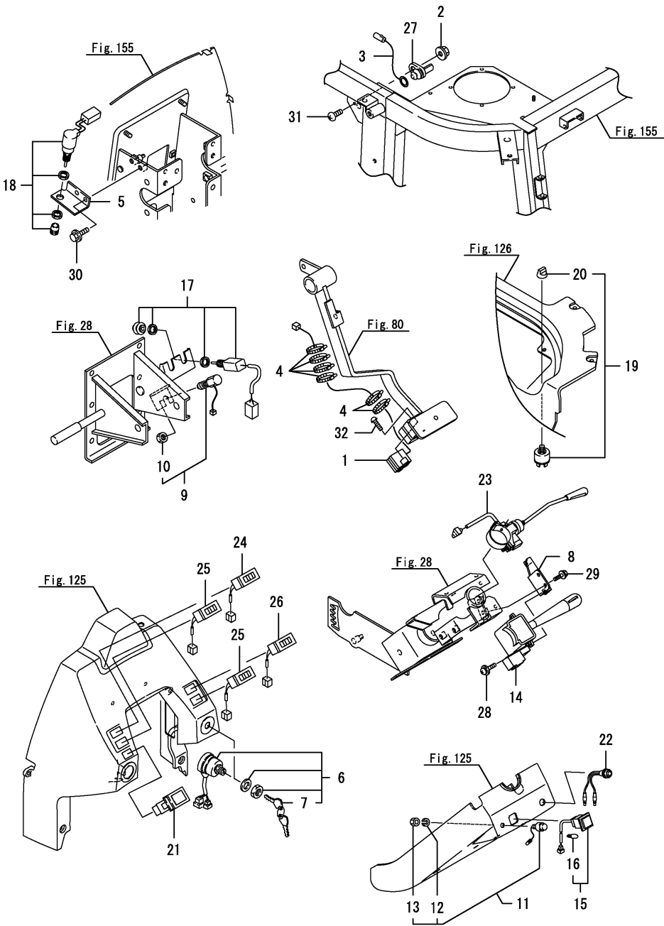
Fig.111. 스위치(2)
