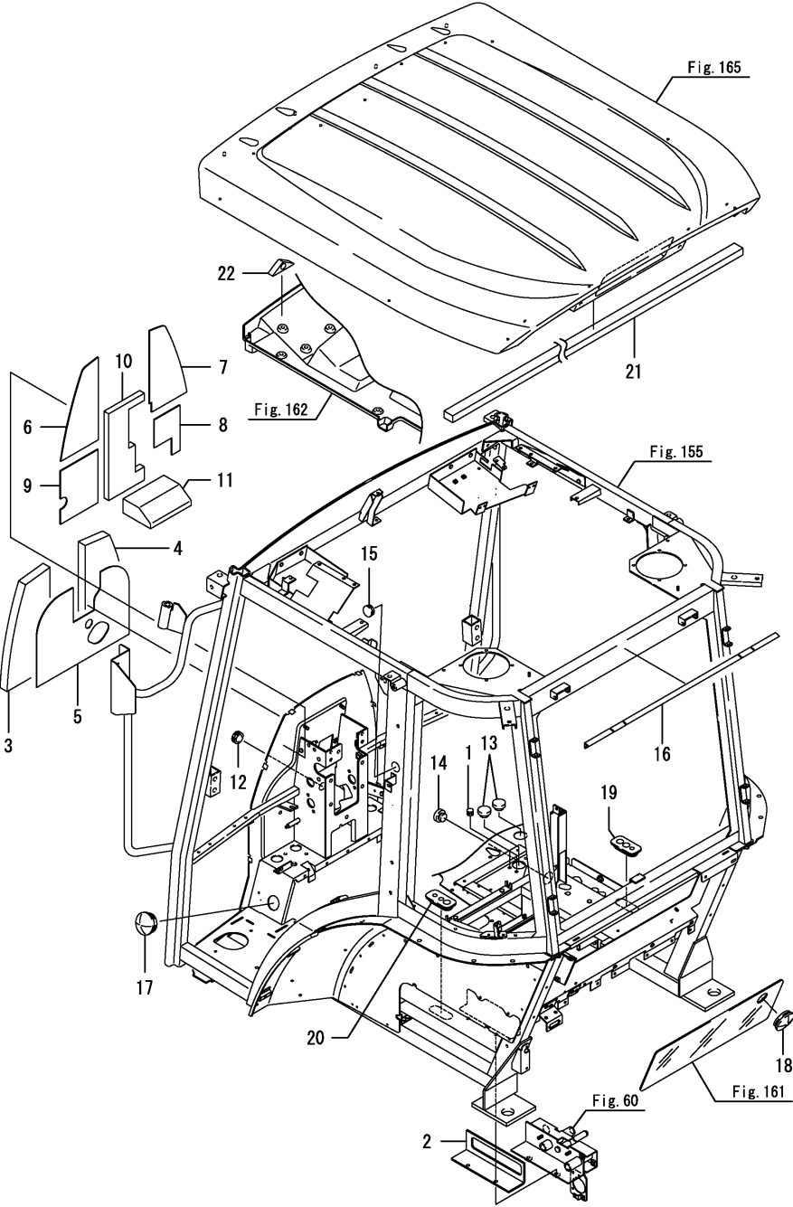
Fig.164. 캐빈시일(2)
