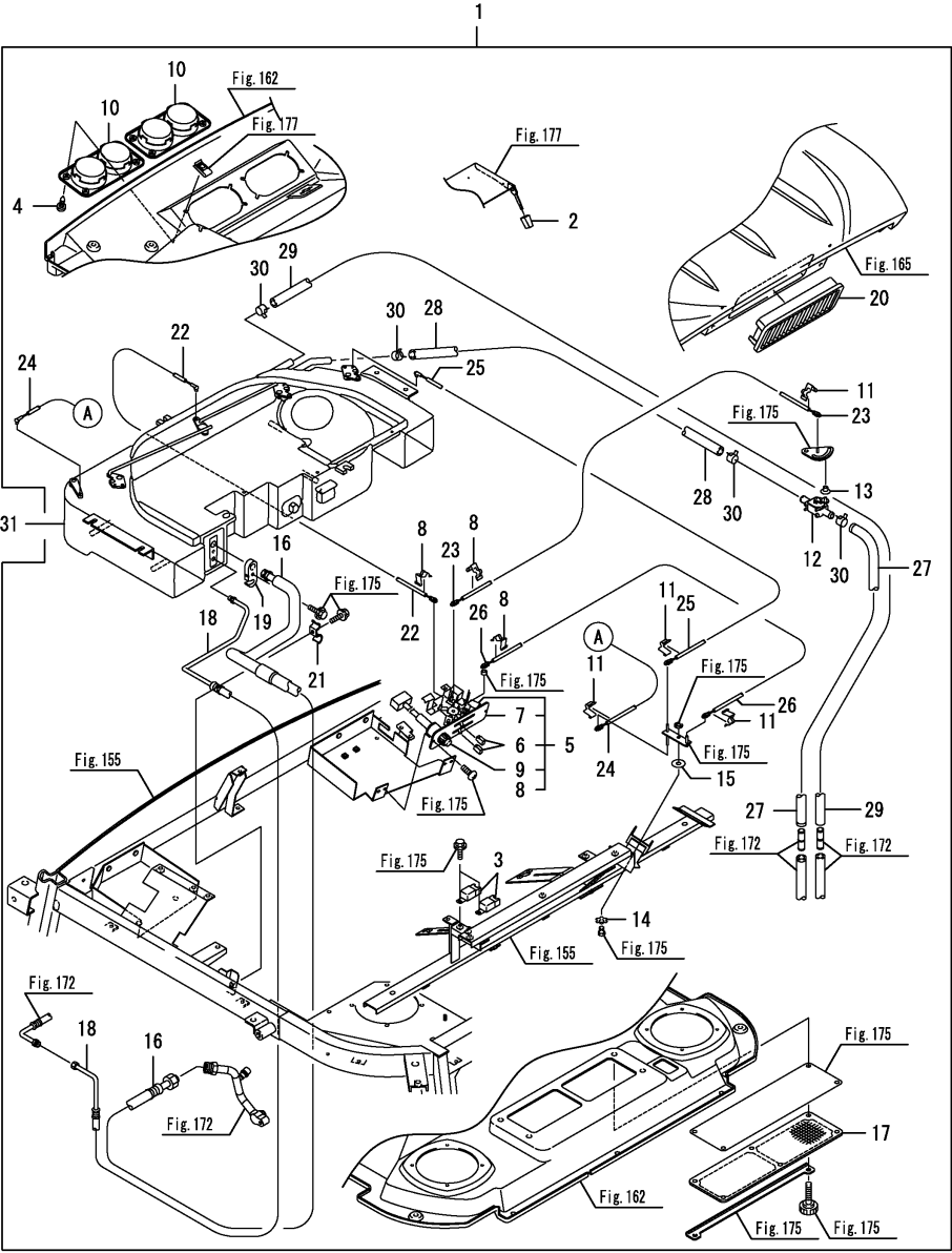
Fig.173. 에어컨(2)
