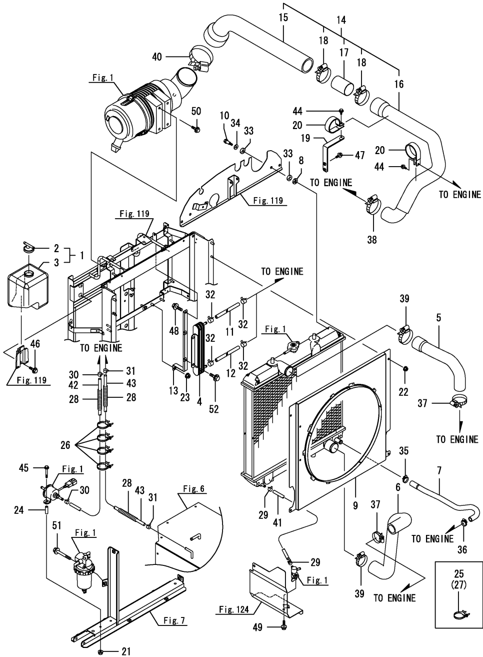
Fig.2. 엔진악세사리
