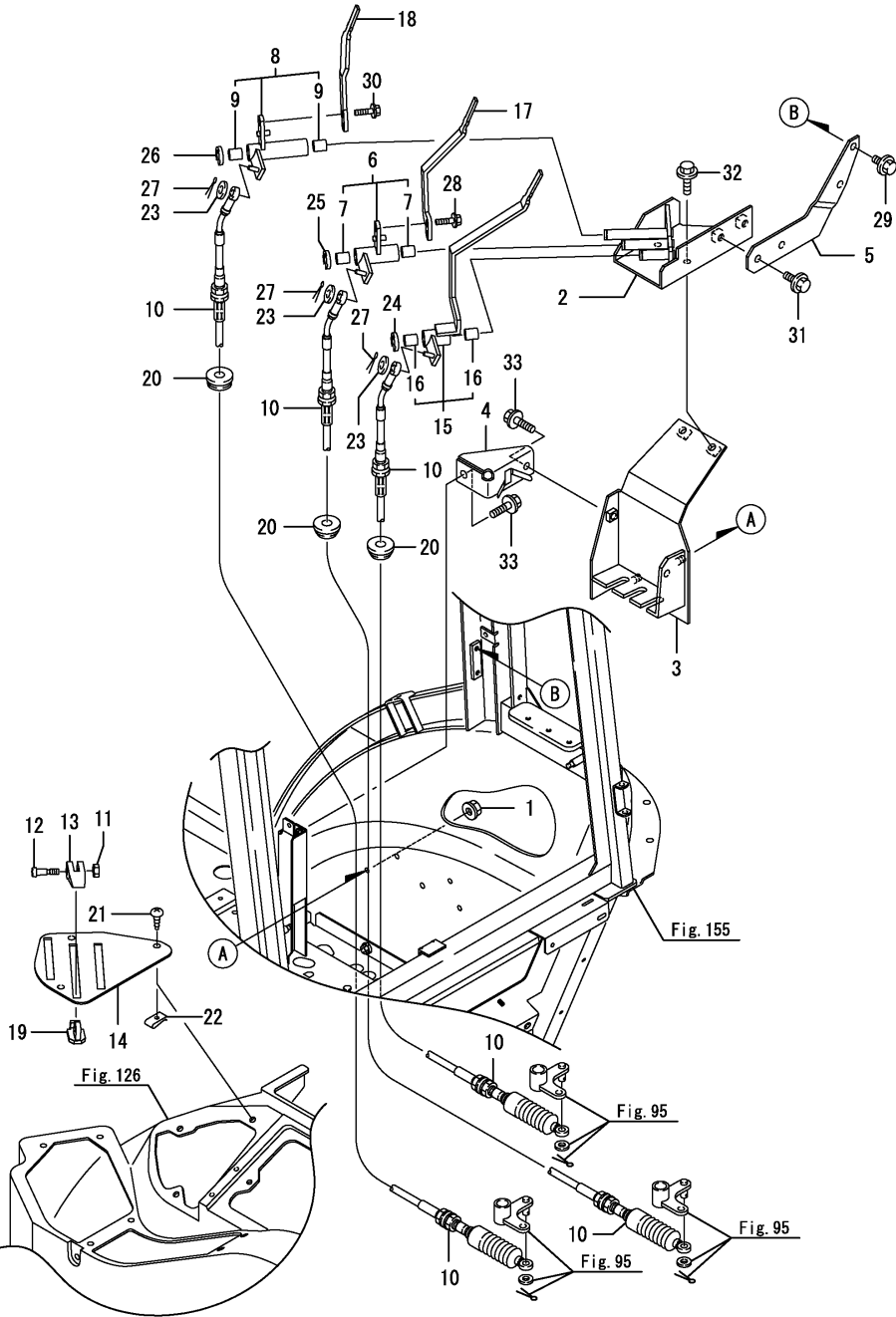
Fig.94. S.C.V.컨트롤(1)
