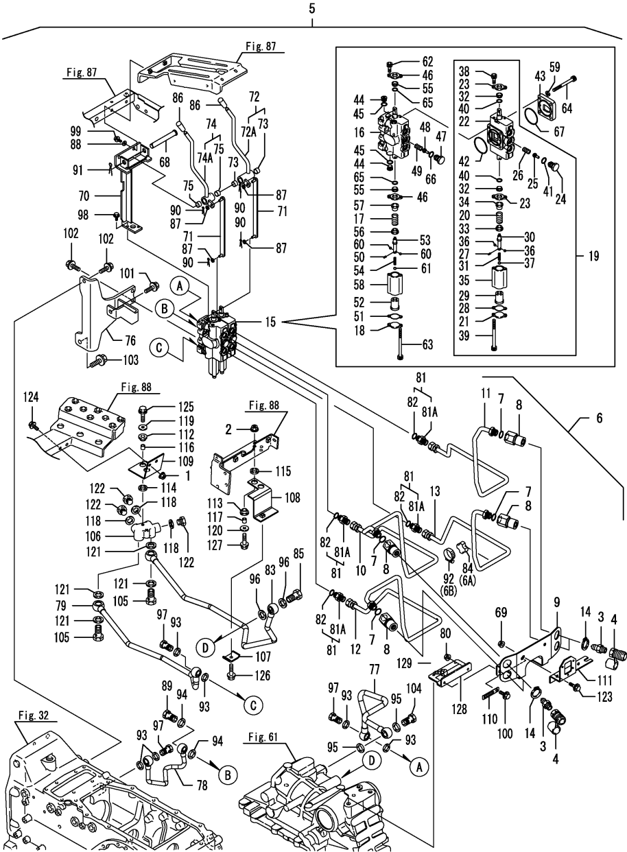
Fig.100. 보조컨트롤밸브
