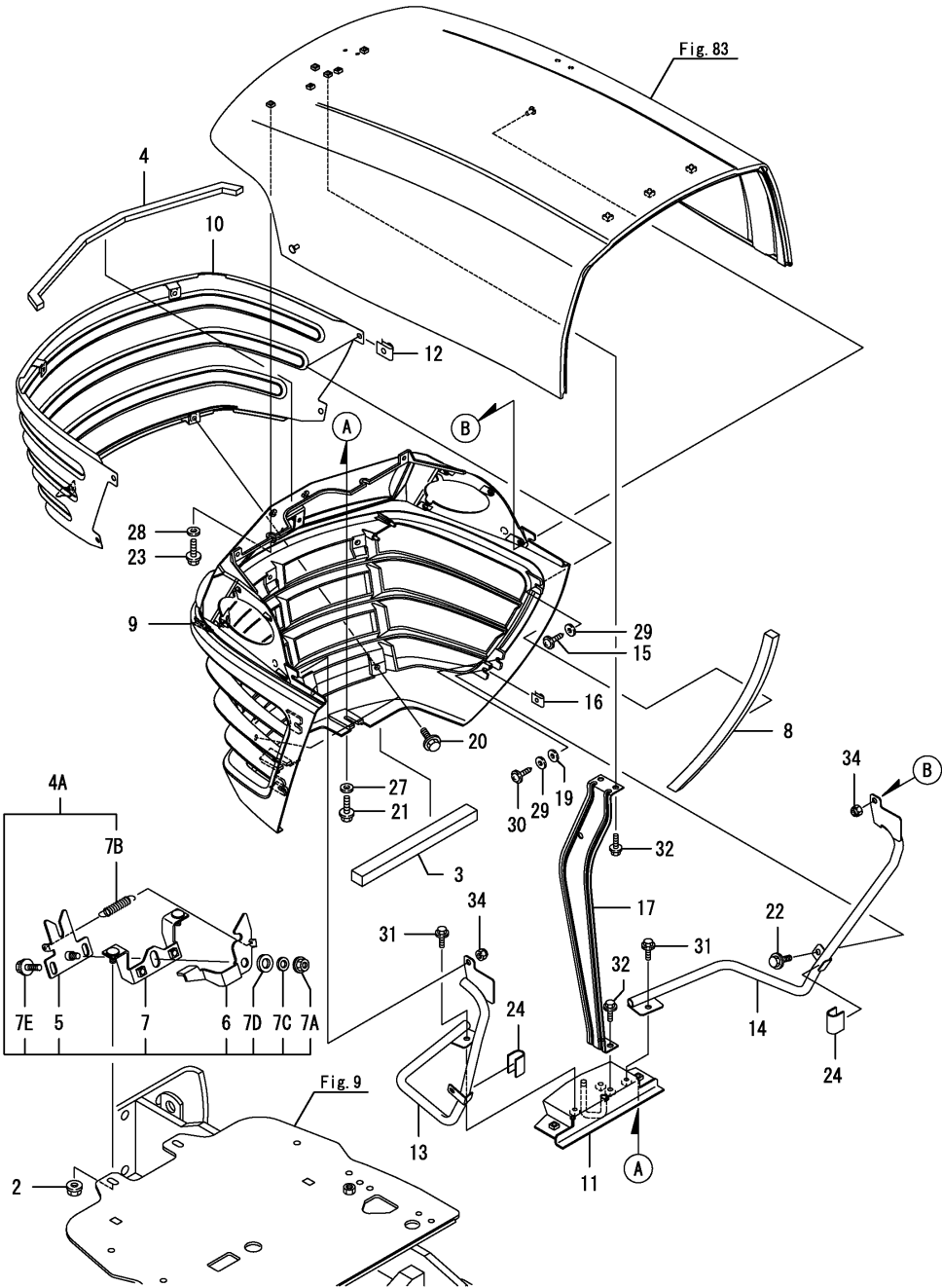
Fig.84. 프론트그릴
