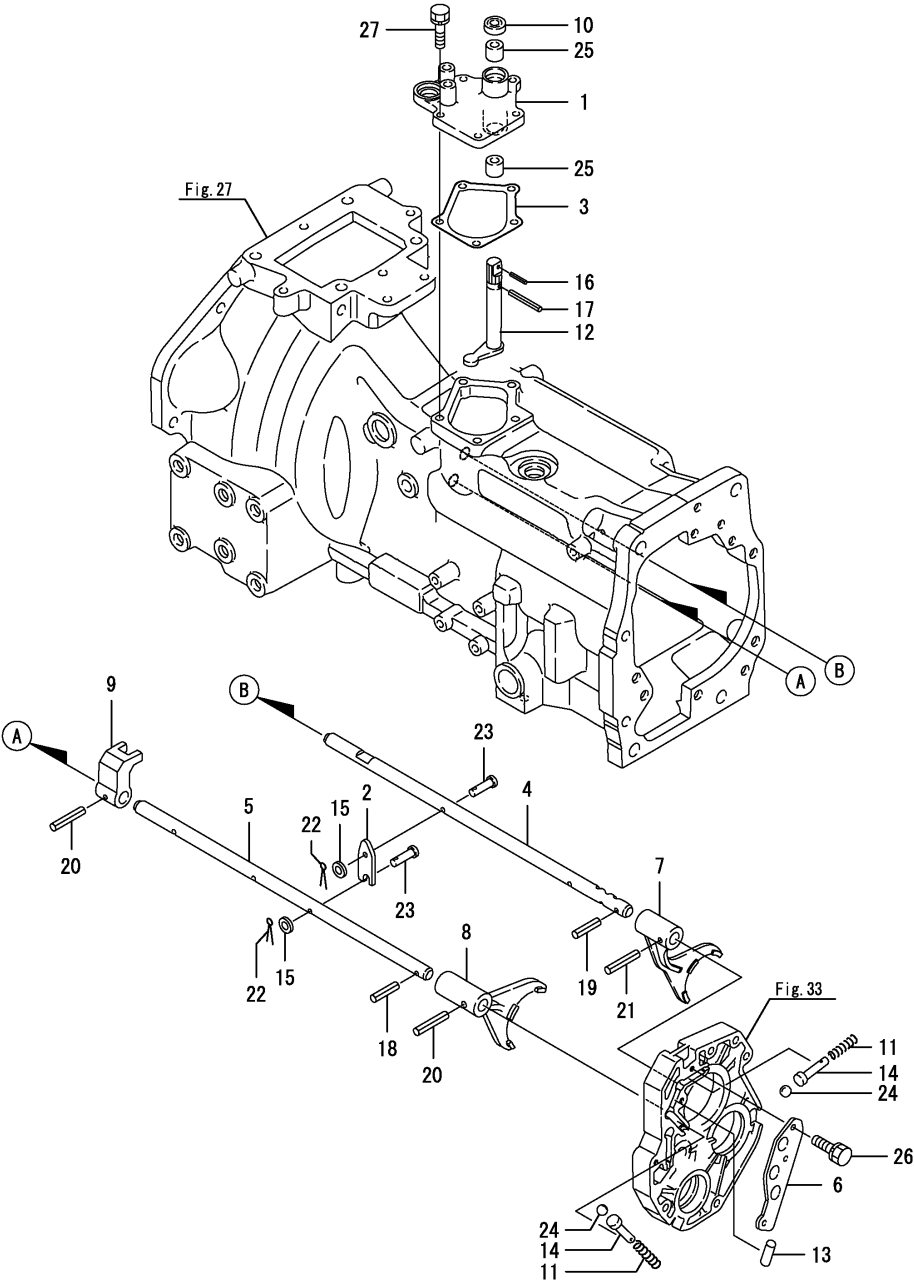
Fig.45. 주변속
