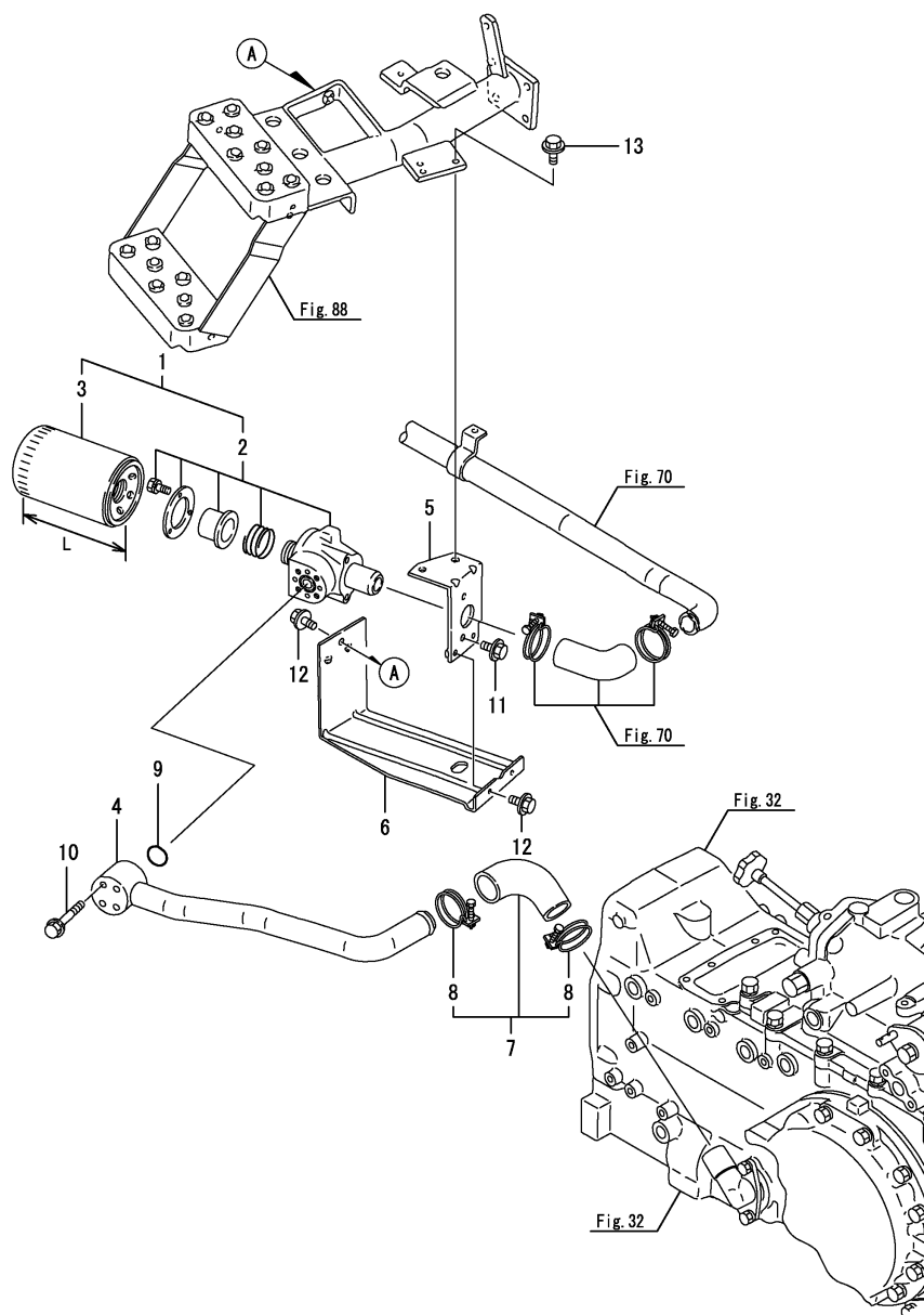
Fig.71. 유압필터
