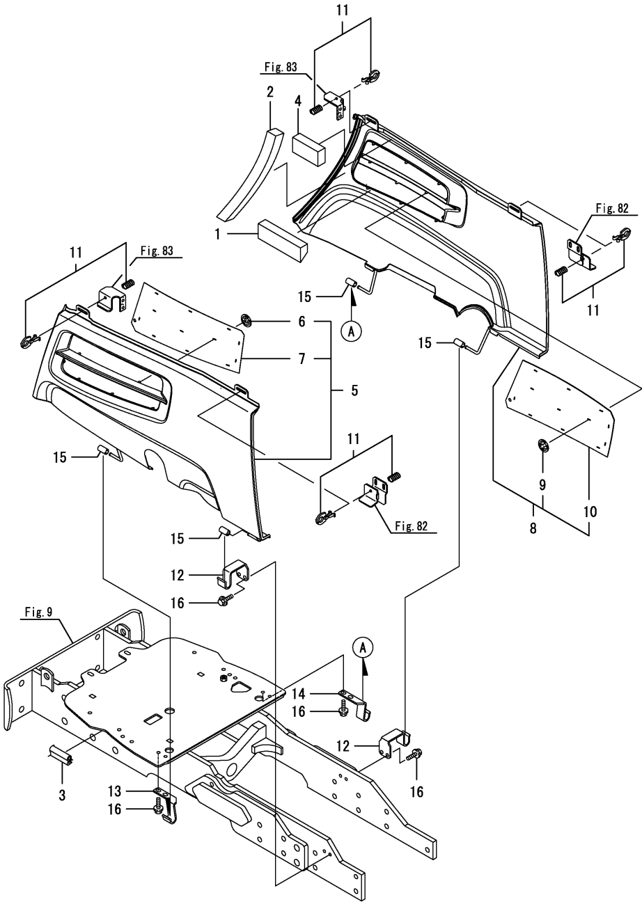
Fig.85. 사이드커버
