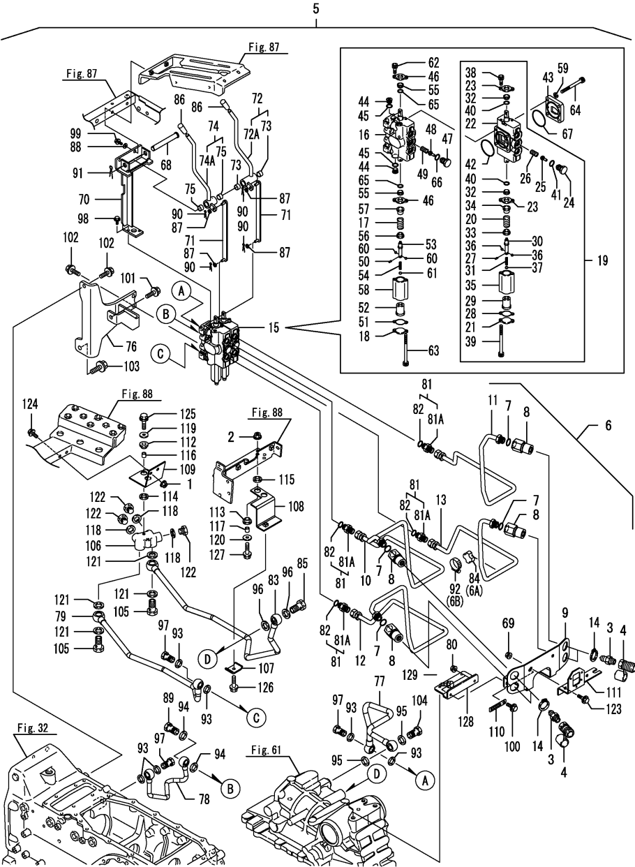
Fig.100. 보조컨트롤밸브
