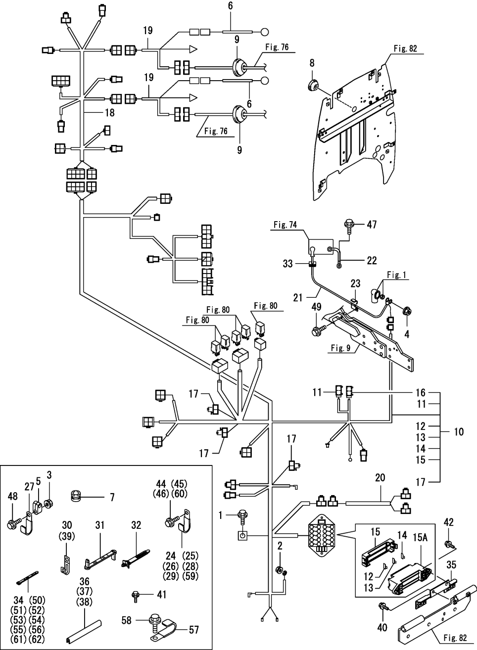
Fig.73. 배선
