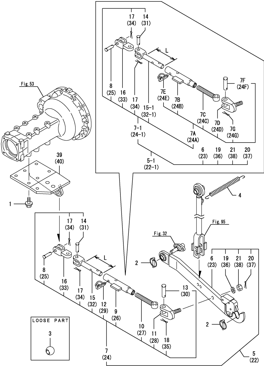
Fig.96. 로워링크&체크체인
