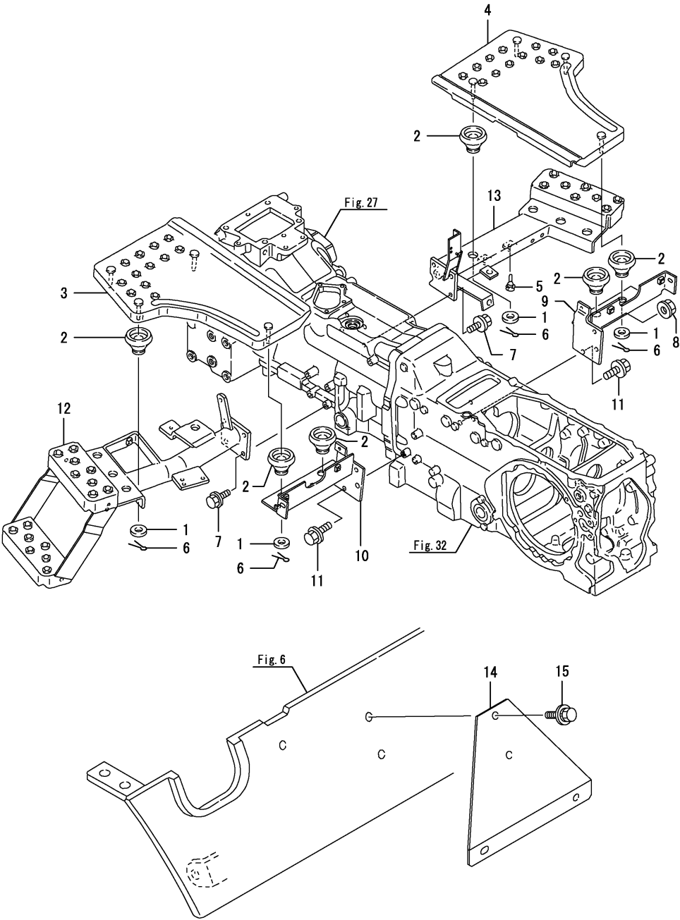
Fig.88. 발판
