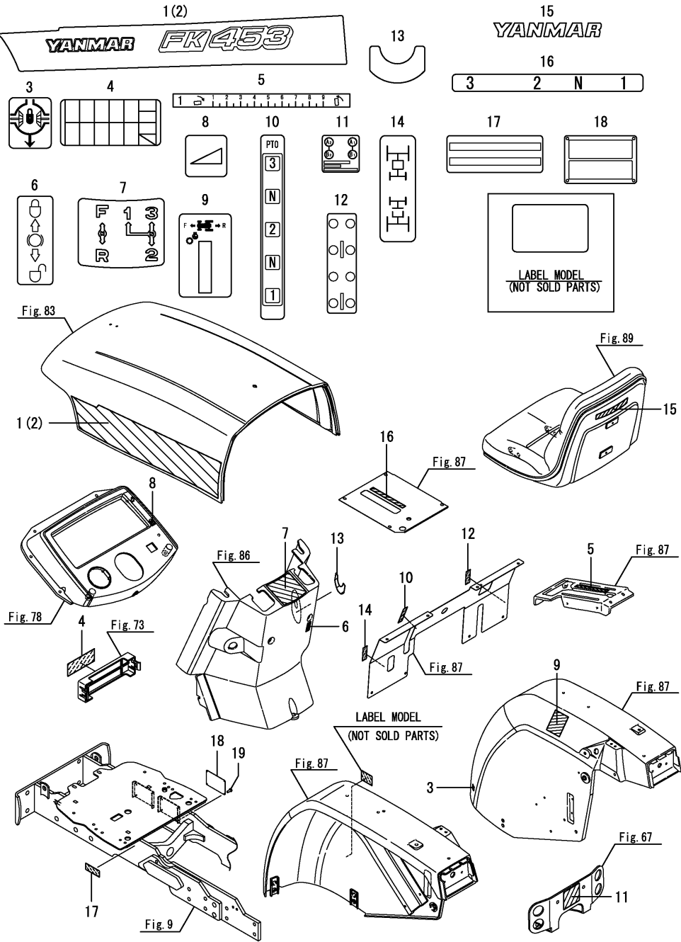
Fig.91. 명판
