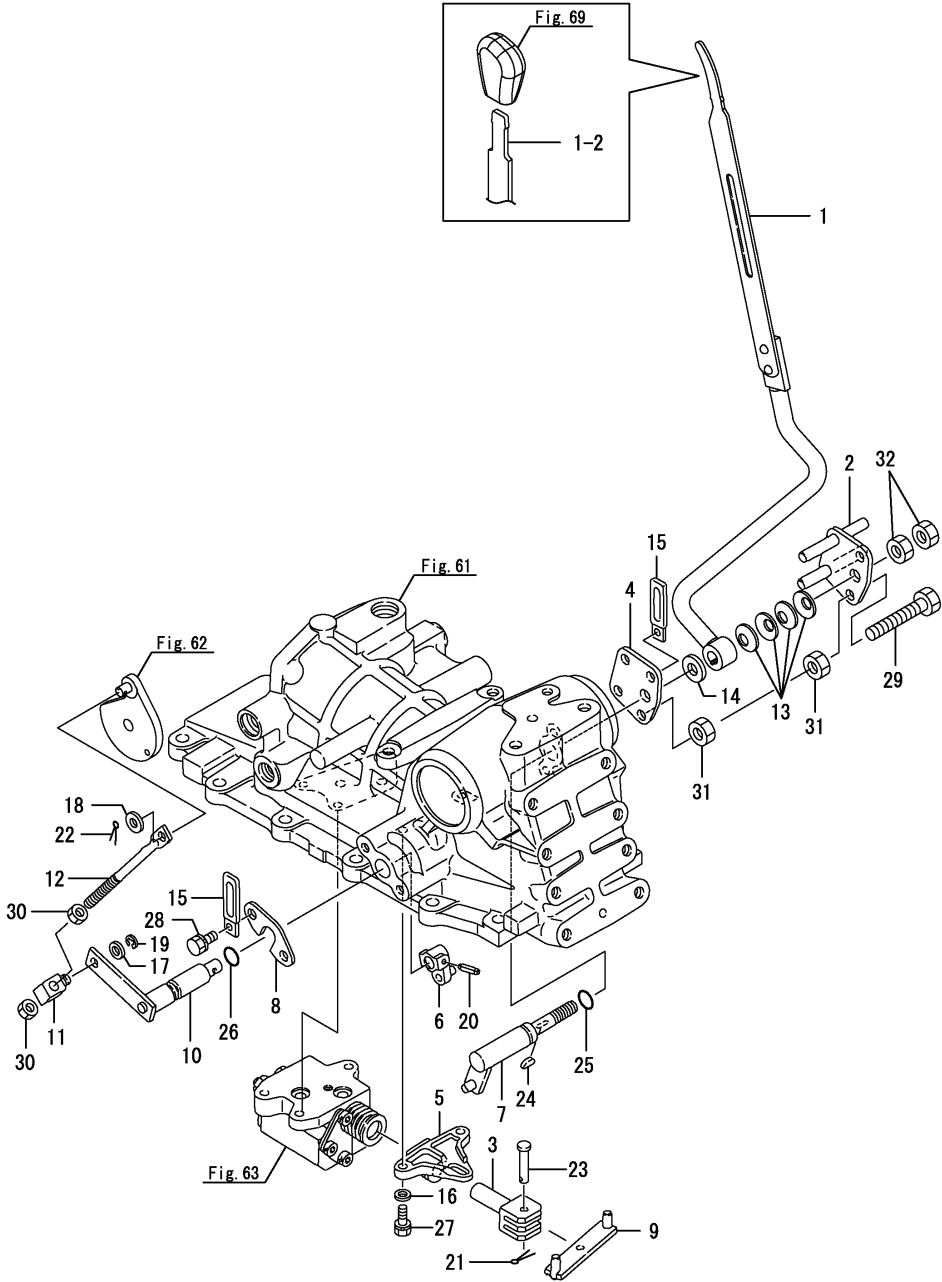
Fig.68. 유압컨트롤
