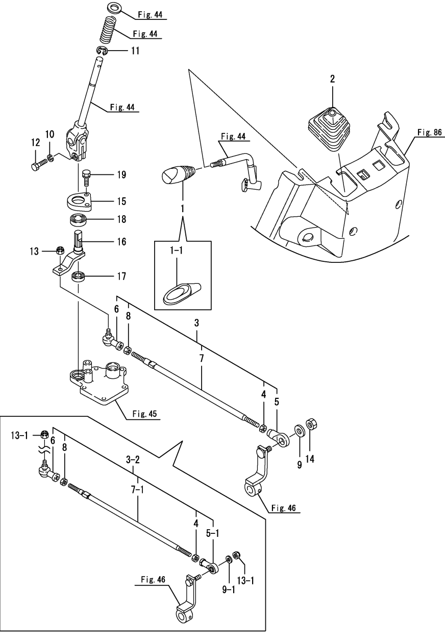
Fig.47. 리버서레버
