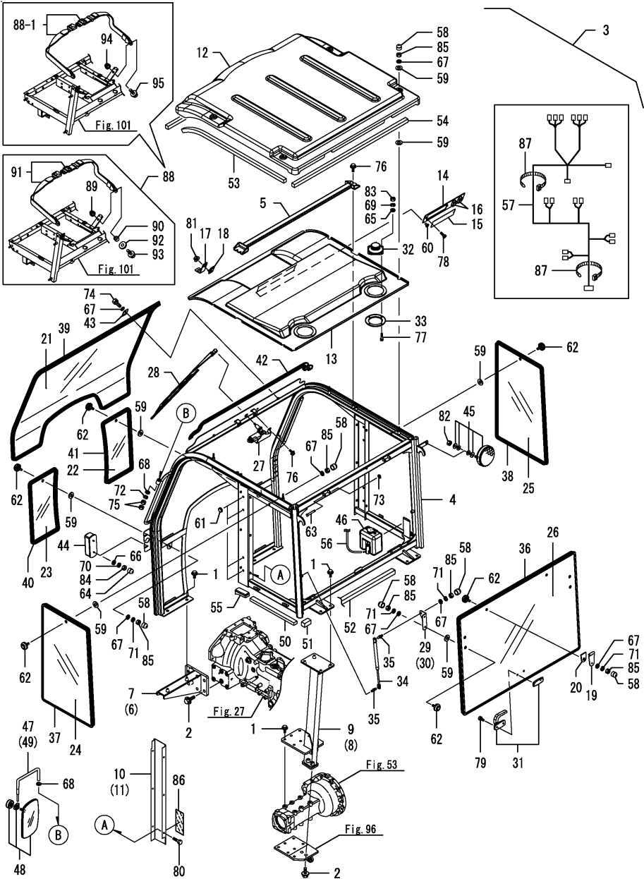
Fig.102. 안전프레임
