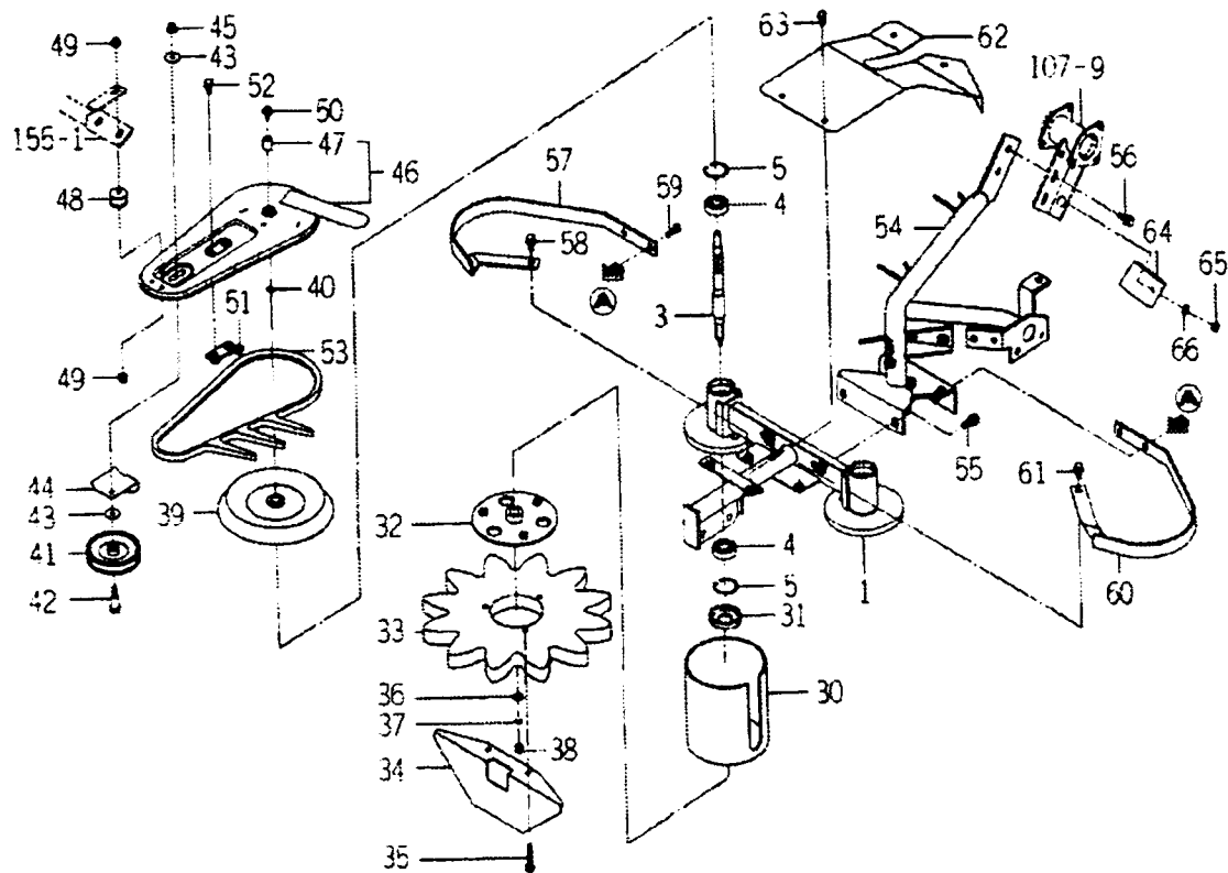
FIG. 114 소입(센터/RH) 관계(그림2/2)
