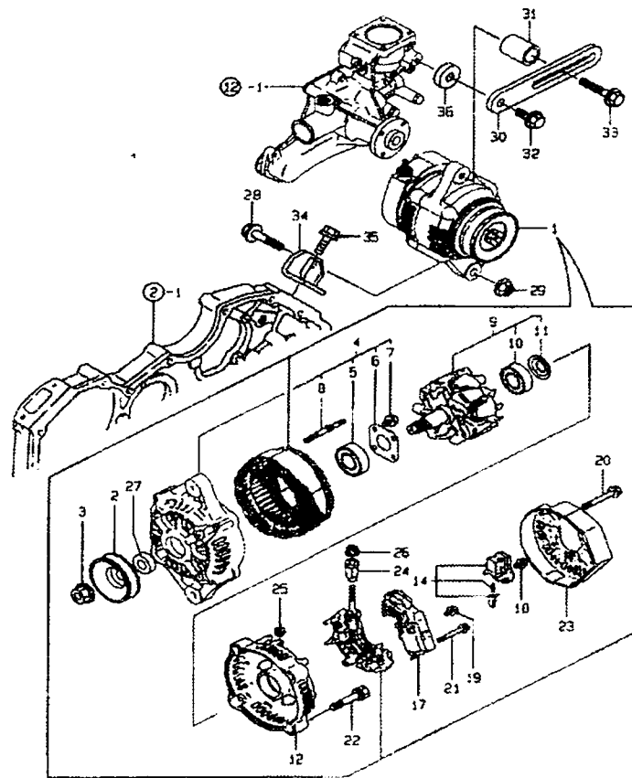
FIG.018 제네레이터
