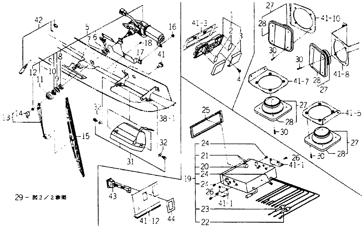
FIG. 45 와이퍼,라디오 관계(C형)(그림1/2)
