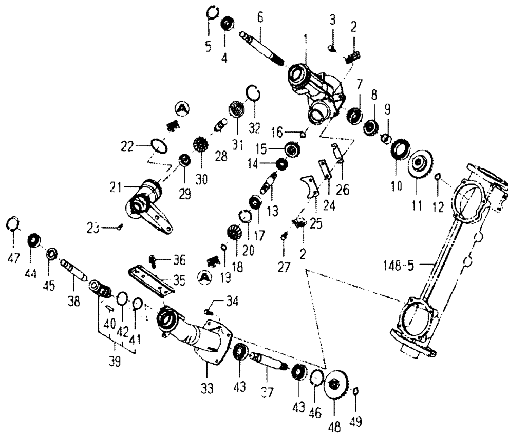
FIG. 149 기어케이스(근원/RH,센터) 관계
