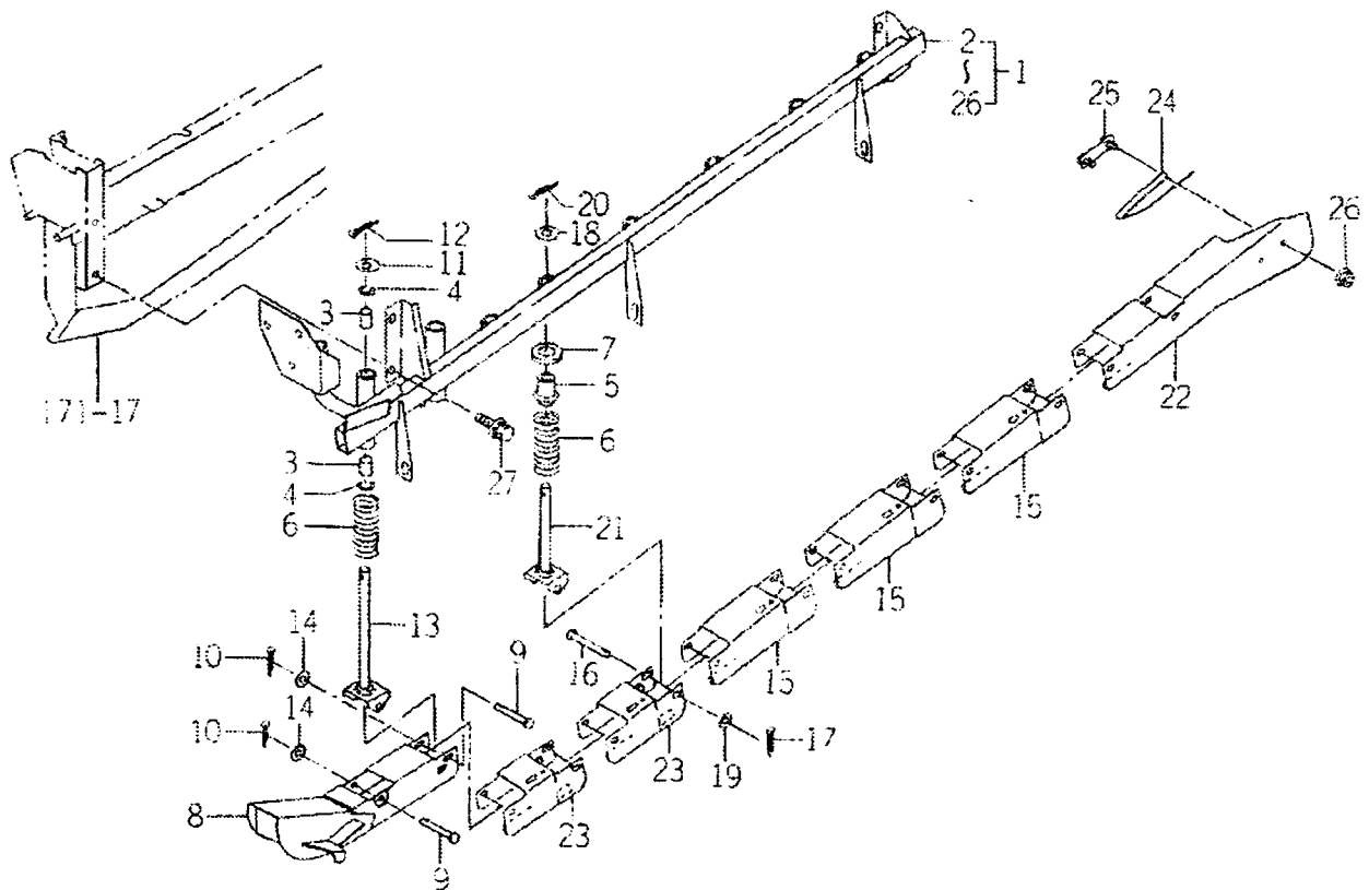
FIG.187 체인 관계
