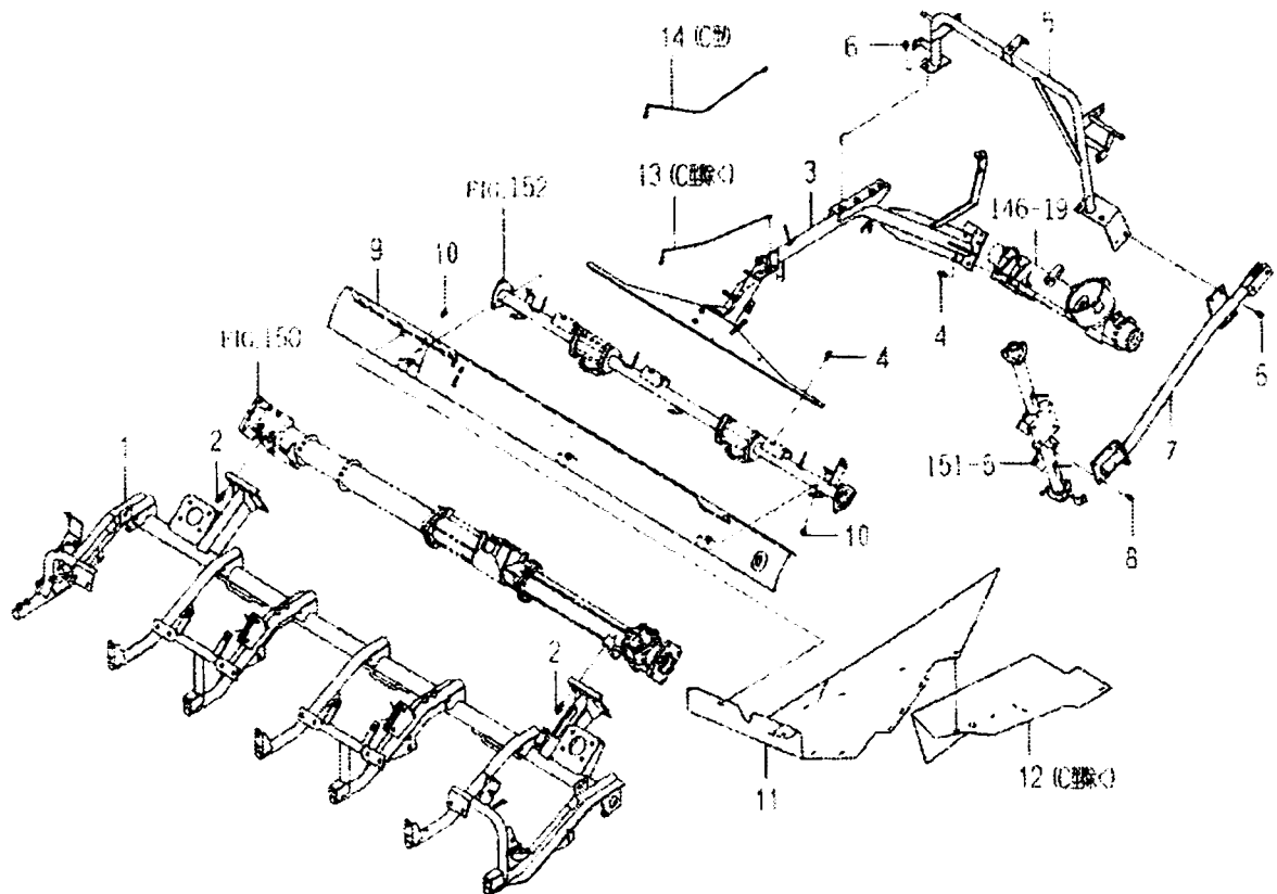
FIG. 155 프레임(프론트), 커버(어퍼) 관계
