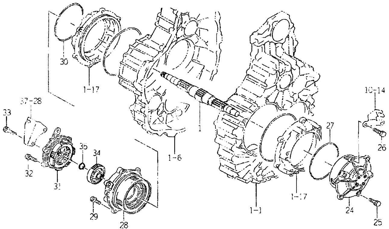
FIG. 5 유성(플래니터리)기어 관계 (그림2/2)
