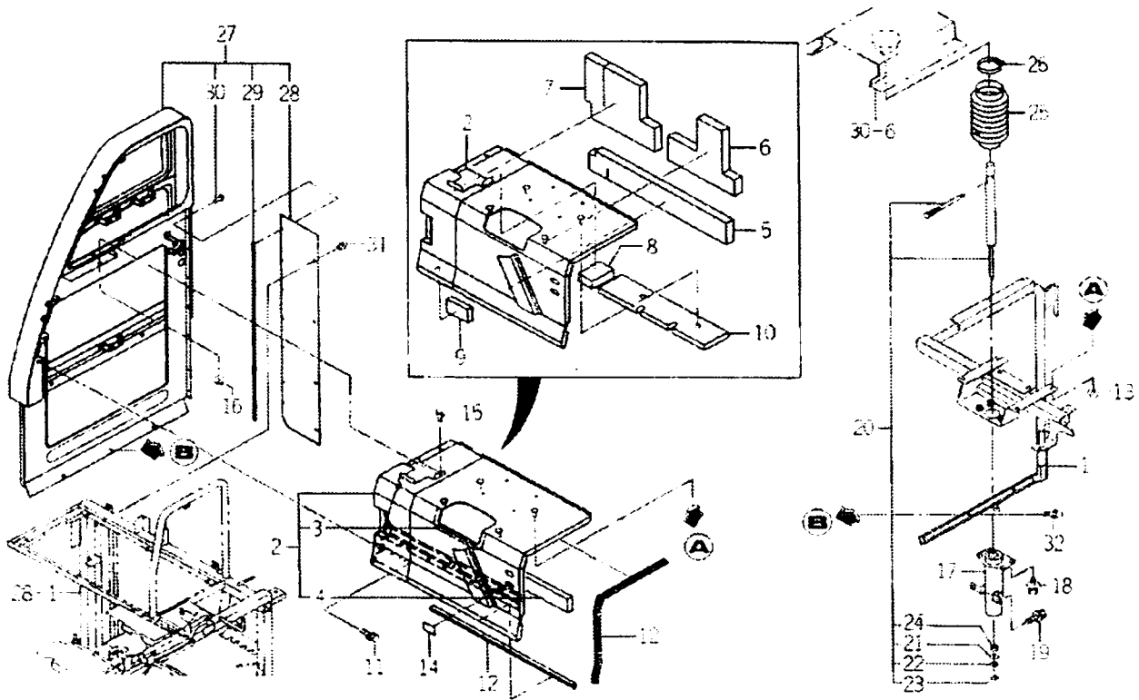
FIG.76 프레임(시트) 관계(C형제외) (그림1/3)
