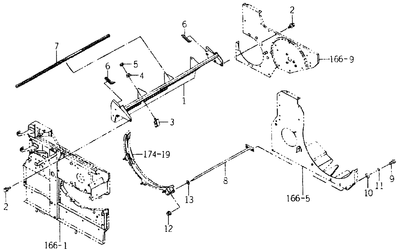
FIG.175 망퇴 상부 관계
