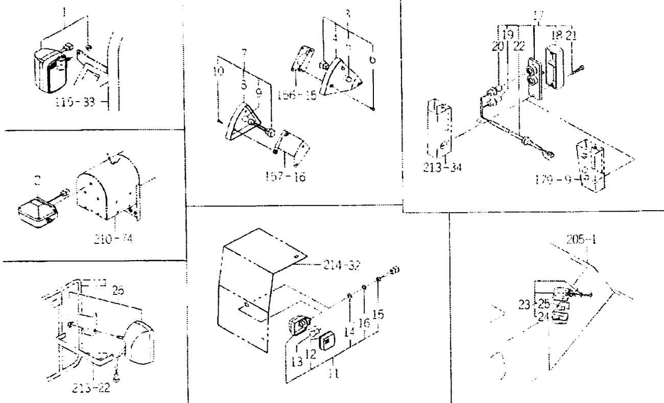
FIG. 64 라이트,윙커 관계
