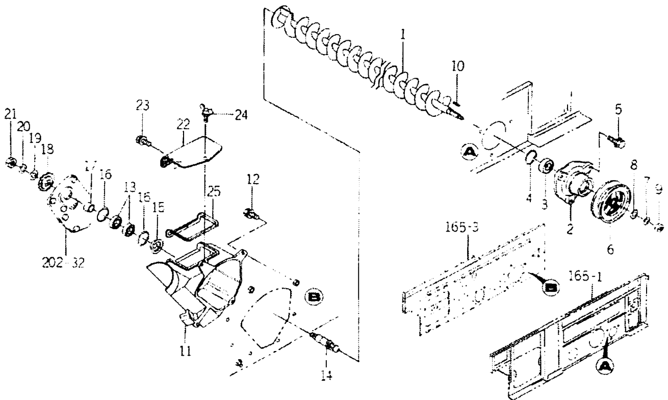
FIG.201 2번(1) 관계
