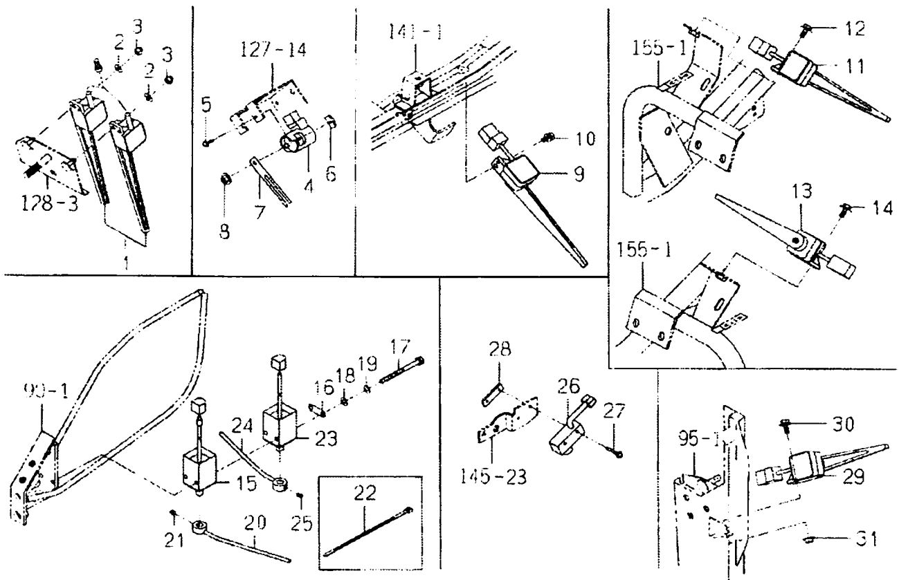
FIG. 62 센서(예취) 관계
