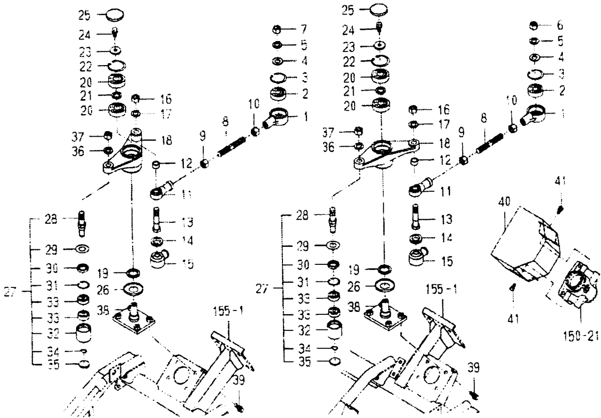
FIG. 111 예취날 구동 관계
