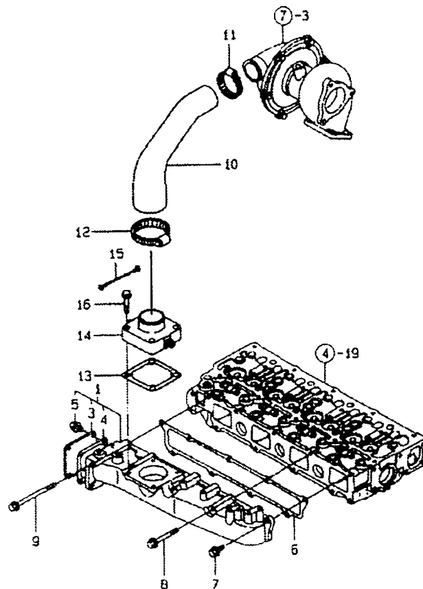
FIG.005 흡기 매니폴드
