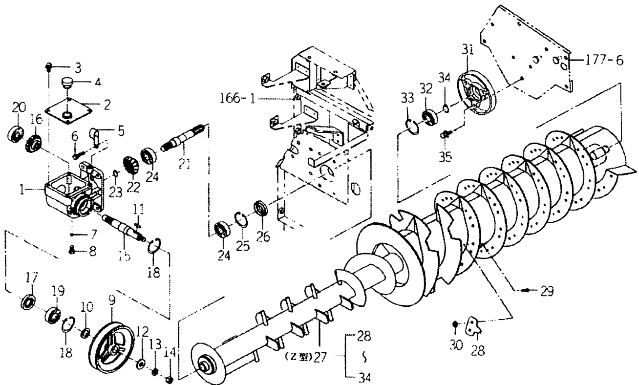
FIG.176 처리통 관계(그림1/2)
