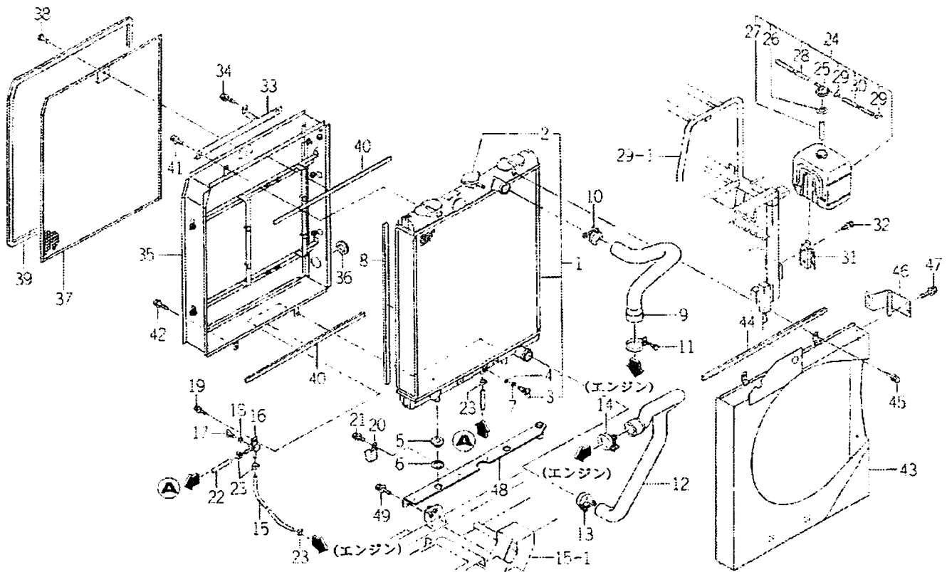
FIG. 71 라디에이터 관계(C형)
