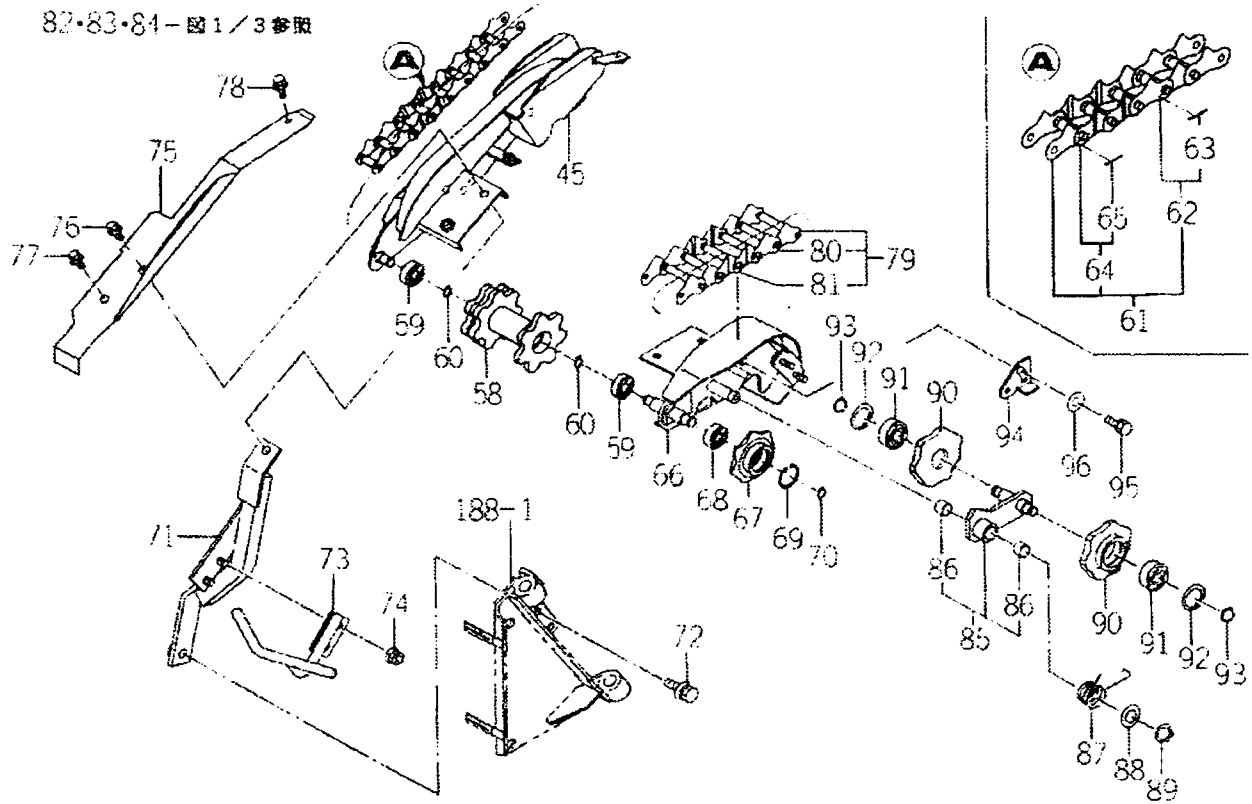
FIG.189 싱크로 관계 (그림3/3)
