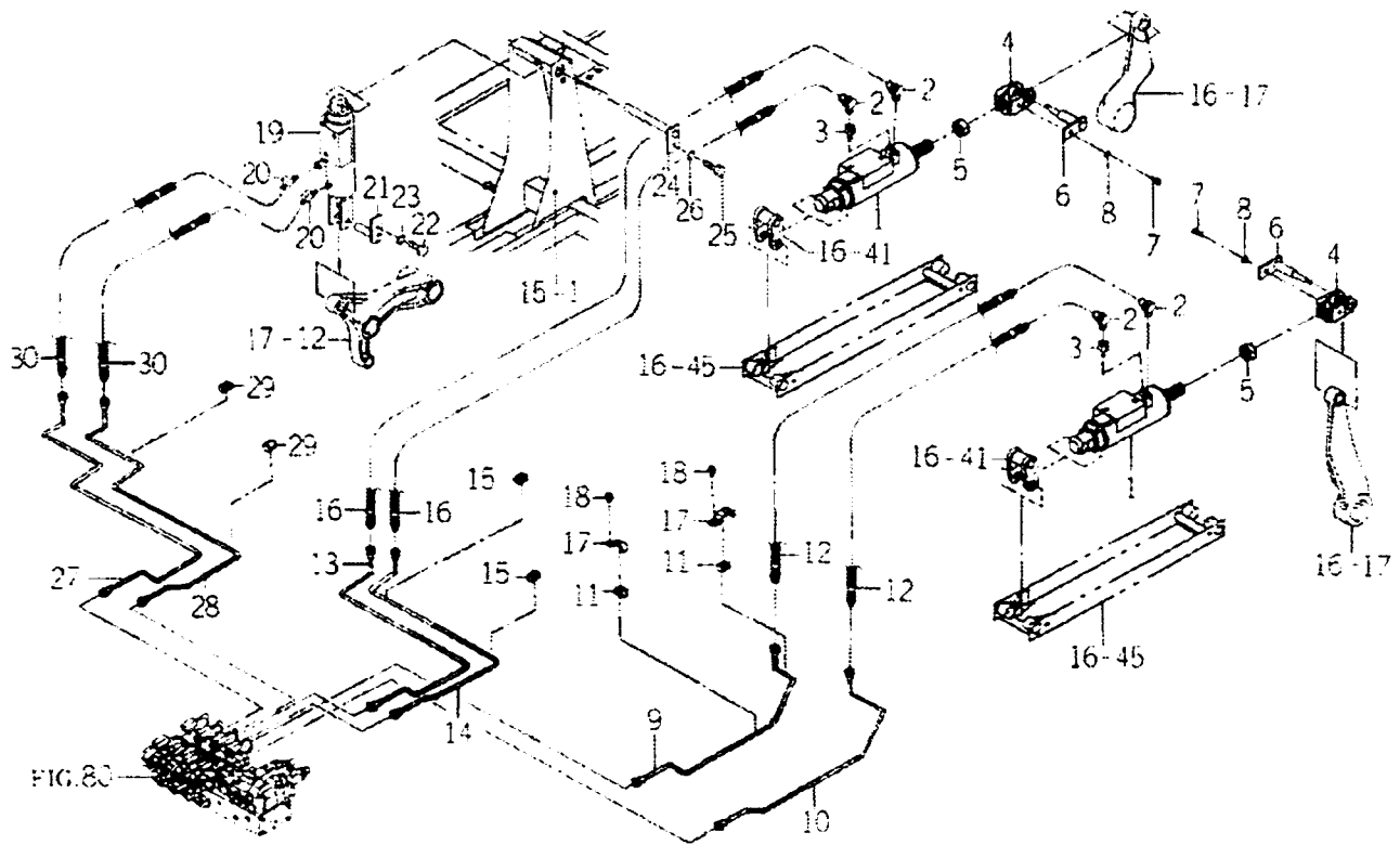
FIG.86 실린더 관계
