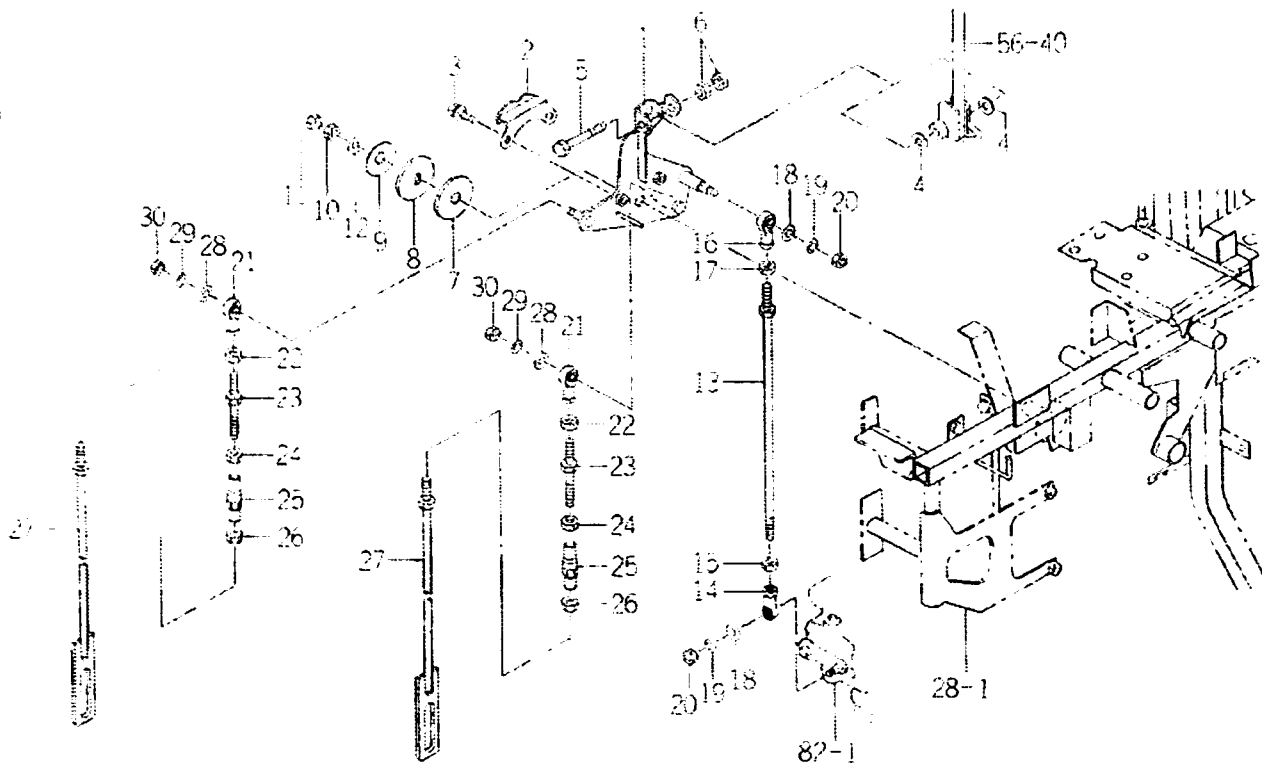
FIG. 32 레버(HST) 관계(그림1/2)
