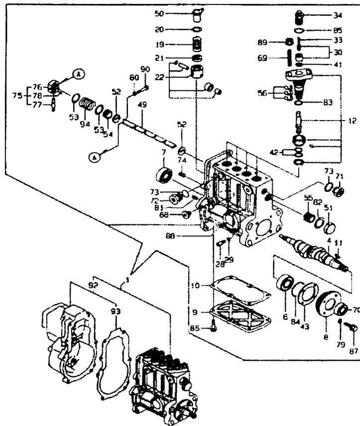
FIG.013 FO 분사 펌프
