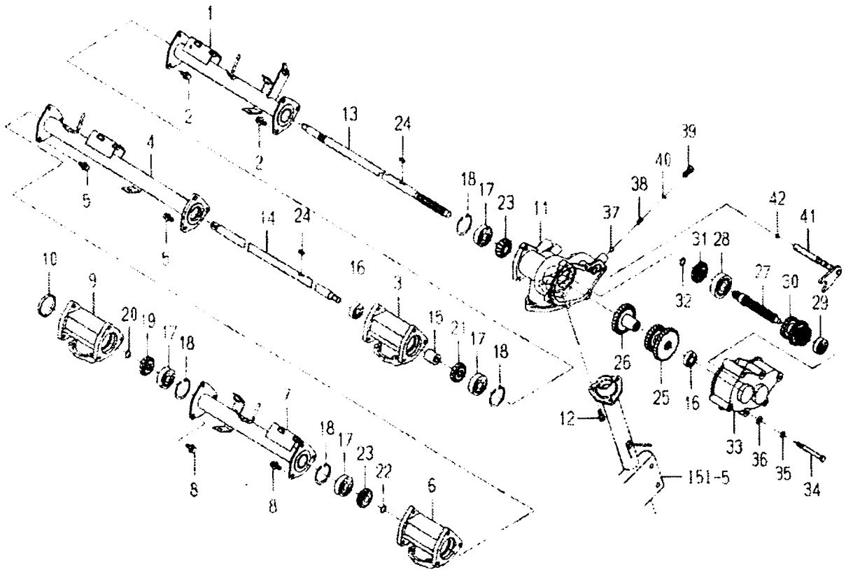
FIG. 152 기어케이스(어퍼) 관계
