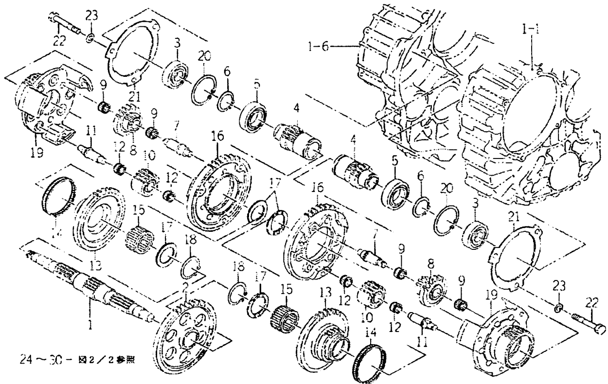
FIG. 5 유성(플래니터리)기어 관계 (그림1/2)
