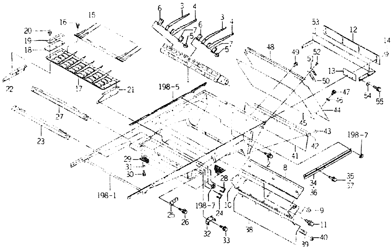
FIG.199 요동 시브 관계
