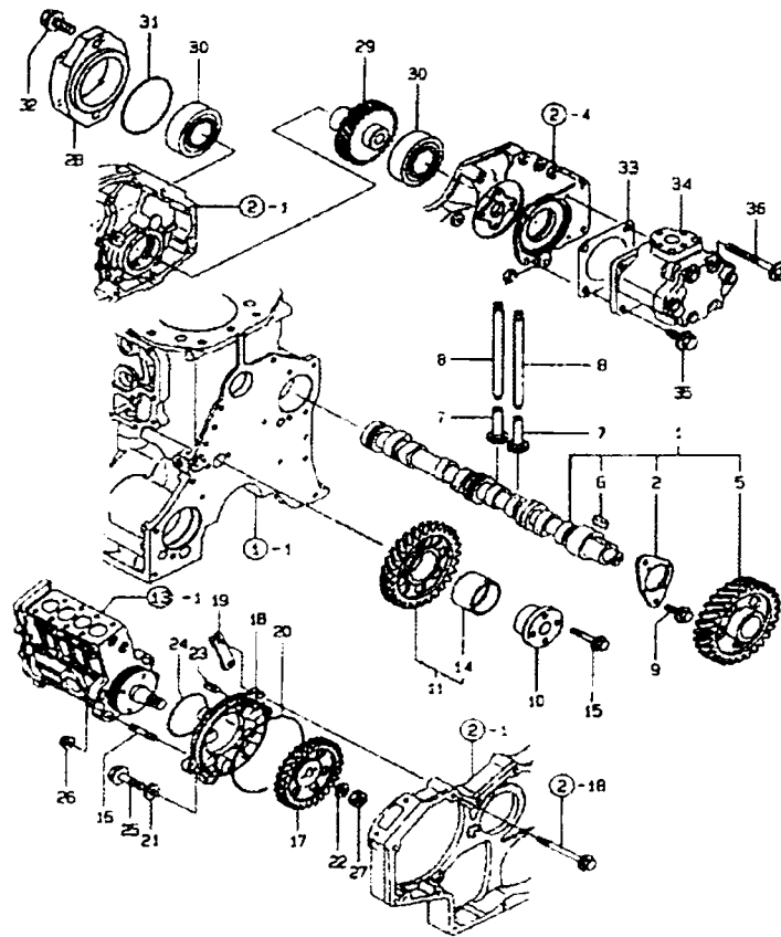
FIG.008 캠 샤프트
