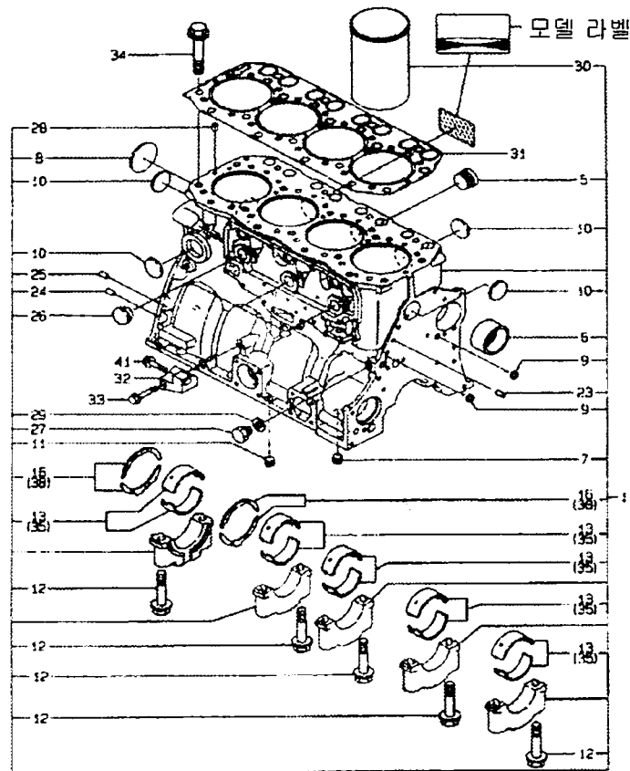
FIG.001 실린더 블록
