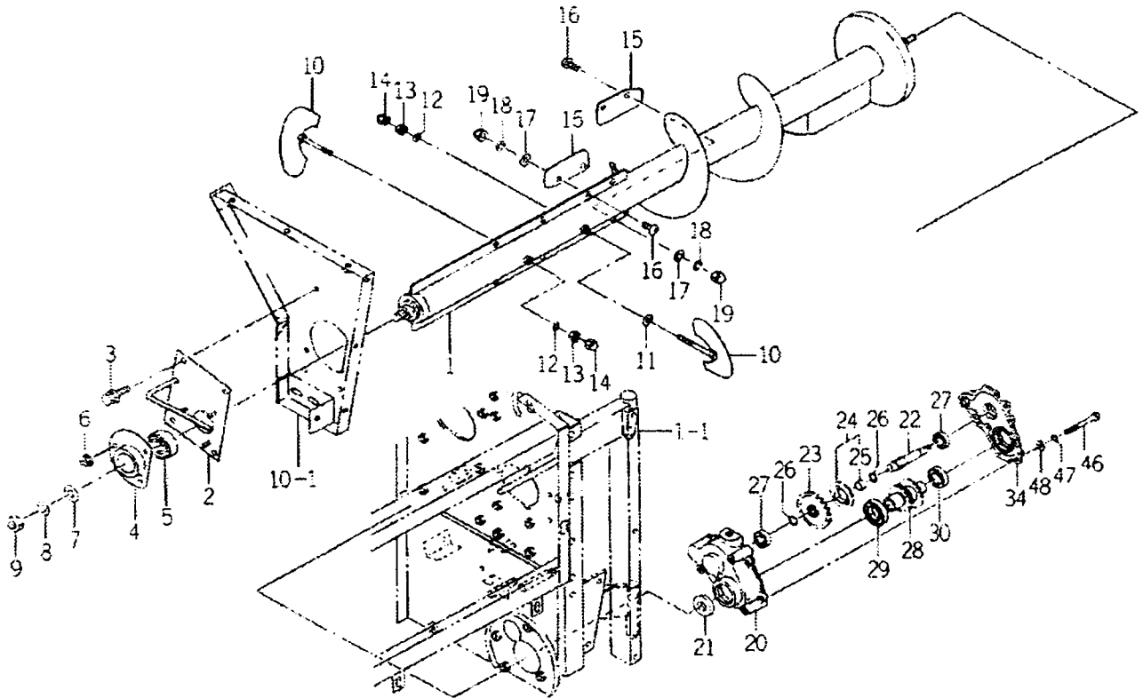
FIG.6 확산축 관계 (그림1/3)
