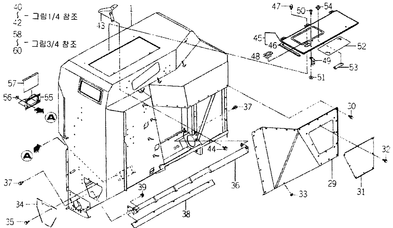
FIG.205 탱크 관계 (그림2/4)
