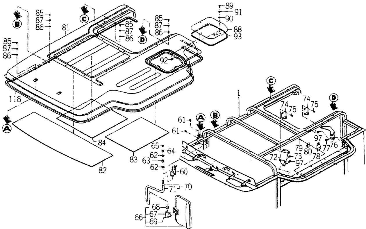
FIG. 38 캐빈프레임 관계(C형)(그림3/4)
