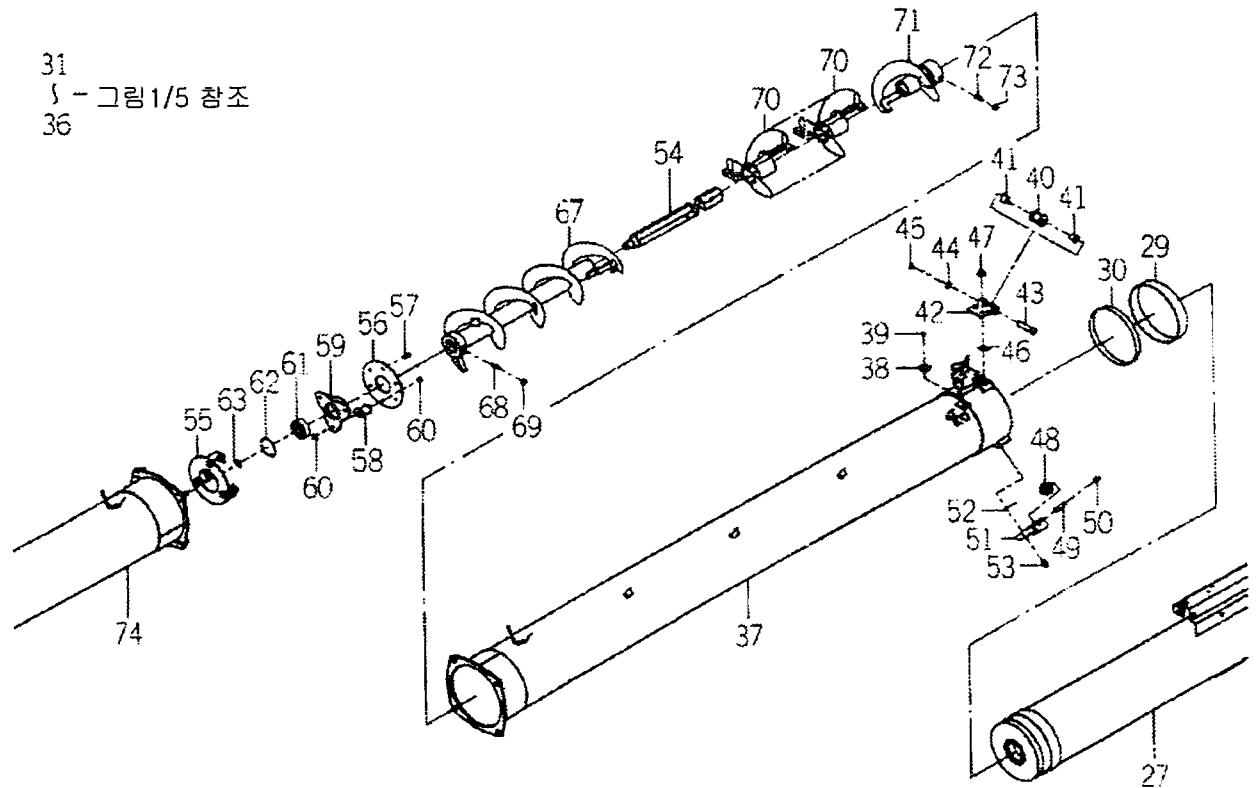
FIG.210 오거(어퍼) 관계(Z형) (그림2/5)
