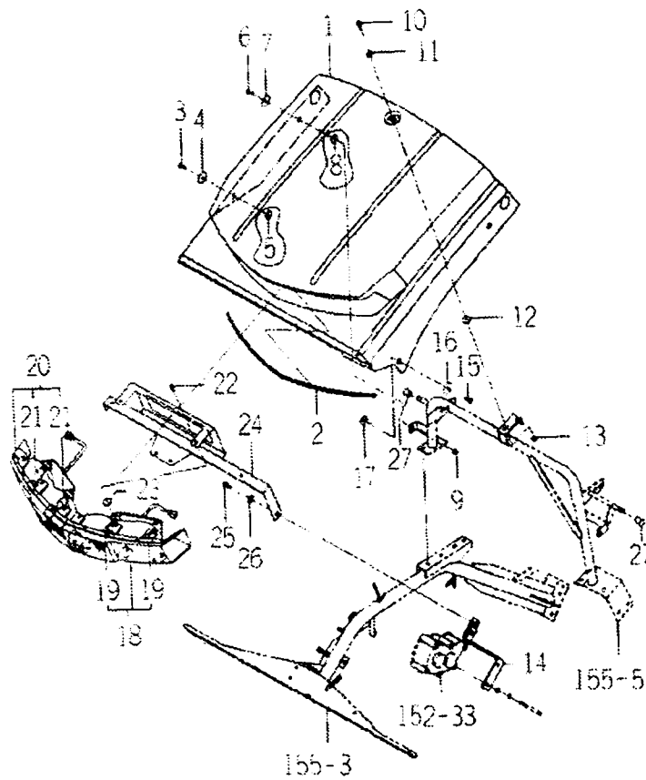
FIG. 159 방진커버(전) 관계(C형)
