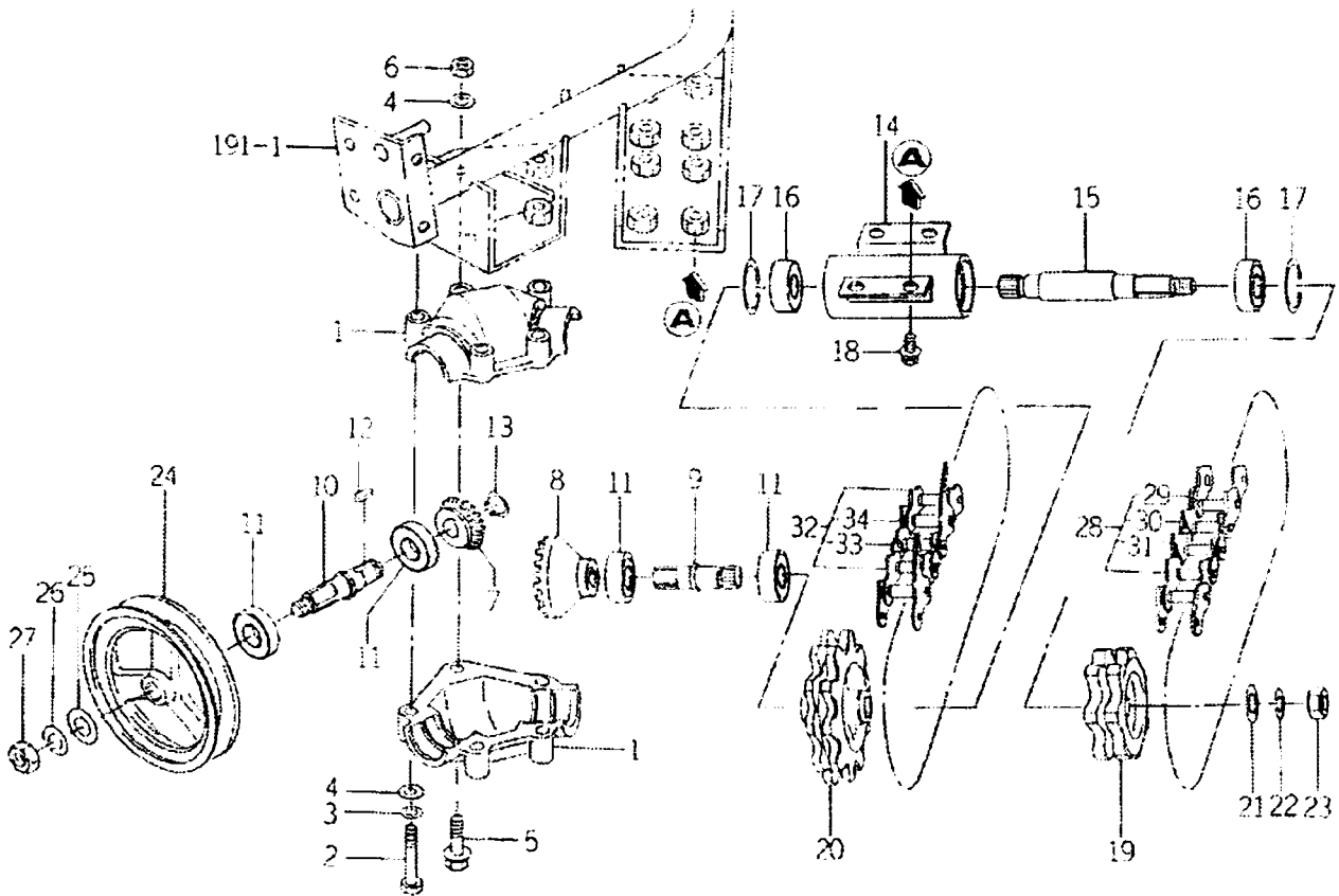
FIG.190 짚 배출 입력 관계
