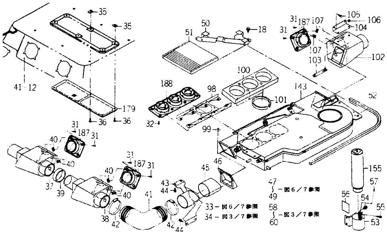
FIG. 47 에어컨 관계(C형)(그림2/7)
