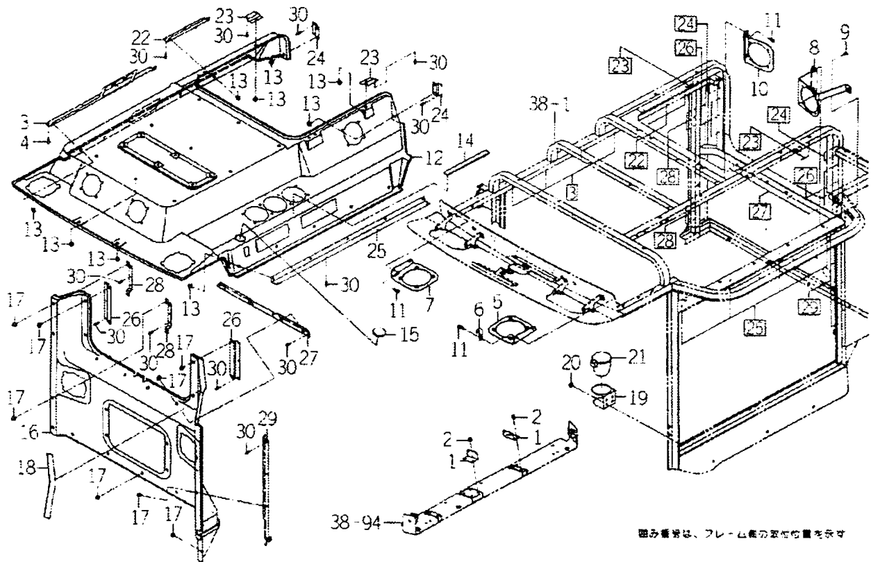
FIG. 41 인테리어 관계(C형)
