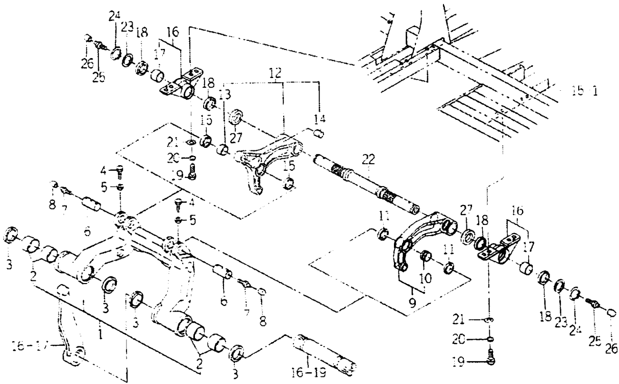
FIG. 17 암(피칭) 관계
