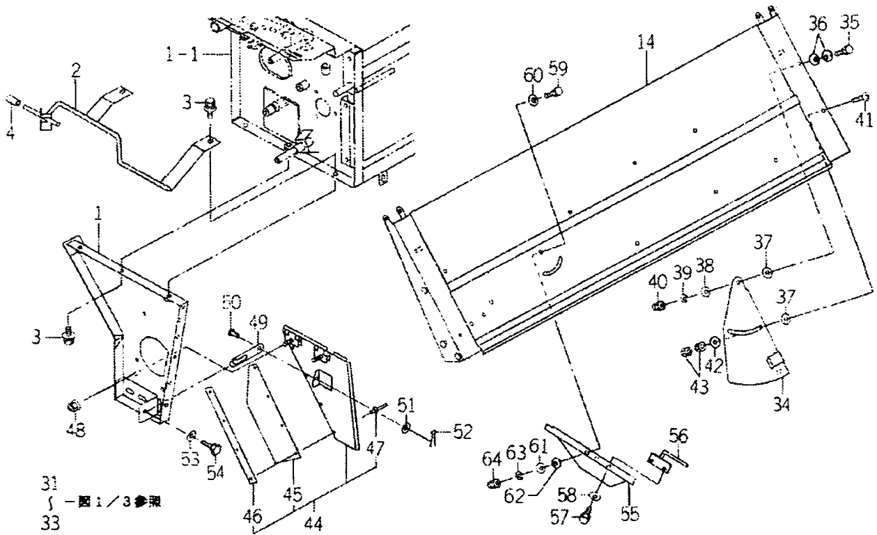
FIG.10 하 커버 관계 (그림2/3)
