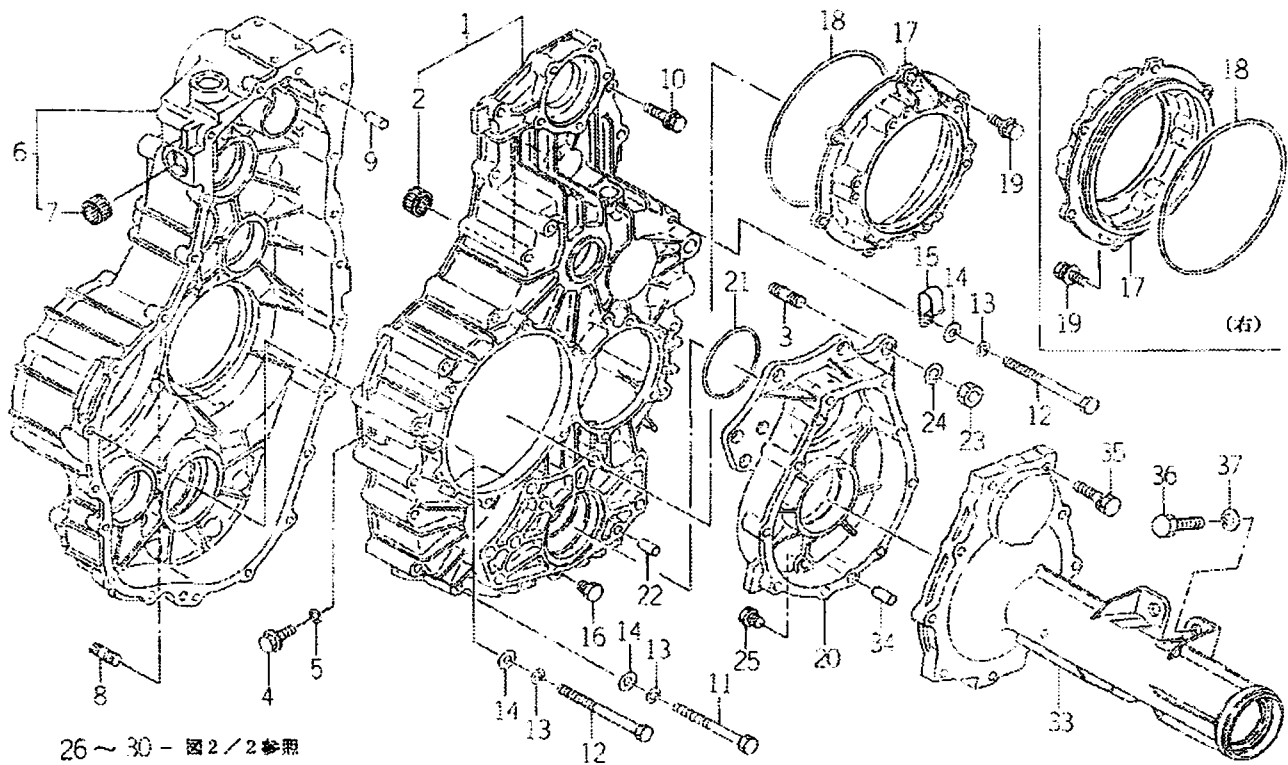
FIG.1 케이스(트랜스미션) 관계 (그림1/2)
