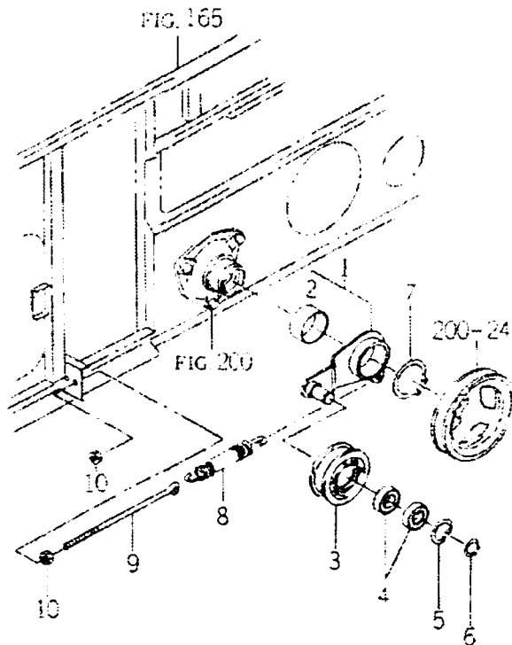
FIG.183 텐션 관계 (그림1/3)
