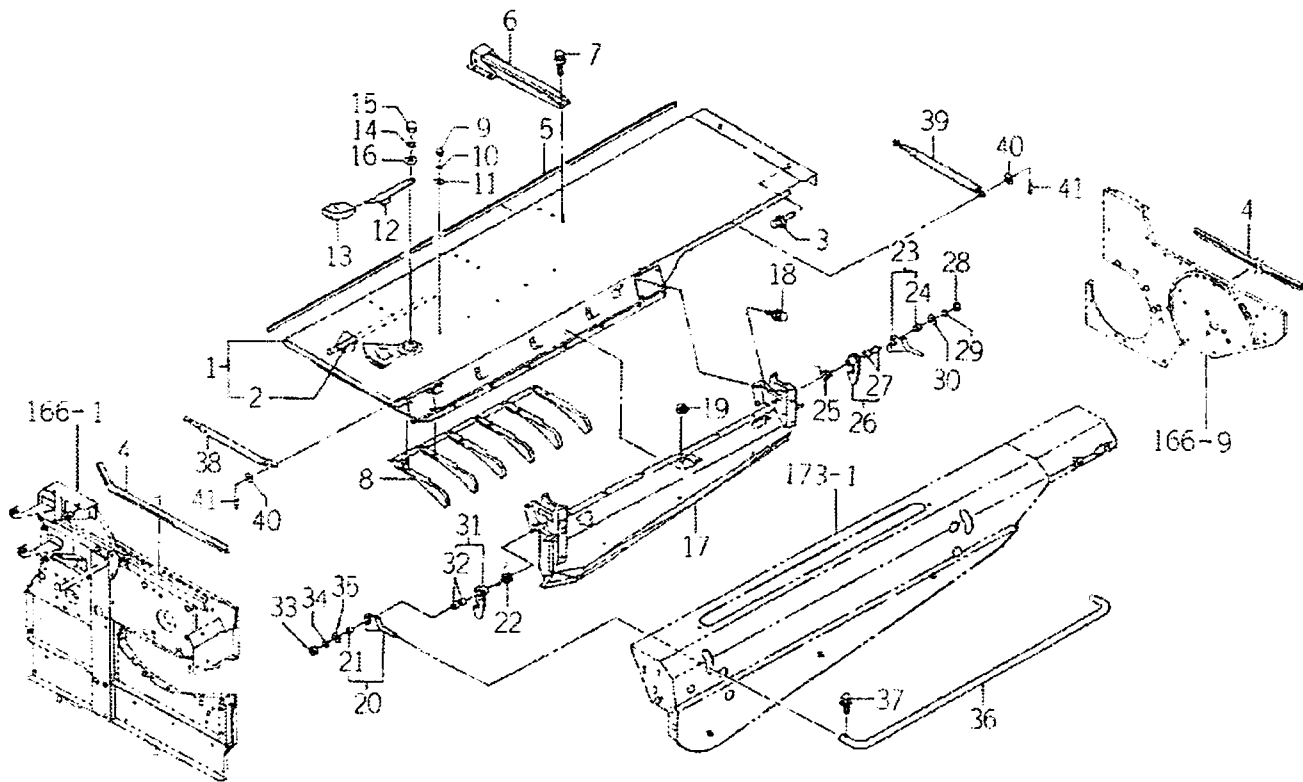
FIG.171 급통 커버 관계(C형 제외)
