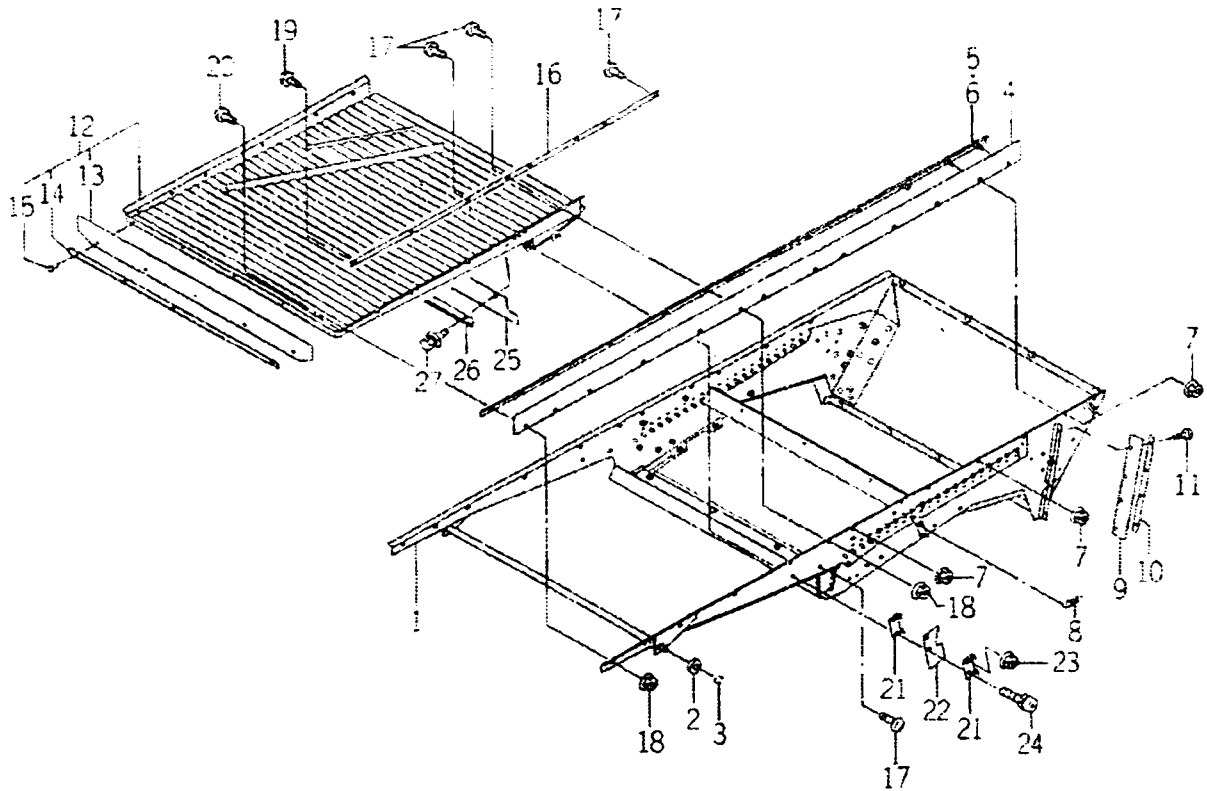
FIG.198 요동 선반 관계
