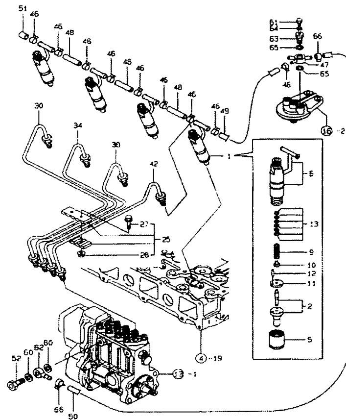
FIG.015 FO 분사 밸브
