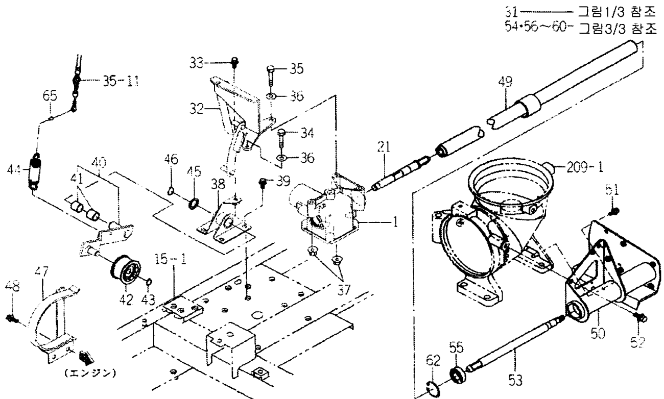
FIG.206 전동(1) 관계 (Z형) (그림2/3)
