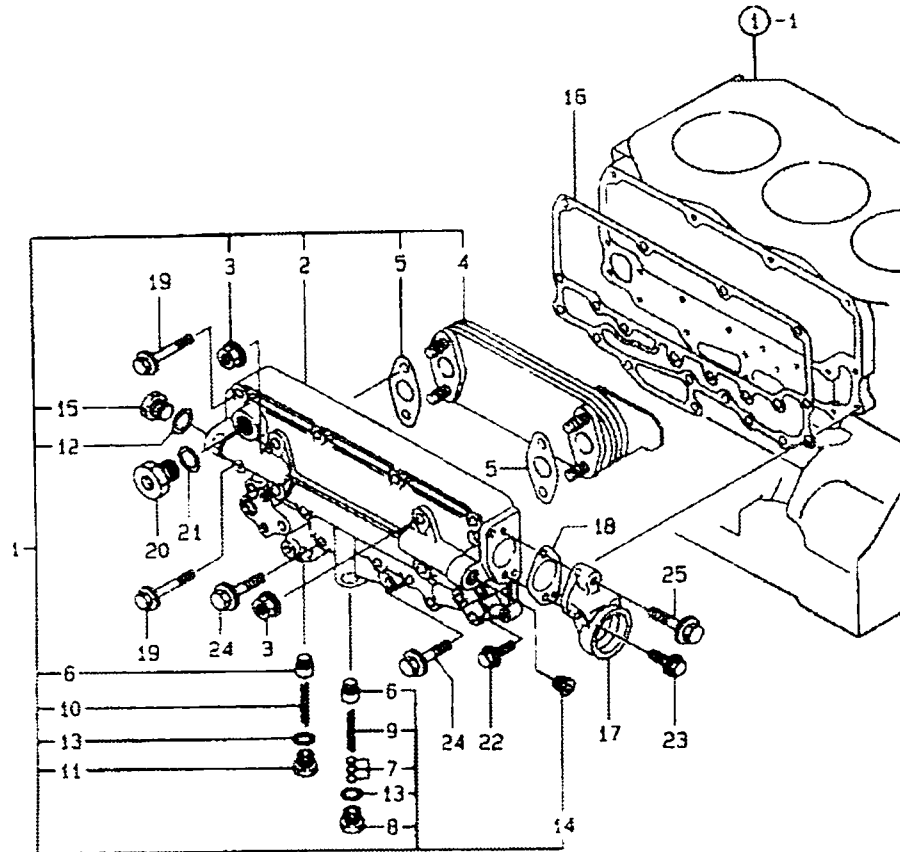
FIG.011 오일 쿨러 케이스
