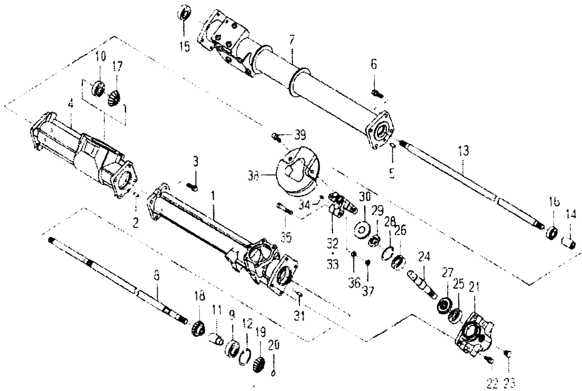
FIG. 150 기어케이스(로어) 관계
