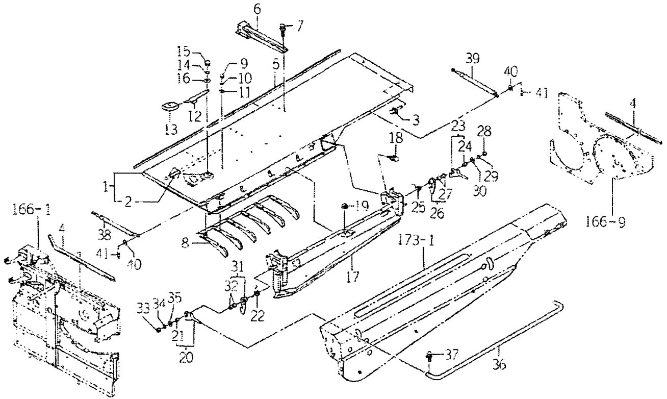
FIG.172 급통 커버 관계(C형)
