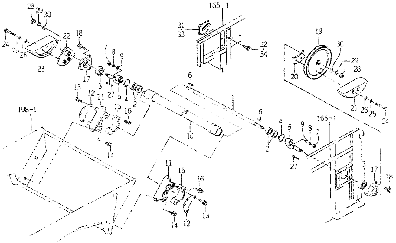
FIG.197 요동 입력 관계
