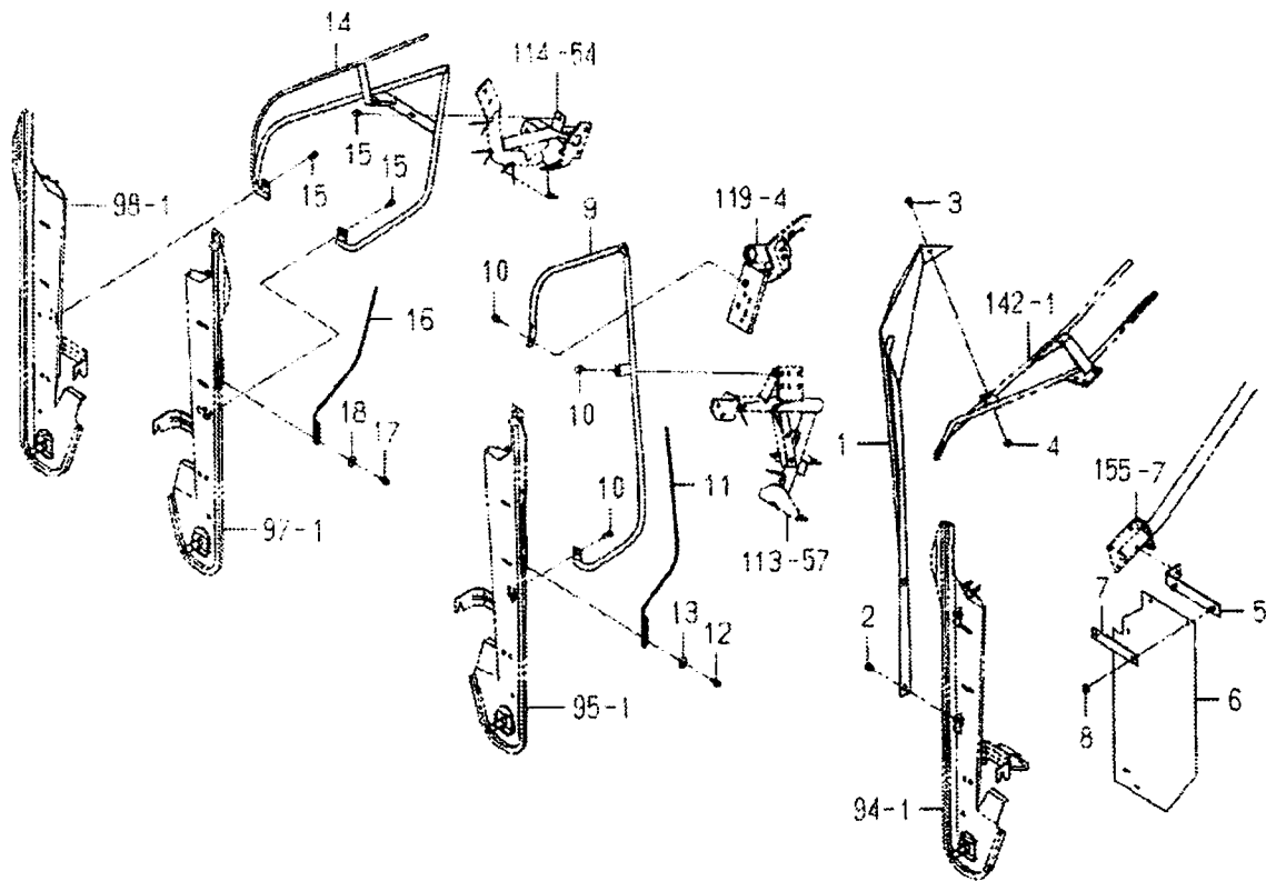
FIG. 102 인기 리어가이드(LH,센터) 관계(H형제외)
