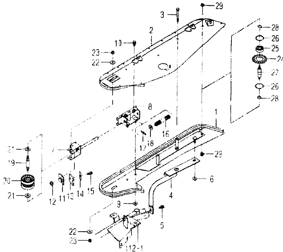
FIG. 133 이삭케이스(LH) 관계
