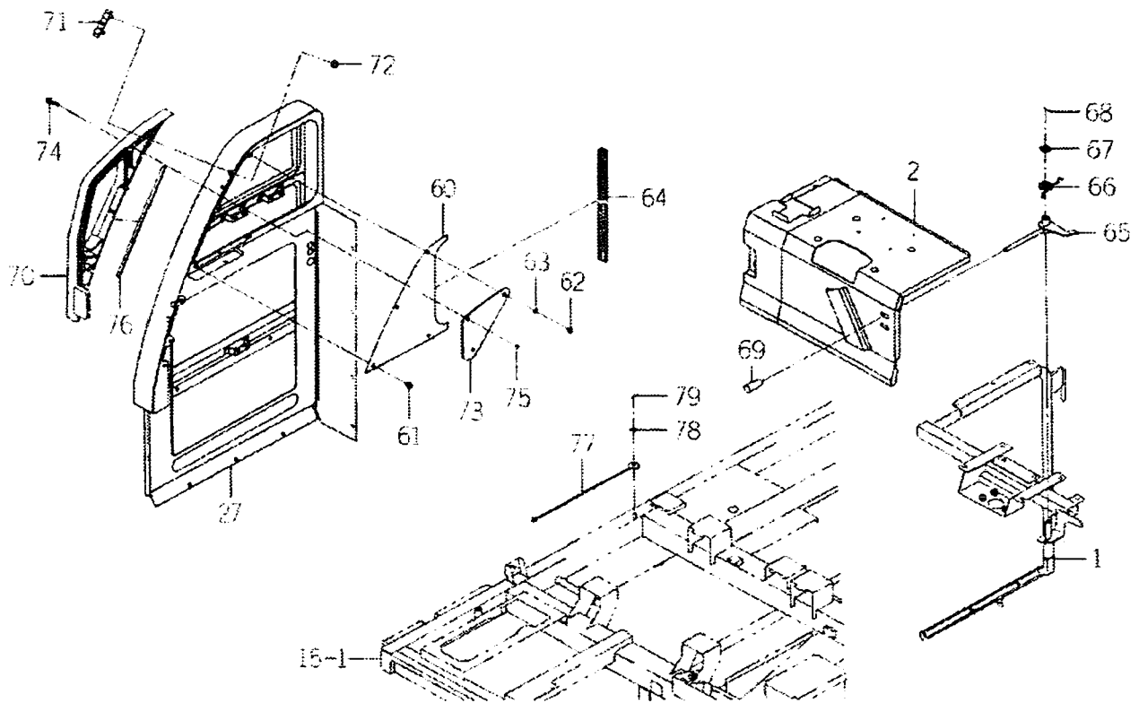
FIG.76 프레임(시트) 관계(C형제외) (그림3/3)
