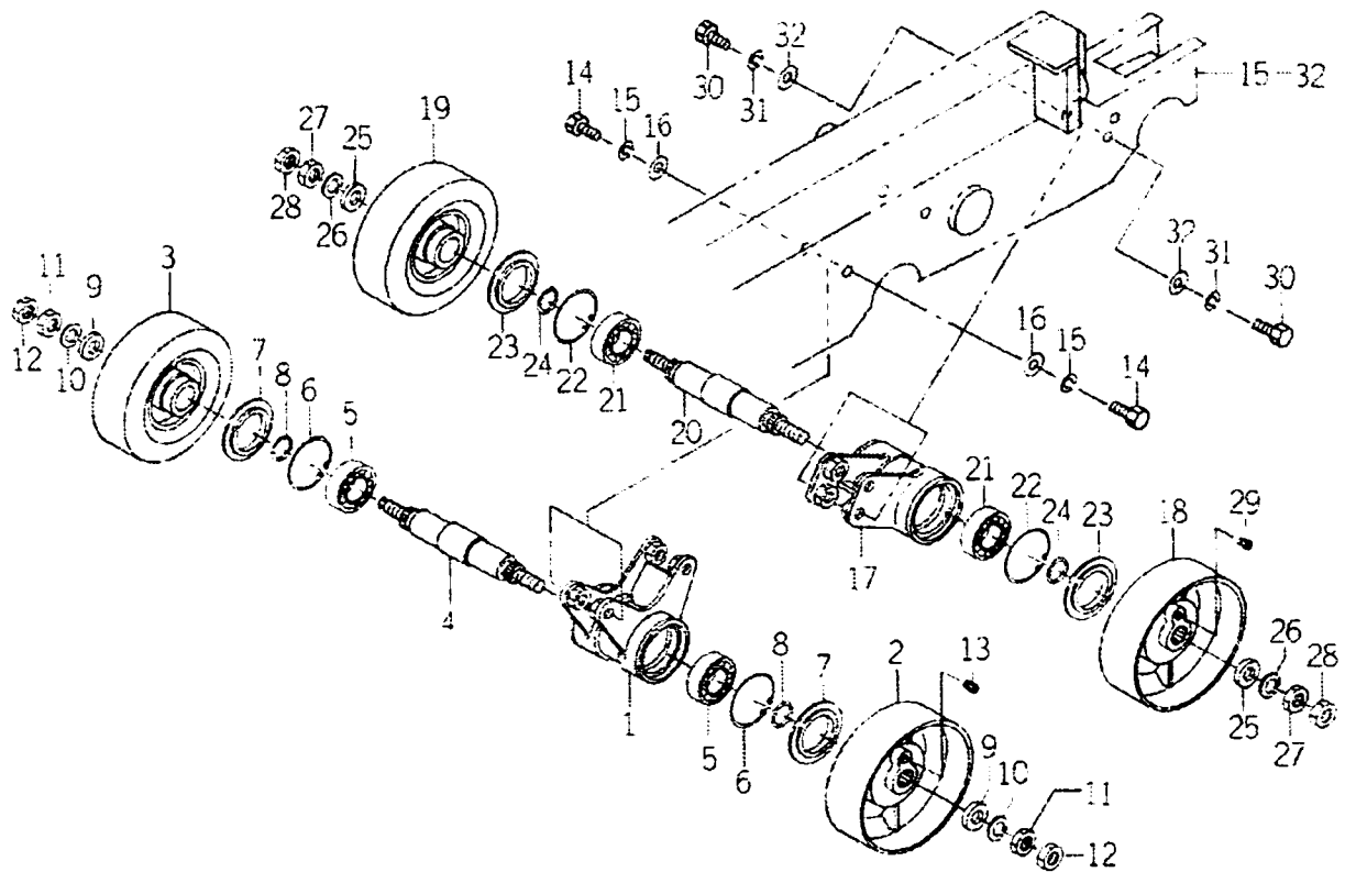
FIG. 18 롤러(트랙) 관계(LHW형제외)
