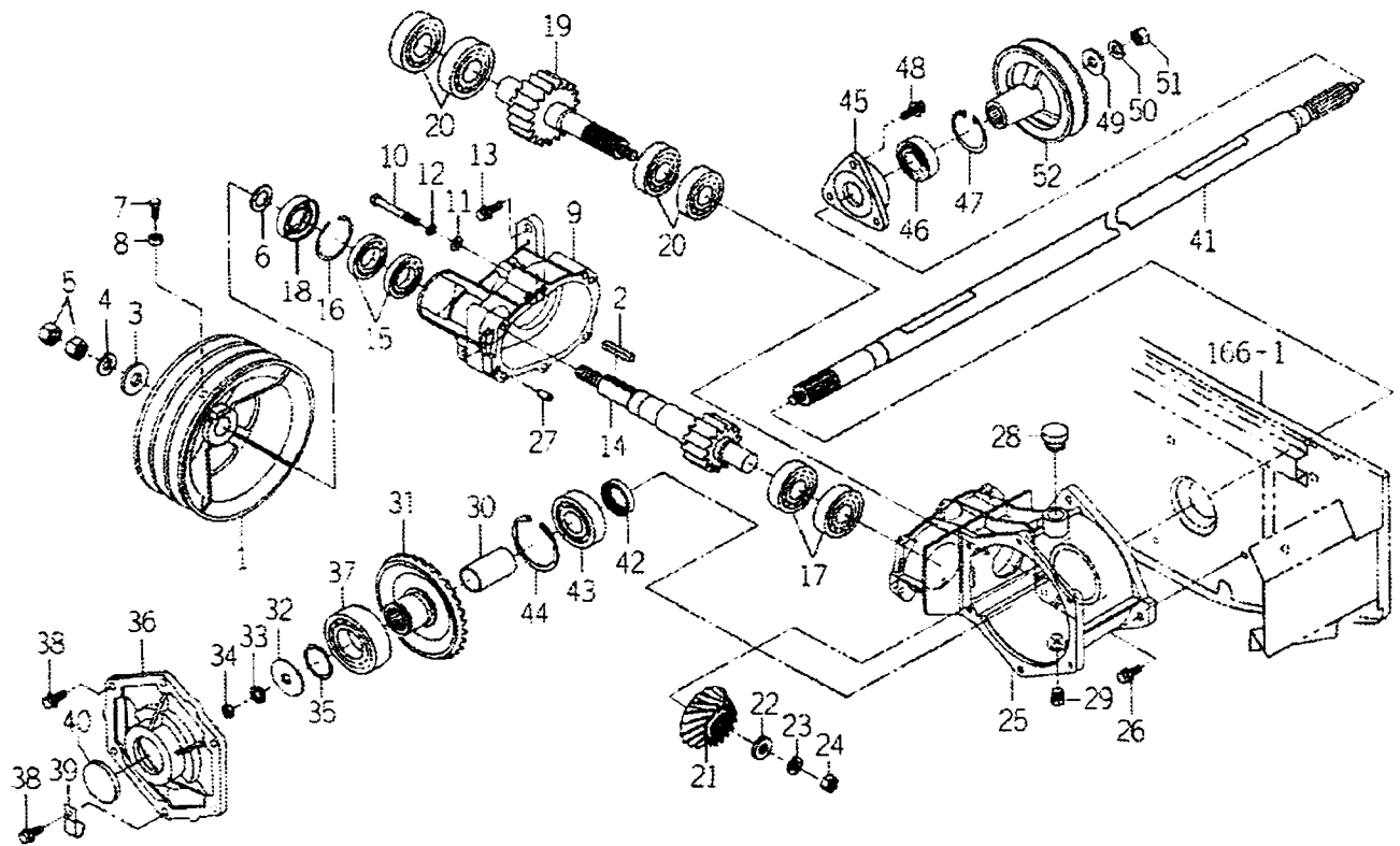
FIG.181 급통 입력 관계
