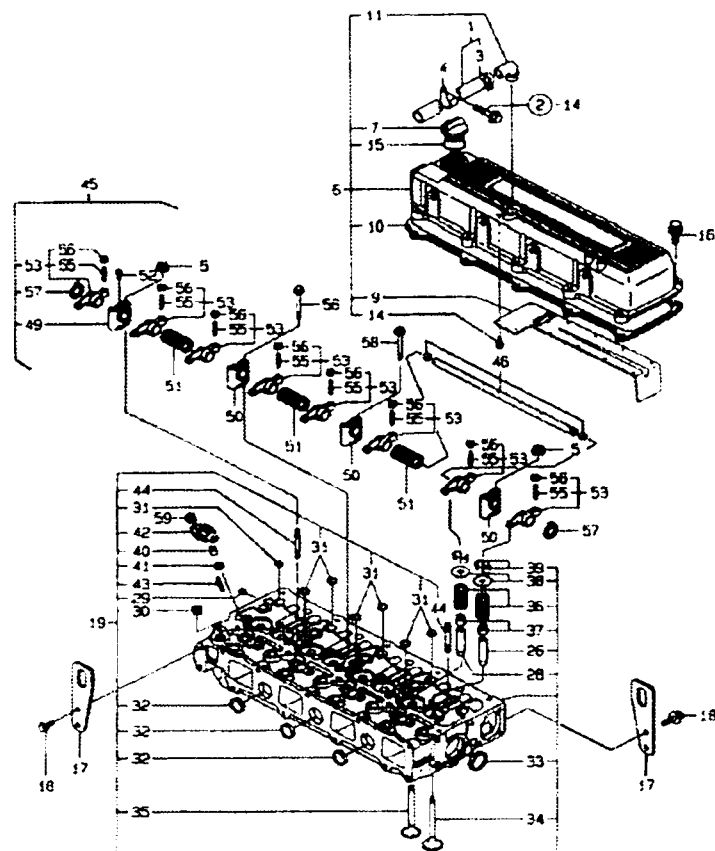
FIG.004 실린더 헤드
