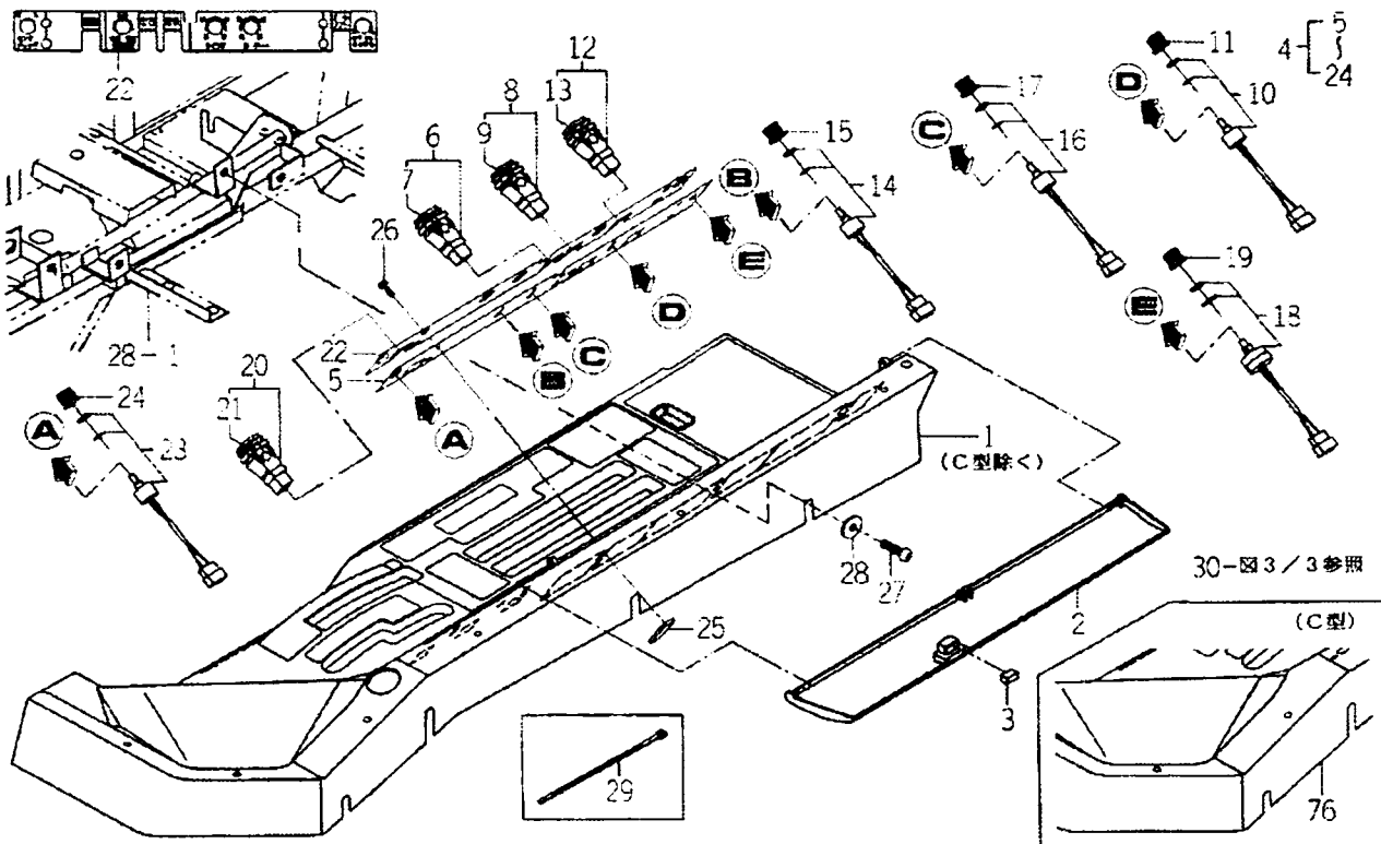
FIG. 56 스위치패널(LH) 관계(그림1/3)
