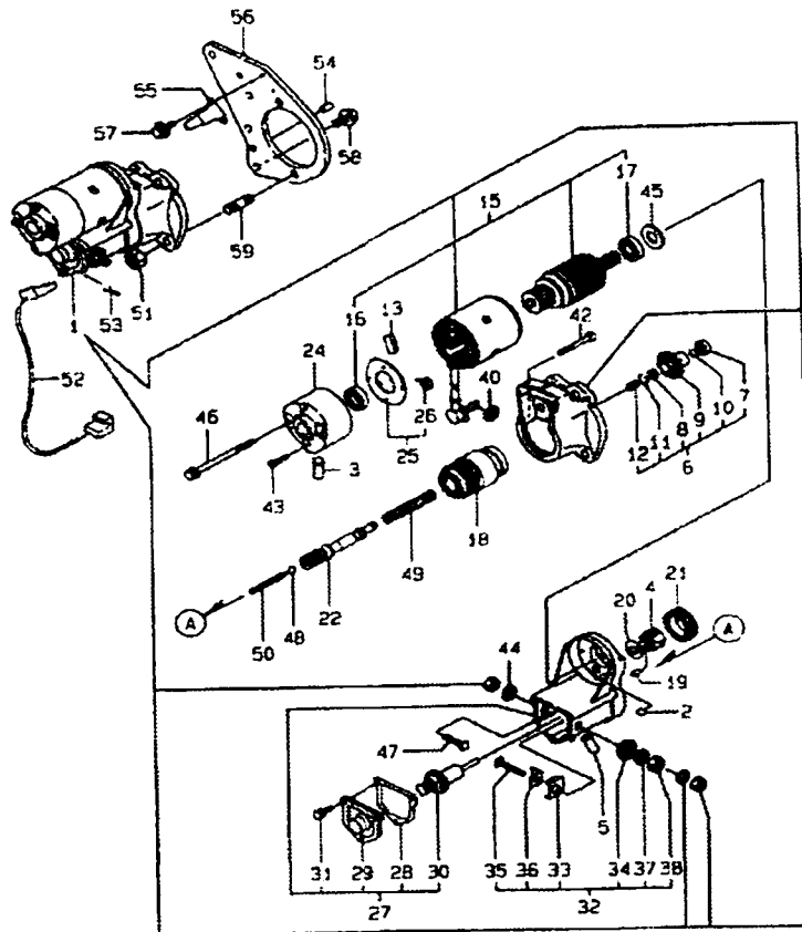
FIG.017 스타팅 모터
