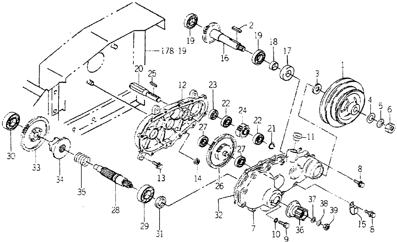
FIG.182 배진 구동 관계 (그림1/2)
