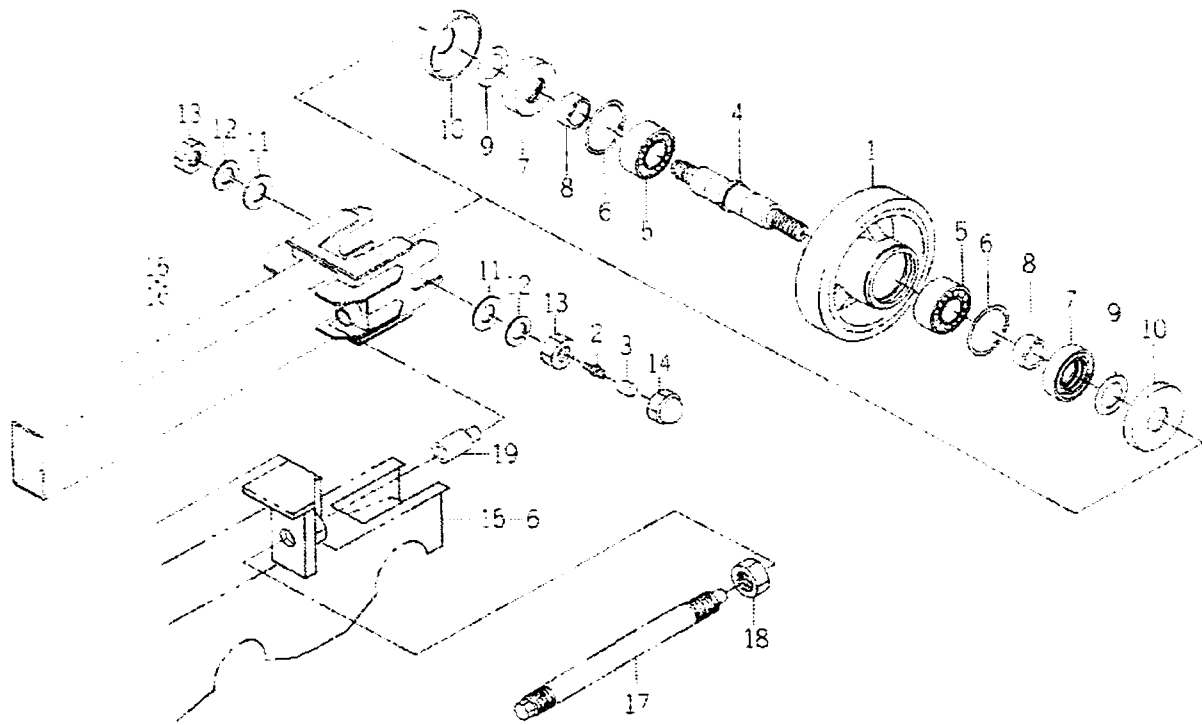
FIG. 21 롤러(아이들) 관계
