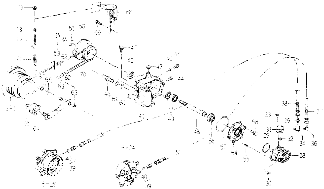
FIG.88 쿨러(미션) 관계 (그림2/2)
