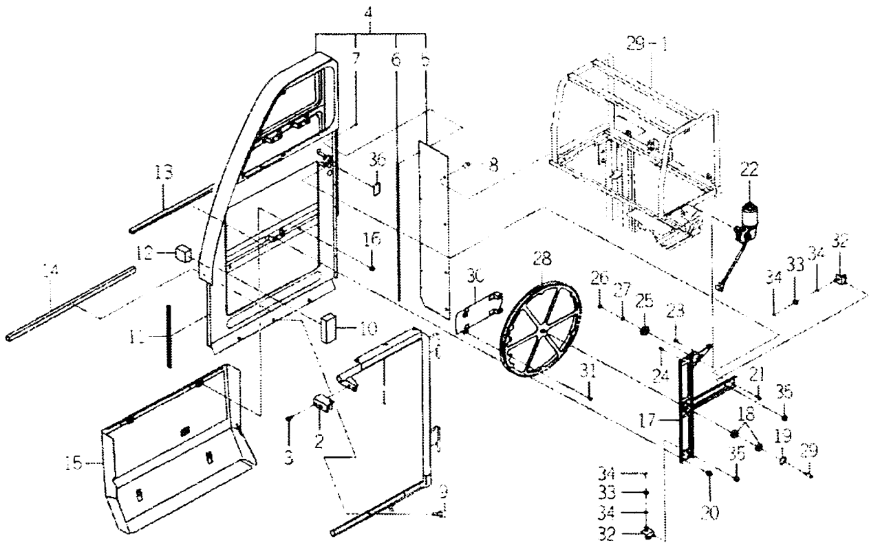
FIG.78 커버(라디에이터) 관계 (C형) (그림1/2)
