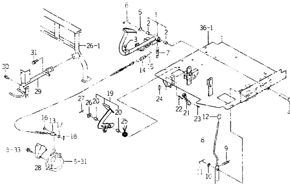
FIG. 37 주차브레이크 관계
