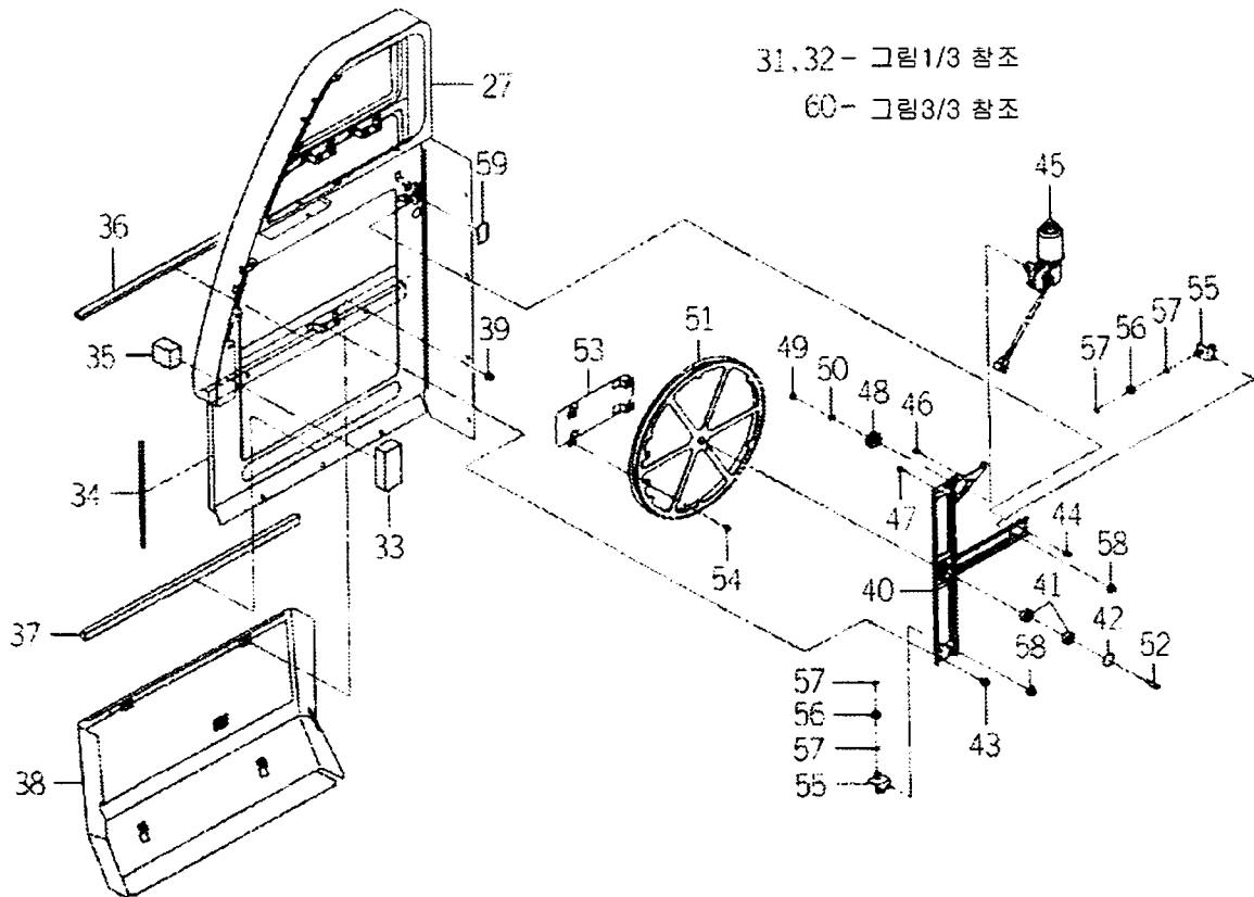
FIG.76 프레임(시트) 관계(C형제외) (그림2/3)
