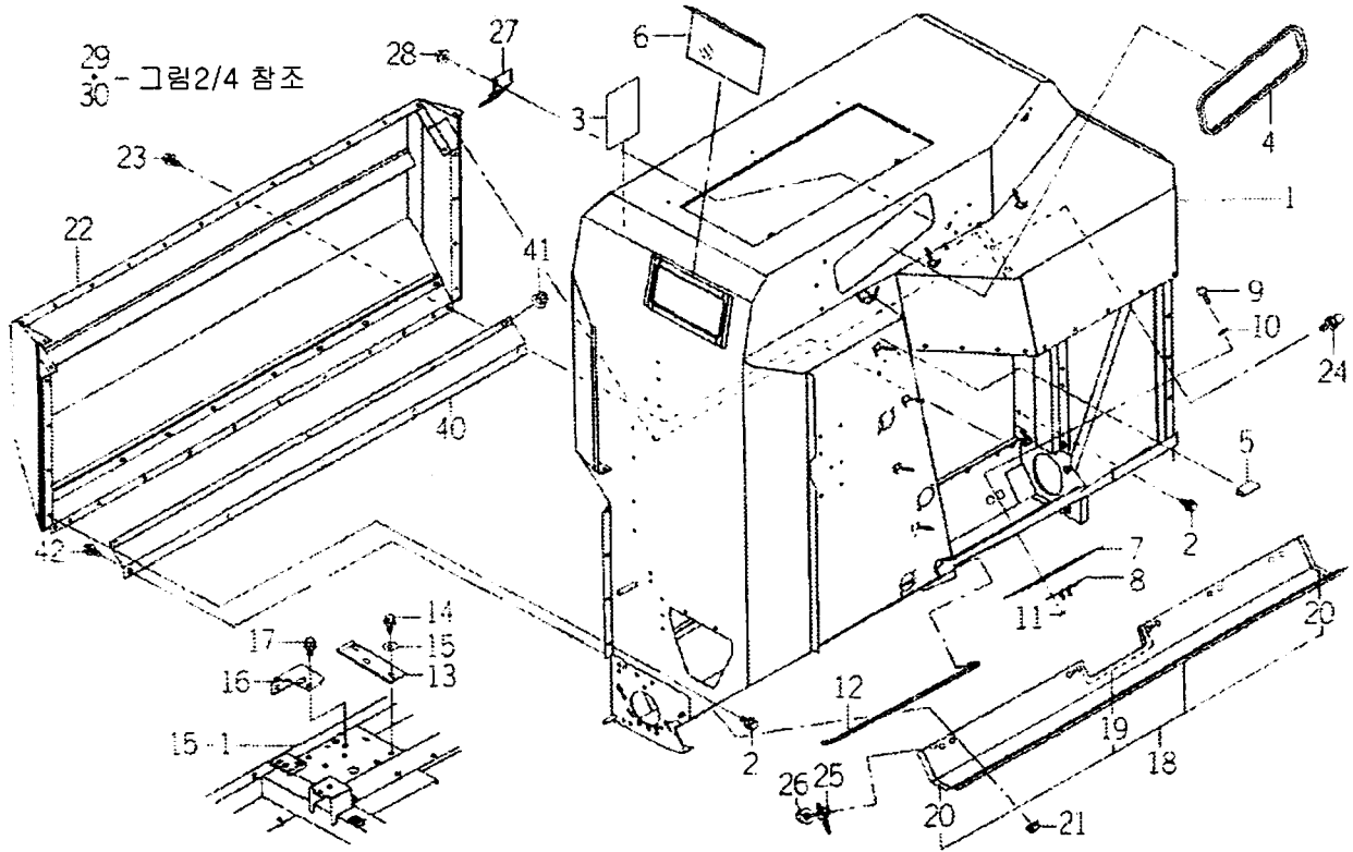
FIG.205 탱크 관계 (그림1/4)
