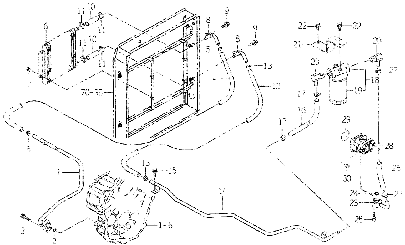
FIG.88 쿨러(미션) 관계 (그림1/2)
