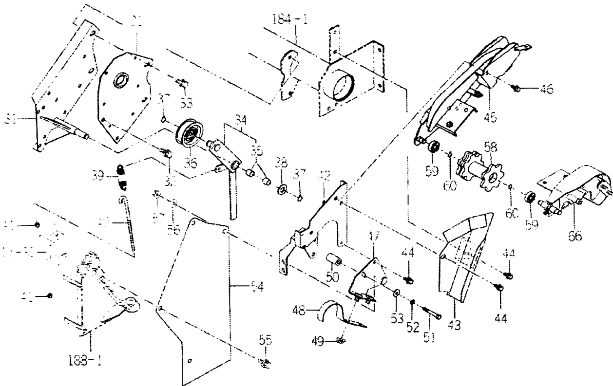
FIG.189 싱크로 관계 (그림2/3)
