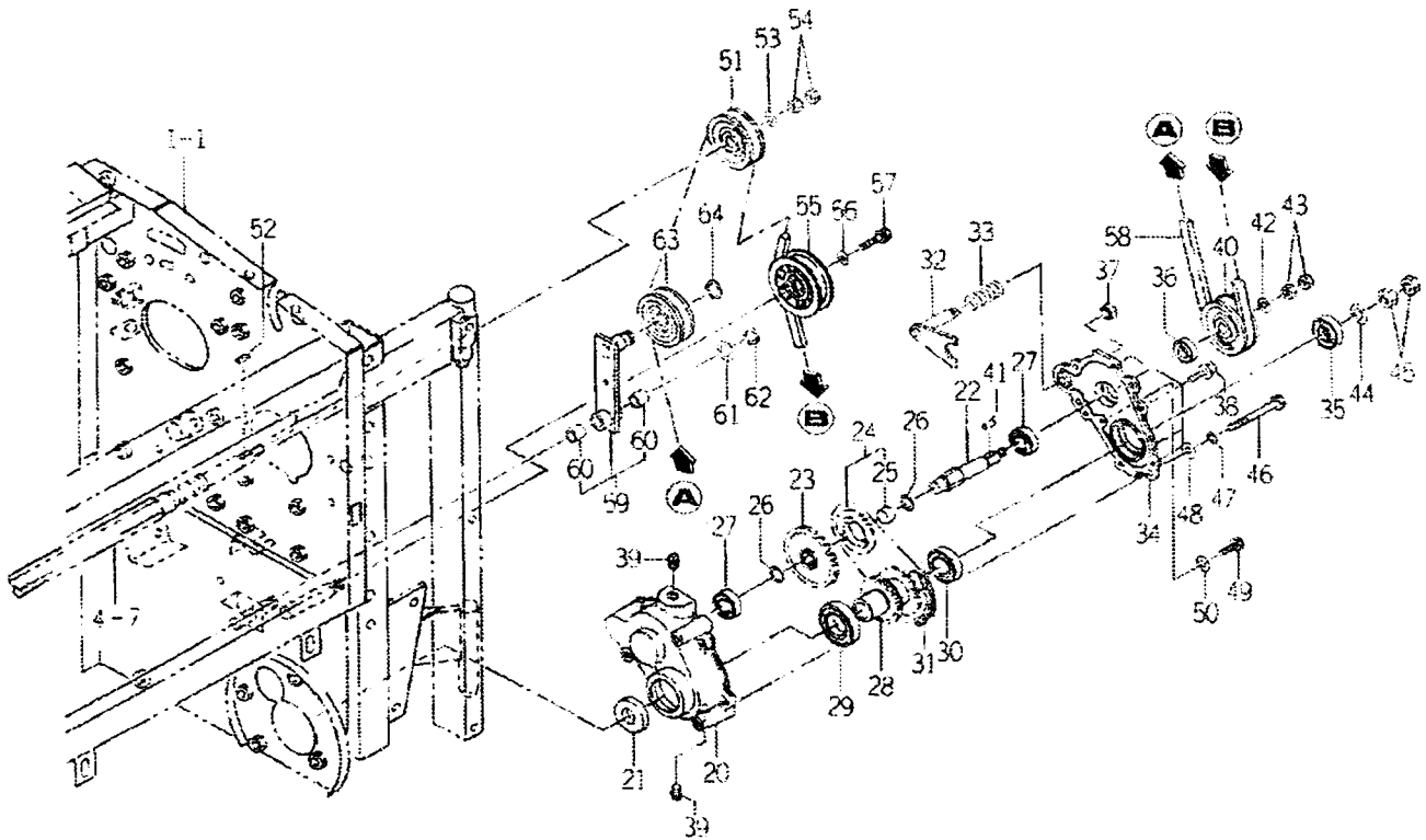
FIG.6 확산축 관계 (그림2/3)
