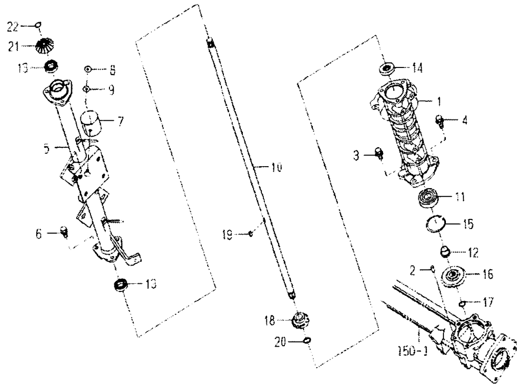
FIG. 151 기어케이스(사이드) 관계(그림1/2)
