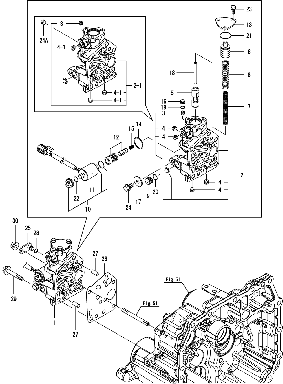
Fig.56. P.T.O. 밸브
