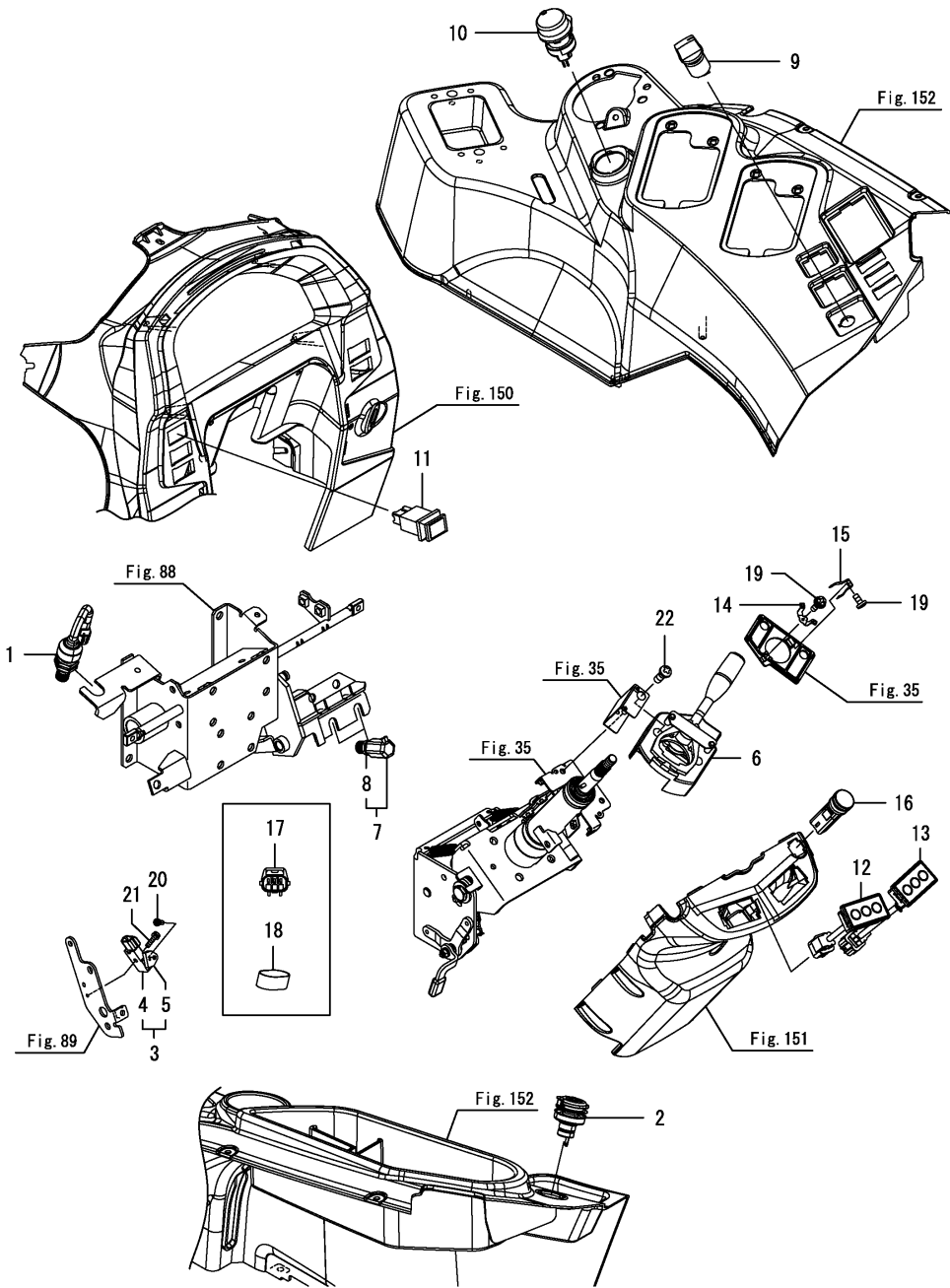
Fig.127. 스위치(바닥)(1)
