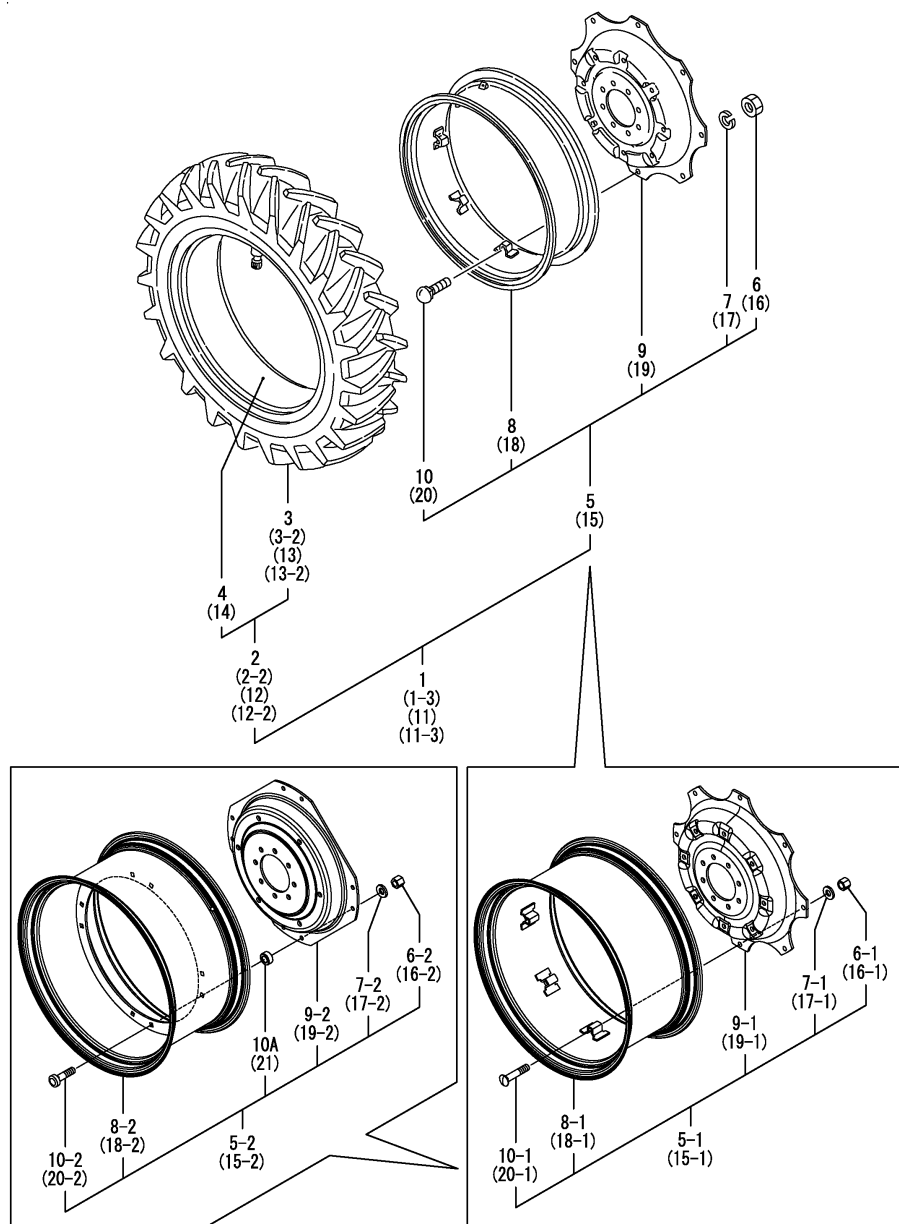
Fig.84. 후륜휠타이어(16.9-30)
