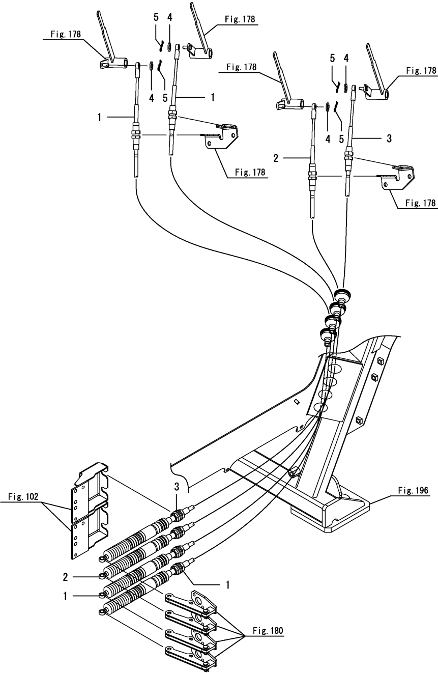
Fig.179. S.C.V.레버와이어(4련)
