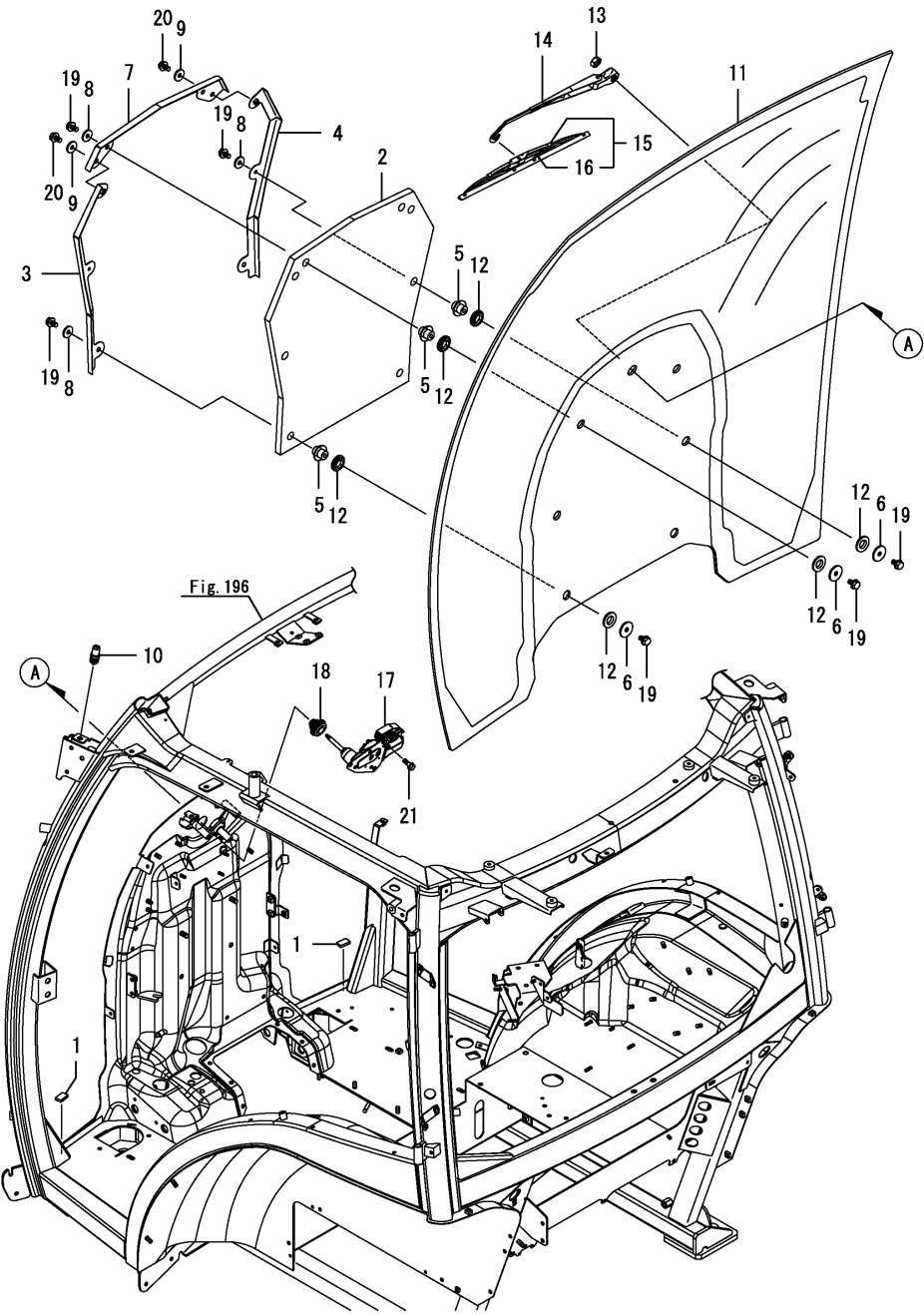
Fig.201. 전방유리
