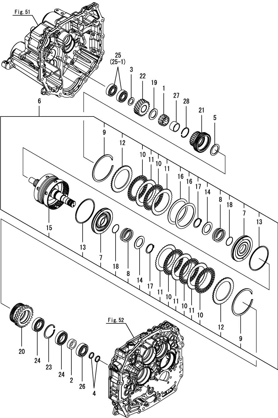
OCNP6-M02150 미션부 Fig.70. 전륜구동
