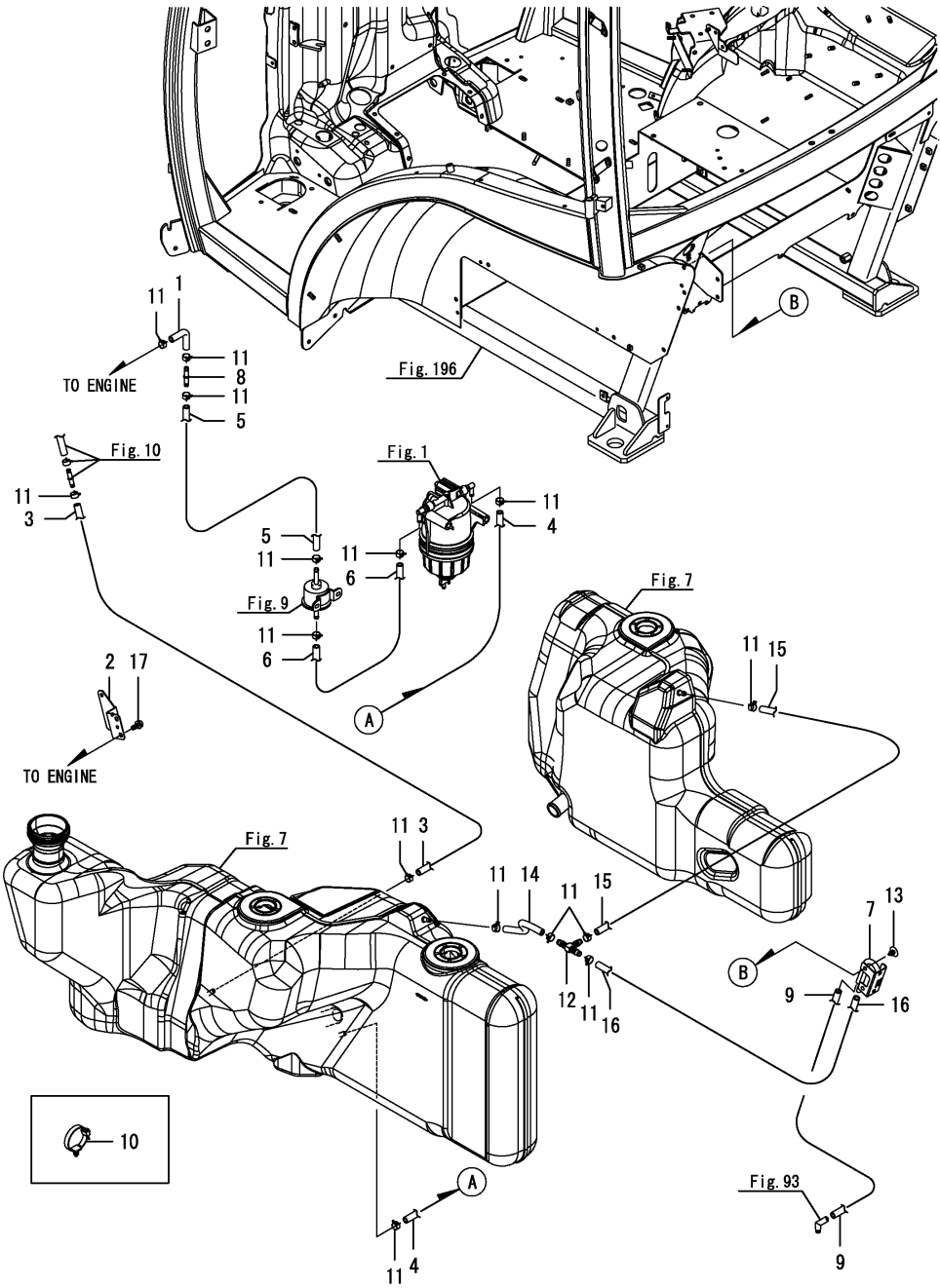
Fig.11. 연료호스
