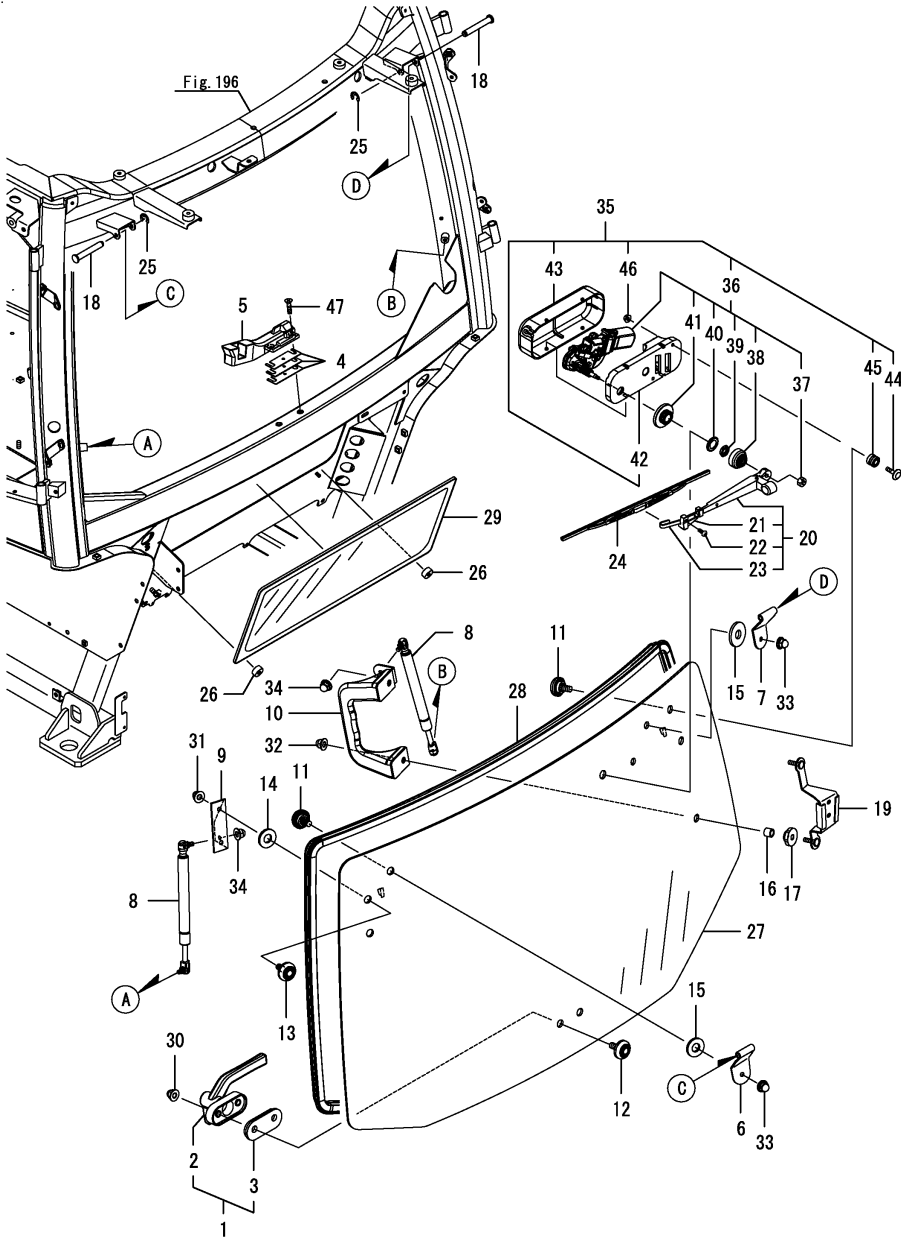
Fig.202. 후방창문
