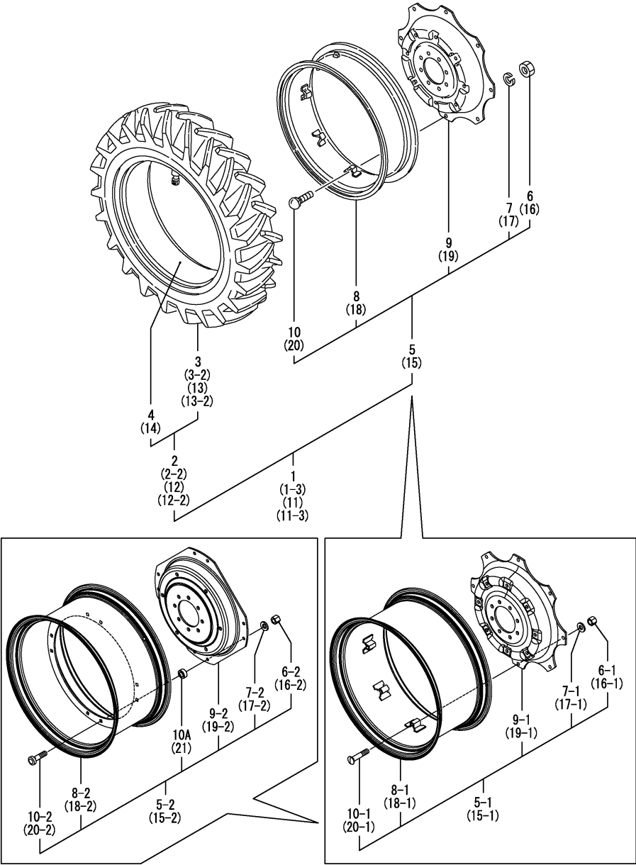
Fig.84. 후륜휠타이어(16.9-30)
