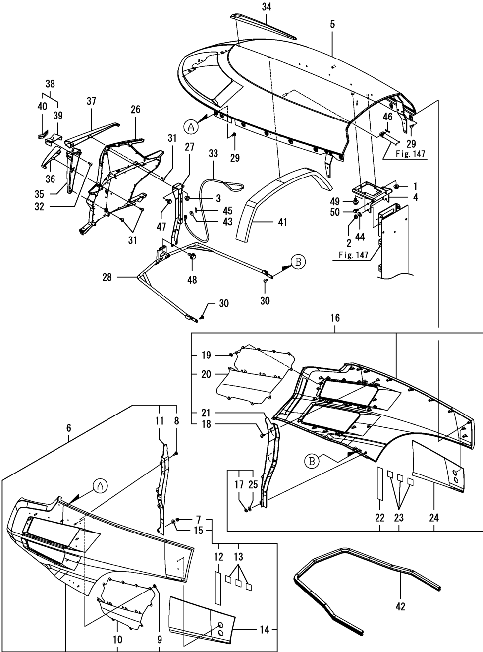
Fig.148. 본네트
