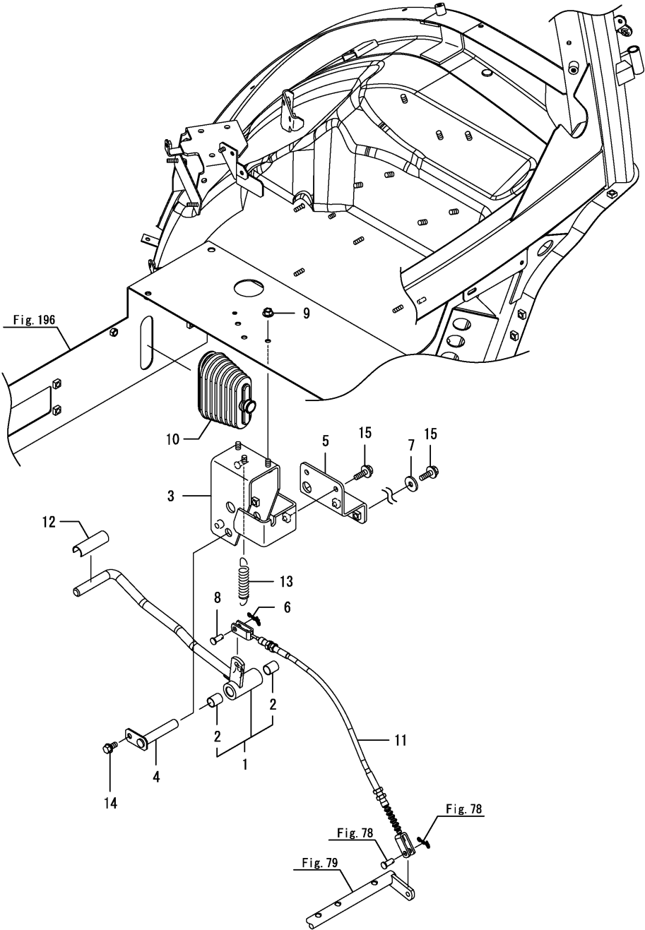
Fig.80. 차동고정페달
