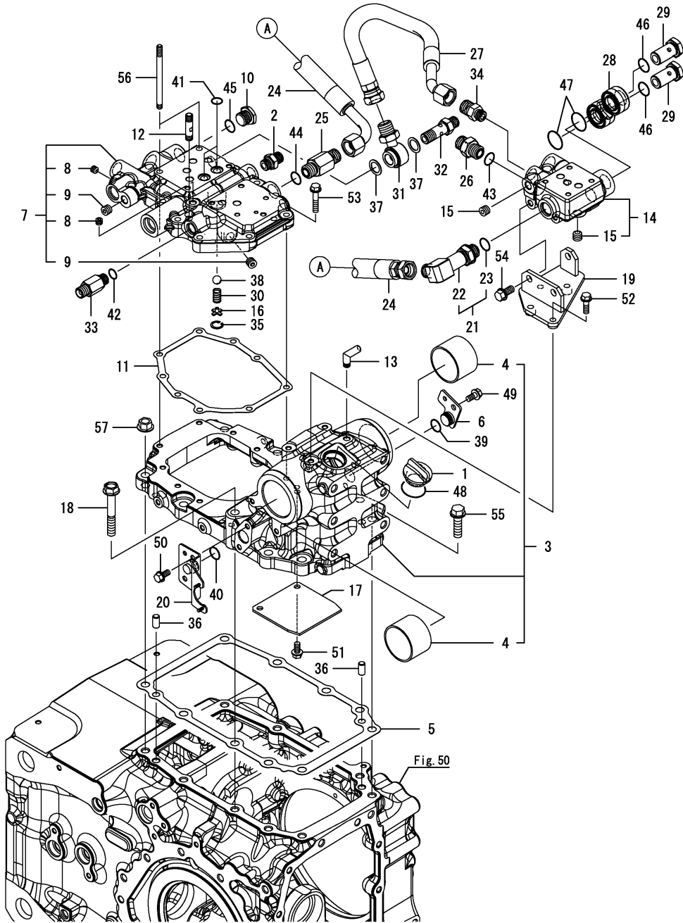
Fig.93. 유압리프트케이스
