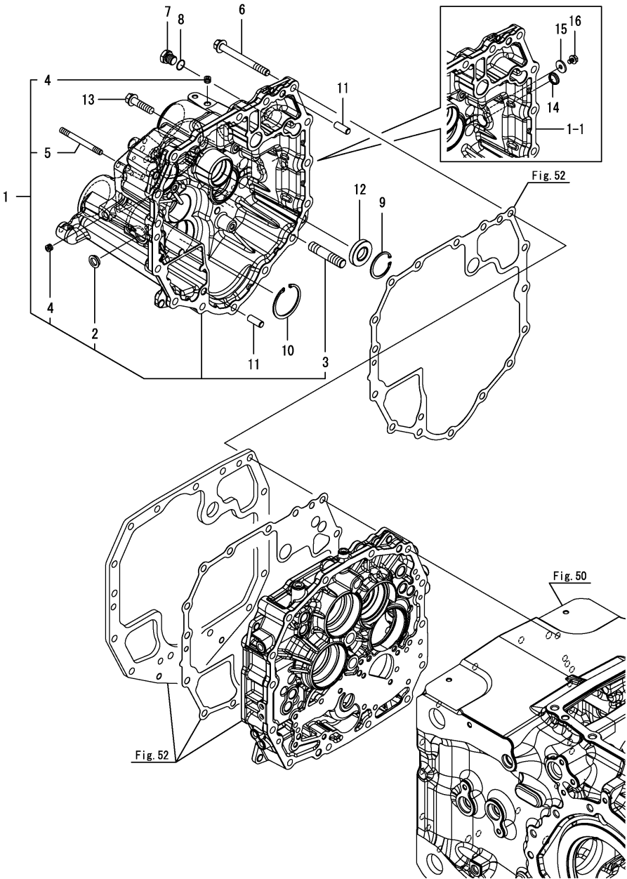
Fig.51. 프론트커버
