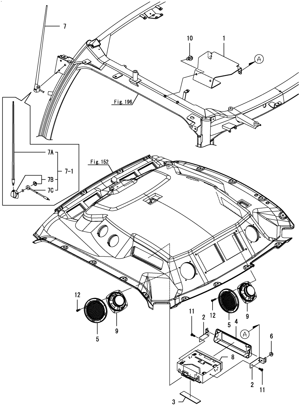
Fig.211. 오디오
