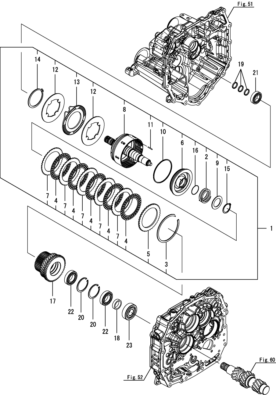
Fig.49. P.T.O. 클러치
