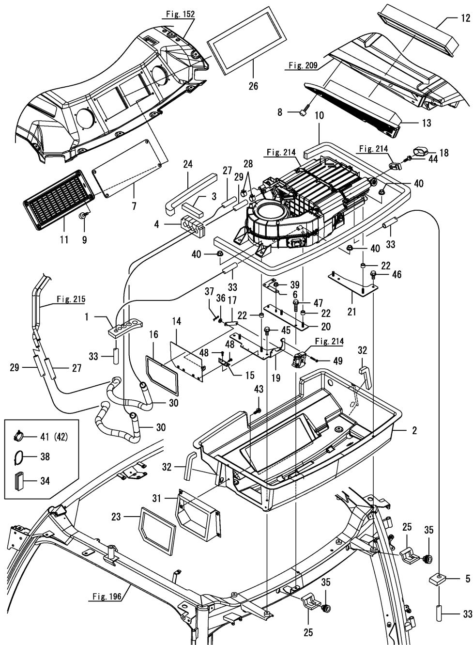
Fig.216. 에어컨(3)
