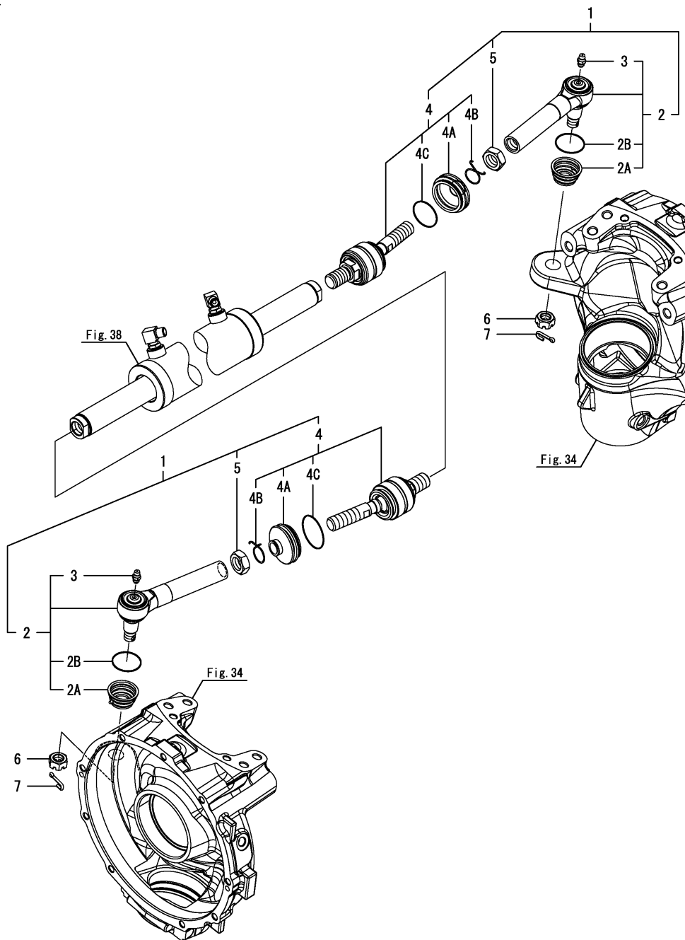
Fig.22. 타이로드
