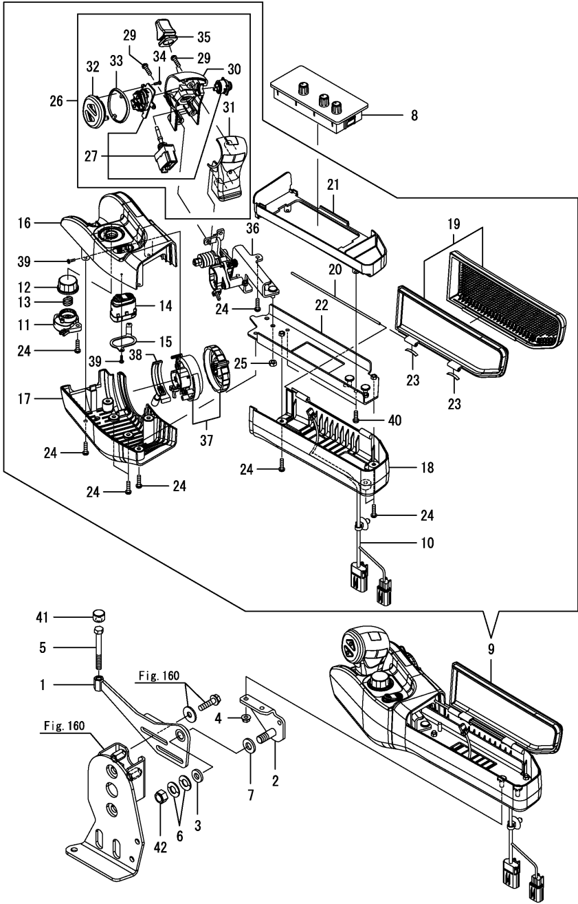
Fig.158. 팔걸이
