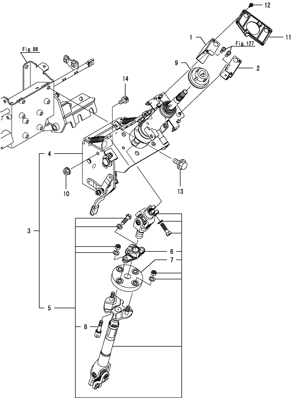
Fig.35. 스티어링칼럼
