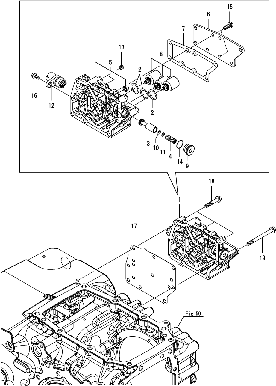
Fig.54. 밸브(I-H.M.T.)
