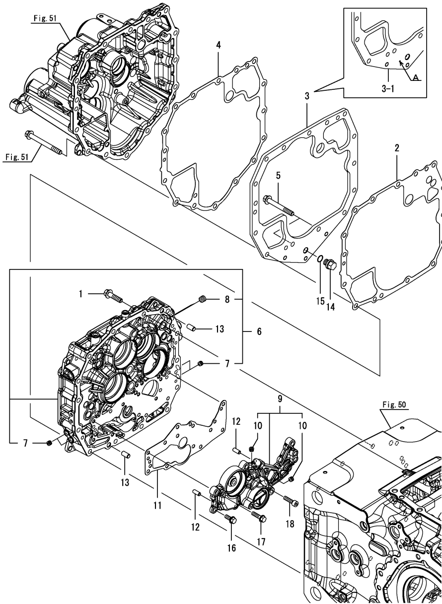
Fig.52. 센터하우징
