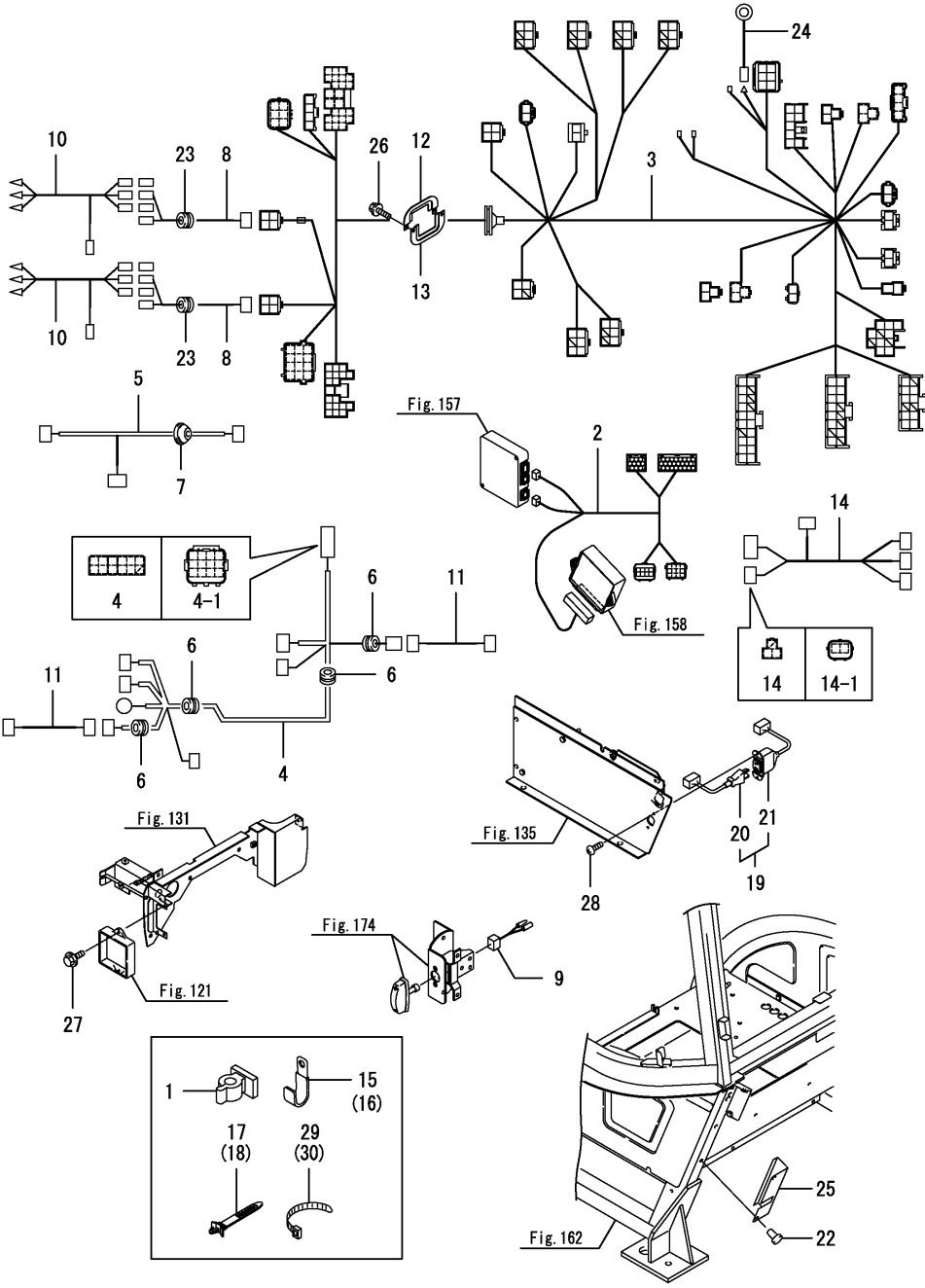
Fig.120. 배선(캐빈)
