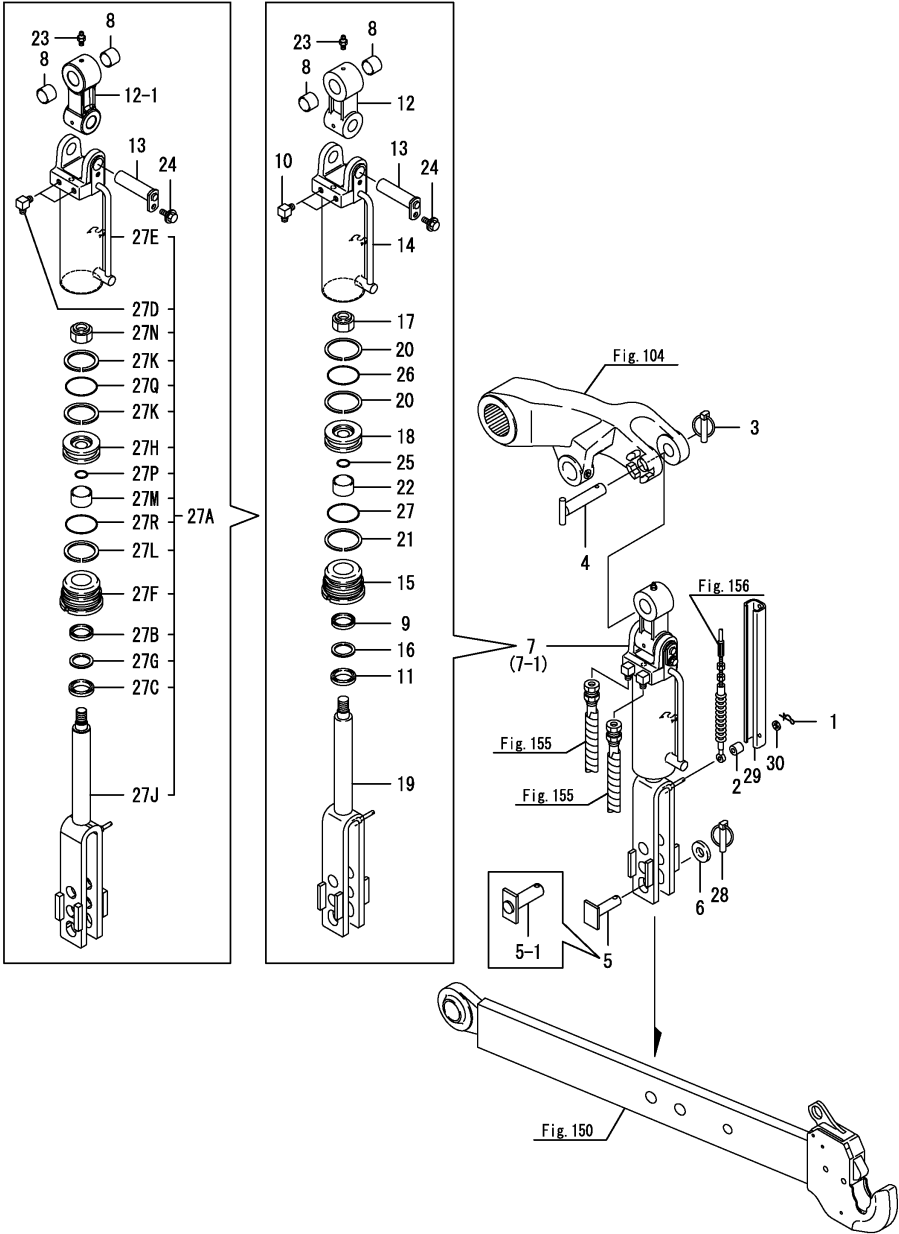
OCNP5-M34601 히치부 Fig.149. 승강실린더
