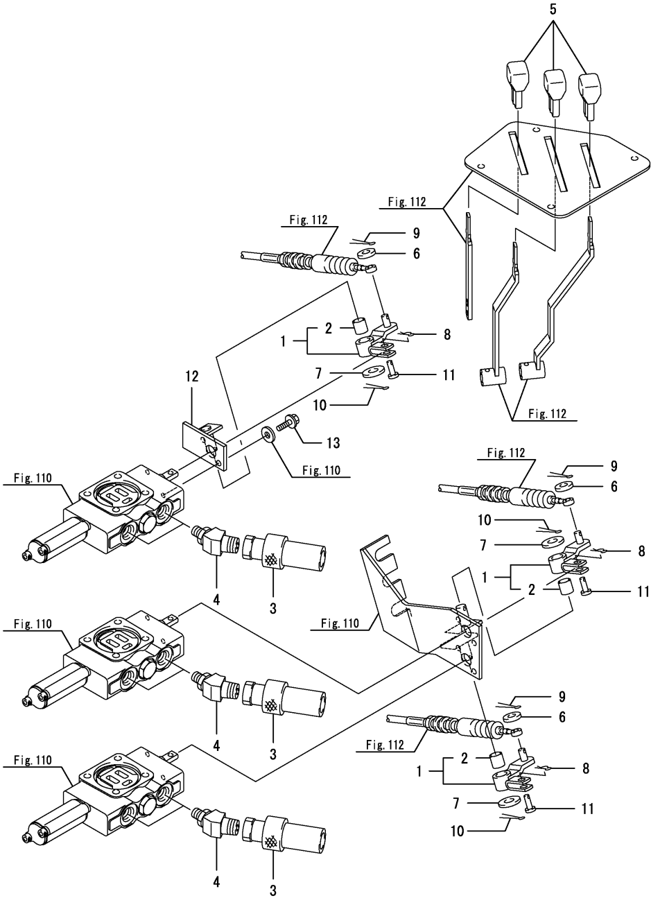
Fig.111. S.C.V.(3연)(커플러)
