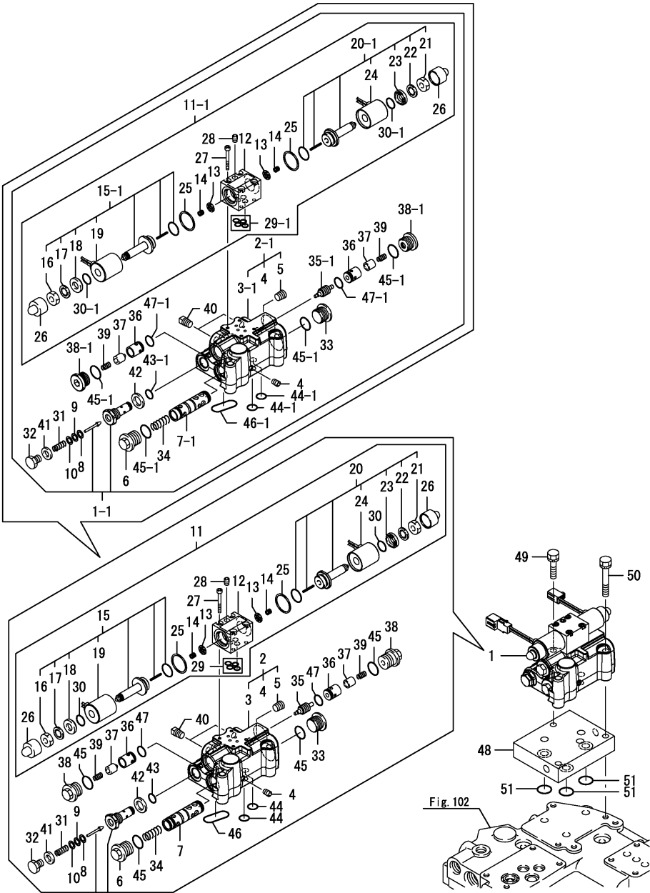
Fig.154. 수평 제어(U.F.O.)
