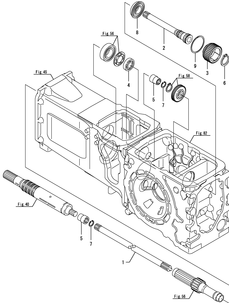
Fig.59. P.T.O. 구동축
