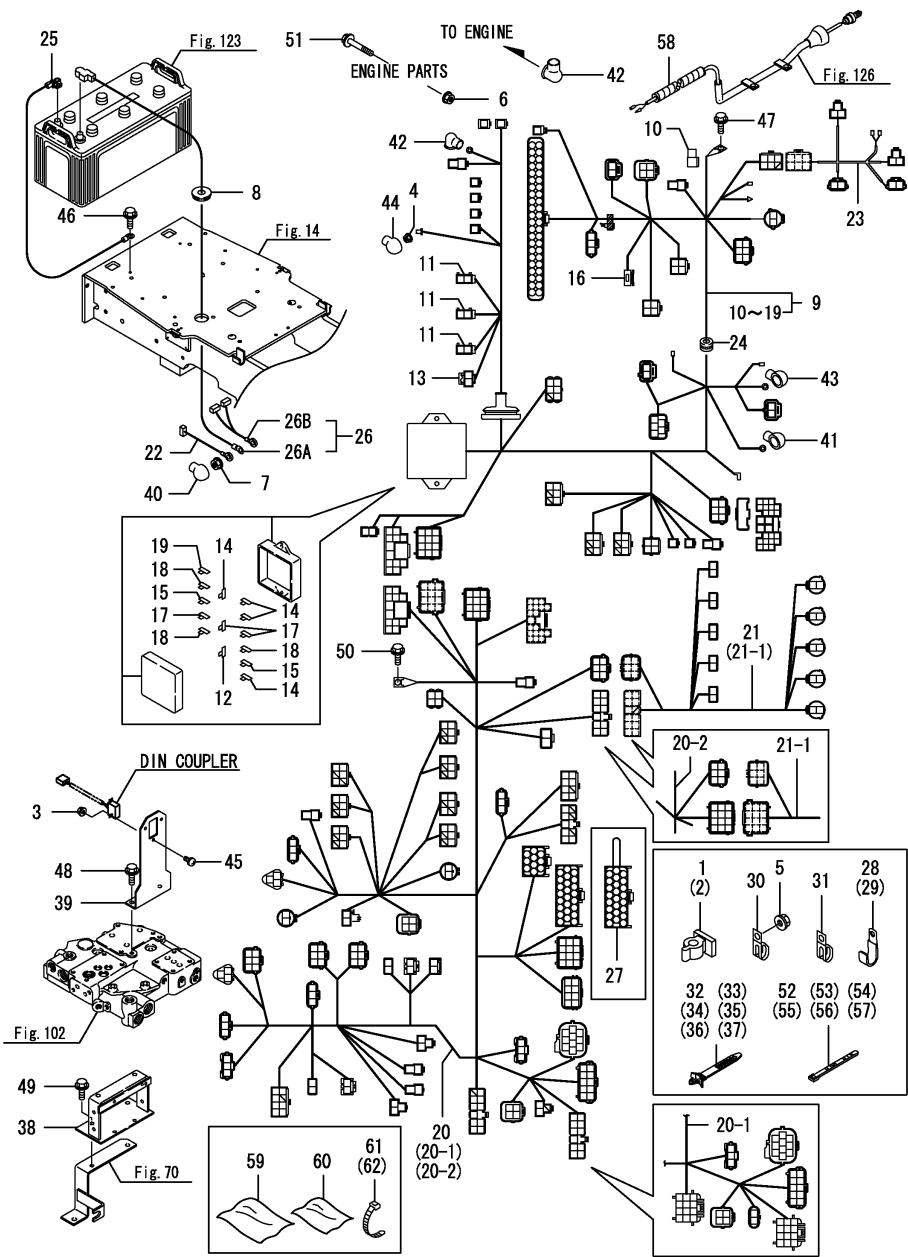
Fig.121. 배선(본기)
