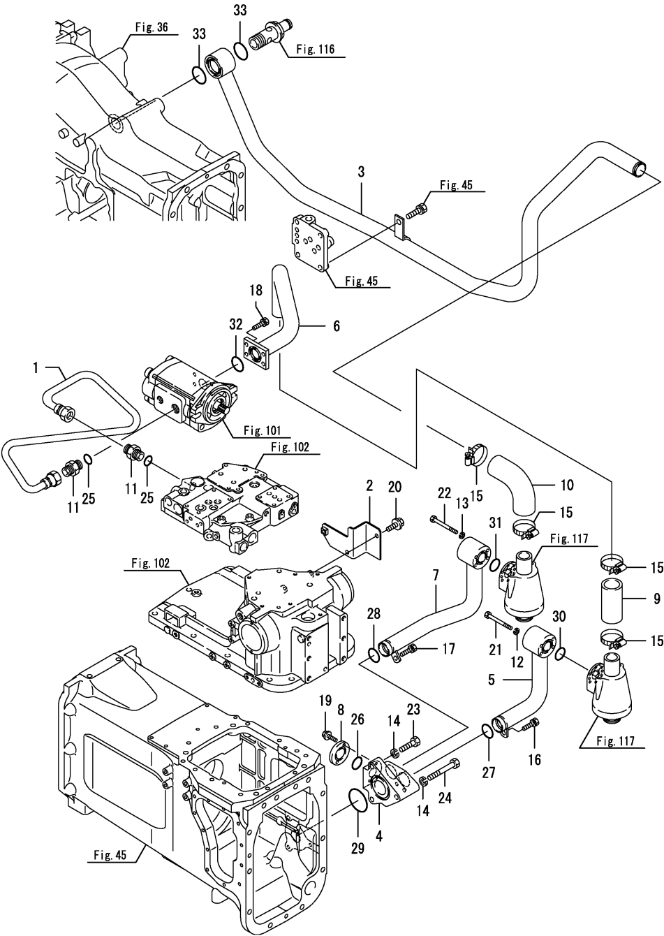
Fig.114. 유압배관(A)
