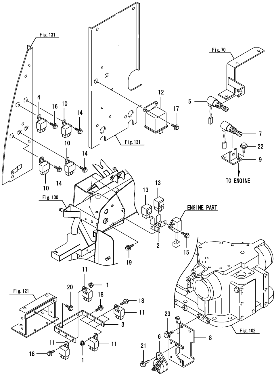
Fig.125. 스위치&릴레이(본기)
