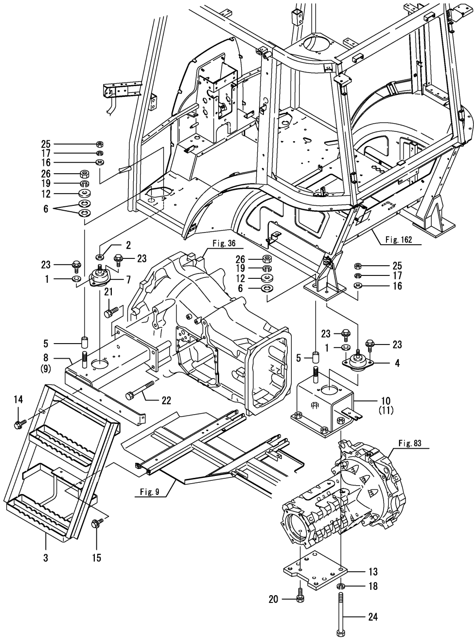
Fig.138. 바닥서포트
