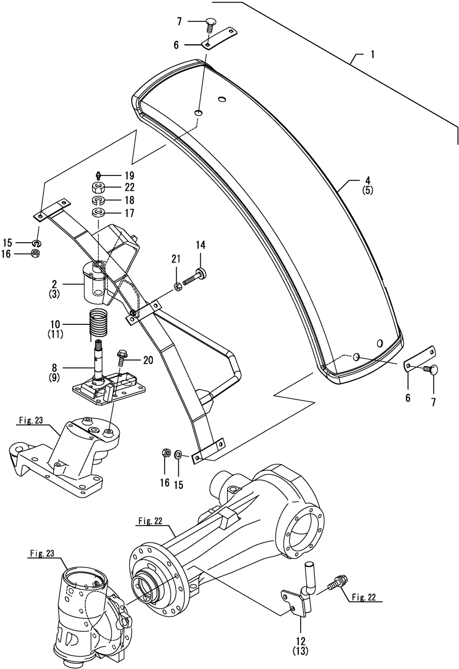
Fig.194. 프론트웬더
