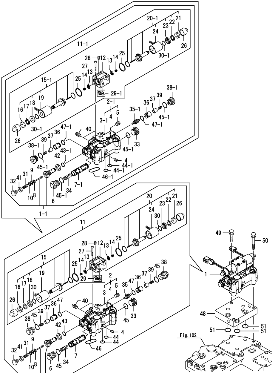
Fig.154. 수평 제어(U.F.O.)
