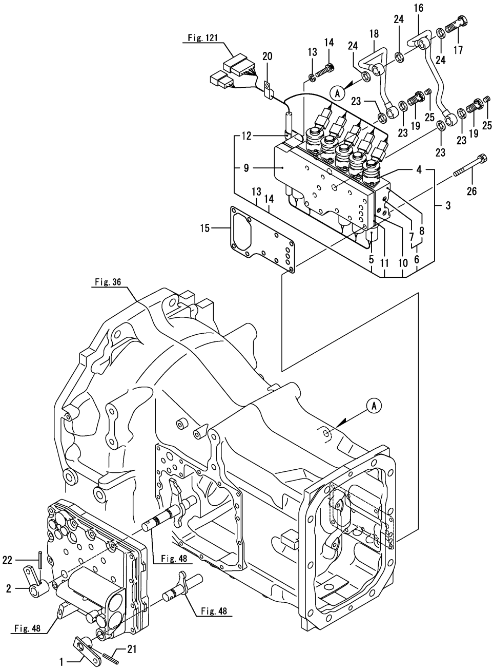
Fig.46. 레귤레이터(파워시프트)
