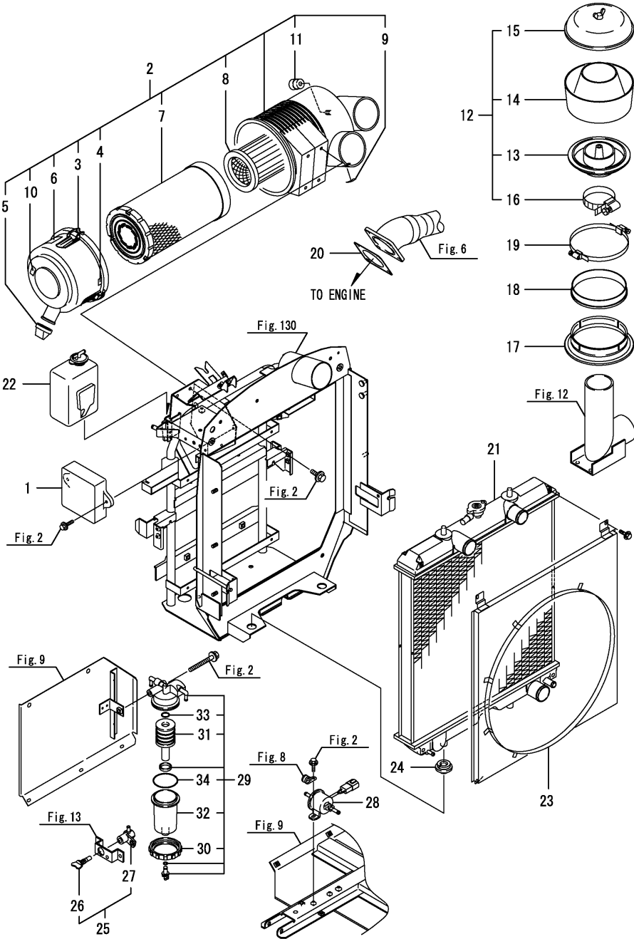
Fig.1. 엔진관련
