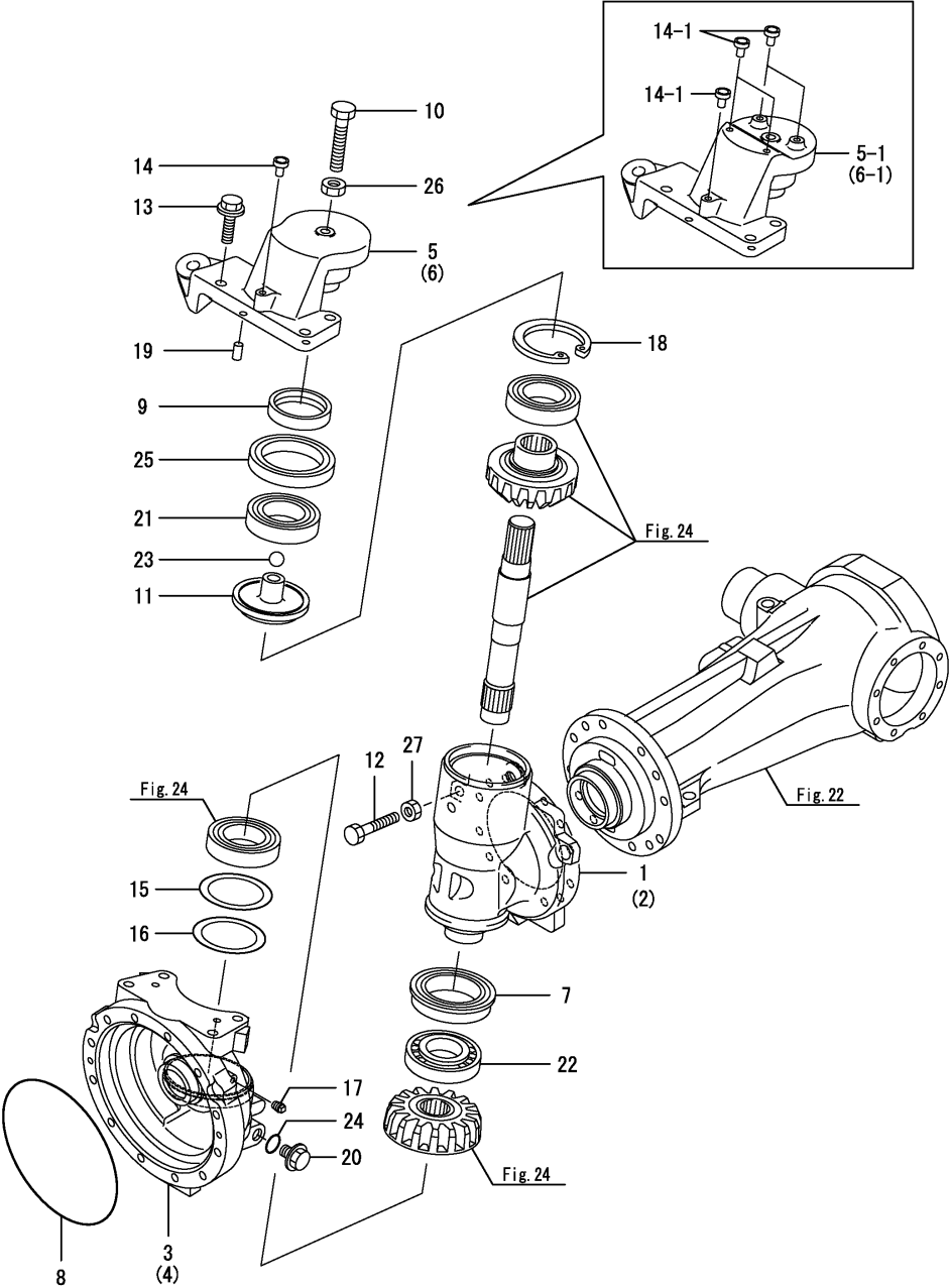
Fig.23. 프론트기어케이스
