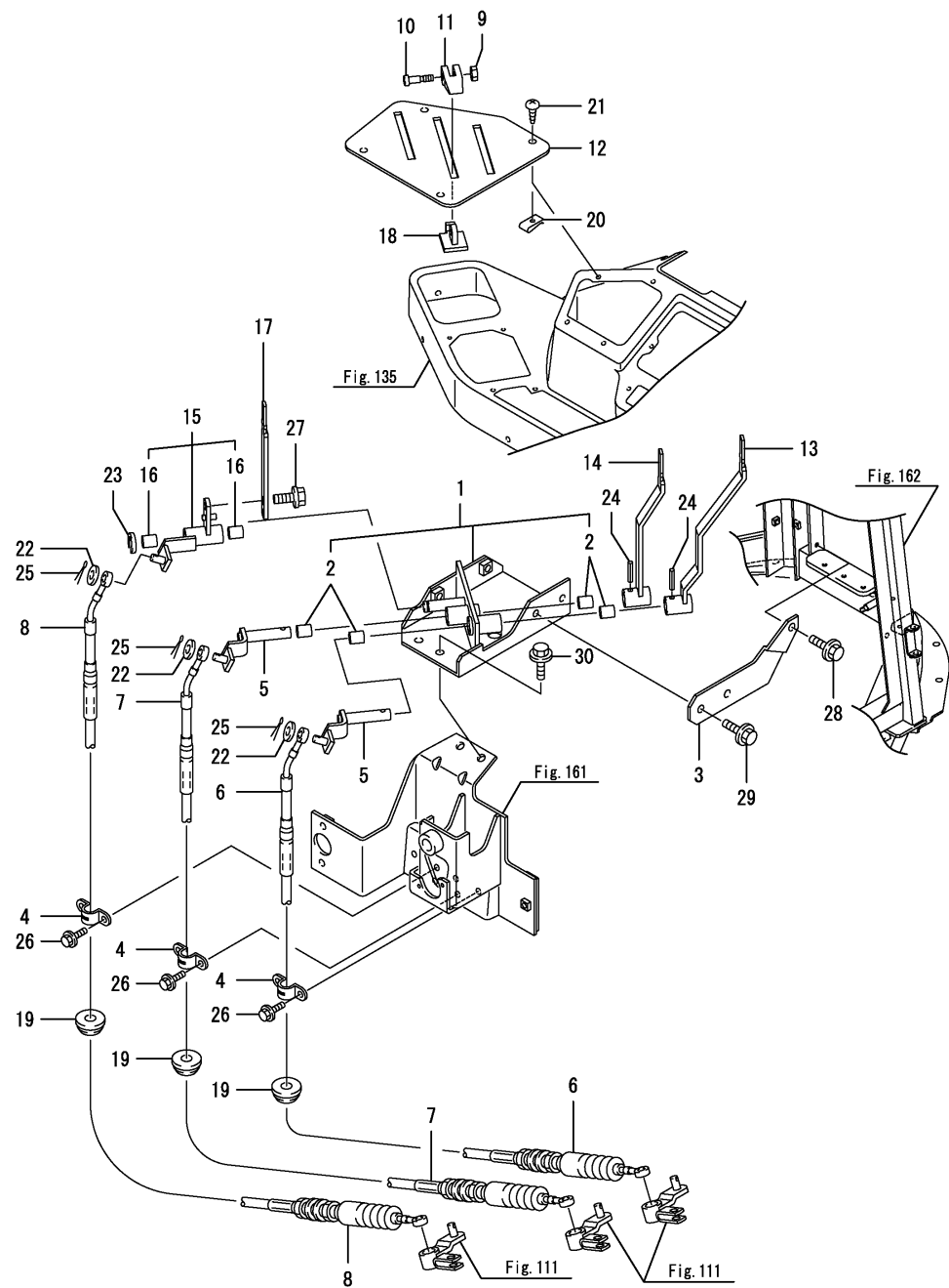
Fig.112. S.C.V.컨트롤(3련)
