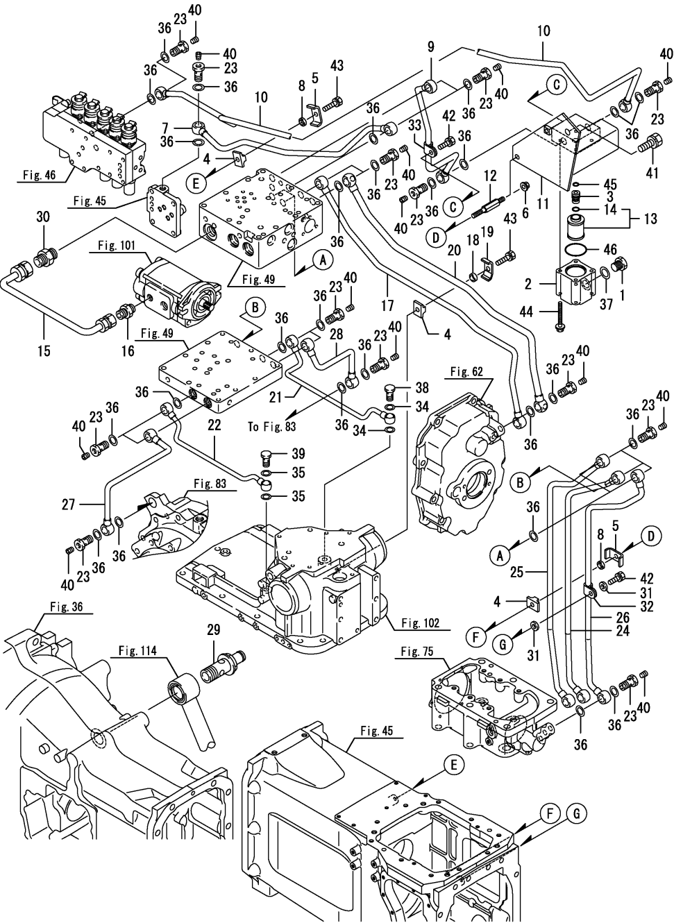
Fig.116. 유압배관(B)
