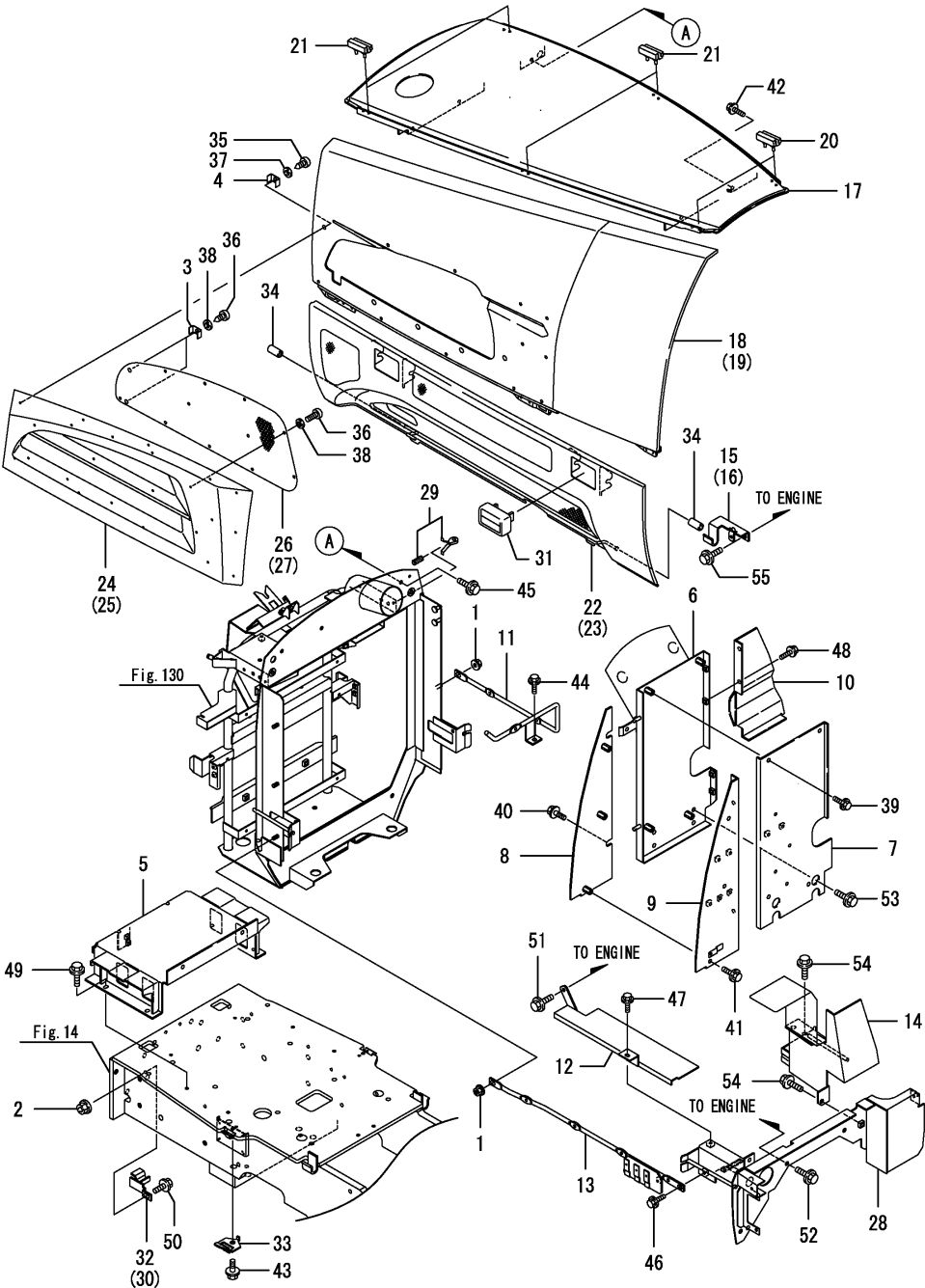
Fig.131. 본네트
