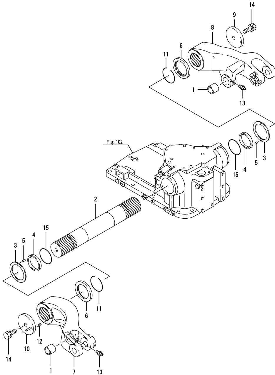
Fig.104. 리프트크랭크
