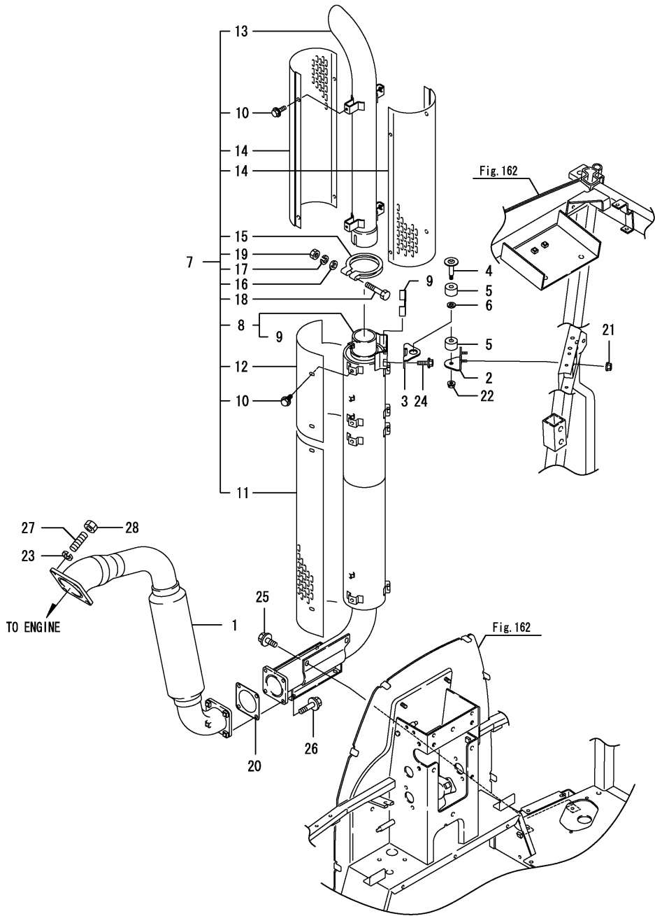
Fig.6. 배기구
