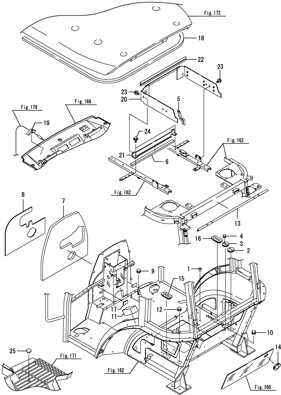
Fig.170. 캐빈시일(캐빈)
