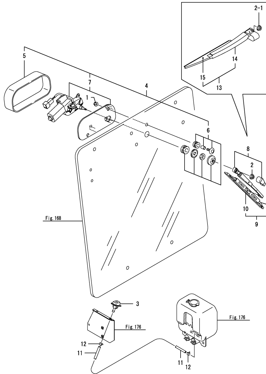
Fig.178. 후방와이퍼
