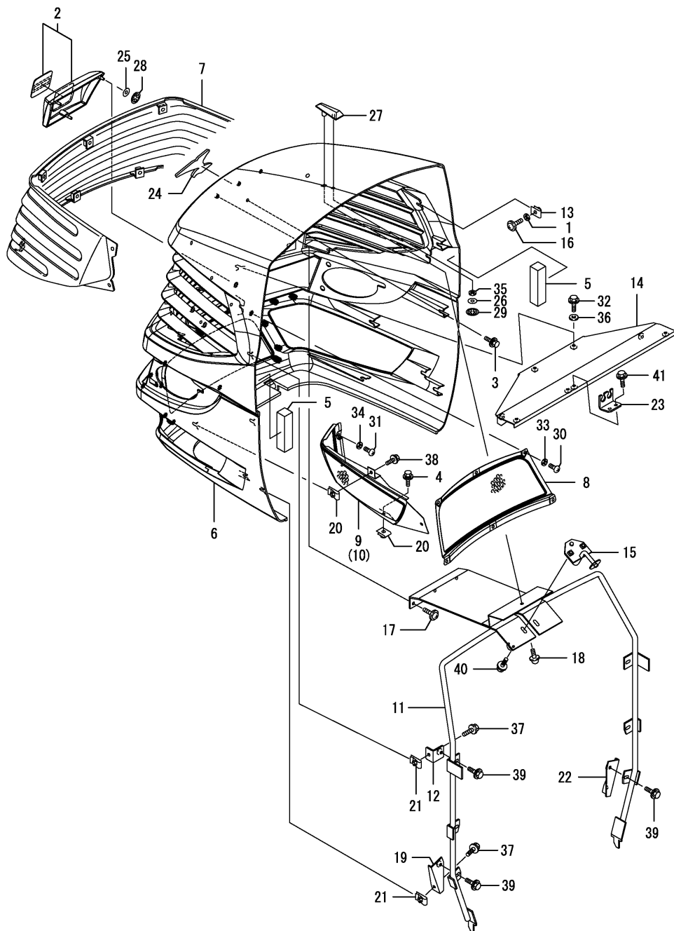
Fig.133. 프론트그릴
