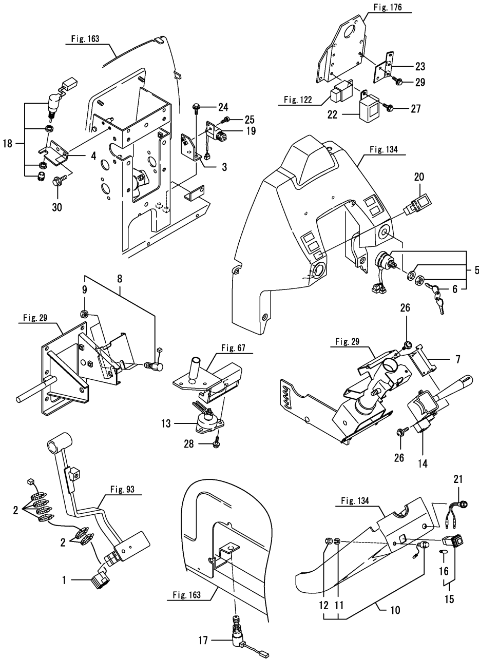
Fig.124. 스위치&릴레이(캐빈)
