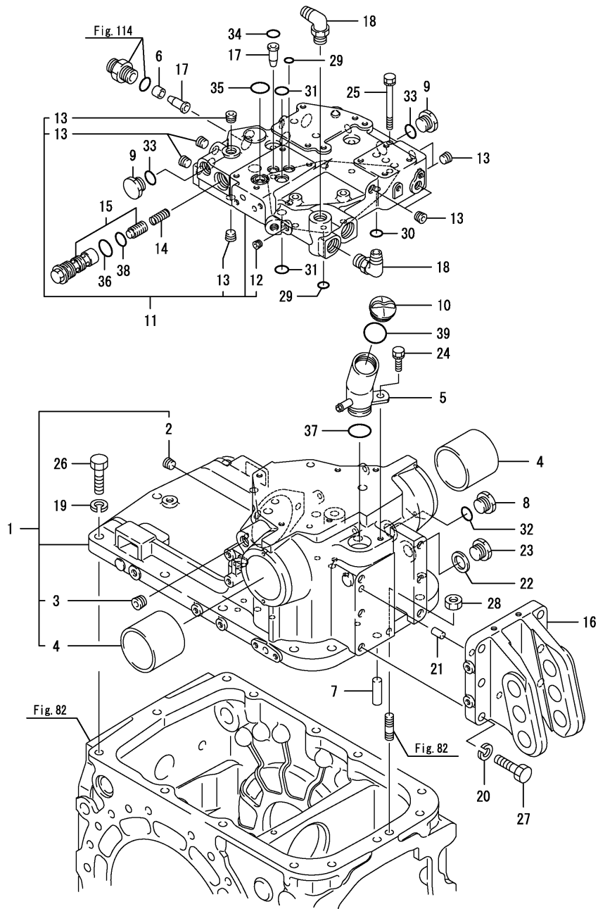
Fig.102. 유압실린더케이스
