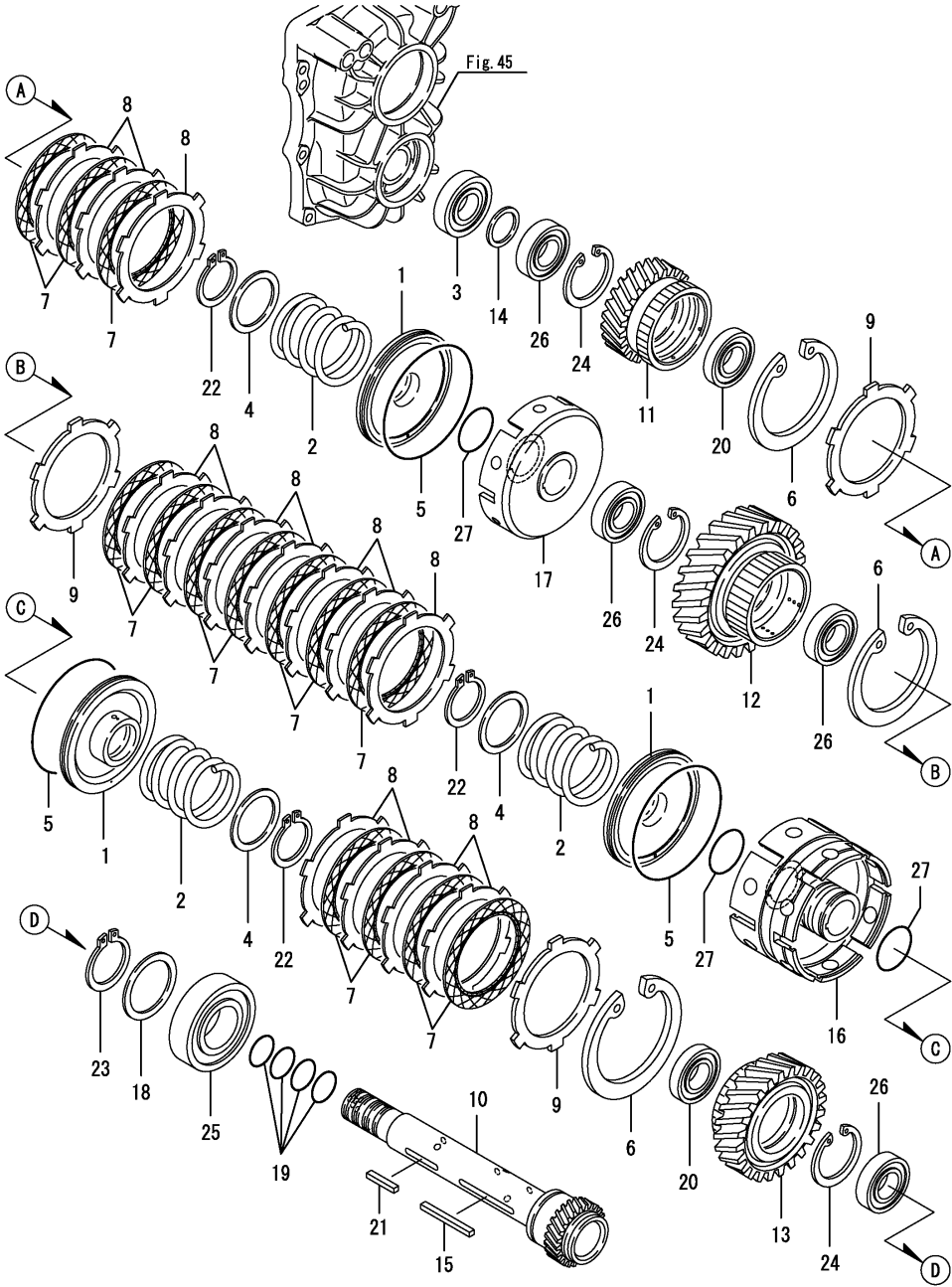
Fig.55. P.S.C.축(후)
