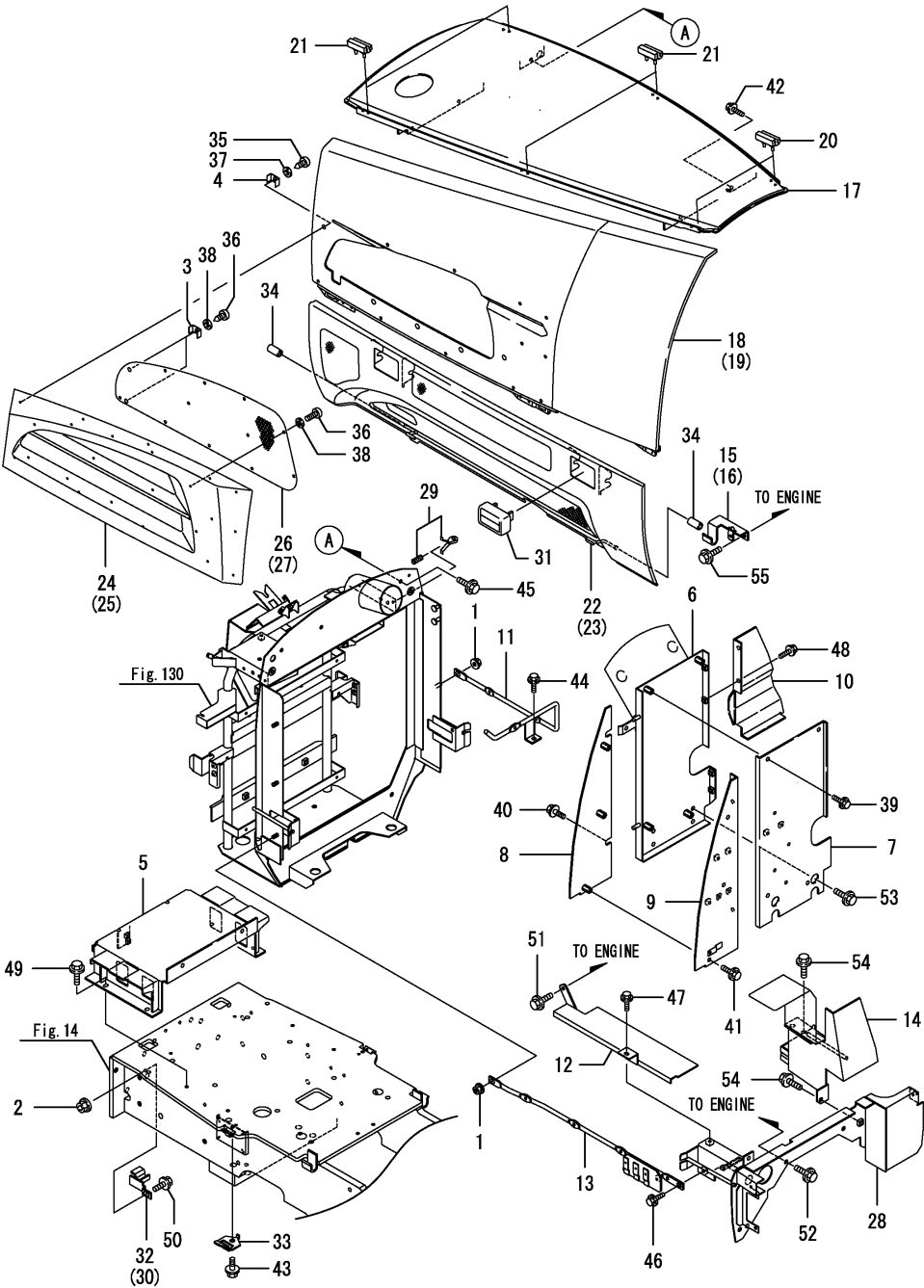
Fig.131. 본넷
