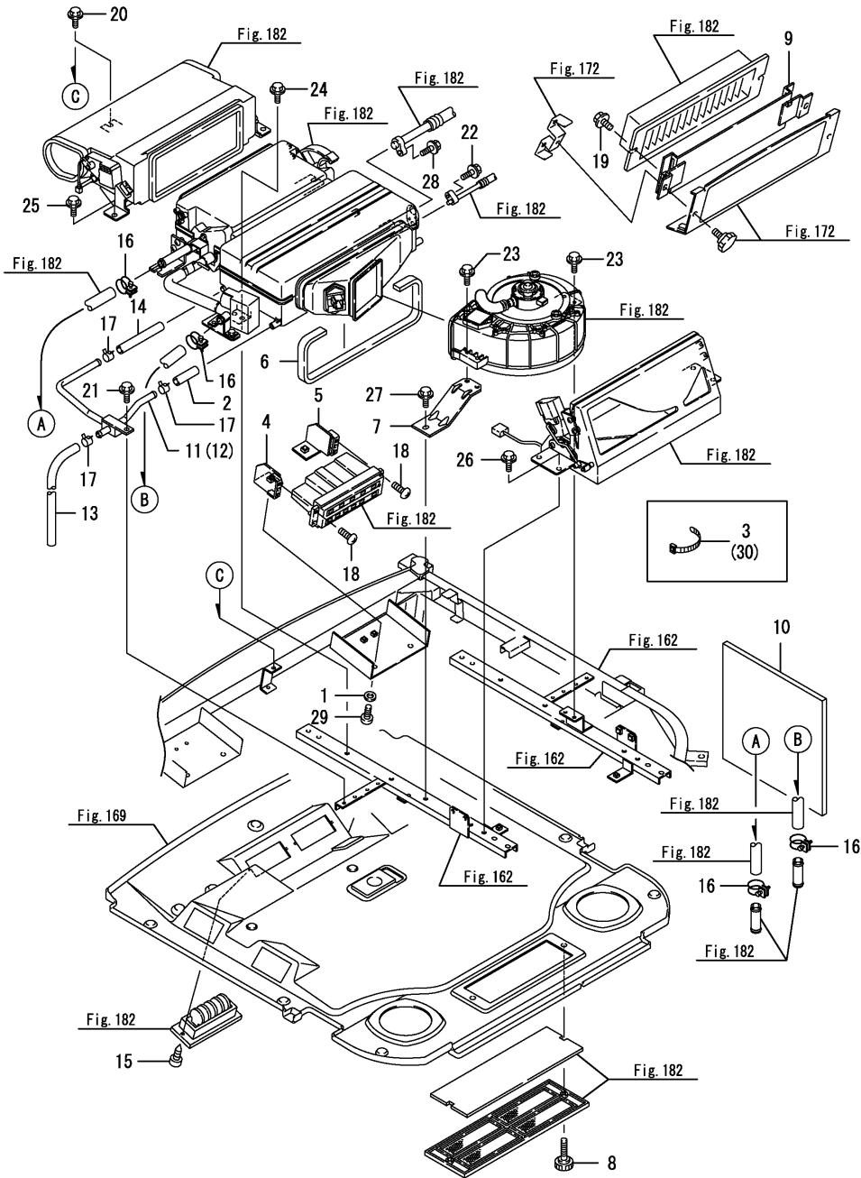
Fig.183. 에어컨(캐빈)
