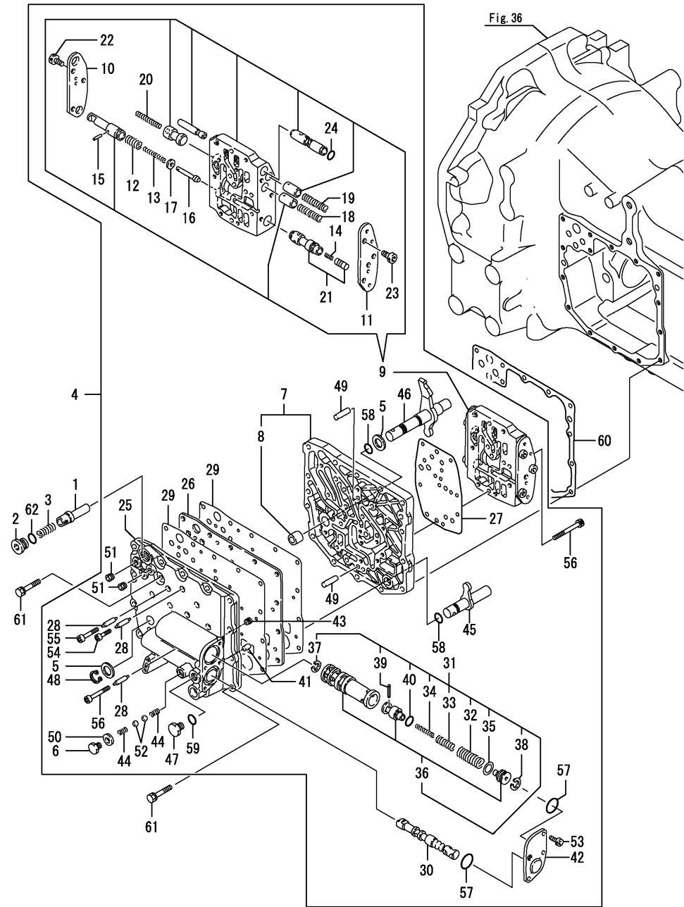
Fig.48. 레클레이터(파워리버서)
