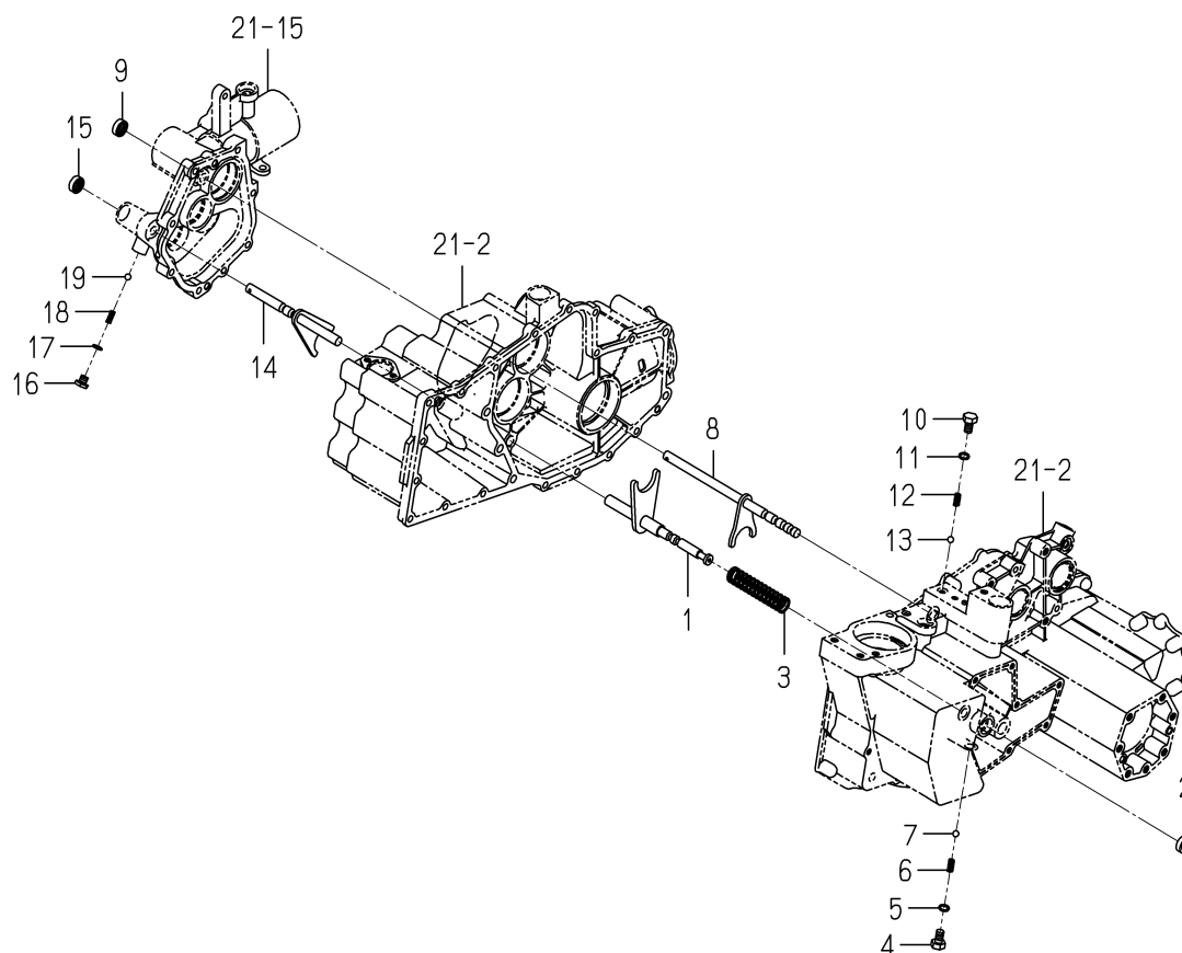
FIG. 35 SHIFTER(CHANGE)SYSTEM
