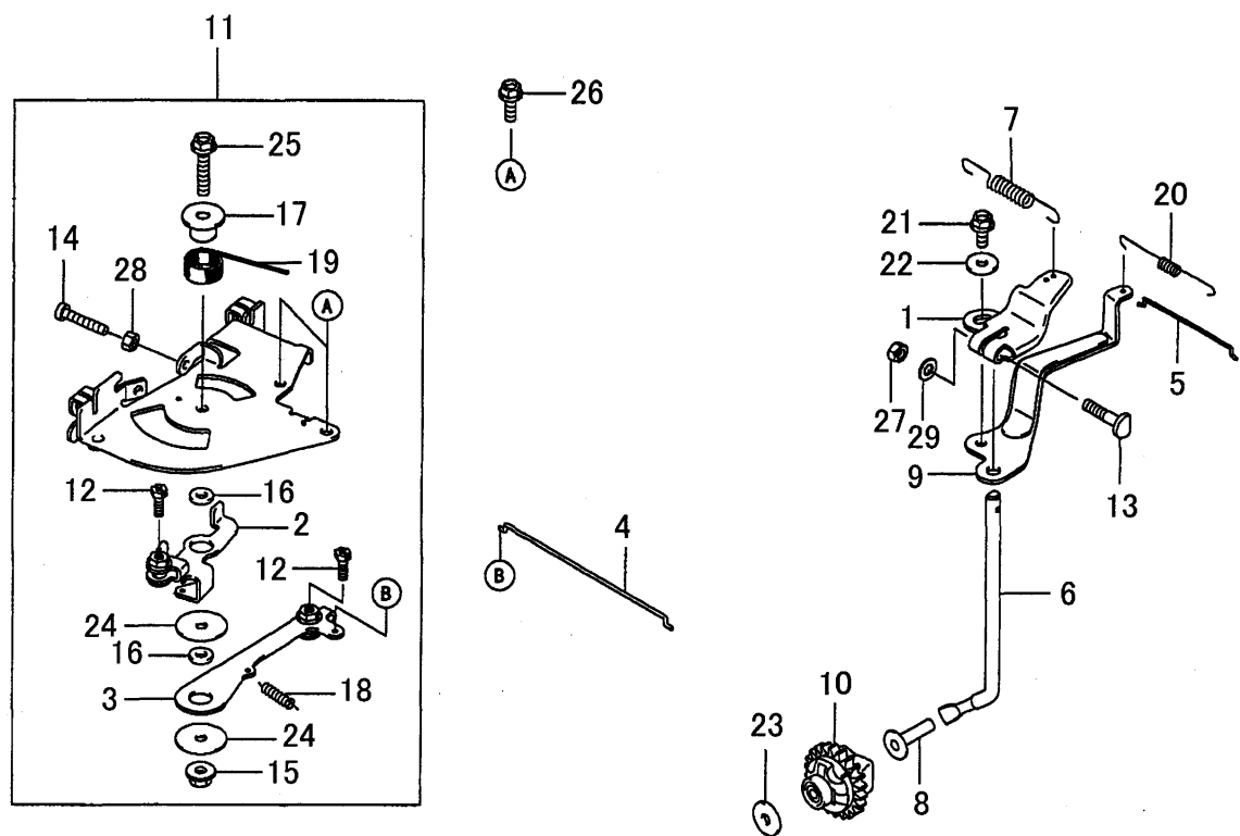
FIG. 7 CONTROL-EQUIPMENT
