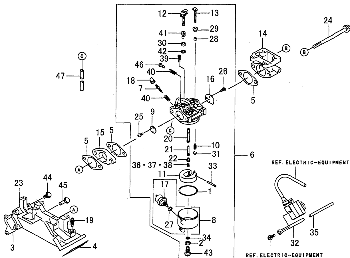
FIG. 8 CARBURETOR
