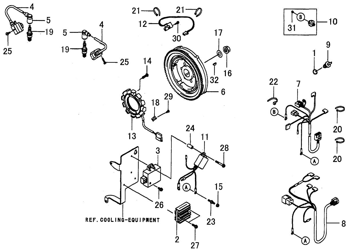
FIG. 6 ELECTRIC-EQUIPMENT
