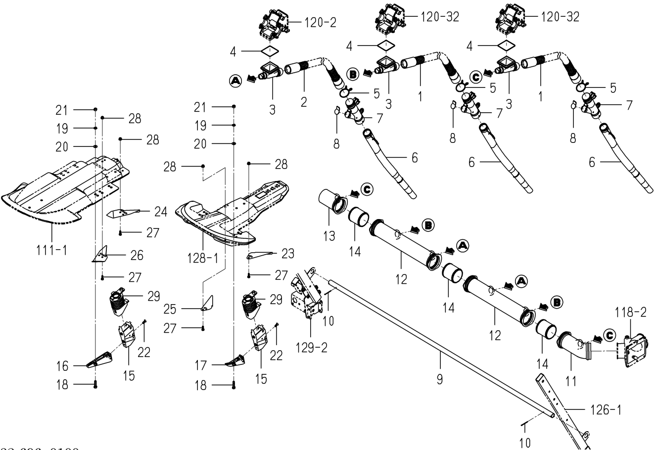
FIG.122 PIPING(FERTILIZER)SYSTEM
