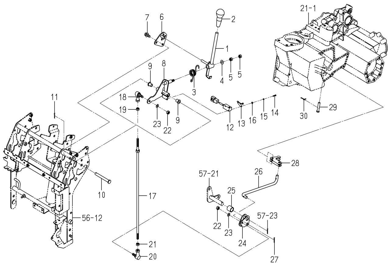
FIG. 14 LEVER(CHANGE)SYSTEM
