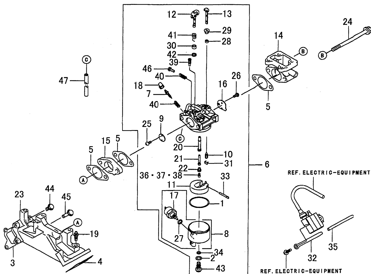
FIG. 8 CARBURETOR
