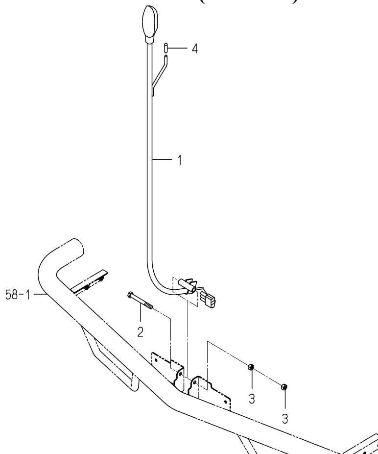
FIG. 86 MARKER(CENTER)SYSTEM
