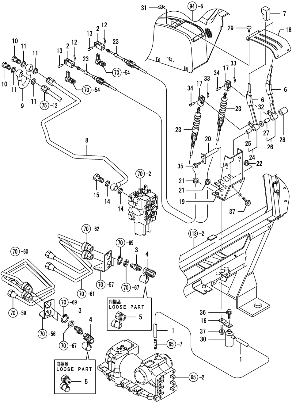
Fig.71. S.C.V.컨트롤
