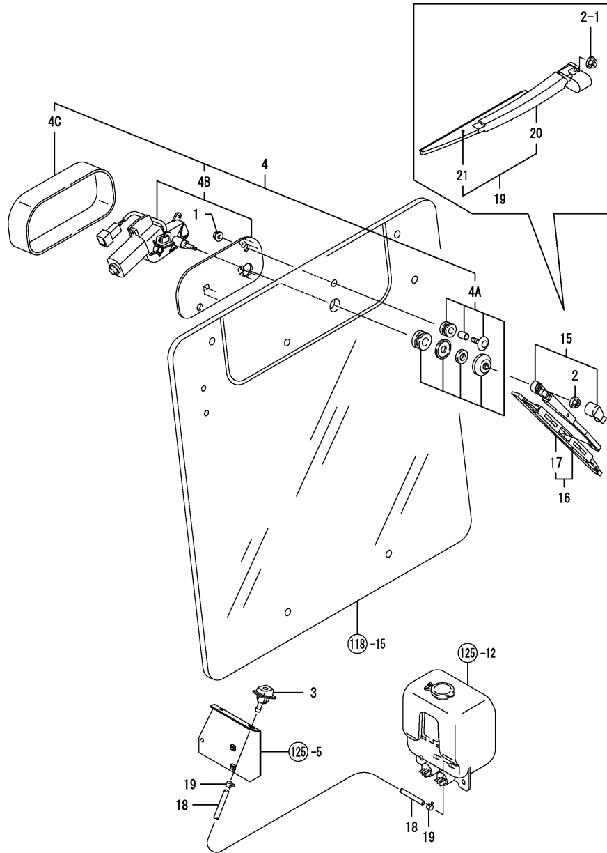
Fig.126. 후방와이퍼
