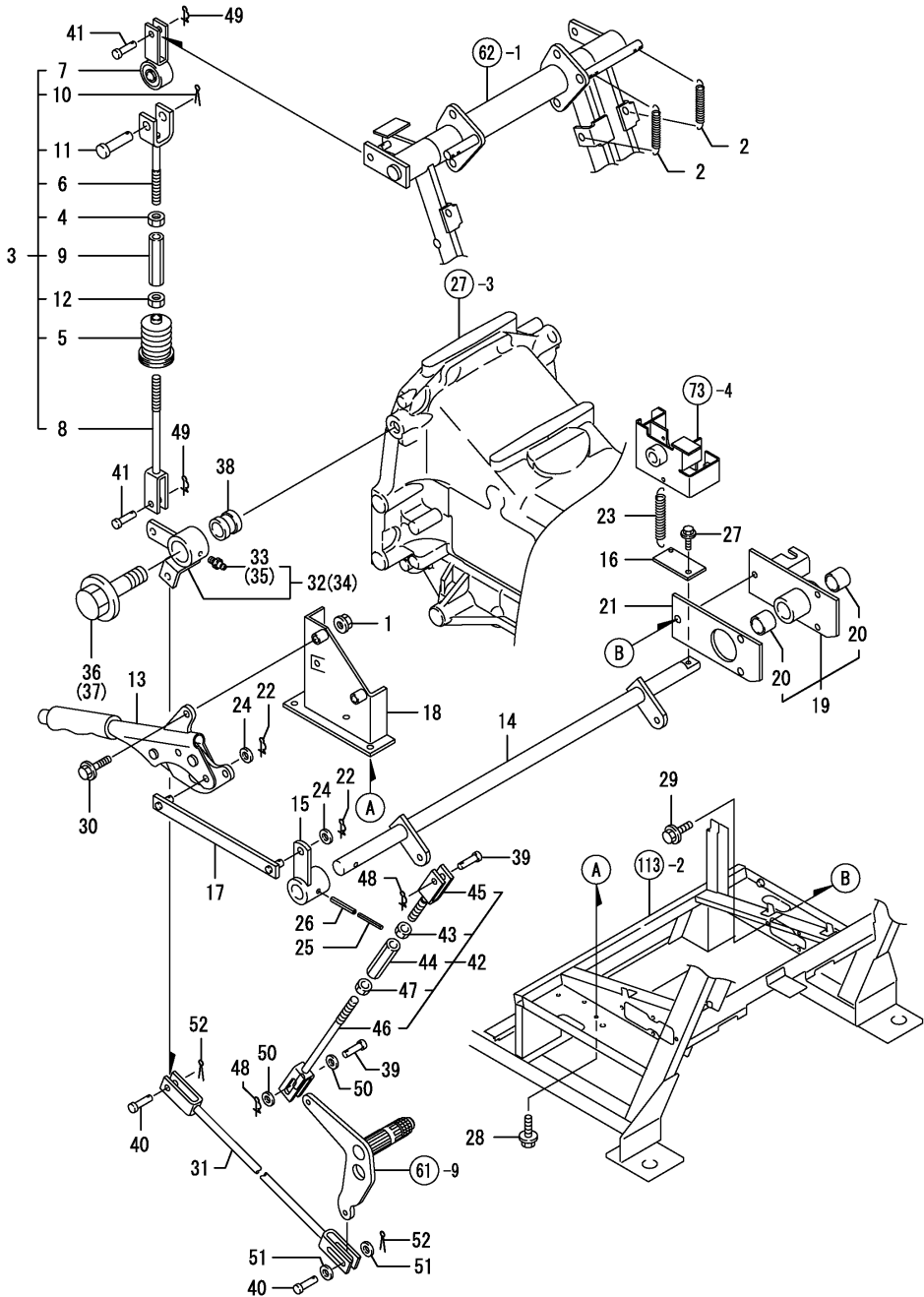
Fig.63. 브레이크링크
