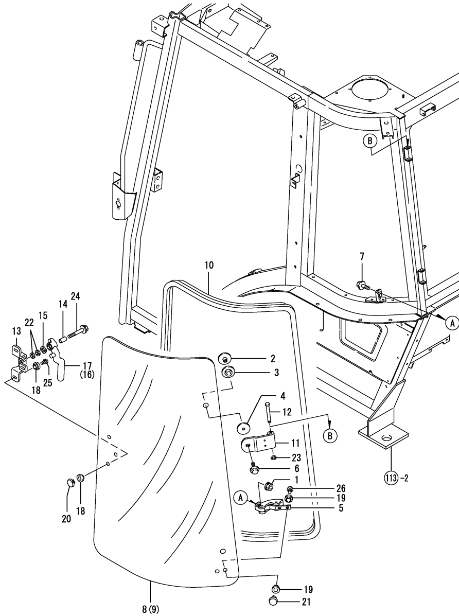
Fig.117. 측방창문
