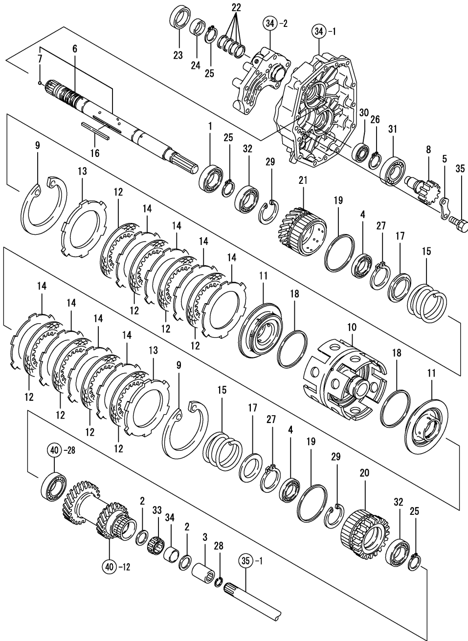
Fig.39. 파워리버서
