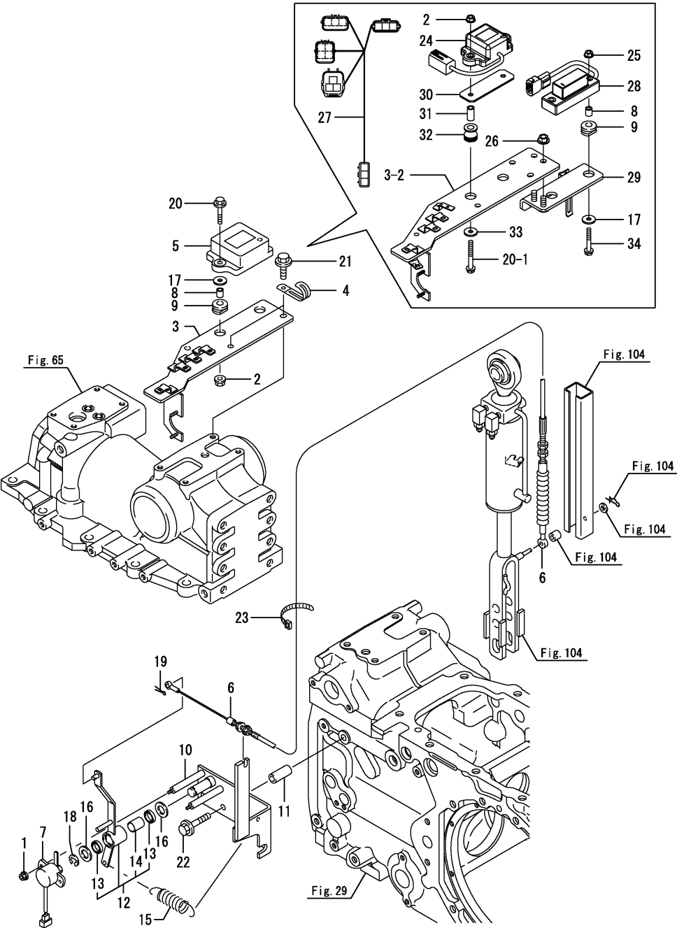
Fig.109. 수평 제어센서
