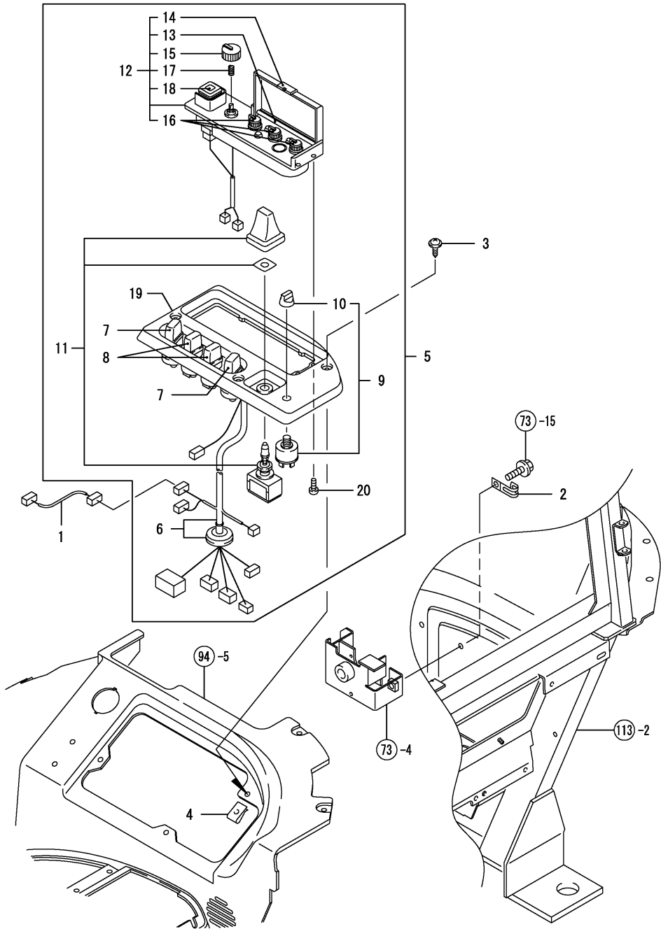
OCNP4-M59400 히치부 Fig.110. 컨트롤박스
