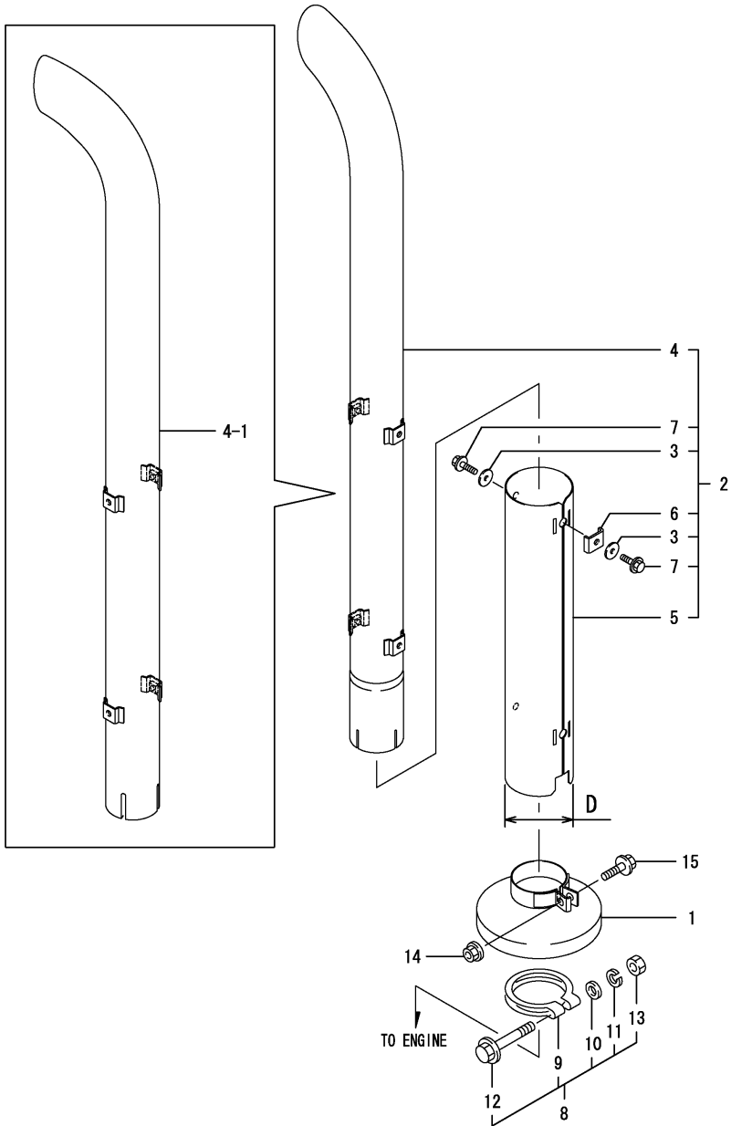
Fig.5. 배기구
