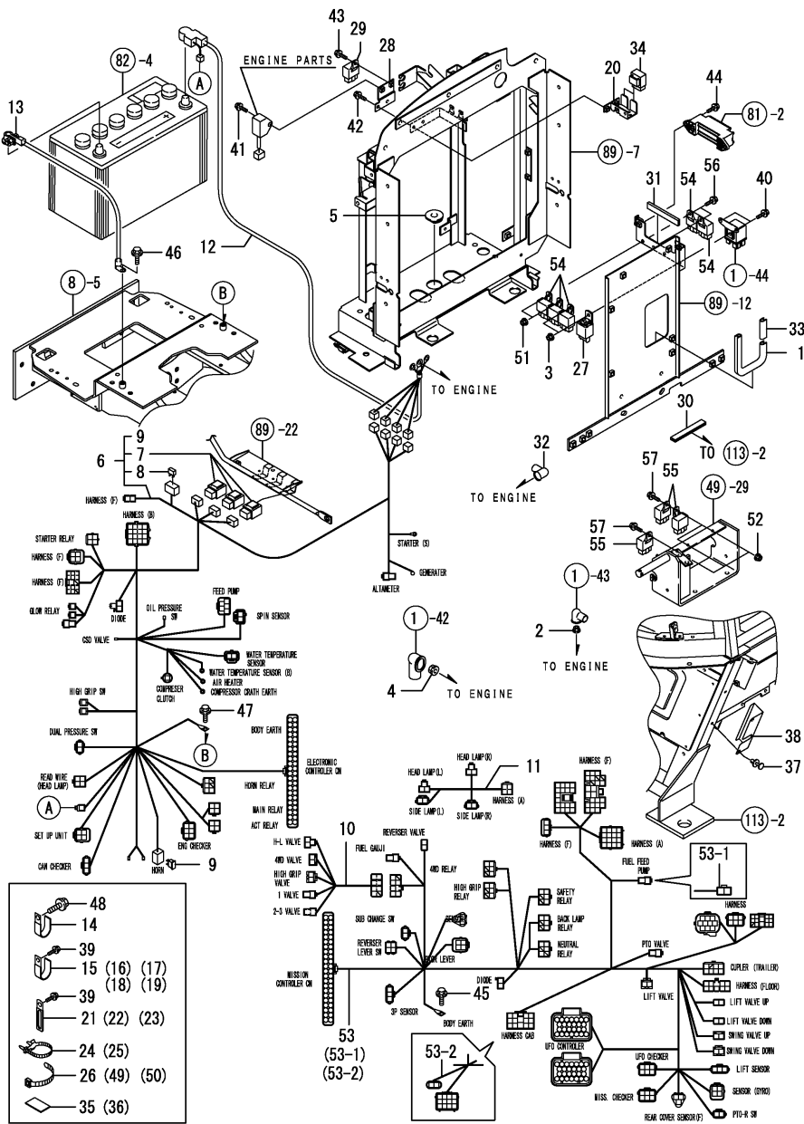
Fig.80. 배선
