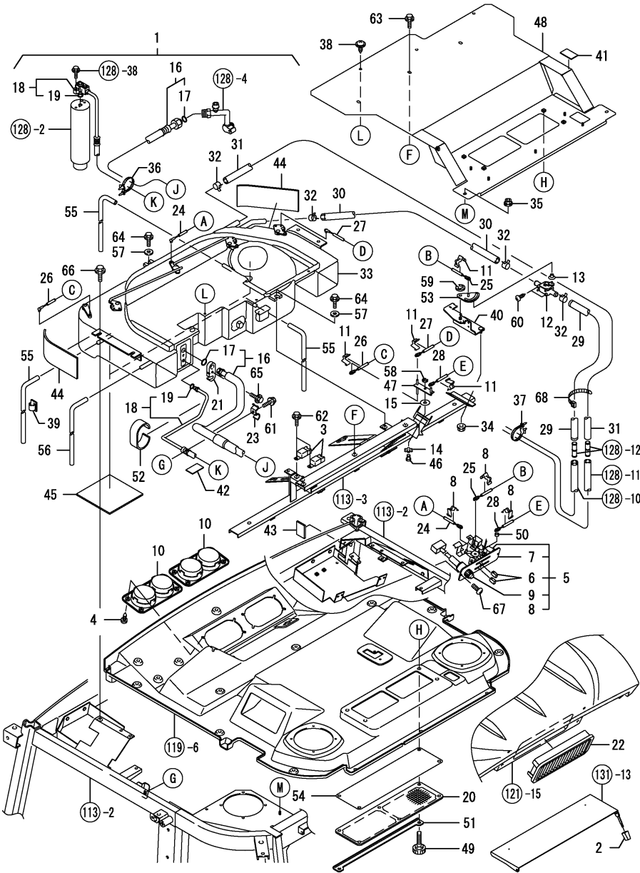
Fig.129. 에어컨(2)
