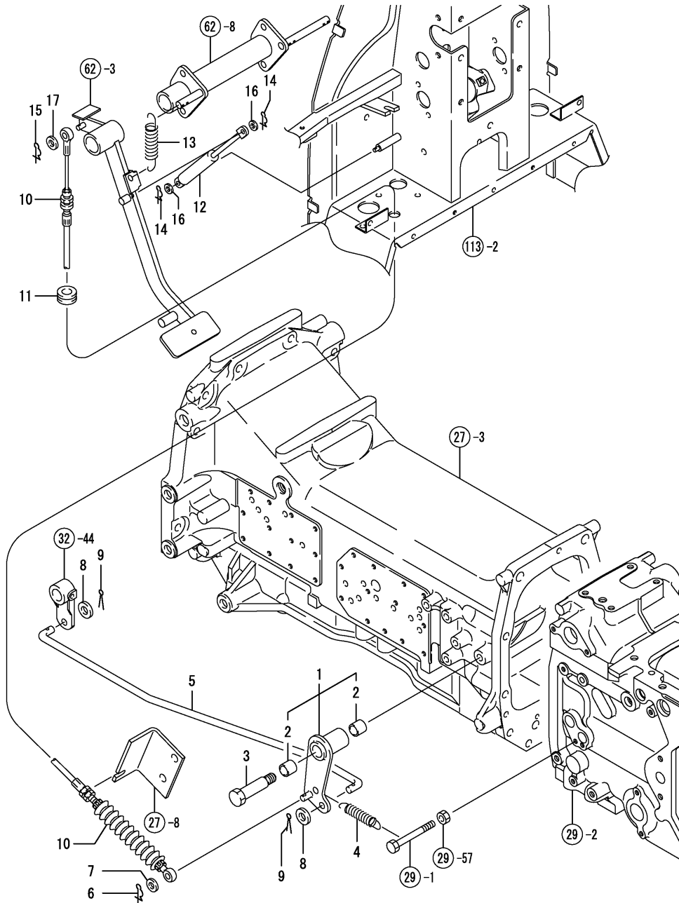
Fig.28. 클러치링크
