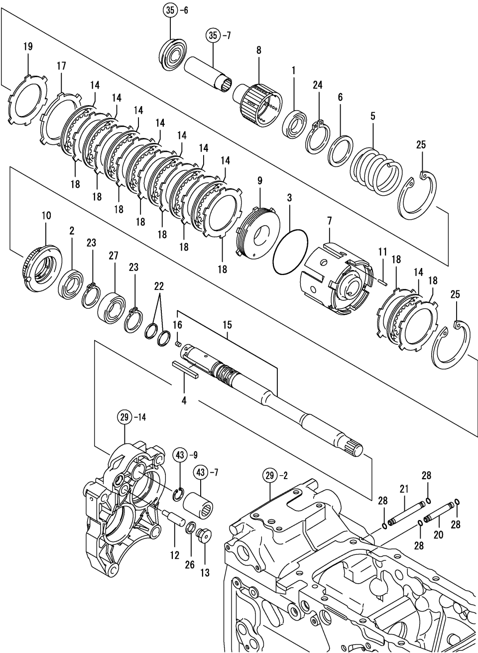
Fig.42. P.T.O. 클러치
