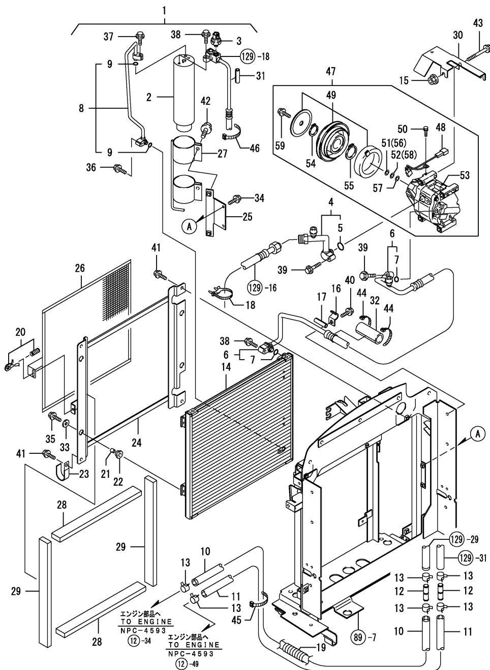
Fig.128. 에어컨(1)
