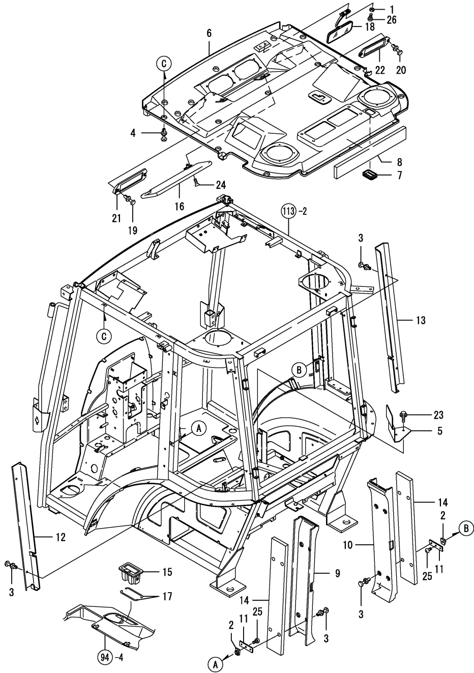
Fig.119. 인테리어
