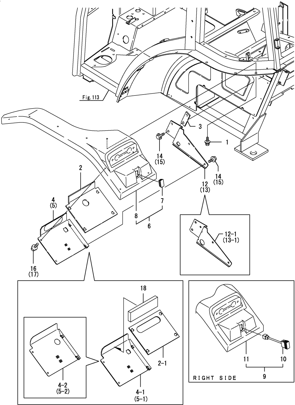
Fig.95. 오버휰더
