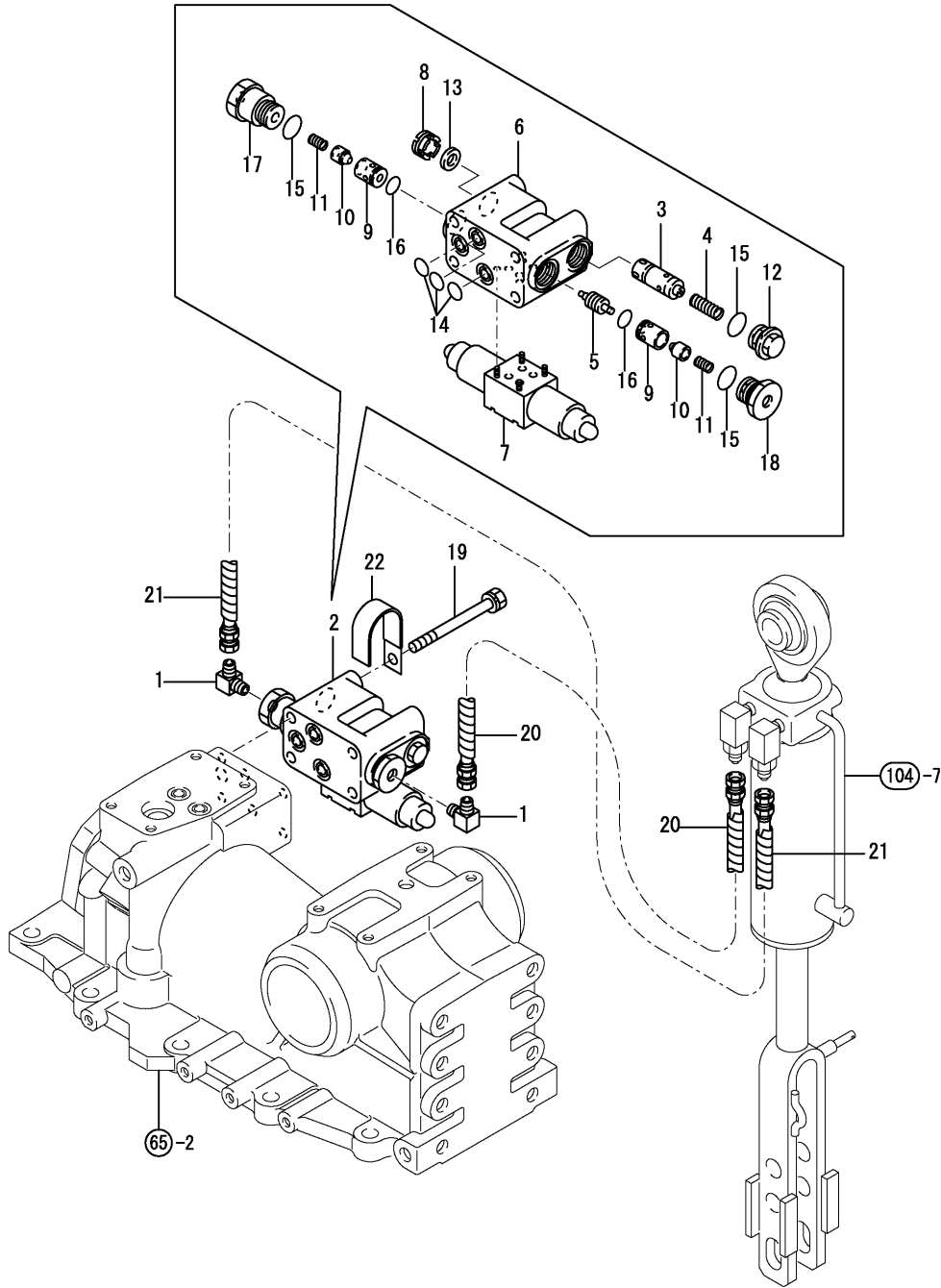
Fig.108. 수평 제어밸브
