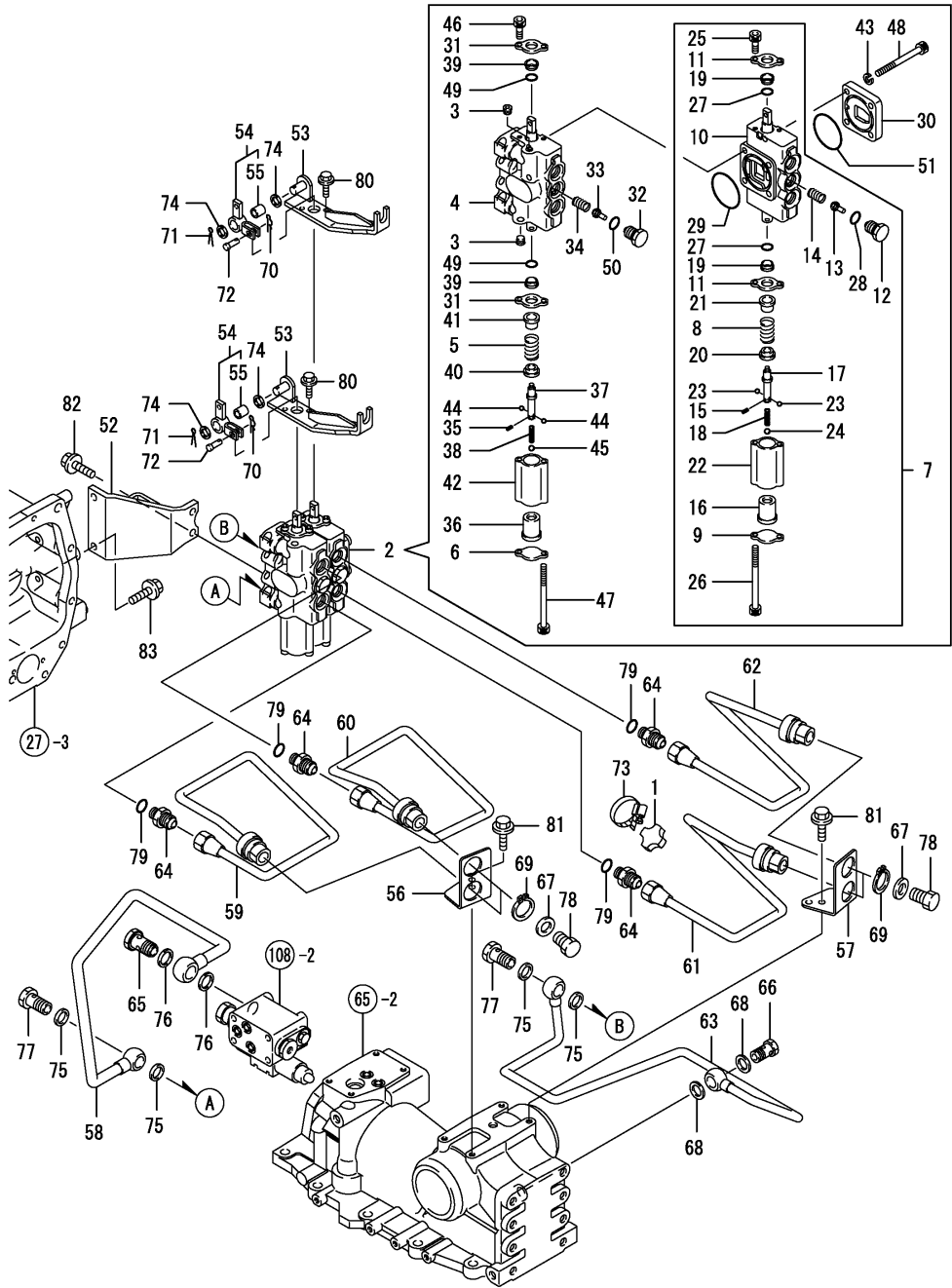
Fig.70. 보조컨트롤밸브
