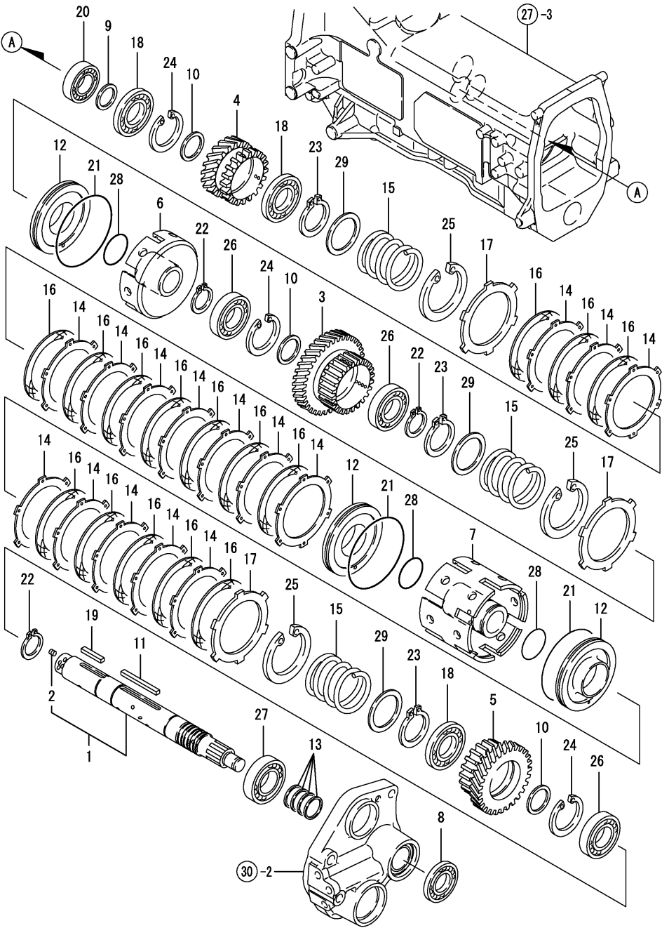
Fig.36. 클러치축
