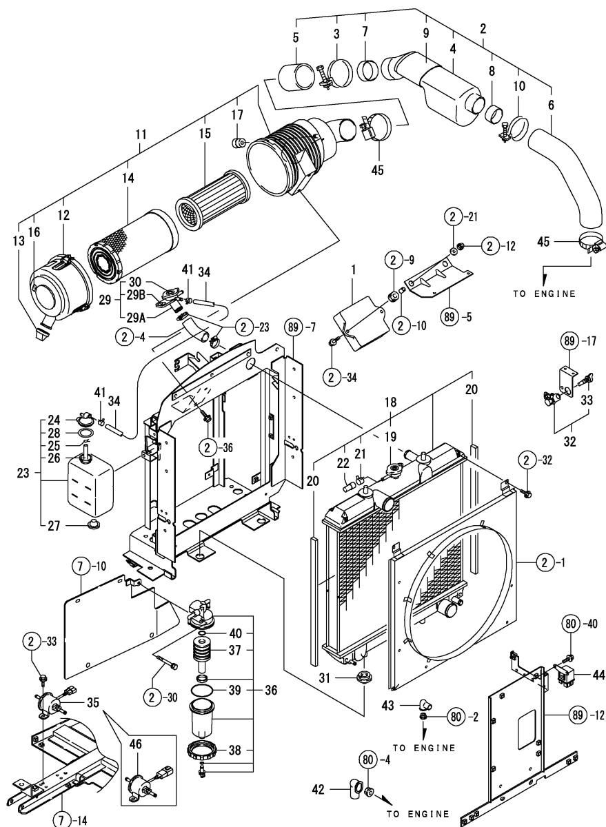
Fig.1. 엔진관련
