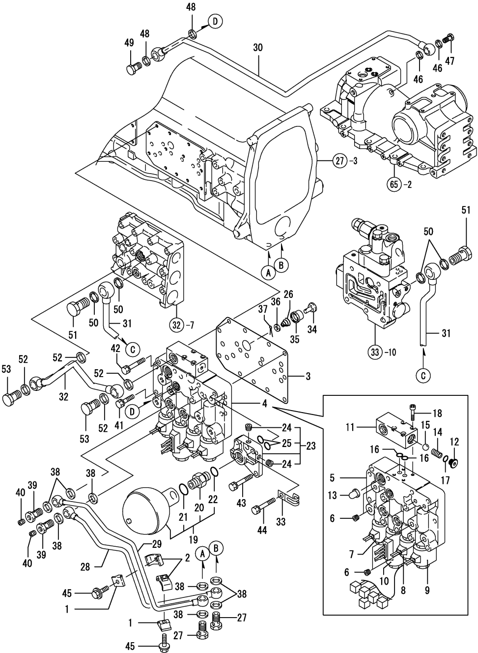
Fig.31. 메인밸브
