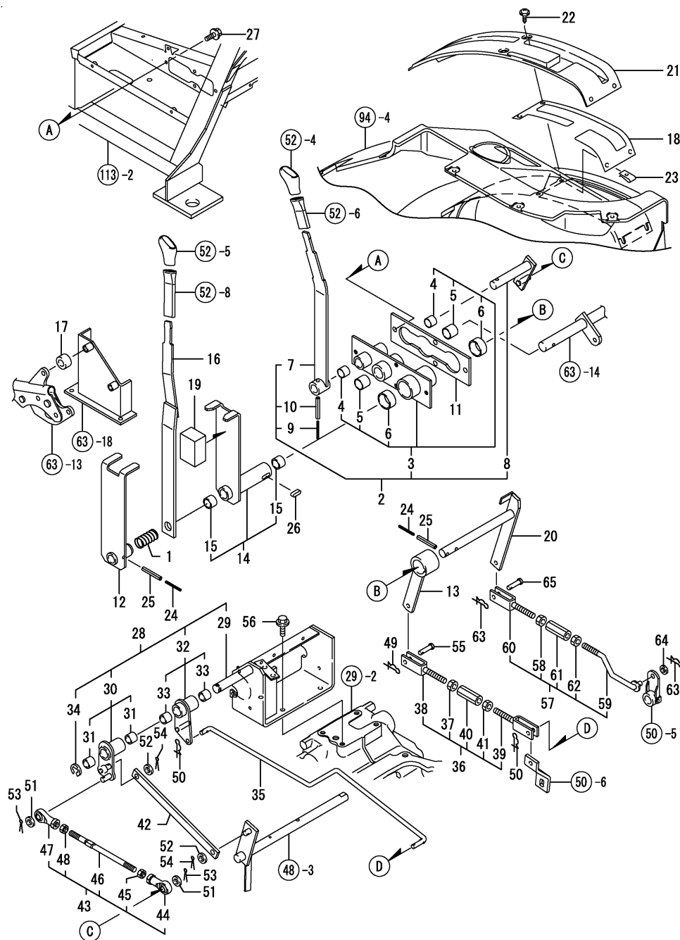
Fig.49. 보조레버
