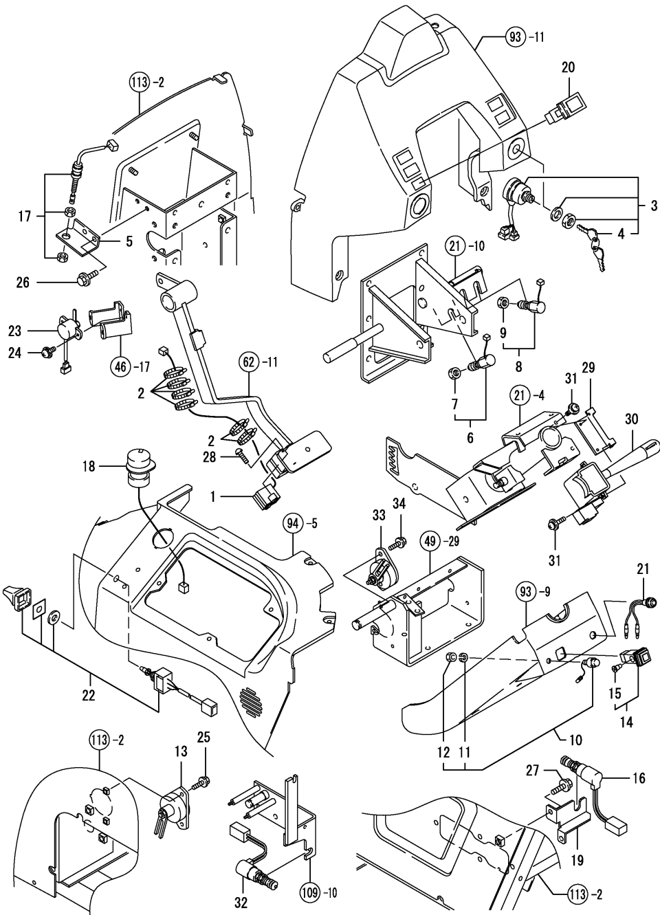
Fig.83. 스위치
