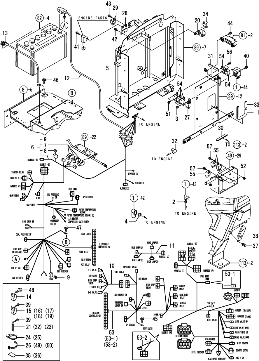
Fig.80. 배선
