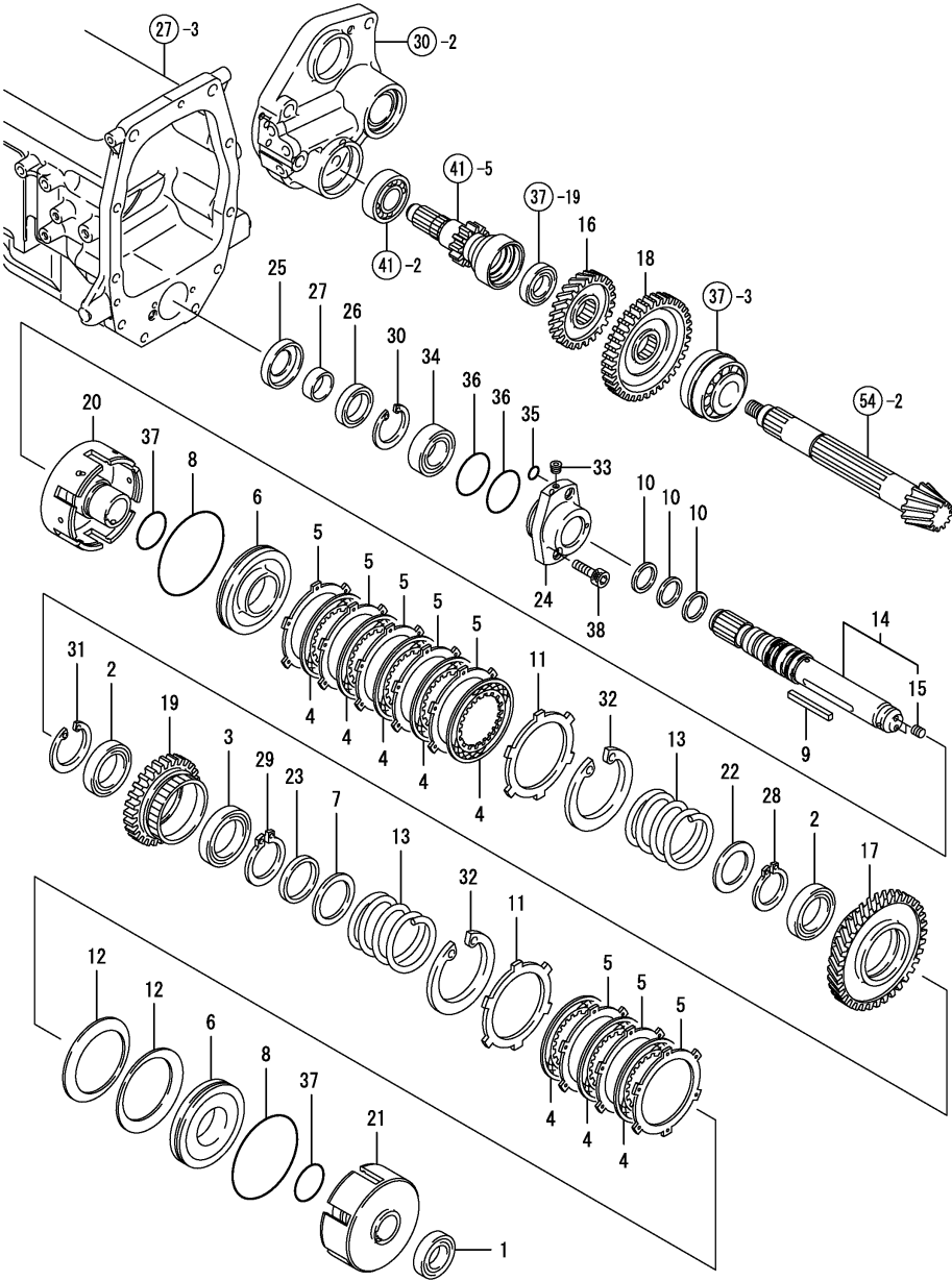
Fig.53. 전륜구동
