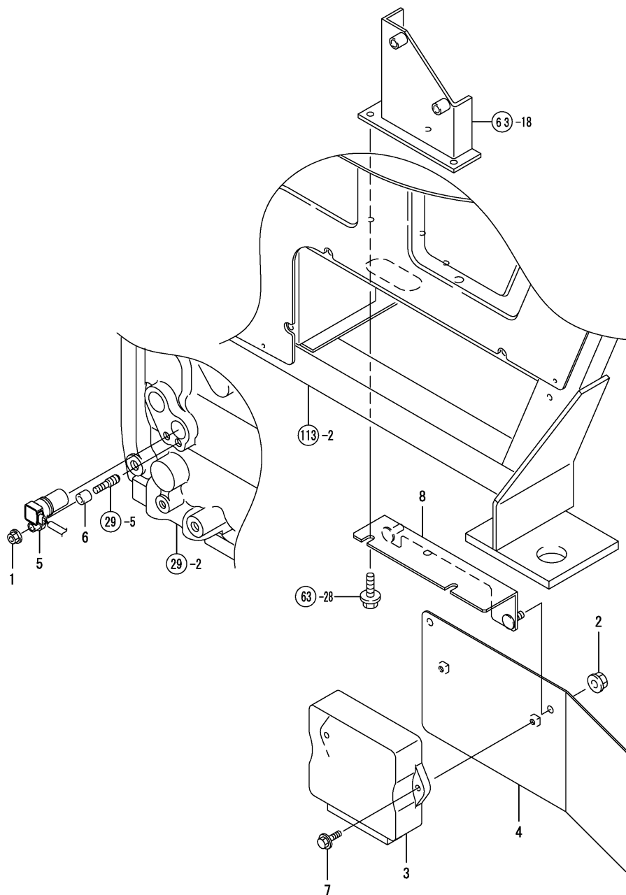
Fig.51. 컨트롤러
