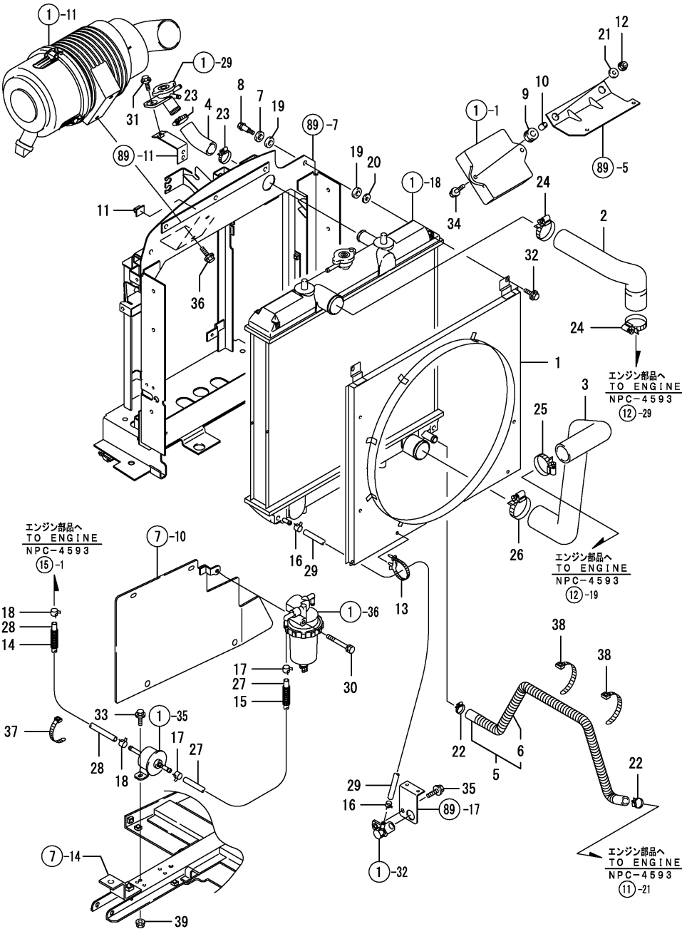
Fig.2. 엔진악세사리
