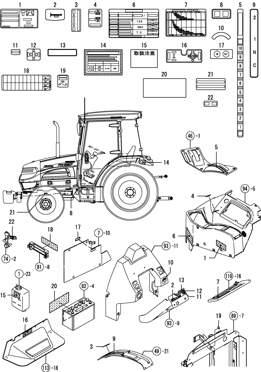
Fig.99. 명판
