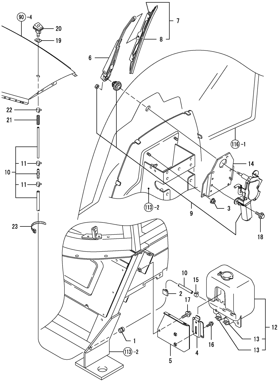
OCNP4-M59400 캐빈부 Fig.125. 전방와이퍼
