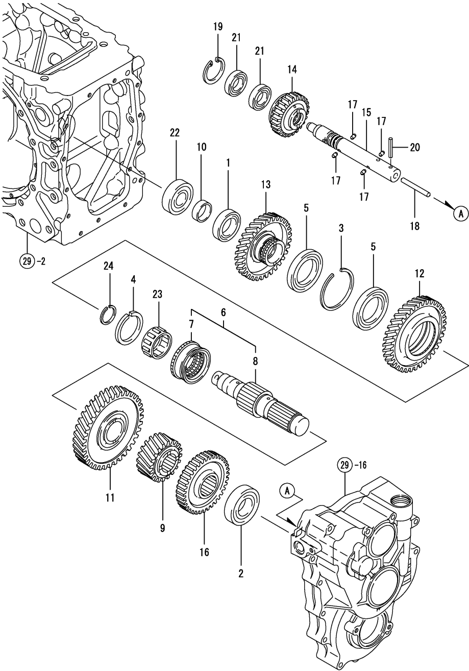
Fig.44. P.T.O. 피구동축
