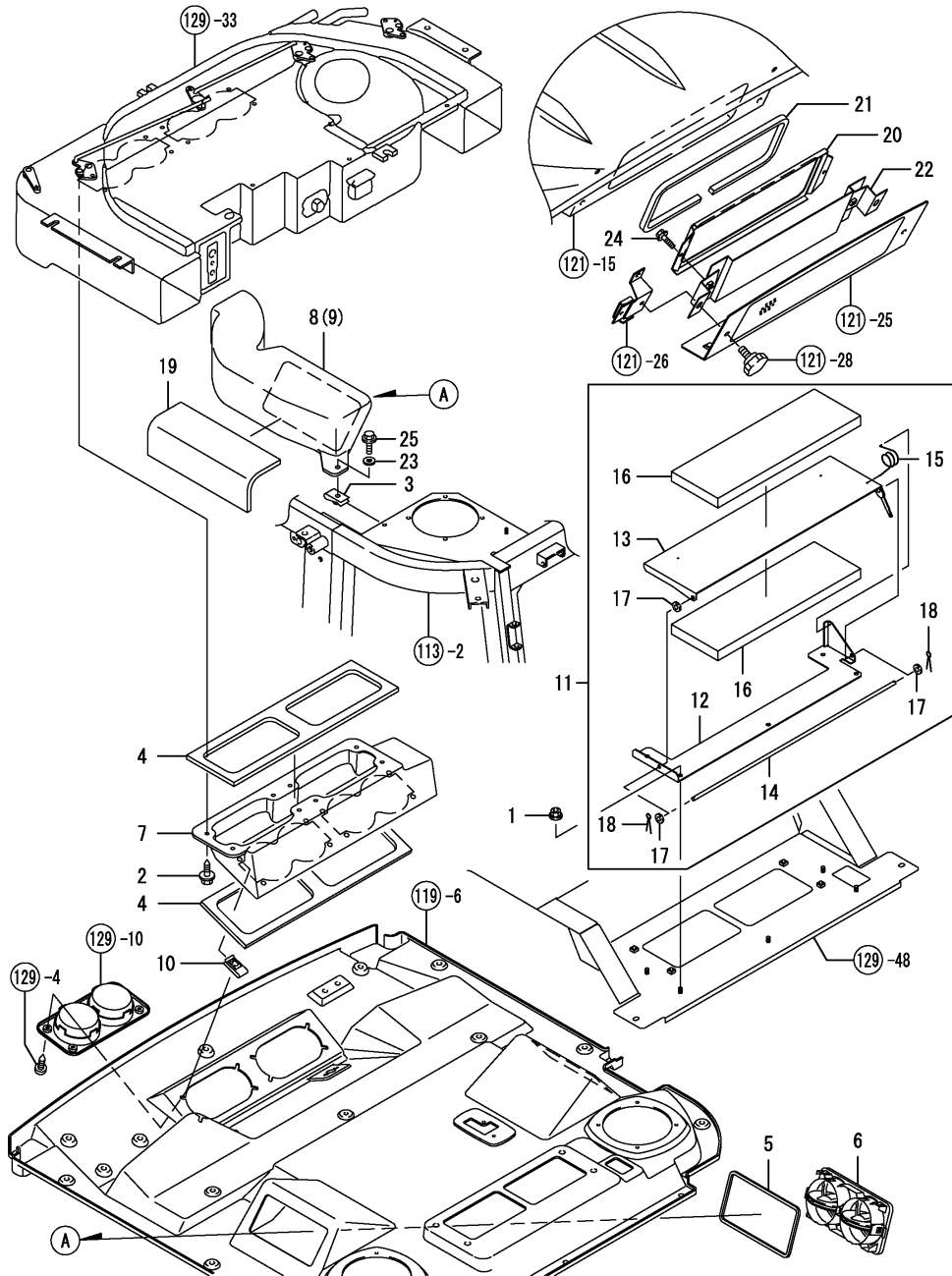
Fig.131. 에어컨덕트
