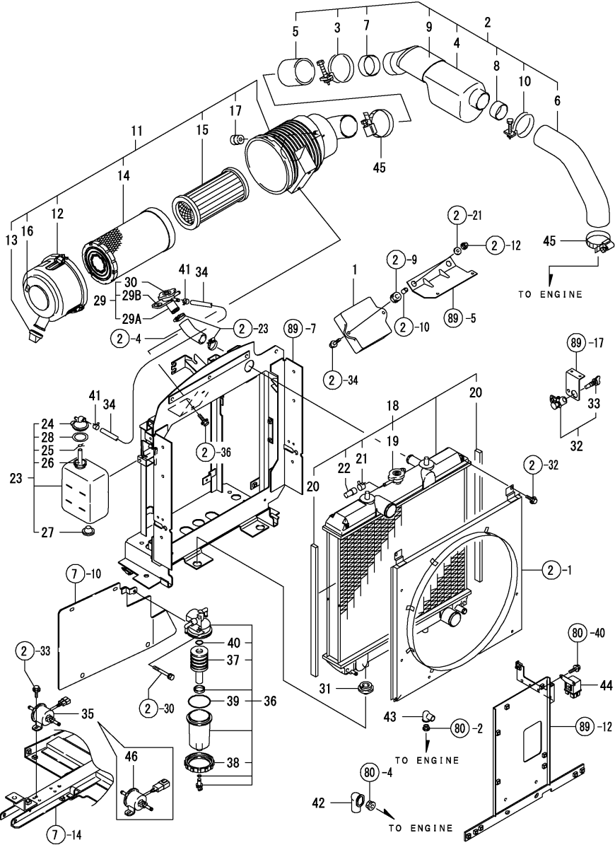
Fig.1. 엔진관련
