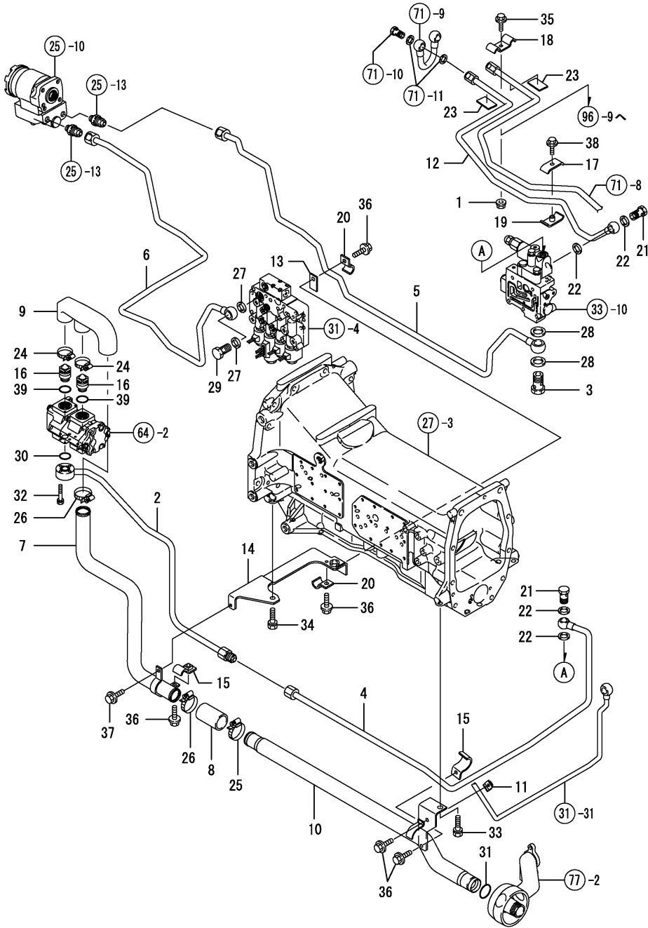
Fig.75. 유압배관
