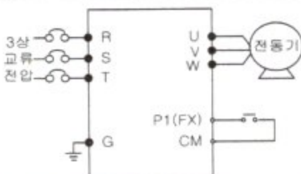
결선도
