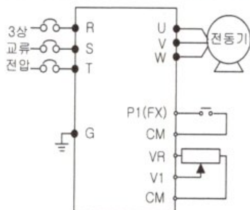
결선도
