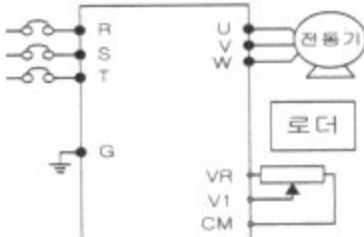
결선도
