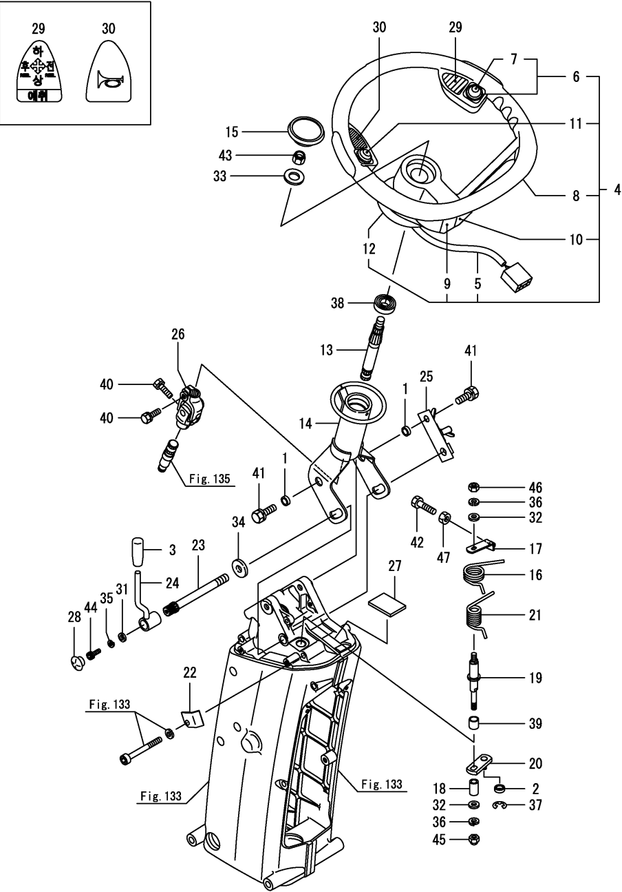
Fig.138. 스티어링
