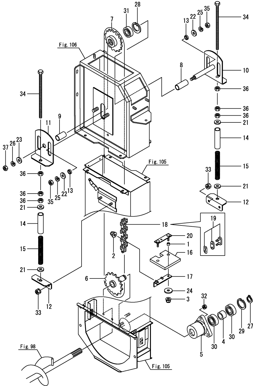
Fig.104. 수직 컨베이어(2차)
