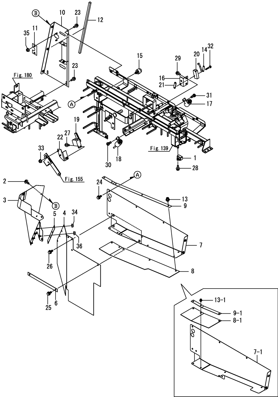
Fig.140. 사이드칼럼(2)
