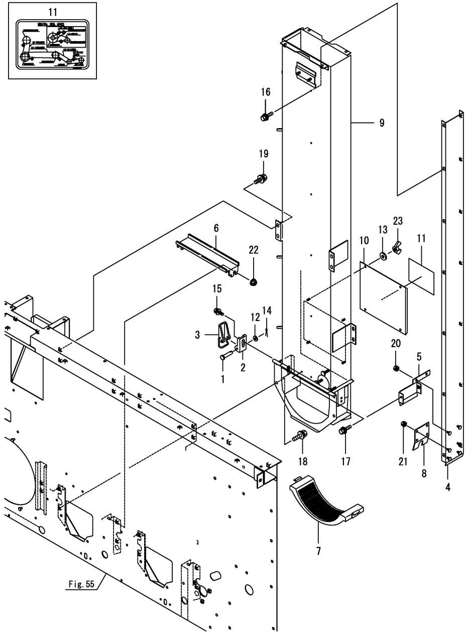
Fig.101. 컨베이어(1번)(센터)
