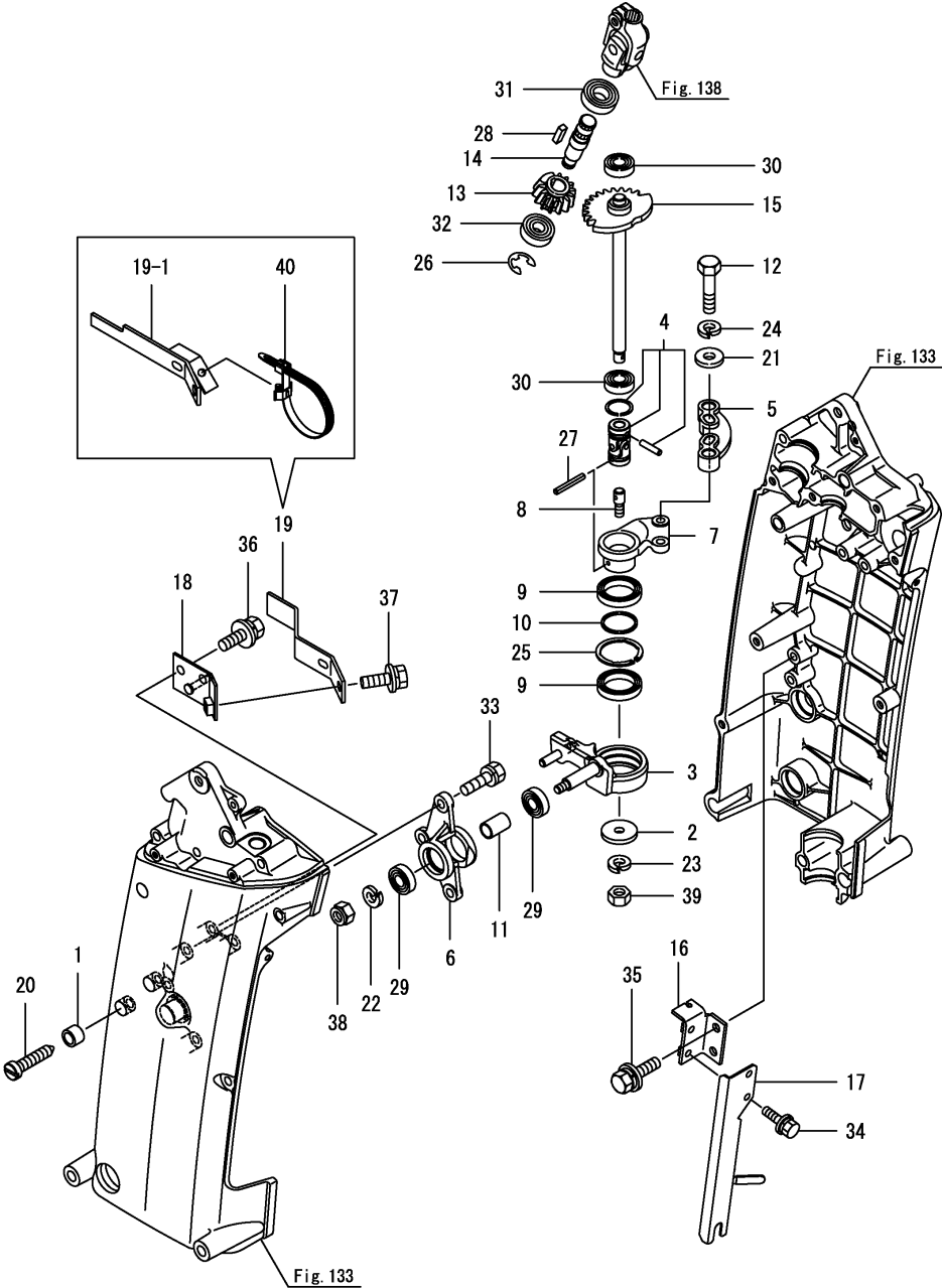
Fig.135. 스티어링 조작(1)
