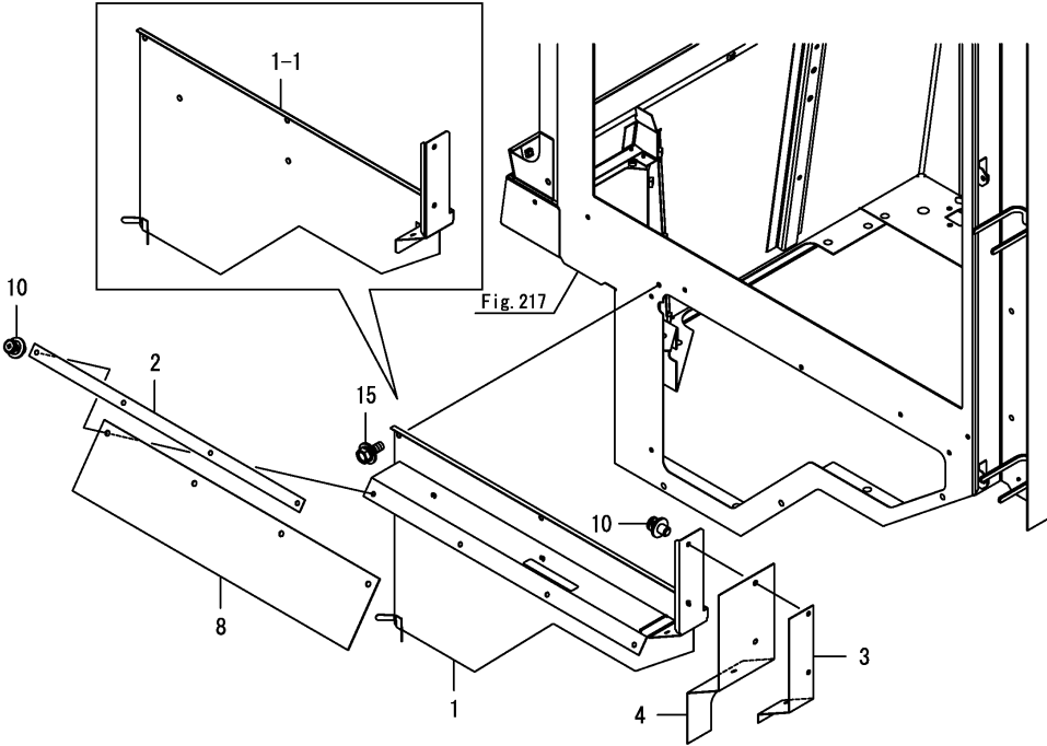
Fig.231. 캐빈시일(2)
