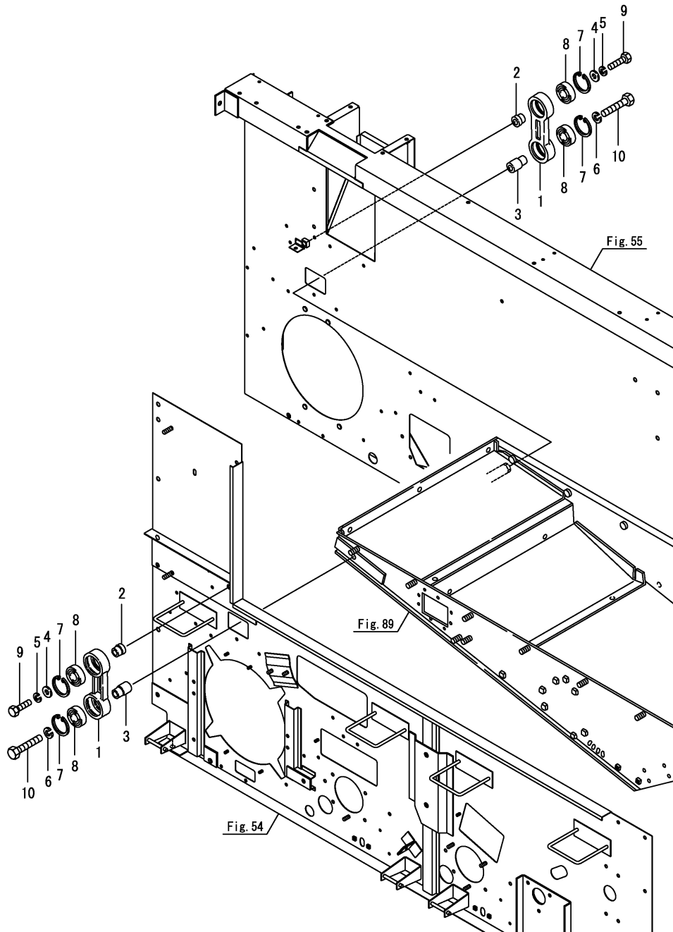
Fig.87. 스윙 암(전면)
