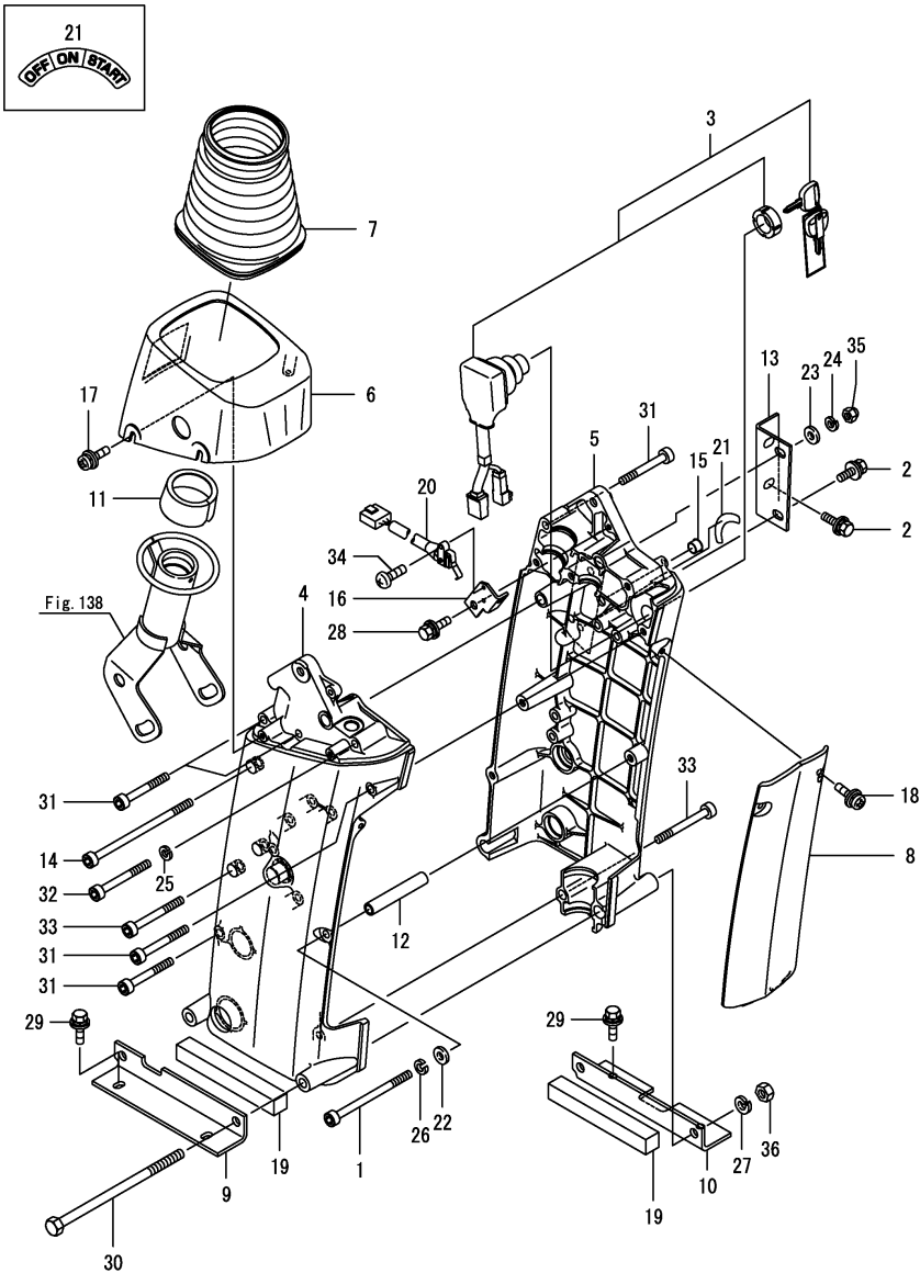
Fig.134. 스티어링칼럼(캐빈)
