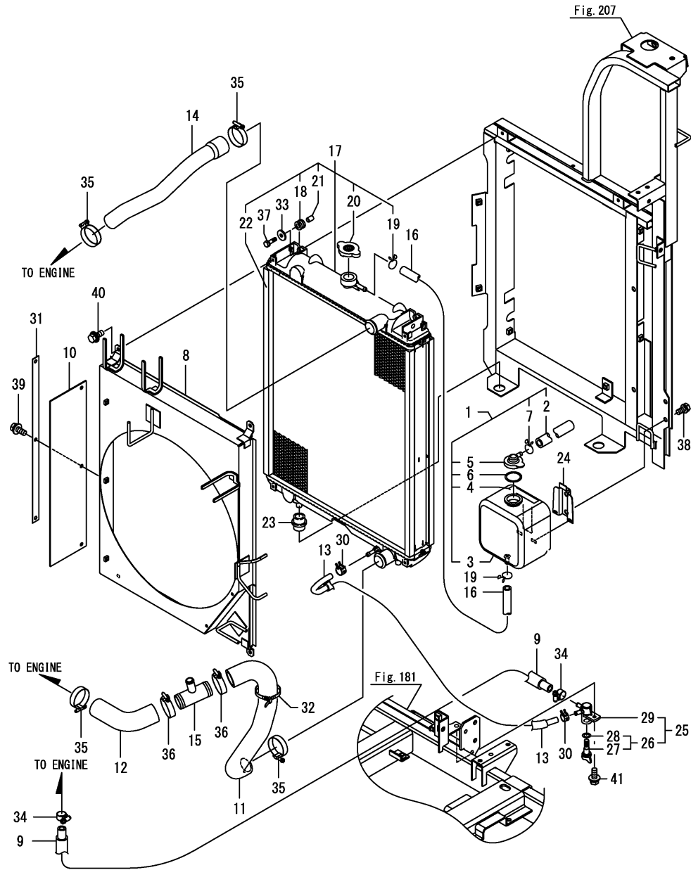
Fig.11. 라디에이터(캐빈)
