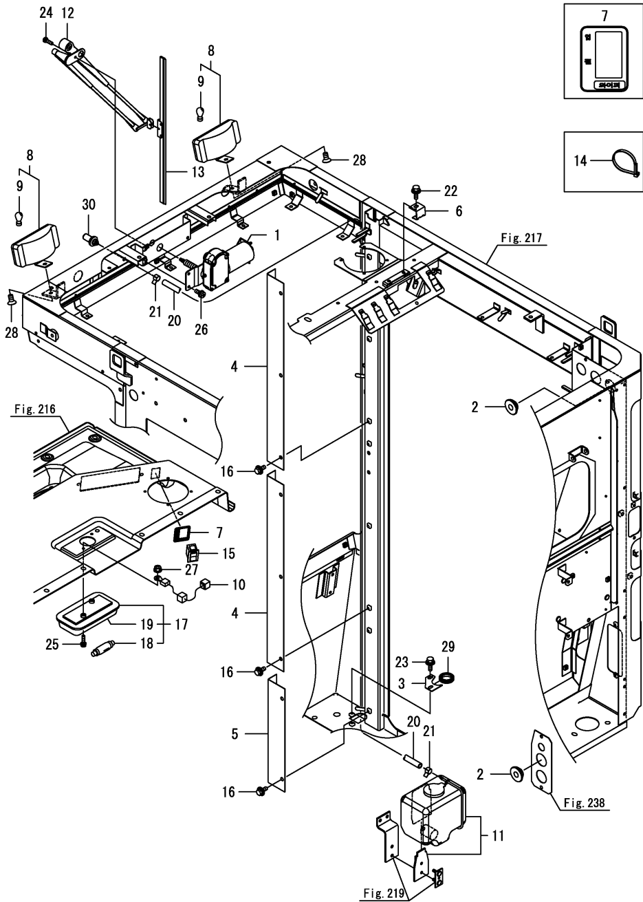
Fig.225. 전장품(캐빈)(1)
