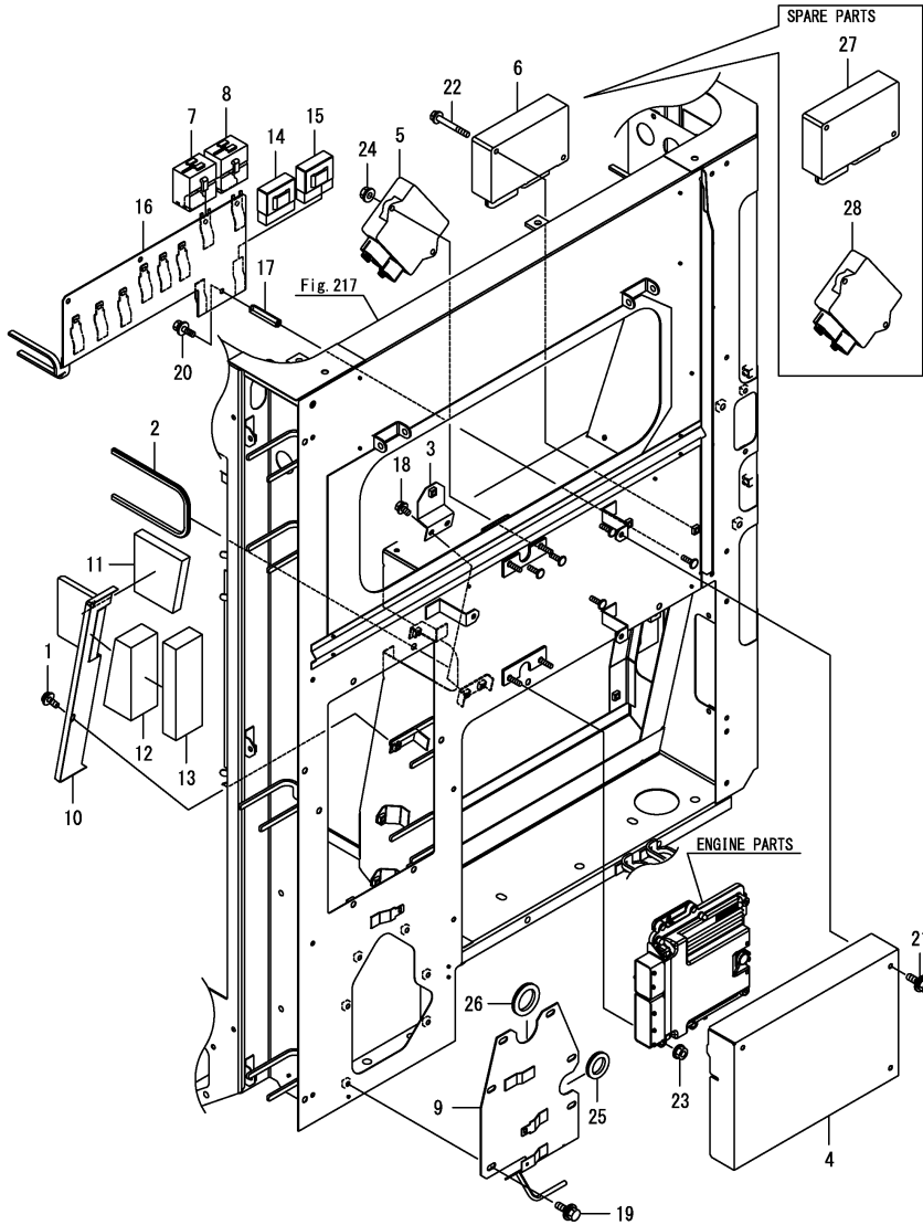
Fig.226. 전장품(캐빈)(2)
