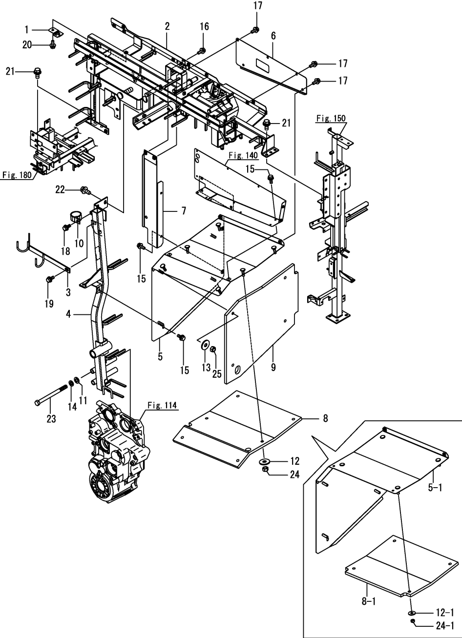
Fig.139. 사이드칼럼(1)
