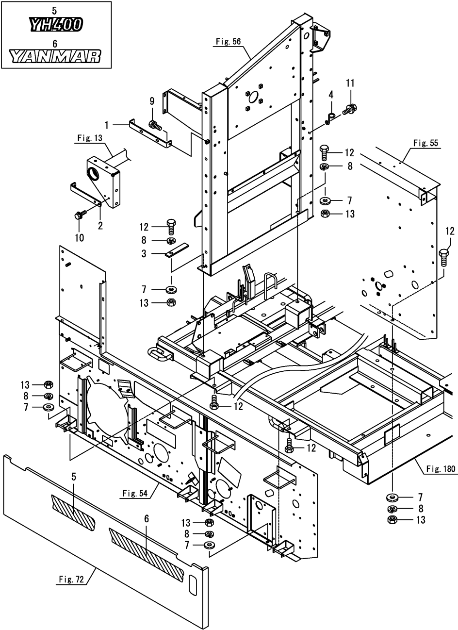
Fig.53. 하부본체취부
