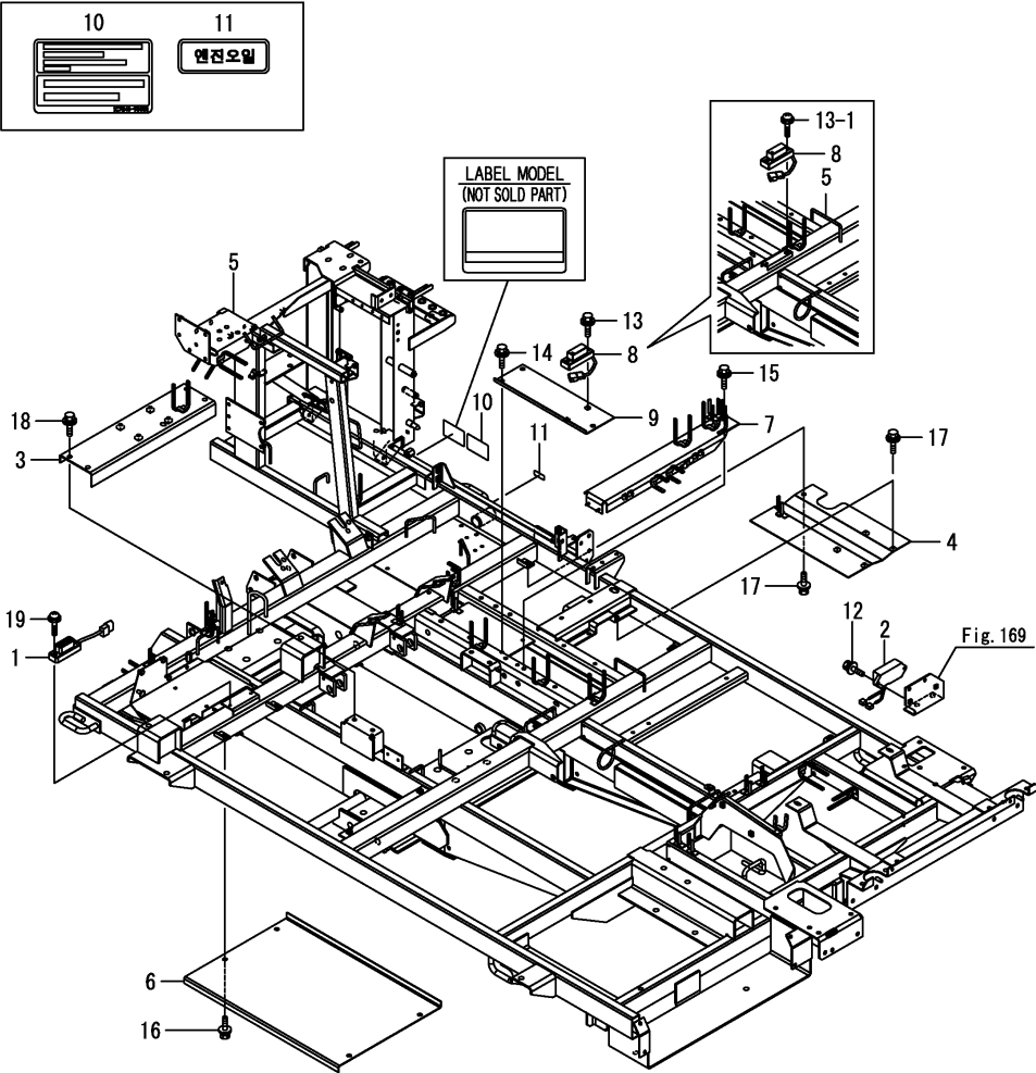
Fig.181. 새시프레임(캐빈)
