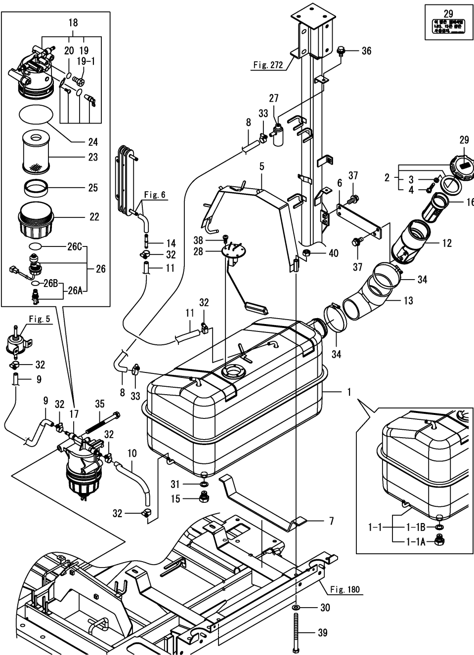
Fig.3. 연료탱크
