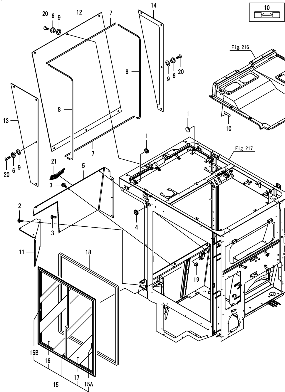
Fig.223. 캐빈의장(1)
