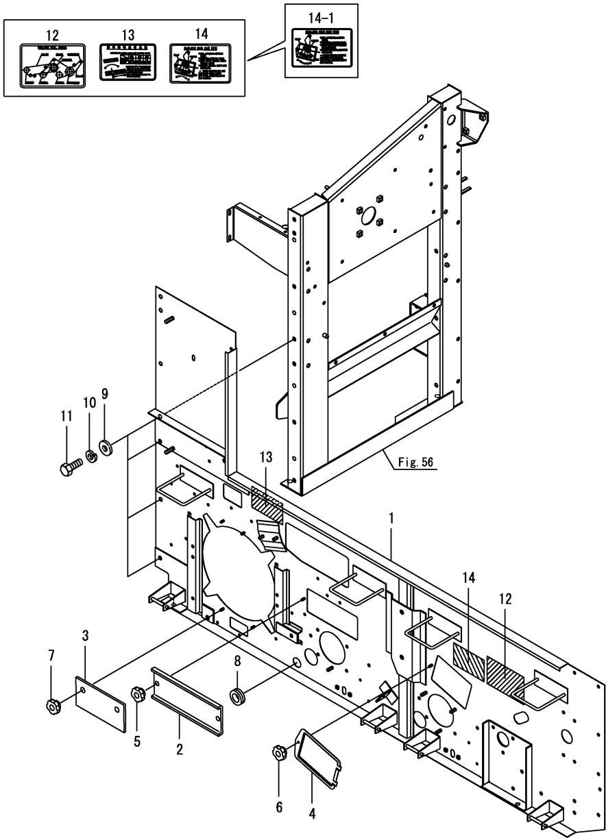
Fig.54. 하부본체(좌)
