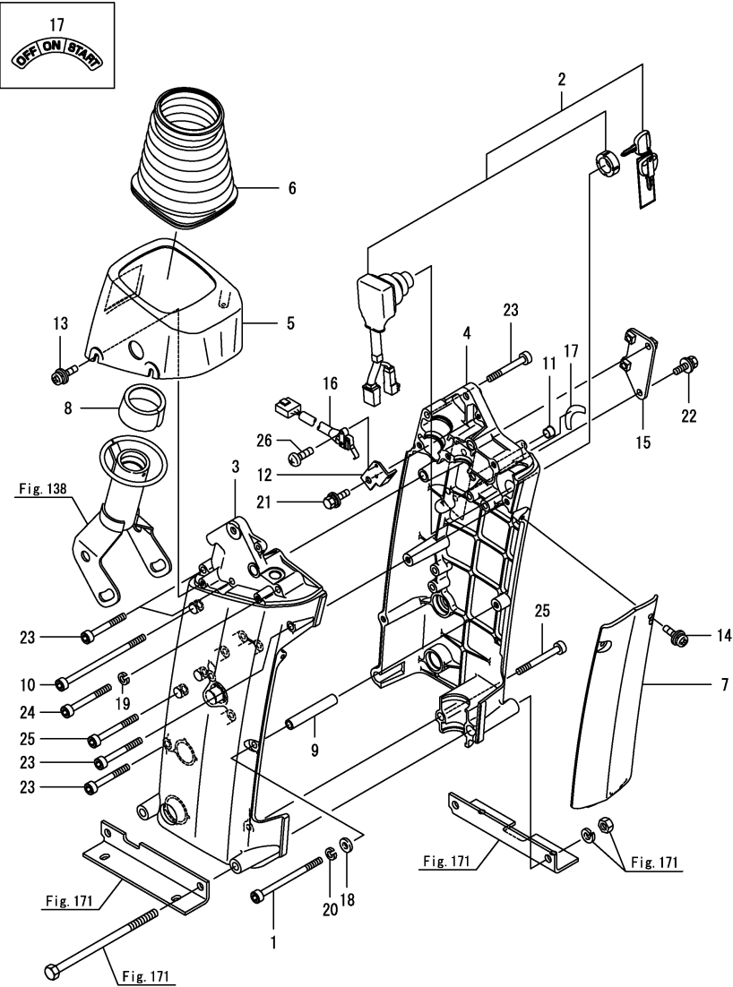
Fig.133. 스티어링칼럼
