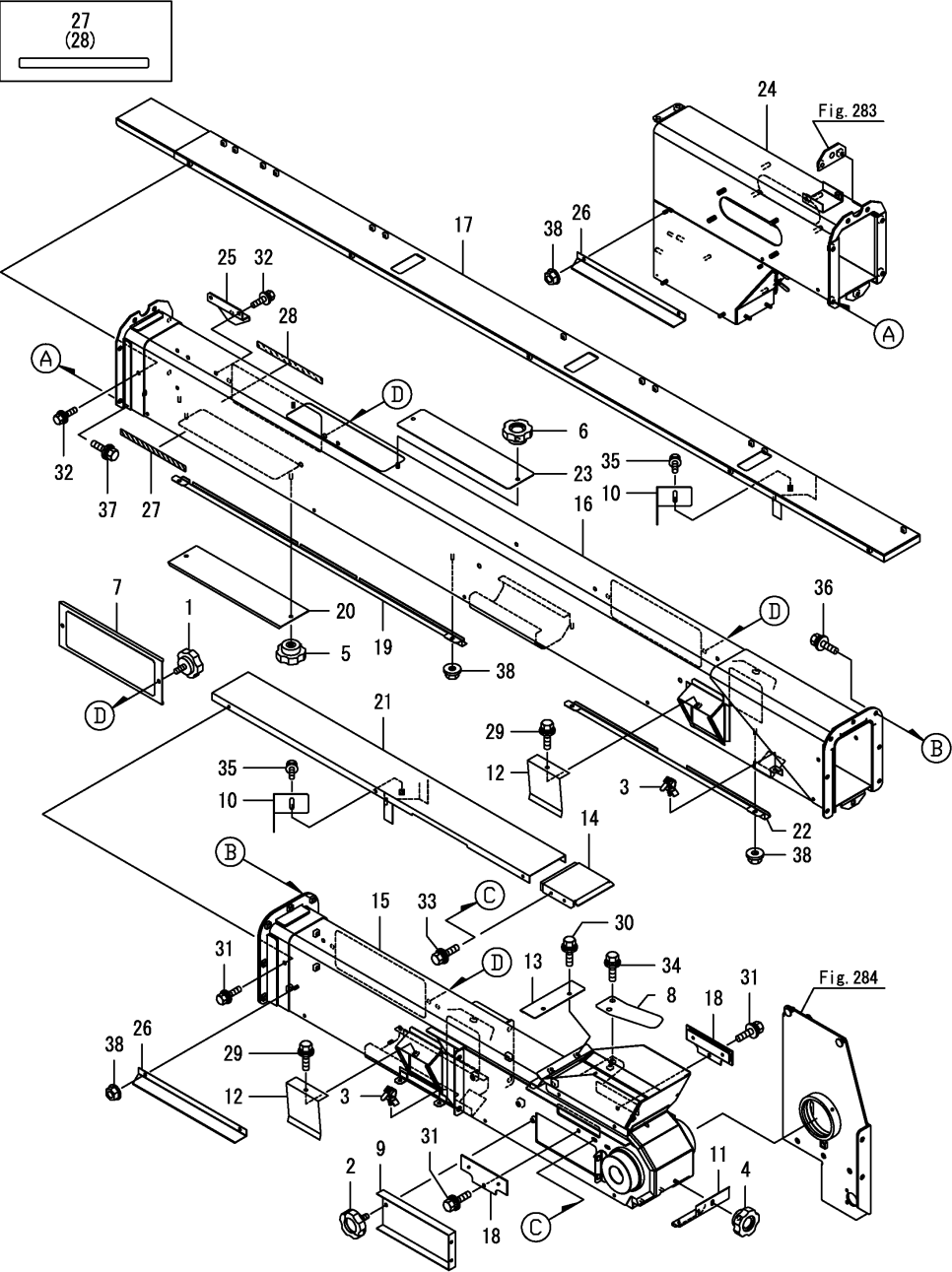
Fig.285. 컨베이어케이스
