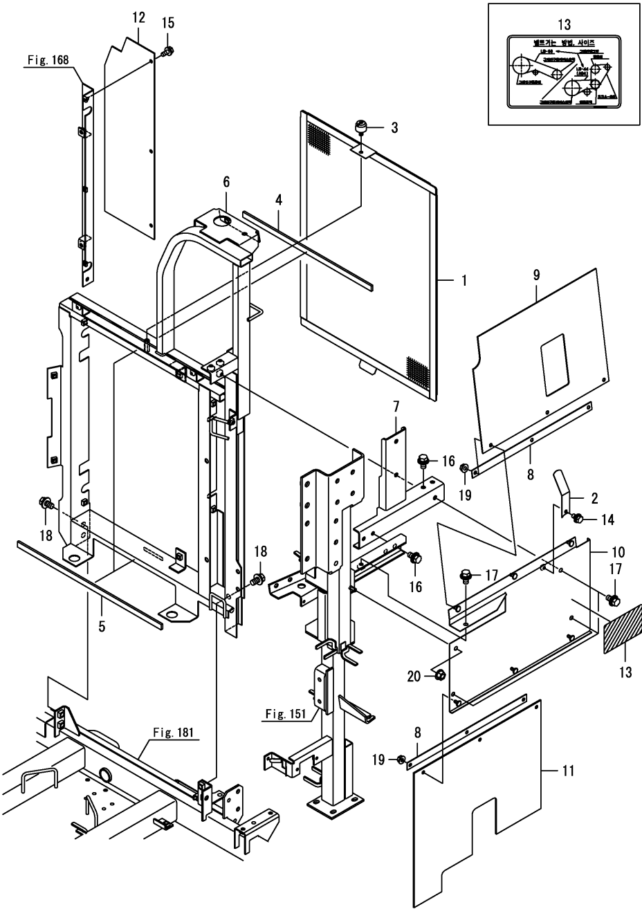
Fig.207. 엔진실프레임(캐빈)
