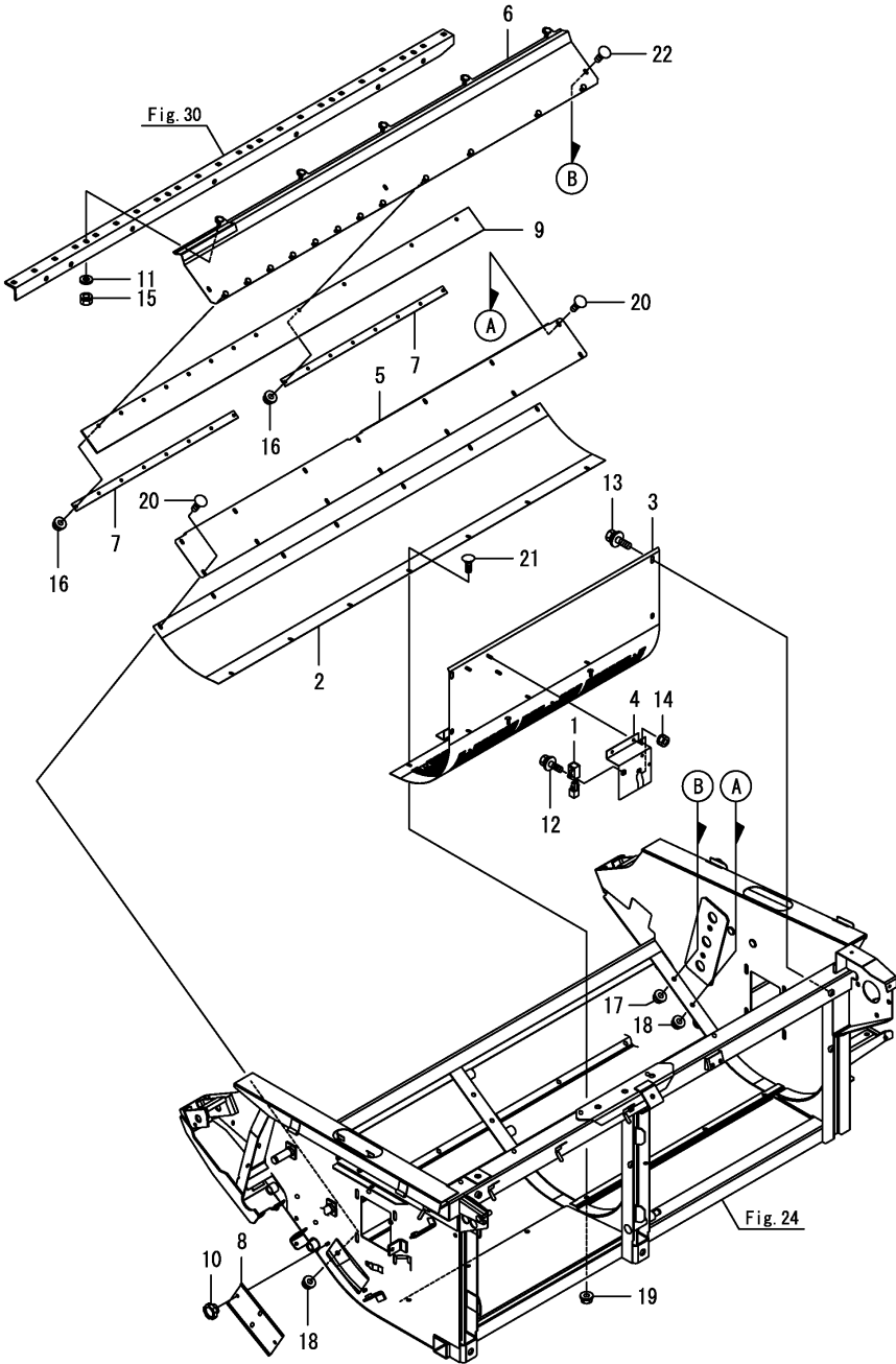
Fig.25. 바닥판
