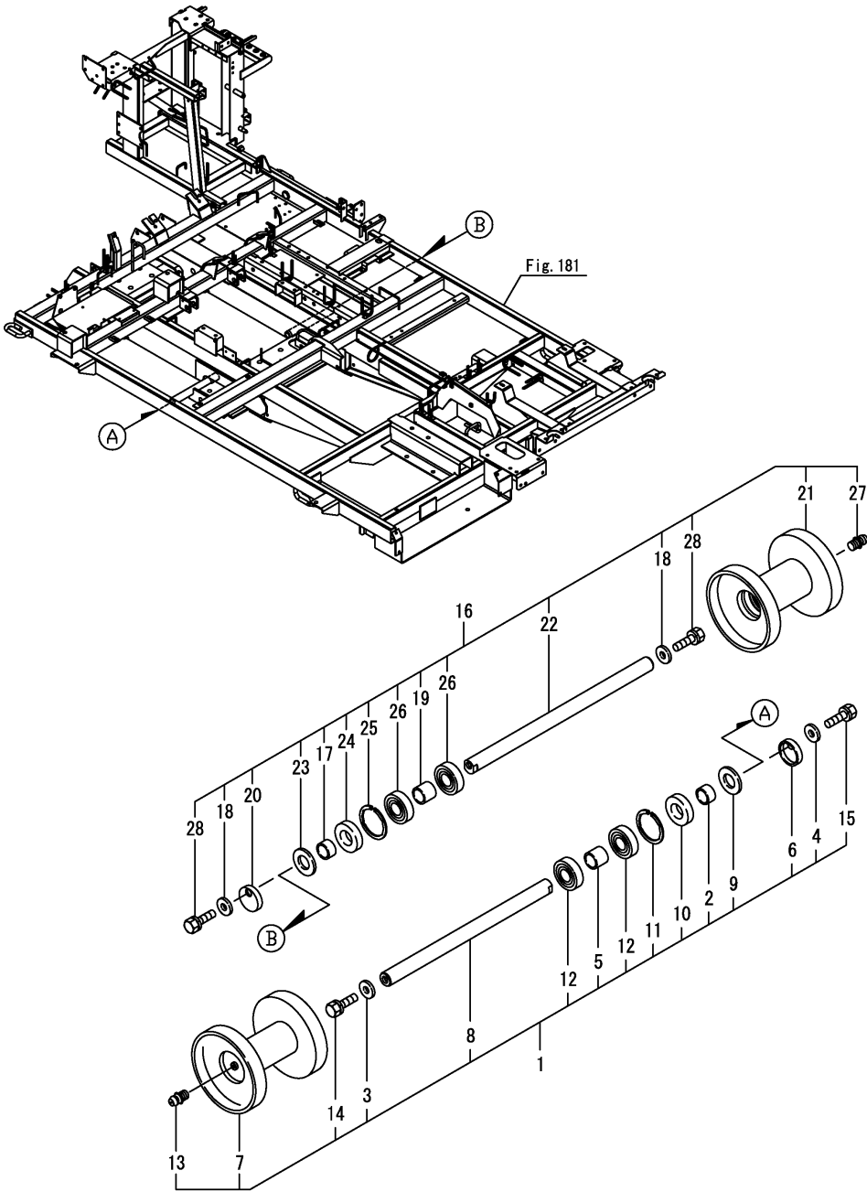
Fig.194. 캐리어롤러(개빈)
