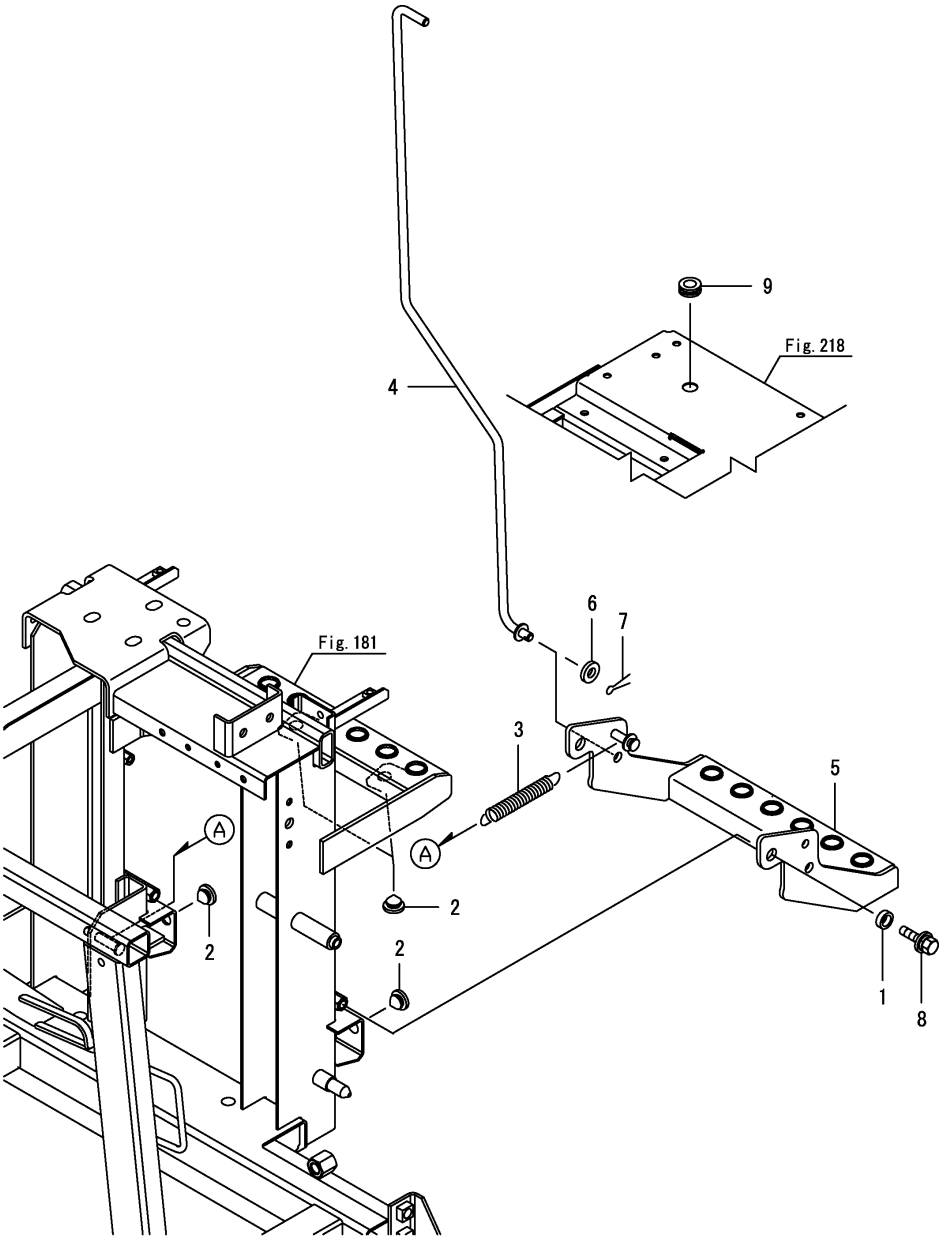
Fig.176. 보조단(캐빈)
