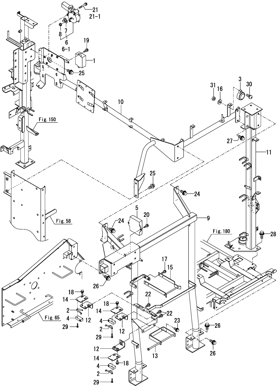
Fig.272. 지주프레임
