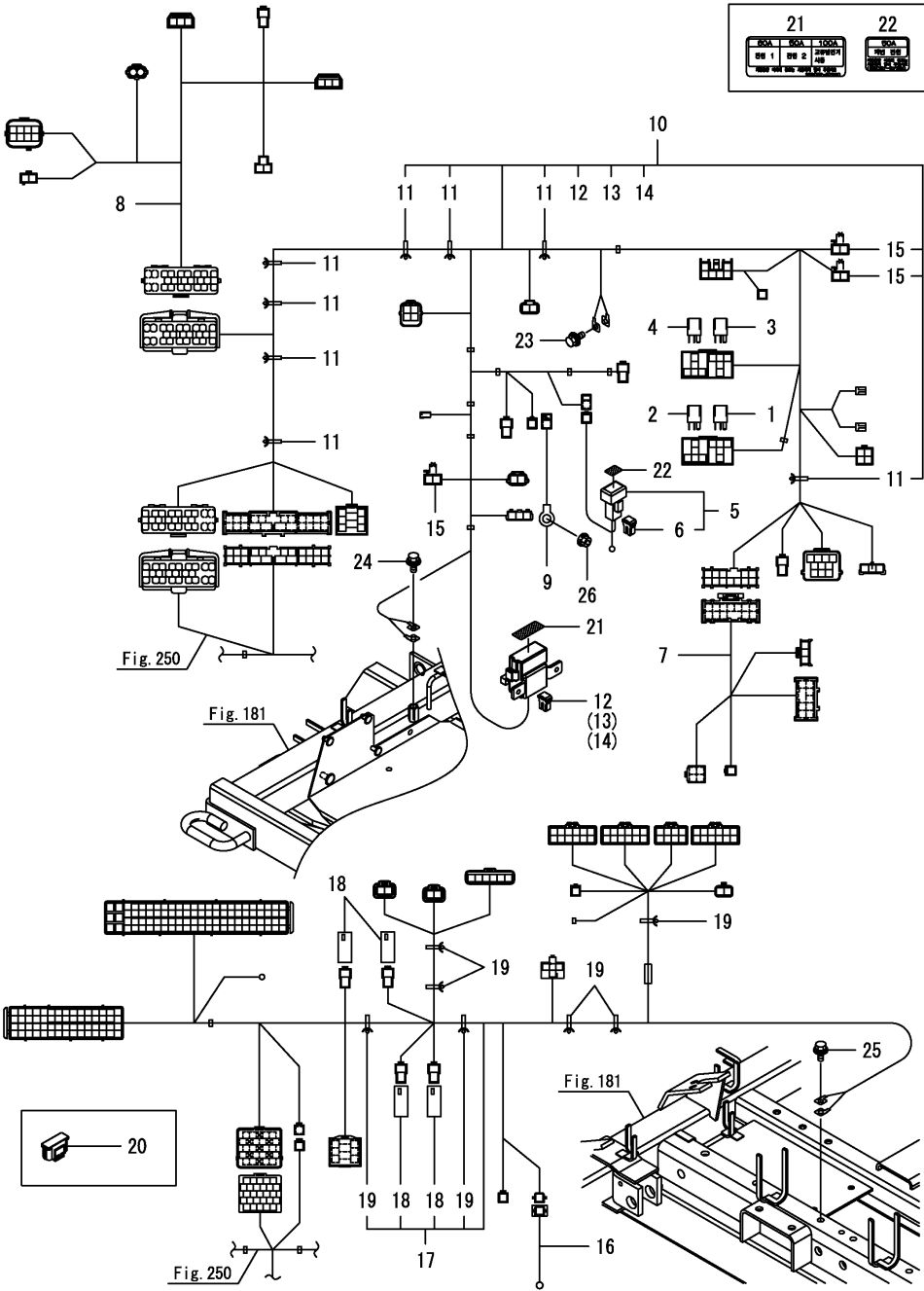
Fig.251. 배선 하네스(2)(캐빈)
