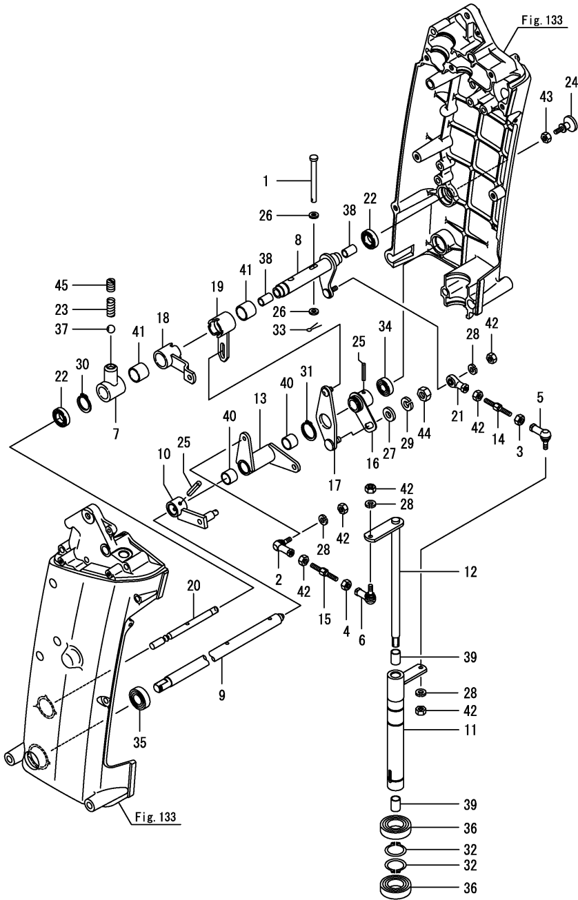
Fig.137. 스티어링 조작(3)
