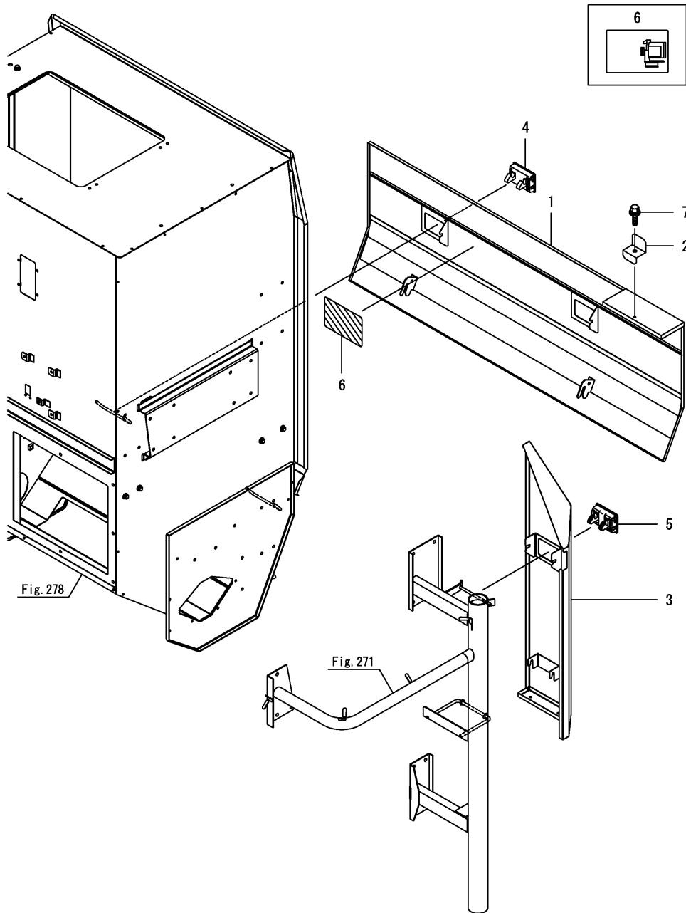
Fig.281. 탱크커버
