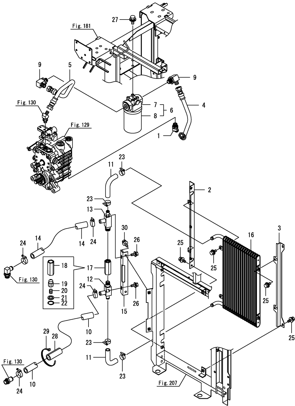
Fig.168. 배관(H.S.T.)(캐빈)
