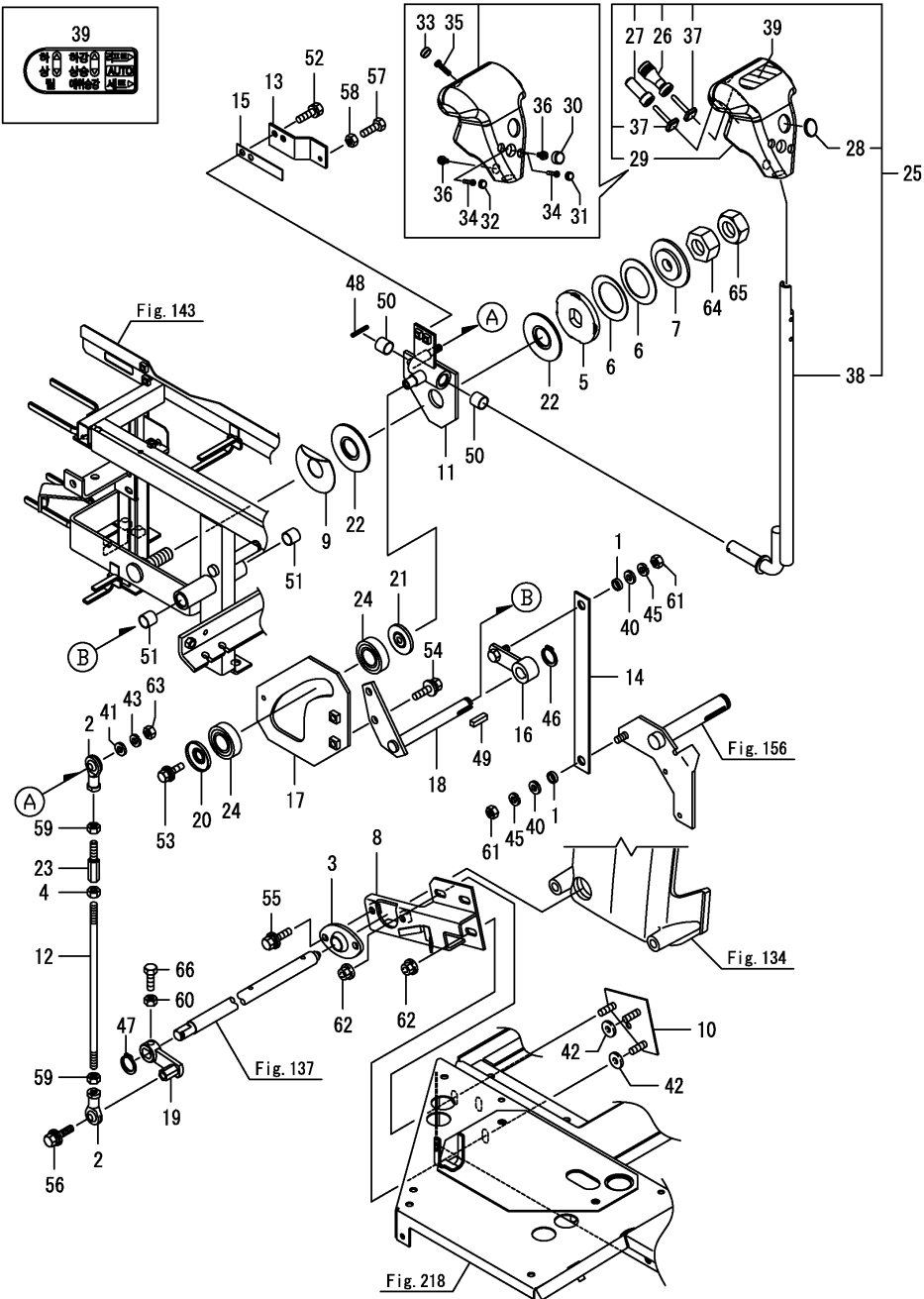
Fig.158. 주변속조작(개빈)
