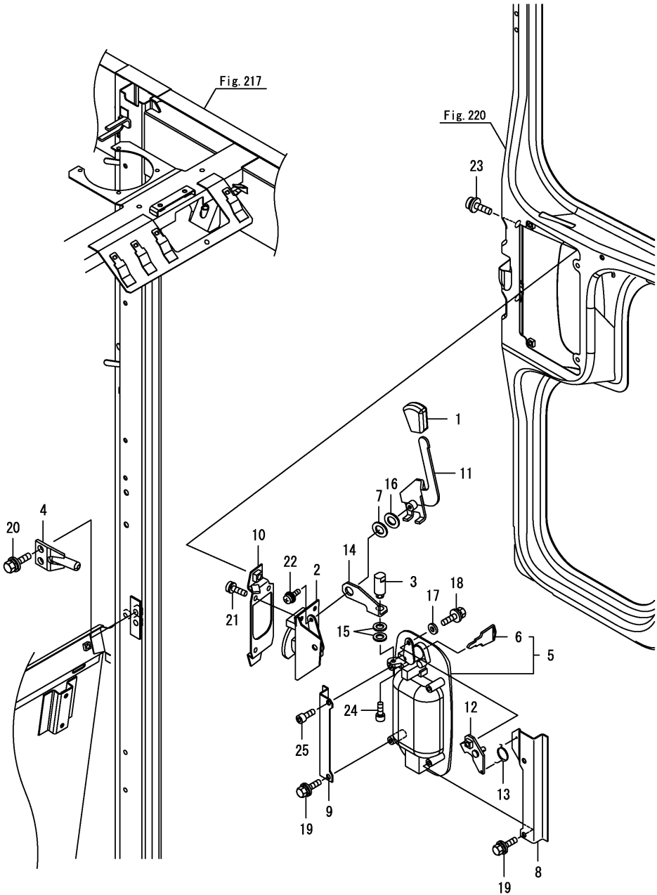
Fig.221. 캐빈 도어(2)
