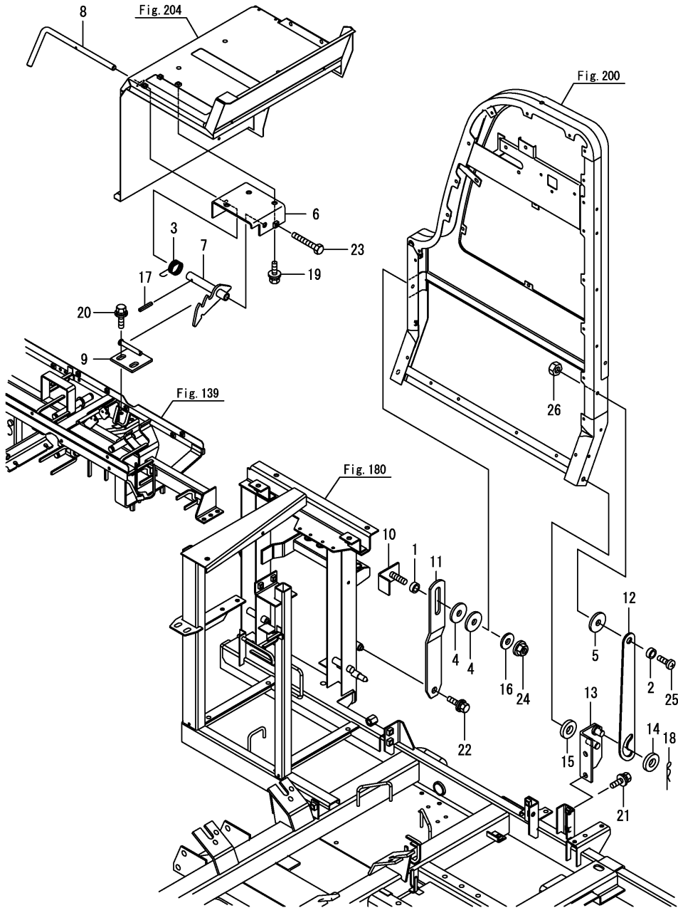
Fig.205. 엔진실커버필크럼
