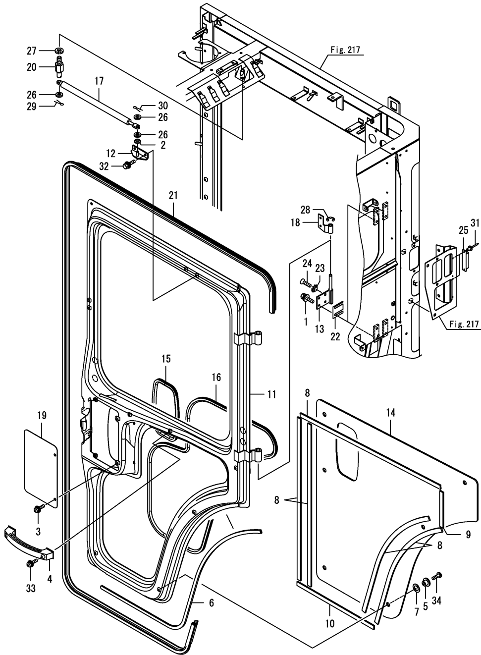
Fig.220. 캐빈 도어(1)
