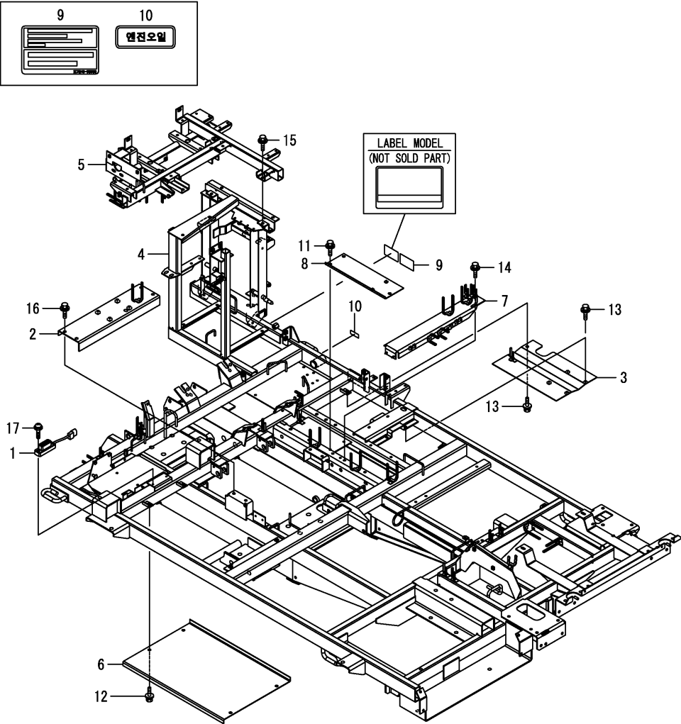
Fig.180. 새시프레임
