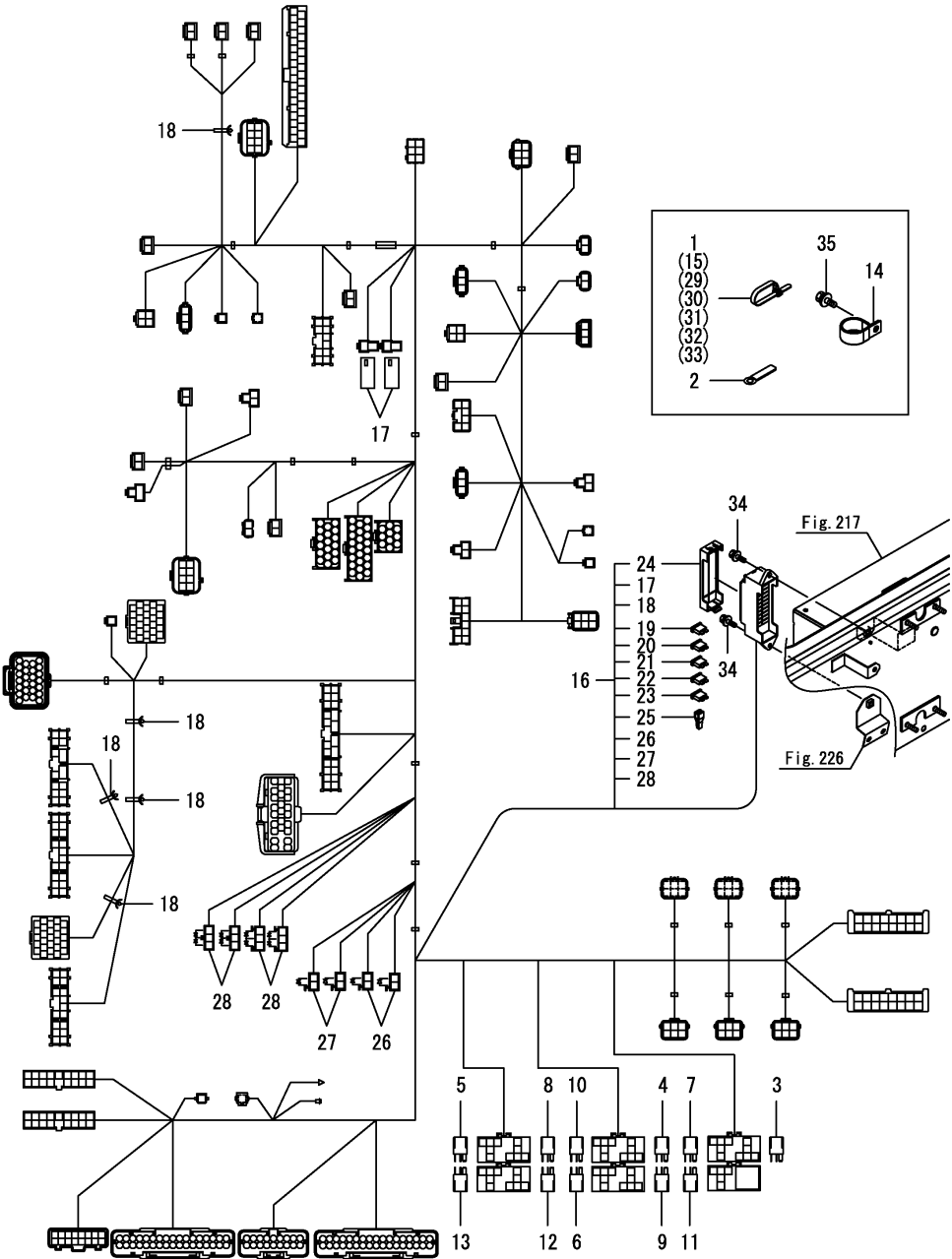
Fig.250. 배선 하네스(1)(캐빈)
