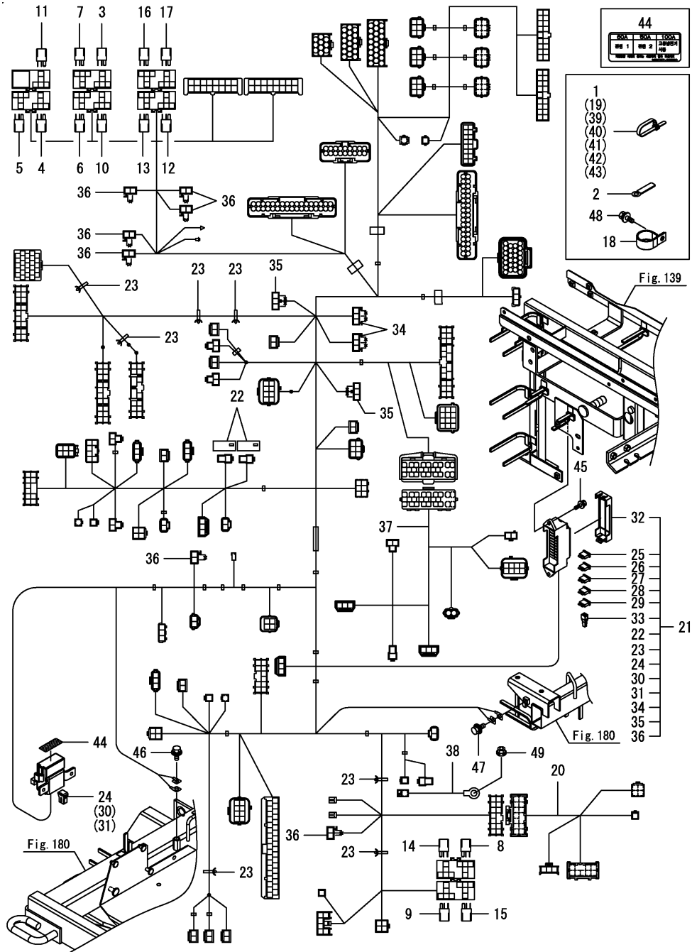
Fig.247. 배선 하네스(1)
