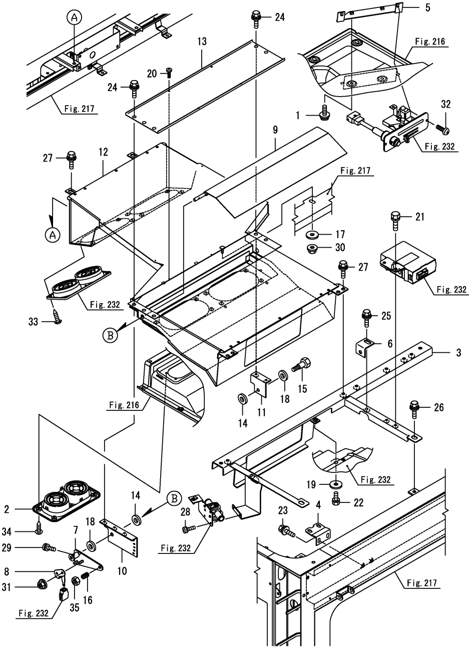
Fig.234. 에어컨취부(1)
