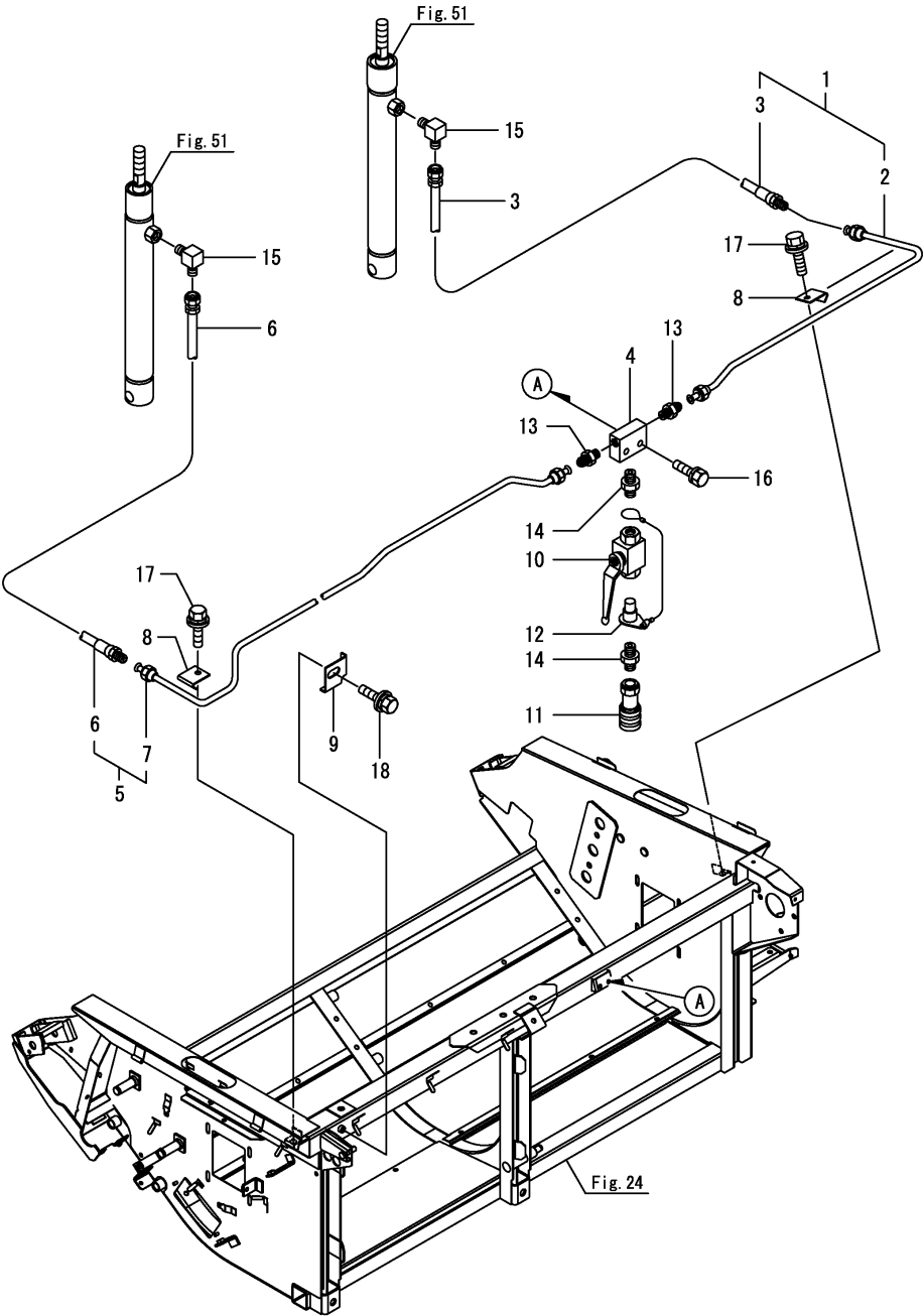
Fig.52. 배관(플랫폼)
