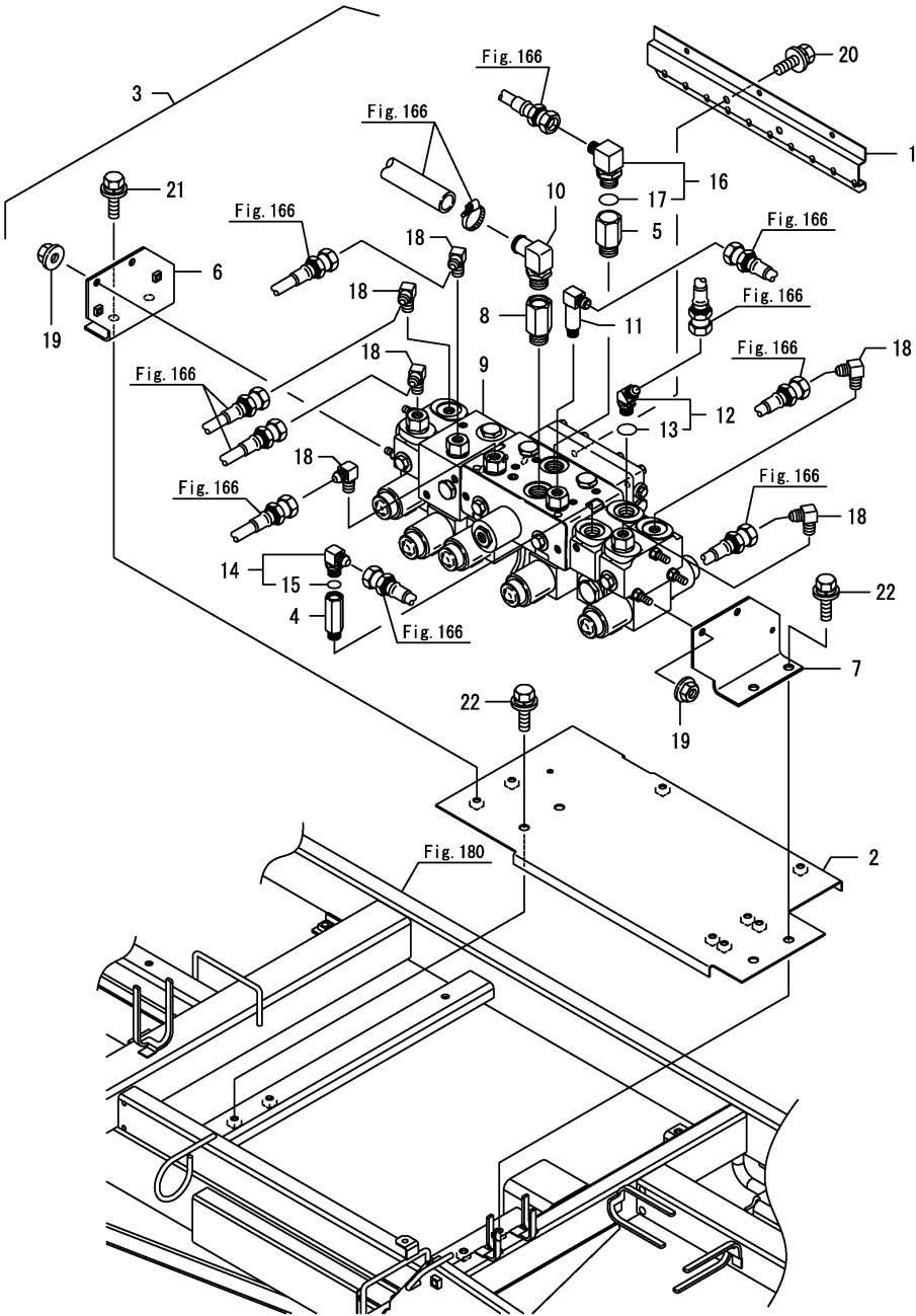
Fig.169. 밸브
