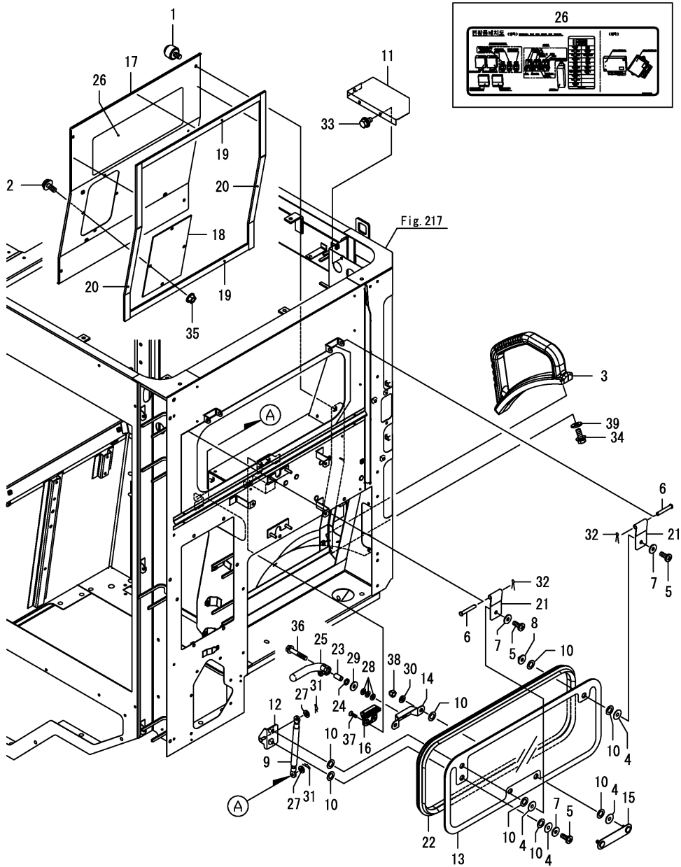
Fig.224. 캐빈의장(2)
