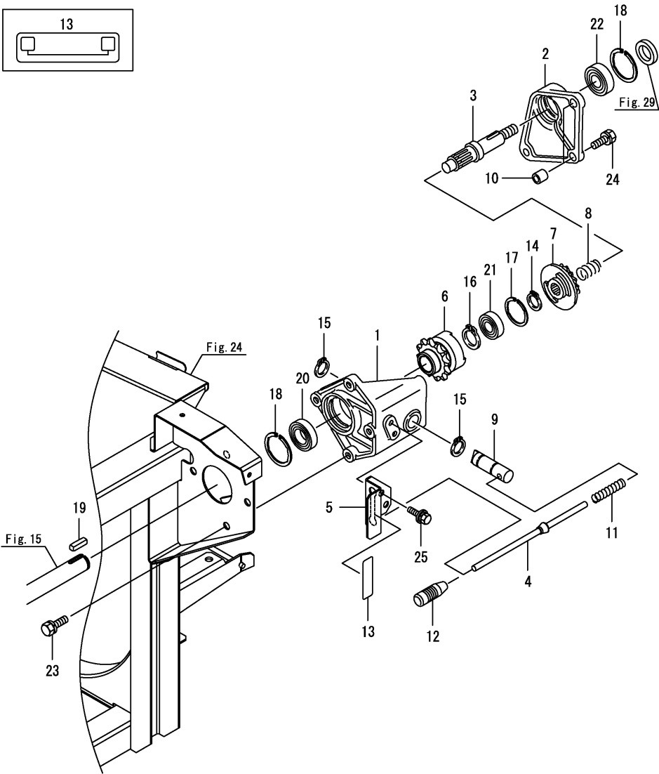
Fig.27. 예취날클러치
