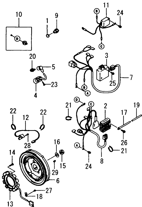
FIG. 6 ELECTRIC-EQUIPMENT
