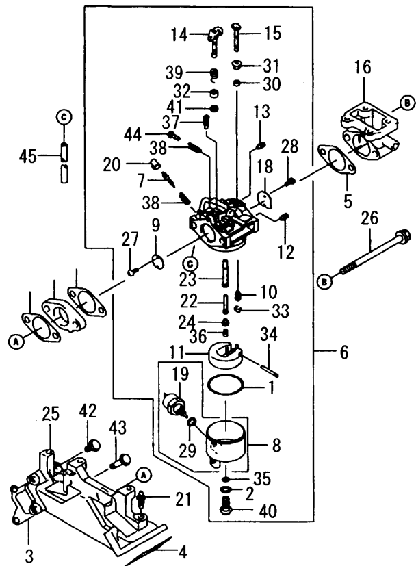
FIG. 8 CARBURETOR
