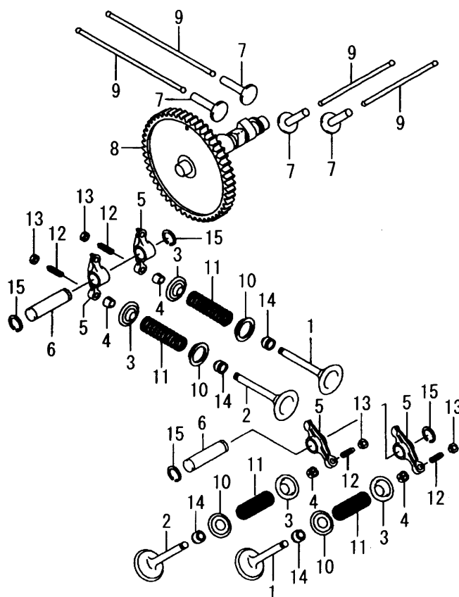
FIG. 3 VALVE/CAMSHAFT
