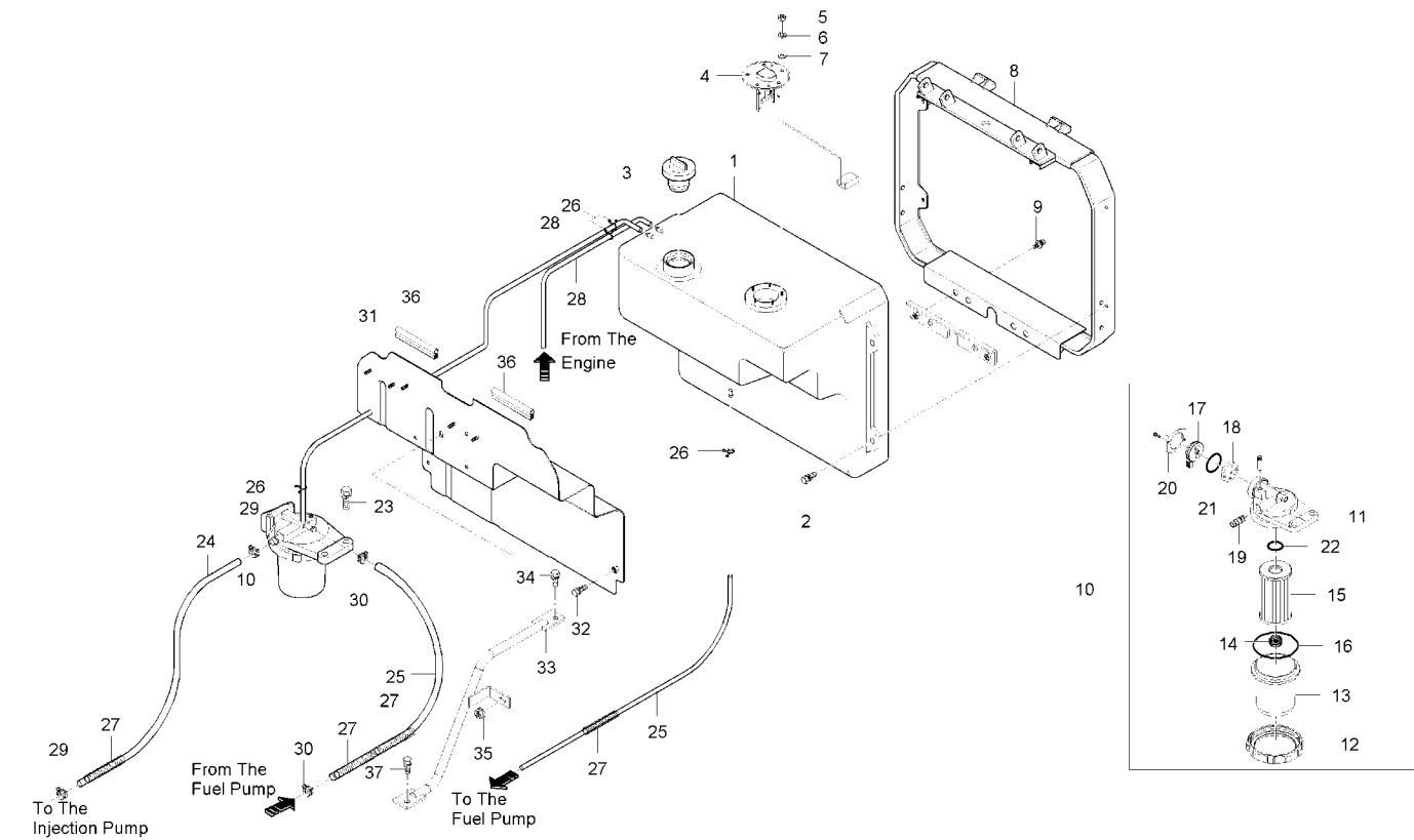
A : CK30
