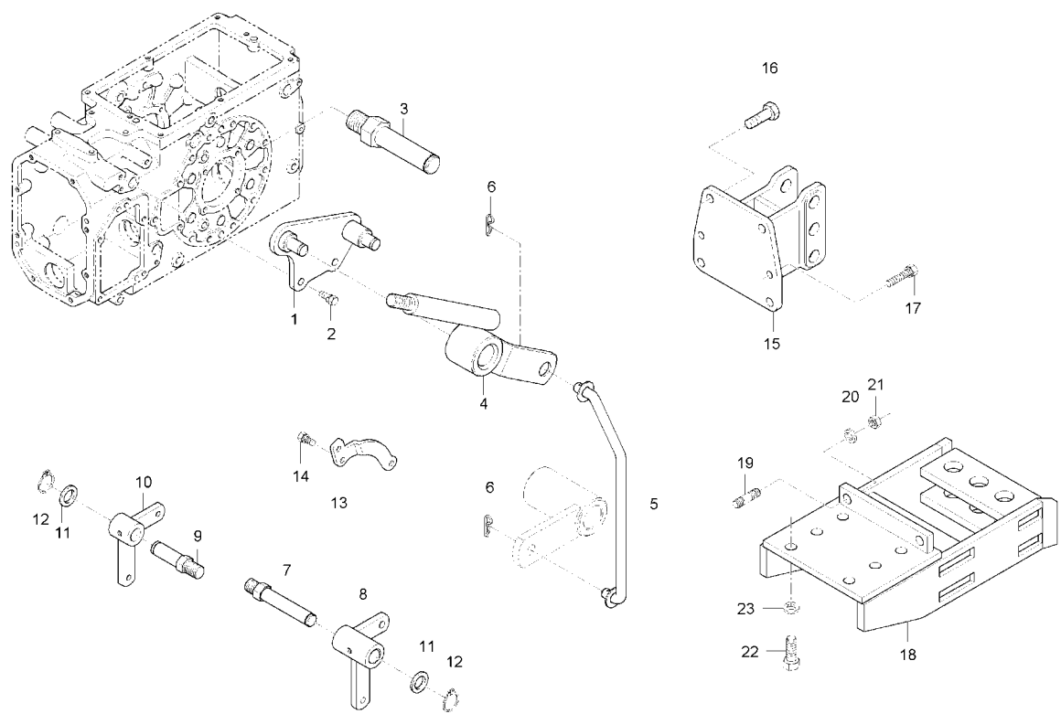
A : CK30
