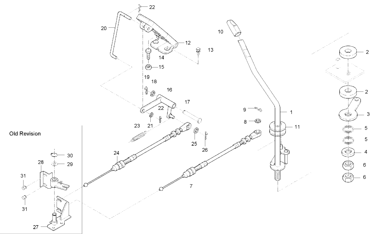
A : CK30
