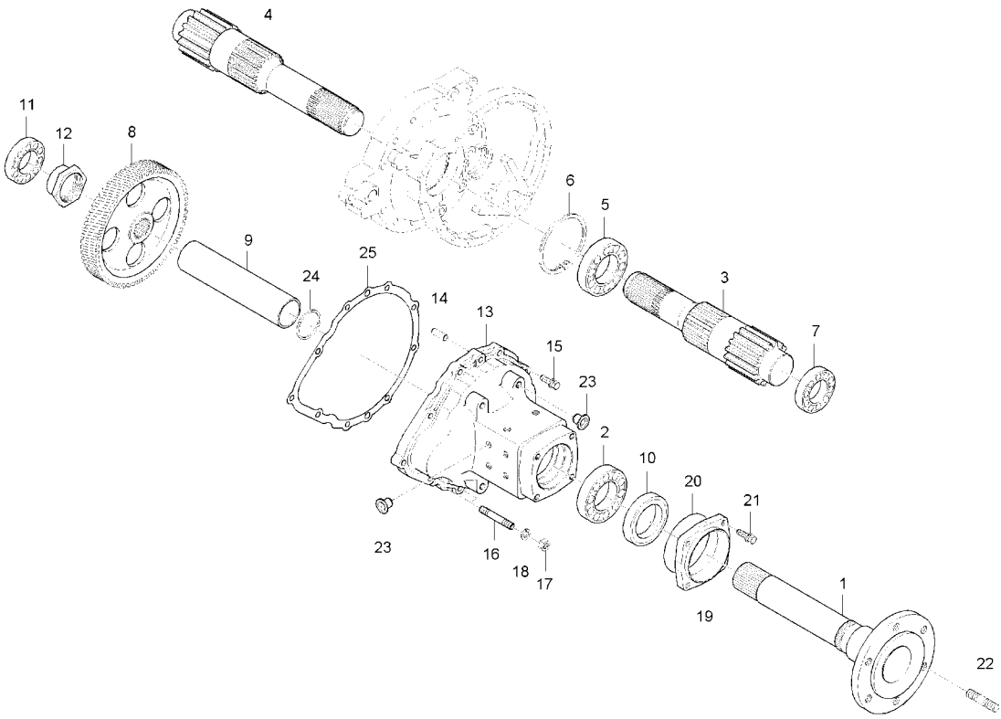
A : CK30
