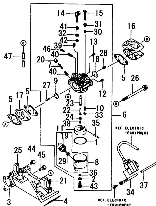
FIG. 8 CARBURETOR
