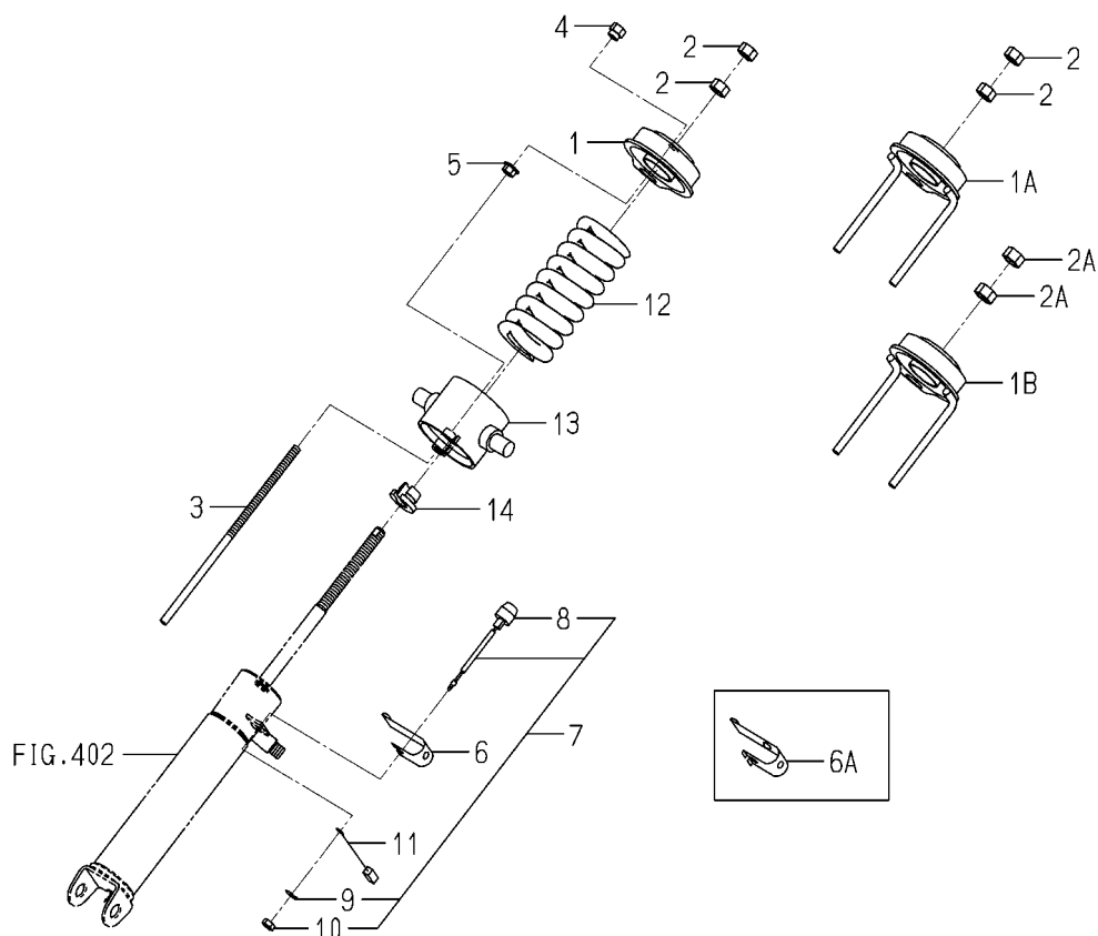
FIG.404 CASE(SPRING)SYSTEM
