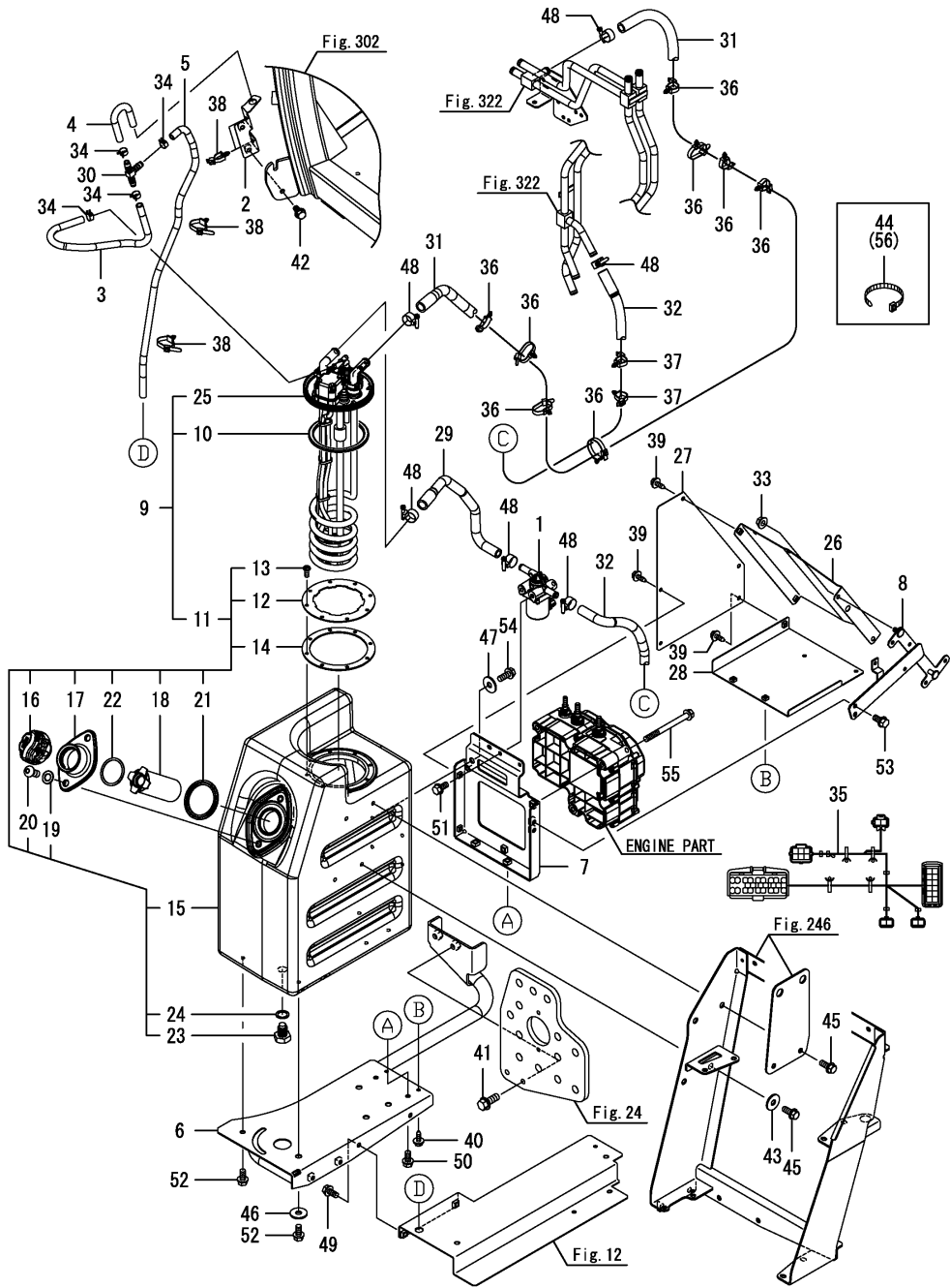
Fig.17. 요소수 탱크
