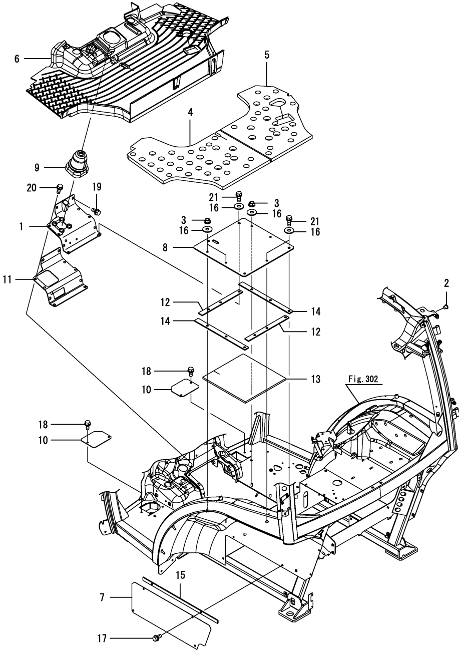
Fig.245. 캐빈(엑세서리)
