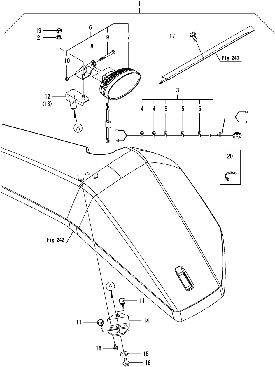
Fig.338. 작업등(펜더)
