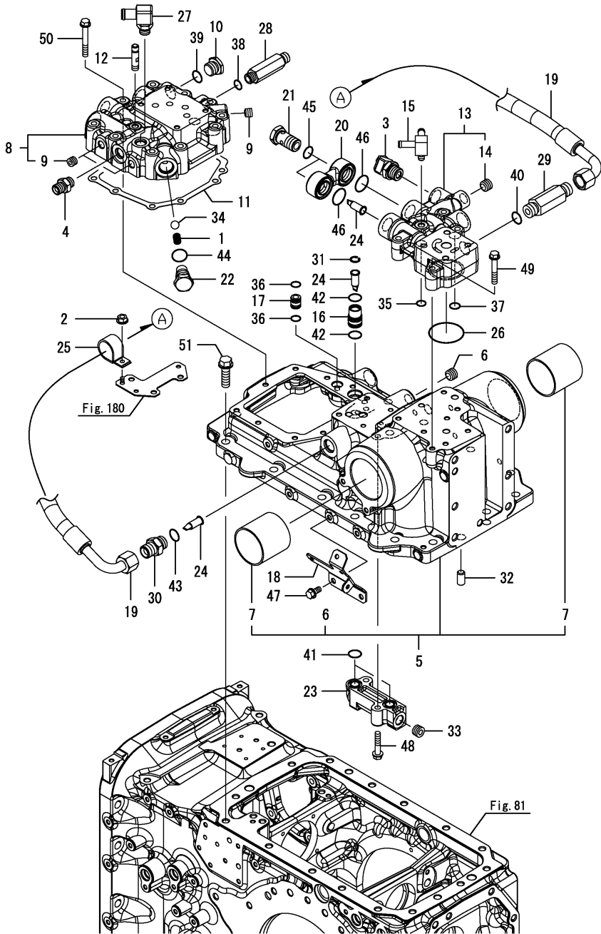
Fig.176. 유압리프트케이스
