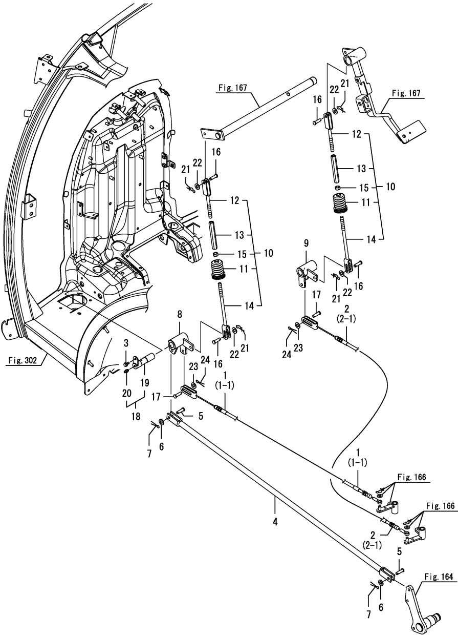
Fig.169. 브레이크링크
