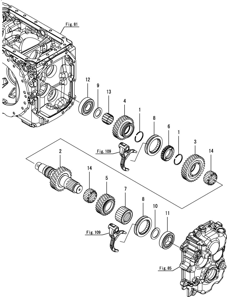
OCNP6-M06810 미션부 Fig.102. P.T.O. 피구동축
