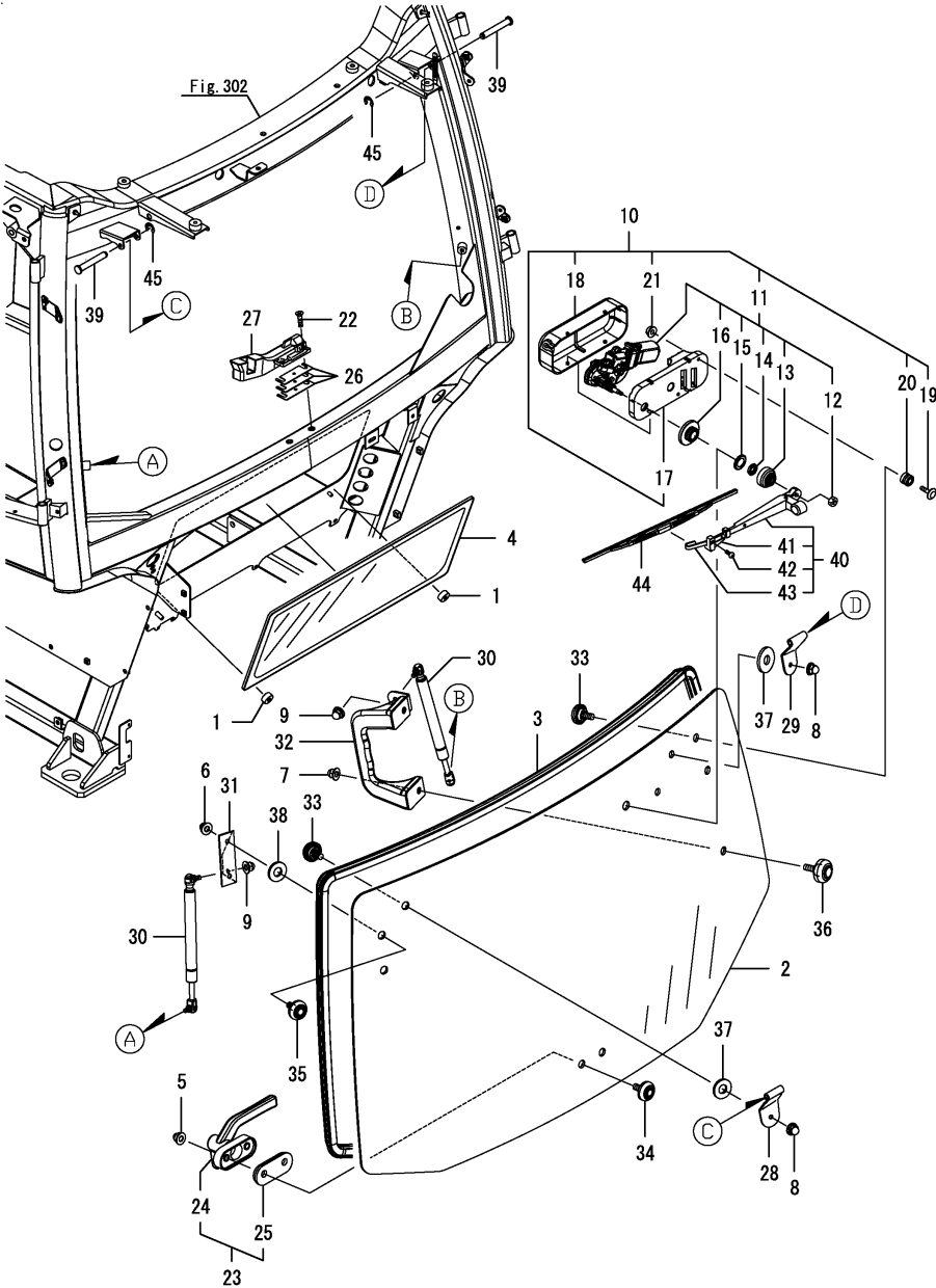
OCNP6-M06810 캐빈부 Fig.308. 후방창문
