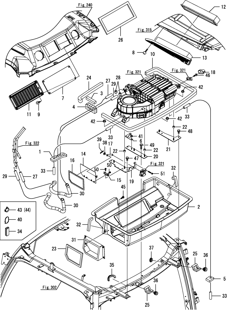
Fig.323. 에어컨(3)
