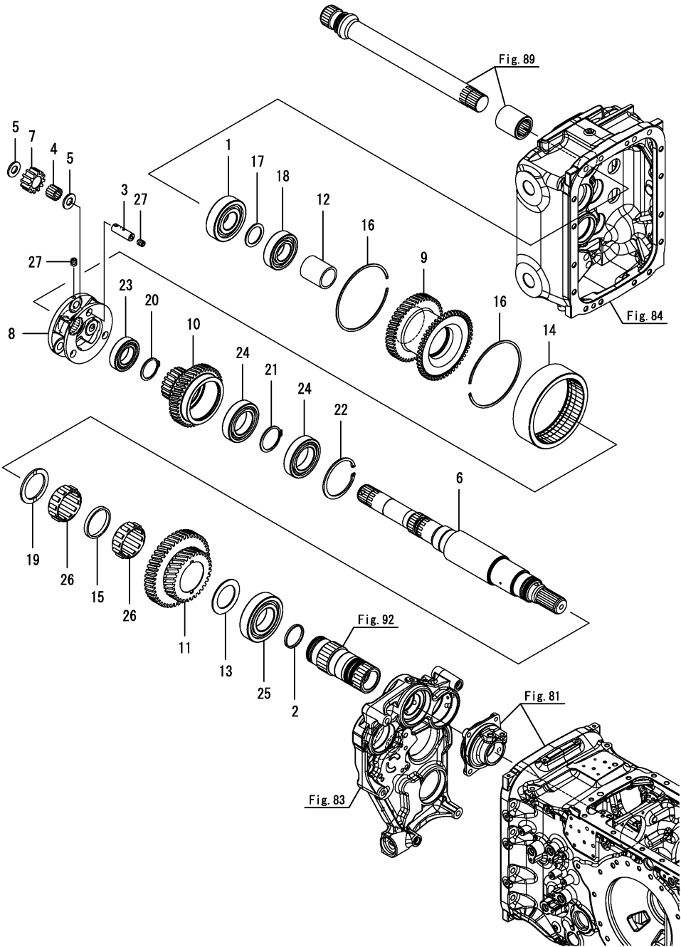
Fig.90. 주축
