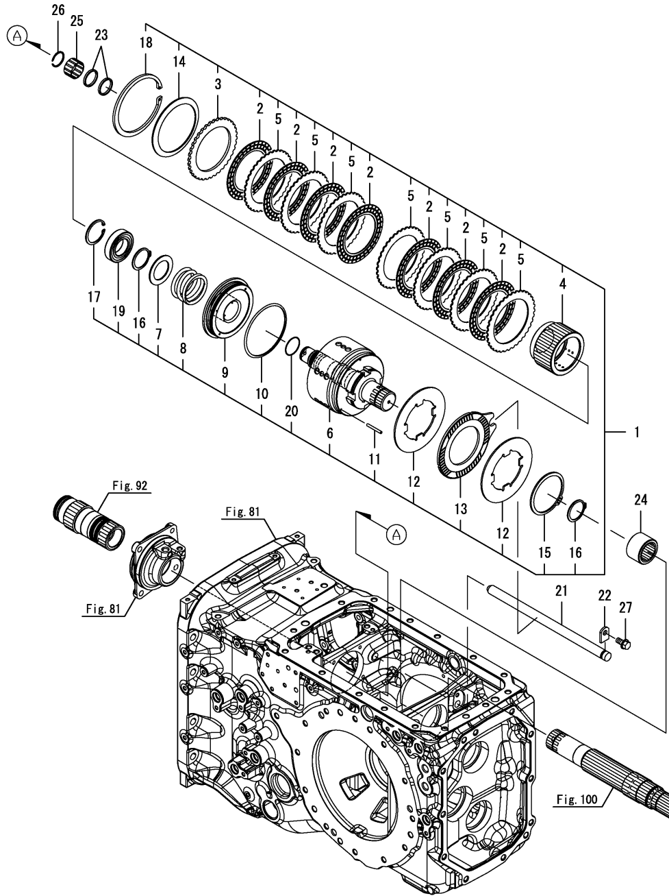
Fig.80. P.T.O. 클러치
