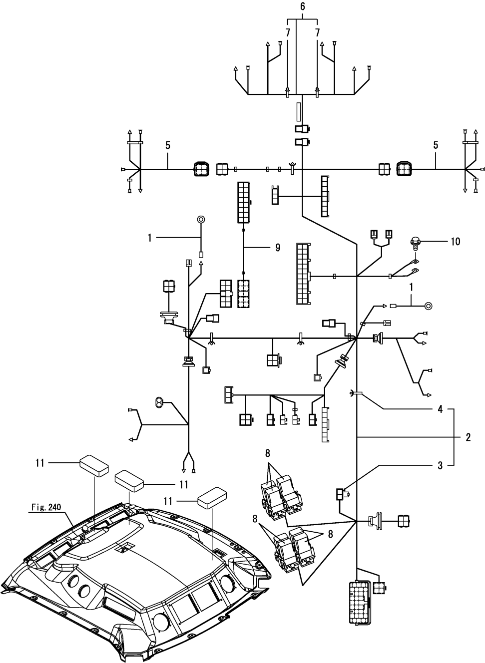
Fig.212. 배선(캐빈)
