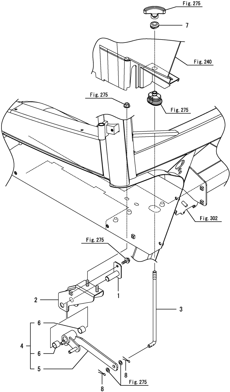
Fig.278. 연동 P.T.O. 레버
