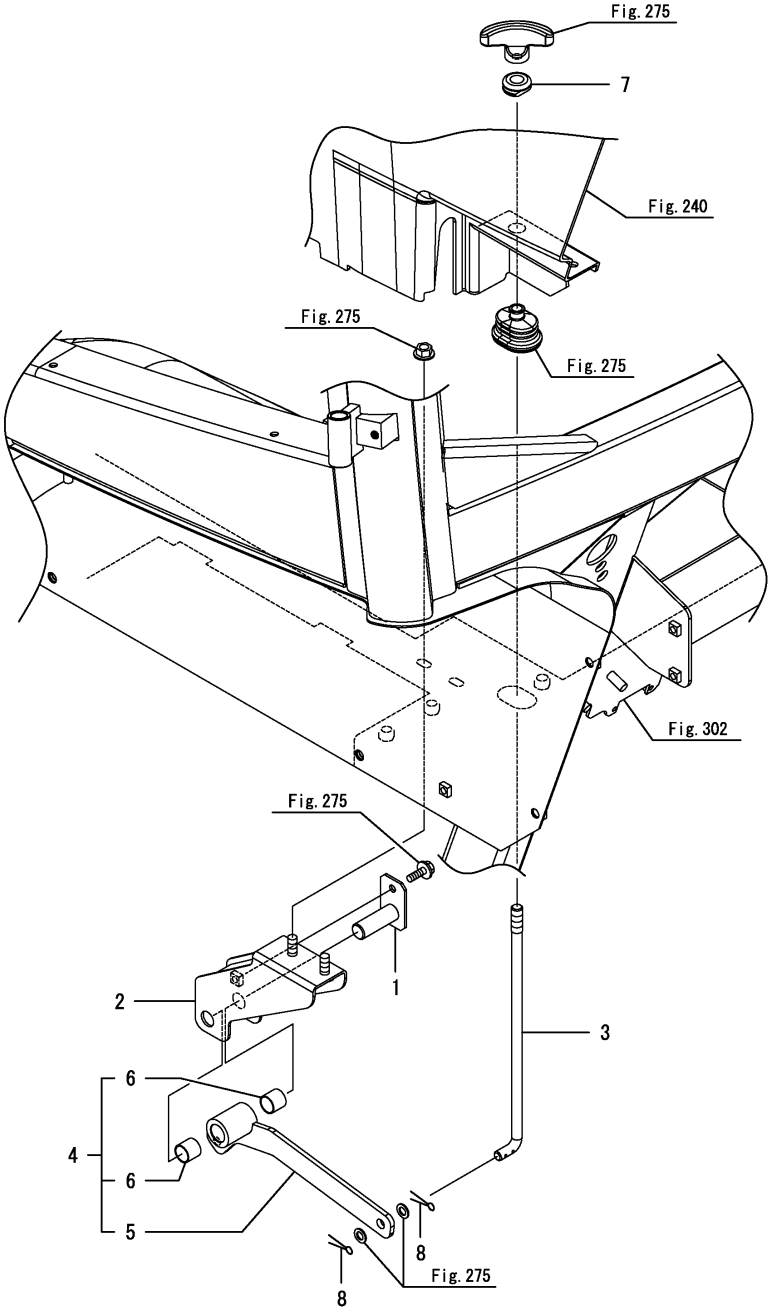
Fig.276. 역전P.T.O. 레버
