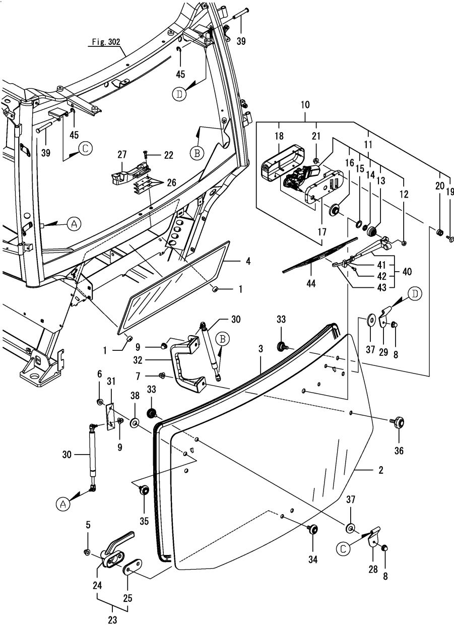
OCNP6-M06810 캐빈부 Fig.309. 후방창문
