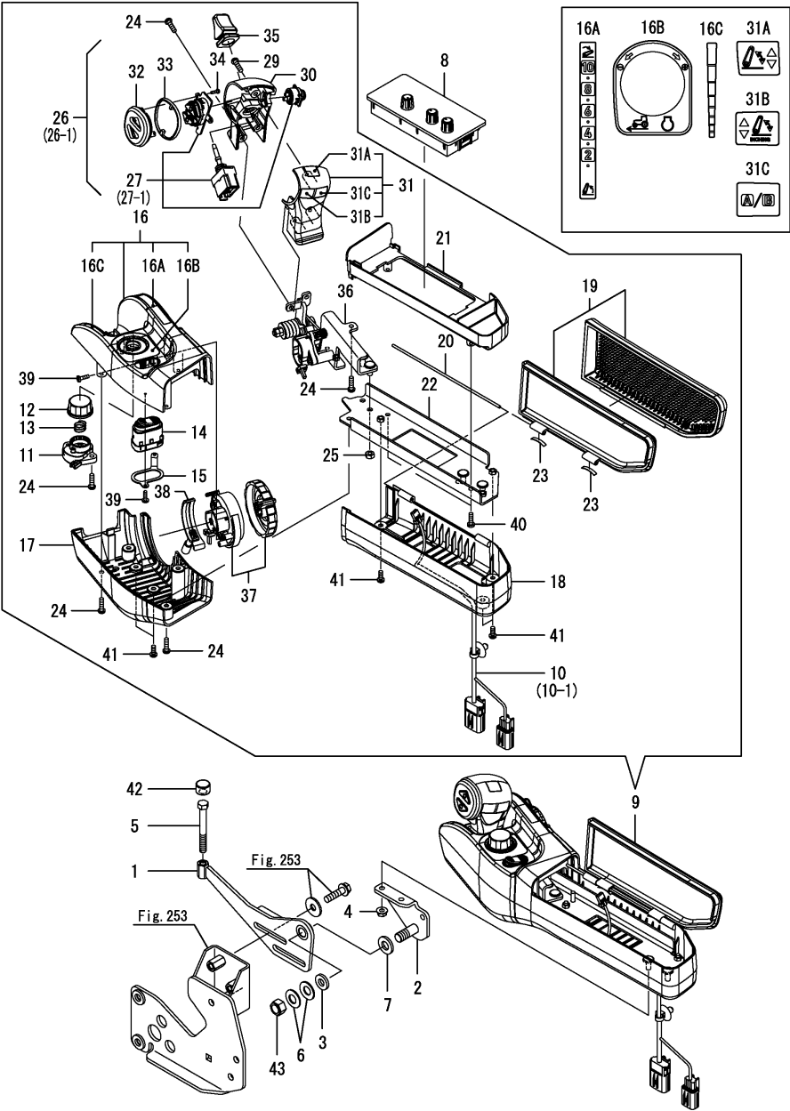
Fig.250. 팔걸이
