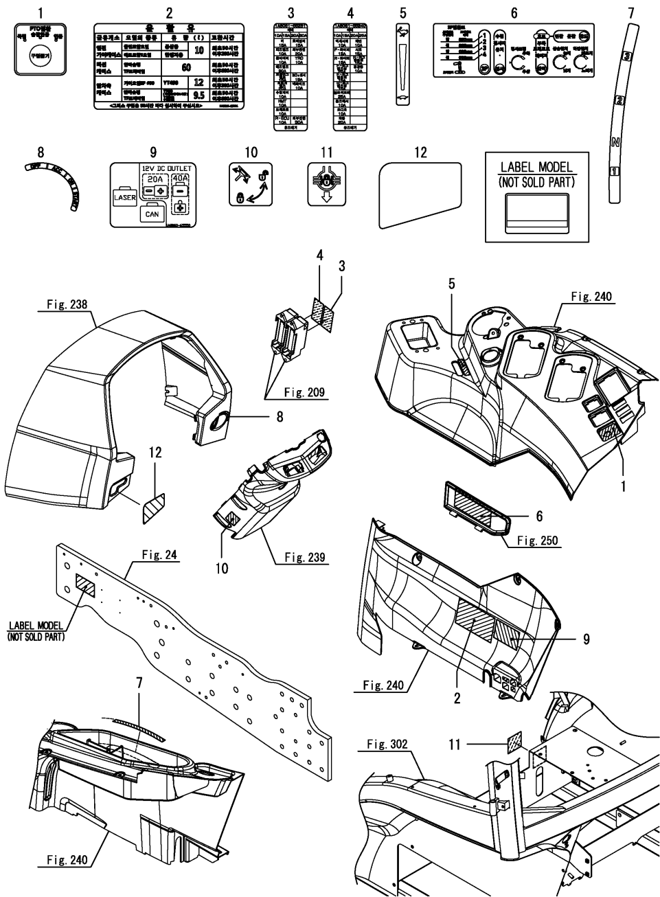
Fig.257. 명판(2)
