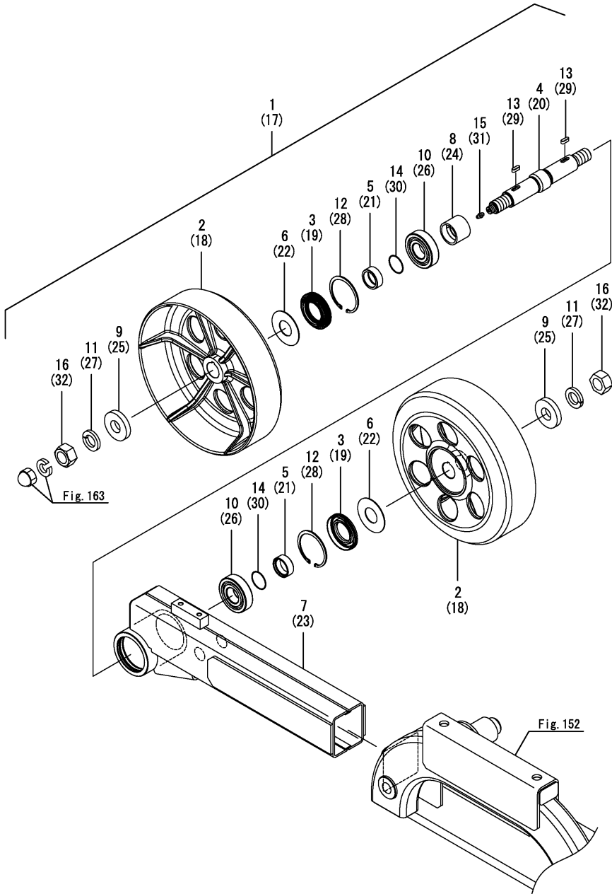
Fig.148. 아이들러(전방)(델타)
