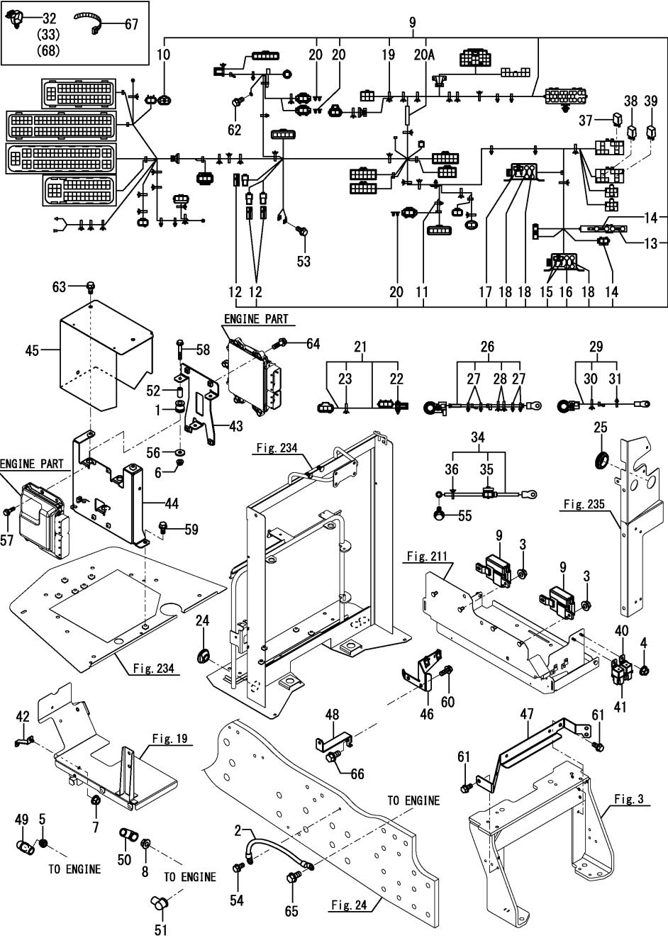
Fig.206. 배선 하네스(엔진)
