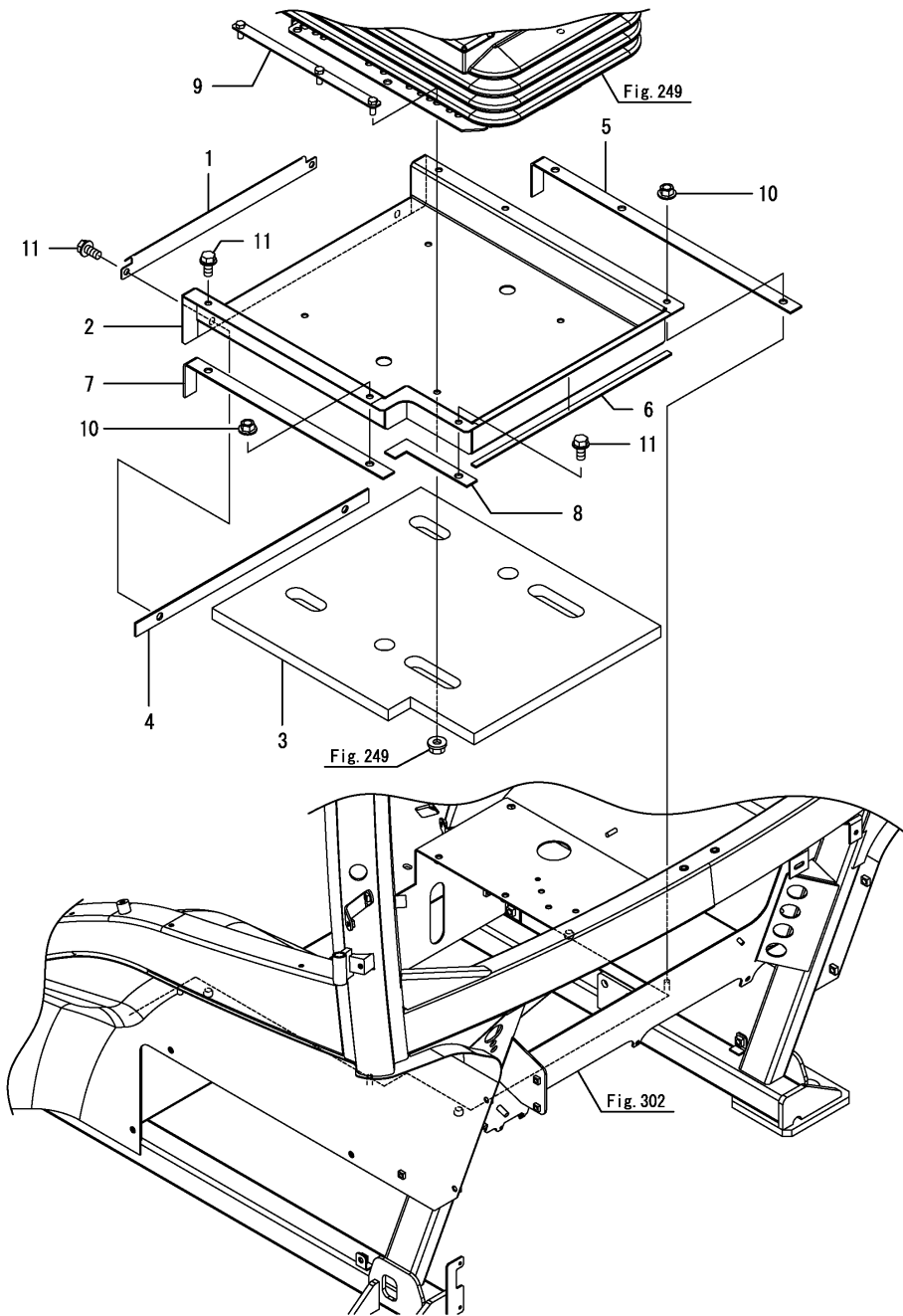
Fig.252. 더스트커버조합
