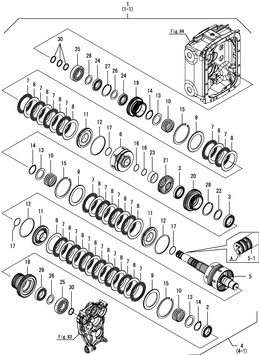
Fig.94. 클러치 샤프트(델타)
