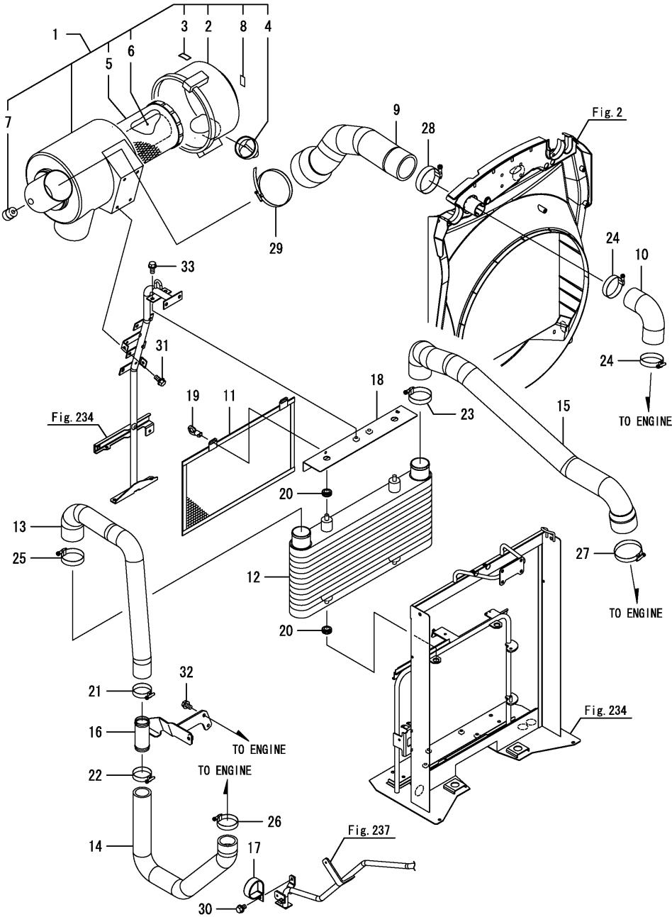
Fig.20. 에어클리너
