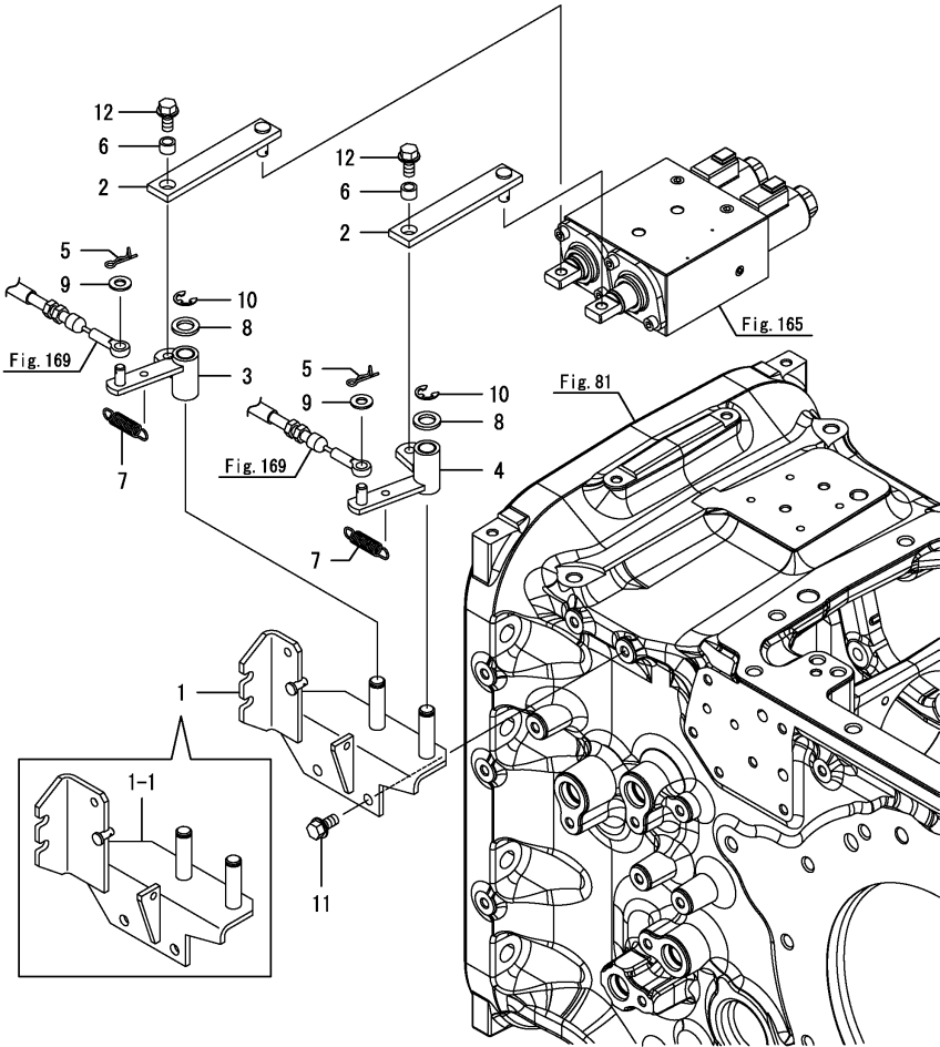
Fig.166. 링크(자동브레이크)
