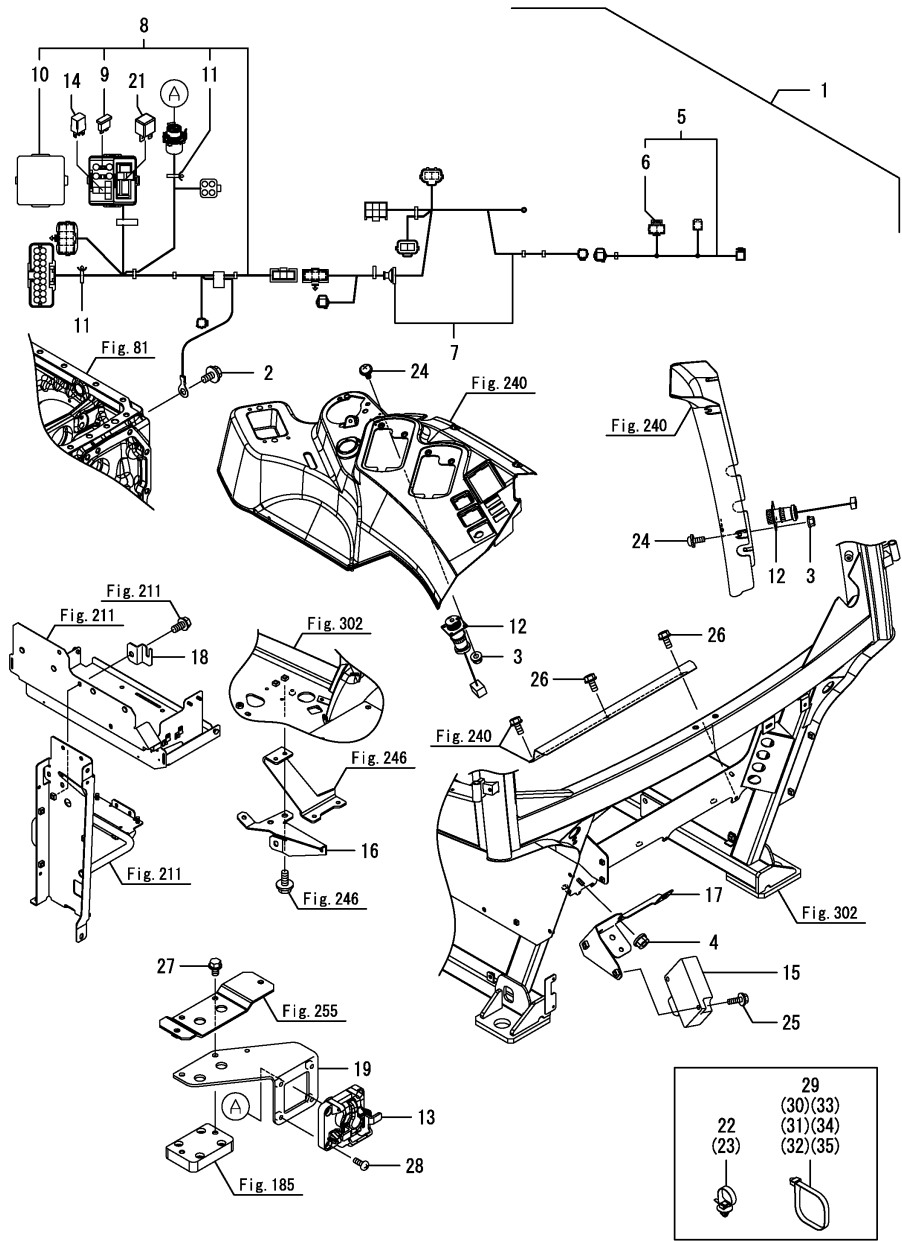
Fig.342. 커넥터(ISOBUS)
