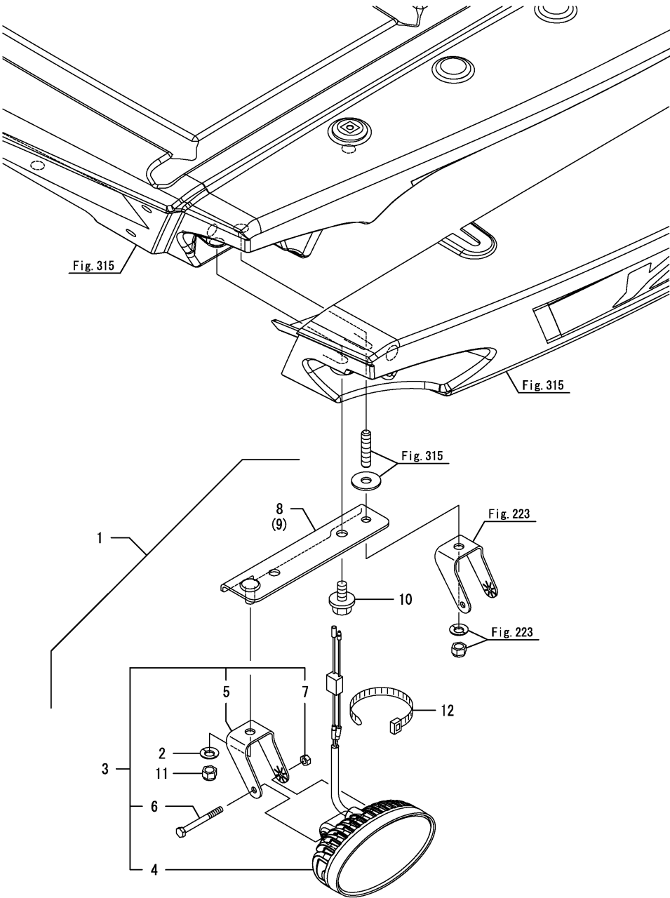
Fig.337. 작업등(루프)(후방)
