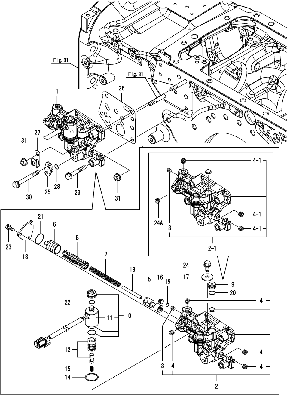
Fig.88. P.T.O. 밸브
