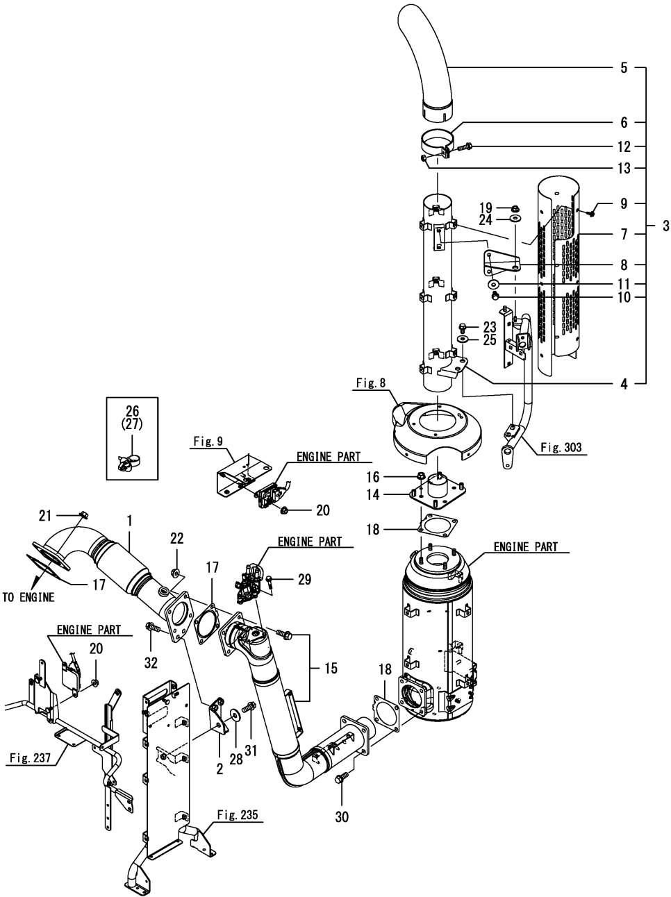
Fig.7. 배기파이프
