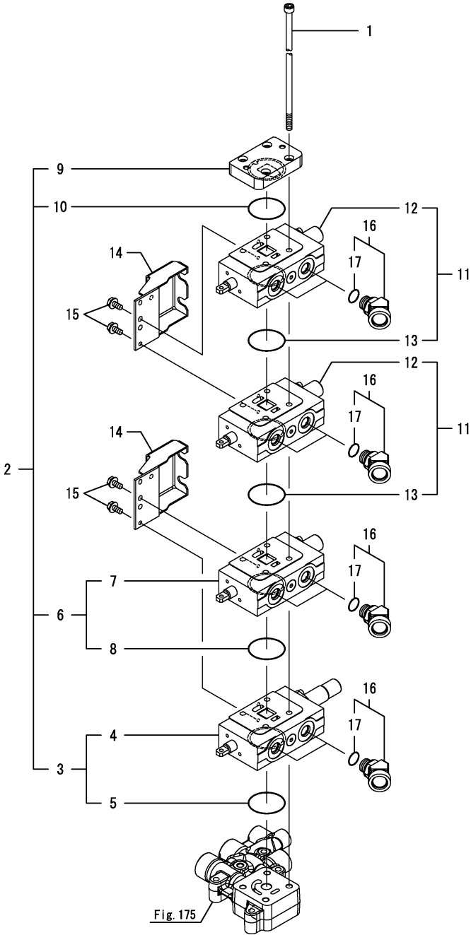
Fig.185. S.C.V.(4런)
