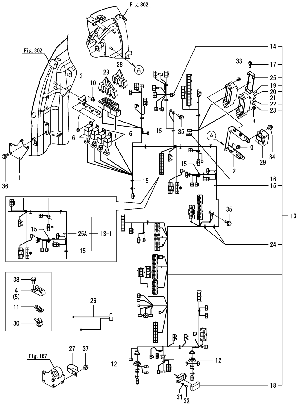
Fig.209. 배선(바닥)
