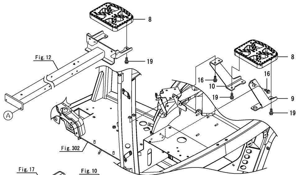
Fig.247. 보조 발판(델타)
