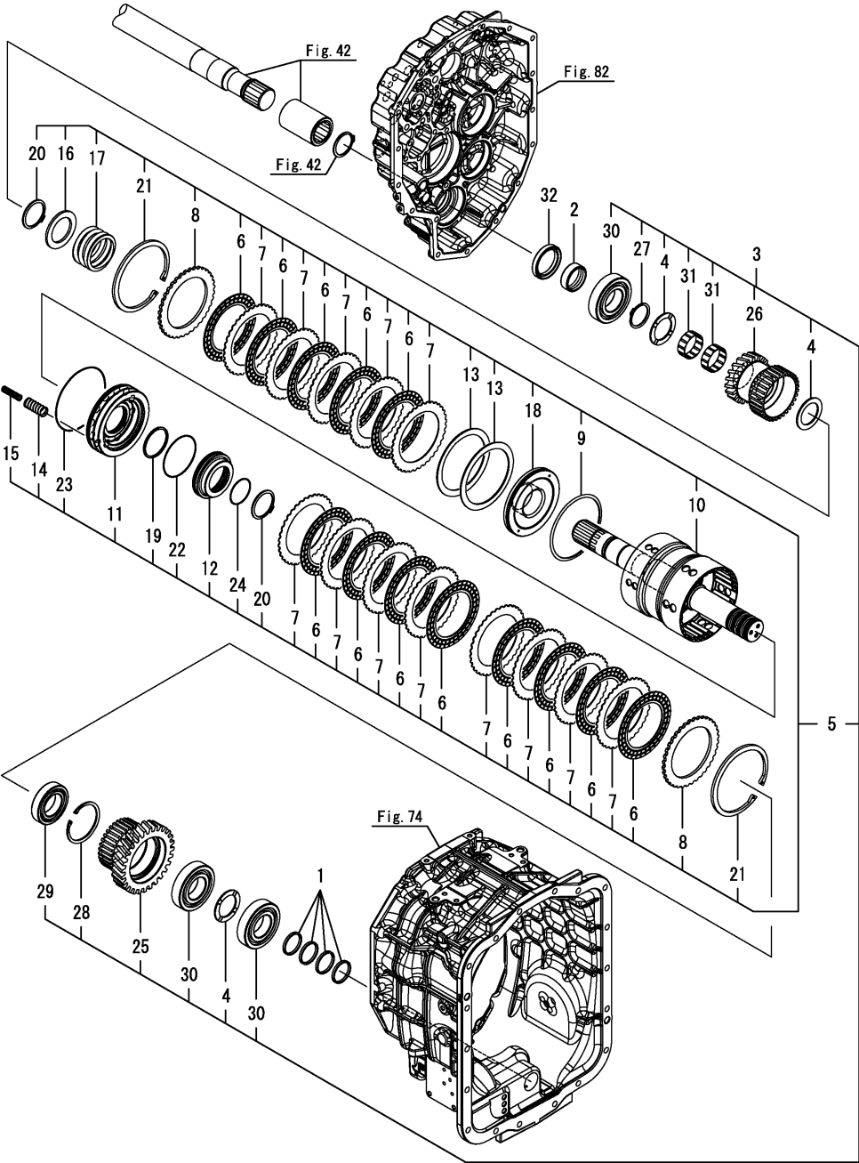
Fig.116. 전륜구동
