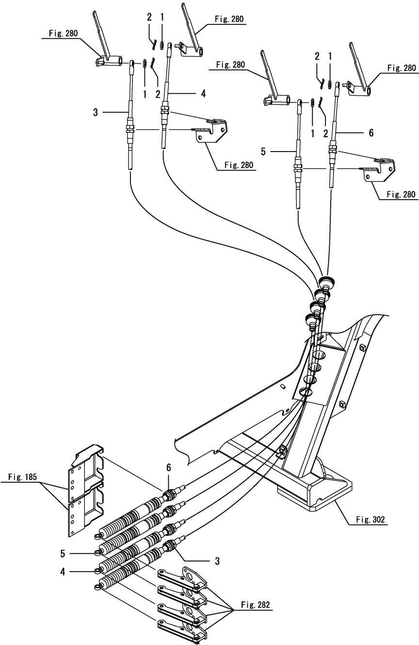
Fig.281. S.C.V.레버와이어(4련)
