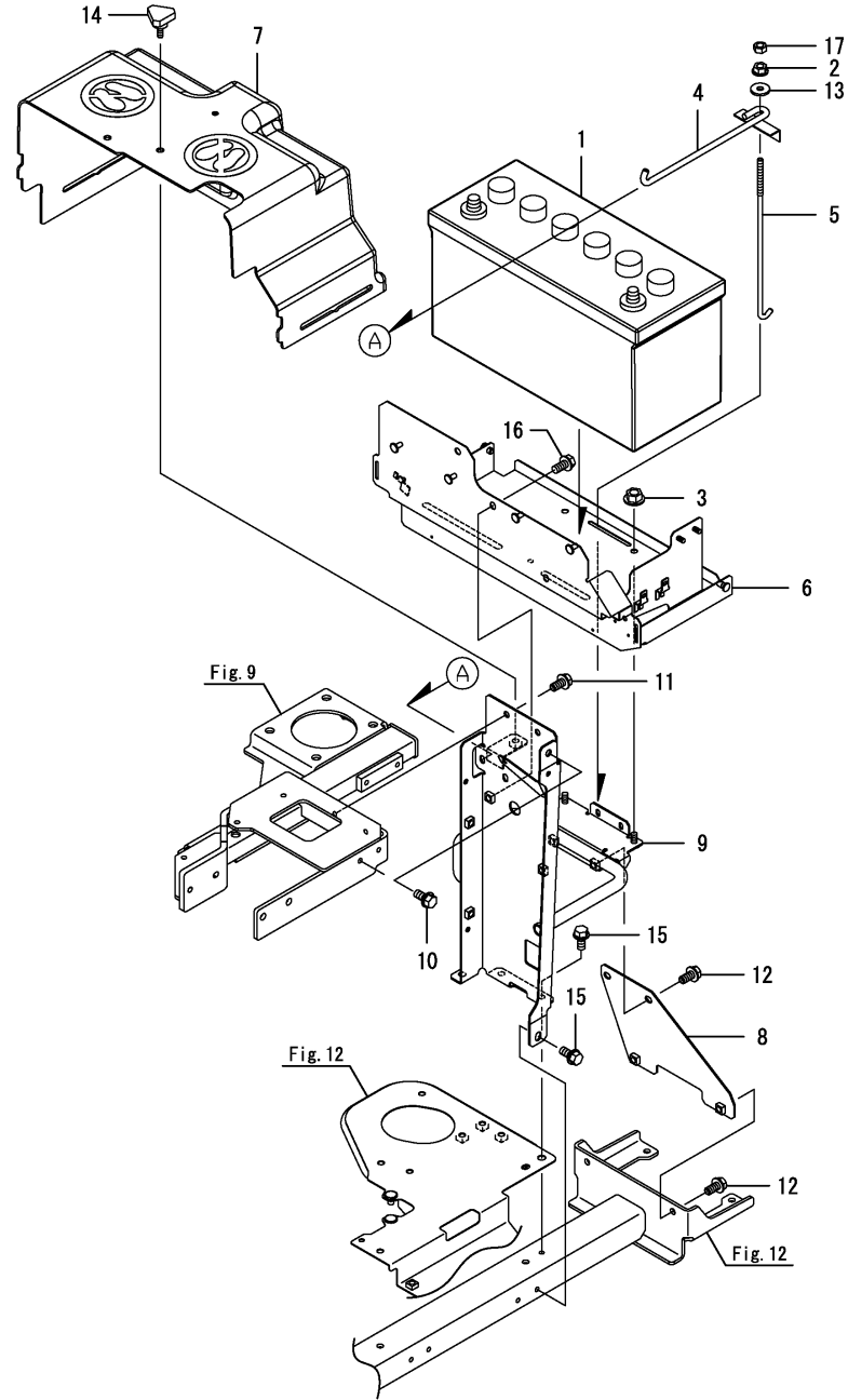
Fig.211. 배터리
