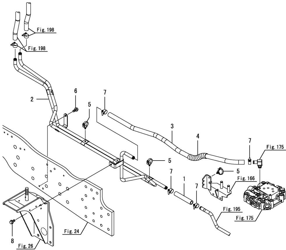
Fig.199. 오일쿨러파이프
