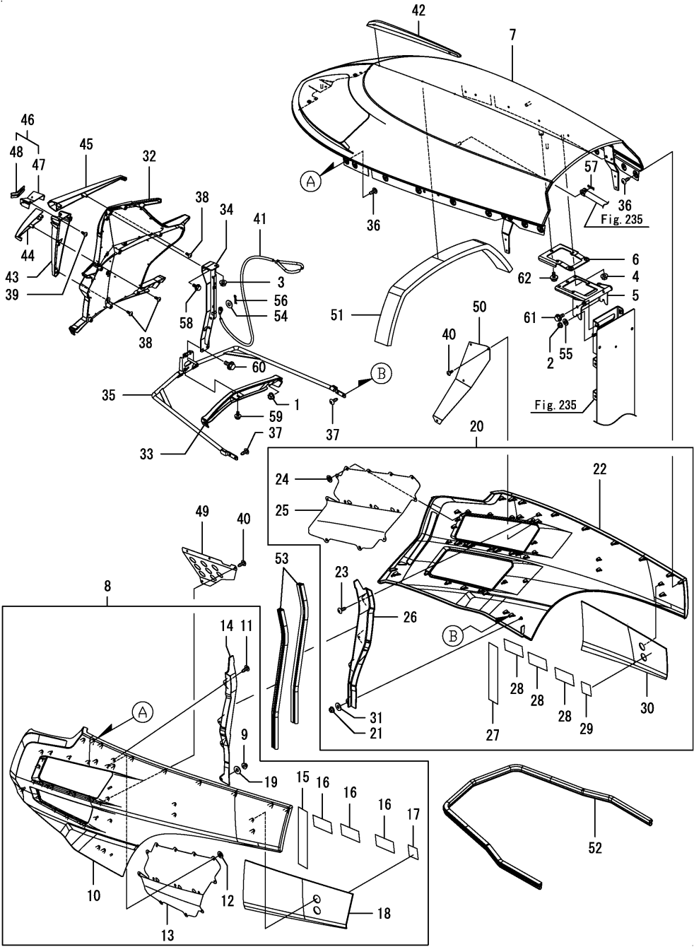
Fig.236. 본네트
