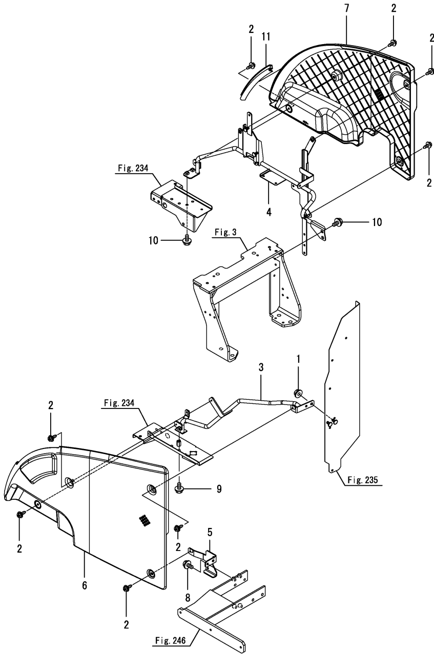
Fig.237. 사이드커버
