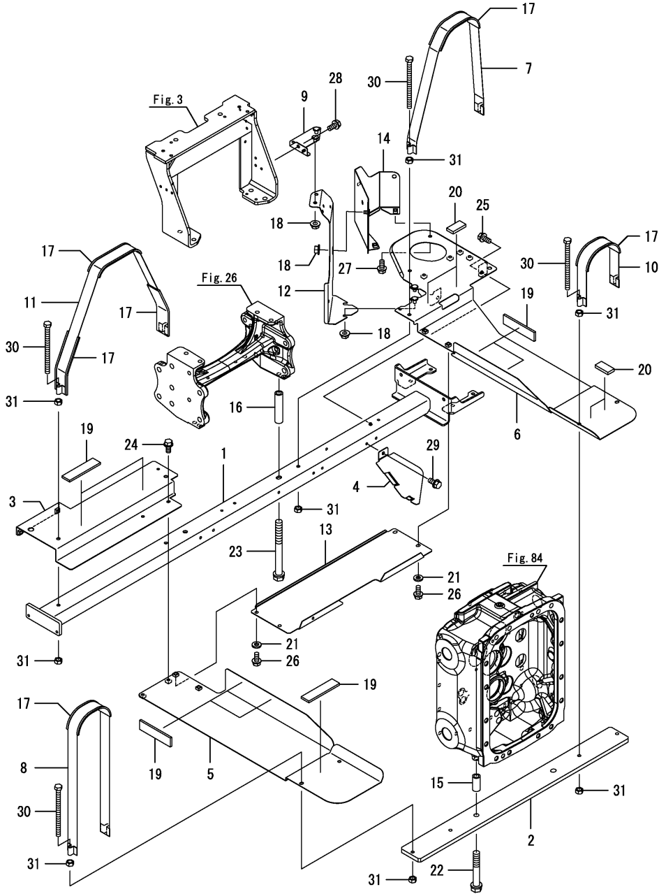
Fig.13. 탱크커버
