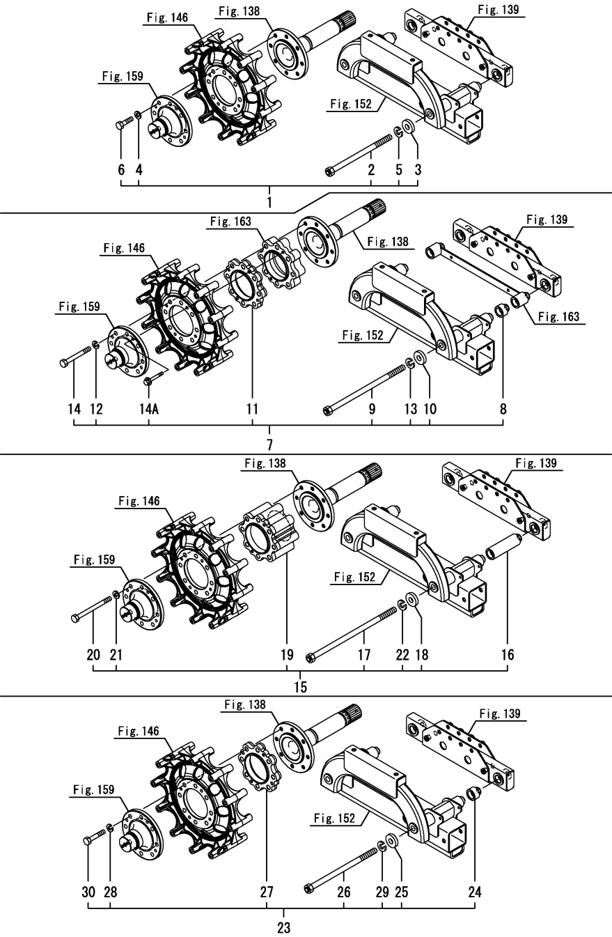
Fig.334. 트레드(후방)(델타)
