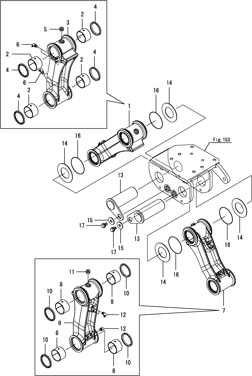
Fig.154. 링크 암(델타)
