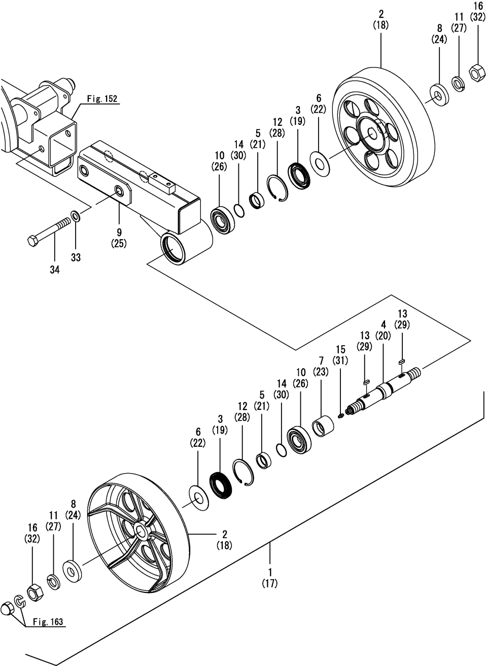
Fig.149. 아이들러(후방)(델타)
