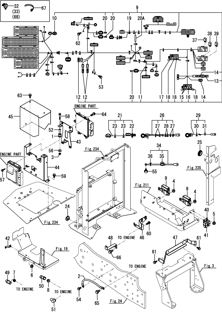
Fig.205. 배선 하네스(엔진)
