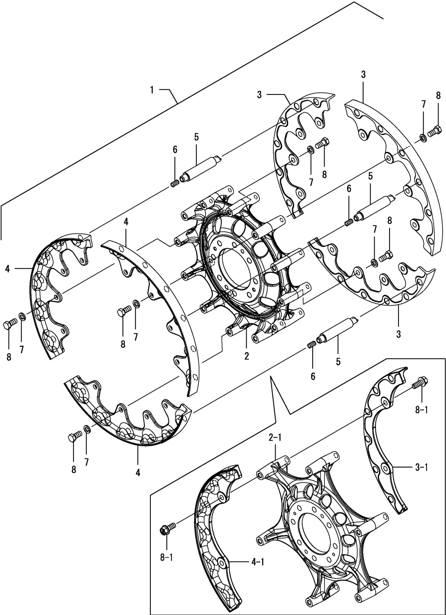
Fig.146. 스프로킷(델타)
