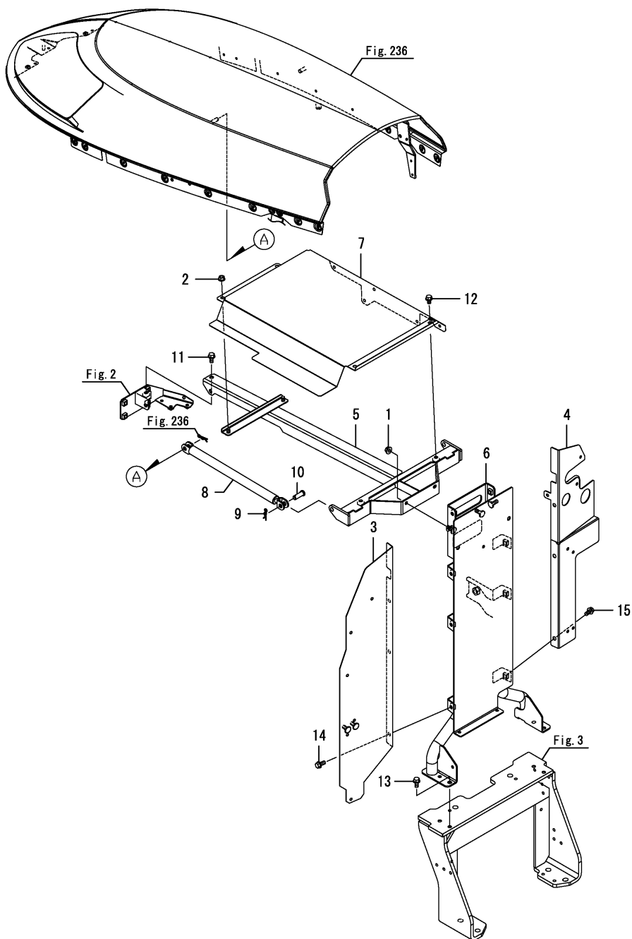
Fig.235. 리어프레임
