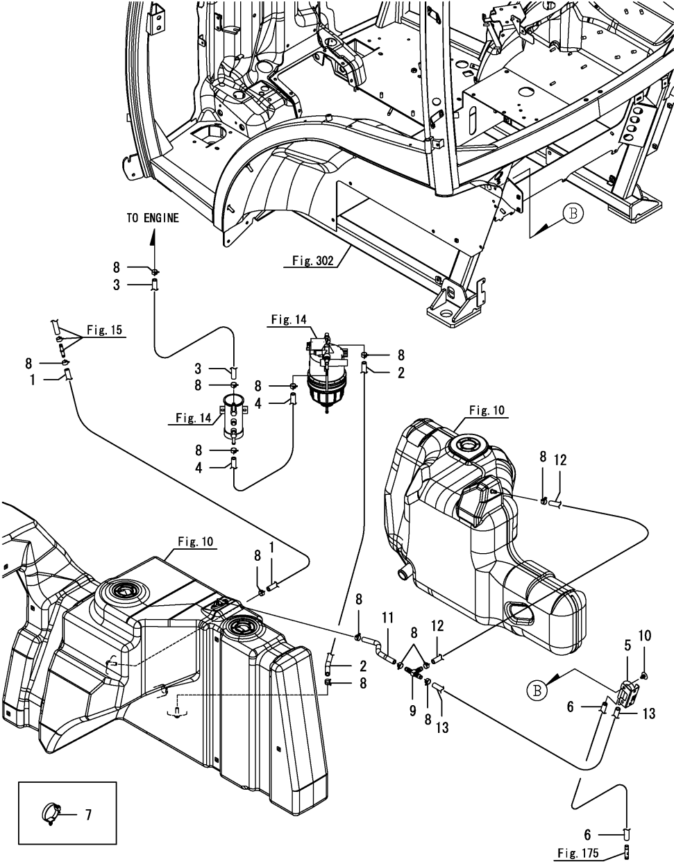
Fig.16. 연료호스
