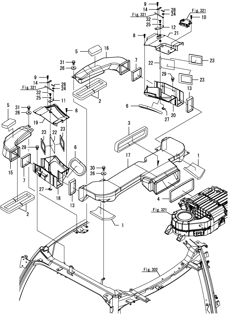
Fig.324. 에어컨덕트
