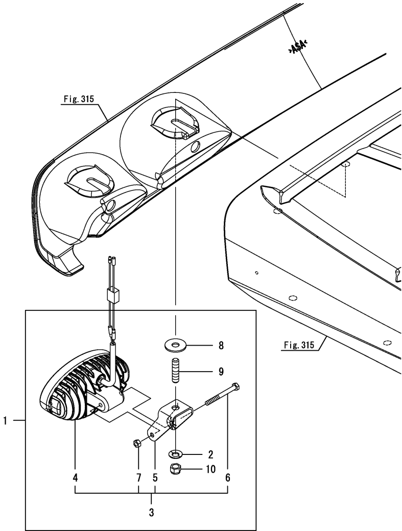
Fig.336. 작업등(루프)(전방)
