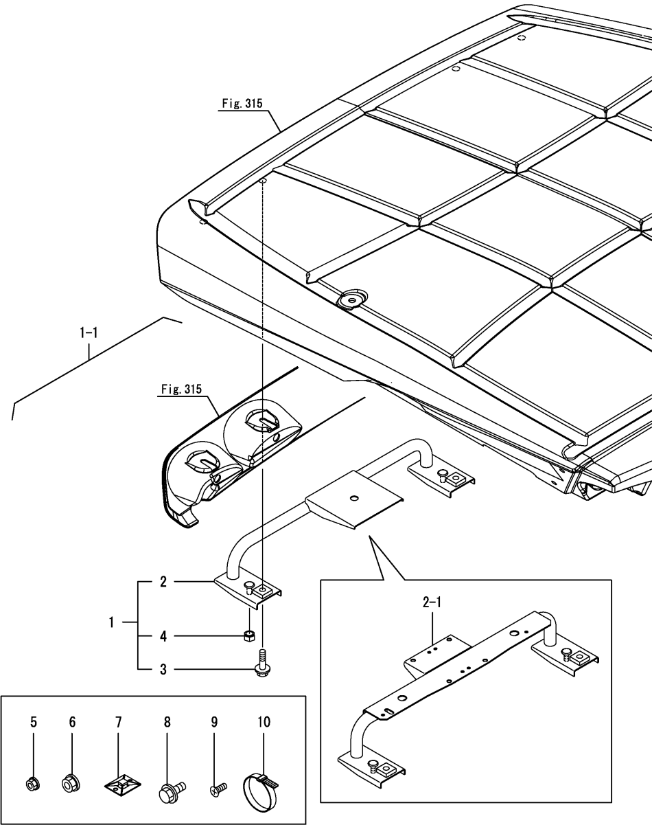
Fig.339. 스테이(GPS)
