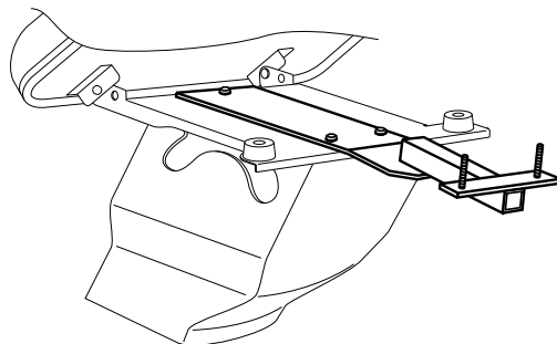
RXD-4, RXC～E型用本体取付金具 （オプション）
