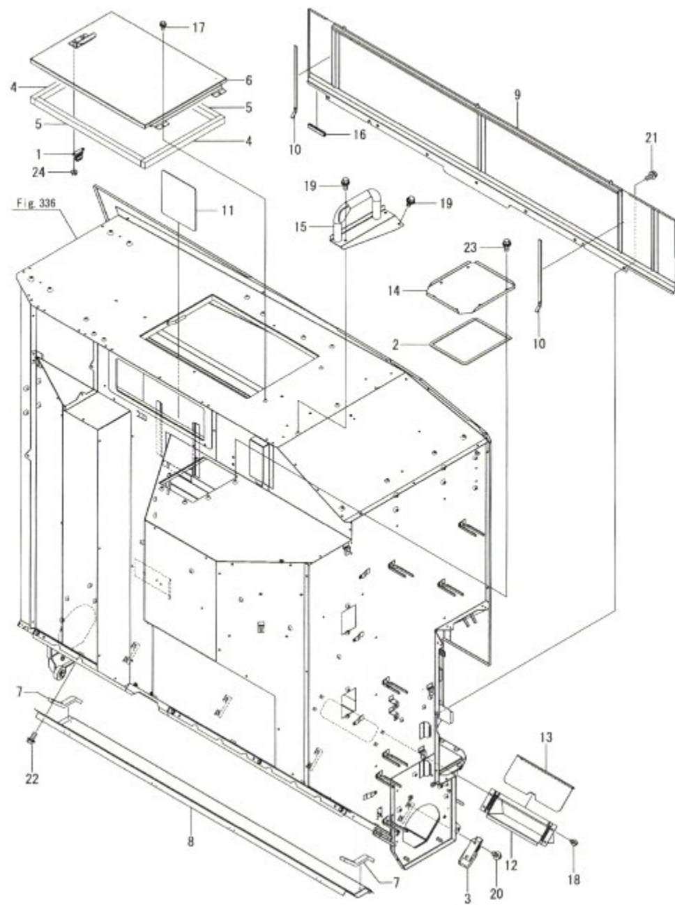
Fig.337. 곡물탱크(2)
