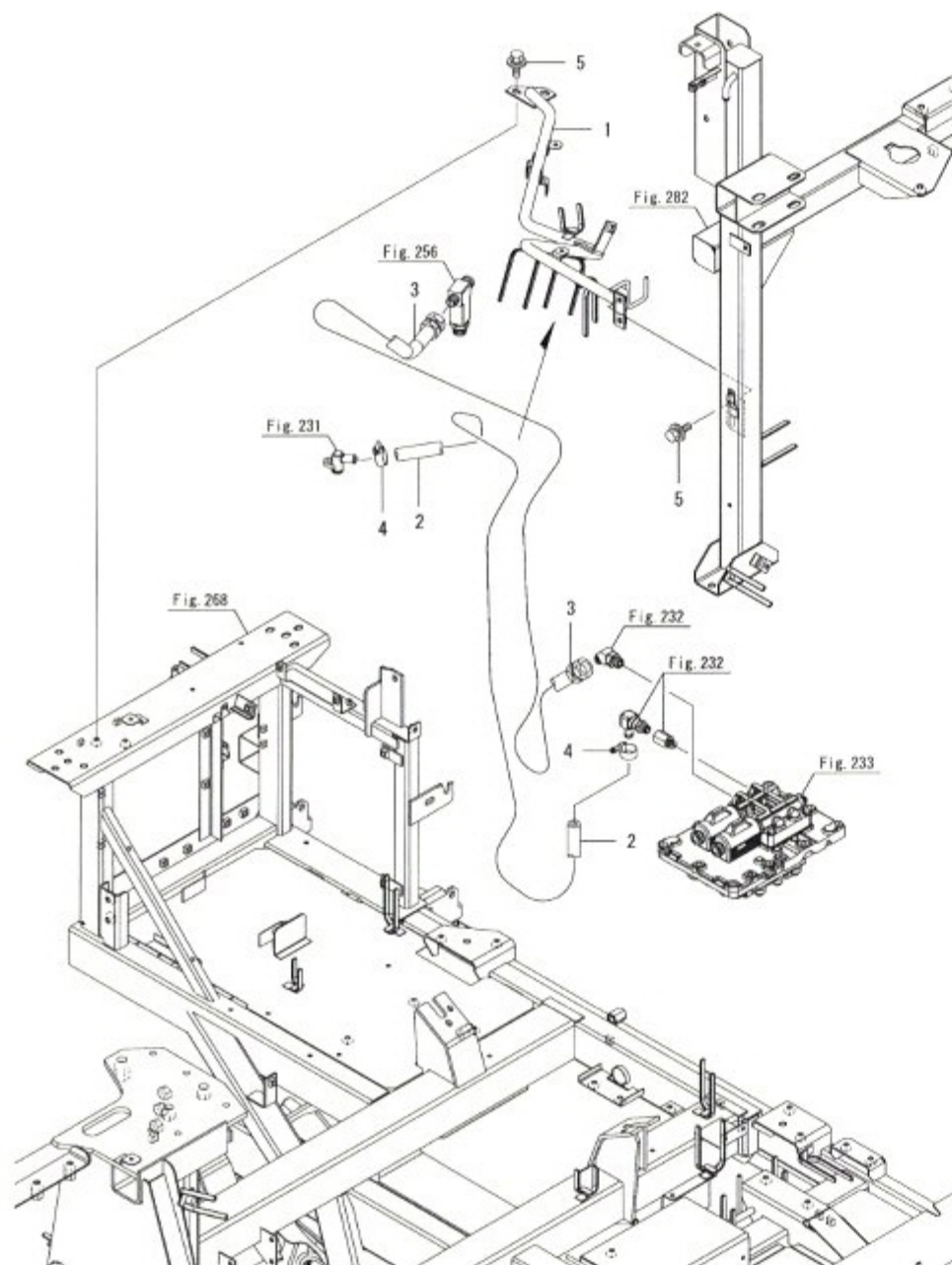
Fig.255. 배관(카운터케이스)
