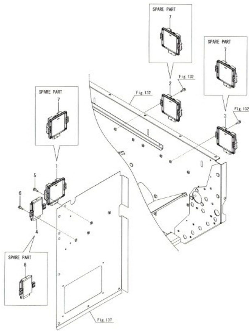
Fig.138. 컨트롤러(탈곡)
