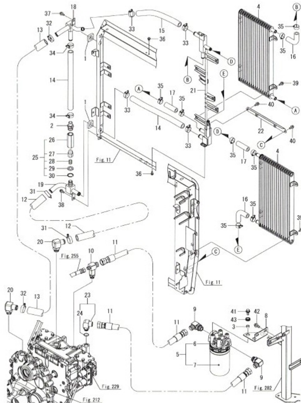
Fig.256. 배관(H.S.T.)
