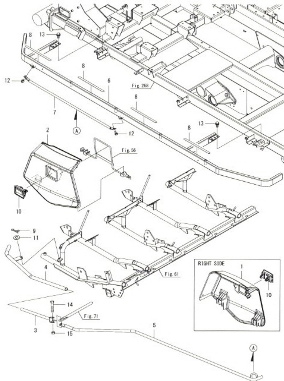
Fig.18. 예취(2)
