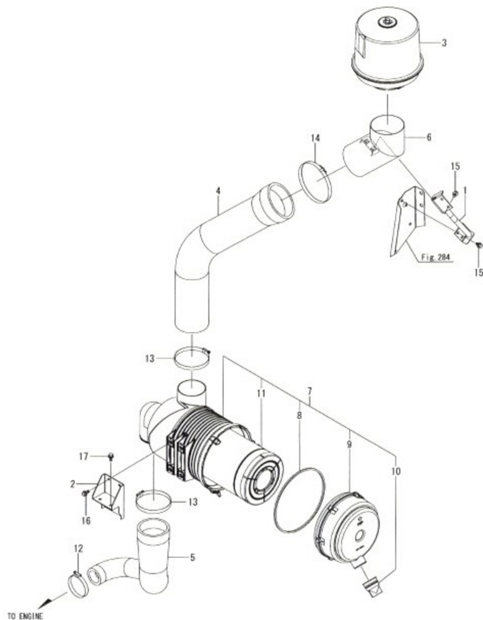
Fig.8. 에어클리너
