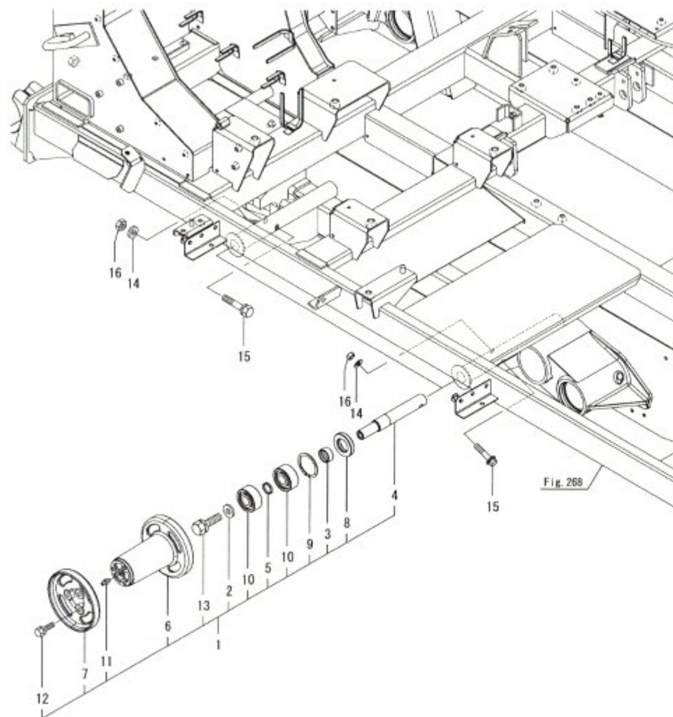
Fig.278. 캐리어 롤러
