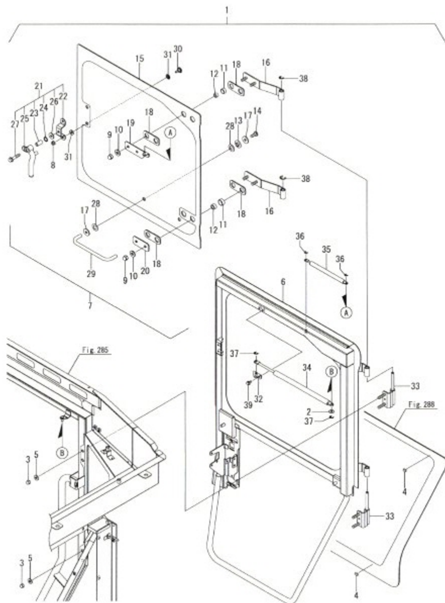
Fig.287. 캐빈 프레임(3)
