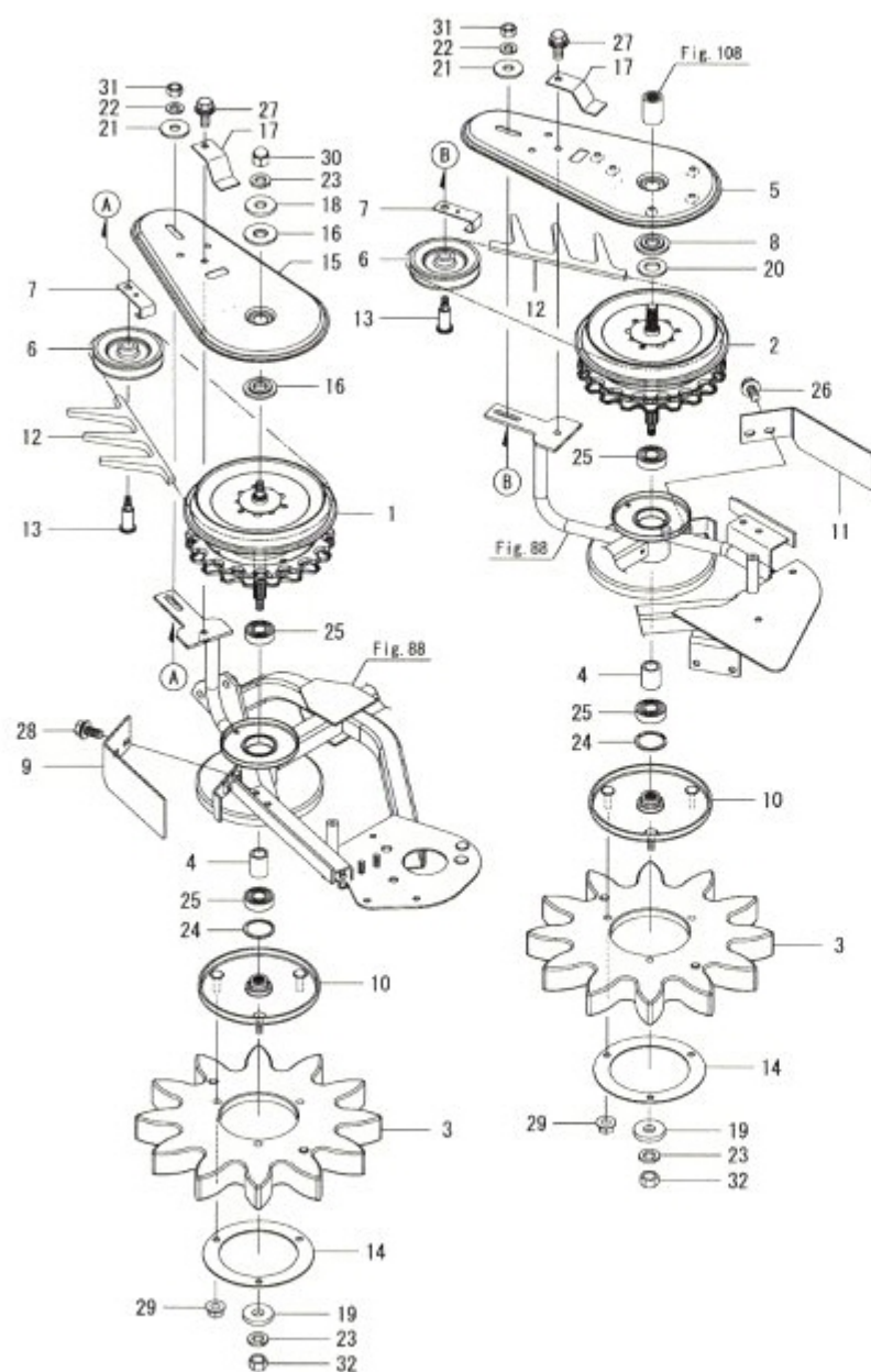
Fig.79. 스타휠(중-우)
