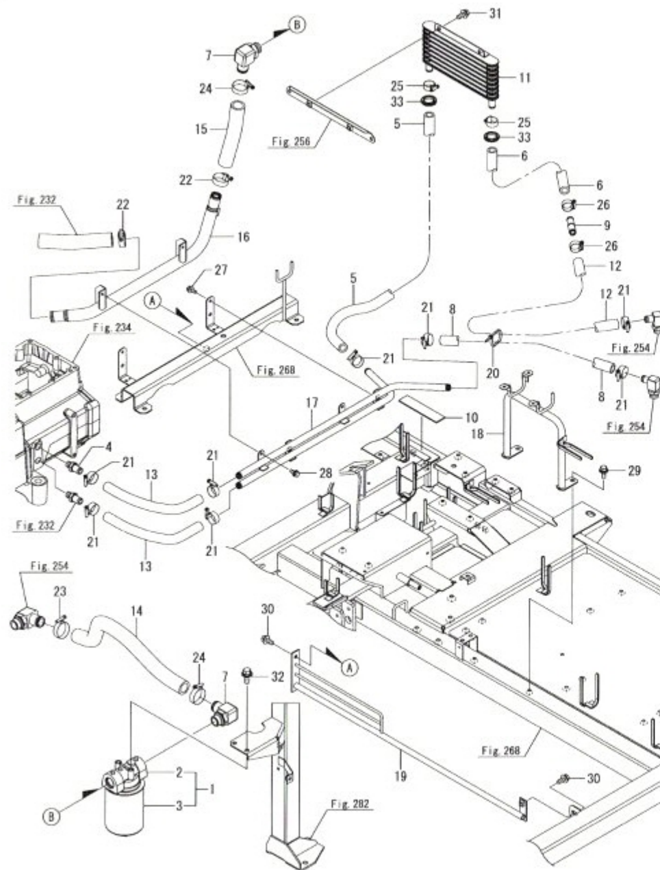
Fig.258. 배관(2)
