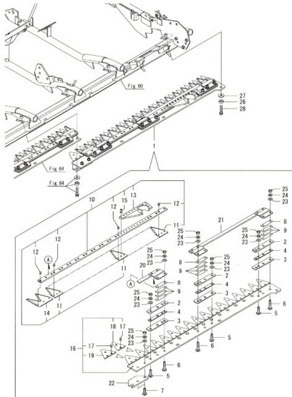
Fig.65. 예취날(우)
