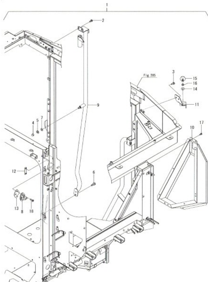
Fig.290. 캐빈 프레임(6)
