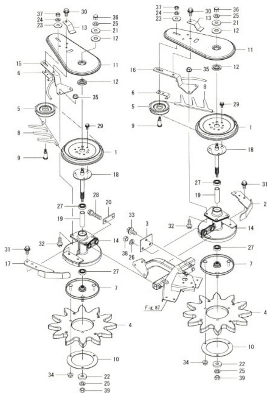
Fig.78. 스타휠(중-우)
