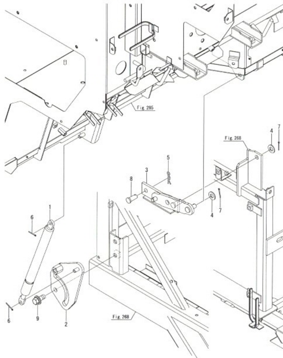
Fig.264. 바닥판오픈
