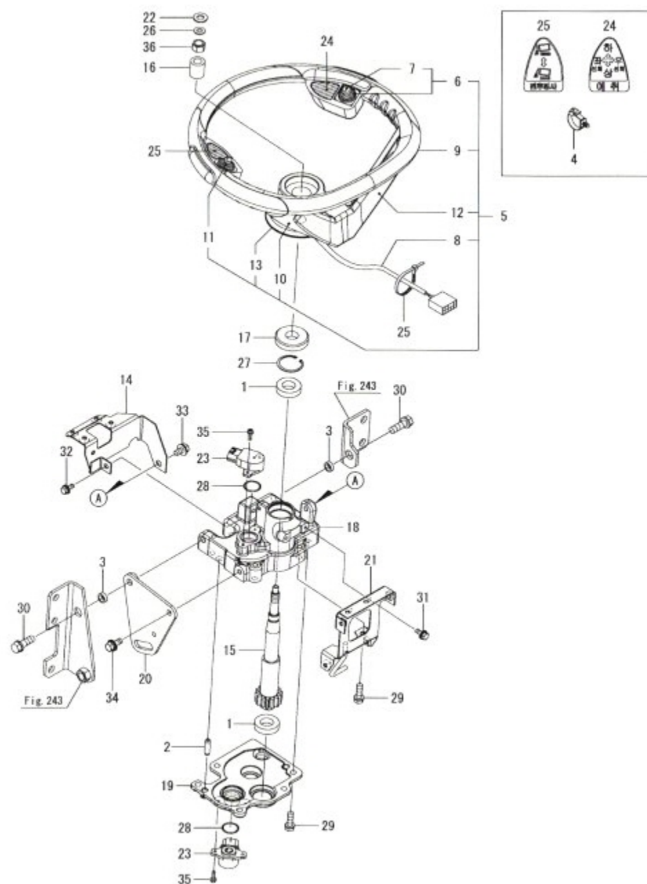
Fig.244. 스티어링(1)
