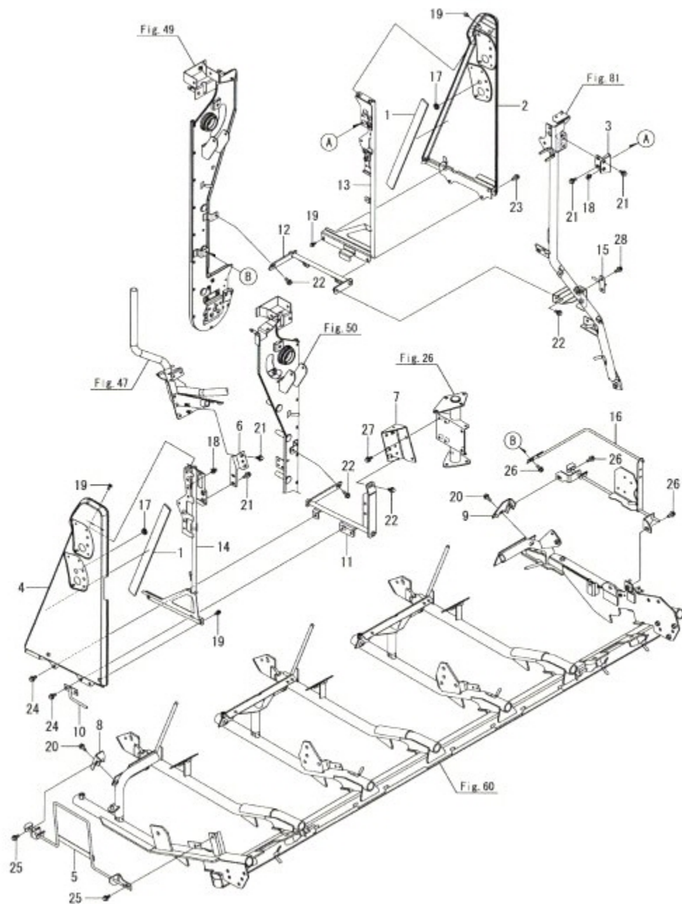
Fig.56. 예취커버(1)
