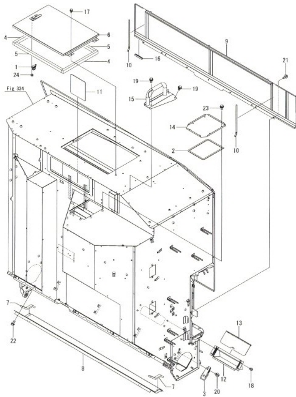
Fig.335. 곡물탱크(2)
