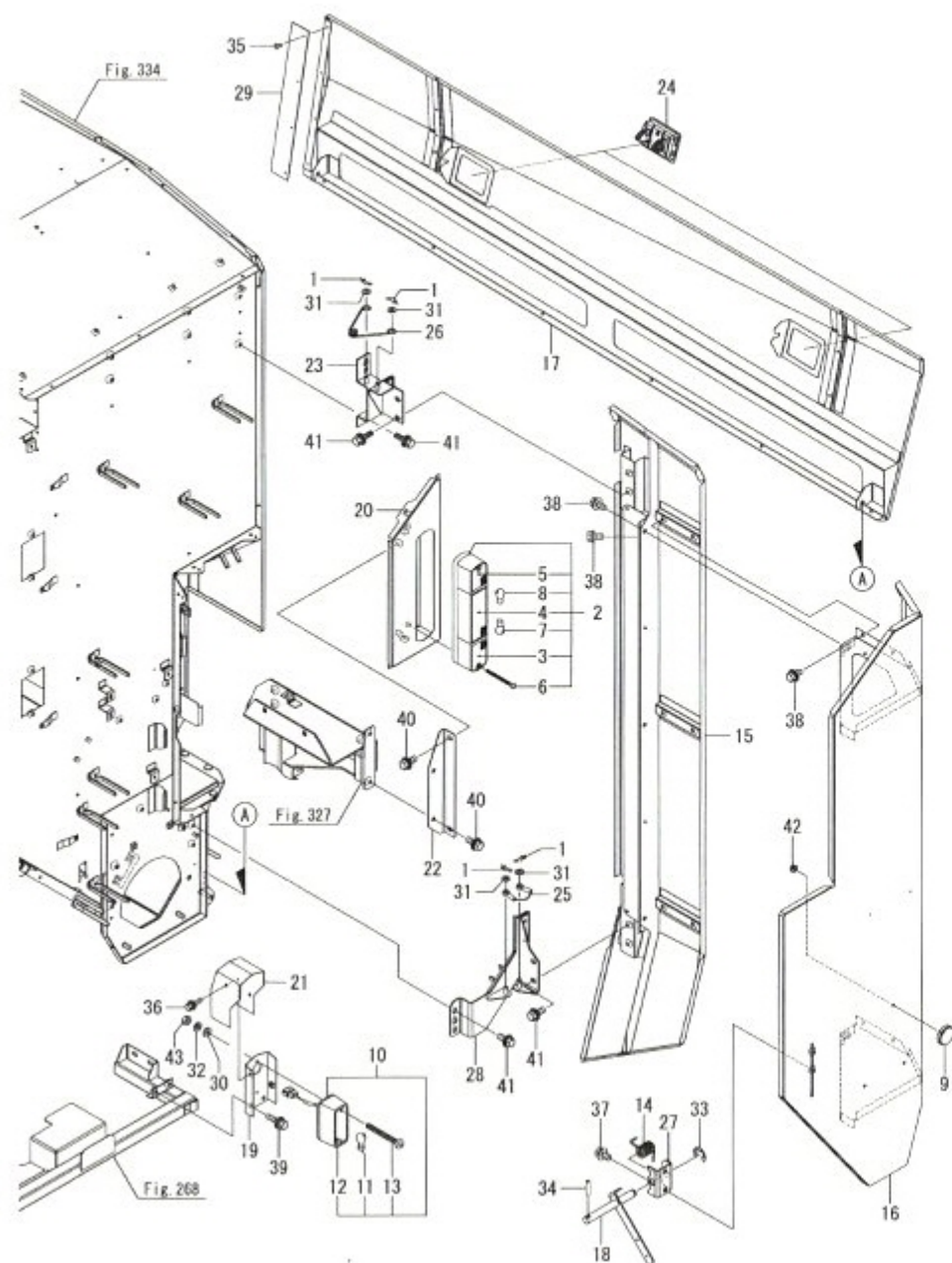
Fig.341. 탱크커버
