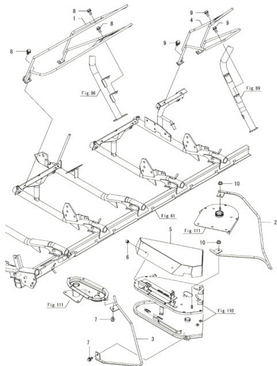
Fig.116. 상반송가이드(중)
