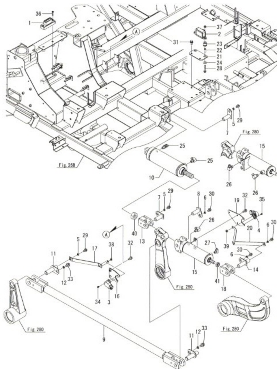
Fig.281. 스윙(2)
