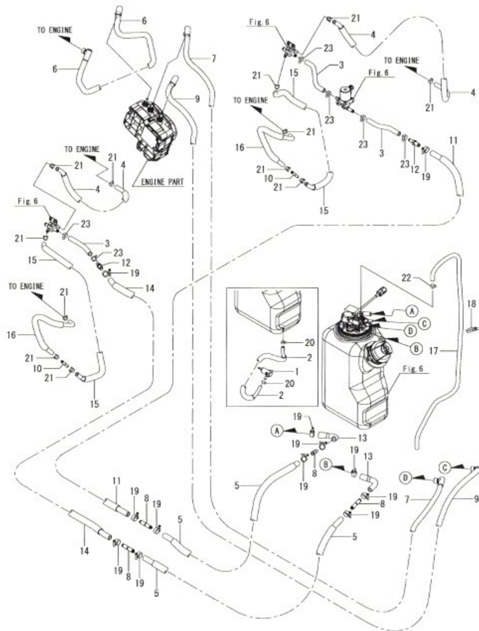
Fig.7. 요소 탱크(2)
