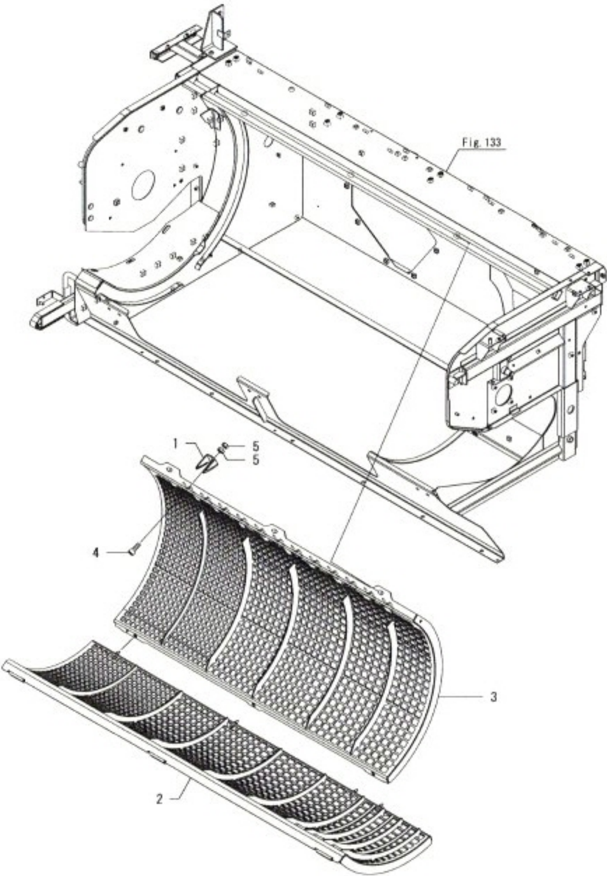
0CNP7-M01360 탈곡(1) Fig.142. 스크린 프레임
