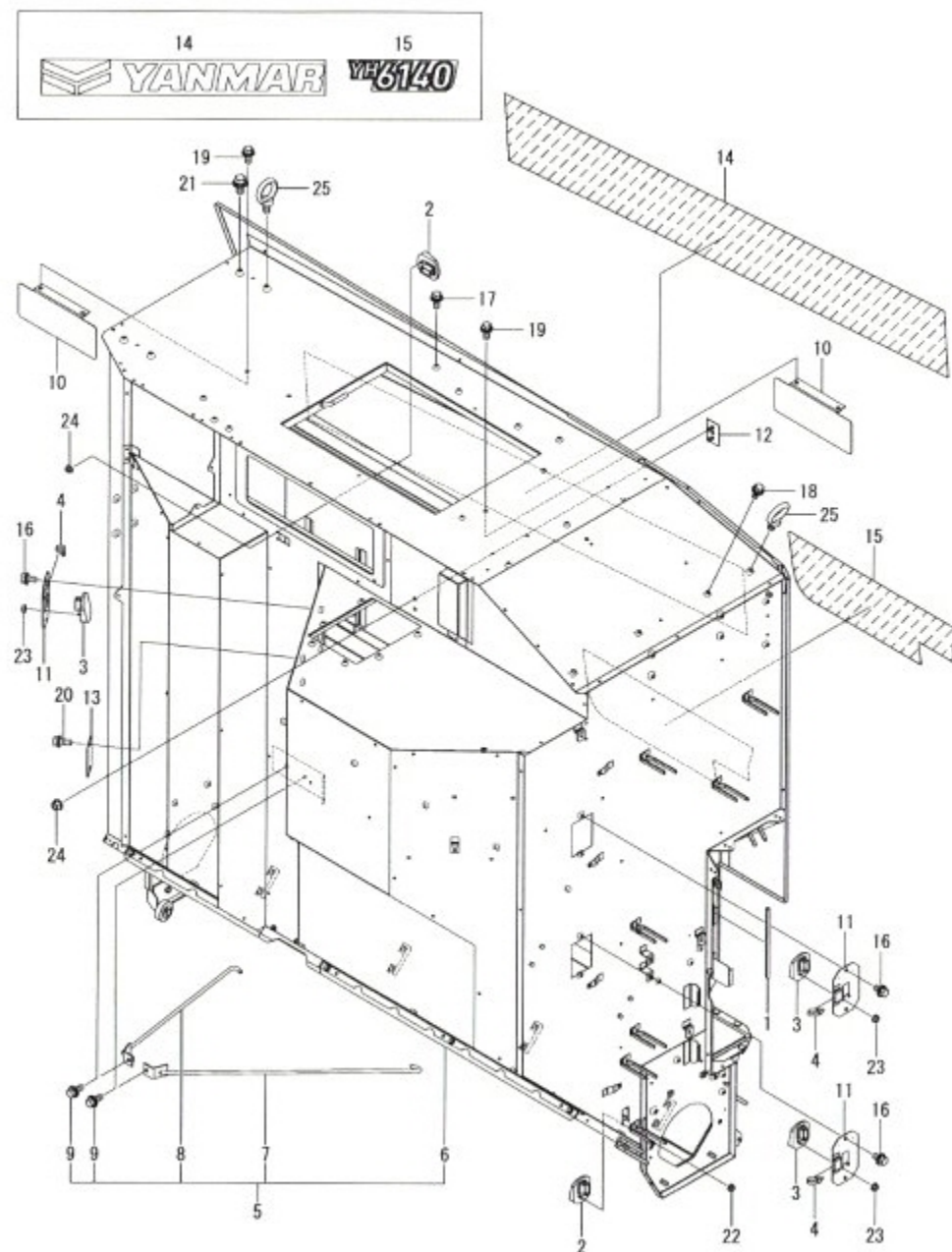
Fig.334. 곡물탱크(1)
