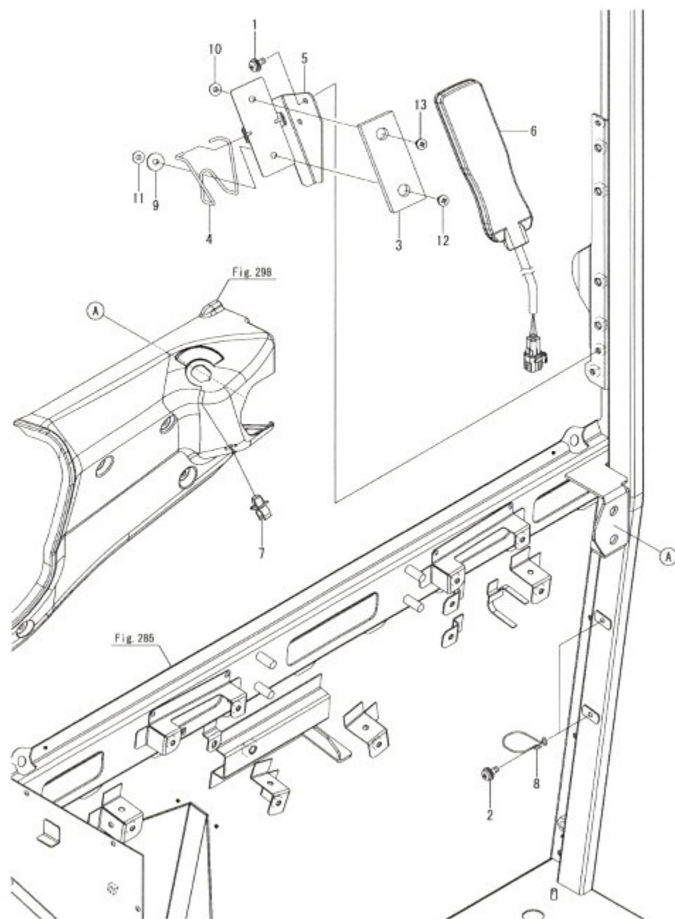
Fig.319. 스위치 마운팅
