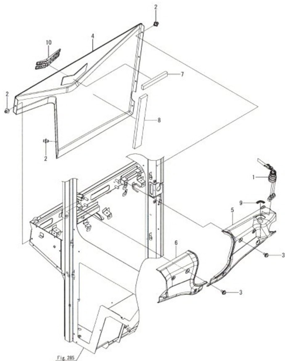
Fig.298. 캐빈의장(앞-하)
