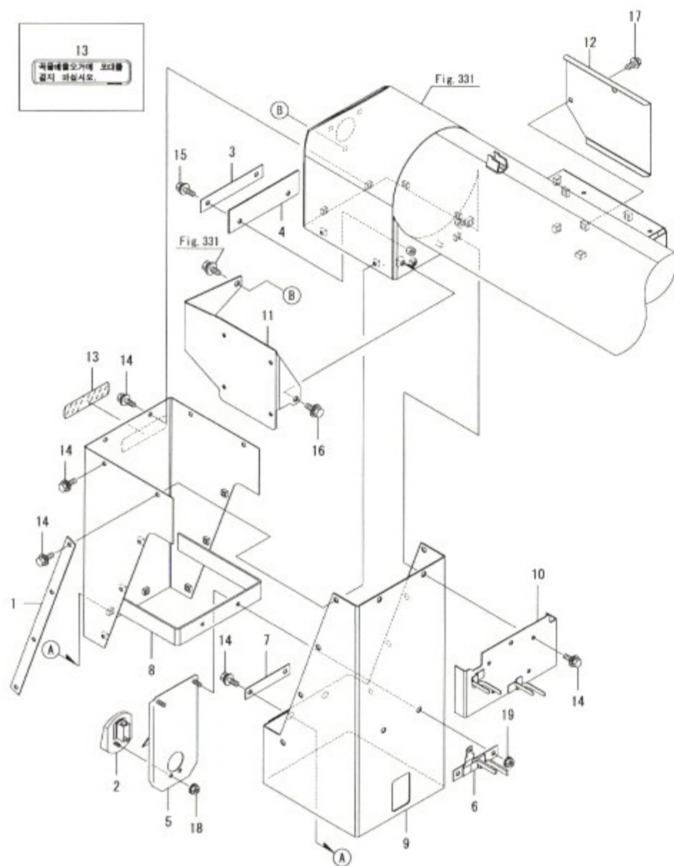
Fig.333. 오거배출구
