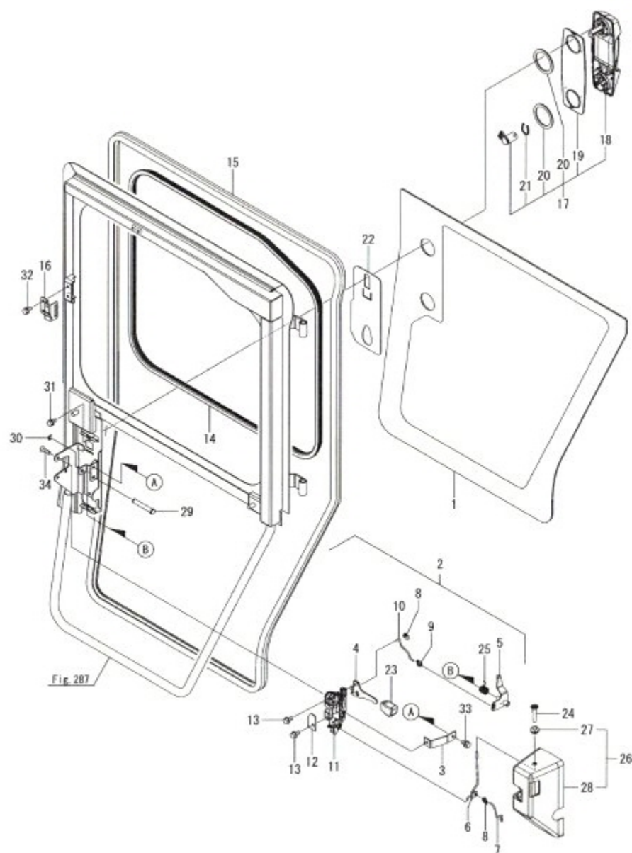
Fig.288. 캐빈 프레임(4)
