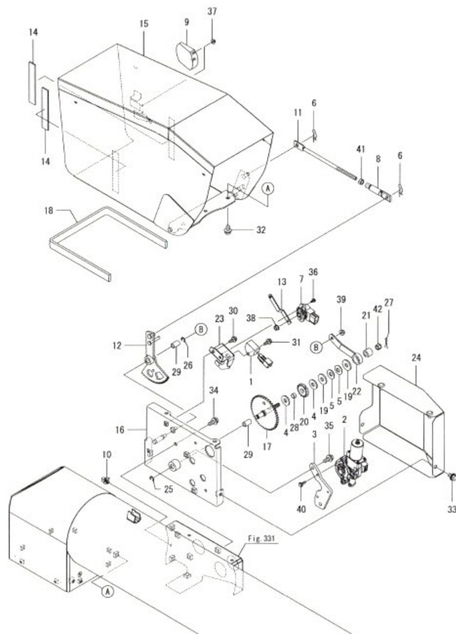
Fig.332. 오거 슈트
