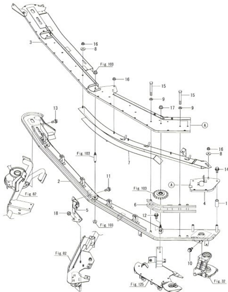
Fig.98. 상단 이송 케이스(오른쪽)
