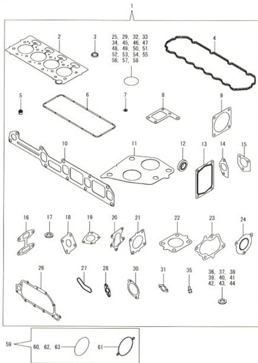
Fig.36. 가스켓 세트 1
