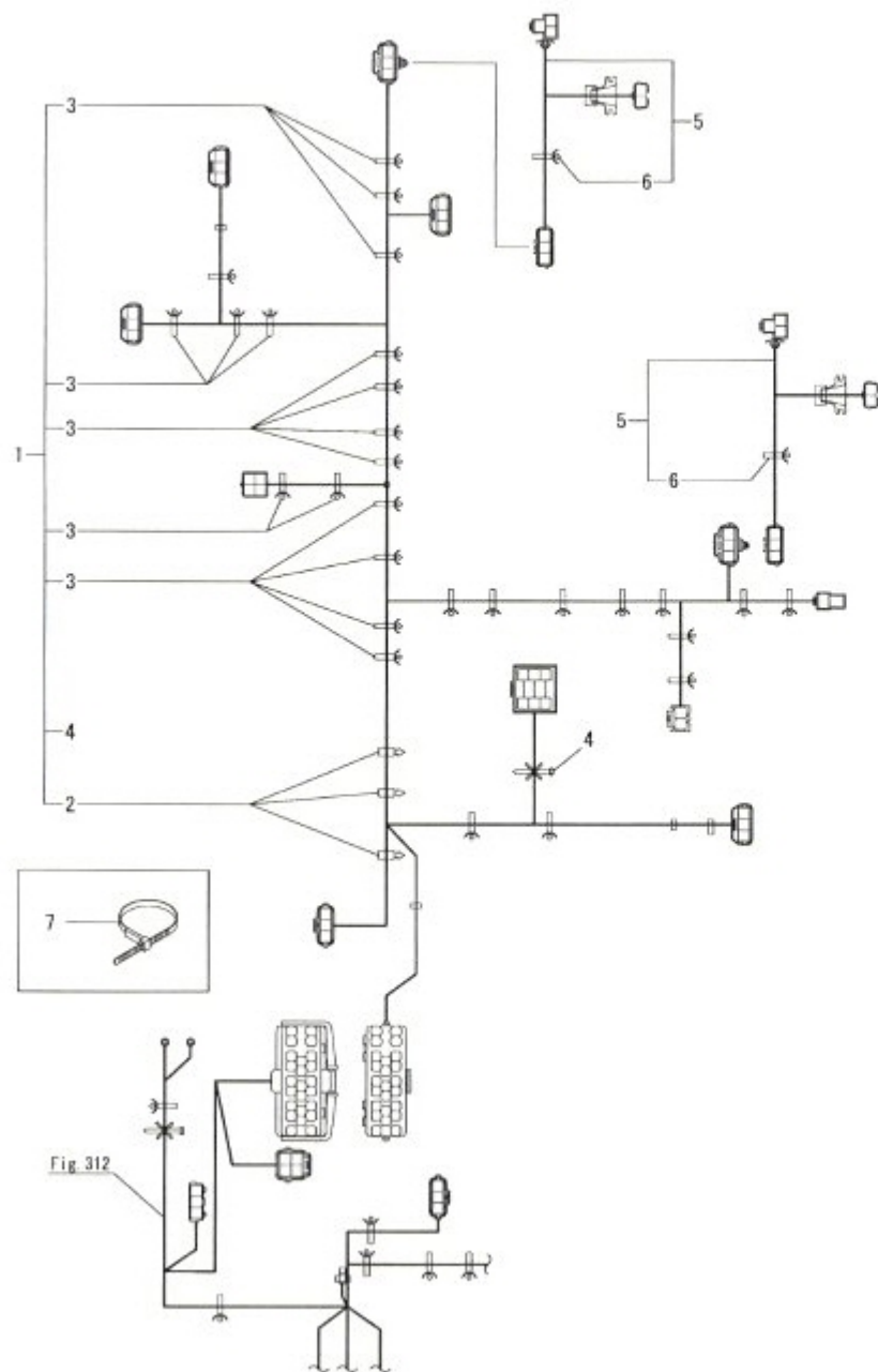
Fig.317. 배선(예취)
