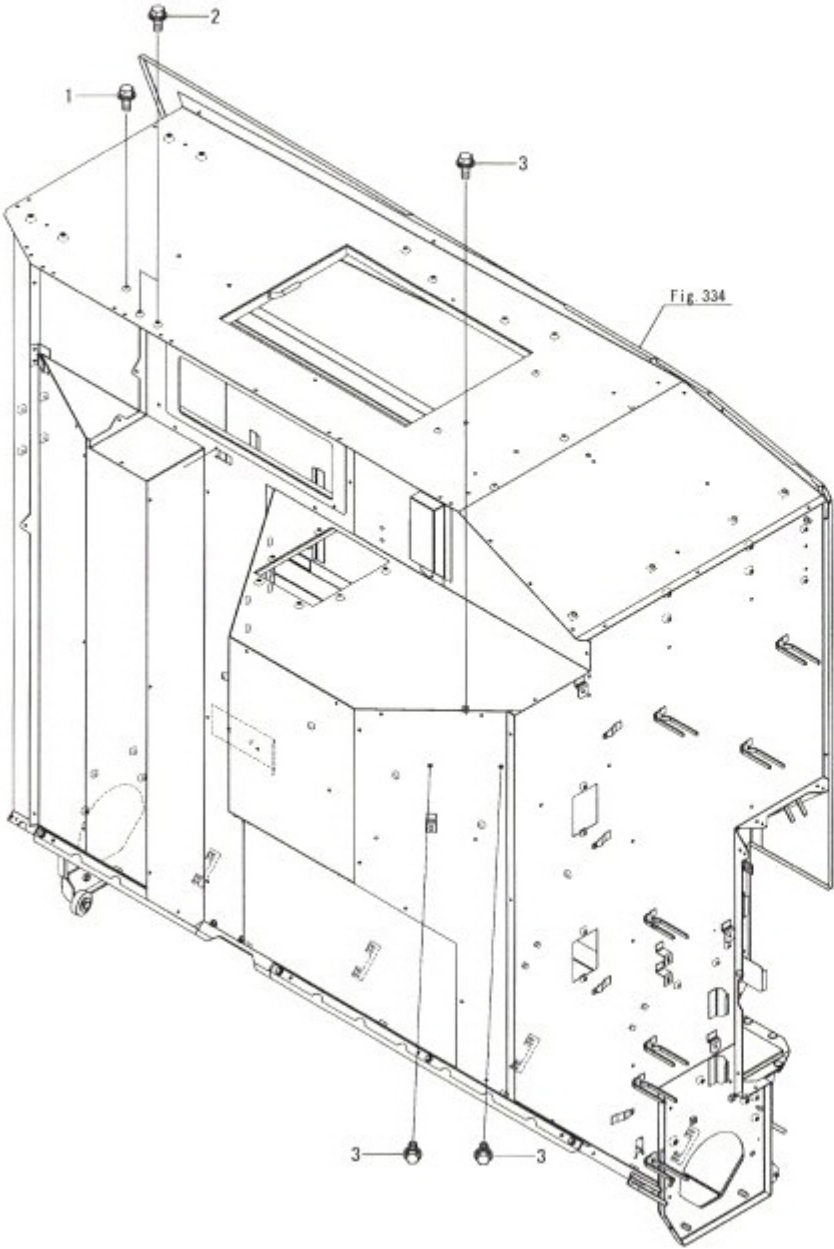
Fig.343. 오거(라디오 없음)
