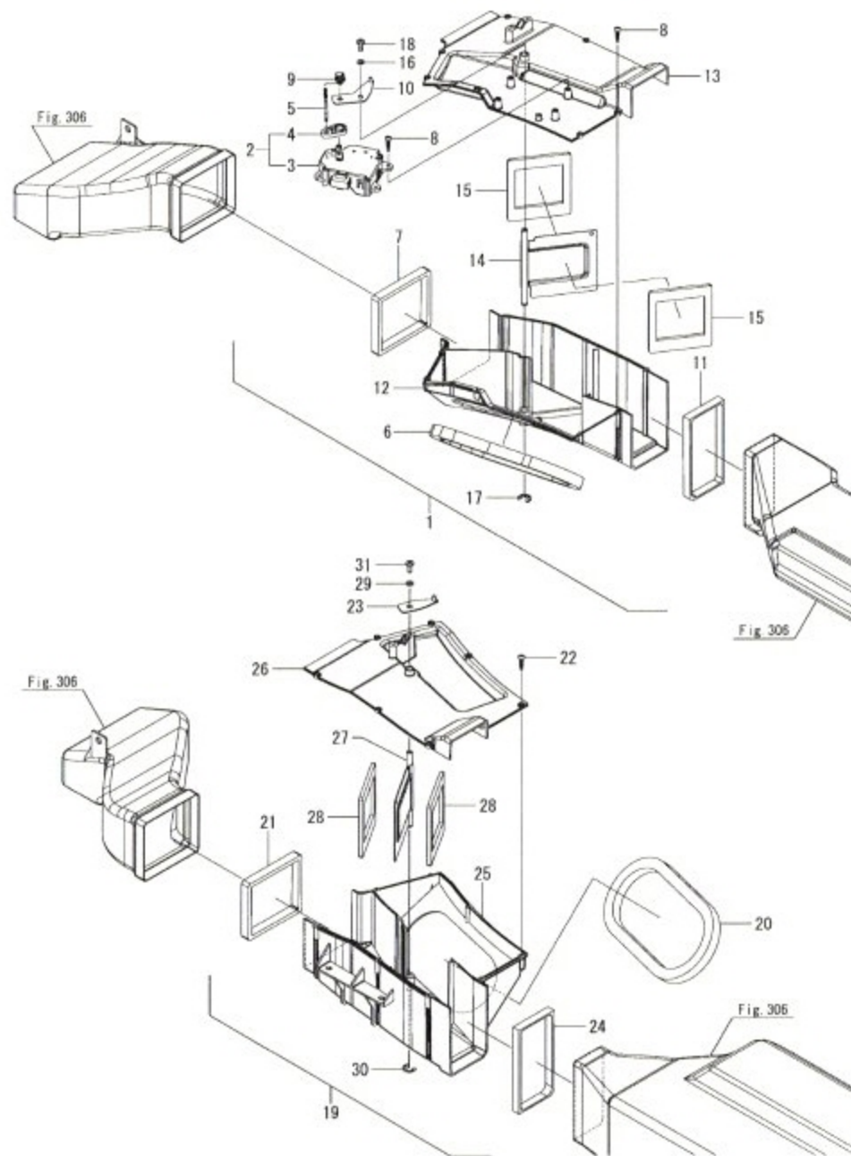
Fig.307. 에어컨 덕트(2)
