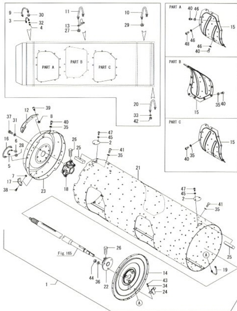
Fig.164. 탈곡통
