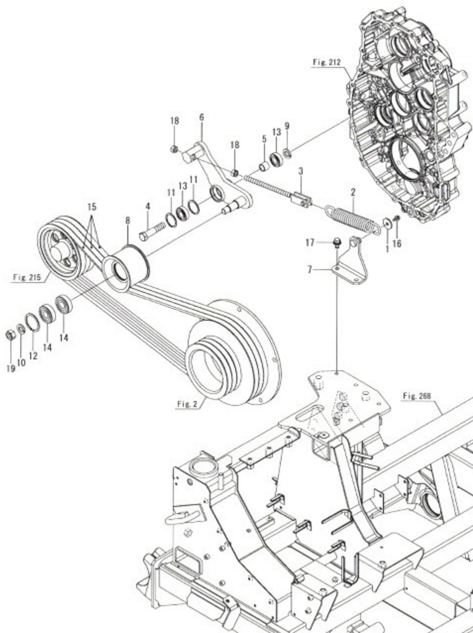
Fig.206. 주행구동
