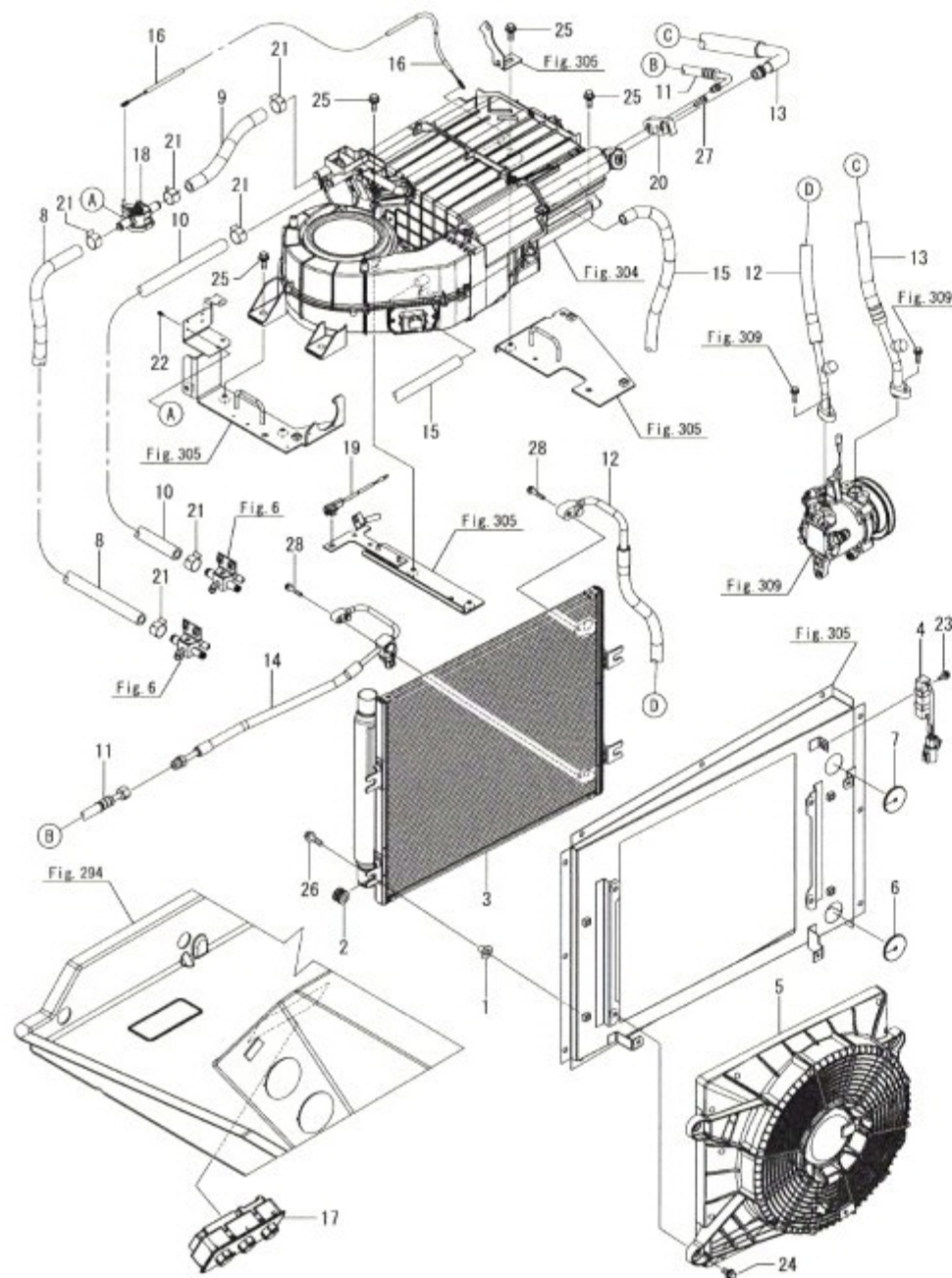
Fig.303. 에어컨(1)
