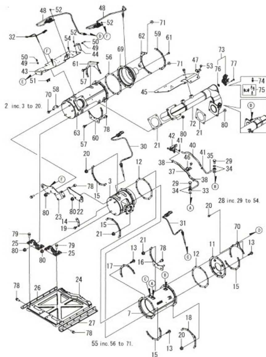
Fig.19. ATD 유닛(DPF, SCR)
