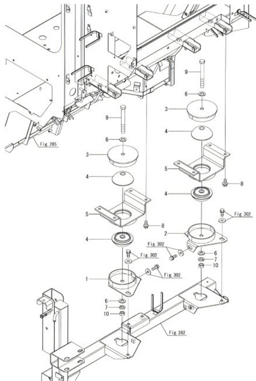
Fig.262. 발판방진(뒤)
