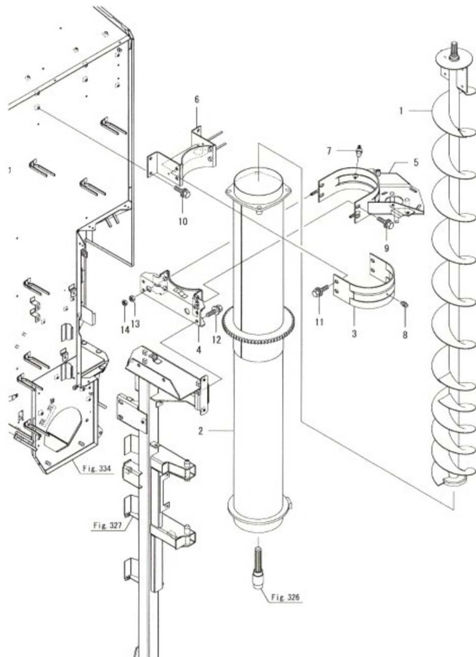
Fig.328. 중오거
