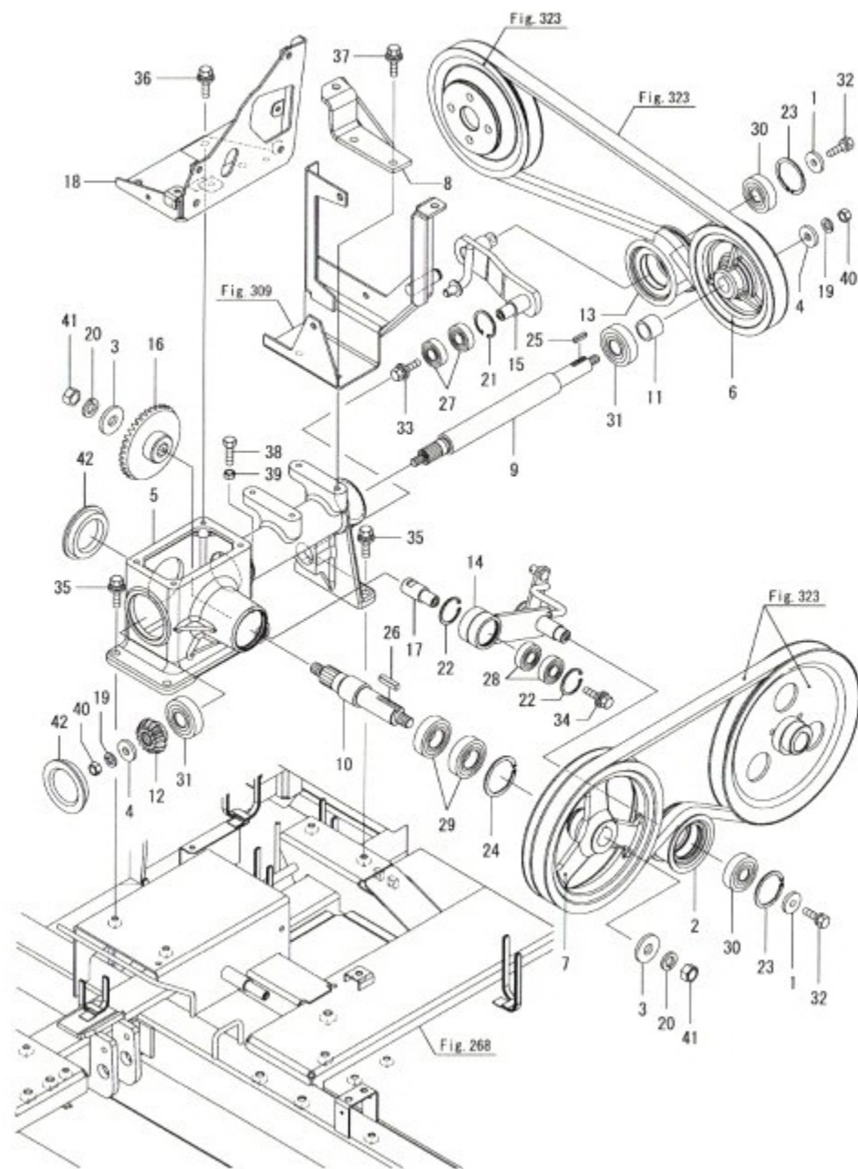
Fig.322. 오거입력
