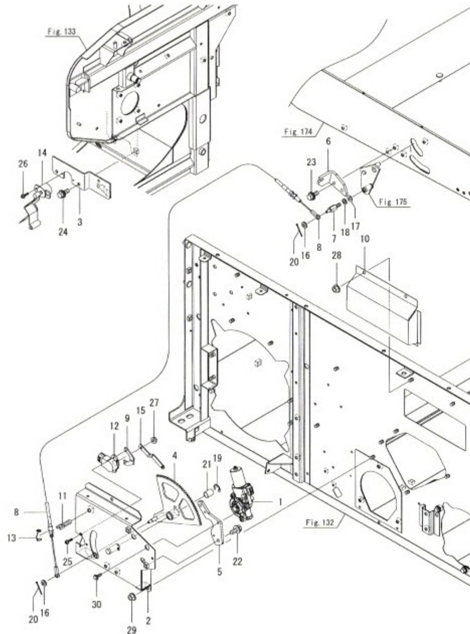
Fig.177. 요동선별조작
