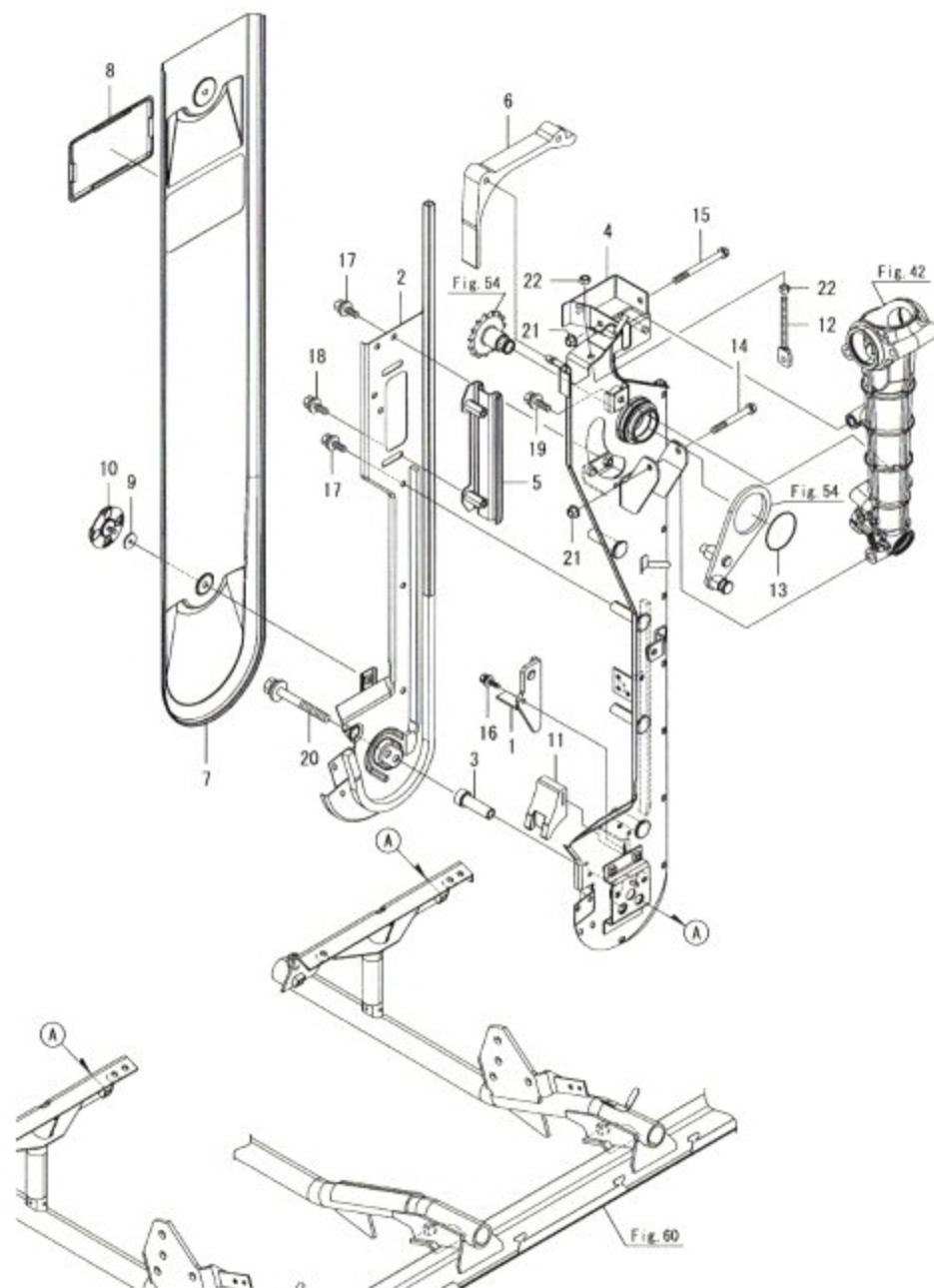
Fig.52. 인기케이스(중-좌)
