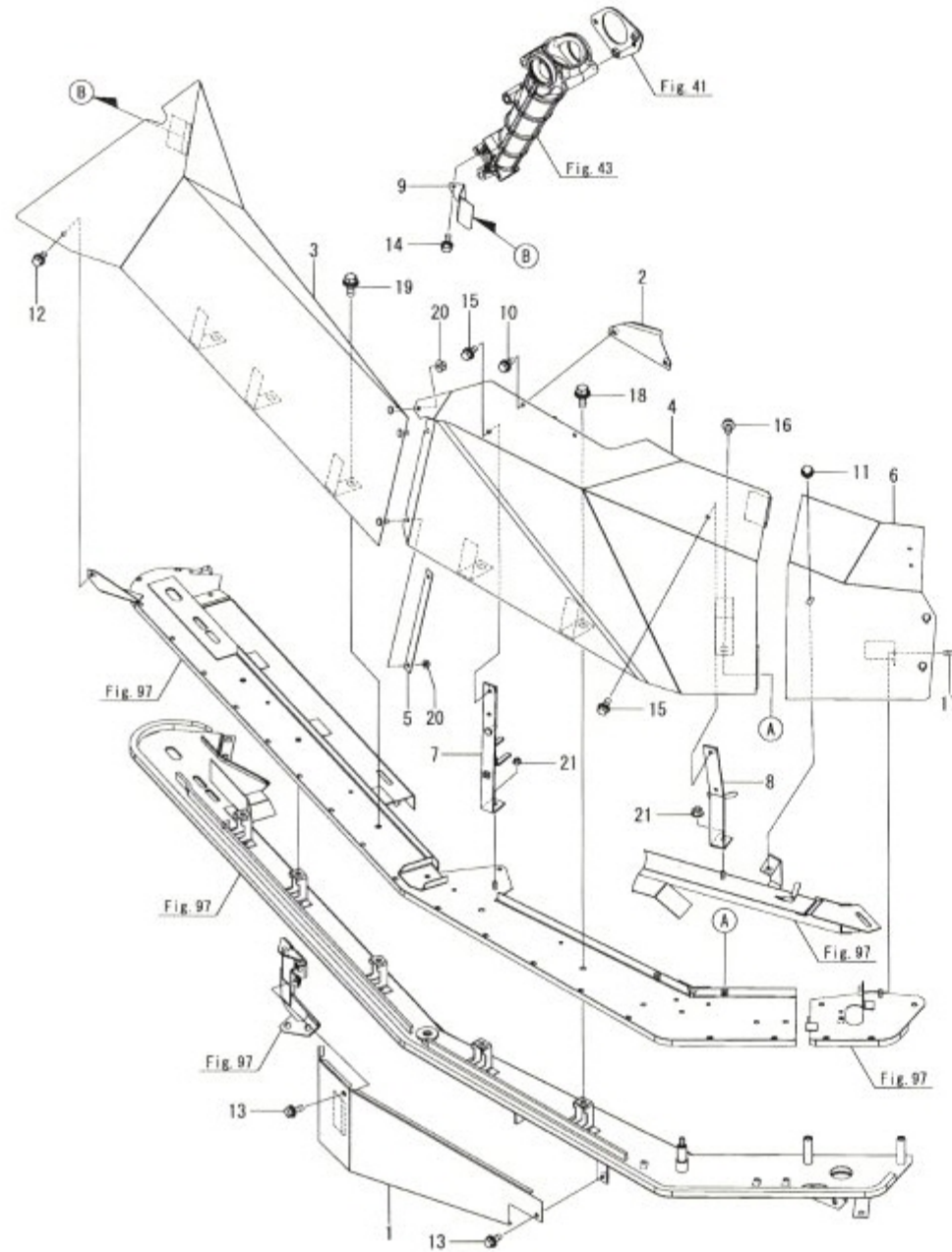
Fig.113. 상단 이송 가이드(오른쪽)
