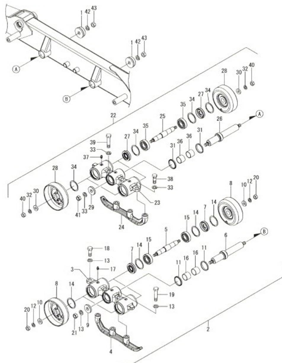
Fig.275. 이퀄라이저
