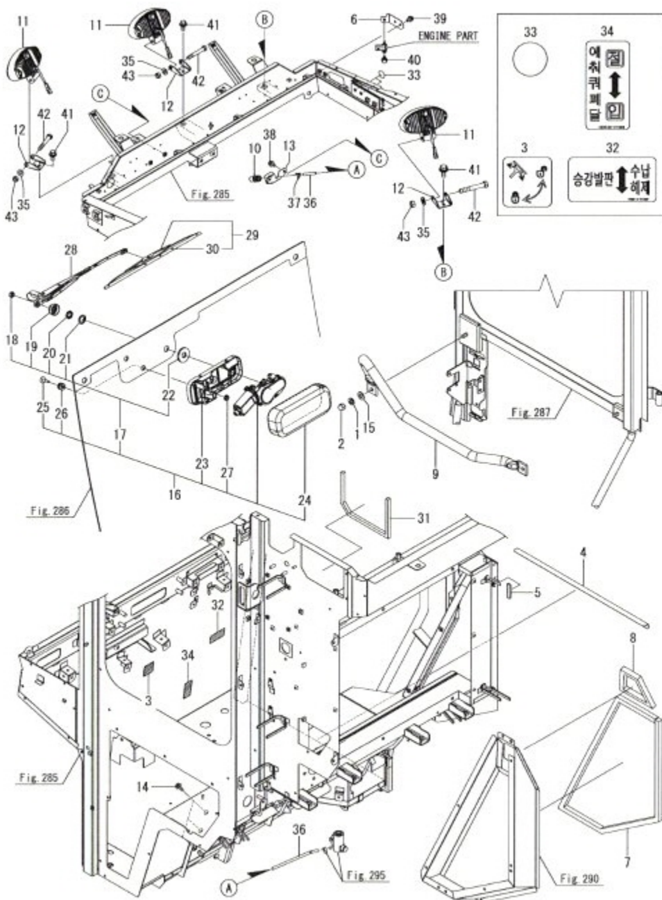
Fig.296. 캐빈 리깅
