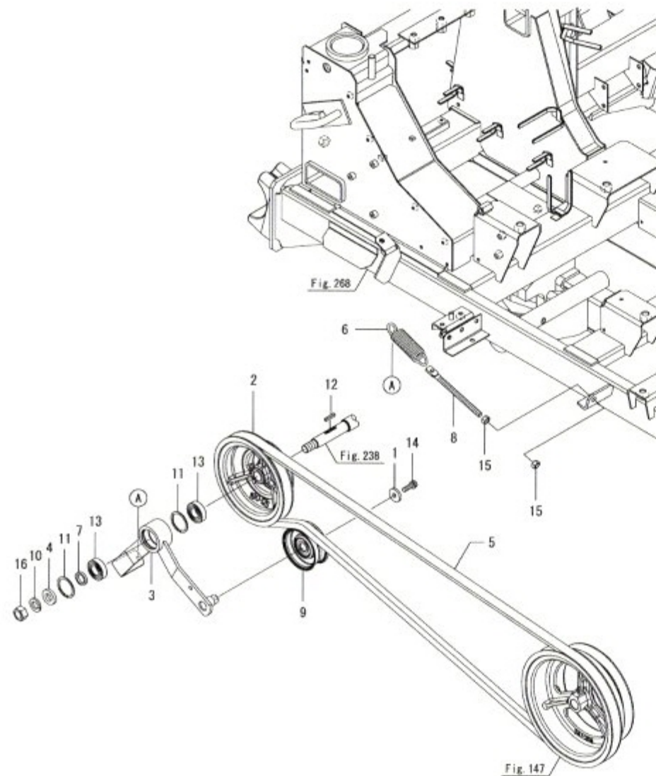
Fig.148. 카운터벨트
