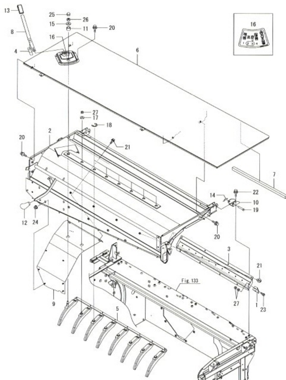
Fig.166. 탈곡실커버(1)
