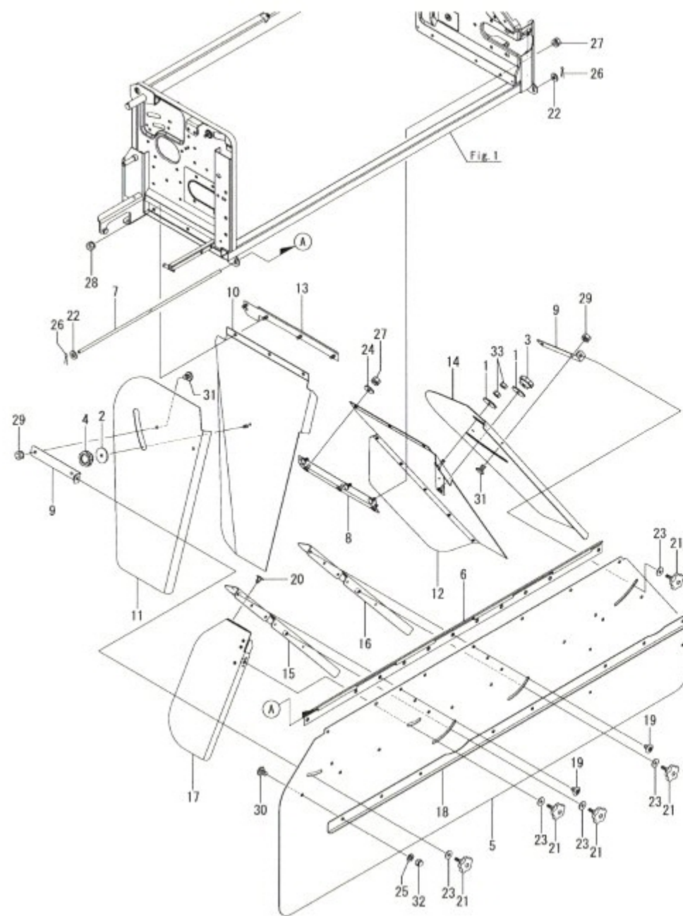
Fig.9. 하부커버
