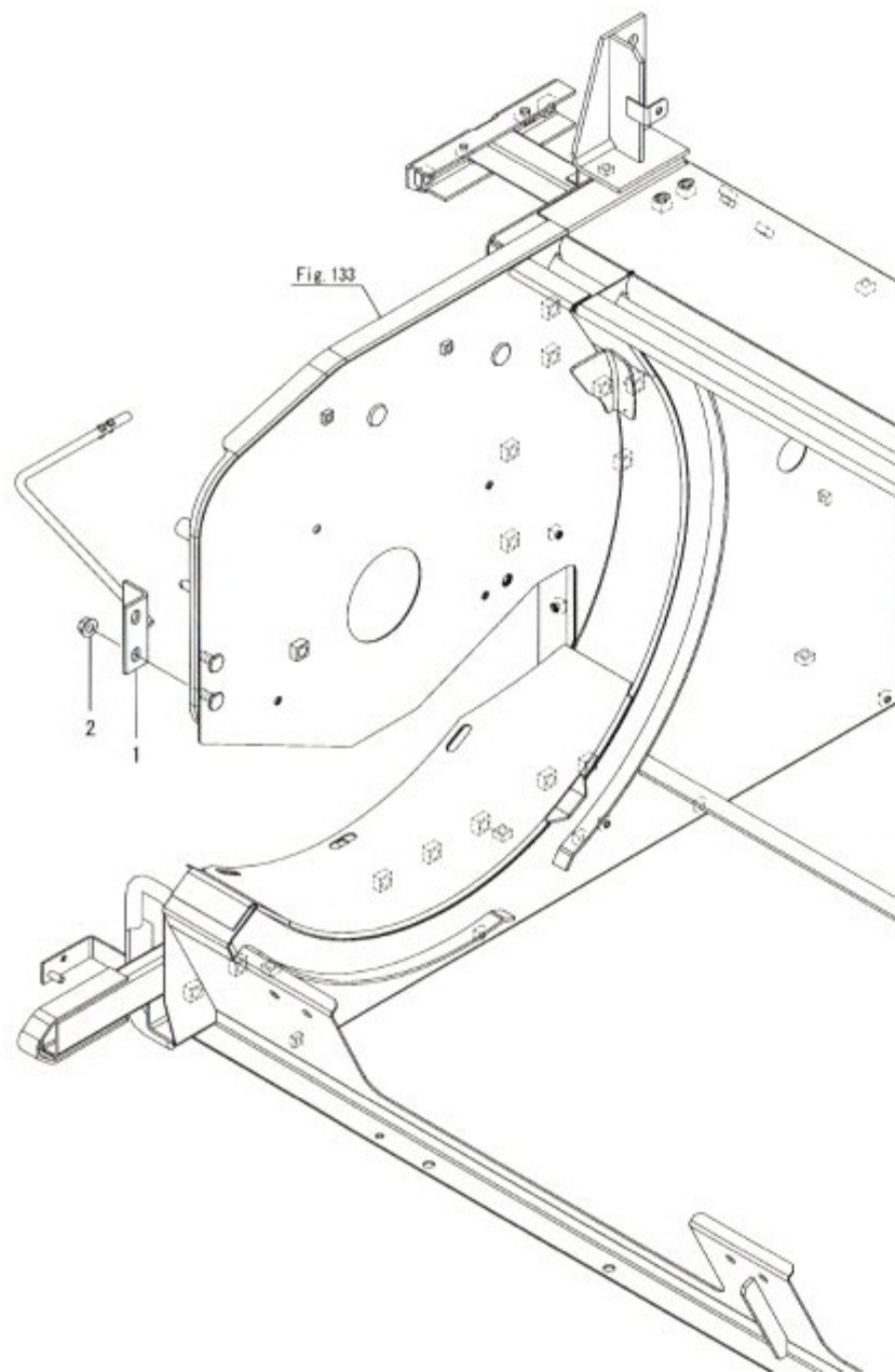
Fig.159. 탈곡통커버(앞)
