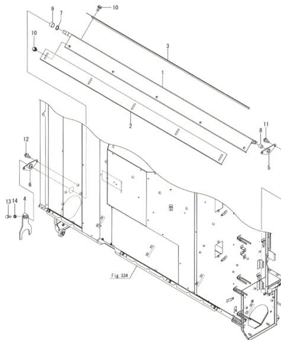
Fig.342. 요동바닥판
