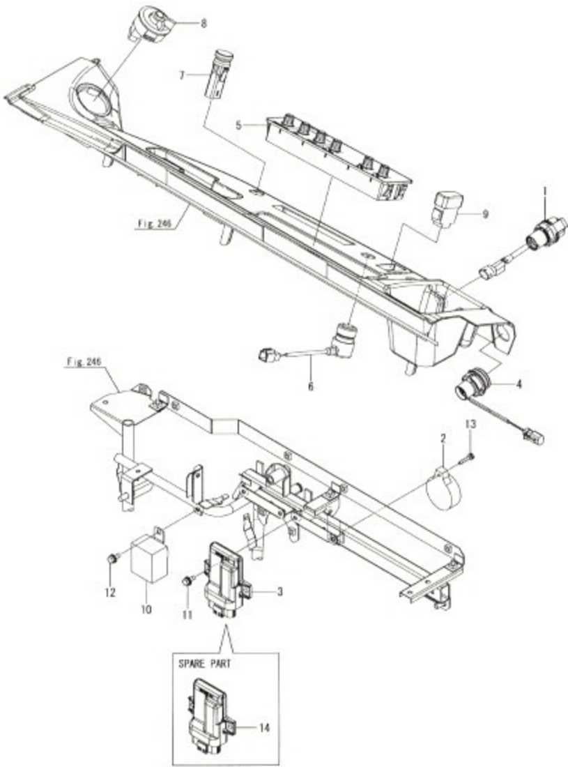
Fig.247. 사이드칼럼(2)
