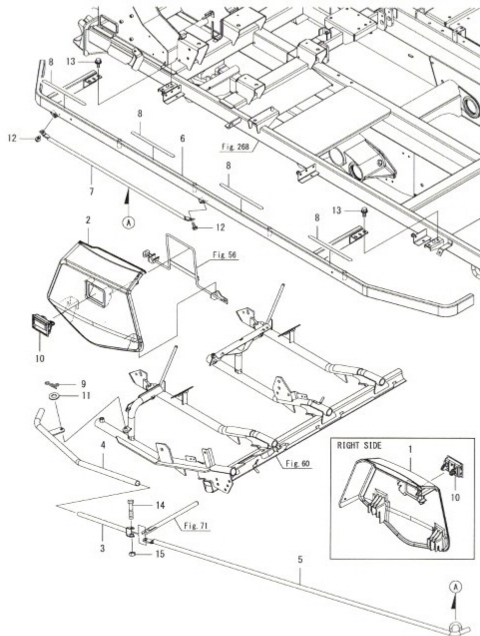
Fig.16. 예취(2)
