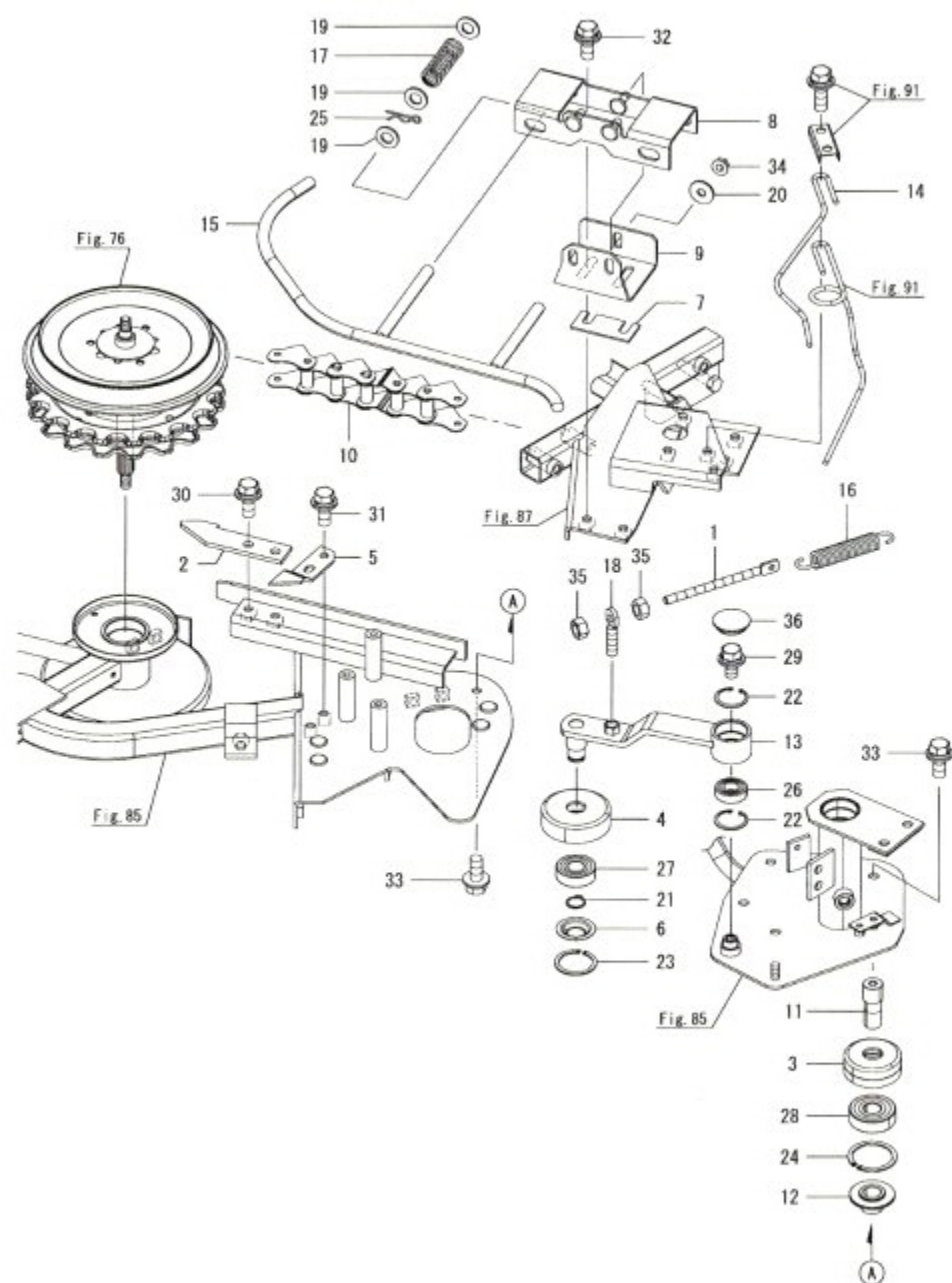
Fig.95. 하부반송가이드(중-좌)
