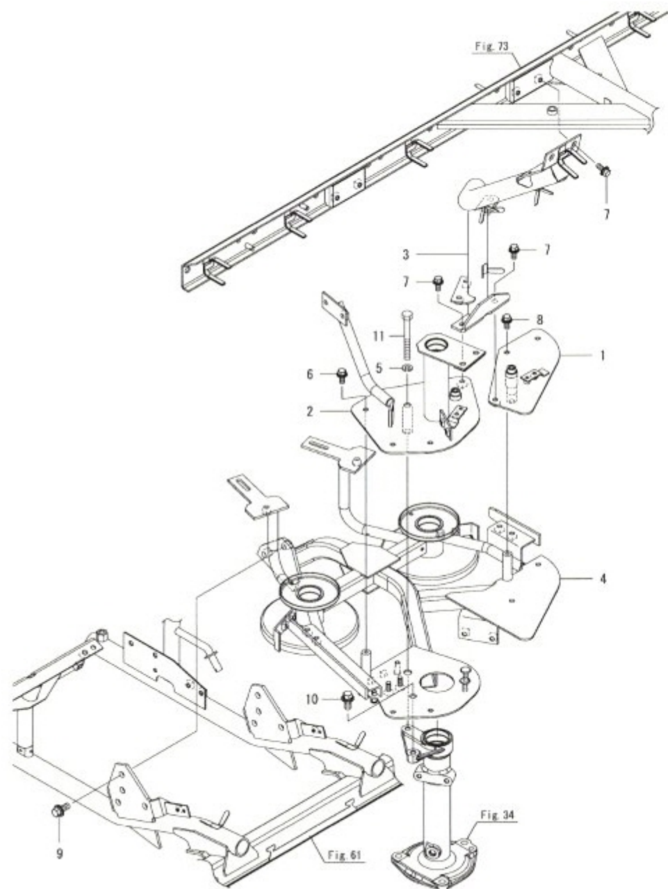
Fig.88. 끌어모음프레임(중-우)
