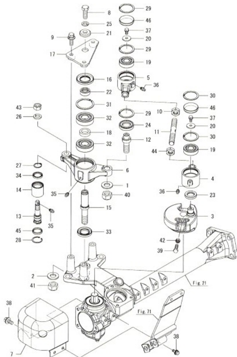
Fig.62. 예취날구동(좌)
