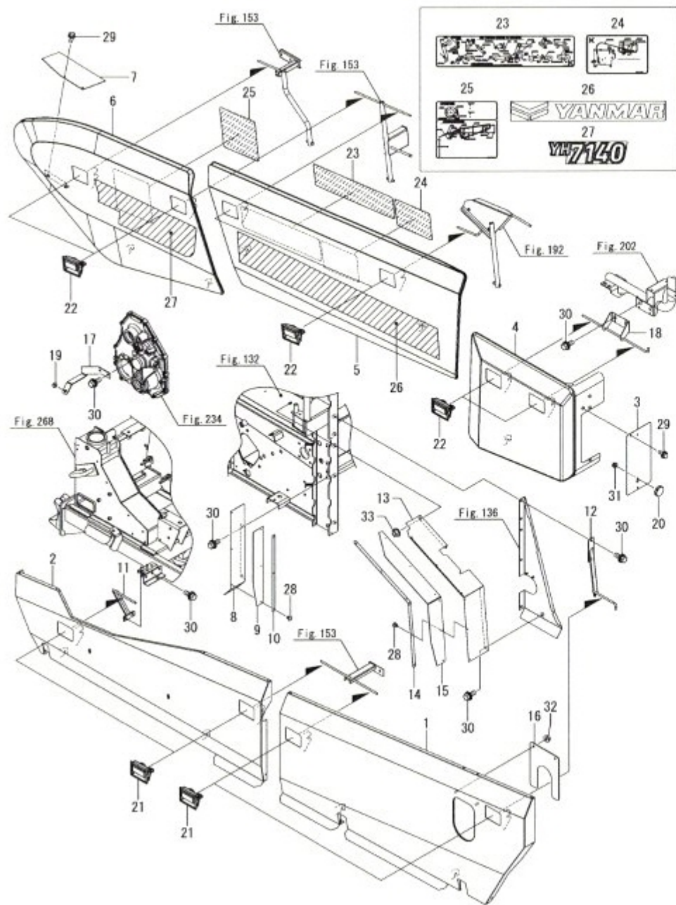
Fig.155. 탈곡 커버(측면)
