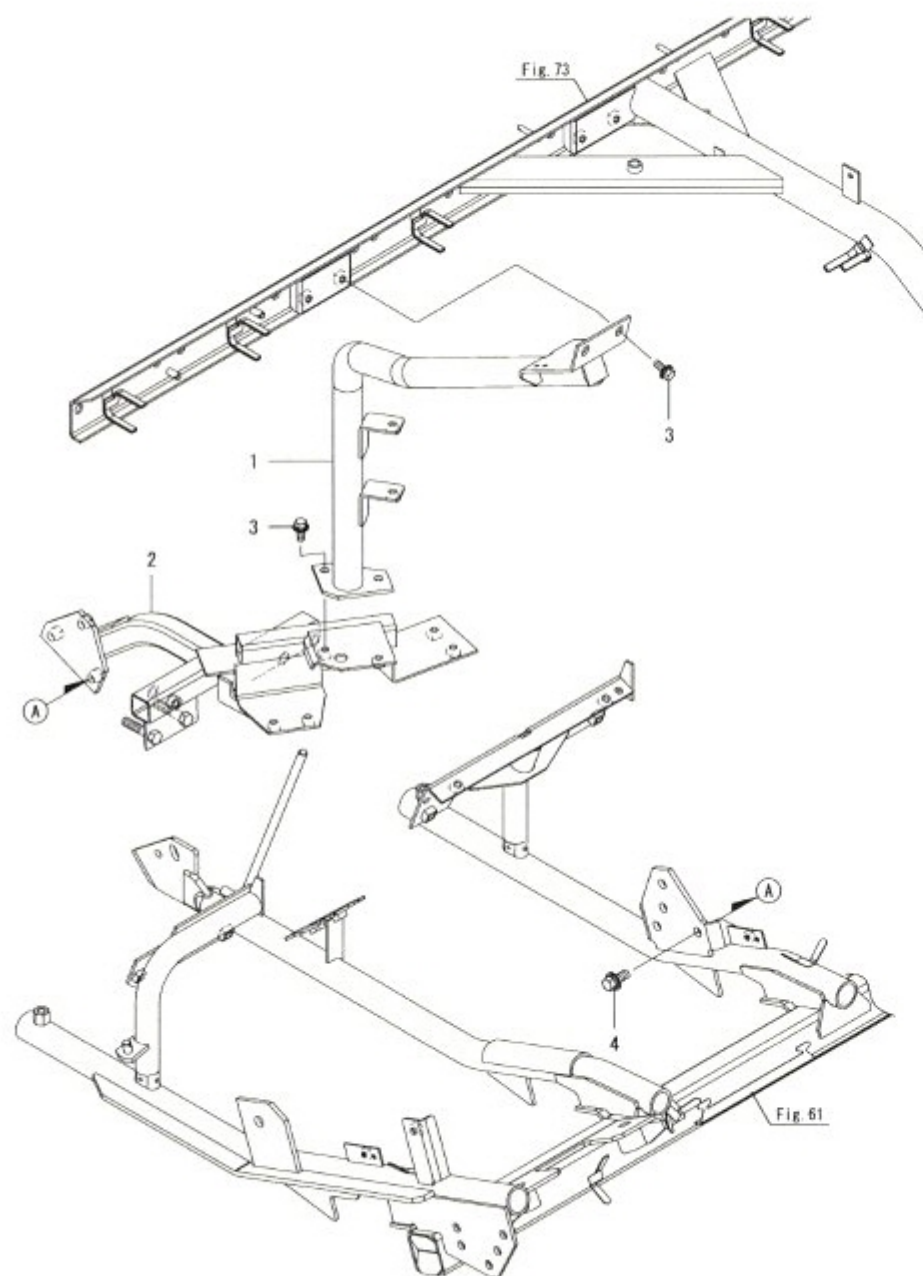
Fig.86. 끌어모음프레임(중-좌)
