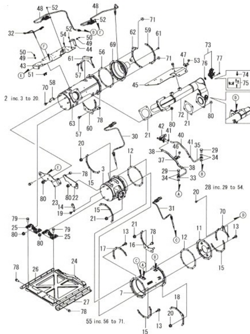
Fig.19. ATD 유닛(DPF, SCR)
