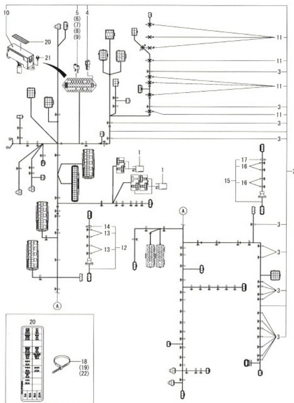
Fig.318. 배선(탈곡)
