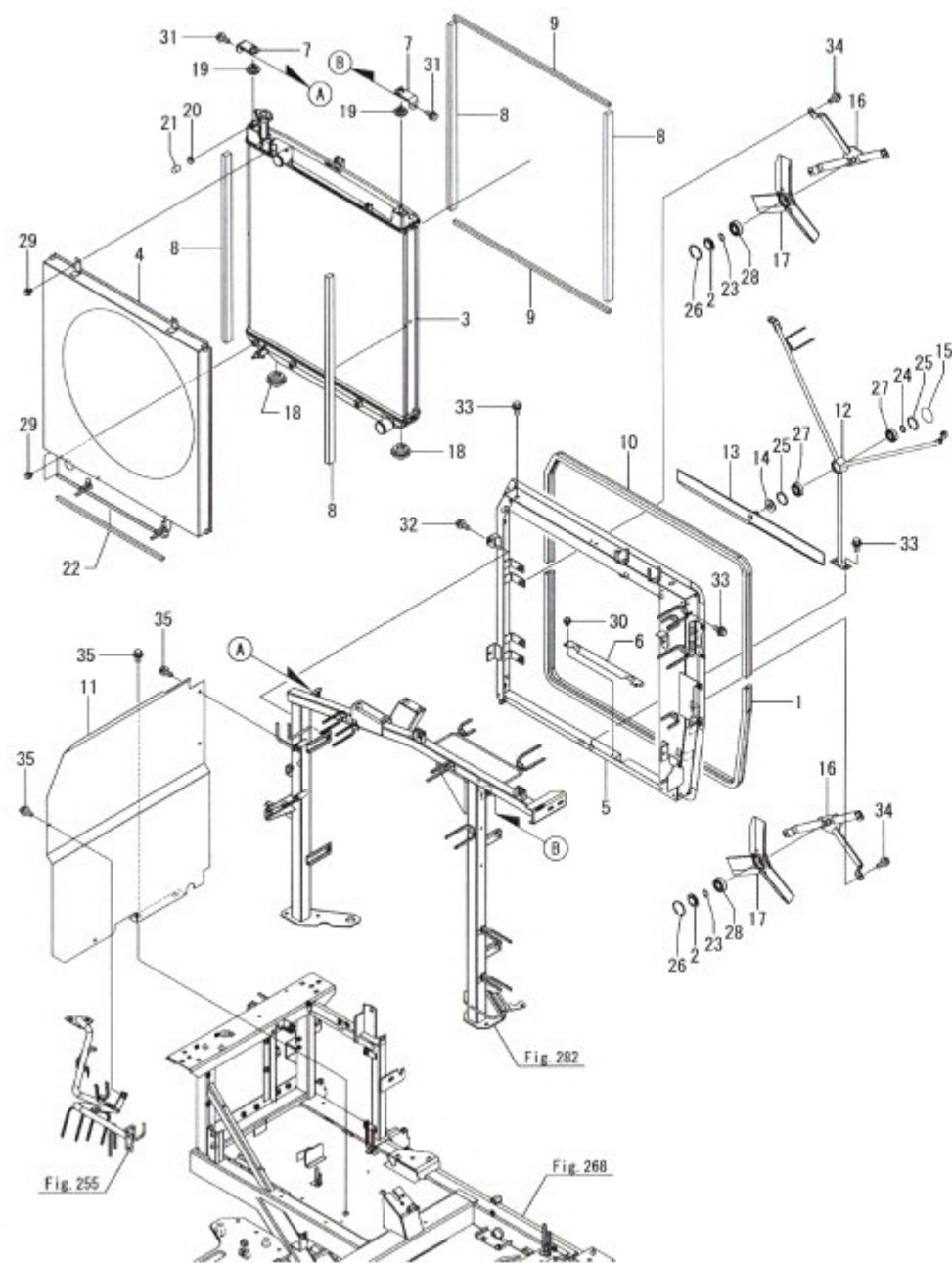
Fig.11. 라디에이터(1)
