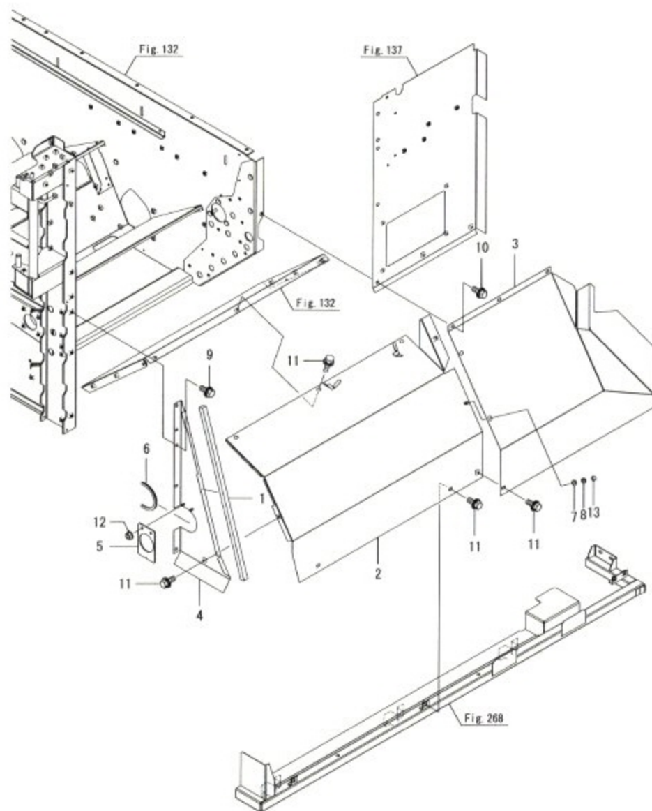
Fig.136. 상부본체(뒤)
