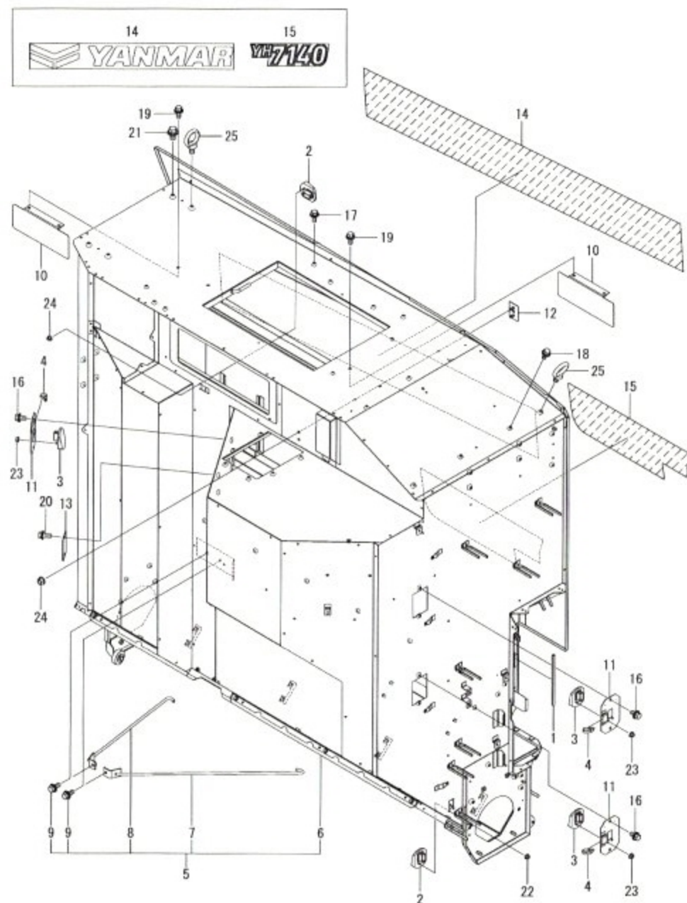
Fig.336. 곡물탱크(1)
