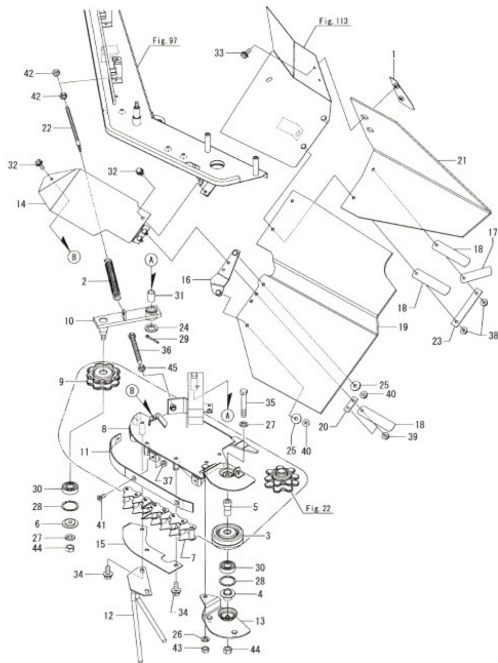
Fig.125. 보조반송케이스
