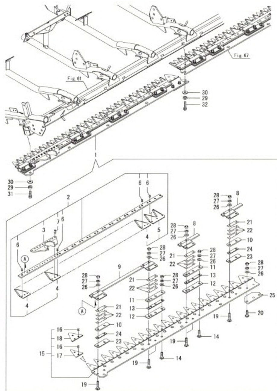
Fig.66. 예취날(좌)
