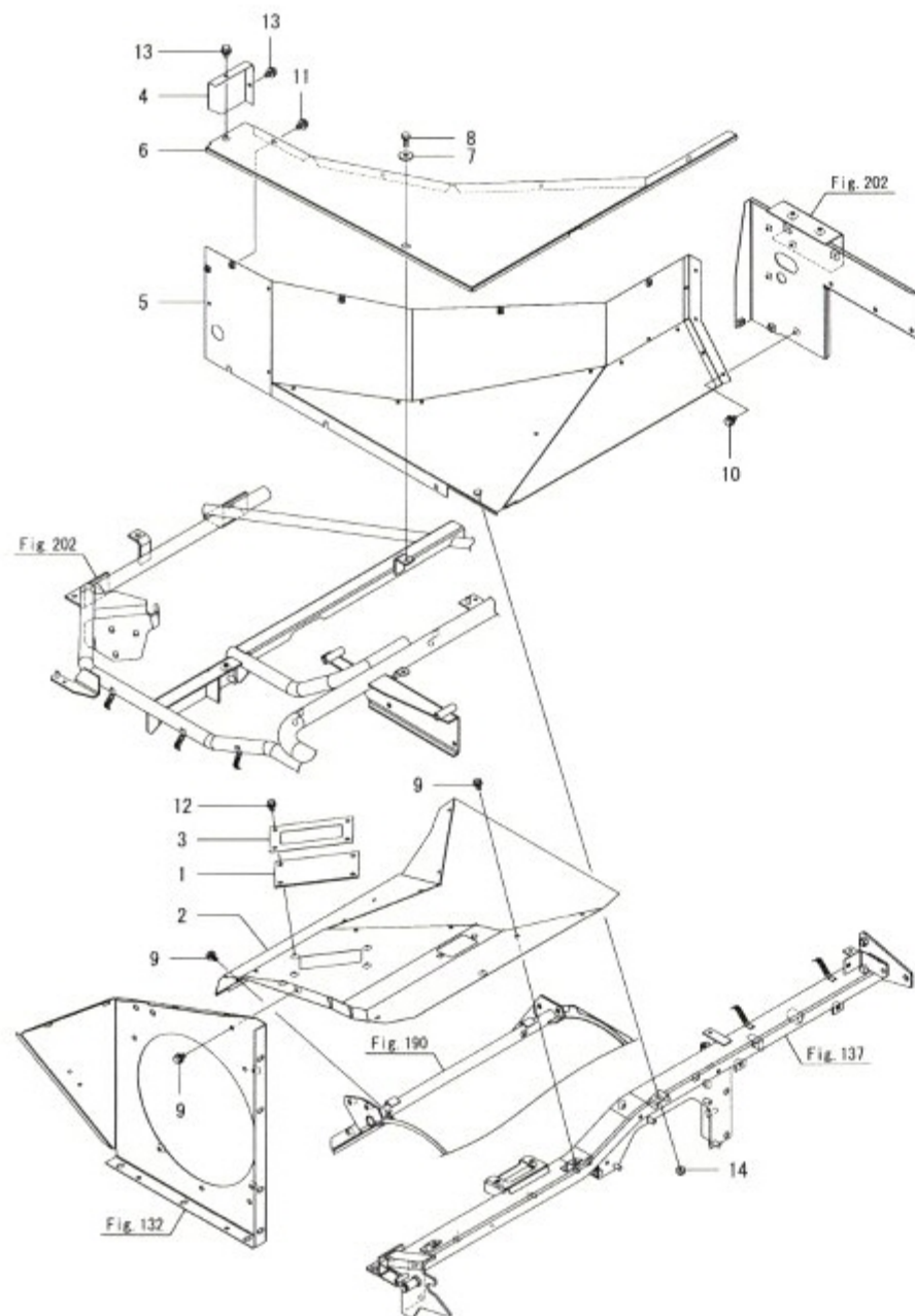
Fig.135. 상부분체(출구)
