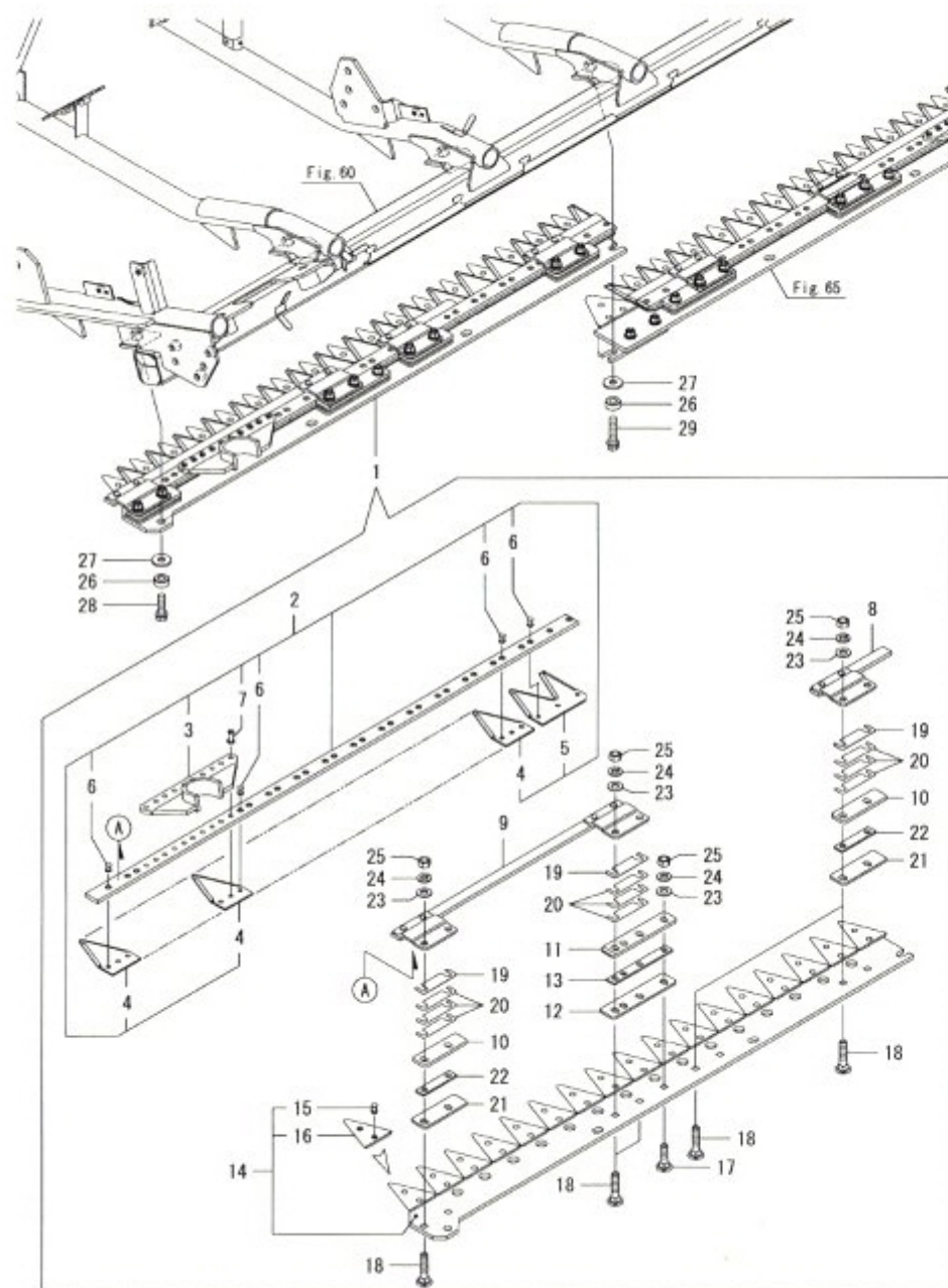
Fig.64. 예취날(좌)
