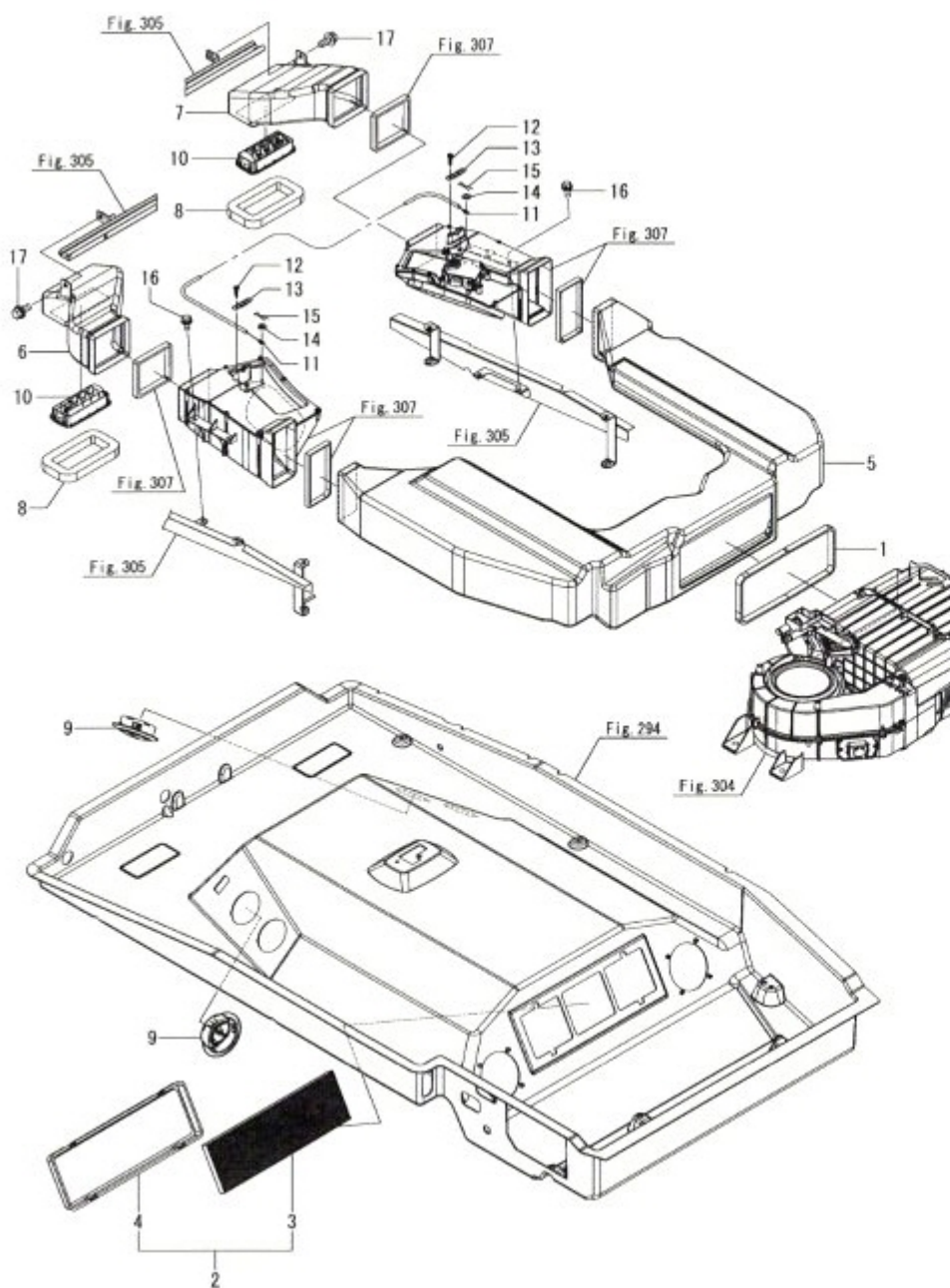
Fig.306. 에어컨 덕트(1)
