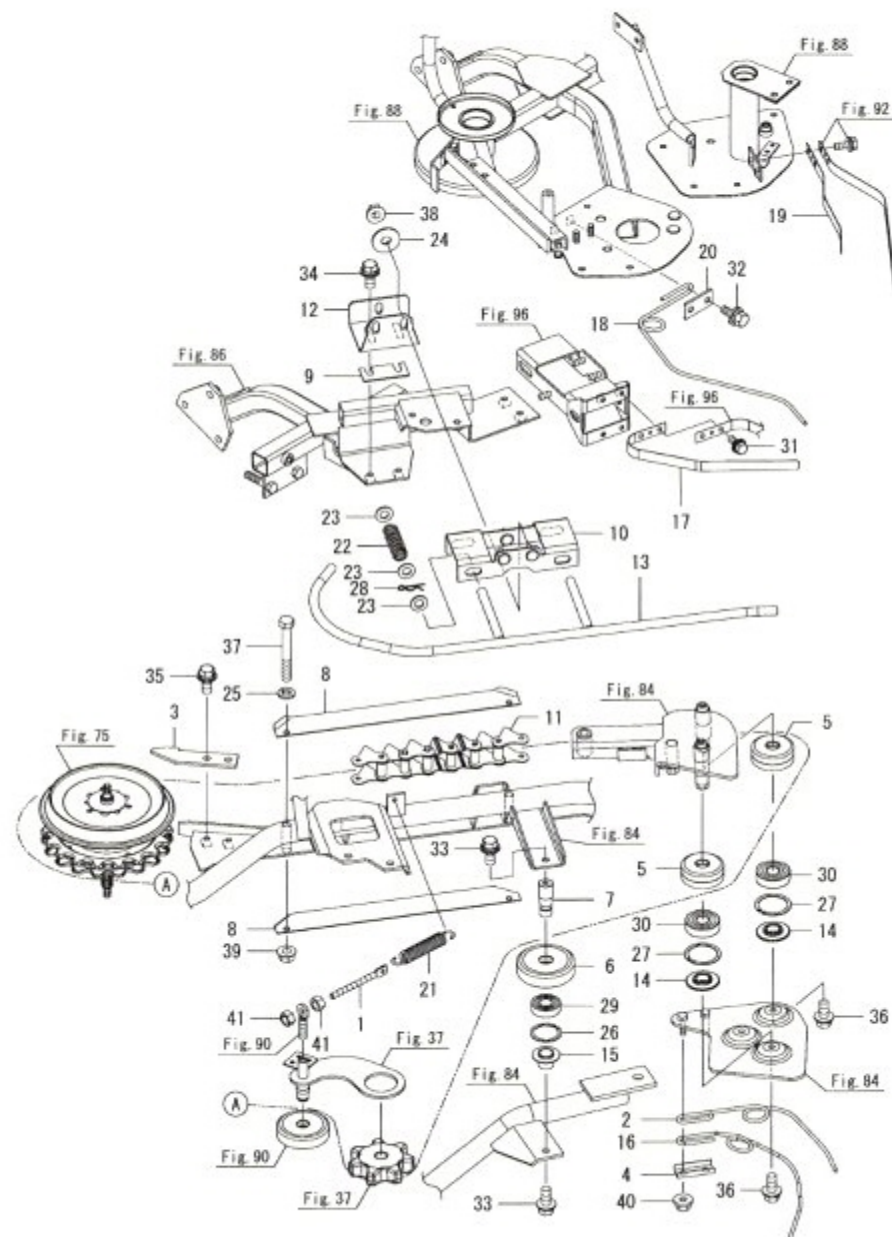
Fig.94. 하단 이송 가이드(왼쪽)
