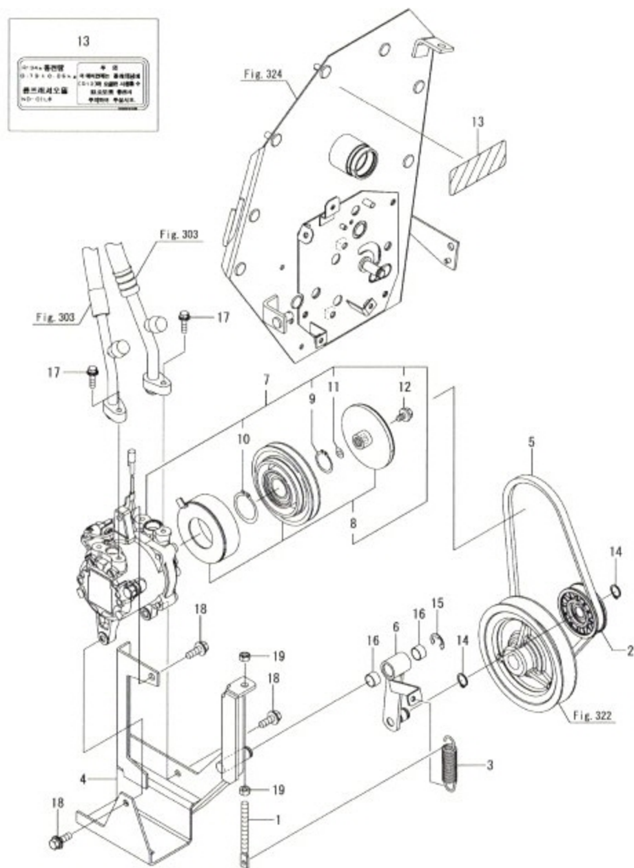
Fig.309. 콤프레셔취부
