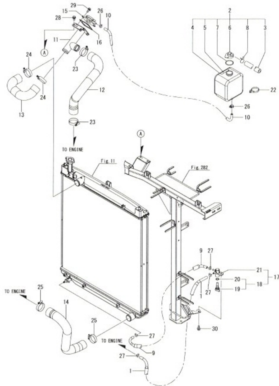
Fig.12. 라디에이터(2)
