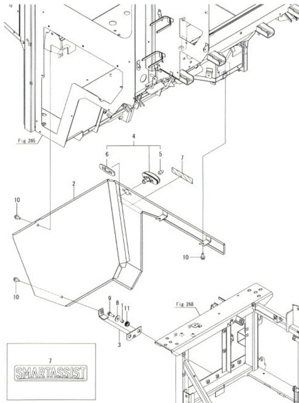
Fig.261. 발판
