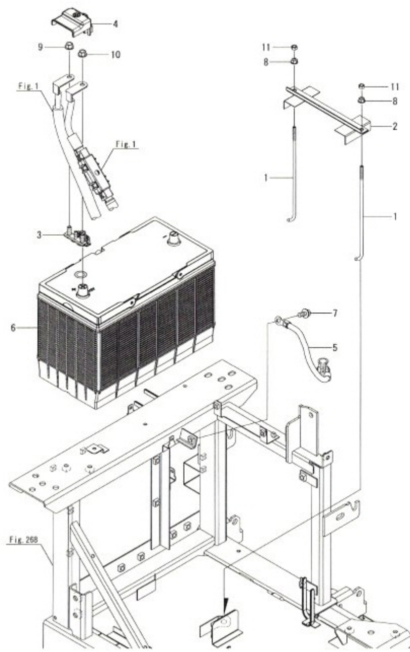
Fig.311. 배터리
