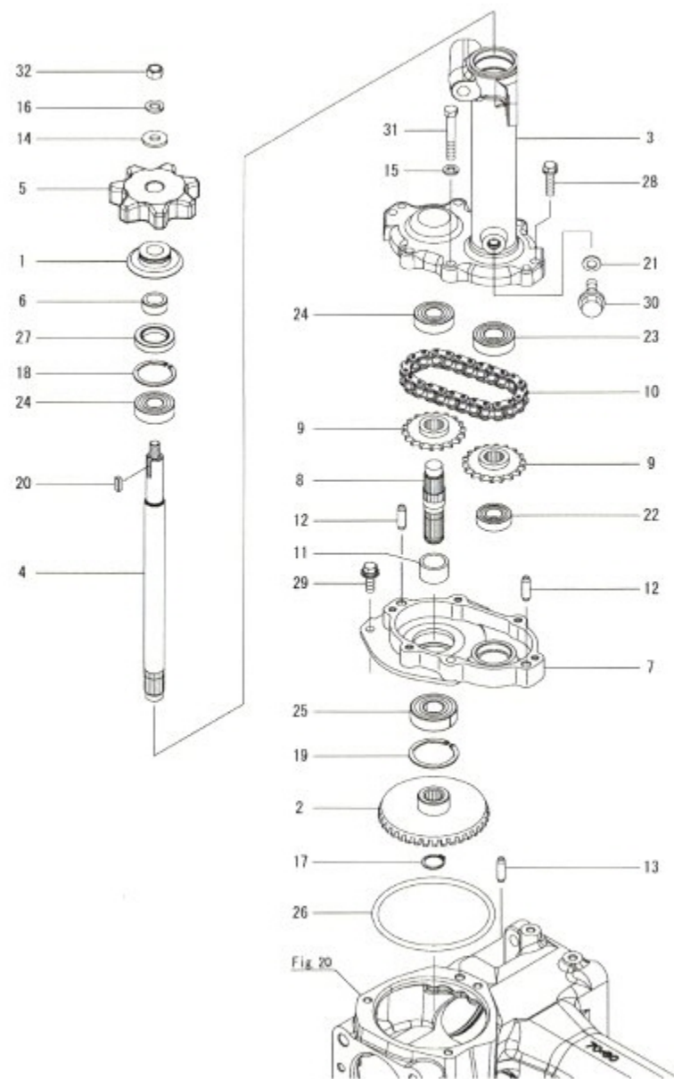
Fig.24. 6조구동케이스(6)
