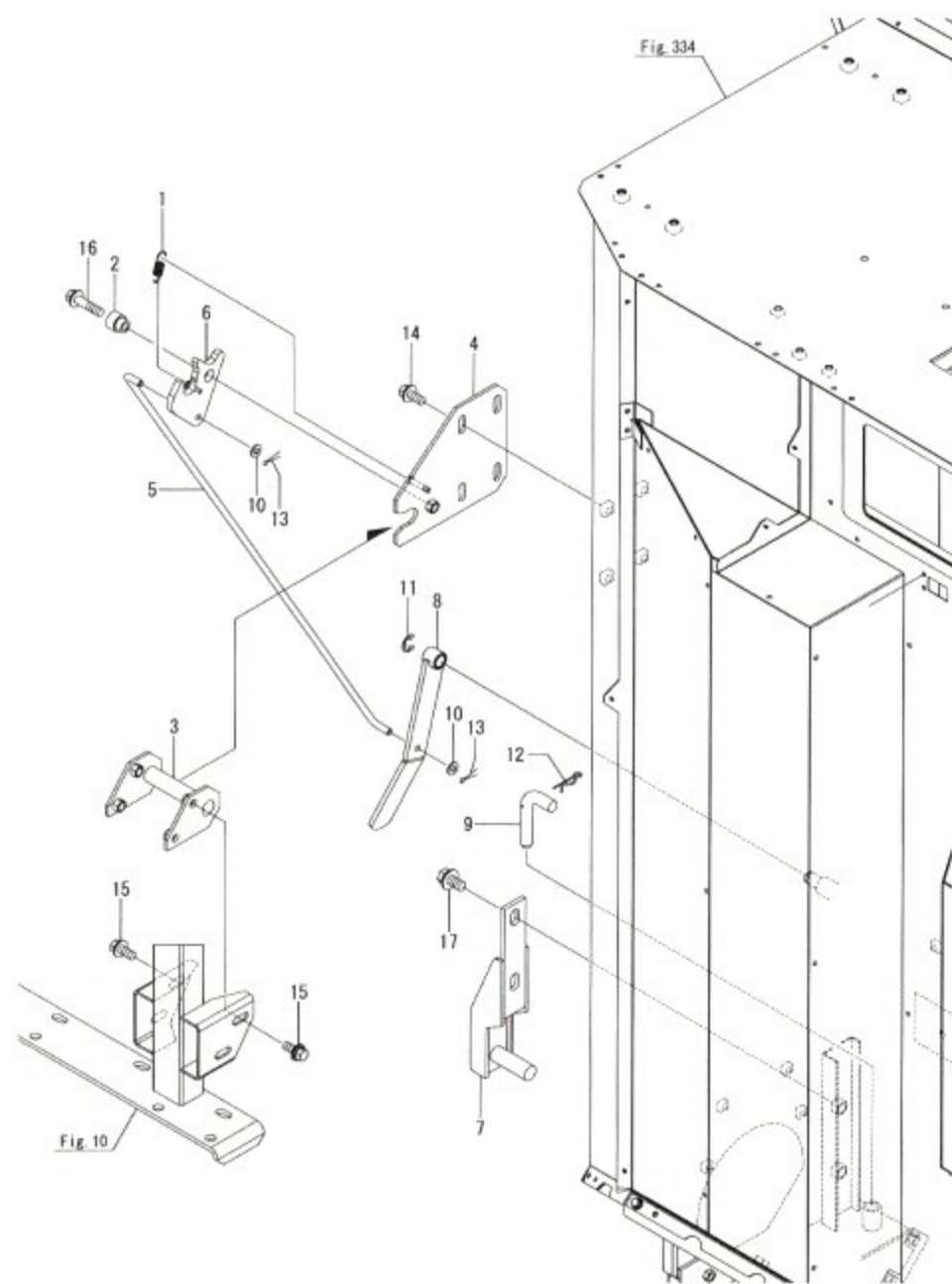
Fig.338. 탱크 고정
