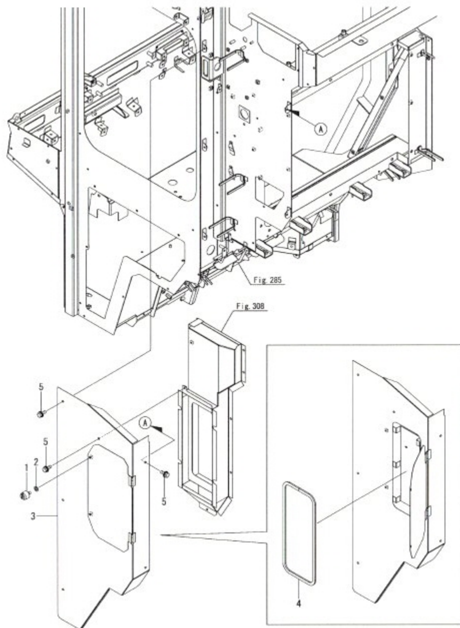
Fig.300. 캐빈시일(2)
