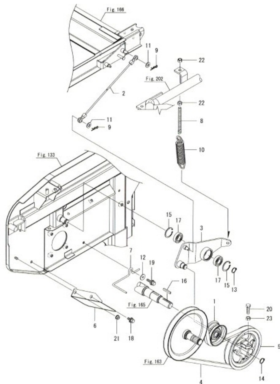
Fig.158. 짚 방출 벨트
