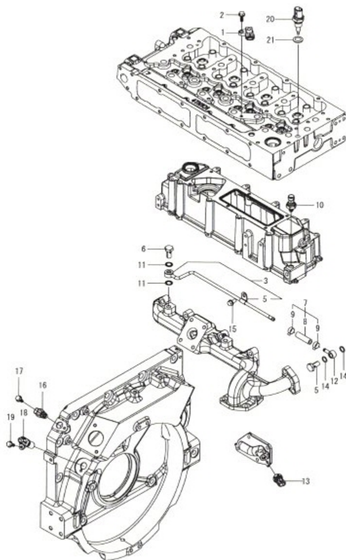
Fig.32. 센서
