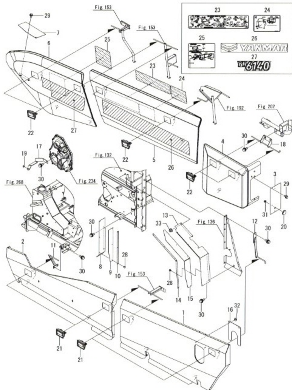
Fig.154. 탈곡 커버(측면)
