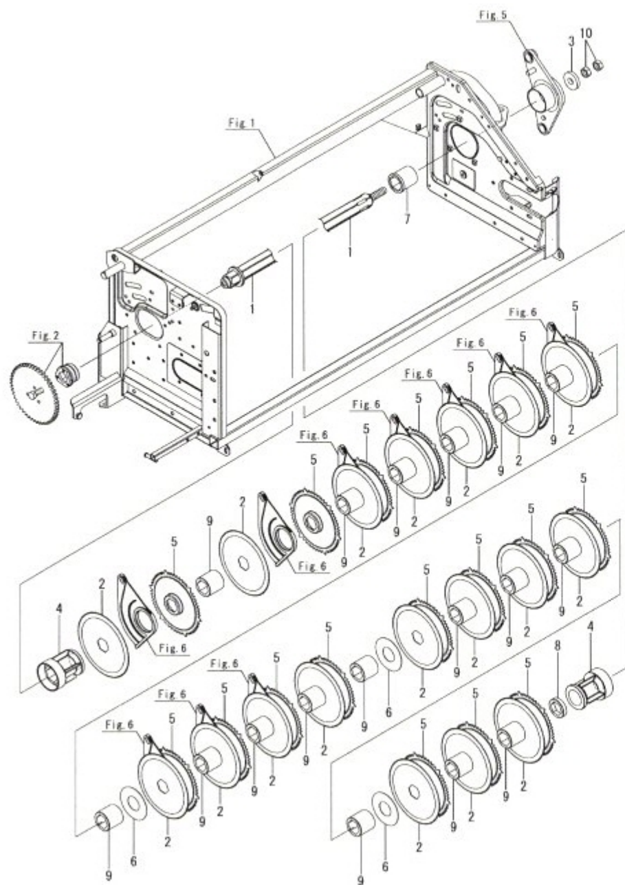
Fig.3. 축(저속)
