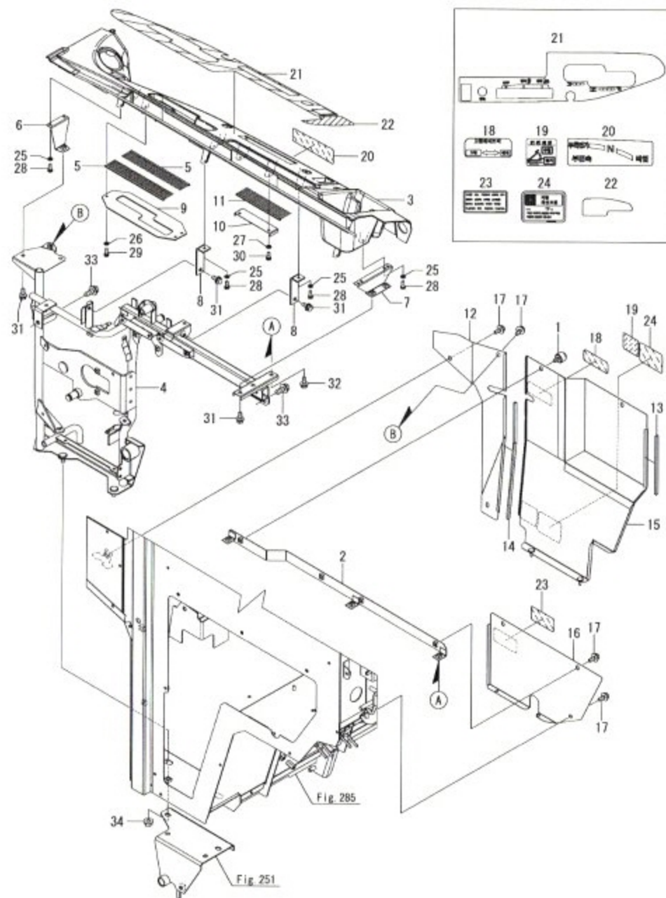
Fig.246. 사이드칼럼(1)
