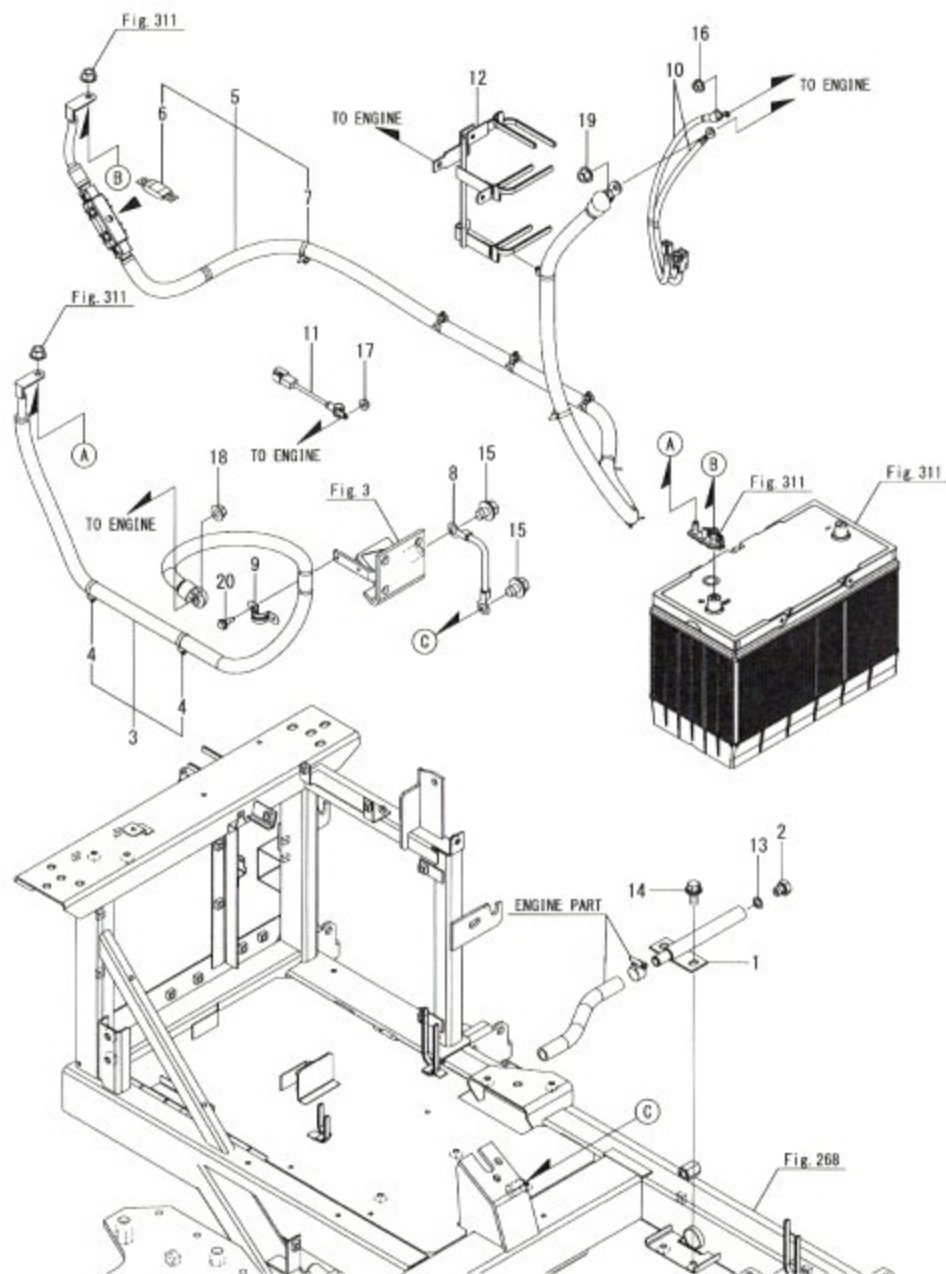
Fig.1. 엔진관련
