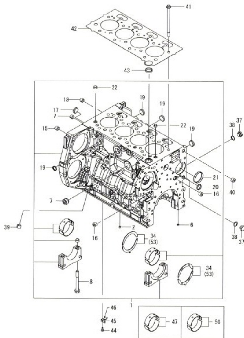
Fig.1. 실린더블럭
