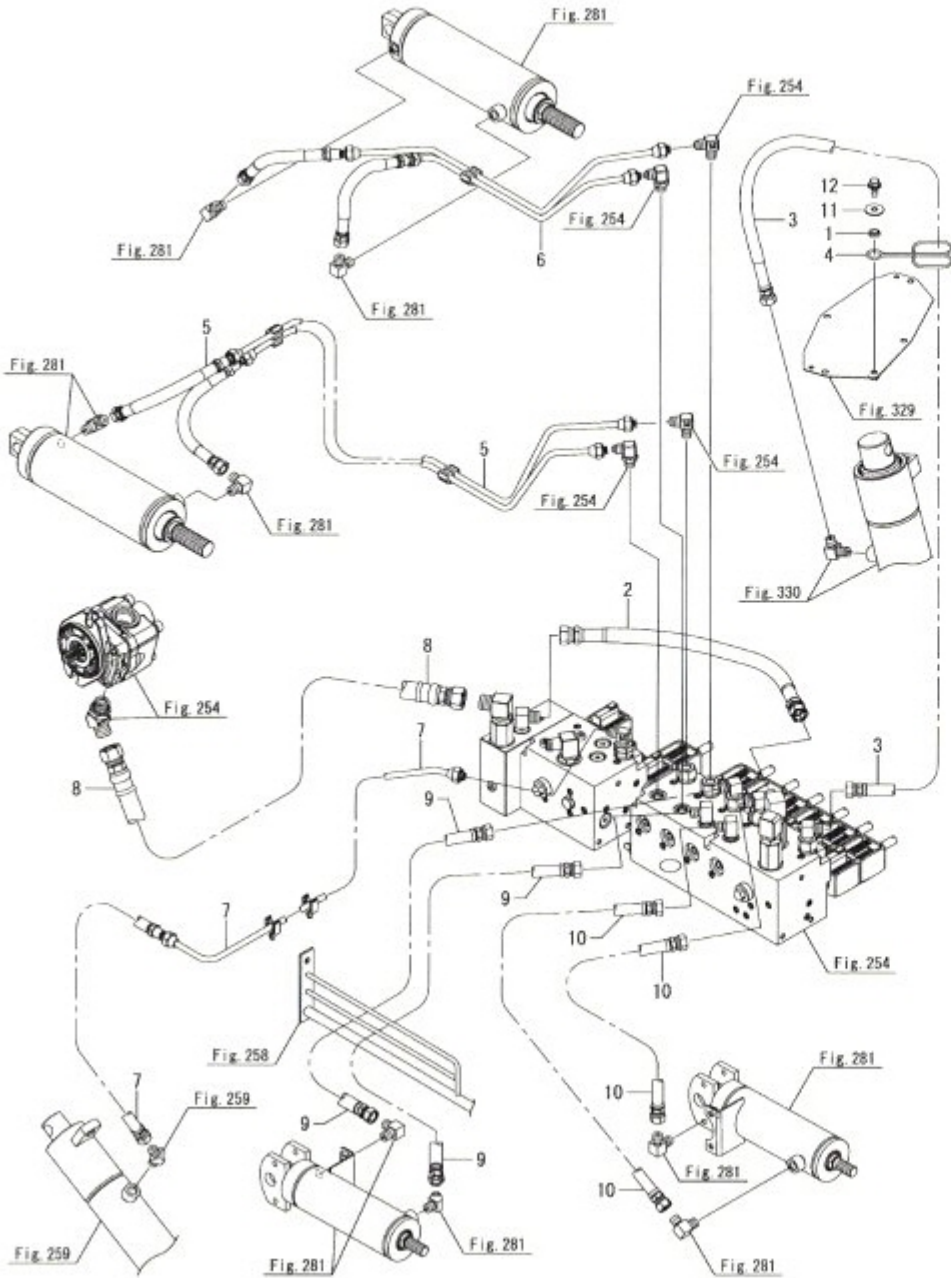
Fig.257. 배관(1)
