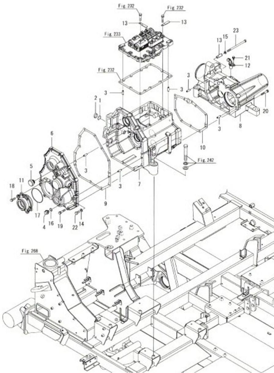
Fig.234. 카운터케이스(3)
