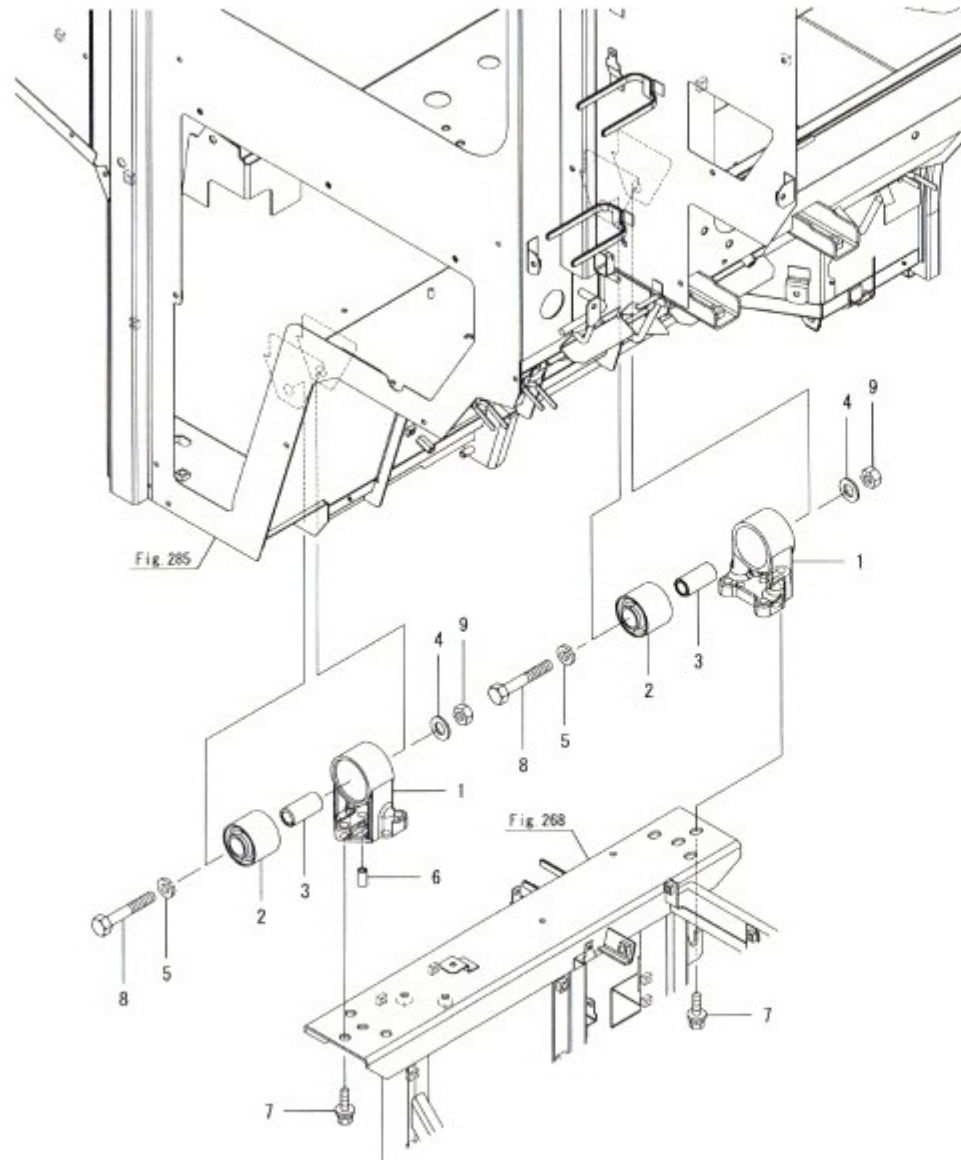
Fig.263. 발판방진(앞)
