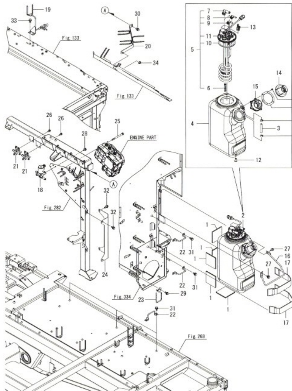
Fig.6. 요소 탱크(1)
