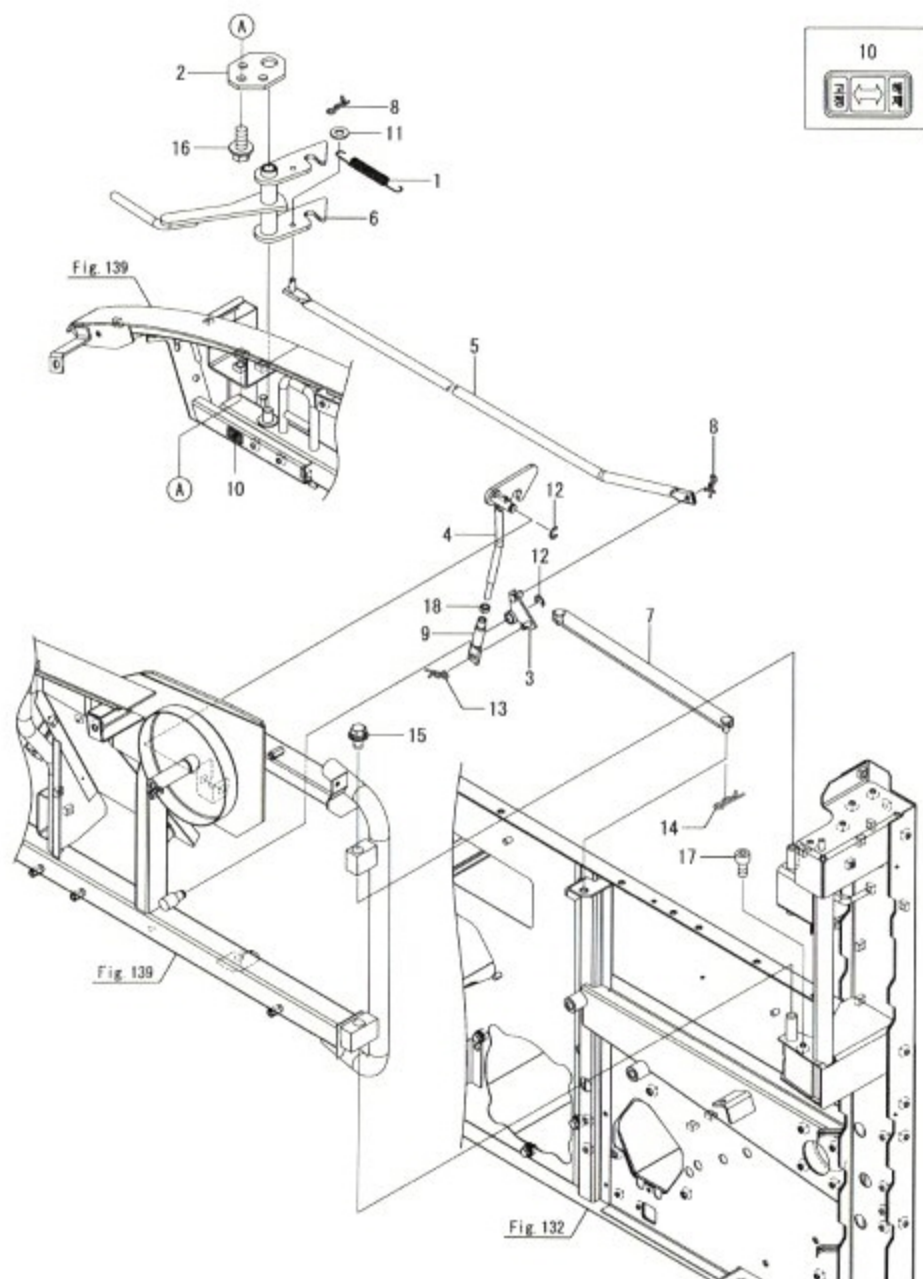
Fig.140. 탈곡실프레임(좌)(2)
