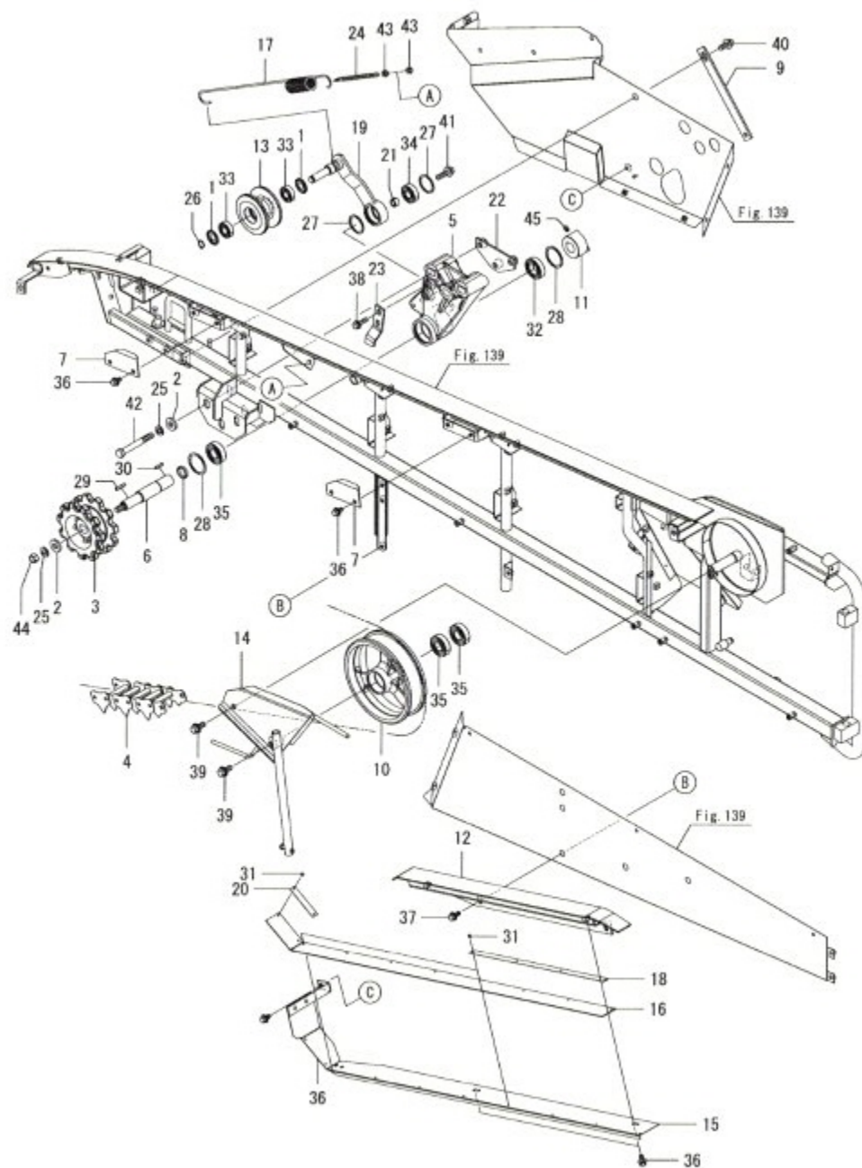
Fig.192. 피드체인
