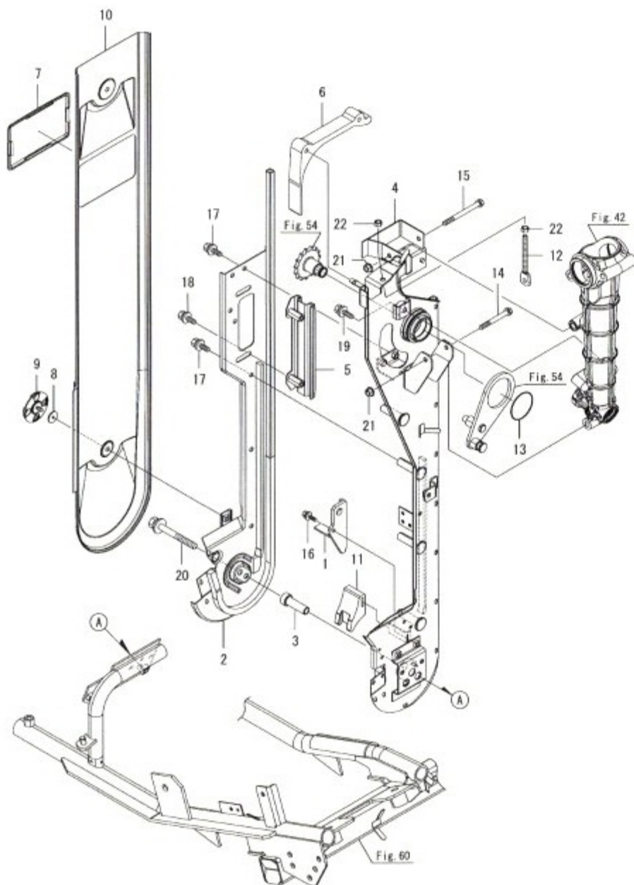
Fig.50. 픽업 케이스(왼쪽)
