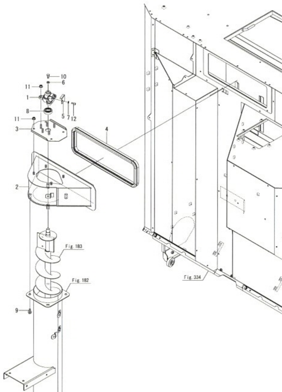
Fig.184. 양곡투입구
