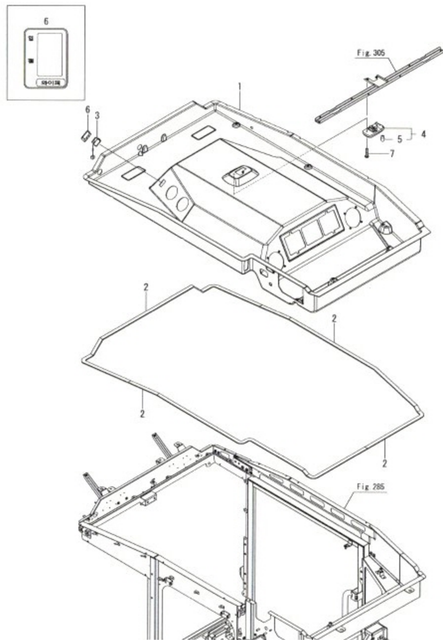
Fig.294. 캐빈(천장)
