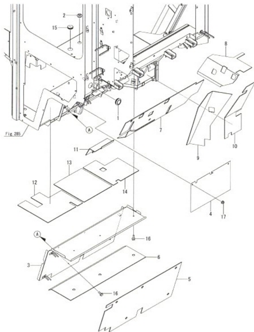
Fig.291. 캐빈 프레임(7)
