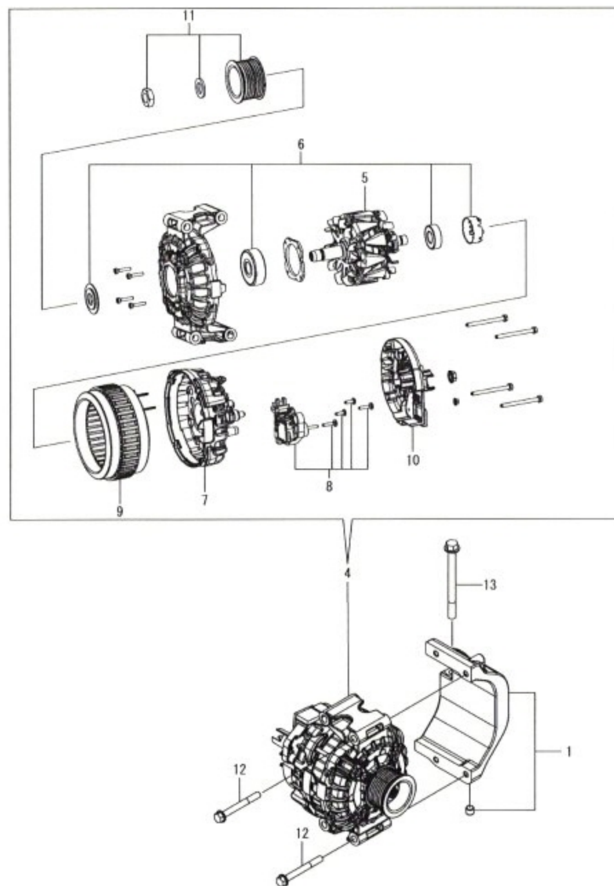
Fig.29. 발전기
