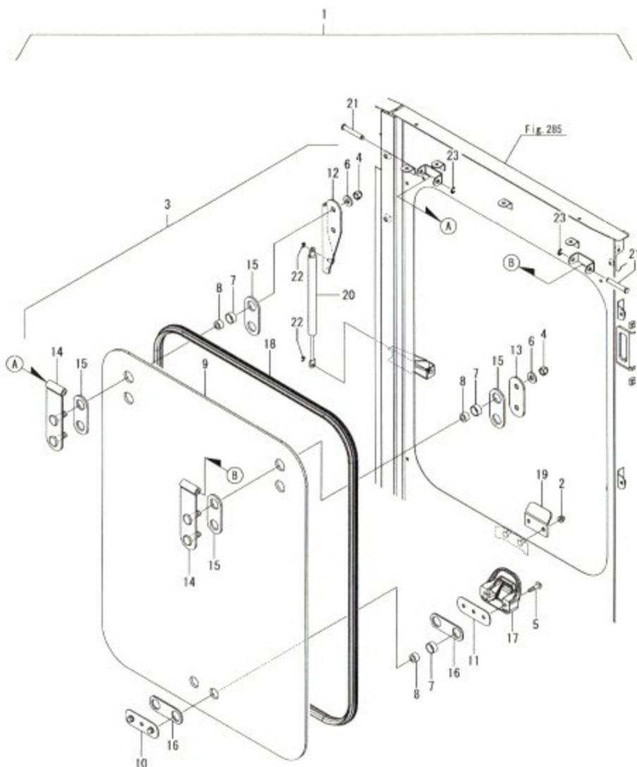
Fig.289. 캐빈 프레임(5)
