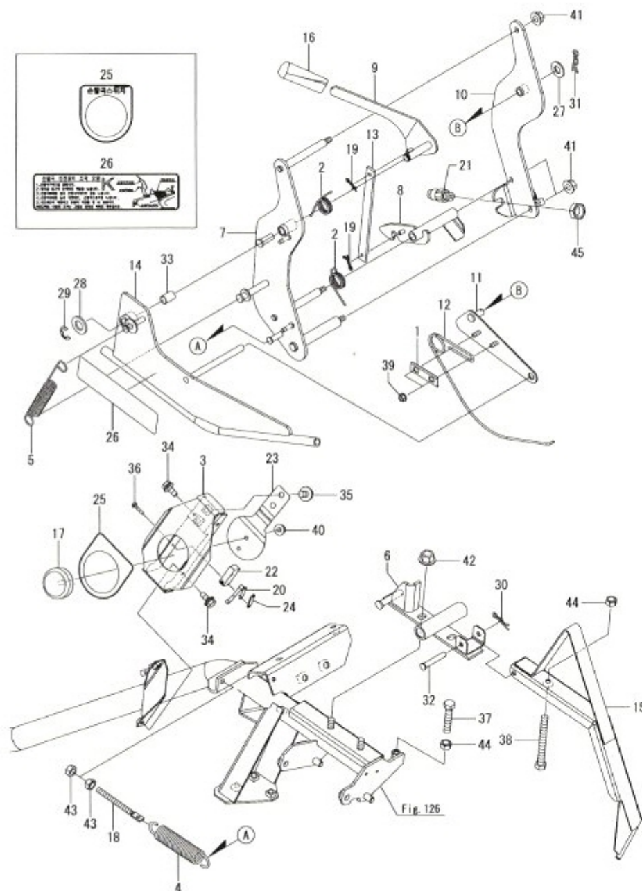
Fig.129. 수동 탈곡 가이드
