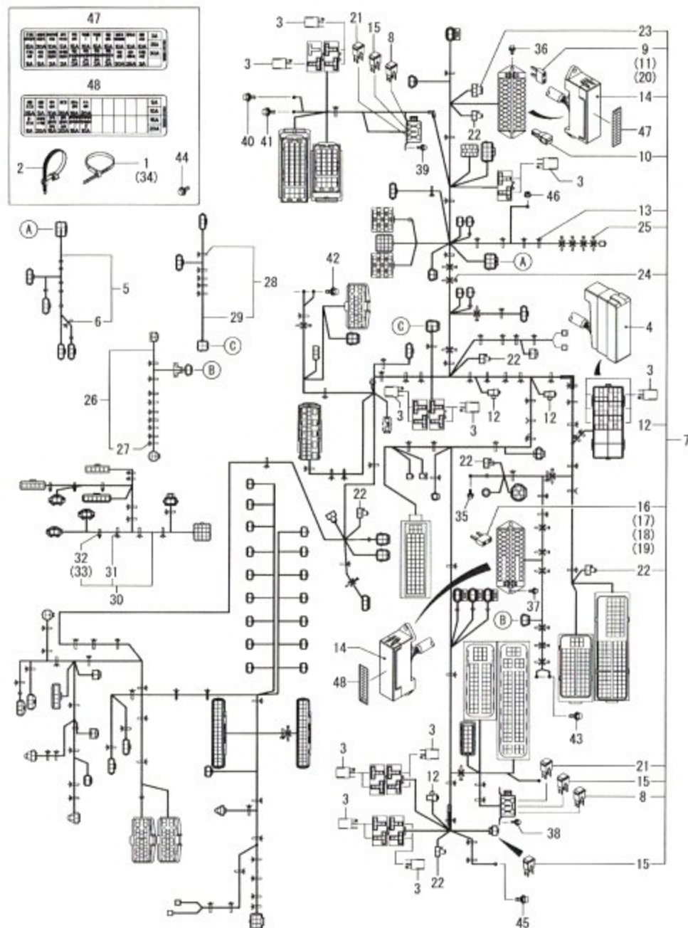
Fig.312. 배선 하네스(메인)
