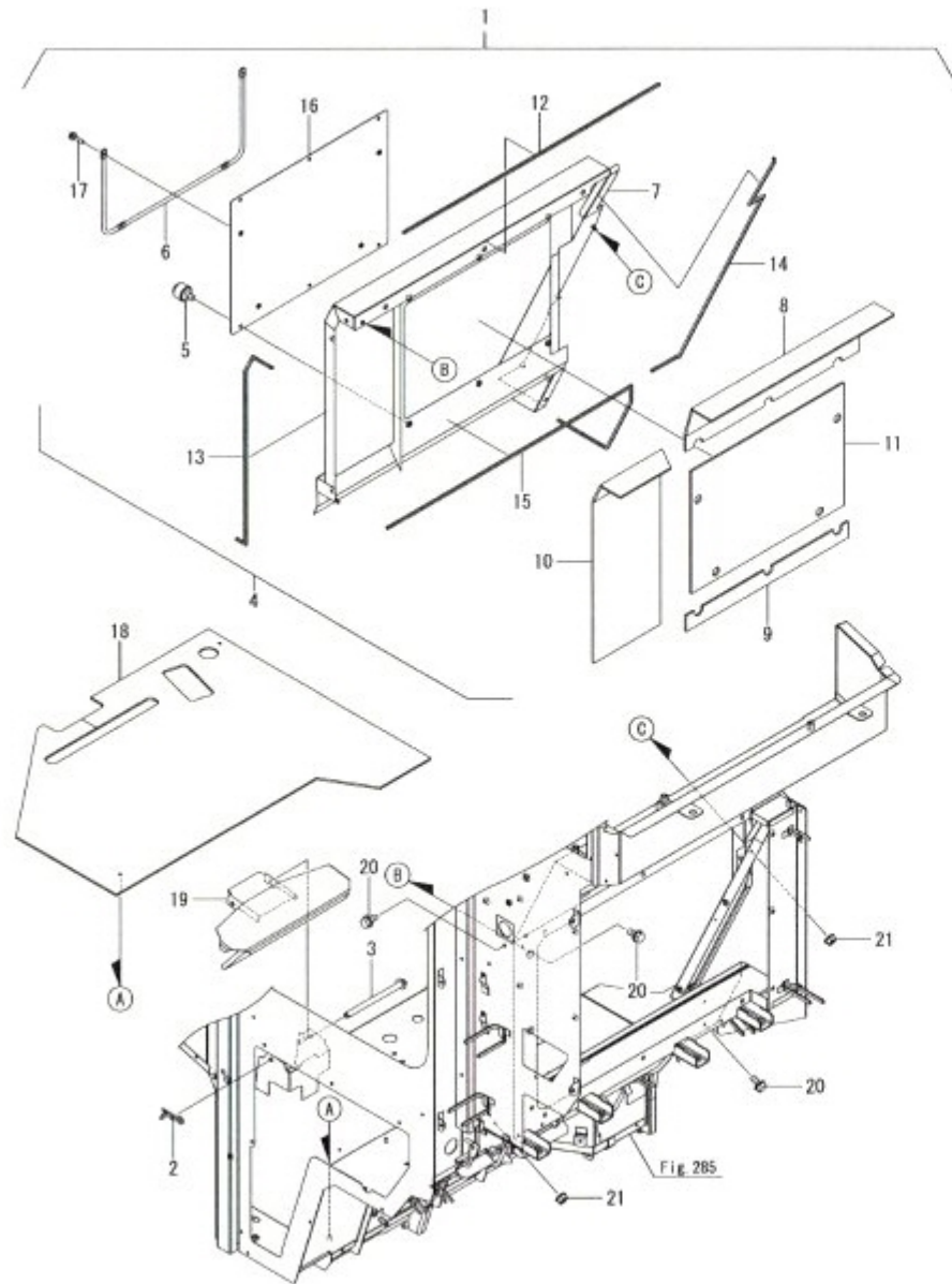
Fig.292. 캐빈 프레임(8)
