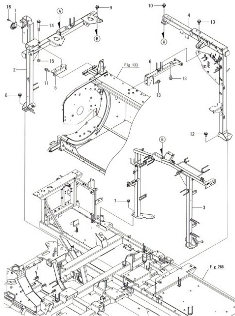
Fig.282. 바닥 프레임
