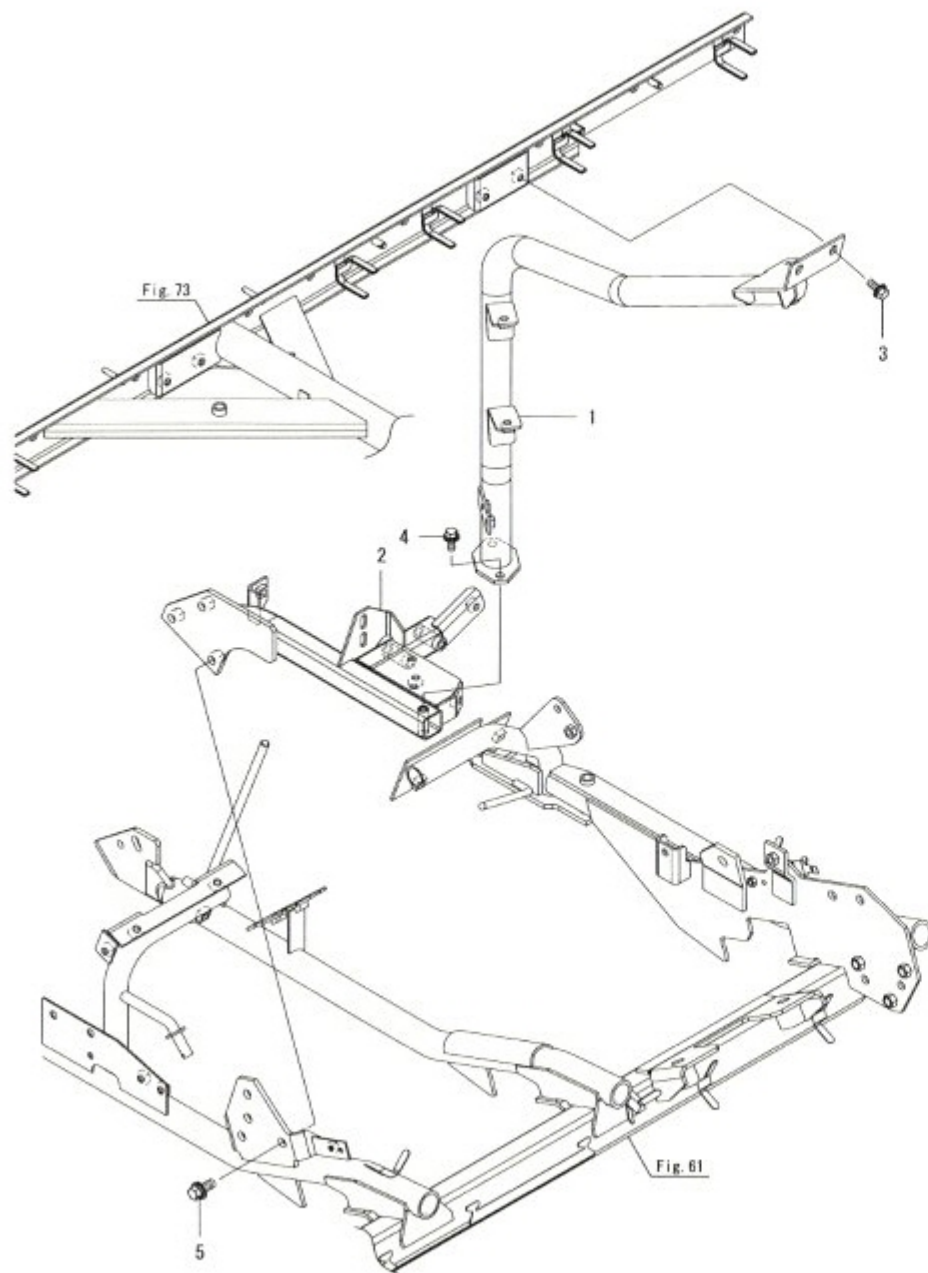
Fig.89. 끌어모음프레임(중-우-우)
