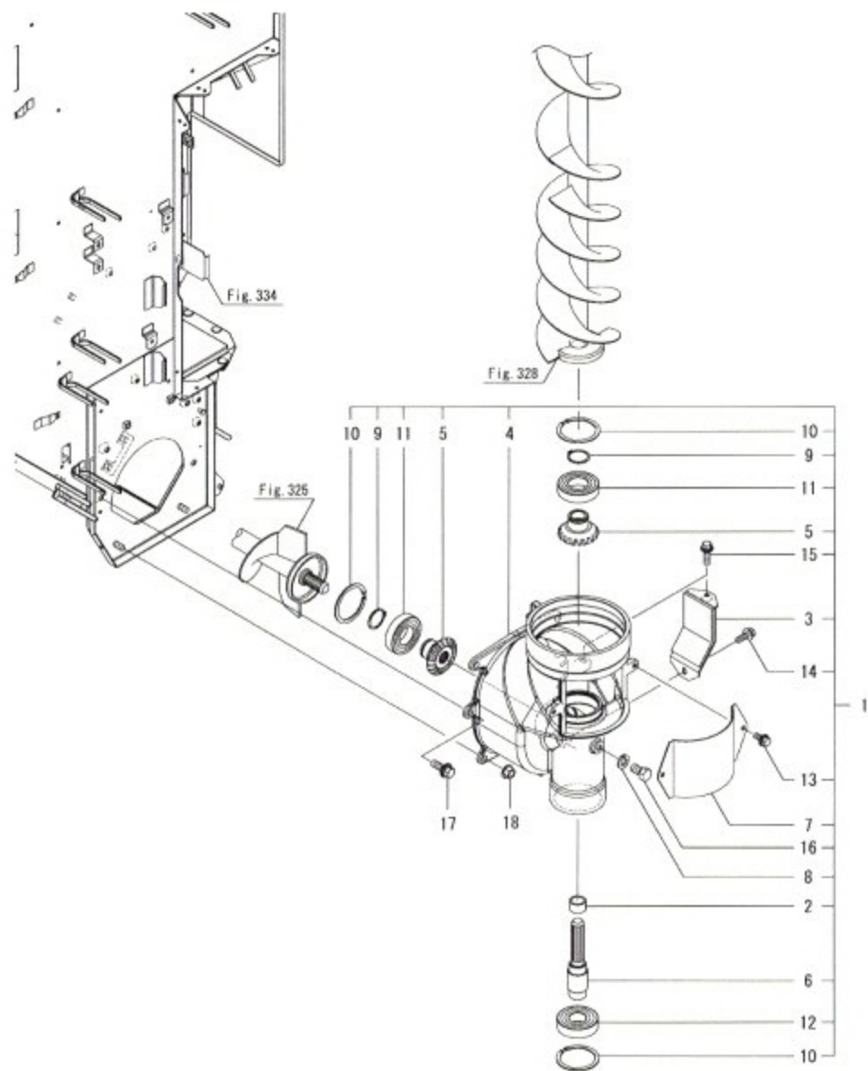
Fig.326. 하부 곡물 컨베이어 연결
