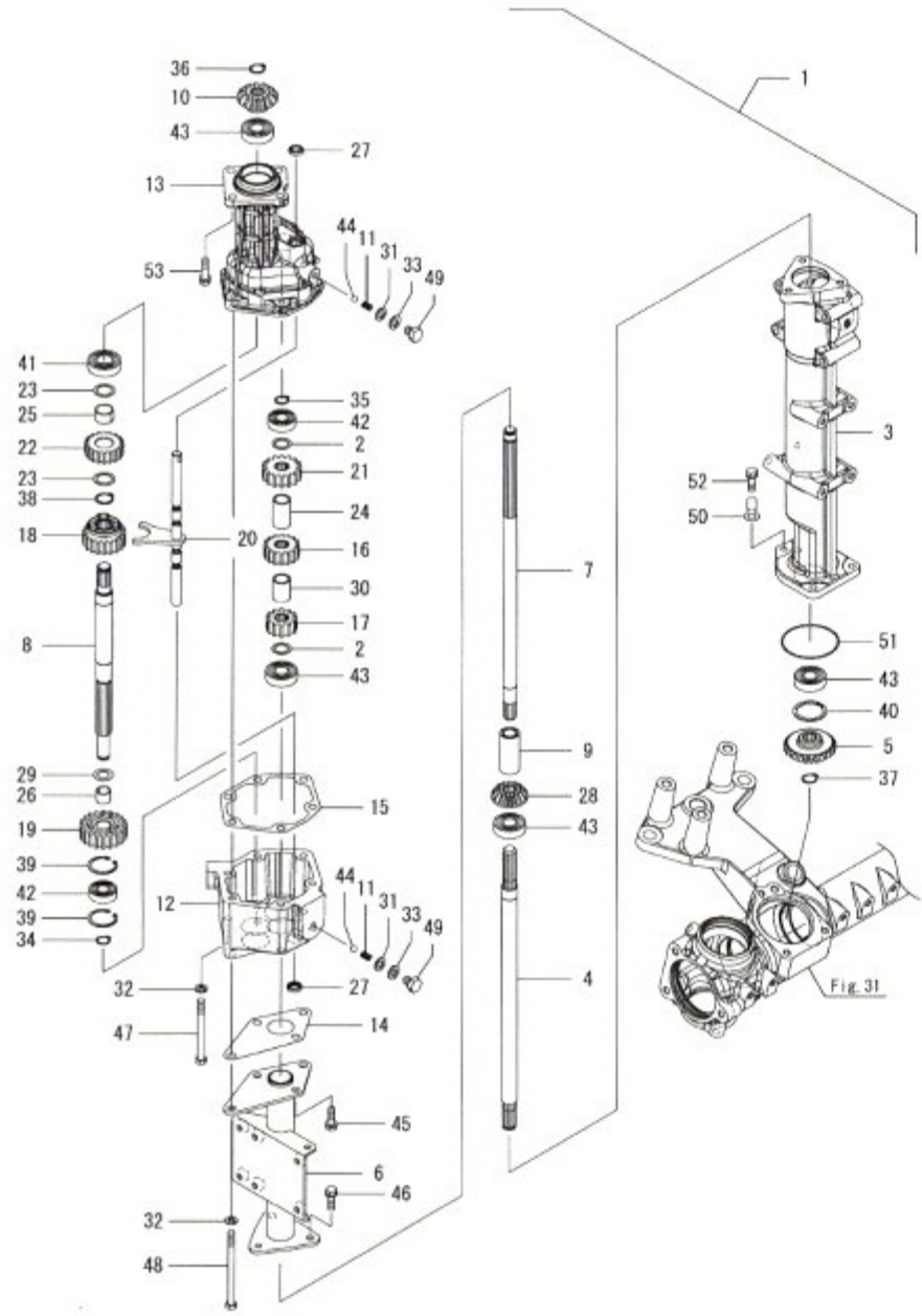
Fig.36. 7조구동케이스(8)
