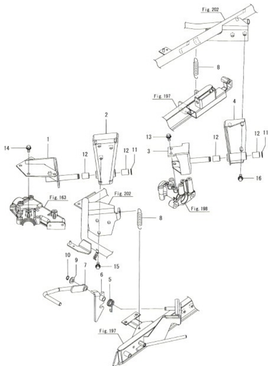
Fig.204. 짚배출오픈
