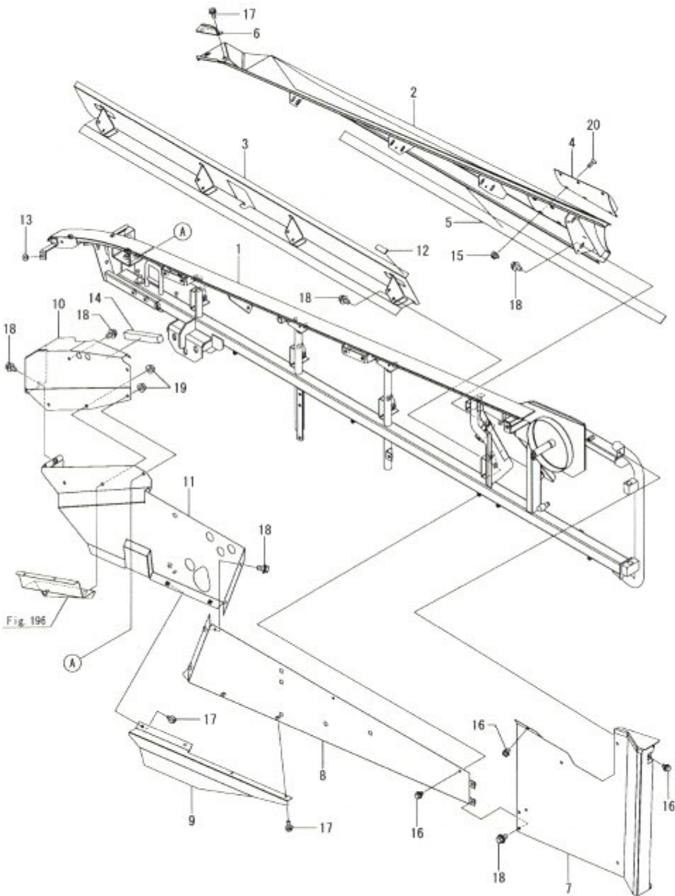
Fig.139. 탈곡실프레임(좌)(1)
