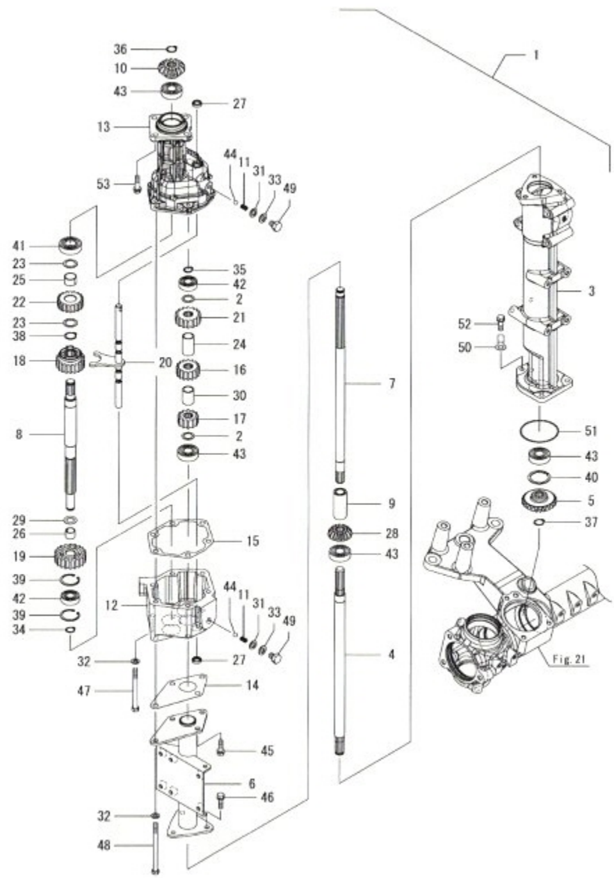
0CNP7-M01360 수확(1) Fig.26. 6조구동케이스(8)
