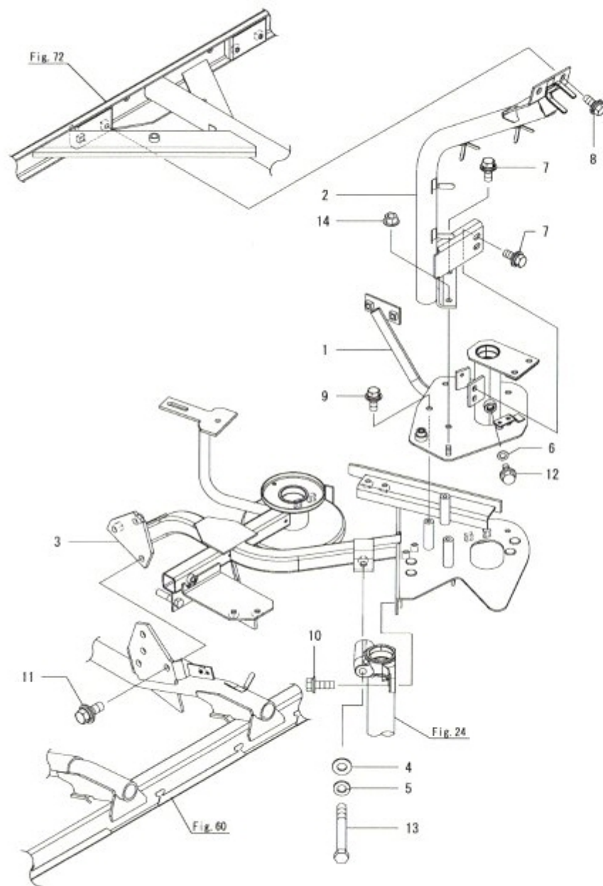
Fig.85. 끌어모음프레임(중-좌)
