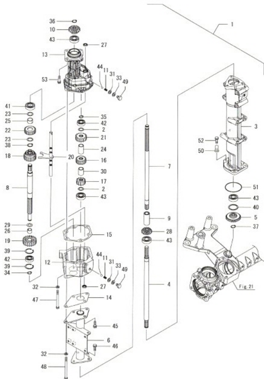
Fig.26. 6조구동케이스(8)
