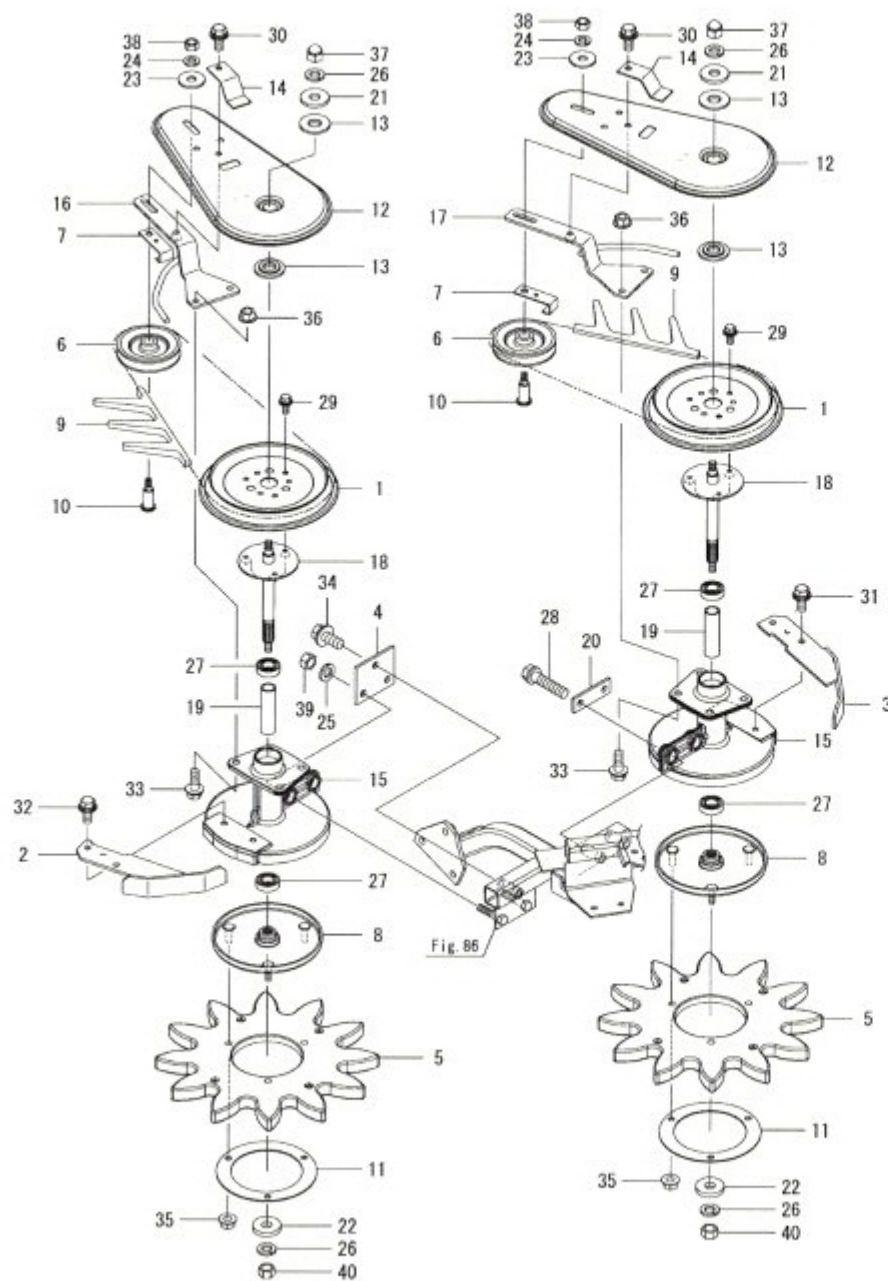
Fig.77. 스타휠(중-좌)
