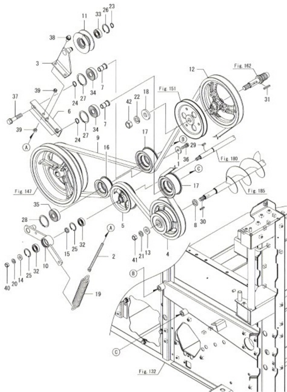
Fig.149. 벨트(2차)
