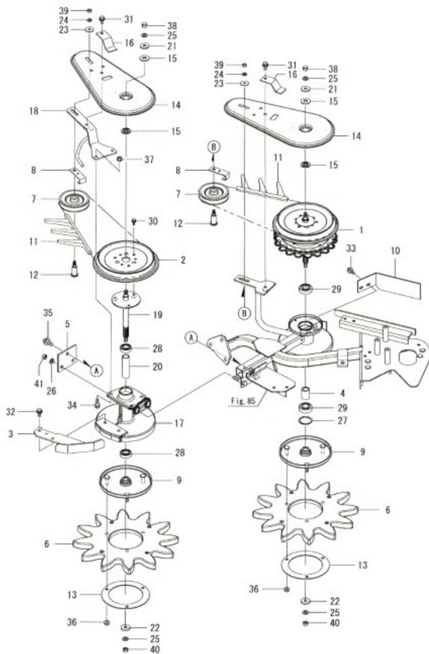
Fig.76. 스타휠(중-좌)
