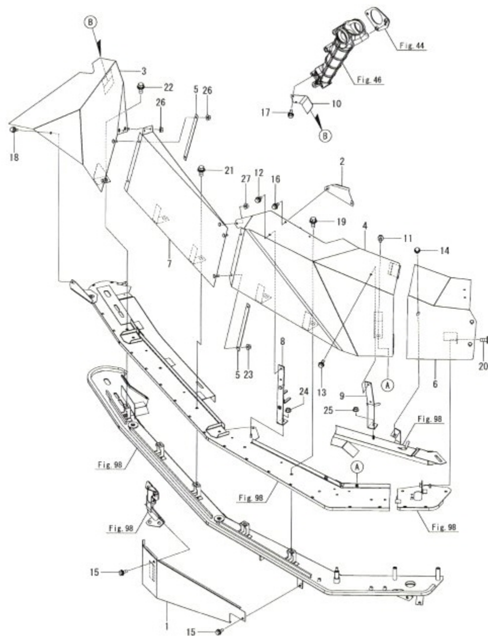
Fig.114. 상단 이송 가이드(오른쪽)
