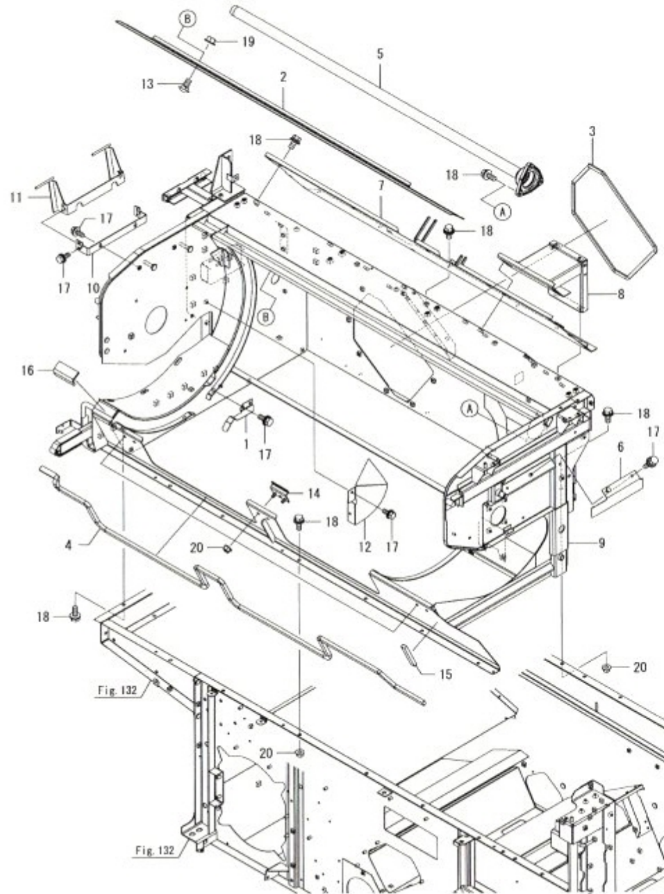
Fig.133. 상부분체(1)
