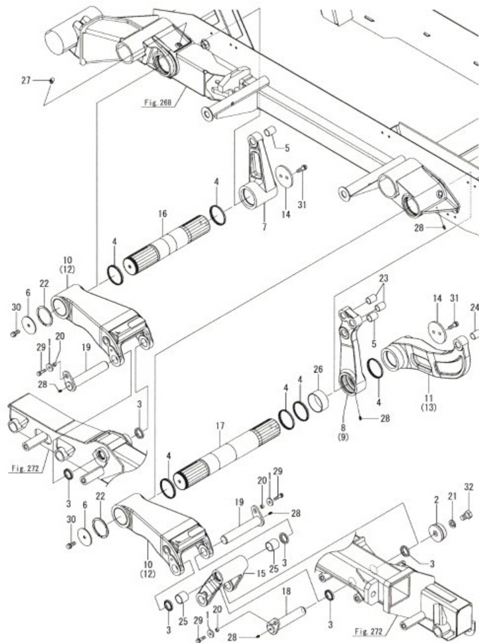
Fig.280. 스윙(1)
