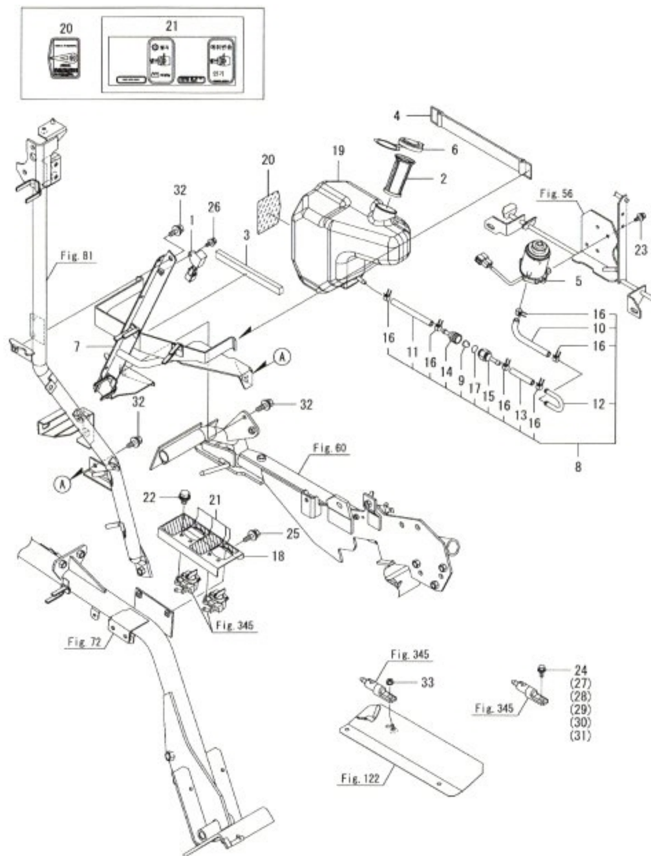
Fig.344. 주유장치(1)
