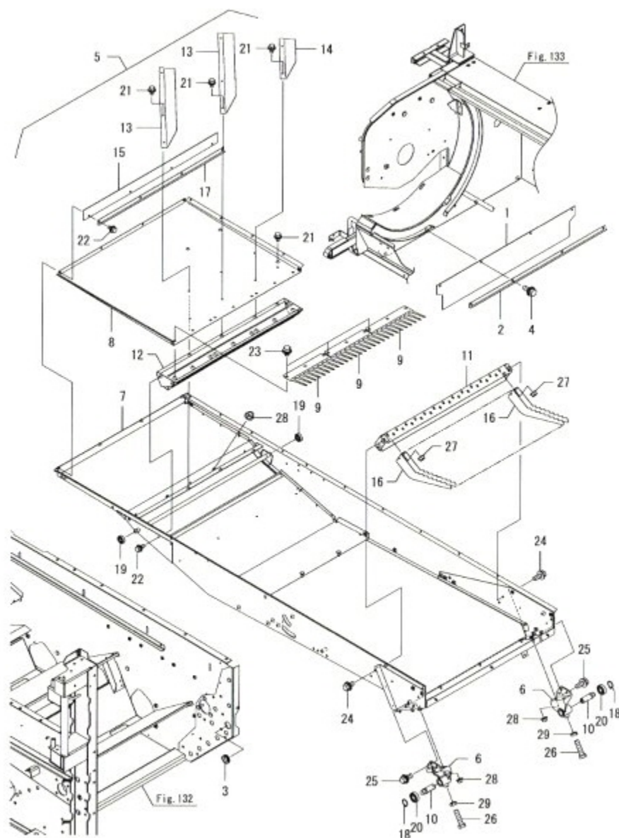
Fig.174. 요동선별프레임(1)
