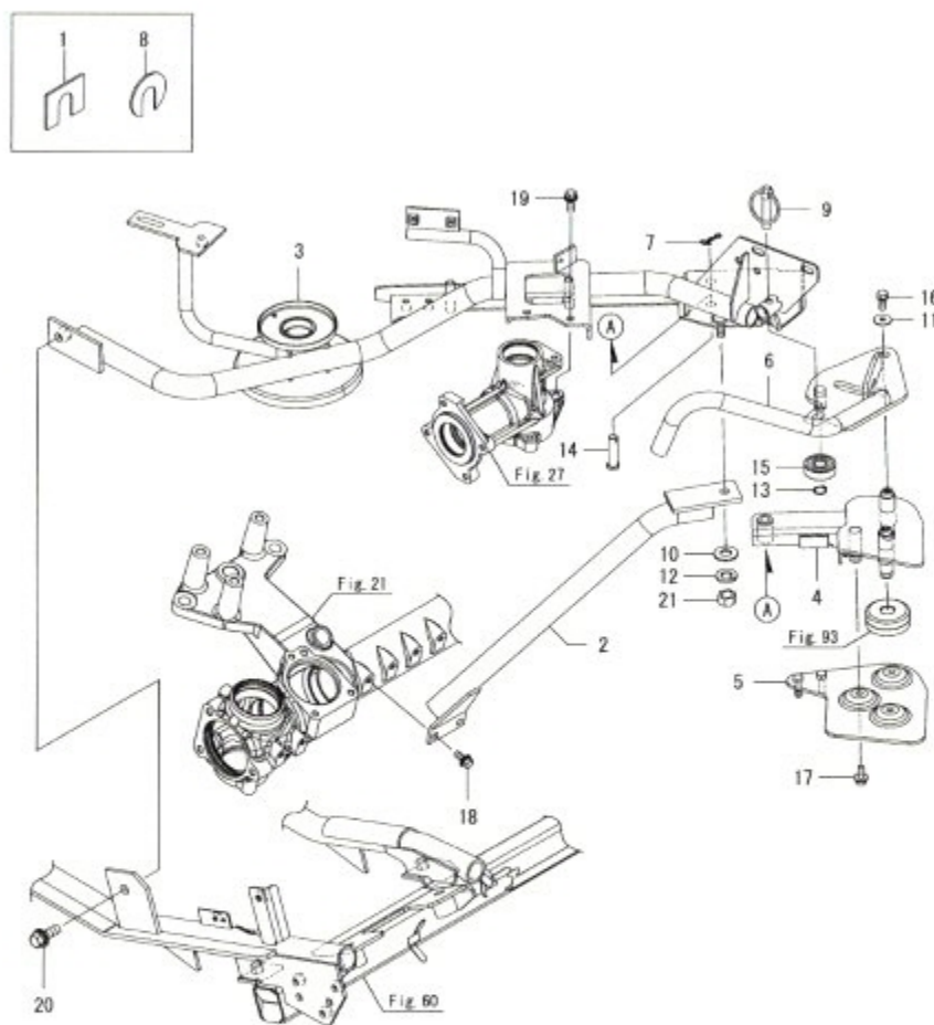
Fig.83. 끌어모음프레임(좌)
