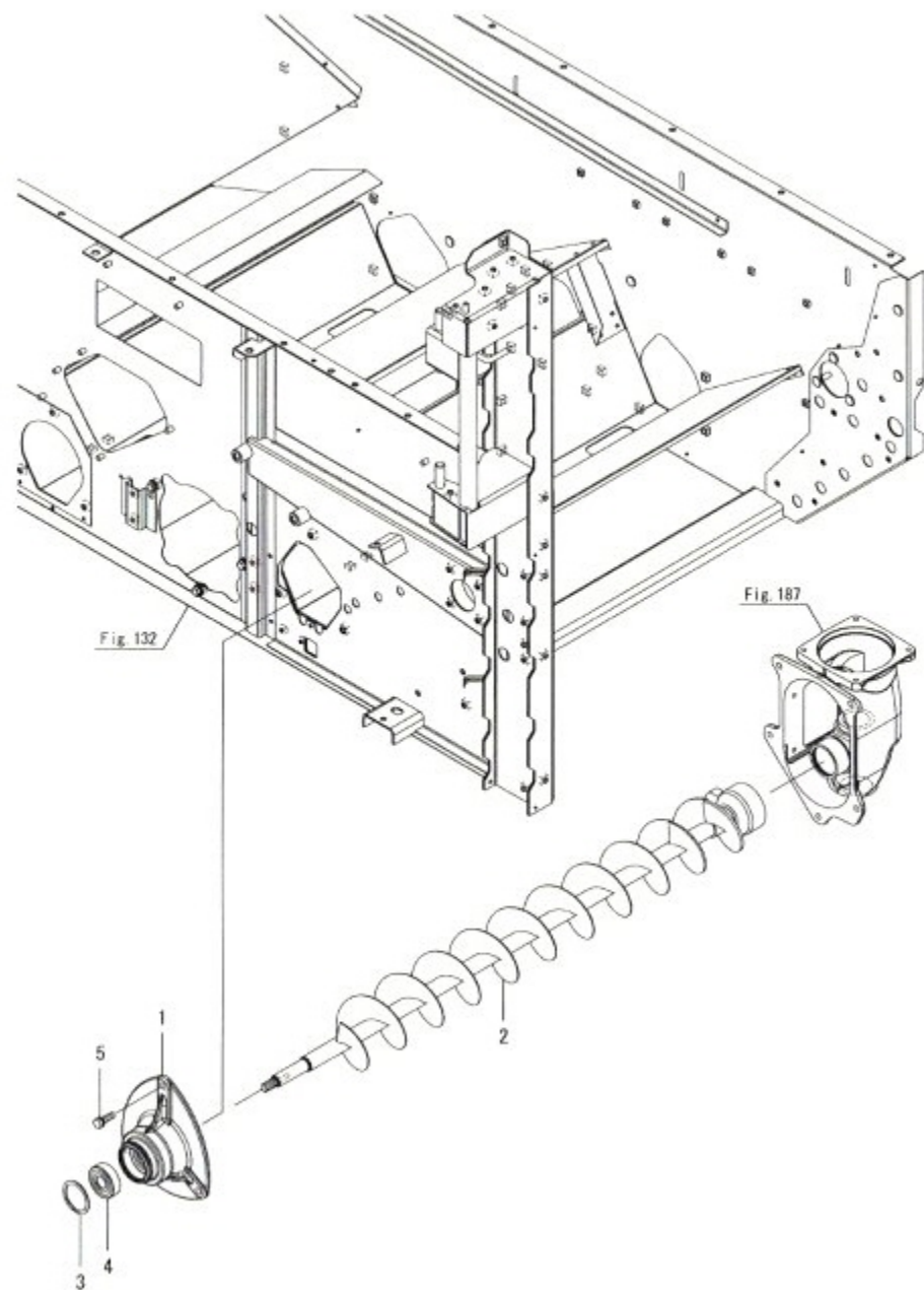
Fig.185. 컨베이어(2차)
