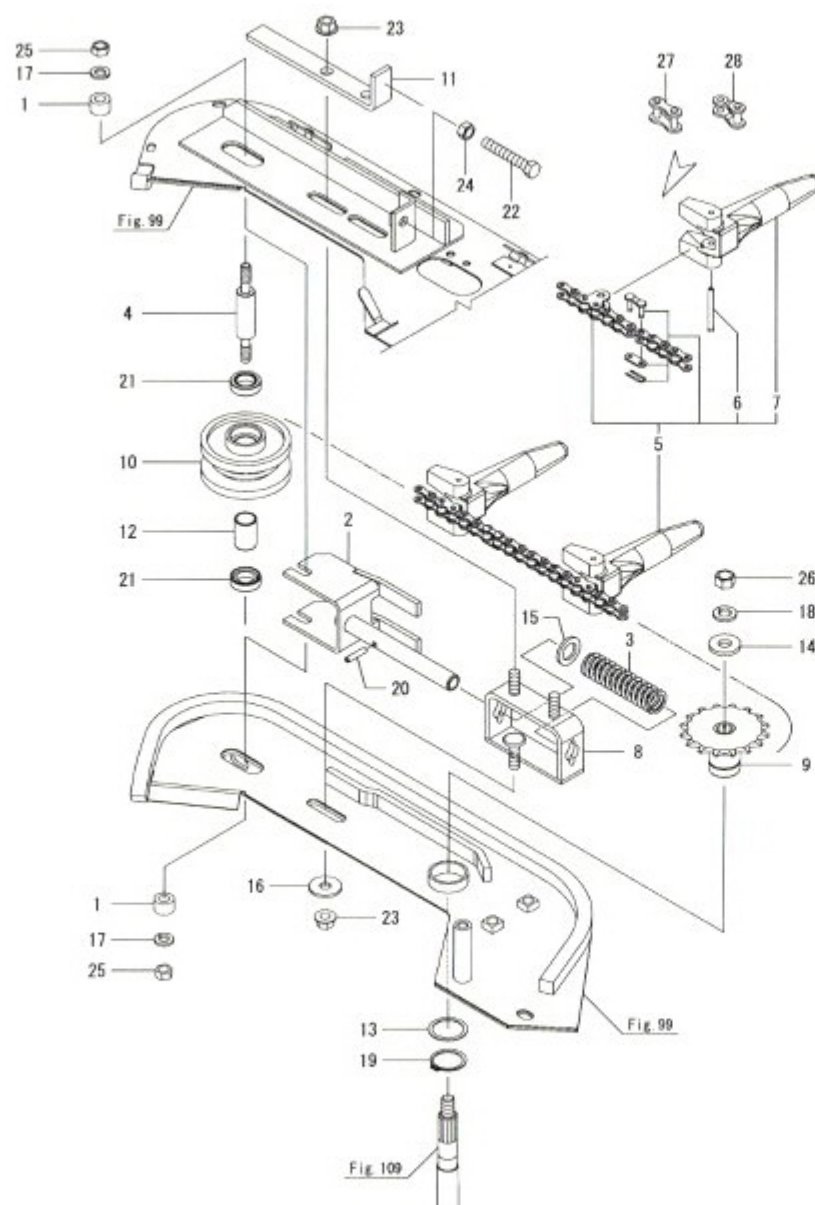
Fig.106. 상반송롤러(중)
