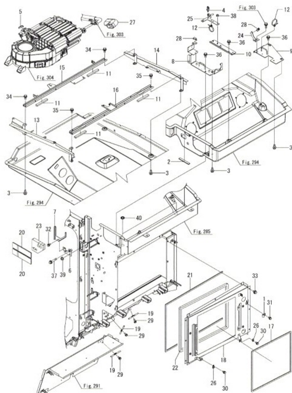
Fig.305. 에어컨취부
