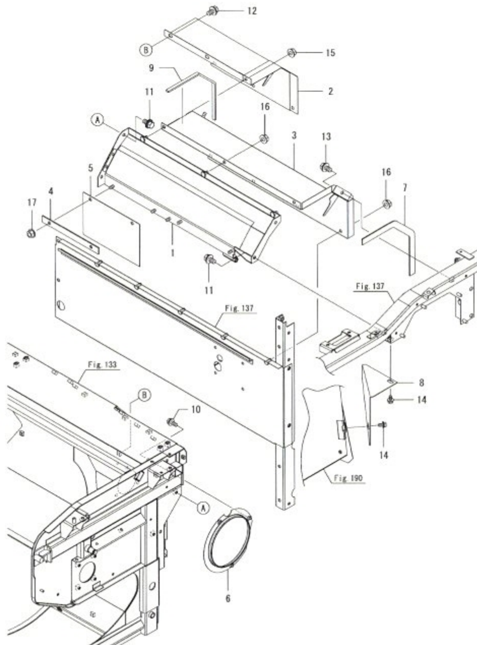
Fig.171. 처리 드럼 커버
