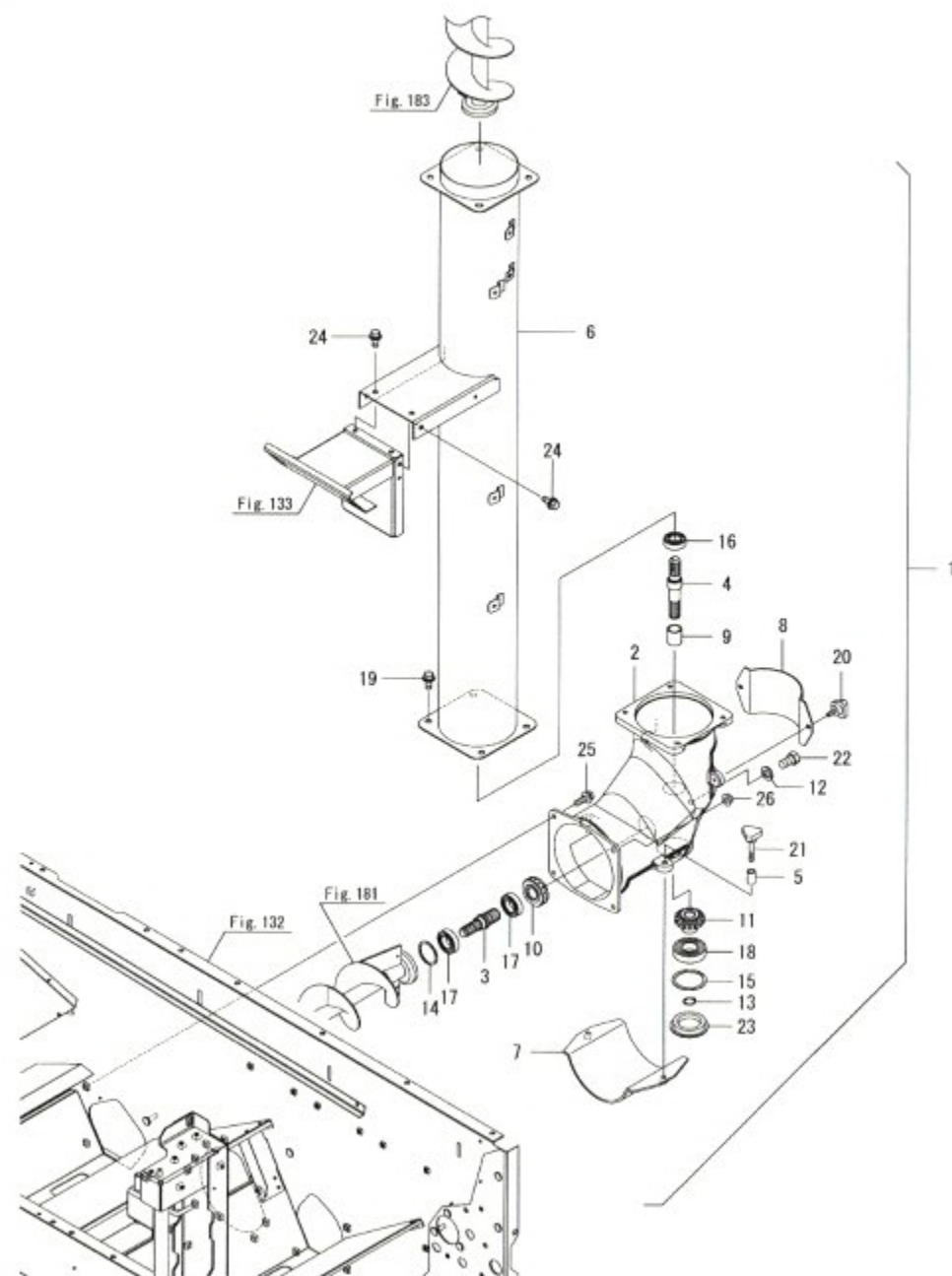
Fig.182. 곡물 승강 컨베이어 케이스
