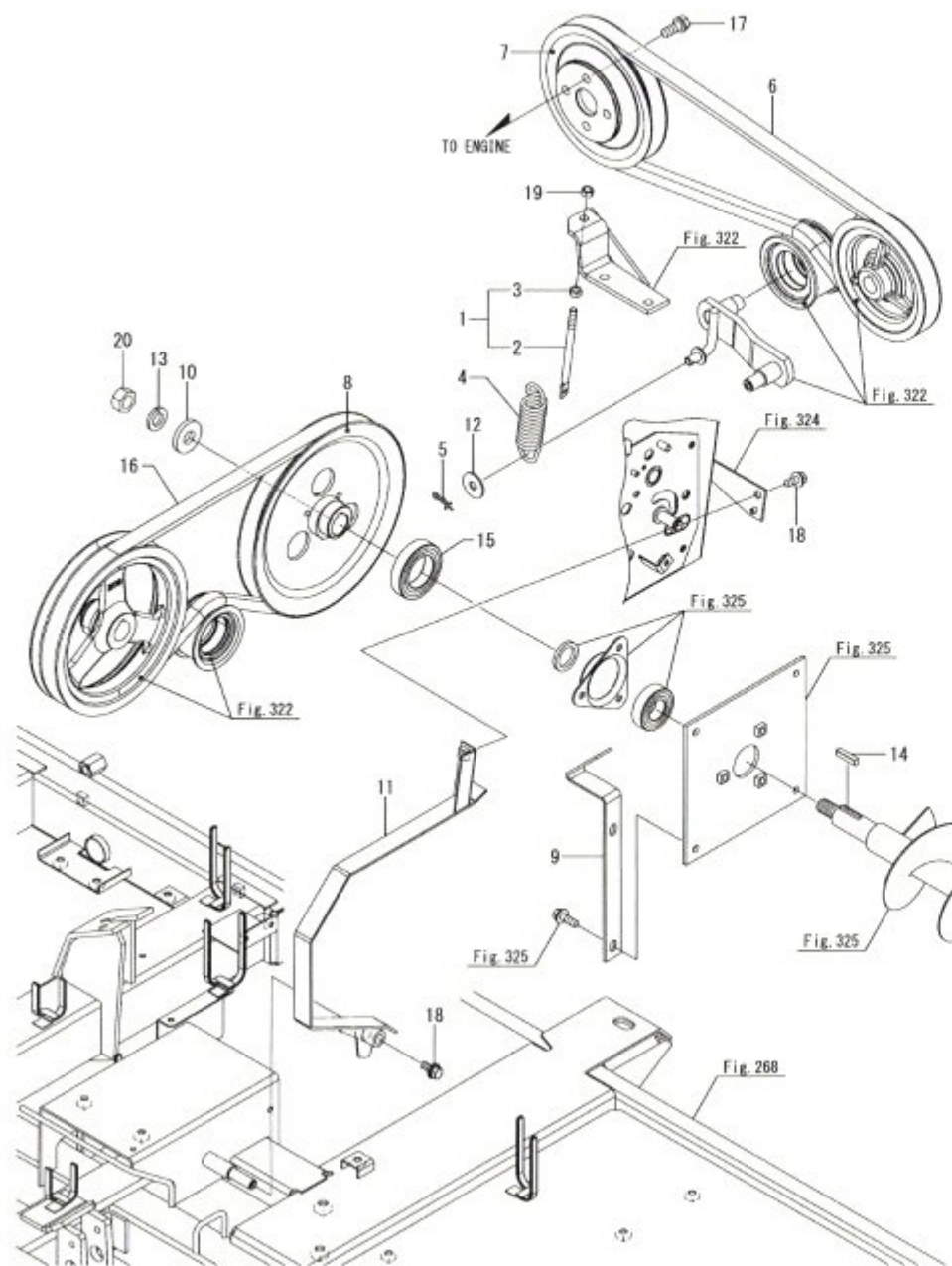
Fig.323. 오거 벨트
