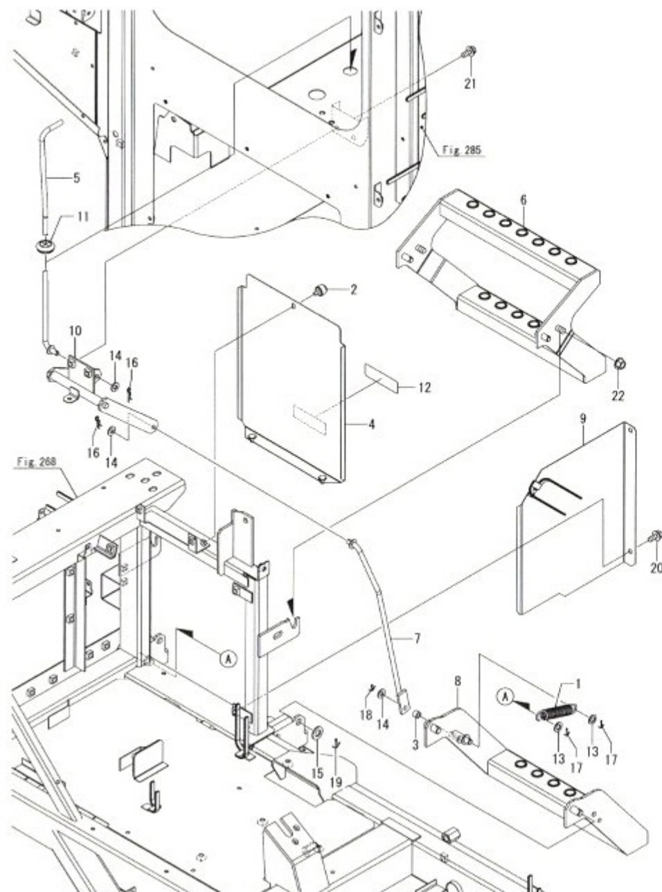
Fig.265. 발판
