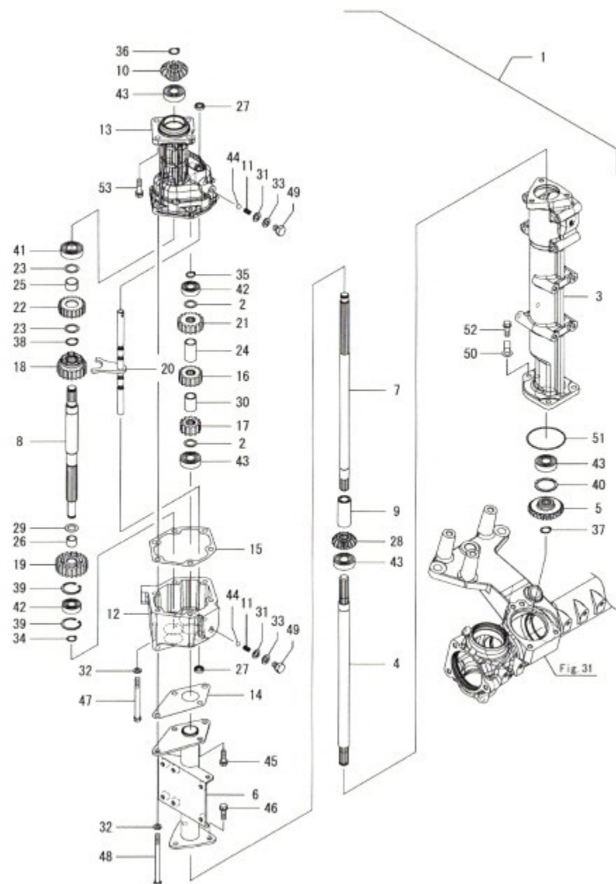
Fig.36. 7조구동케이스(8)
