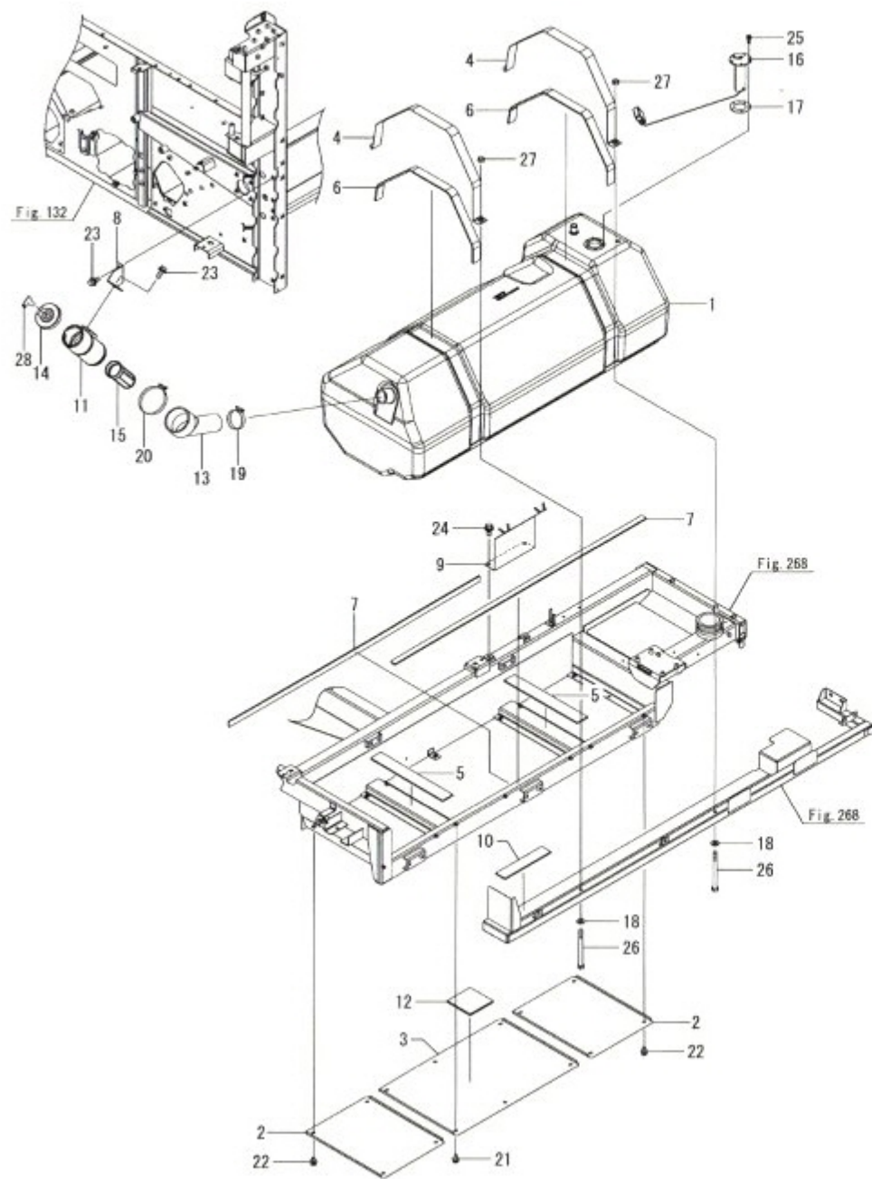
Fig.4. 연료탱크(1)
