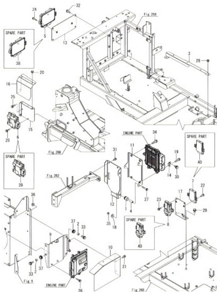
Fig.269. 컨트롤(새시)
