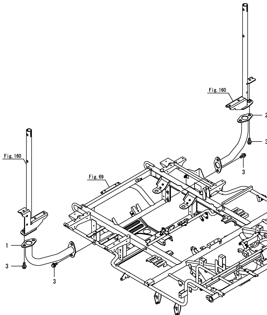
Fig.164. 예비묘탑재대
