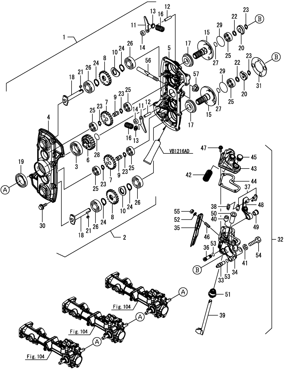
Fig.118. 식부 로터 암(우측)(가득찬 묘)
