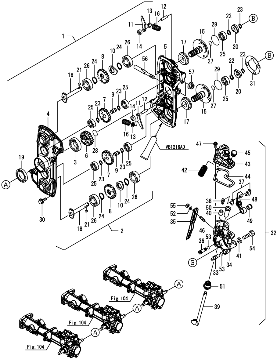
Fig.118. 식부 로터 암(우측)(가득찬 묘)
