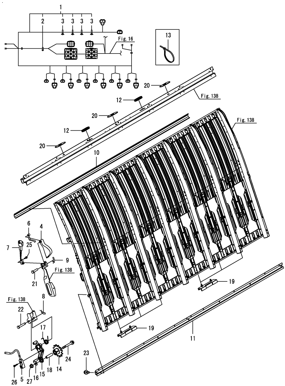
Fig.137. 묘 트레이(1)
