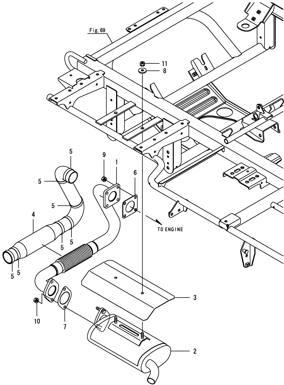
Fig.5. 소음기
