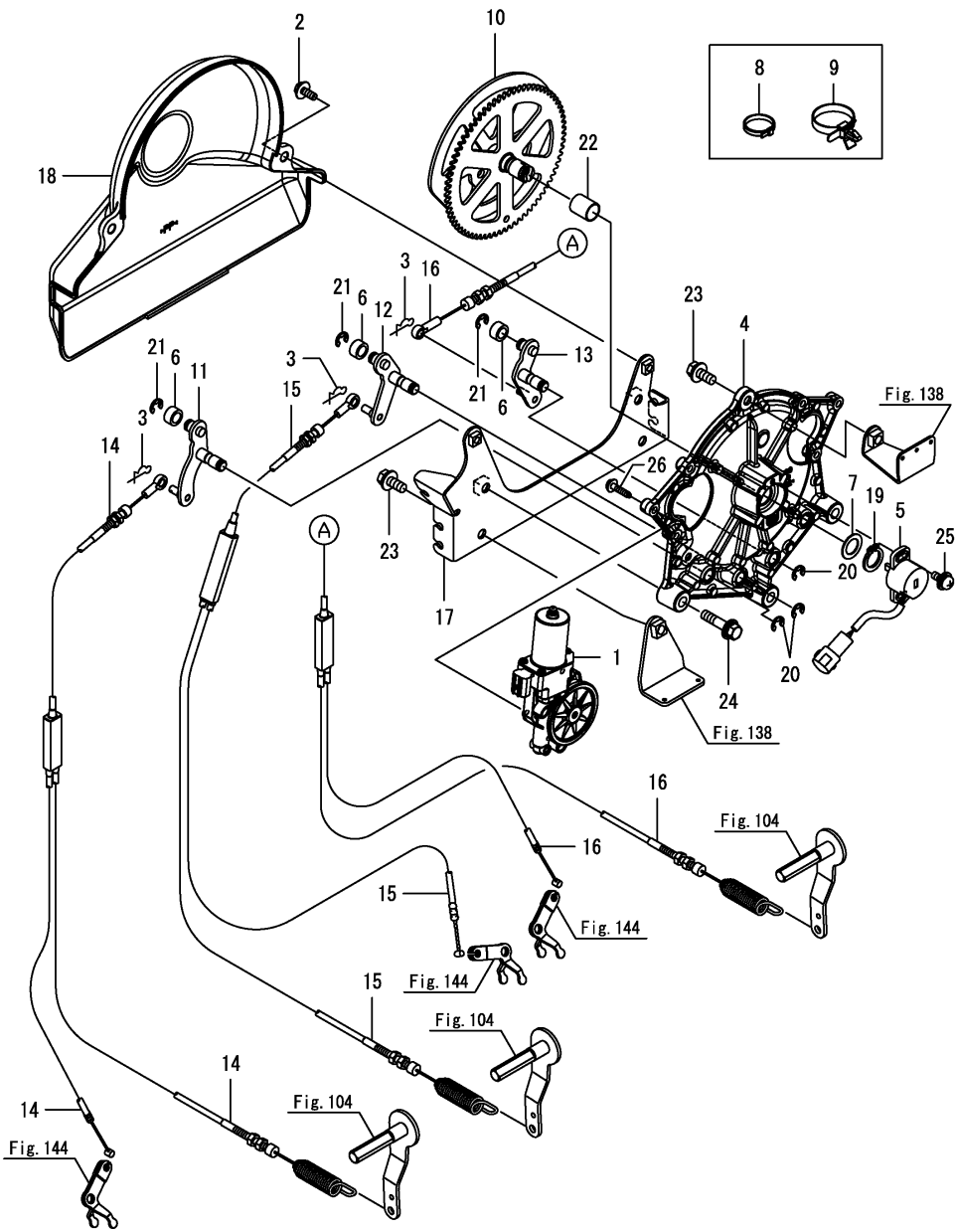
Fig.158. 유니트클러치조작
