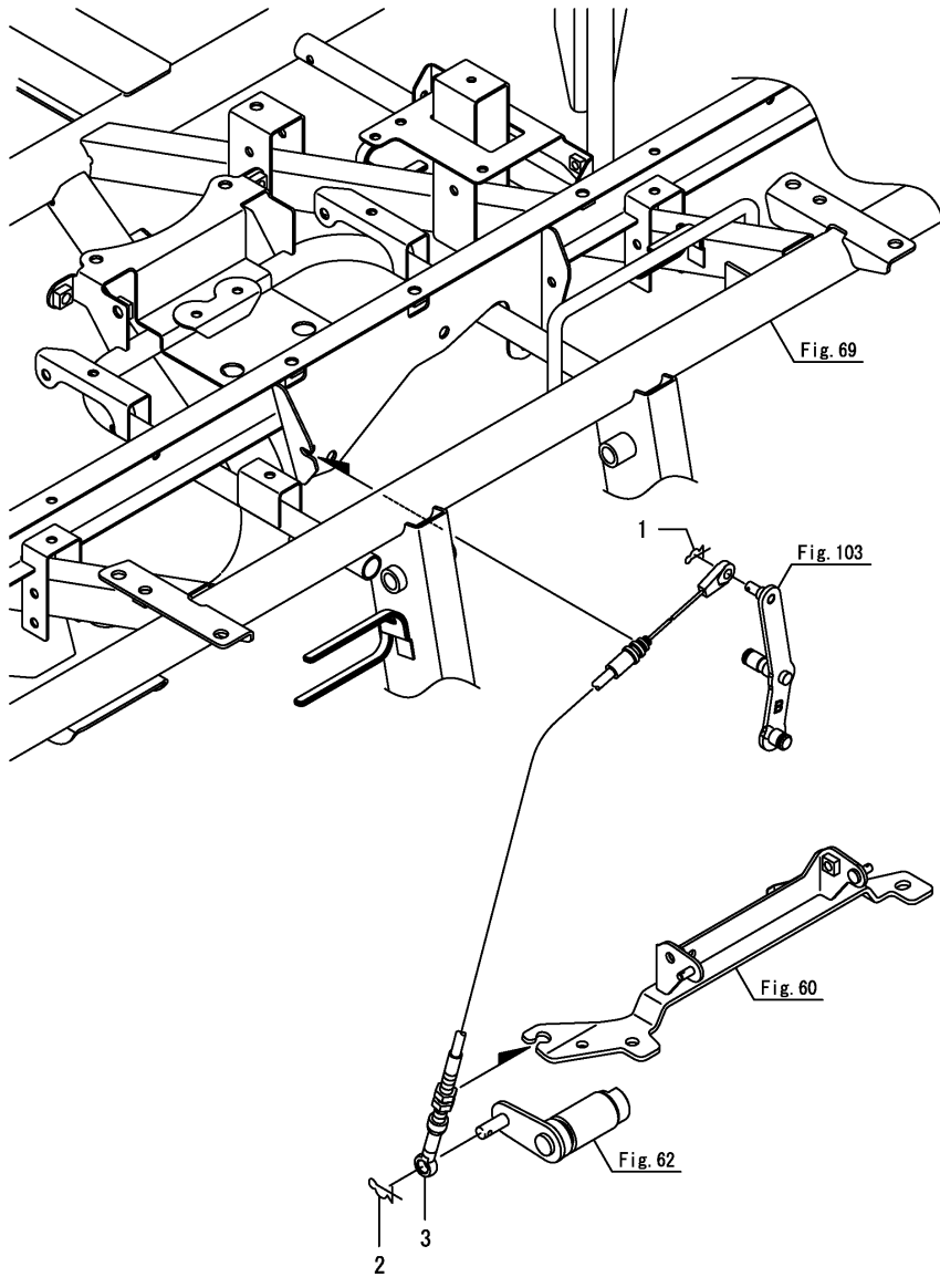
Fig.121. 로터와이어
