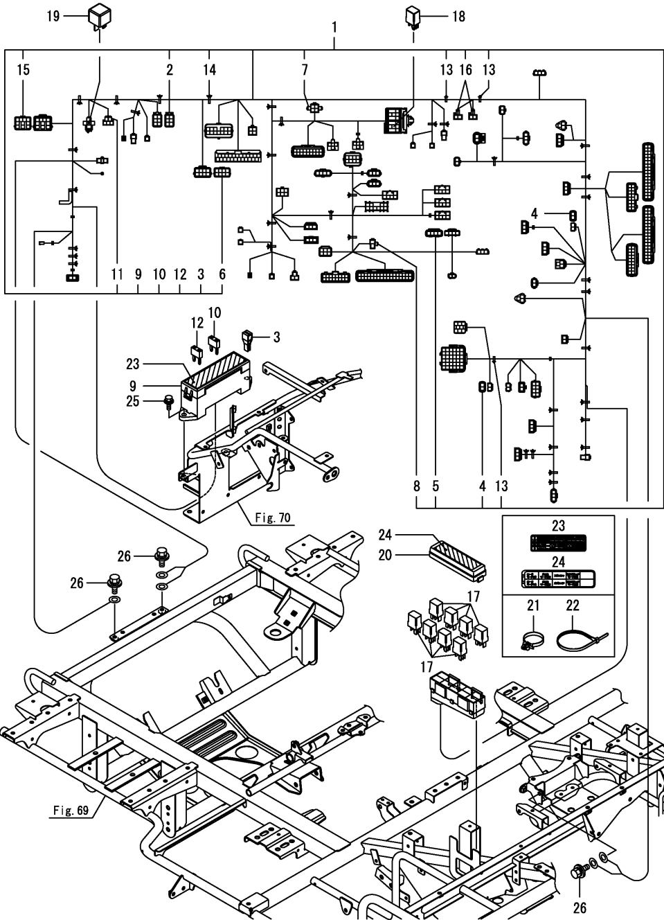
Fig.14. 전장품(1)
