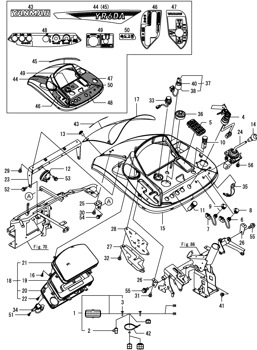
Fig.75. 조작패널
