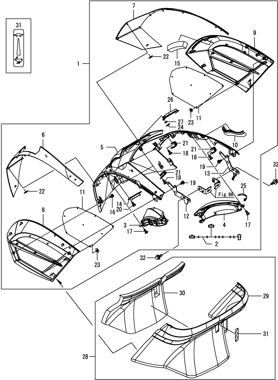
Fig.73. 본네트
