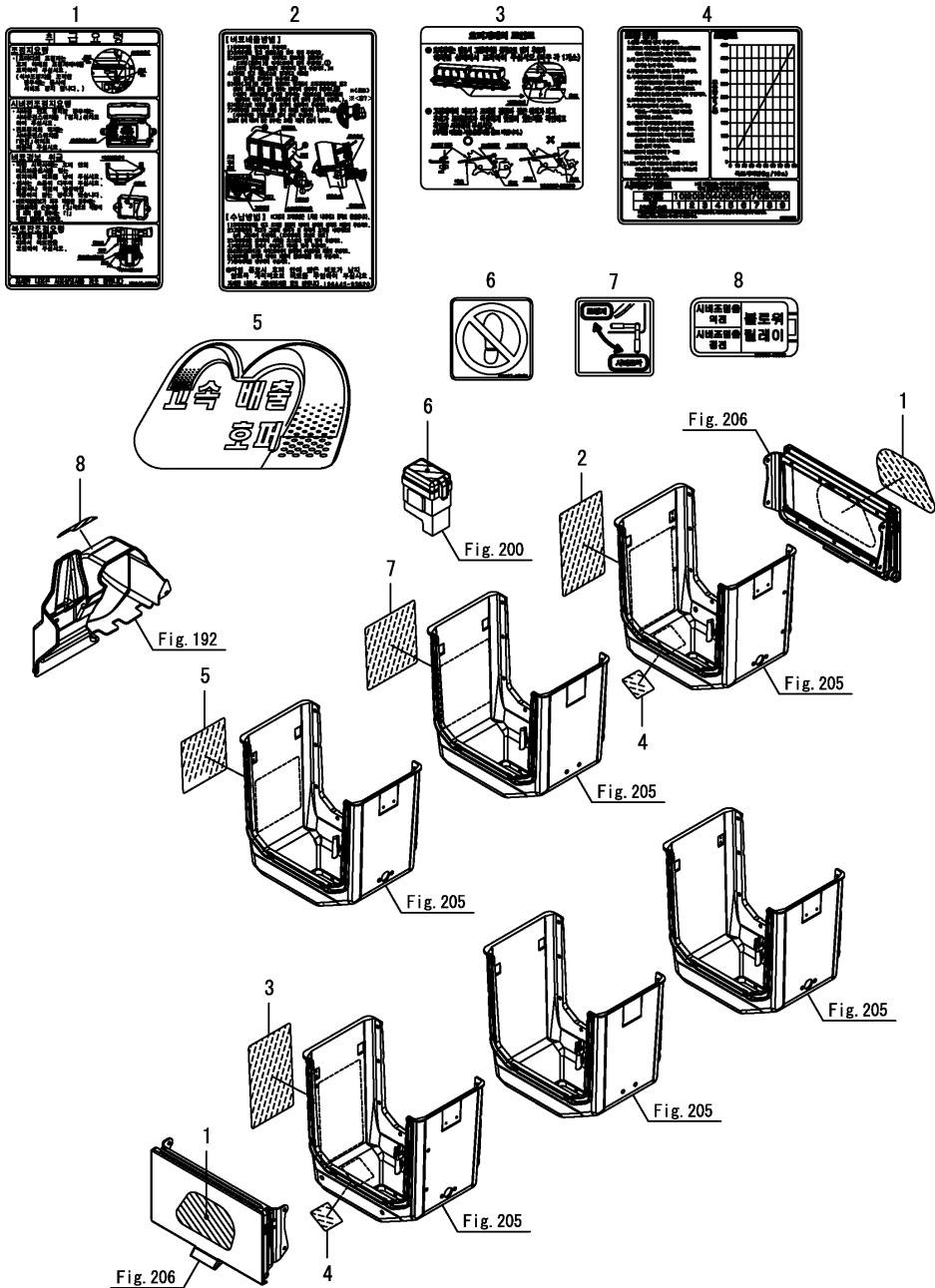
Fig.208. 명판
