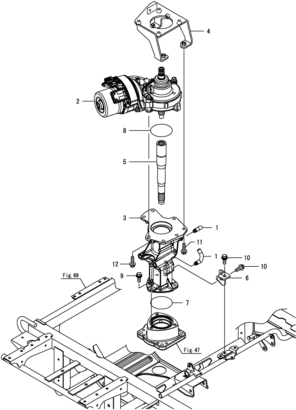
Fig.87. 스티어링 유닛
