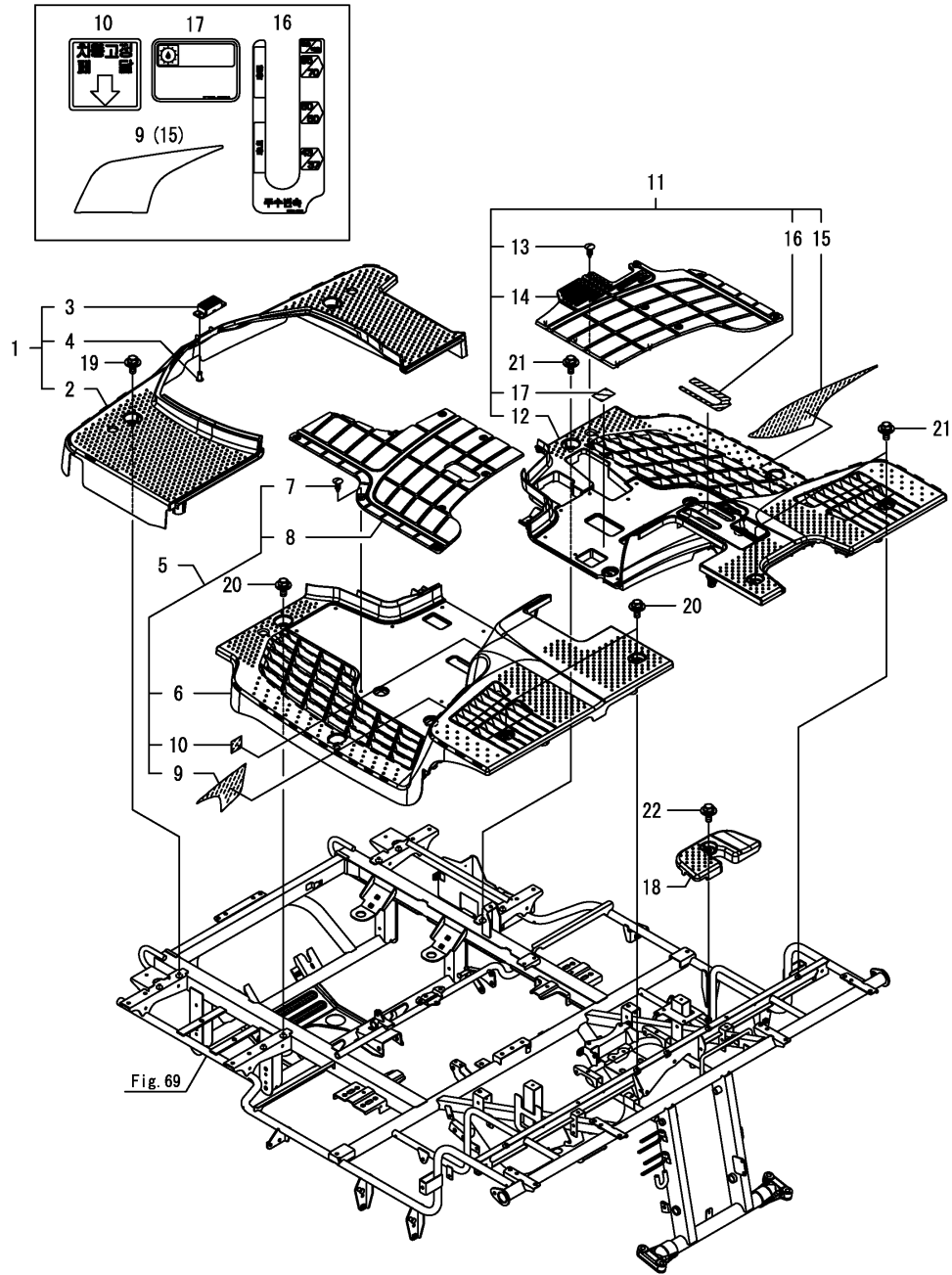
Fig.76. 발판
