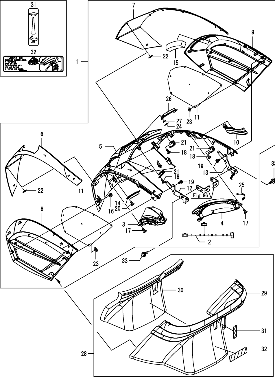
Fig.74. 본넷
