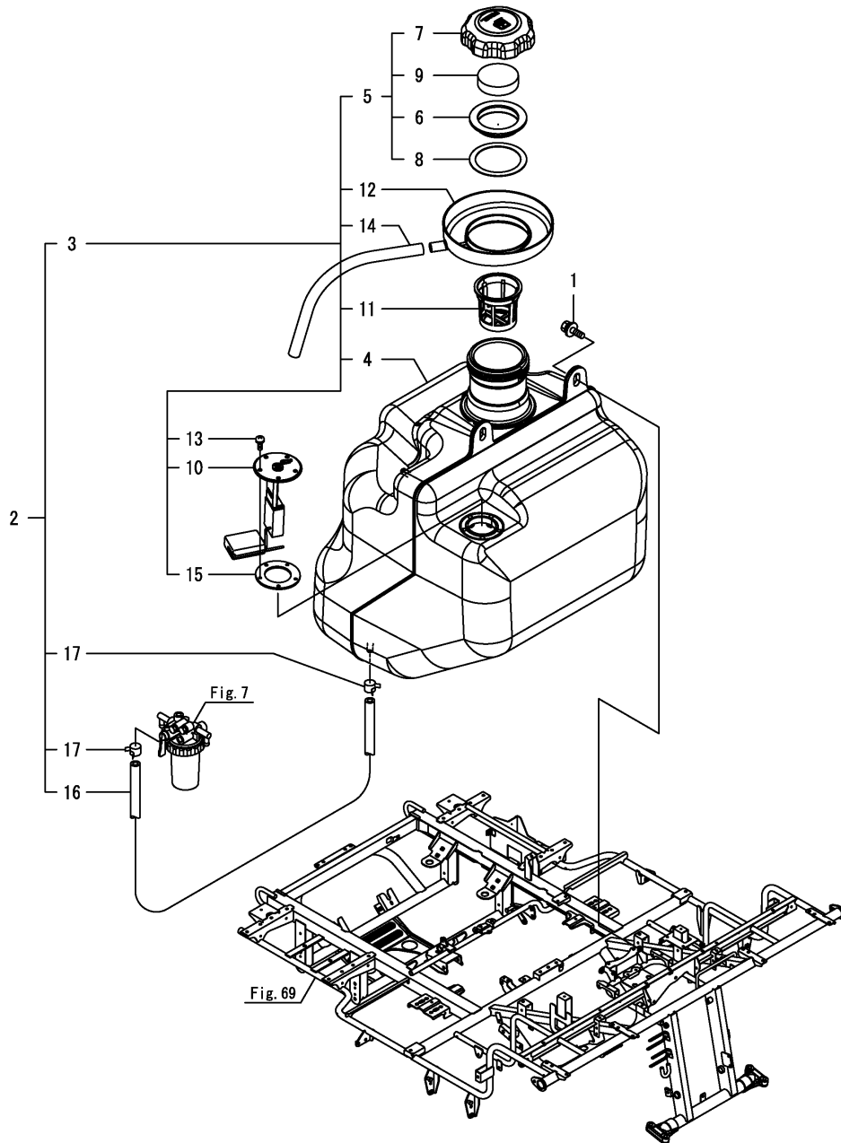
Fig.6. 연료탱크
