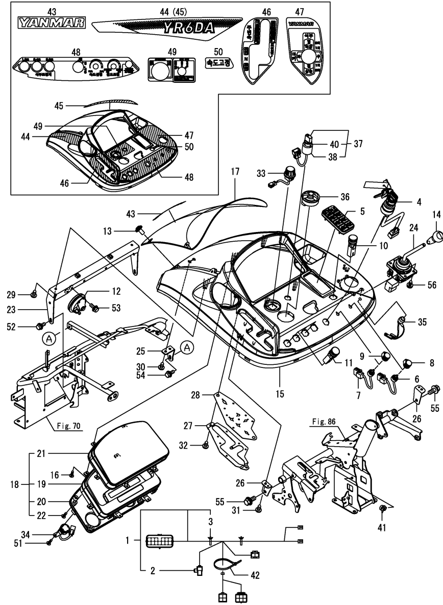
Fig.75. 조작패널
