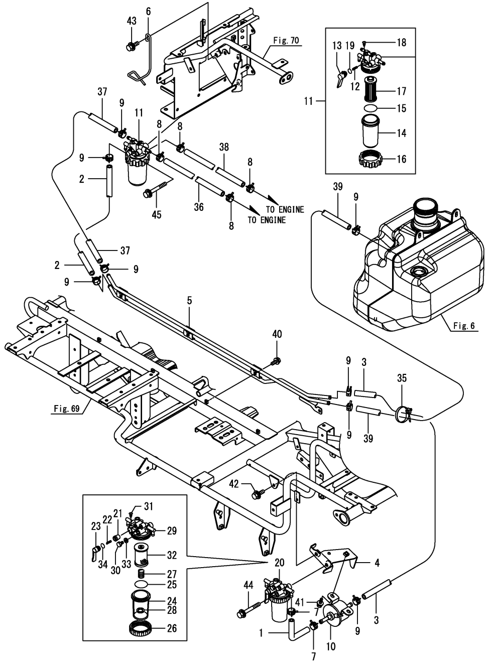
Fig.7. 연료배관
