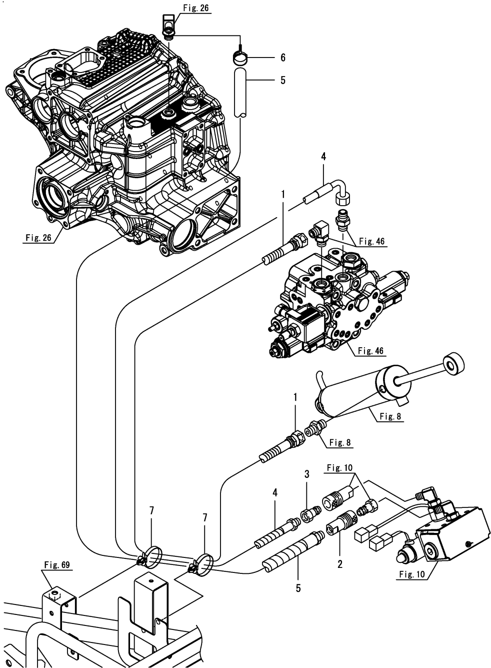
Fig.12. 유압배관
