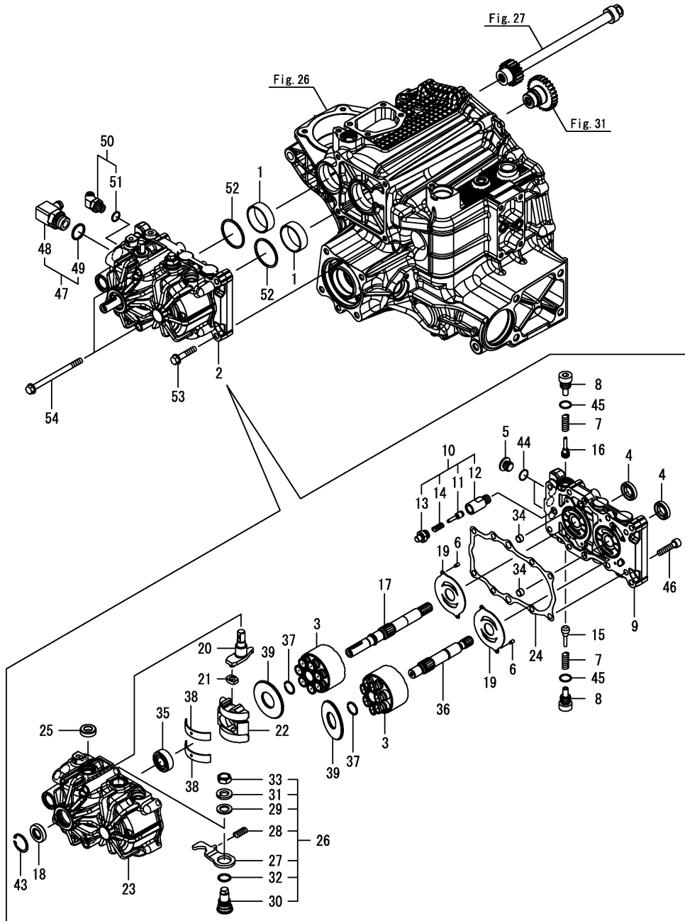
Fig.43. H.S.T.
