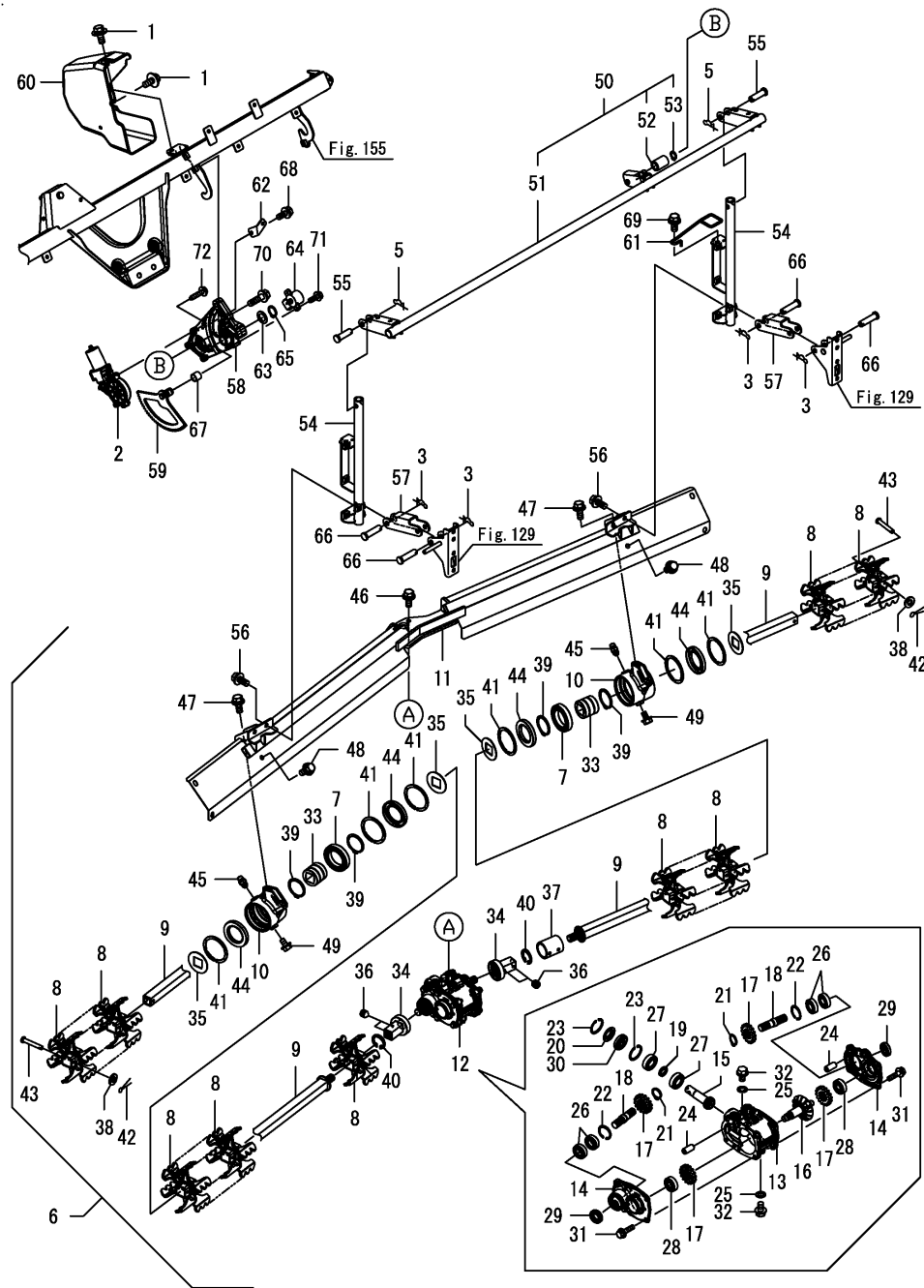
Fig.119. 로터
