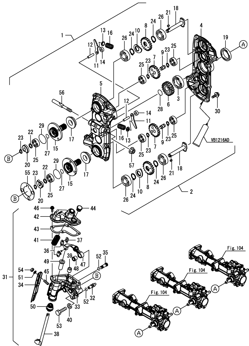
Fig.116. 식부 로터 암(좌측)(가득찬 묘)
