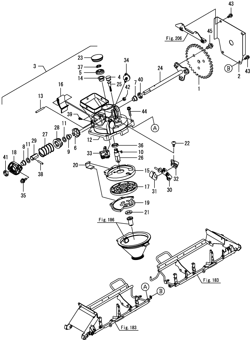
Fig.188. 롤구동(B)
