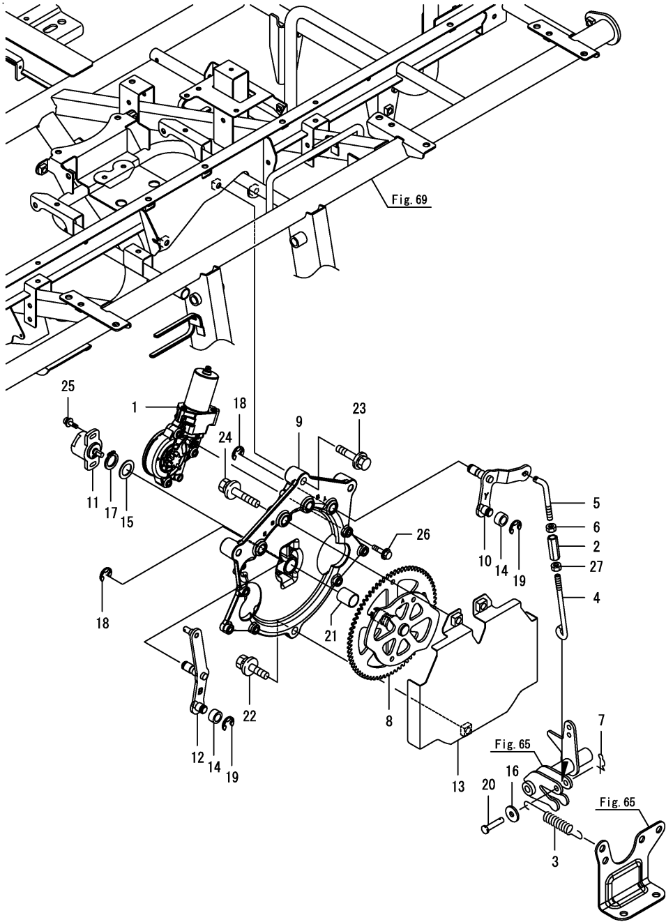
Fig.103. P.T.O. 클러치조작
