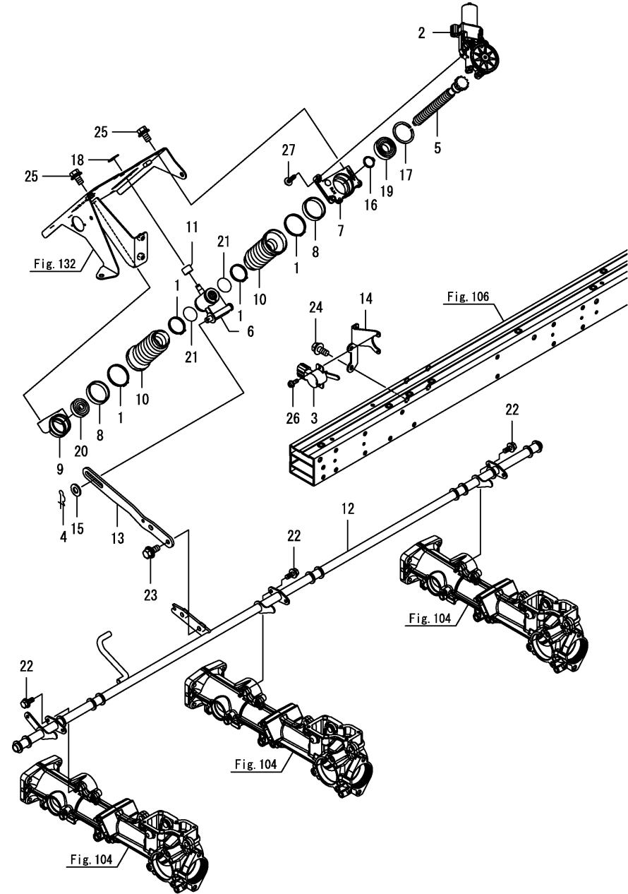
Fig.135. 픽업 조정
