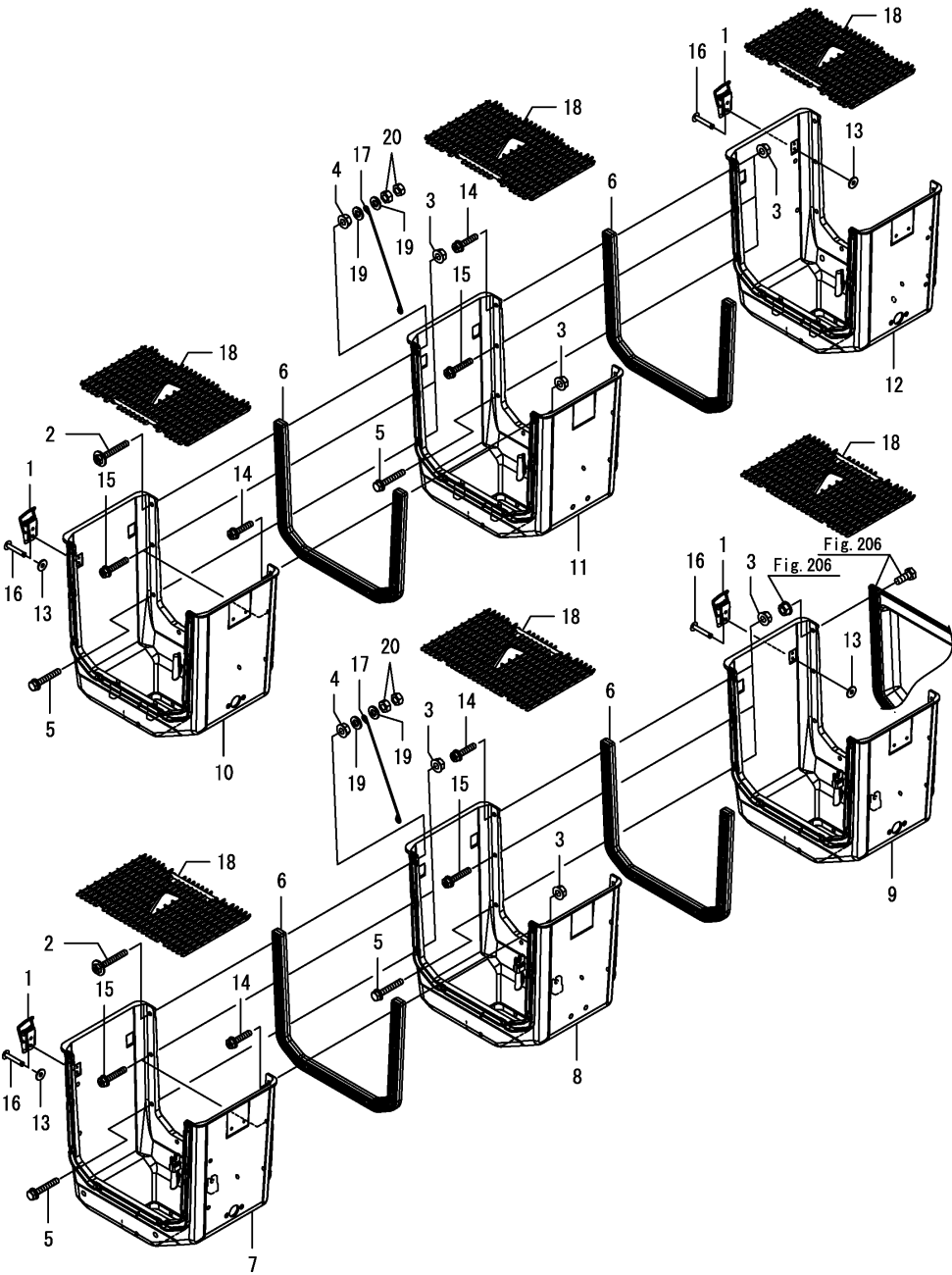
Fig.205. 호퍼(1)
