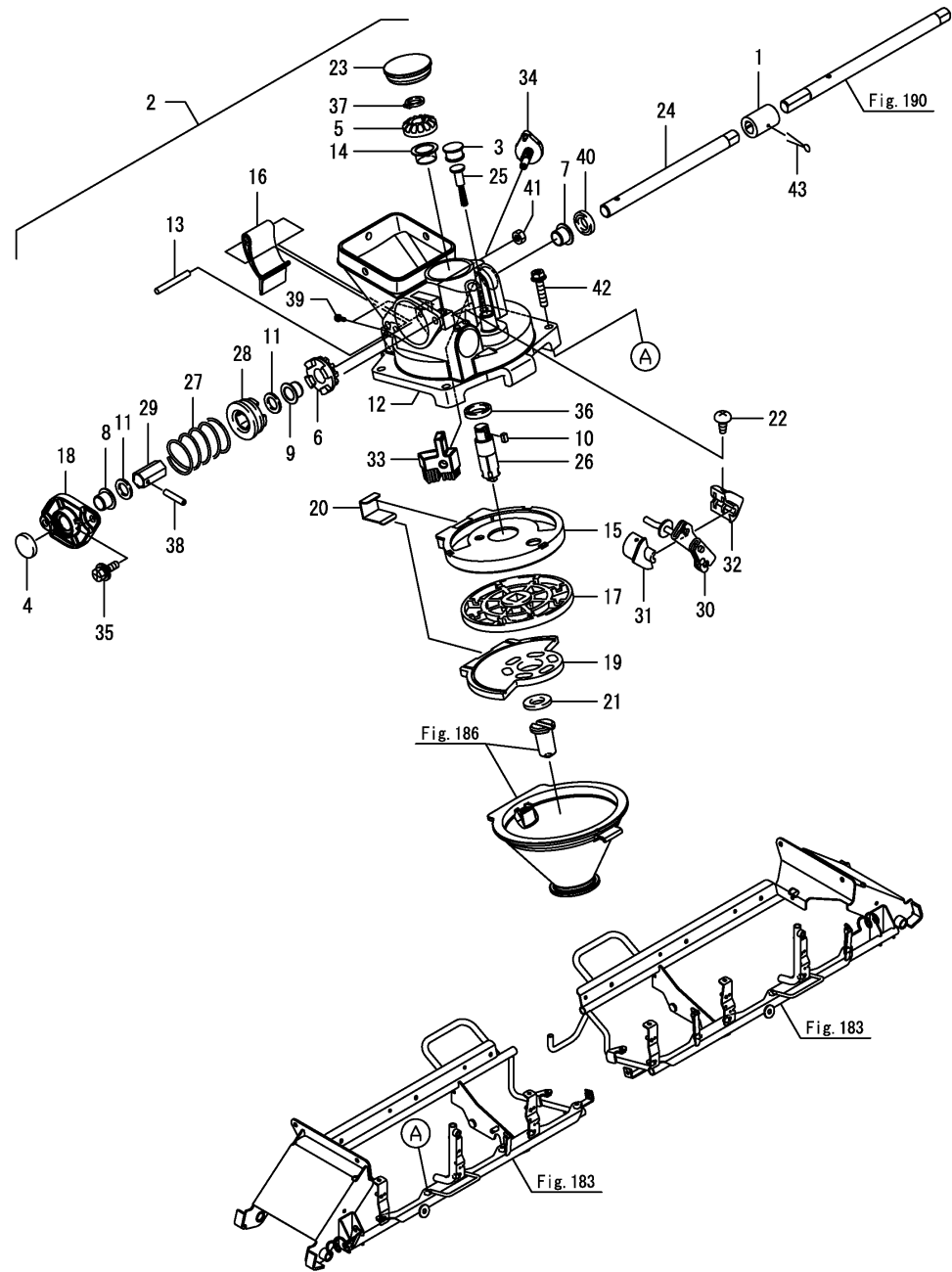
Fig.187. 롤구동(A)
