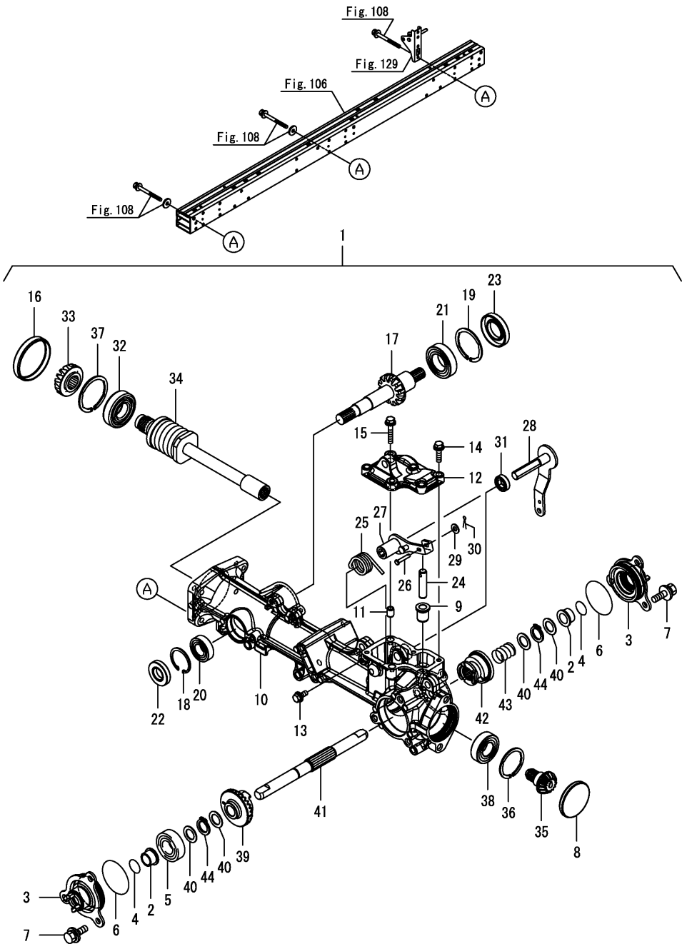
Fig.104. 식부베벨케이스
