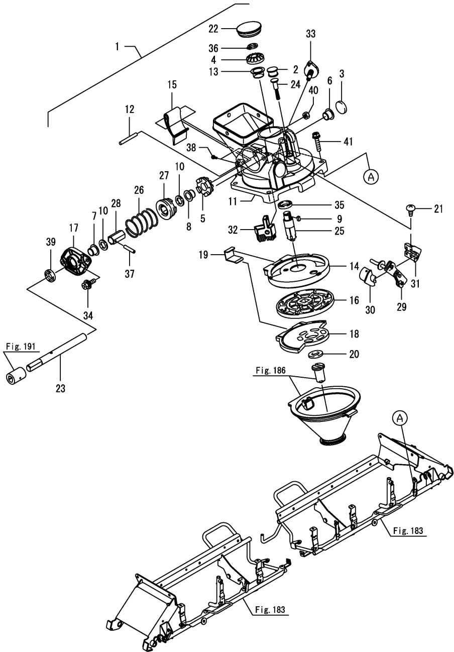
Fig.190. 롤구동(D)
