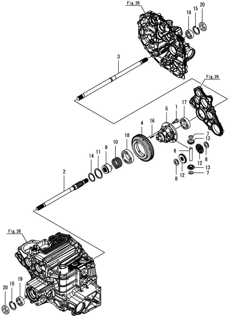
Fig.32. 전방디퍼런설
