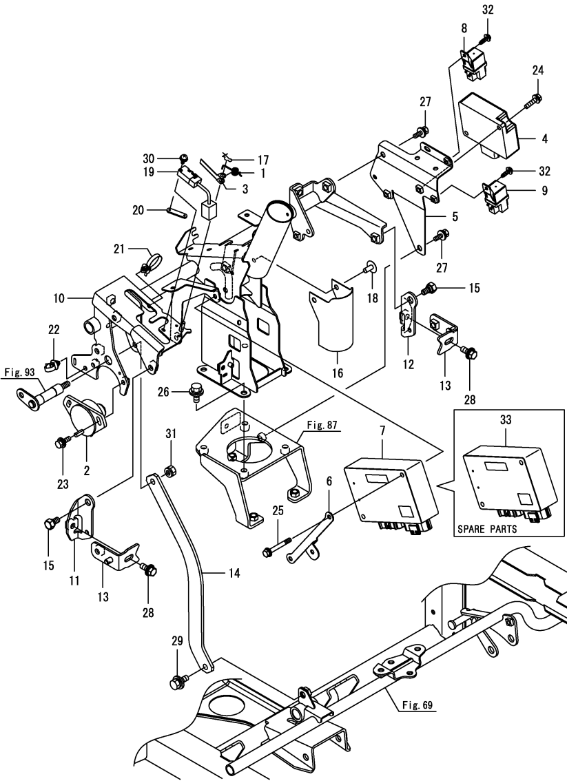
Fig.86. 스티어링칼럼
