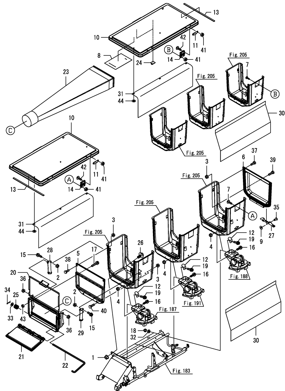
Fig.206. 호퍼(2)
