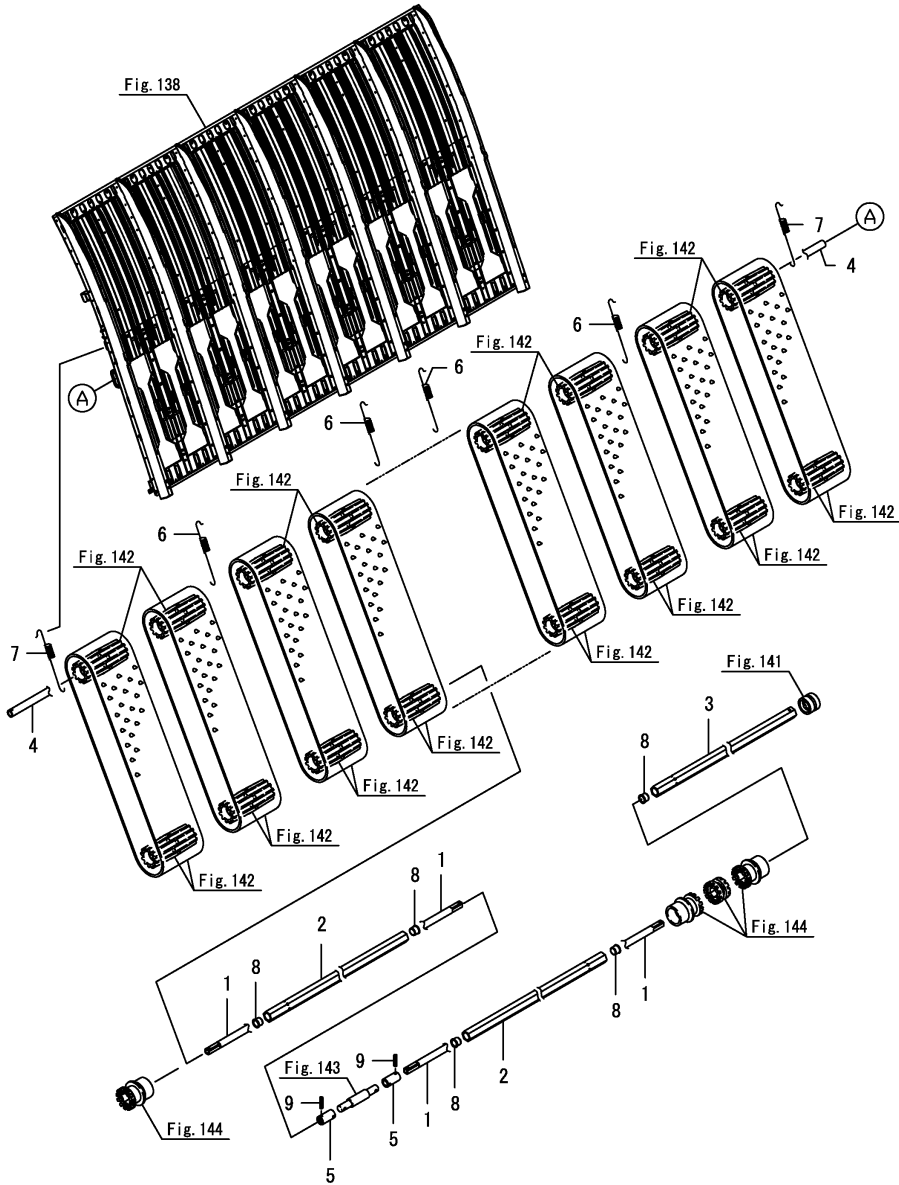
Fig.140. 종이송축
