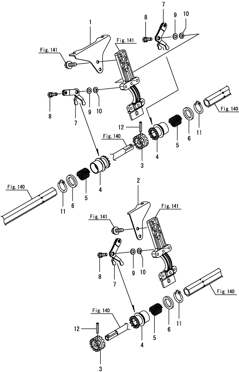
Fig.144. 종이송클러치
