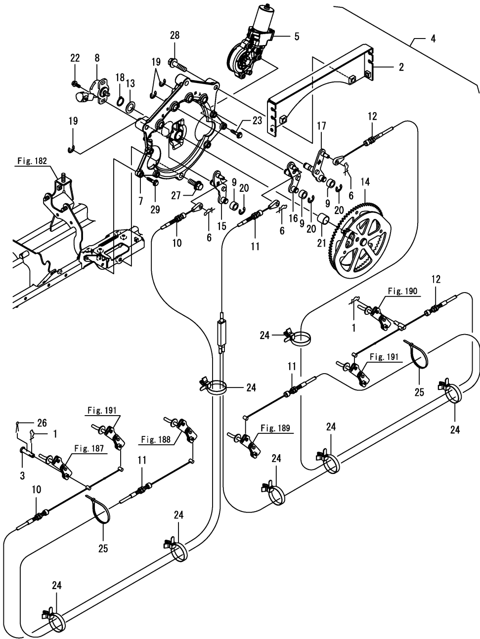
Fig.202. 유니트클러치와이어
