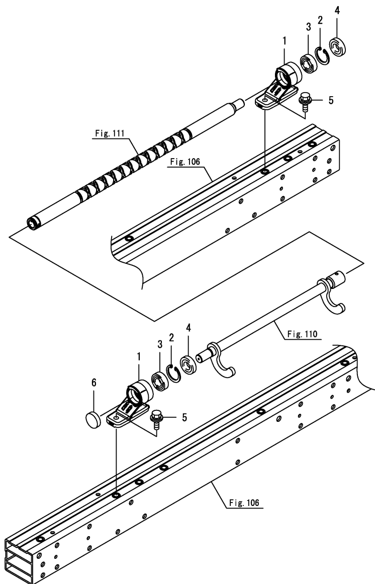
Fig.113. 베어링
