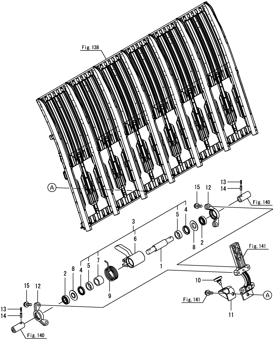
Fig.143. 종이송캠
