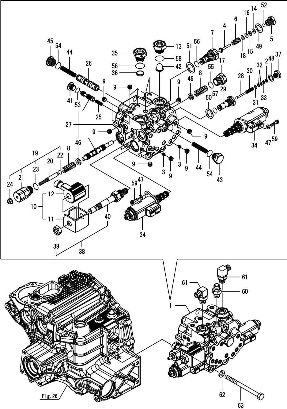
Fig.46. 컨트롤밸브
