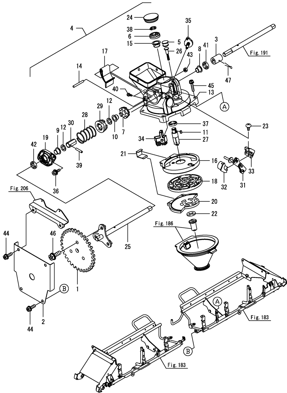
Fig.189. 롤구동(C)
