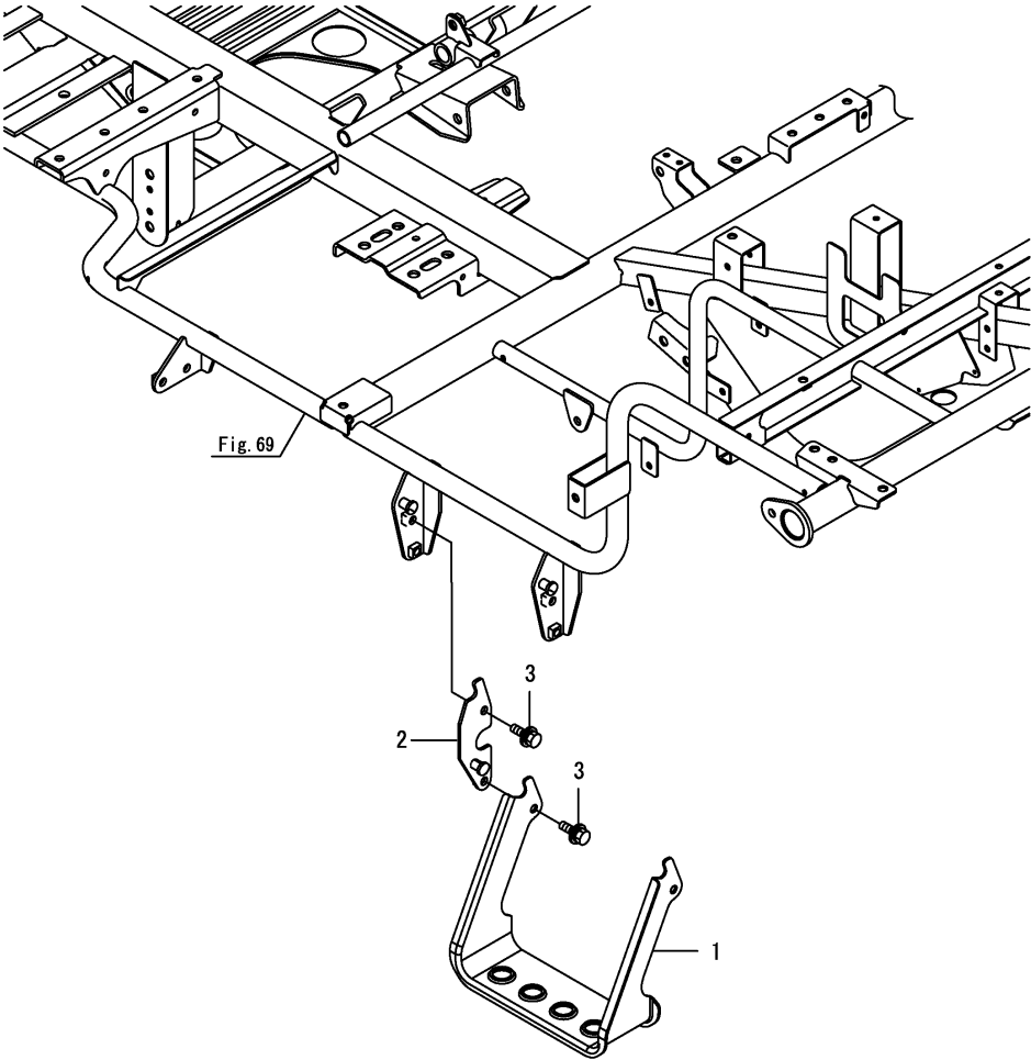
Fig.78. 보조발판
