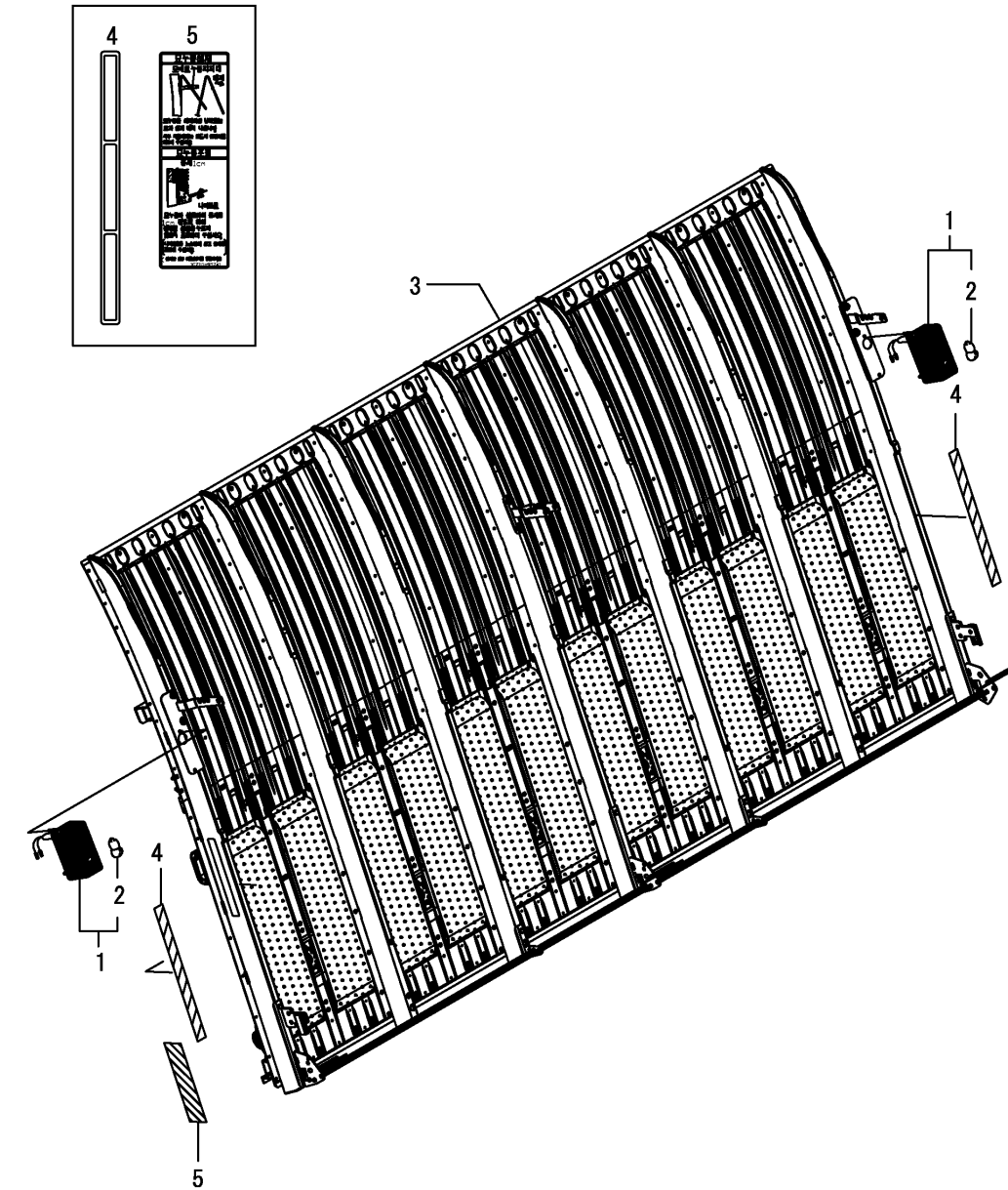
Fig.136. 요탑재대(조립)
