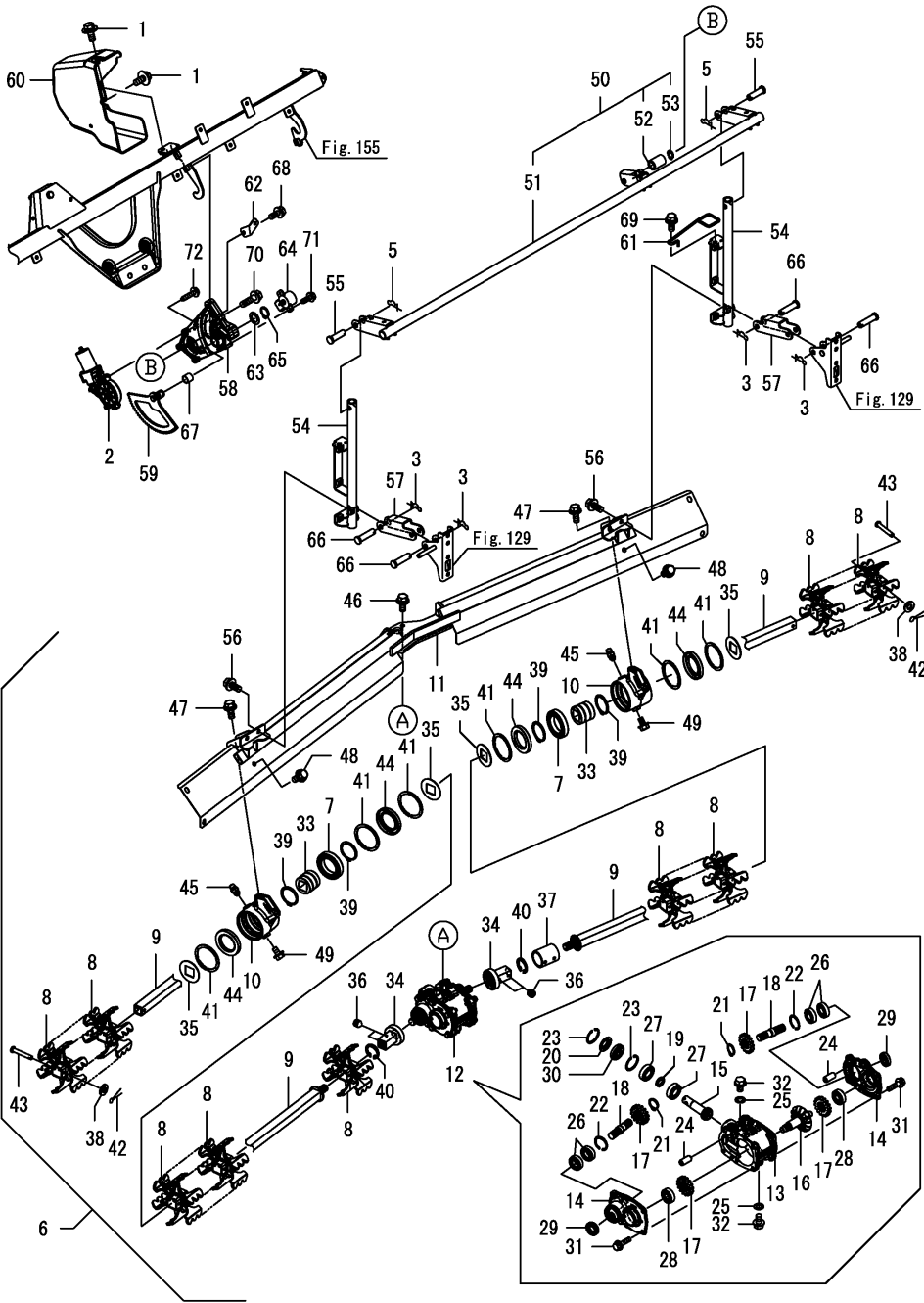
Fig.119. 로터
