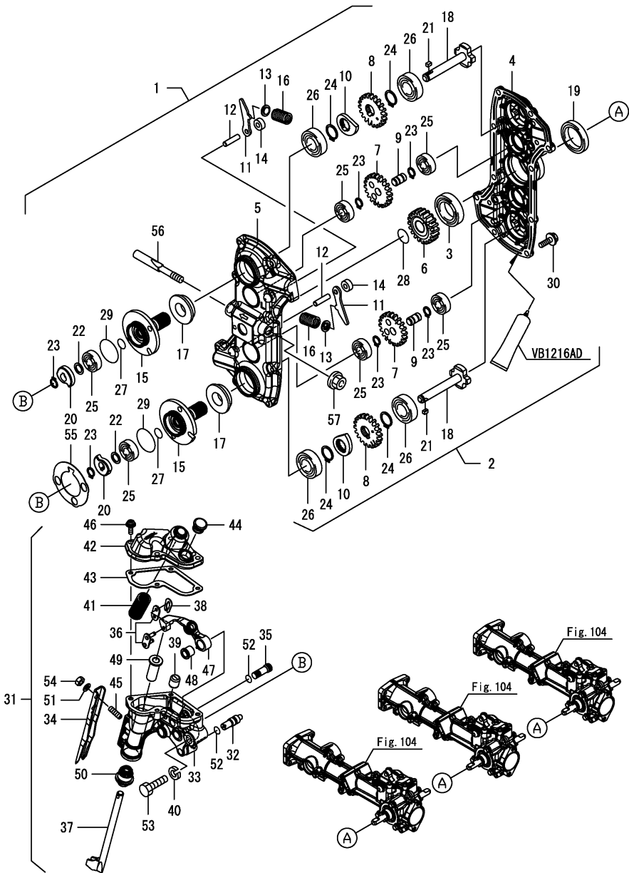
Fig.115. 식부암조합(좌)
