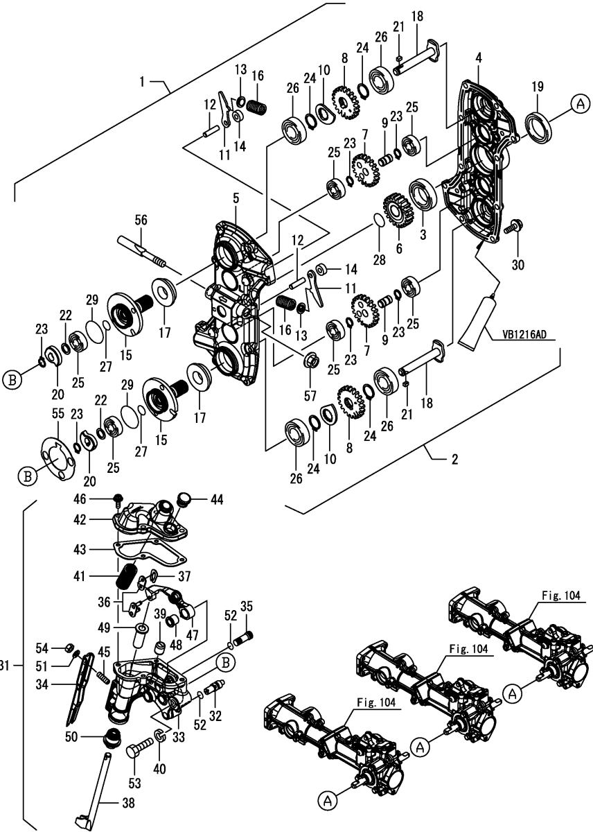
Fig.116. 식부 로터 암(좌측)(가득찬 묘)
