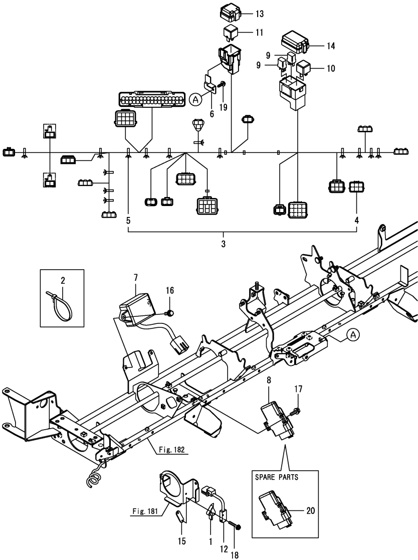
Fig.200. 전장품
