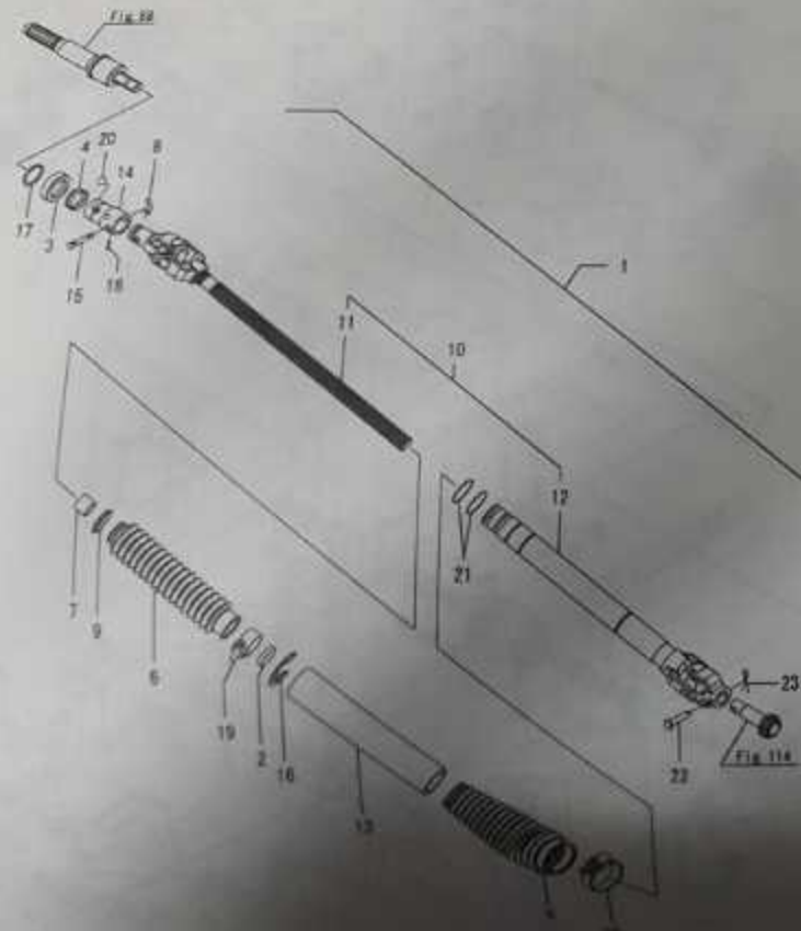
Fig.115. 청치로터구동축(Z사양)
