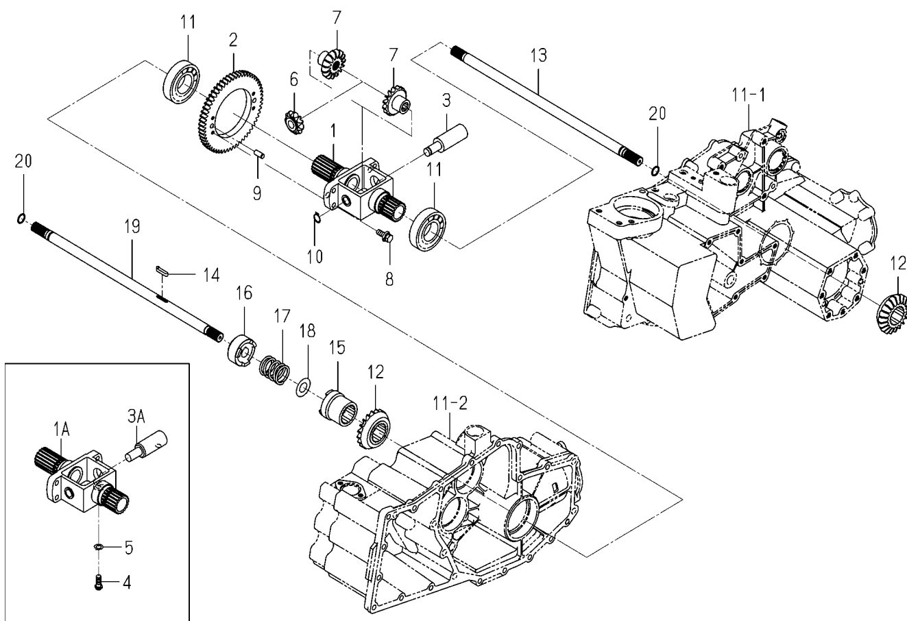
FIG. 16 SHAFT(DRIVE/FRONT)SYSTEM
