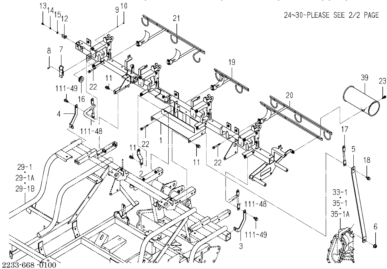
FIG.112 FRAME(FERTILIZER)SYSTEM(F TYPE)(1/2)
