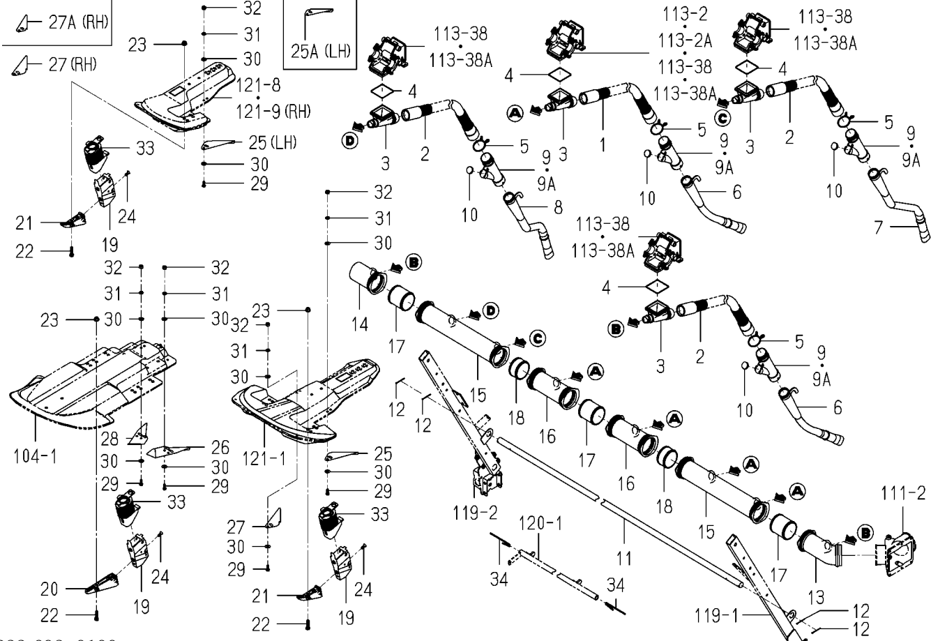
FIG.115 PIPING(FERTILIZER)SYSTEM(F TYPE)
