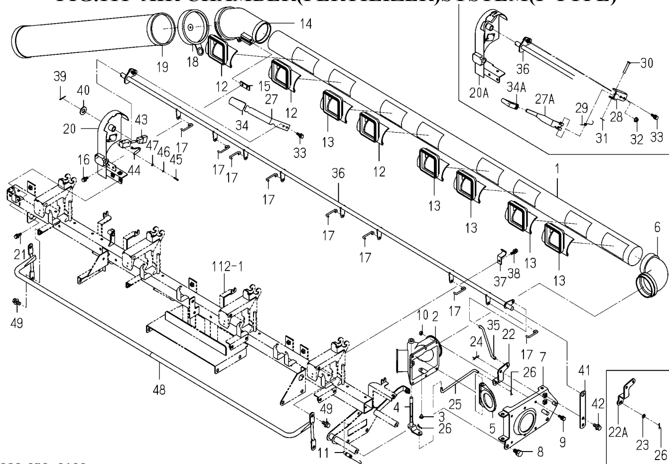
FIG.111 AIR CHAMBER(FERTILIZER)SYSTEM(F TYPE)
