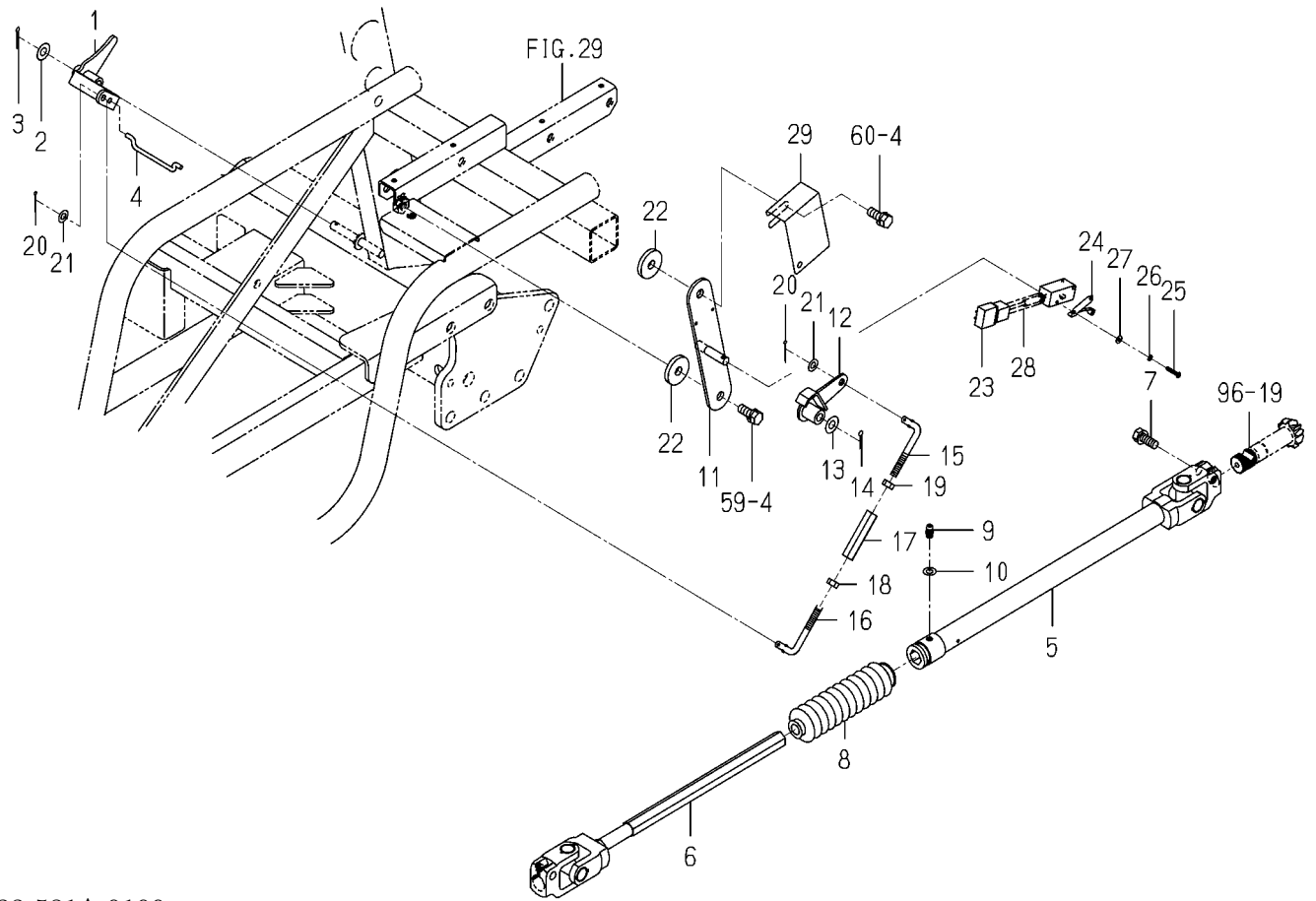
FIG. 92 DRIVE(ROTOR)SYSTEM(Z TYPE)
