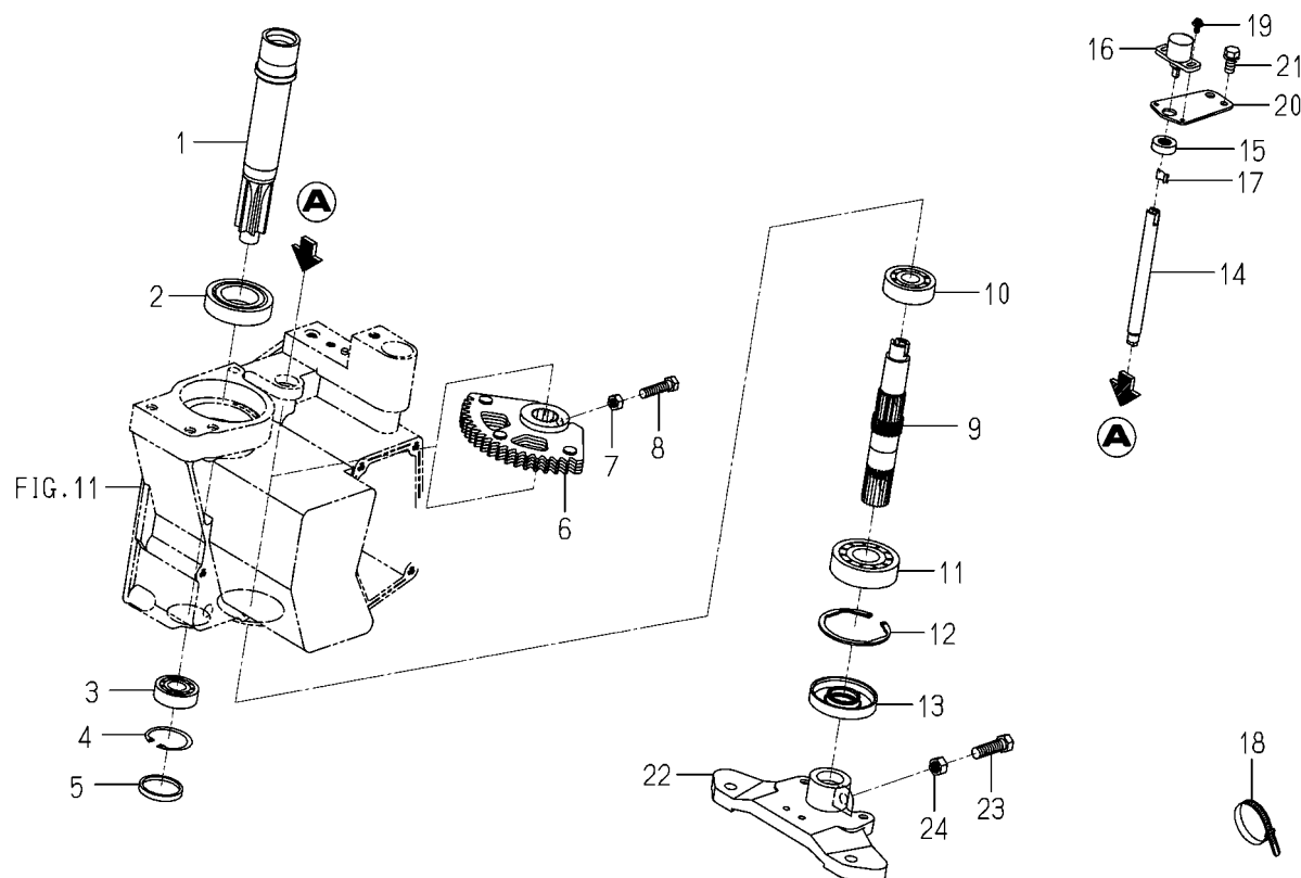
FIG. 23 SHAFT(STEERING)SYSTEM
