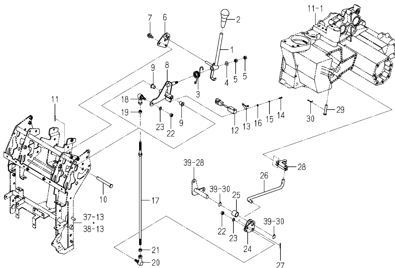
FIG. 7 LEVER(SUB)SYSTEM
