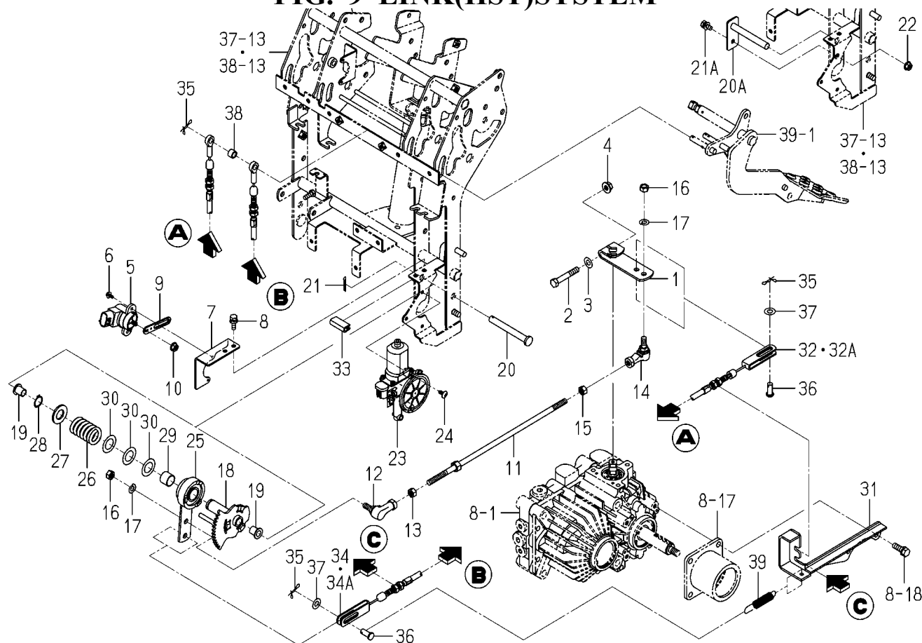
FIG. 9 LINK(HST)SYSTEM
