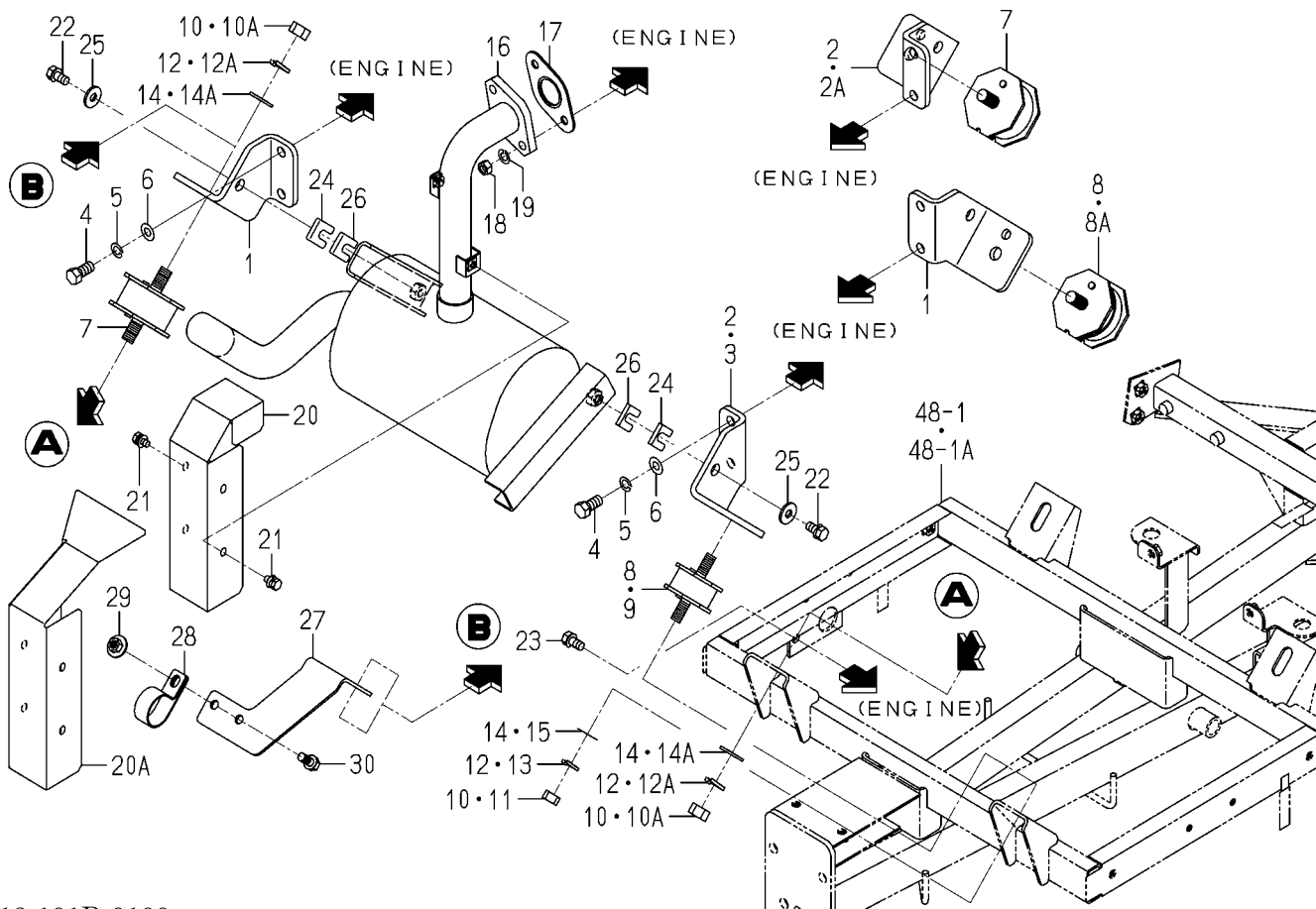
FIG. 3 BRACKET(ENGINE)SYSTEM(D TYPE)
