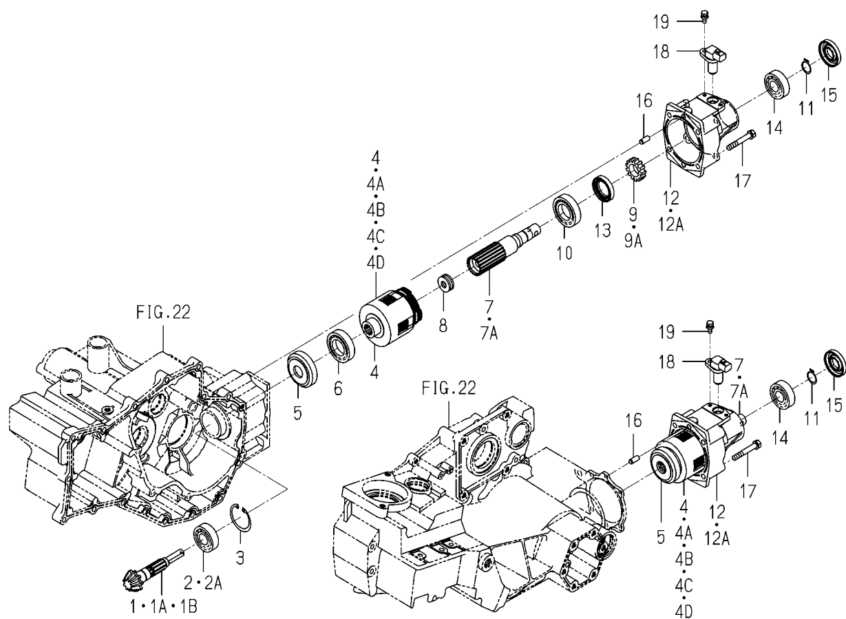
FIG. 28 SHAFT(OUTPUT)SYSTEM
