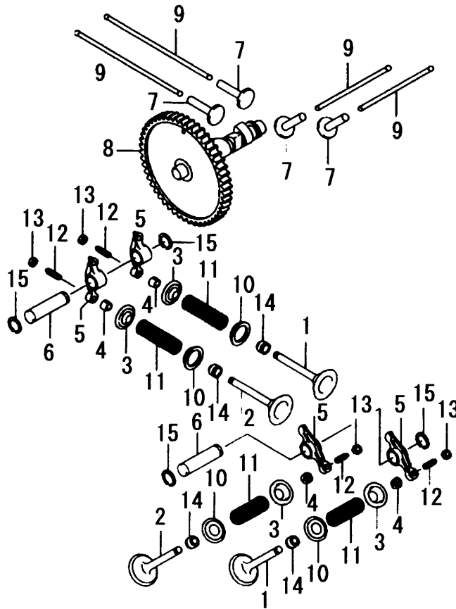
FIG. 3 VALVE/CAMSHAFT
