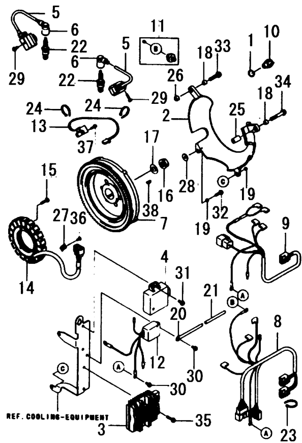
FIG. 6 ELECTRIC-EQUIPMENT
