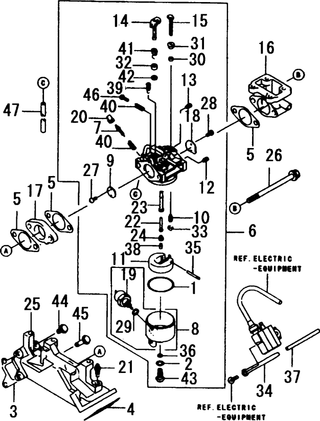
FIG. 8 CARBURETOR
