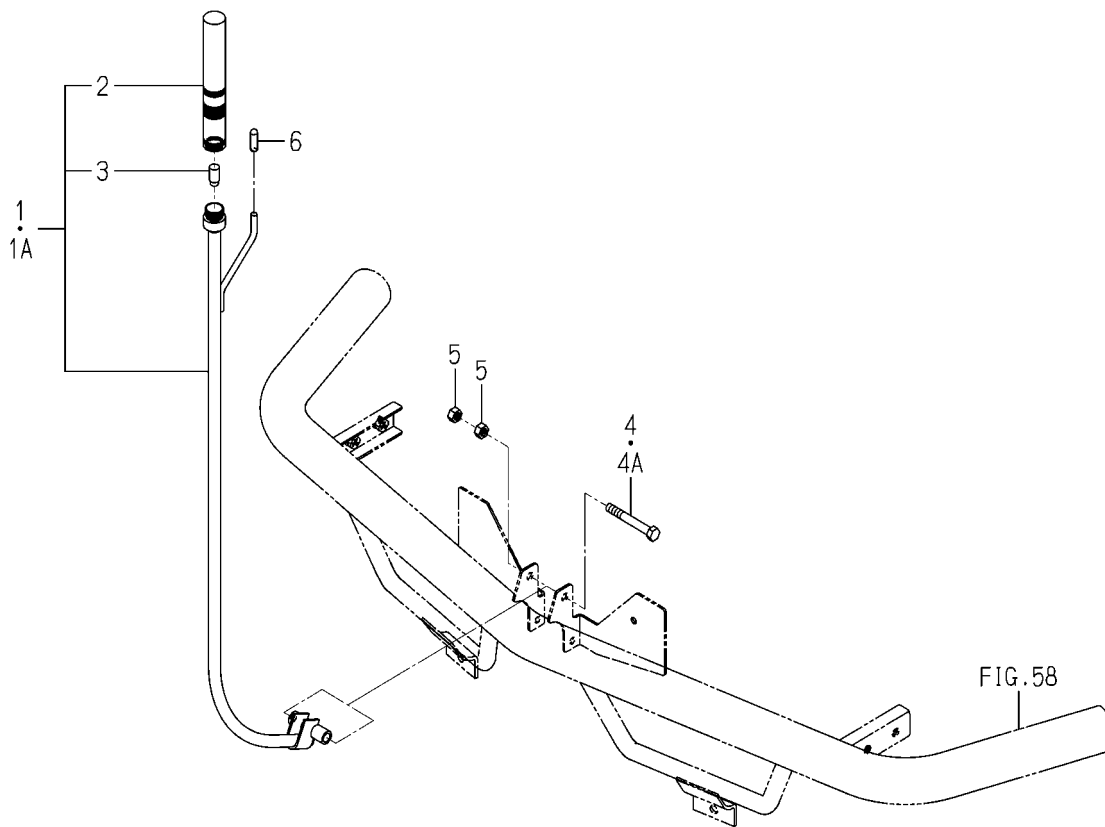
FIG. 92 MARKER(CENTER)SYSTEM
