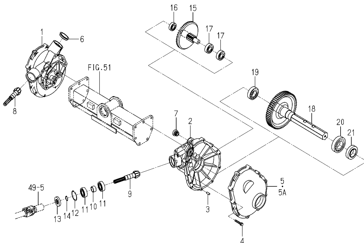
FIG. 54 CASE(REAR)SYSTEM
