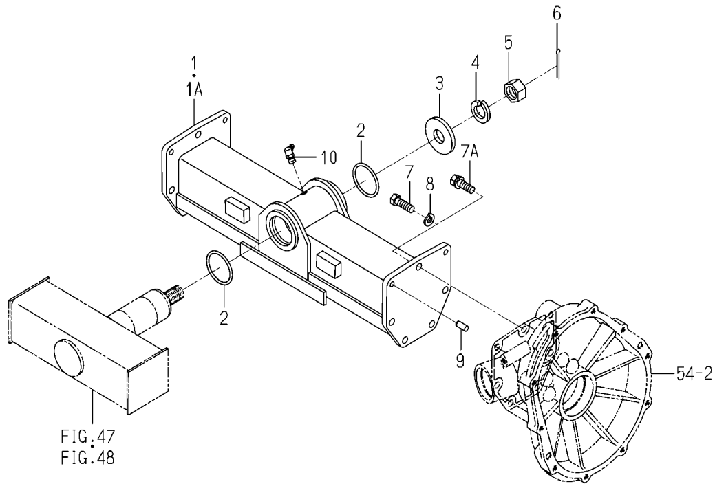
FIG. 51 FRAME(ROLLING)SYSTEM
