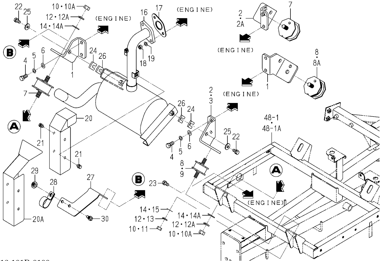
FIG. 3 BRACKET(ENGINE)SYSTEM(D TYPE)
