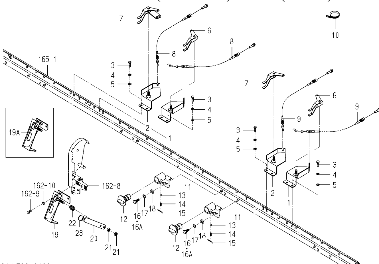
FIG.173 CLUTCH(FERTILIZE)SYSTEM(F TYPE)
