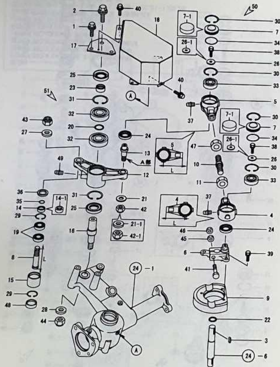
Fig.45. 예취날구동 R
