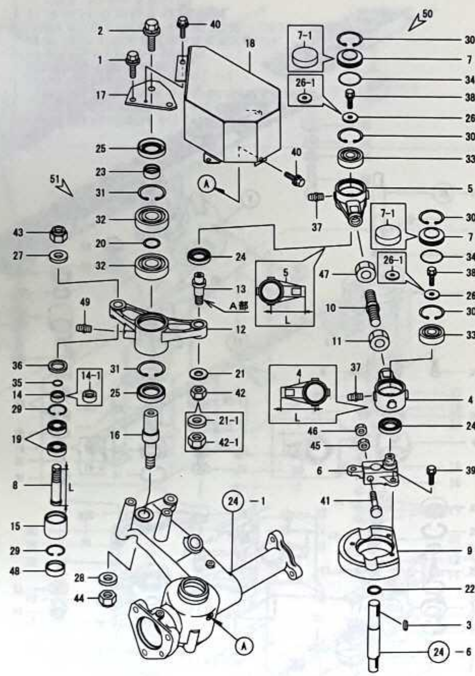
Fig.45. 예취날구동 R
