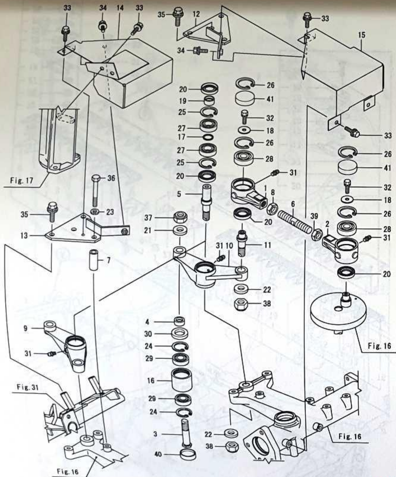
Fig.32. 수확 에지 드라이브
